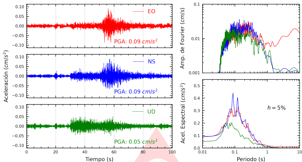
Figura A.1: Registros tiempo-historia, espectros de Fourier y de respuesta en las direcciones EO, NS y vertical de la estación SCCHI. Sismo de Trujillo, Trujillo - La Libertad del 2024-09-25, 10:28:38 (Hora local)
