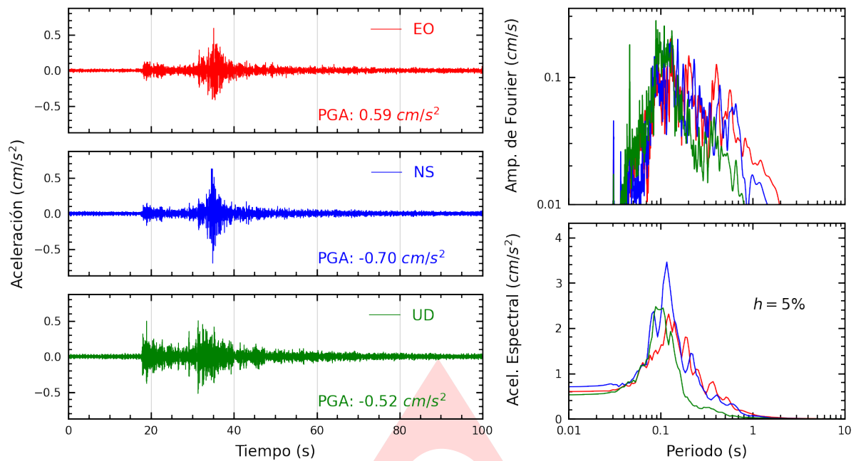
Figura A.1: Registros tiempo-historia, espectros de Fourier y de respuesta en las direcciones EO, NS y vertical de la estación UNIA. Sismo de Curimana, Padre Abad - Ucayali del 2024-10-22, 10:03:59 (Hora local)
