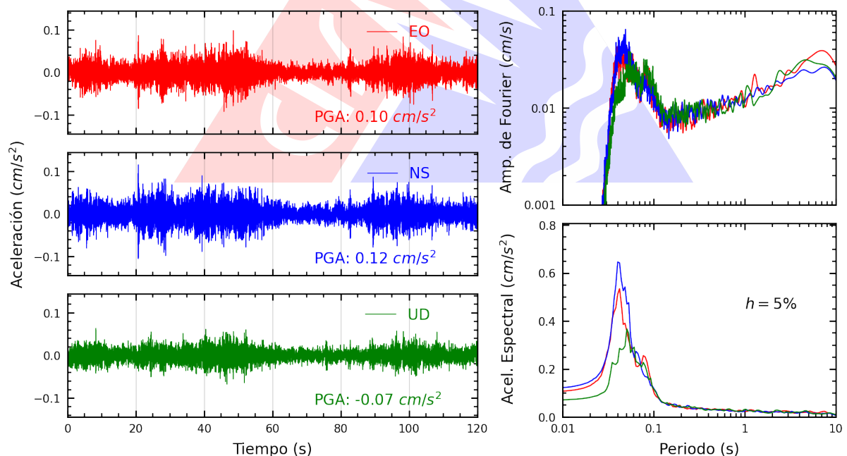
Figura A.2: Registros tiempo-historia, espectros de Fourier y de respuesta en las direcciones EO, NS y vertical de la estación COMAS. Sismo de Curimana, Padre Abad - Ucayali del 2024-10-22, 10:03:59 (Hora local)
