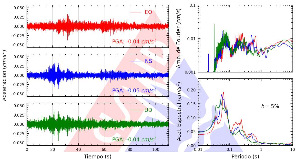
Figura A.3: Registros tiempo-historia, espectros de Fourier y de respuesta en las direcciones EO, NS y vertical de la estación CARAL. Sismo de Curimana, Padre Abad - Ucayali del 2024-10-22, 10:03:59 (Hora local)
