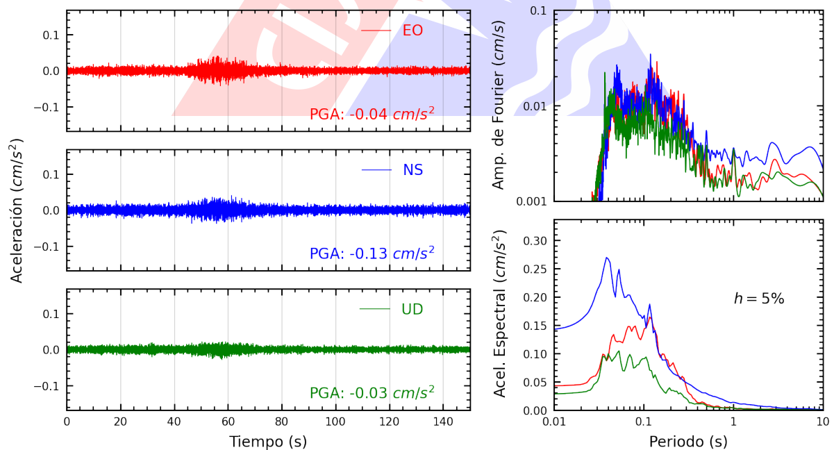
Figura A.10: Registros tiempo-historia, espectros de Fourier y de respuesta en las direcciones EO, NS y vertical de la estación ATARJ. Sismo de Palpa, Palpa - Ica del 2024-10-27, 04:36:54 (Hora local)
