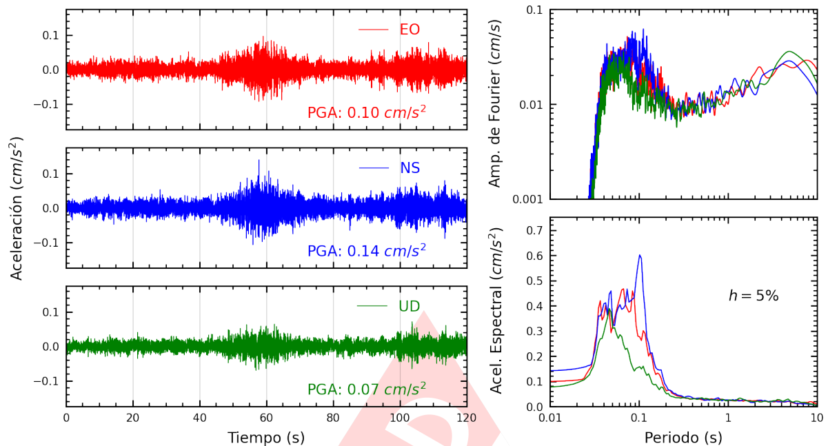
Figura A.9: Registros tiempo-historia, espectros de Fourier y de respuesta en las direcciones EO, NS y vertical de la estación JOSEO. Sismo de Palpa, Palpa - Ica del 2024-10-27, 04:36:54 (Hora local)
