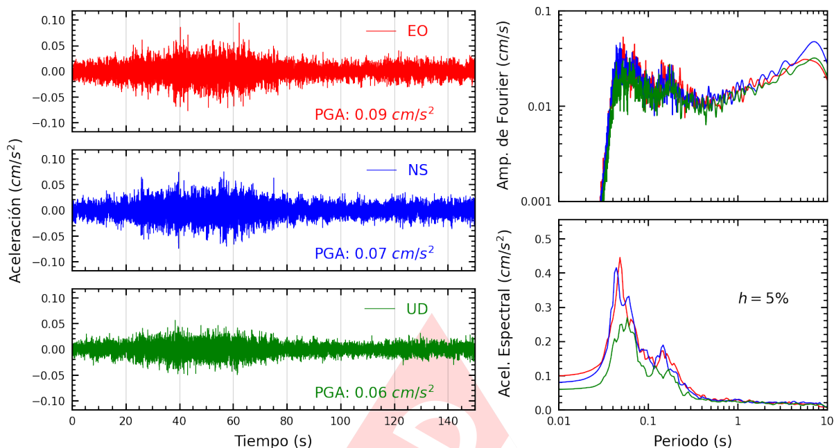
Figura A.15: Registros tiempo-historia, espectros de Fourier y de respuesta en las direcciones EO, NS y vertical de la estación FICPE. Sismo de Palpa, Palpa - Ica del 2024-10-27, 04:36:54 (Hora local)
