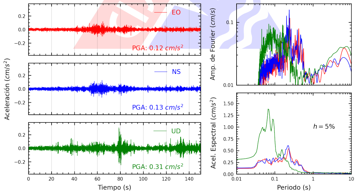
Figura A.4: Registros tiempo-historia, espectros de Fourier y de respuesta en las direcciones EO, NS y vertical de la estación MDPP. Sismo de Palpa, Palpa - Ica del 2024-10-27, 04:36:54 (Hora local)
