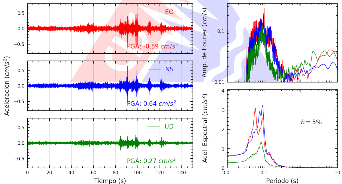
Figura A.2: Registros tiempo-historia, espectros de Fourier y de respuesta en las direcciones EO, NS y vertical de la estación USILM. Sismo de Palpa, Palpa - Ica del 2024-10-27, 04:36:54 (Hora local)
