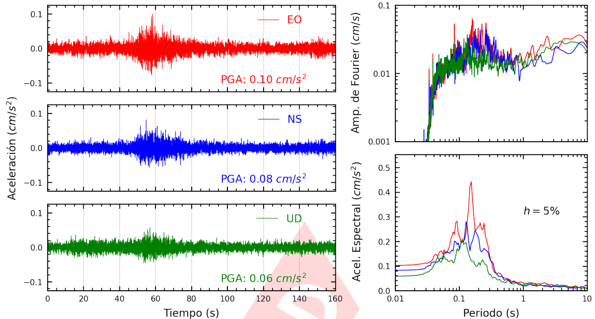
Figura A.13: Registros tiempo-historia, espectros de Fourier y de respuesta en las direcciones EO, NS y vertical de la estación USILP. Sismo de Palpa, Palpa - Ica del 2024-10-27, 04:36:54 (Hora local)
