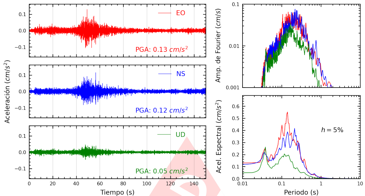
Figura A.11: Registros tiempo-historia, espectros de Fourier y de respuesta en las direcciones EO, NS y vertical de la estación BRIS2. Sismo de Palpa, Palpa - Ica del 2024-10-27, 04:36:54 (Hora local)
