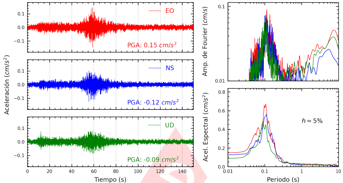
Figura A.7: Registros tiempo-historia, espectros de Fourier y de respuesta en las direcciones EO, NS y vertical de la estación AMORE. Sismo de Palpa, Palpa - Ica del 2024-10-27, 04:36:54 (Hora local)
