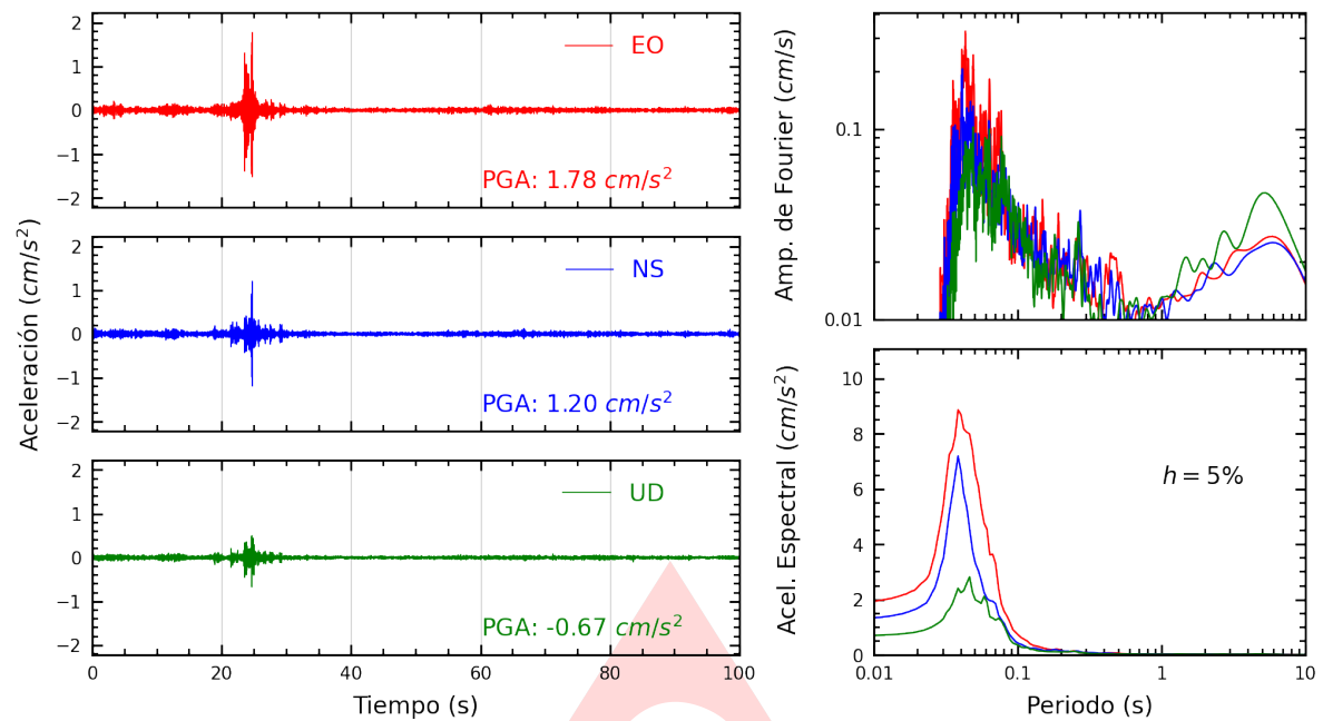
Figura A.1: Registros tiempo-historia, espectros de Fourier y de respuesta en las direcciones EO, NS y vertical de la estación OLIVO. Sismo de Palpa, Palpa - Ica del 2024-10-27, 04:36:54 (Hora local)
