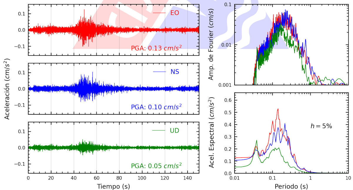
Figura A.12: Registros tiempo-historia, espectros de Fourier y de respuesta en las direcciones EO, NS y vertical de la estación BRISA. Sismo de Palpa, Palpa - Ica del 2024-10-27, 04:36:54 (Hora local)
