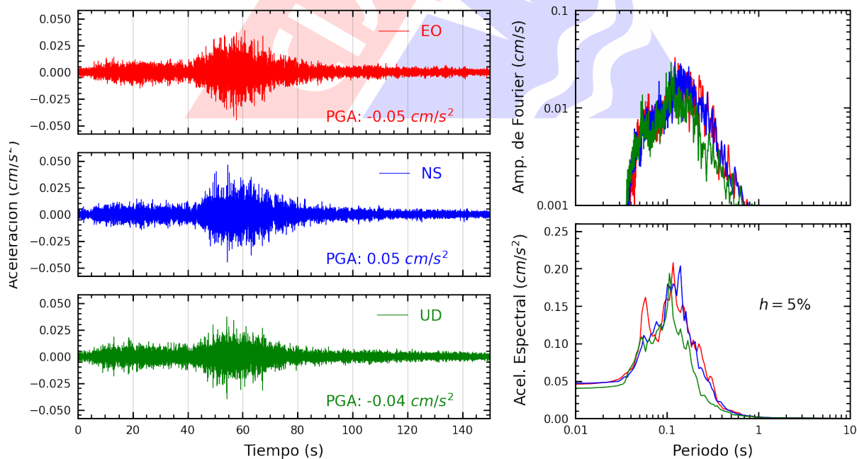
Figura A.20: Registros tiempo-historia, espectros de Fourier y de respuesta en las direcciones EO, NS y vertical de la estación JALV2. Sismo de Palpa, Palpa - Ica del 2024-10-27, 04:36:54 (Hora local)
