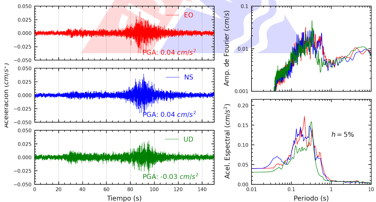
Figura A.22: Registros tiempo-historia, espectros de Fourier y de respuesta en las direcciones EO, NS y vertical de la estación CARAL. Sismo de Palpa, Palpa - Ica del 2024-10-27, 04:36:54 (Hora local)
