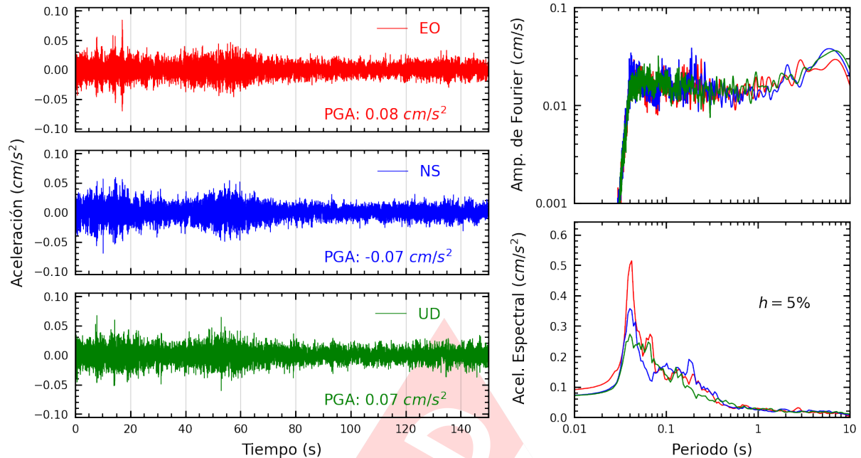
Figura A.17: Registros tiempo-historia, espectros de Fourier y de respuesta en las direcciones EO, NS y vertical de la estación IMCA. Sismo de Palpa, Palpa - Ica del 2024-10-27, 04:36:54 (Hora local)
