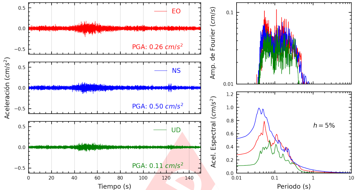
Figura A.3: Registros tiempo-historia, espectros de Fourier y de respuesta en las direcciones EO, NS y vertical de la estación UNTEL. Sismo de Palpa, Palpa - Ica del 2024-10-27, 04:36:54 (Hora local)
