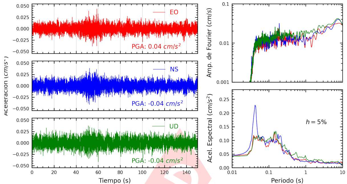
Figura A.21: Registros tiempo-historia, espectros de Fourier y de respuesta en las direcciones EO, NS y vertical de la estación UNFV. Sismo de Palpa, Palpa - Ica del 2024-10-27, 04:36:54 (Hora local)
