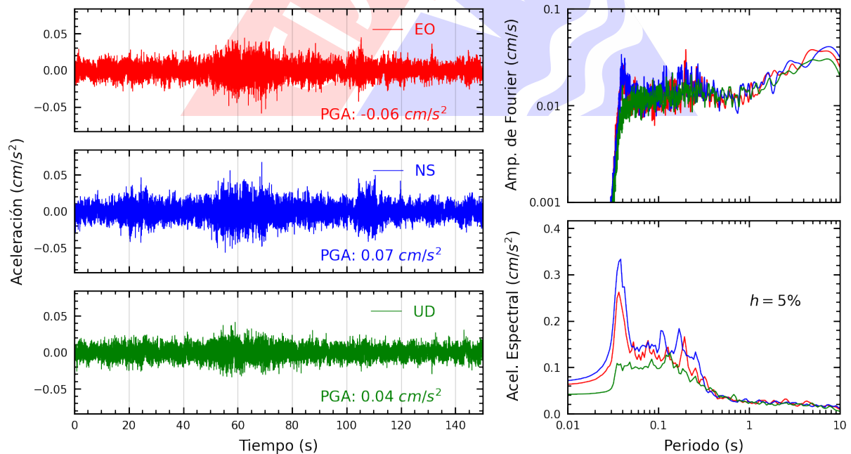
Figura A.18: Registros tiempo-historia, espectros de Fourier y de respuesta en las direcciones EO, NS y vertical de la estación COMAS. Sismo de Palpa, Palpa - Ica del 2024-10-27, 04:36:54 (Hora local)
