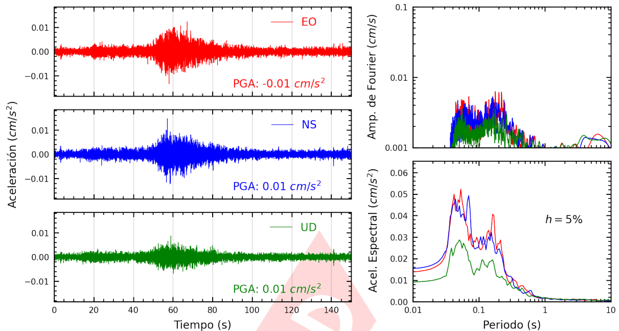
Figura A.23: Registros tiempo-historia, espectros de Fourier y de respuesta en las direcciones EO, NS y vertical de la estación UNSA2. Sismo de Palpa, Palpa - Ica del 2024-10-27, 04:36:54 (Hora local)
