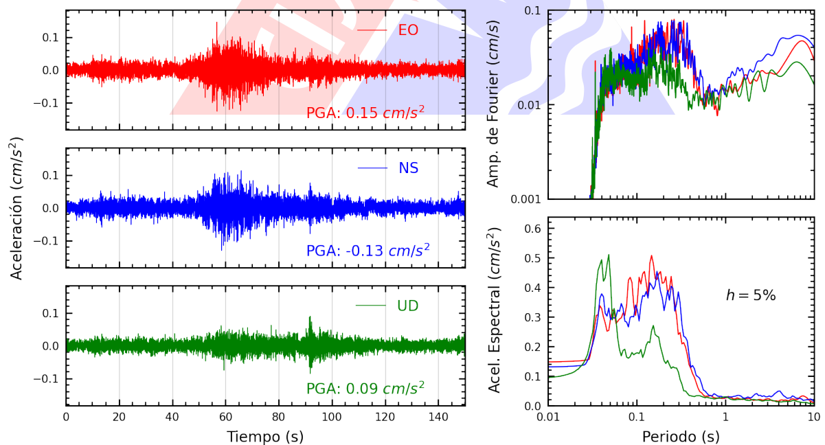
Figura A.8: Registros tiempo-historia, espectros de Fourier y de respuesta en las direcciones EO, NS y vertical de la estación DEFEN. Sismo de Palpa, Palpa - Ica del 2024-10-27, 04:36:54 (Hora local)
