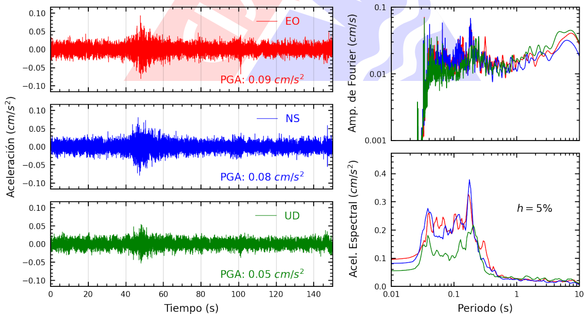
Figura A.16: Registros tiempo-historia, espectros de Fourier y de respuesta en las direcciones EO, NS y vertical de la estación UPCVI. Sismo de Palpa, Palpa - Ica del 2024-10-27, 04:36:54 (Hora local)
