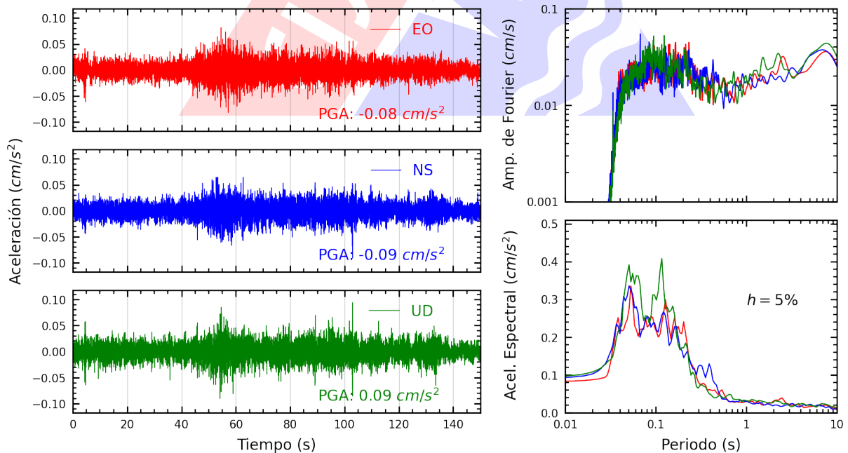
Figura A.14: Registros tiempo-historia, espectros de Fourier y de respuesta en las direcciones EO, NS y vertical de la estación UCVAT. Sismo de Palpa, Palpa - Ica del 2024-10-27, 04:36:54 (Hora local)
