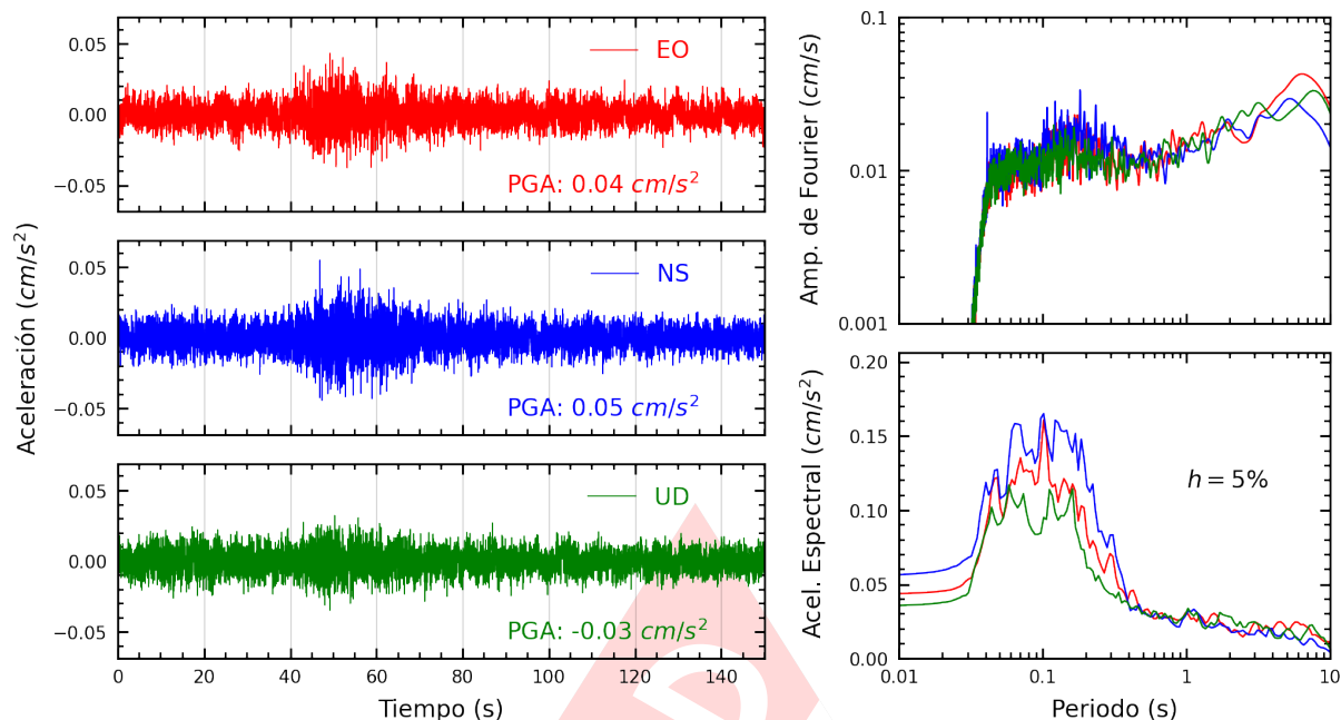
Figura A.19: Registros tiempo-historia, espectros de Fourier y de respuesta en las direcciones EO, NS y vertical de la estación SERVI. Sismo de Palpa, Palpa - Ica del 2024-10-27, 04:36:54 (Hora local)
