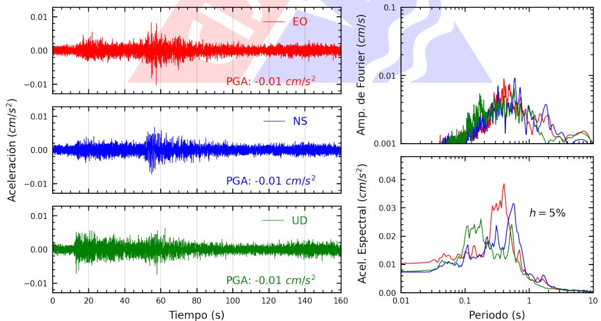
Figura A.24: Registros tiempo-historia, espectros de Fourier y de respuesta en las direcciones EO, NS y vertical de la estación UNCP. Sismo de Palpa, Palpa - Ica del 2024-10-27, 04:36:54 (Hora local)
