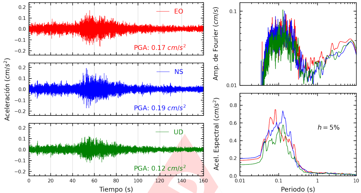
Figura A.5: Registros tiempo-historia, espectros de Fourier y de respuesta en las direcciones EO, NS y vertical de la estación PHERM. Sismo de Palpa, Palpa - Ica del 2024-10-27, 04:36:54 (Hora local)
