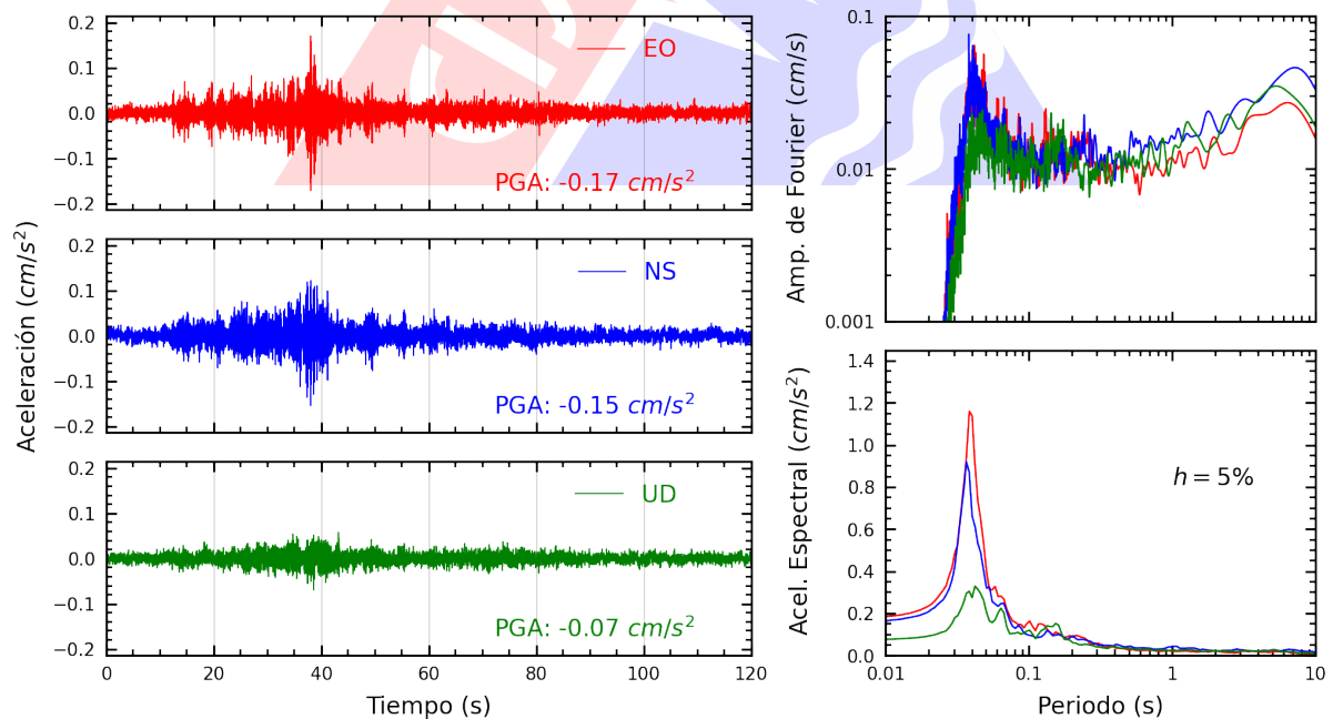
Figura A.6: Registros tiempo-historia, espectros de Fourier y de respuesta en las direcciones EO, NS y vertical de la estación CEPRE. Sismo de Palpa, Palpa - Ica del 2024-10-27, 04:36:54 (Hora local)
