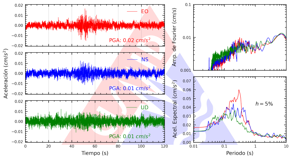
Figura A.3: Registros tiempo-historia, espectros de Fourier y de respuesta en las direcciones EO, NS y vertical de la estación UNJ. Sismo de Sullana, Sullana - Piura del 2024-11-01, 23:53:56 (Hora local)
