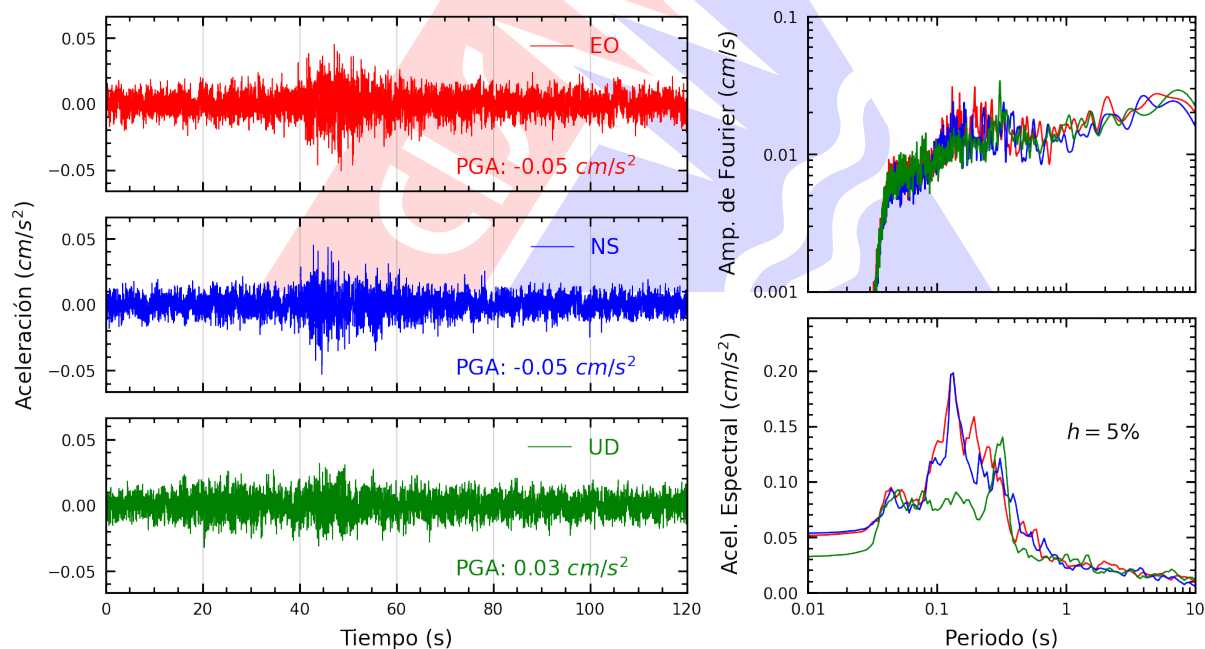
Figura A.2: Registros tiempo-historia, espectros de Fourier y de respuesta en las direcciones EO, NS y vertical de la estación UCVCH. Sismo de Sullana, Sullana - Piura del 2024-11-01, 23:53:56 (Hora local)
