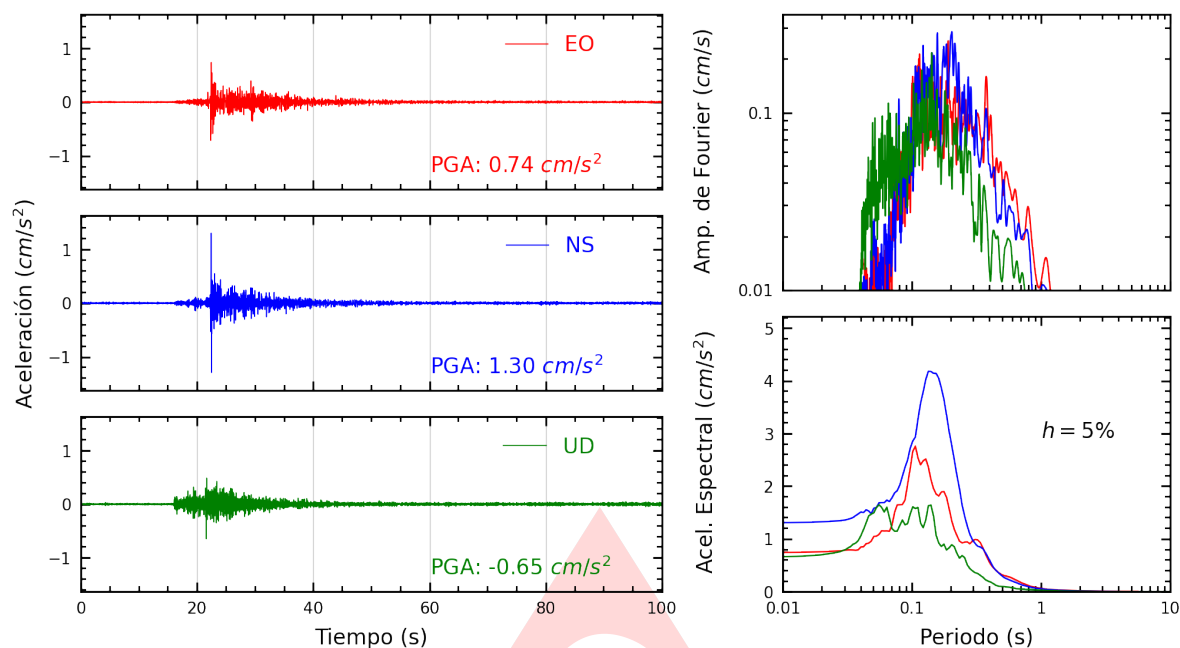
Figura A.1: Registros tiempo-historia, espectros de Fourier y de respuesta en las direcciones EO, NS y vertical de la estación UNP. Sismo de Sullana, Sullana - Piura del 2024-11-01, 23:53:56 (Hora local)
