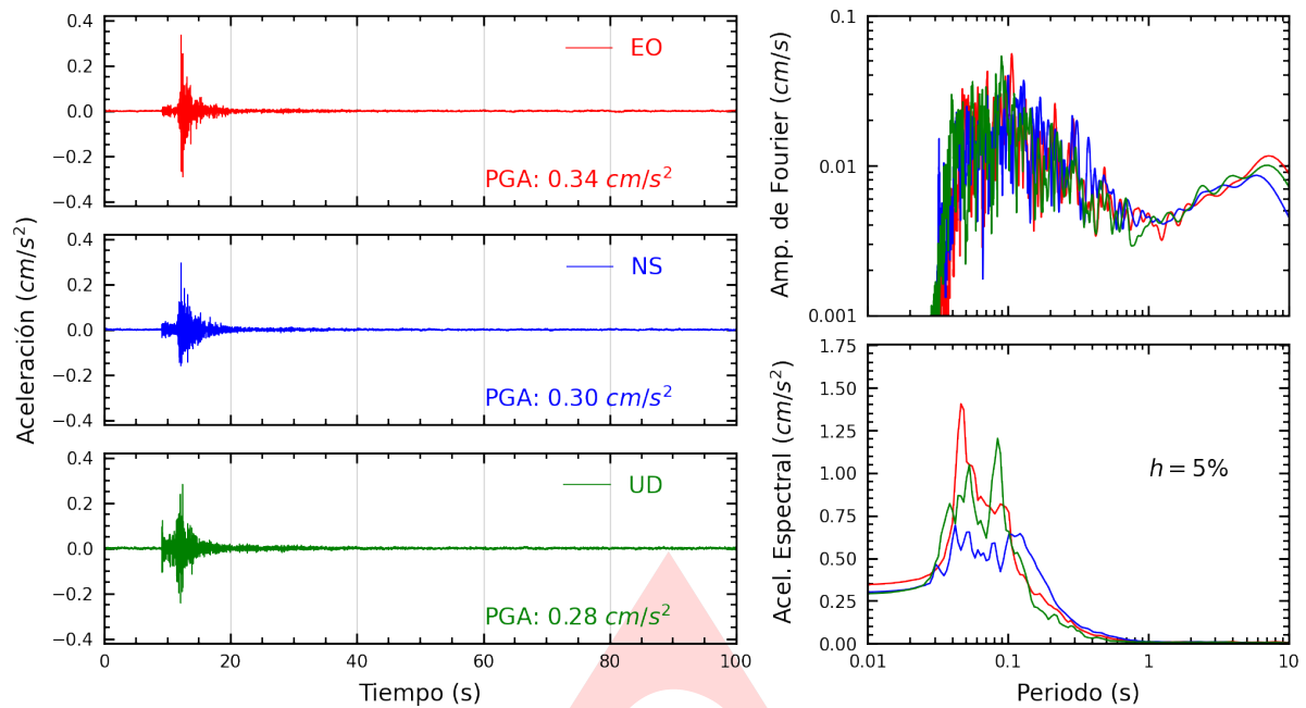
Figura A.1: Registros tiempo-historia, espectros de Fourier y de respuesta en las direcciones EO, NS y vertical de la estación UNJ. Sismo de Jaen, Jaen - Cajamarca del 2024-11-03, 01:07:15 (Hora local)
