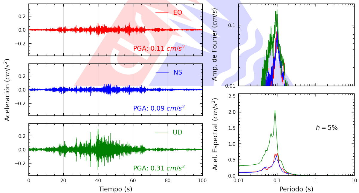
Figura A.2: Registros tiempo-historia, espectros de Fourier y de respuesta en las direcciones EO, NS y vertical de la estación UNP. Sismo de Jaen, Jaen - Cajamarca del 2024-11-03, 01:07:15 (Hora local)
