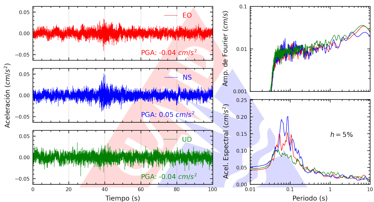
Figura A.3: Registros tiempo-historia, espectros de Fourier y de respuesta en las direcciones EO, NS y vertical de la estación UNTRM. Sismo de Jaen, Jaen - Cajamarca del 2024-11-03, 01:07:15 (Hora local)
