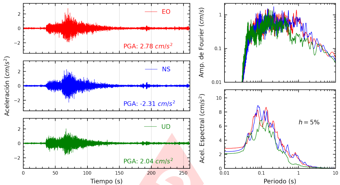
Figura A.21: Registros tiempo-historia, espectros de Fourier y de respuesta en las direcciones EO, NS y vertical de la estación UPCSM. Sismo de Lunahuana, Cañete - Lima del 2024-11-05, 14:39:42 (Hora local)
