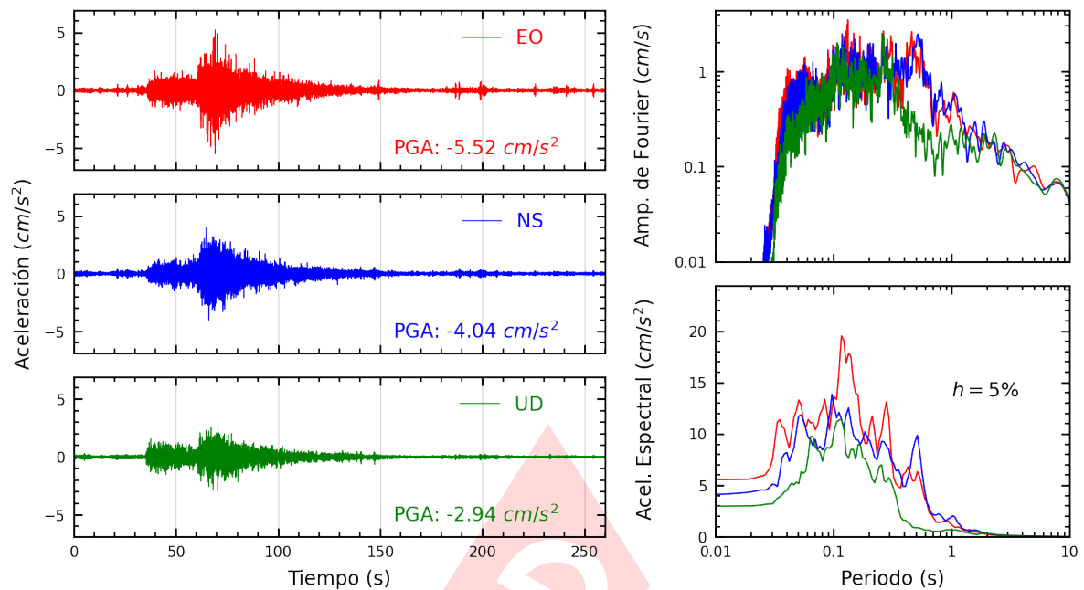
Figura A.11: Registros tiempo-historia, espectros de Fourier y de respuesta en las direcciones EO, NS y vertical de la estación OLIVO. Sismo de Lunahuana, Cañete - Lima del 2024-11-05, 14:39:42 (Hora local)
