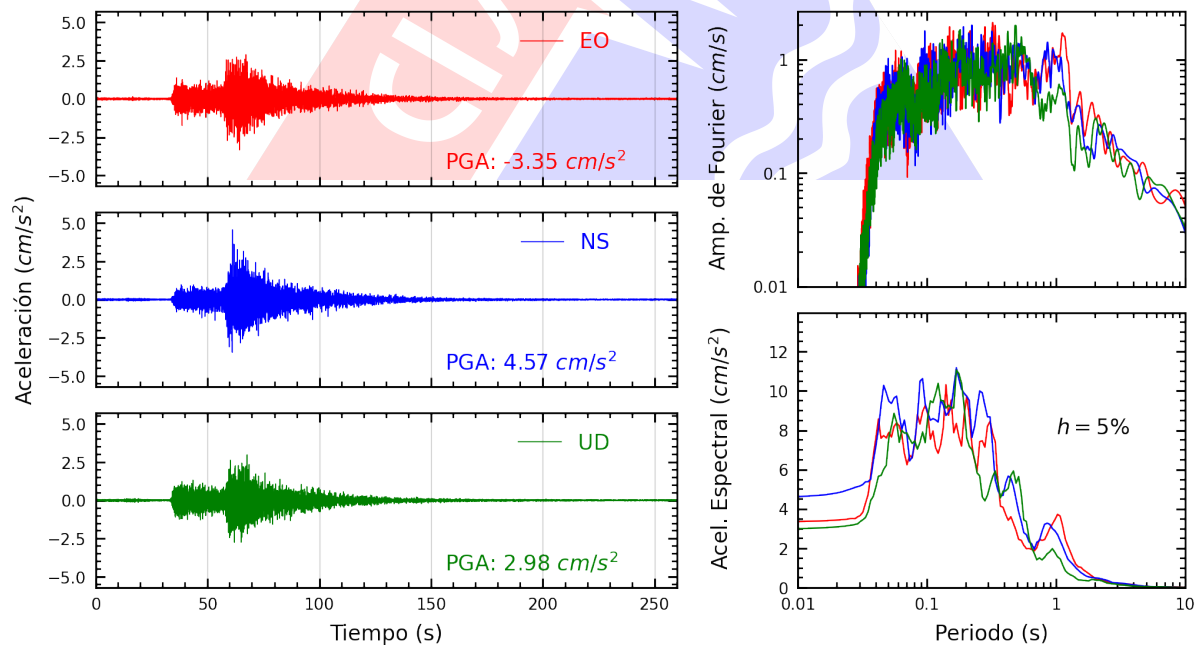
Figura A.12: Registros tiempo-historia, espectros de Fourier y de respuesta en las direcciones EO, NS y vertical de la estación IMCA. Sismo de Lunahuana, Cañete - Lima del 2024-11-05, 14:39:42 (Hora local)
