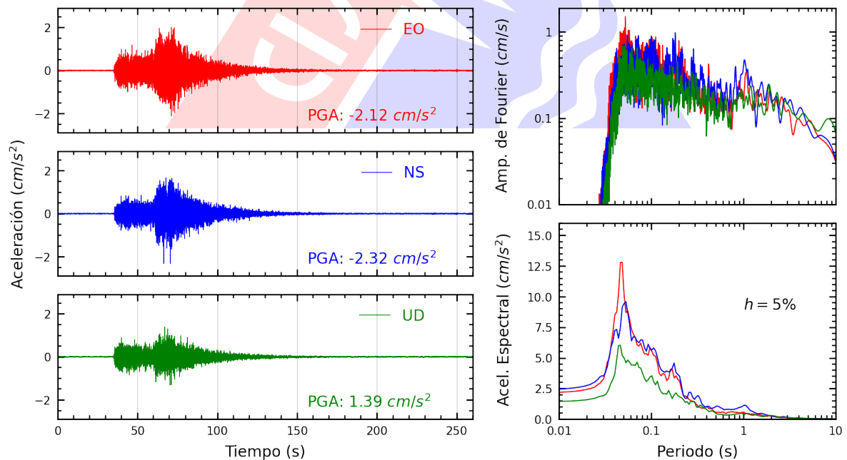
Figura A.26: Registros tiempo-historia, espectros de Fourier y de respuesta en las direcciones EO, NS y vertical de la estación UCSS. Sismo de Lunahuana, Cañete - Lima del 2024-11-05, 14:39:42 (Hora local)
