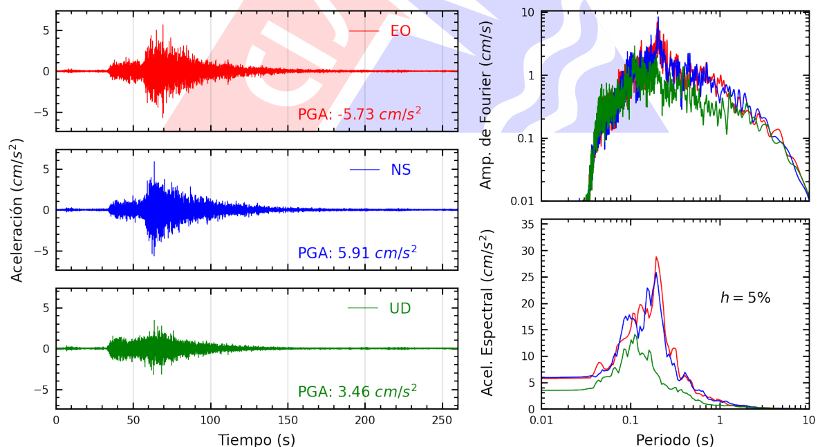
Figura A.10: Registros tiempo-historia, espectros de Fourier y de respuesta en las direcciones EO, NS y vertical de la estación SCCHO. Sismo de Lunahuana, Cañete - Lima del 2024-11-05, 14:39:42 (Hora local)
