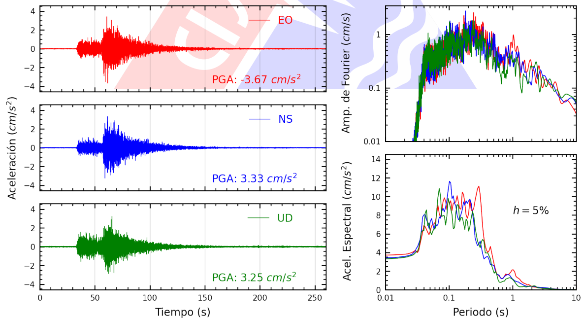
Figura A.14: Registros tiempo-historia, espectros de Fourier y de respuesta en las direcciones EO, NS y vertical de la estación USMP. Sismo de Lunahuana, Cañete - Lima del 2024-11-05, 14:39:42 (Hora local)
