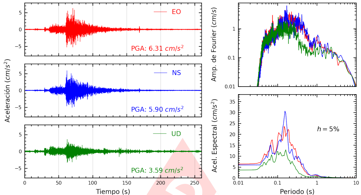
Figura A.9: Registros tiempo-historia, espectros de Fourier y de respuesta en las direcciones EO, NS y vertical de la estación SCOLI. Sismo de Lunahuana, Cañete - Lima del 2024-11-05, 14:39:42 (Hora local)
