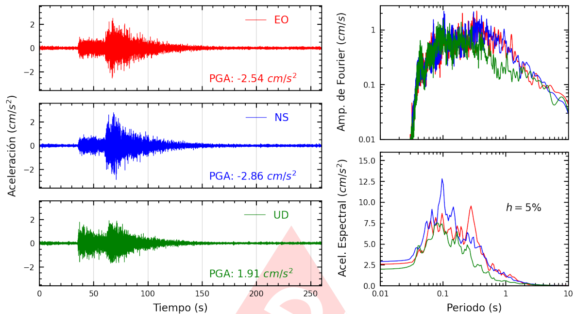
Figura A.19: Registros tiempo-historia, espectros de Fourier y de respuesta en las direcciones EO, NS y vertical de la estación MADRE. Sismo de Lunahuana, Cañete - Lima del 2024-11-05, 14:39:42 (Hora local)
