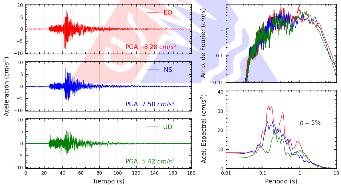
Figura A.2: Registros tiempo-historia, espectros de Fourier y de respuesta en las direcciones EO, NS y vertical de la estación SCAYA. Sismo de Lunahuana, Cañete - Lima del 2024-11-05, 14:39:42 (Hora local)
