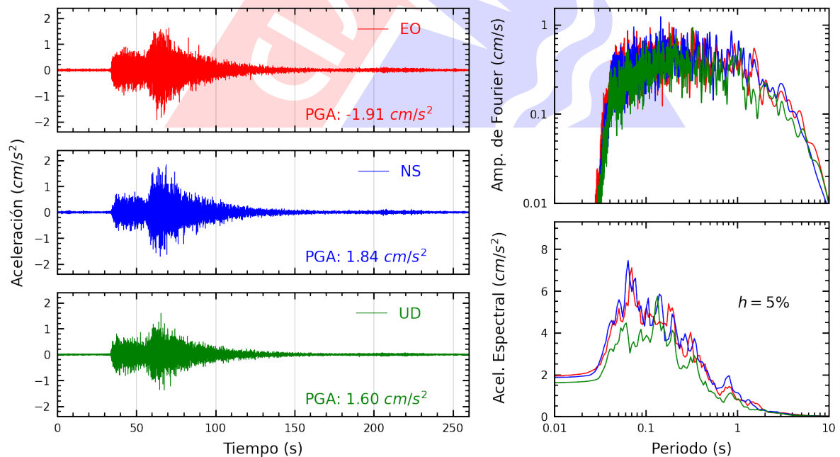
Figura A.28: Registros tiempo-historia, espectros de Fourier y de respuesta en las direcciones EO, NS y vertical de la estación BORJA. Sismo de Lunahuana, Cañete - Lima del 2024-11-05, 14:39:42 (Hora local)
