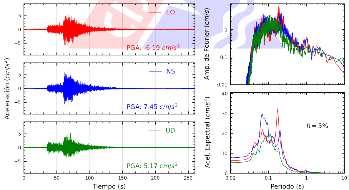
Figura A.8: Registros tiempo-historia, espectros de Fourier y de respuesta en las direcciones EO, NS y vertical de la estación INDEP. Sismo de Lunahuana, Cañete - Lima del 2024-11-05, 14:39:42 (Hora local)
