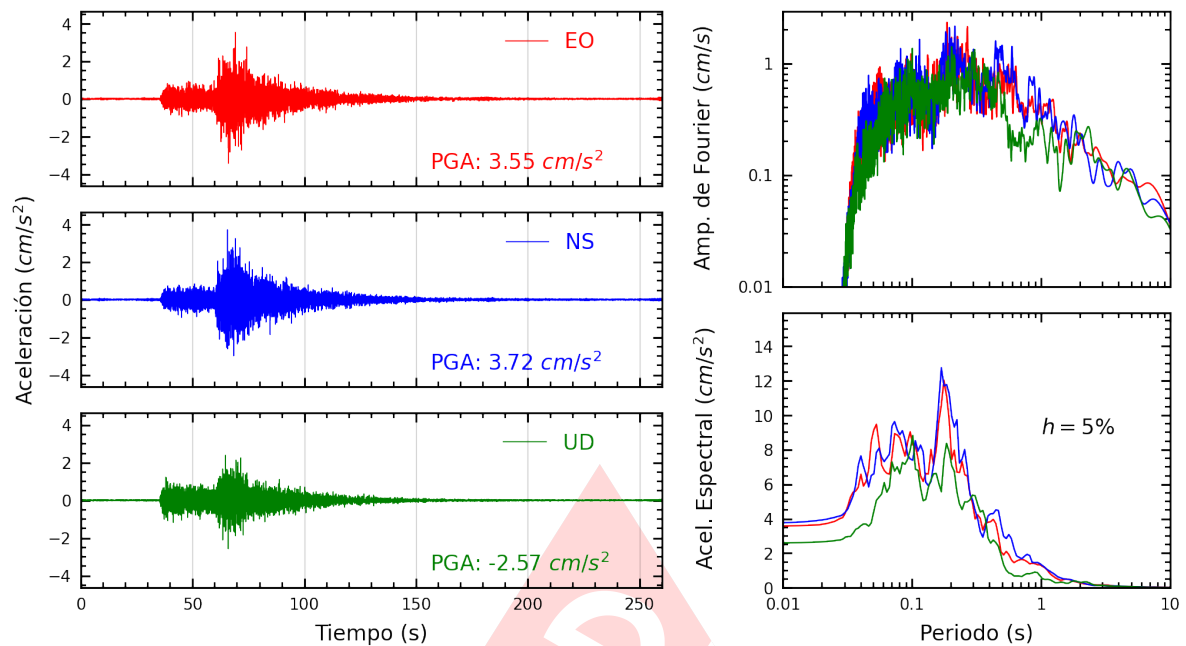
Figura A.13: Registros tiempo-historia, espectros de Fourier y de respuesta en las direcciones EO, NS y vertical de la estación COMAS. Sismo de Lunahuana, Cañete - Lima del 2024-11-05, 14:39:42 (Hora local)
