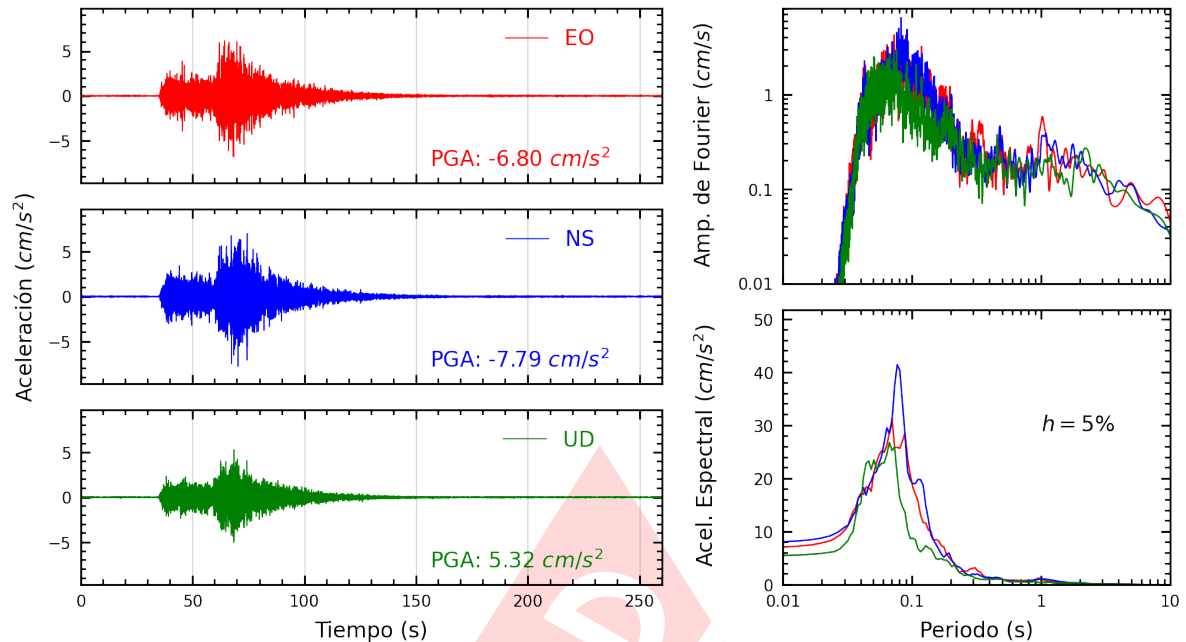
Figura A.7: Registros tiempo-historia, espectros de Fourier y de respuesta en las direcciones EO, NS y vertical de la estación JOSEO. Sismo de Lunahuana, Cañete - Lima del 2024-11-05, 14:39:42 (Hora local)
