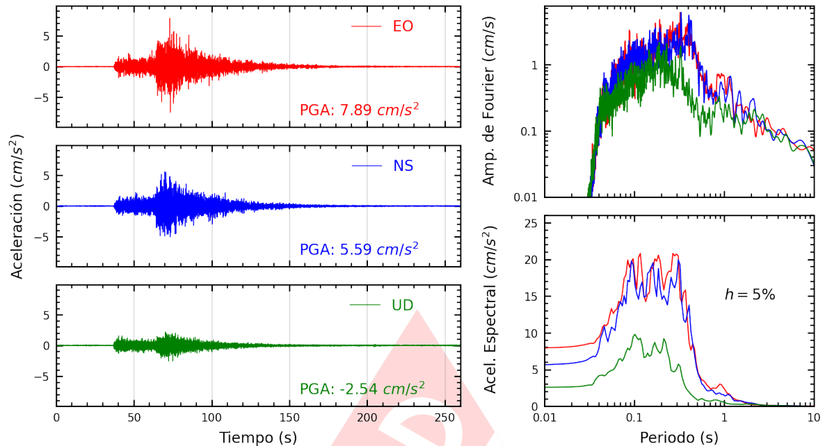
Figura A.5: Registros tiempo-historia, espectros de Fourier y de respuesta en las direcciones EO, NS y vertical de la estación DEFEN. Sismo de Lunahuana, Cañete - Lima del 2024-11-05, 14:39:42 (Hora local)
