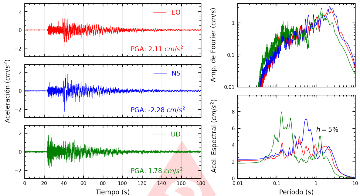
Figura A.27: Registros tiempo-historia, espectros de Fourier y de respuesta en las direcciones EO, NS y vertical de la estación SCHYO. Sismo de Lunahuana, Cañete - Lima del 2024-11-05, 14:39:42 (Hora local)
