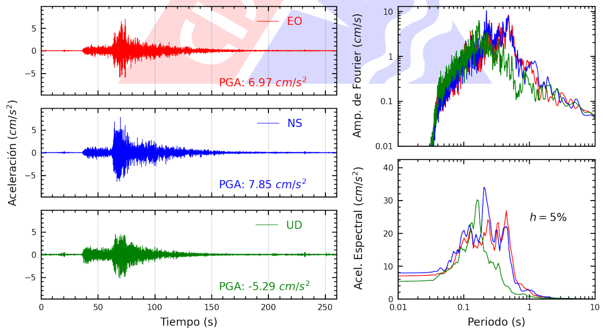
Figura A.6: Registros tiempo-historia, espectros de Fourier y de respuesta en las direcciones EO, NS y vertical de la estación MDPP. Sismo de Lunahuana, Cañete - Lima del 2024-11-05, 14:39:42 (Hora local)
