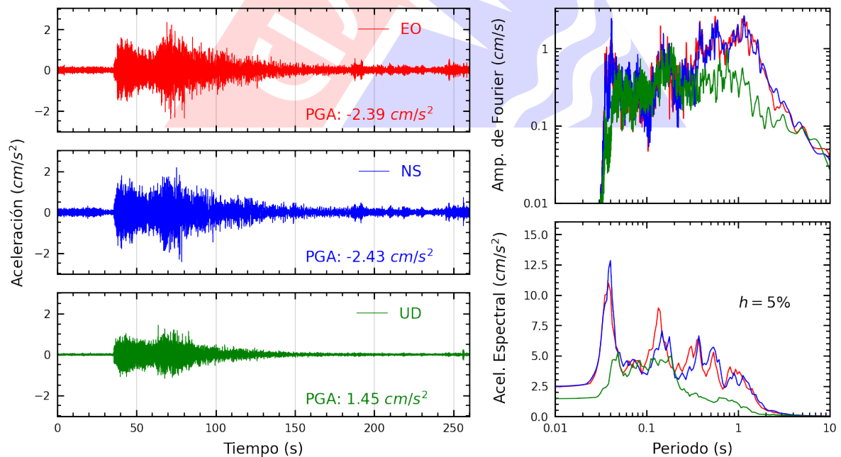
Figura A.24: Registros tiempo-historia, espectros de Fourier y de respuesta en las direcciones EO, NS y vertical de la estación DHNPE. Sismo de Lunahuana, Cañete - Lima del 2024-11-05, 14:39:42 (Hora local)
