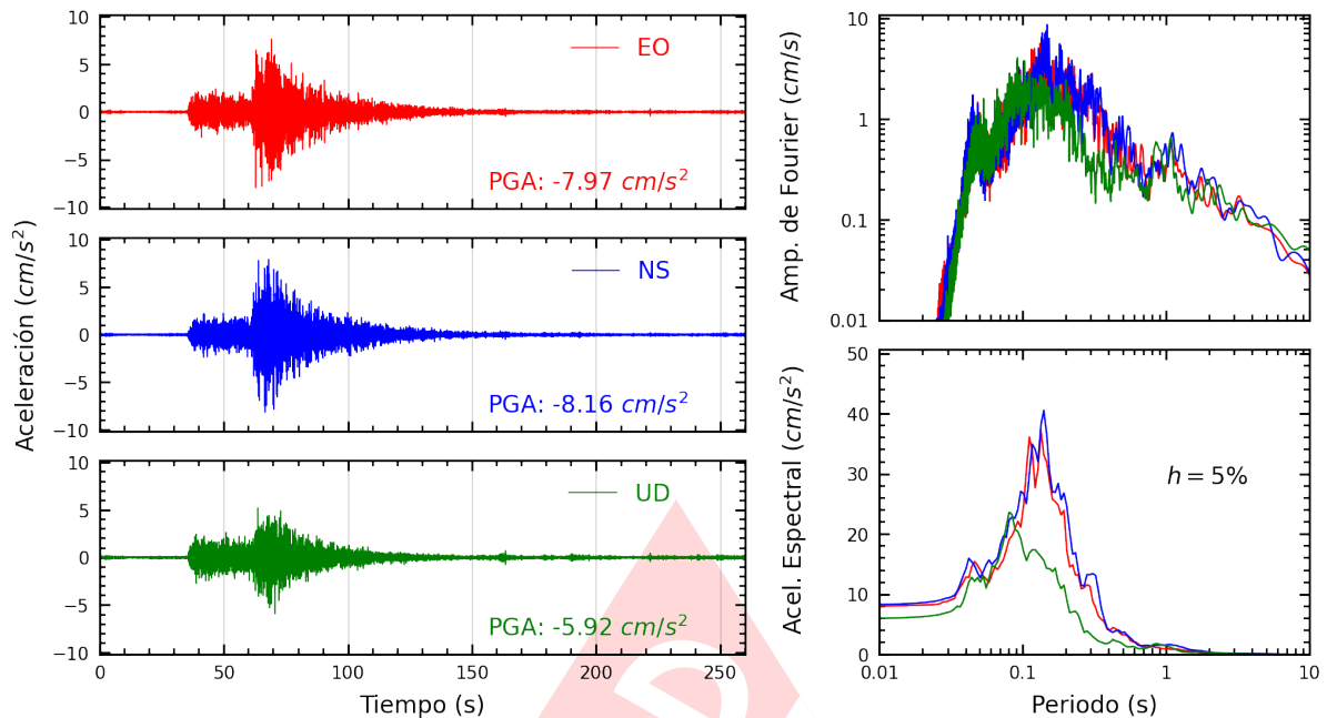
Figura A.3: Registros tiempo-historia, espectros de Fourier y de respuesta en las direcciones EO, NS y vertical de la estación CARAB. Sismo de Lunahuana, Cañete - Lima del 2024-11-05, 14:39:42 (Hora local)
