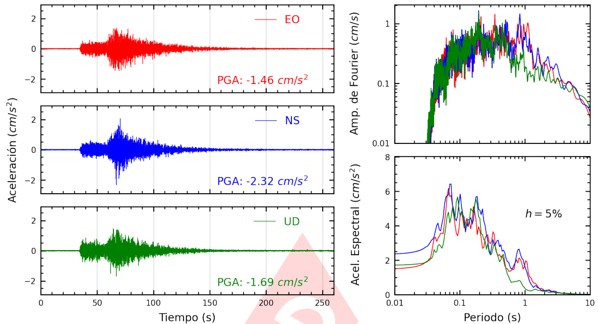
Figura A.25: Registros tiempo-historia, espectros de Fourier y de respuesta en las direcciones EO, NS y vertical de la estación UNFV. Sismo de Lunahuana, Cañete - Lima del 2024-11-05, 14:39:42 (Hora local)
