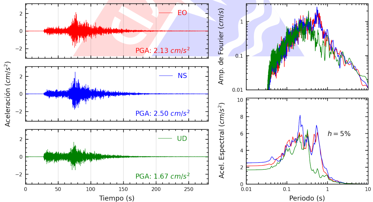
Figura A.22: Registros tiempo-historia, espectros de Fourier y de respuesta en las direcciones EO, NS y vertical de la estación CARAL. Sismo de Lunahuana, Cañete - Lima del 2024-11-05, 14:39:42 (Hora local)
