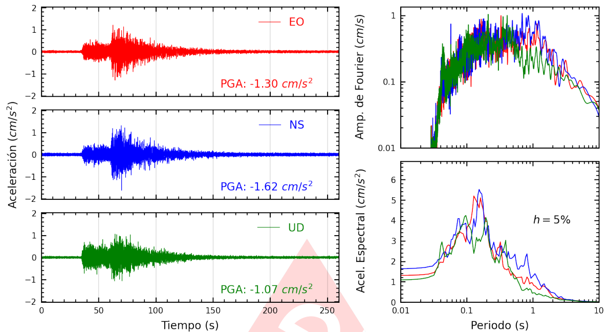
Figura A.29: Registros tiempo-historia, espectros de Fourier y de respuesta en las direcciones EO, NS y vertical de la estación BONDY. Sismo de Lunahuana, Cañete - Lima del 2024-11-05, 14:39:42 (Hora local)
