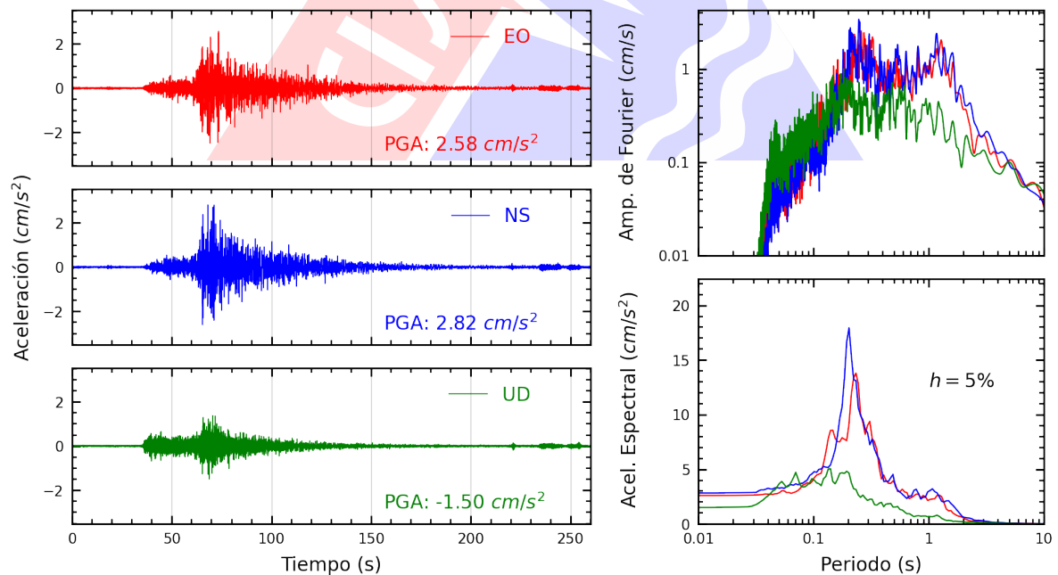
Figura A.20: Registros tiempo-historia, espectros de Fourier y de respuesta en las direcciones EO, NS y vertical de la estación DSMI. Sismo de Lunahuana, Cañete - Lima del 2024-11-05, 14:39:42 (Hora local)
