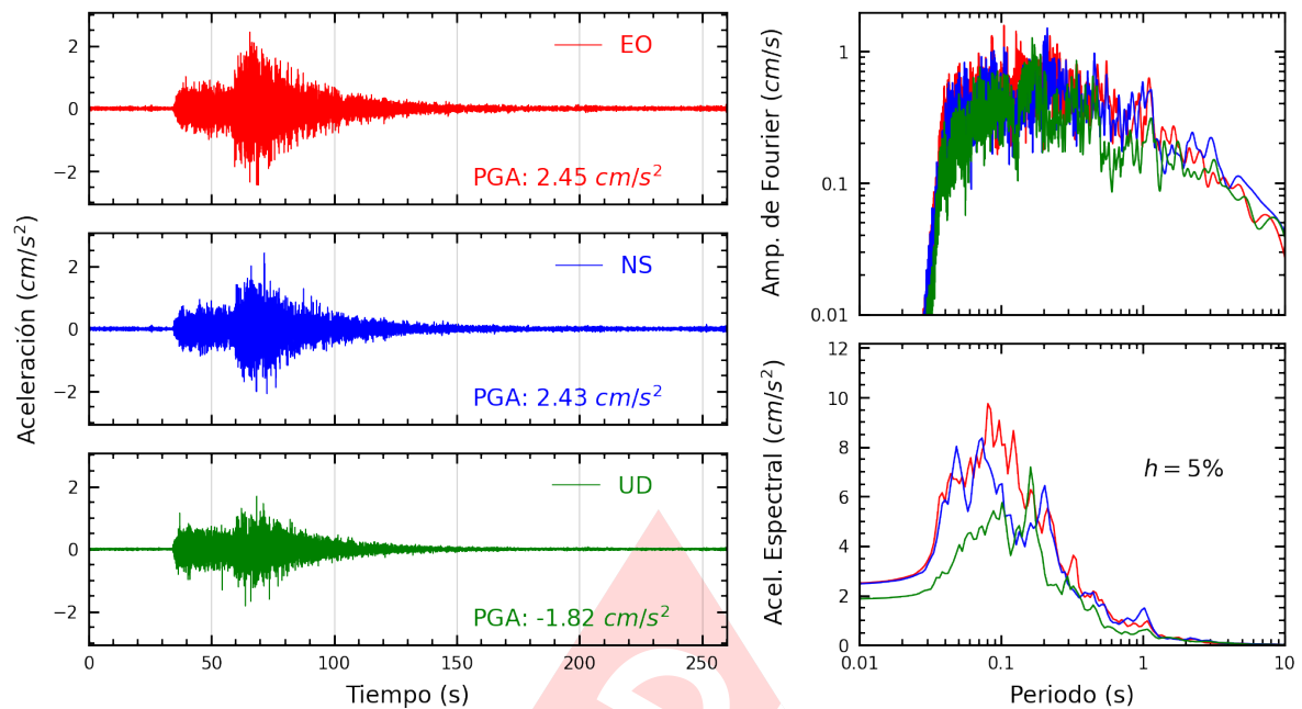
Figura A.23: Registros tiempo-historia, espectros de Fourier y de respuesta en las direcciones EO, NS y vertical de la estación CEPRE. Sismo de Lunahuana, Cañete - Lima del 2024-11-05, 14:39:42 (Hora local)
