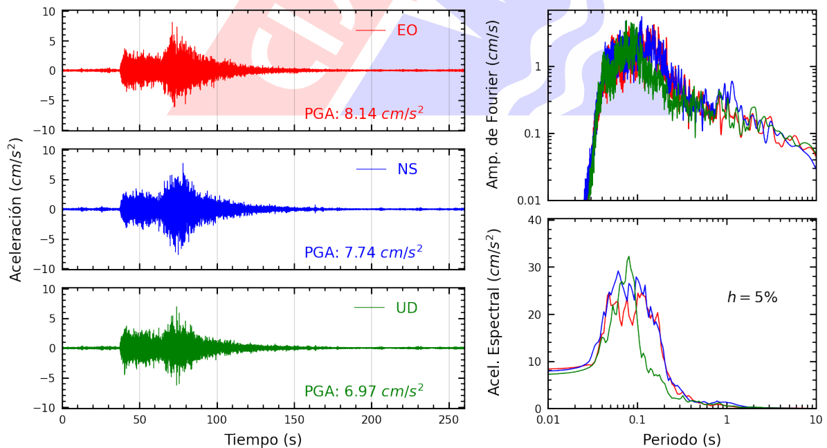
Figura A.4: Registros tiempo-historia, espectros de Fourier y de respuesta en las direcciones EO, NS y vertical de la estación SROSA. Sismo de Lunahuana, Cañete - Lima del 2024-11-05, 14:39:42 (Hora local)
