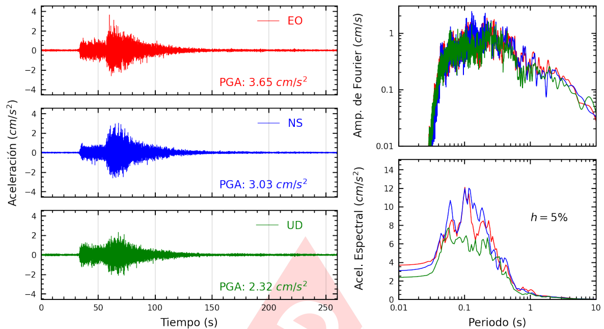
Figura A.15: Registros tiempo-historia, espectros de Fourier y de respuesta en las direcciones EO, NS y vertical de la estación URPPE. Sismo de Lunahuana, Cañete - Lima del 2024-11-05, 14:39:42 (Hora local)
