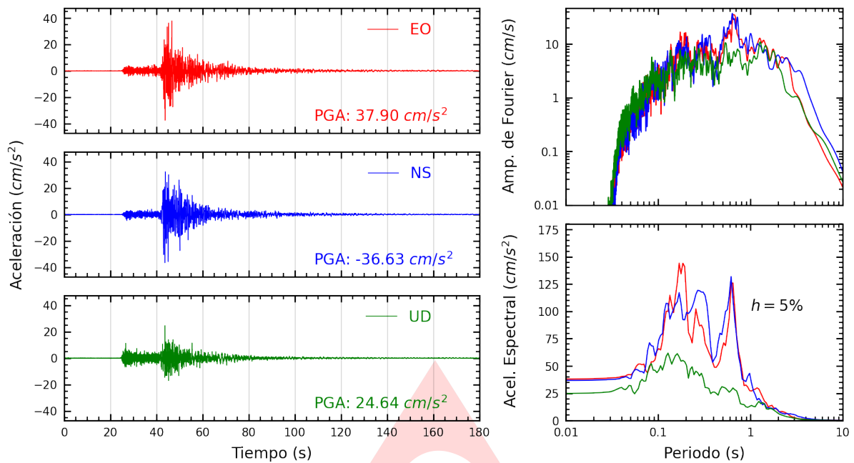
Figura A.1: Registros tiempo-historia, espectros de Fourier y de respuesta en las direcciones EO, NS y vertical de la estación SCICA. Sismo de Lunahuana, Cañete - Lima del 2024-11-05, 14:39:42 (Hora local)
