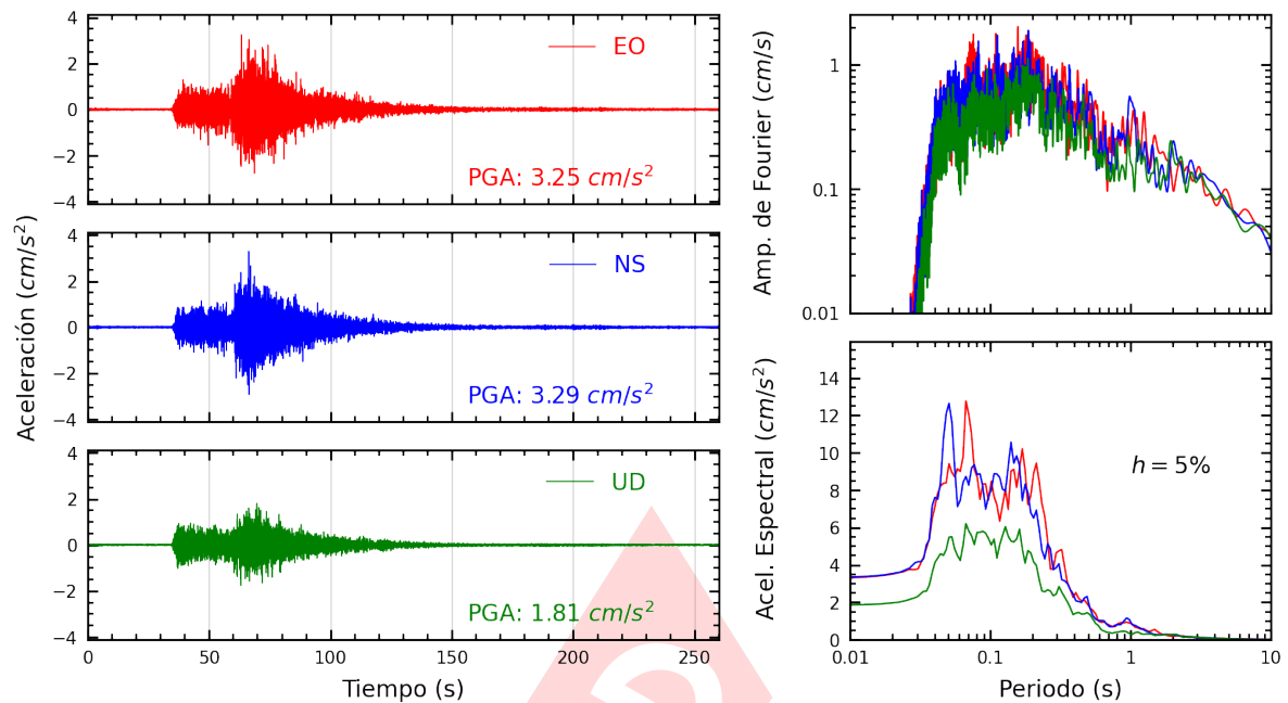
Figura A.17: Registros tiempo-historia, espectros de Fourier y de respuesta en las direcciones EO, NS y vertical de la estación FICPE. Sismo de Lunahuana, Cañete - Lima del 2024-11-05, 14:39:42 (Hora local)
