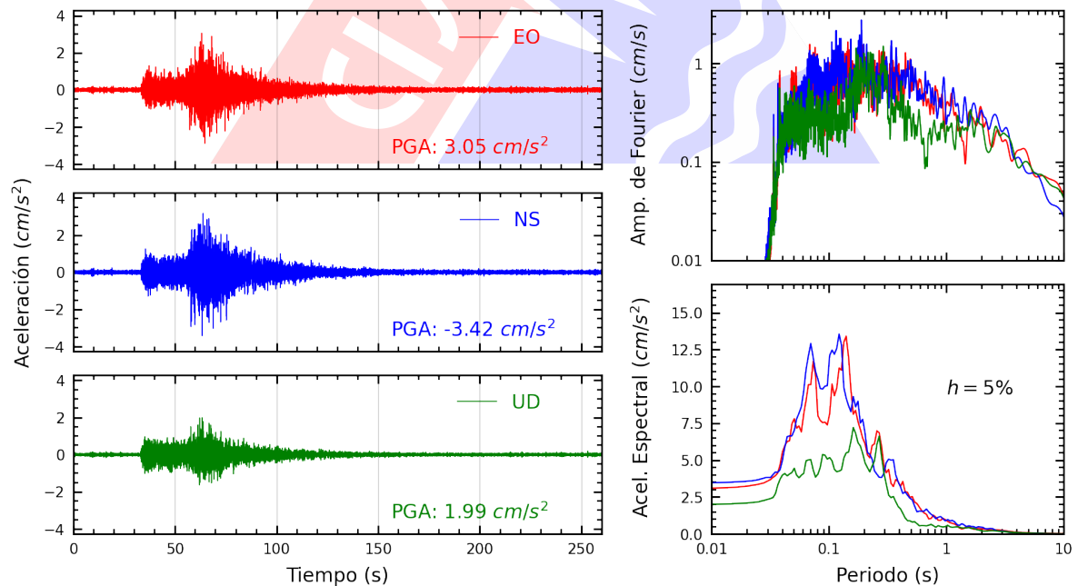
Figura A.16: Registros tiempo-historia, espectros de Fourier y de respuesta en las direcciones EO, NS y vertical de la estación UPCVI. Sismo de Lunahuana, Cañete - Lima del 2024-11-05, 14:39:42 (Hora local)
