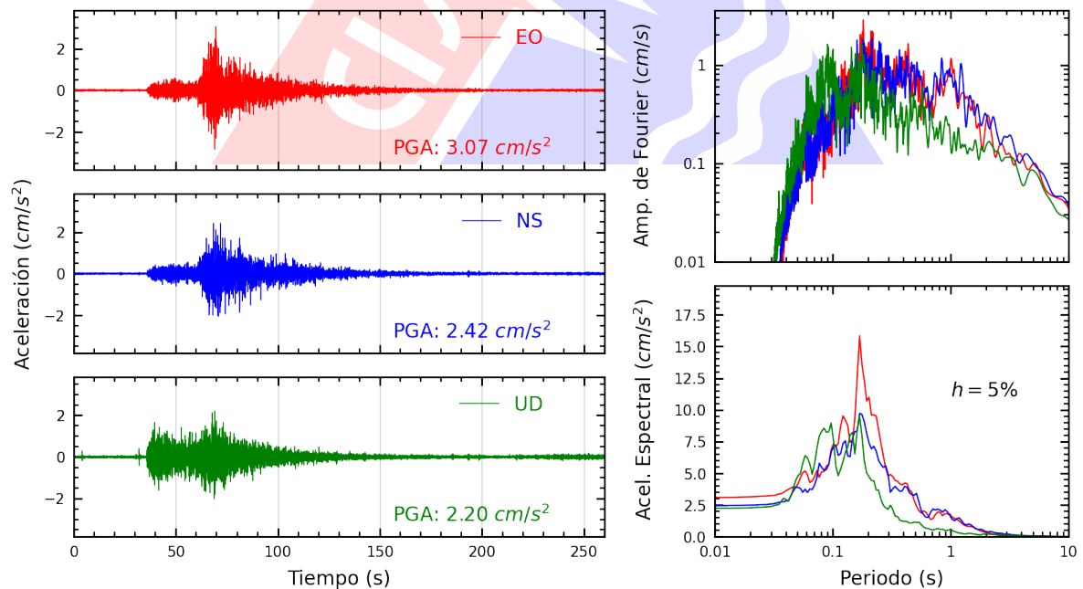
Figura A.18: Registros tiempo-historia, espectros de Fourier y de respuesta en las direcciones EO, NS y vertical de la estación RAMON. Sismo de Lunahuana, Cañete - Lima del 2024-11-05, 14:39:42 (Hora local)
