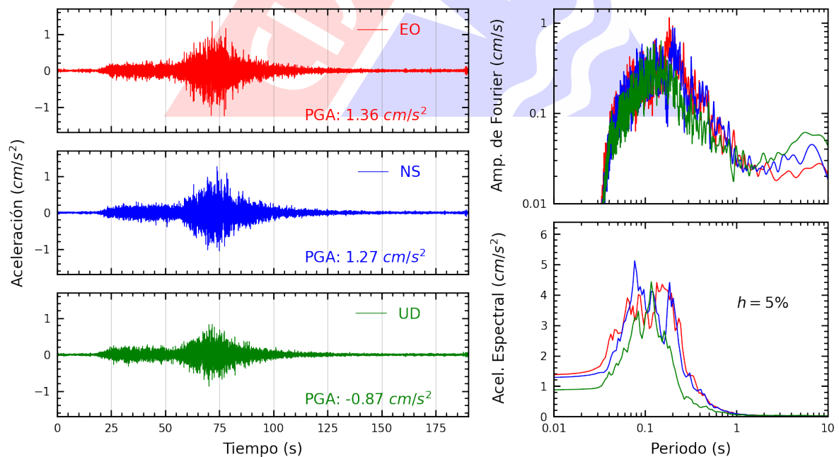
Figura A.12: Registros tiempo-historia, espectros de Fourier y de respuesta en las direcciones EO, NS y vertical de la estación INDEP. Sismo de Palpa, Palpa - Ica del 2024-11-07, 01:24:37 (Hora local)
