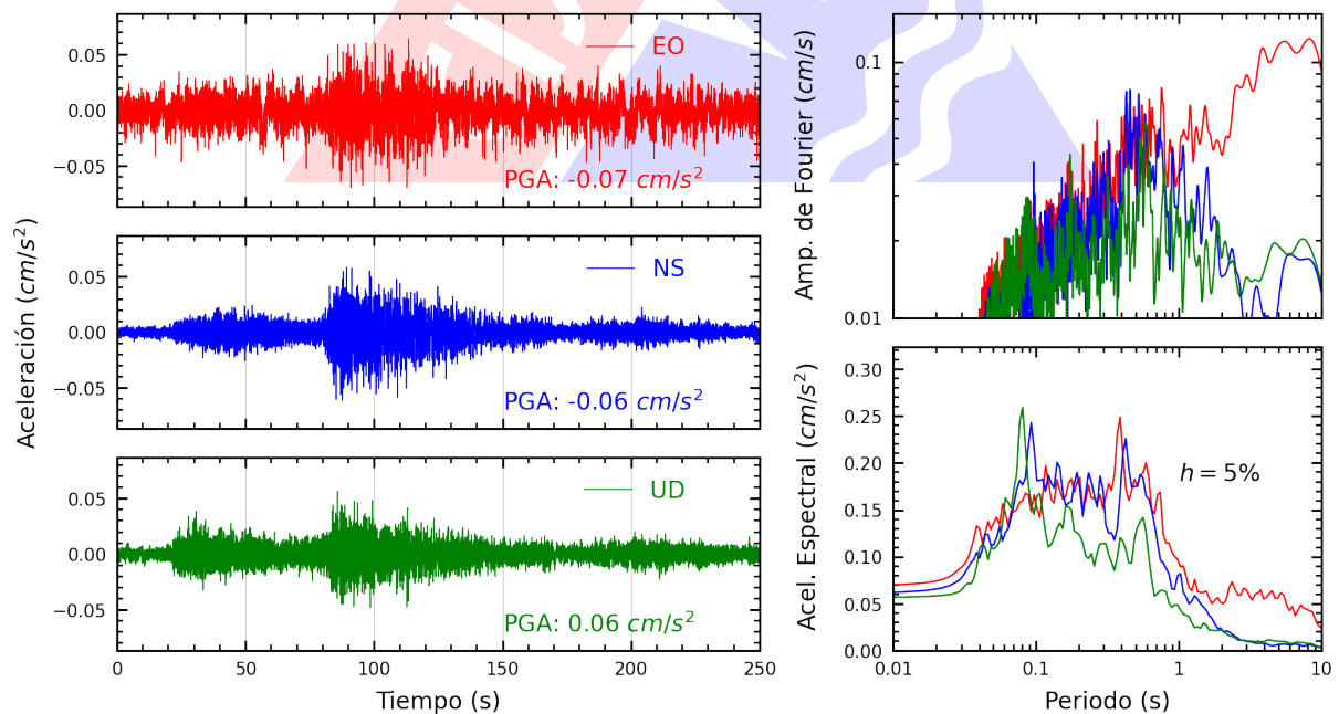
Figura A.48: Registros tiempo-historia, espectros de Fourier y de respuesta en las direcciones EO, NS y vertical de la estación UJBG3. Sismo de Palpa, Palpa - Ica del 2024-11-07, 01:24:37 (Hora local)
