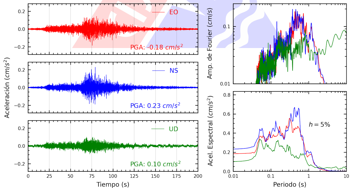
Figura A.42: Registros tiempo-historia, espectros de Fourier y de respuesta en las direcciones EO, NS y vertical de la estación SCARQ. Sismo de Palpa, Palpa - Ica del 2024-11-07, 01:24:37 (Hora local)
