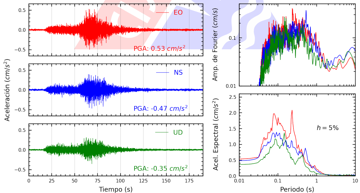
Figura A.34: Registros tiempo-historia, espectros de Fourier y de respuesta en las direcciones EO, NS y vertical de la estación CEPRE. Sismo de Palpa, Palpa - Ica del 2024-11-07, 01:24:37 (Hora local)
