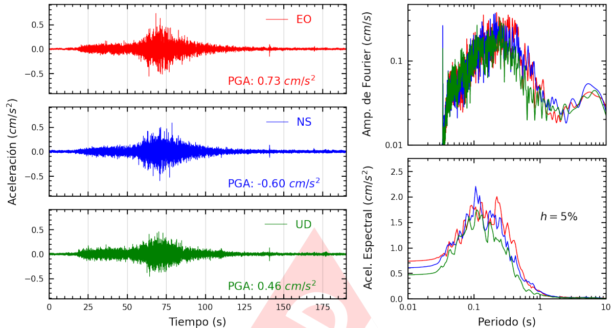
Figura A.23: Registros tiempo-historia, espectros de Fourier y de respuesta en las direcciones EO, NS y vertical de la estación USMP. Sismo de Palpa, Palpa - Ica del 2024-11-07, 01:24:37 (Hora local)
