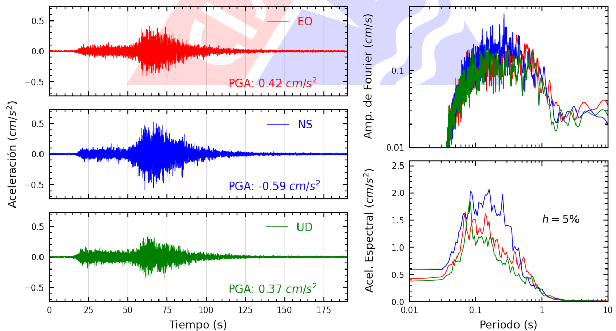
Figura A.30: Registros tiempo-historia, espectros de Fourier y de respuesta en las direcciones EO, NS y vertical de la estación SERVI. Sismo de Palpa, Palpa - Ica del 2024-11-07, 01:24:37 (Hora local)
