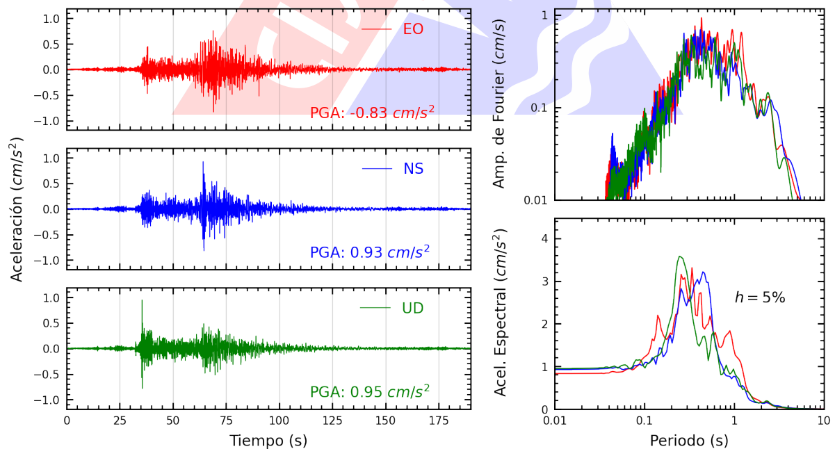
Figura A.18: Registros tiempo-historia, espectros de Fourier y de respuesta en las direcciones EO, NS y vertical de la estación SCAYA. Sismo de Palpa, Palpa - Ica del 2024-11-07, 01:24:37 (Hora local)
