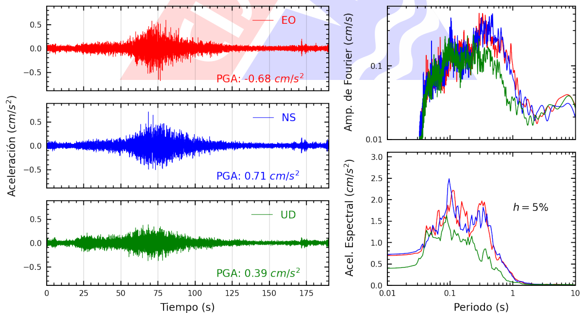
Figura A.24: Registros tiempo-historia, espectros de Fourier y de respuesta en las direcciones EO, NS y vertical de la estación MADRE. Sismo de Palpa, Palpa - Ica del 2024-11-07, 01:24:37 (Hora local)
