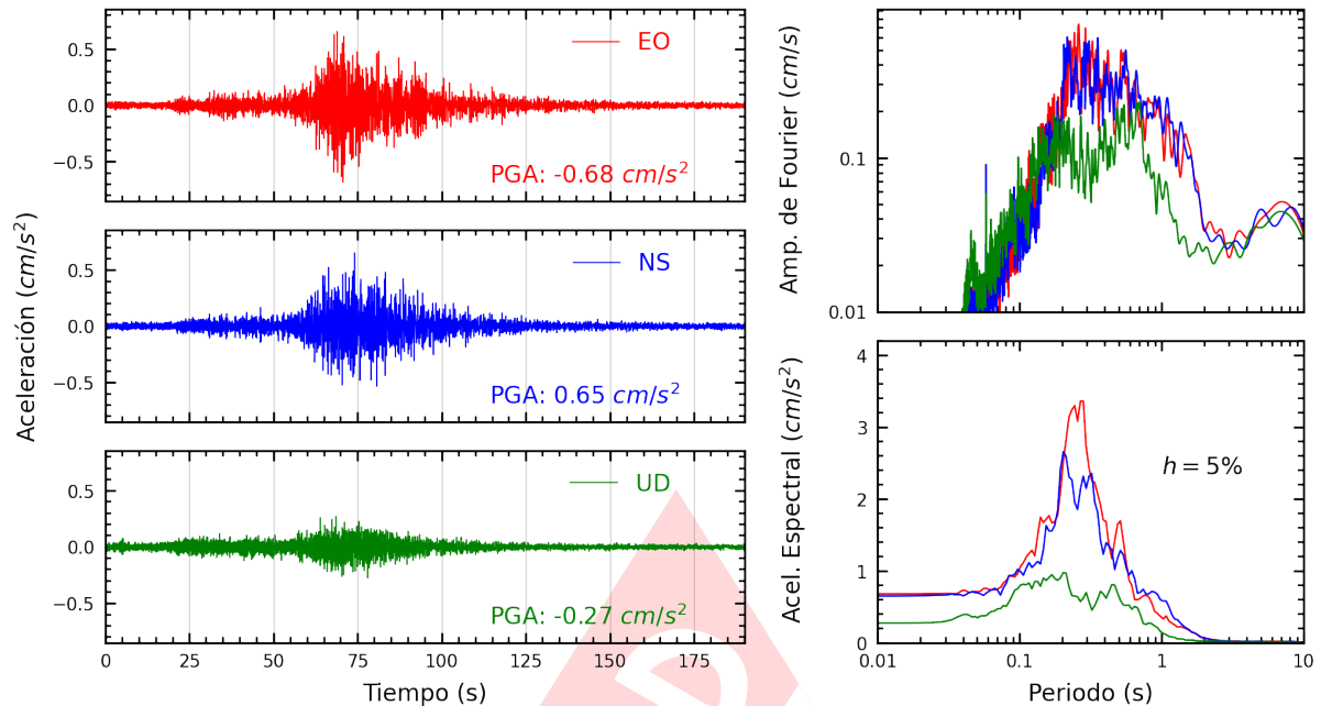
Figura A.25: Registros tiempo-historia, espectros de Fourier y de respuesta en las direcciones EO, NS y vertical de la estación DSML. Sismo de Palpa, Palpa - Ica del 2024-11-07, 01:24:37 (Hora local)
