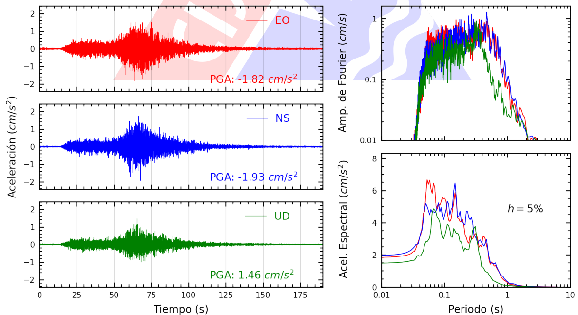
Figura A.6: Registros tiempo-historia, espectros de Fourier y de respuesta en las direcciones EO, NS y vertical de la estación UNTEL. Sismo de Palpa, Palpa - Ica del 2024-11-07, 01:24:37 (Hora local)
