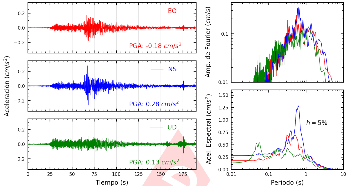
Figura A.41: Registros tiempo-historia, espectros de Fourier y de respuesta en las direcciones EO, NS y vertical de la estación SCHYO. Sismo de Palpa, Palpa - Ica del 2024-11-07, 01:24:37 (Hora local)
