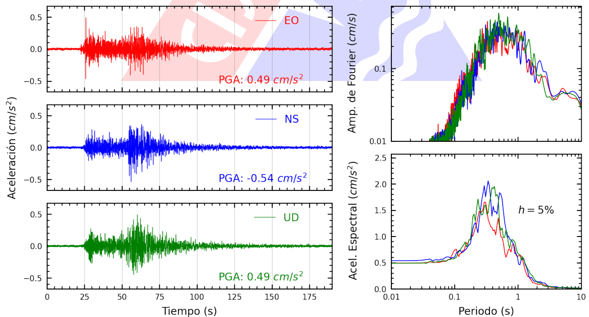
Figura A.32: Registros tiempo-historia, espectros de Fourier y de respuesta en las direcciones EO, NS y vertical de la estación UNSCH. Sismo de Palpa, Palpa - Ica del 2024-11-07, 01:24:37 (Hora local)
