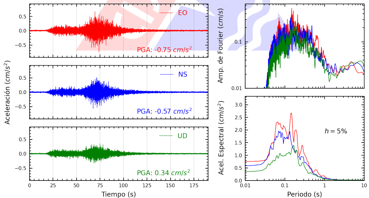
Figura A.22: Registros tiempo-historia, espectros de Fourier y de respuesta en las direcciones EO, NS y vertical de la estación FICPE. Sismo de Palpa, Palpa - Ica del 2024-11-07, 01:24:37 (Hora local)
