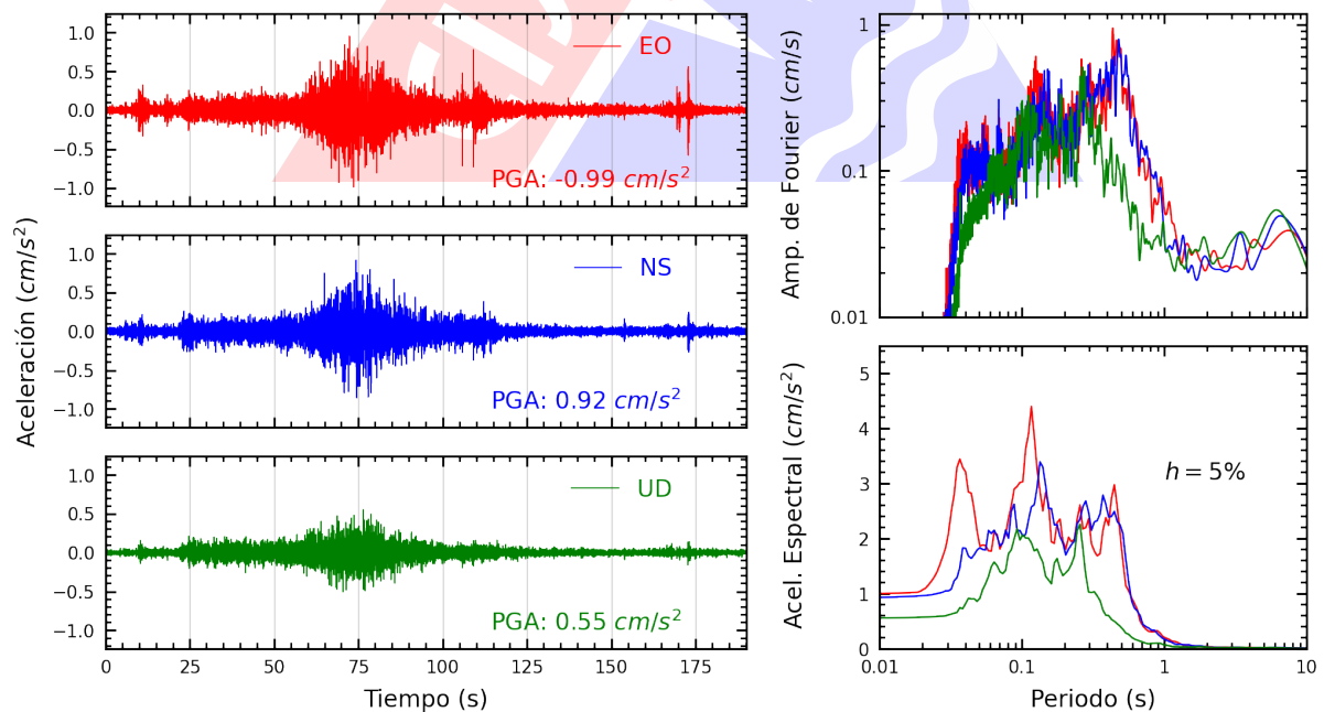
Figura A.16: Registros tiempo-historia, espectros de Fourier y de respuesta en las direcciones EO, NS y vertical de la estación OLIVO. Sismo de Palpa, Palpa - Ica del 2024-11-07, 01:24:37 (Hora local)
