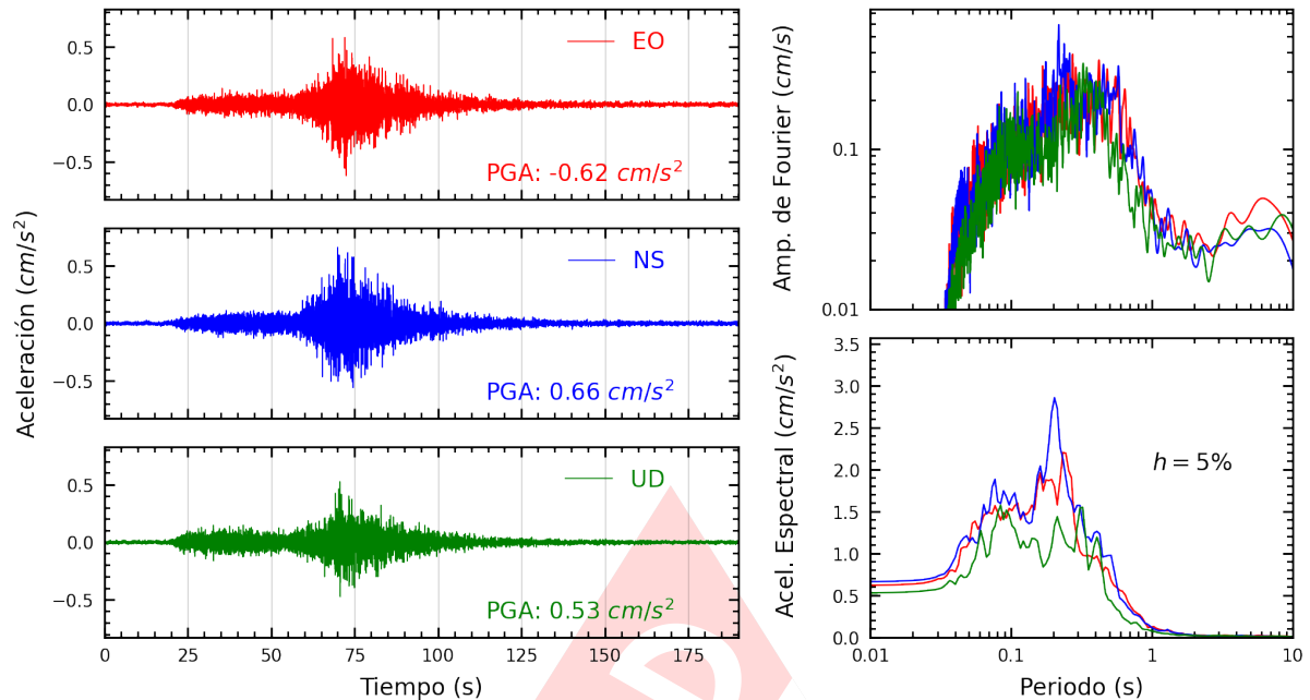
Figura A.27: Registros tiempo-historia, espectros de Fourier y de respuesta en las direcciones EO, NS y vertical de la estación COMAS. Sismo de Palpa, Palpa - Ica del 2024-11-07, 01:24:37 (Hora local)
