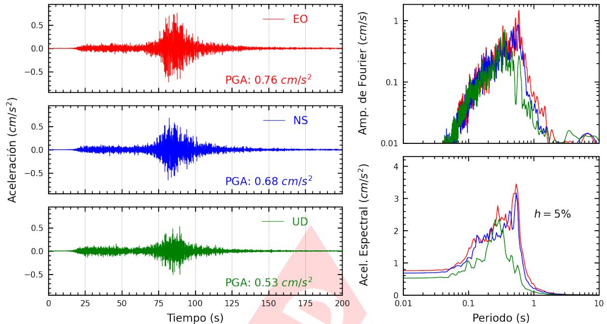
Figura A.21: Registros tiempo-historia, espectros de Fourier y de respuesta en las direcciones EO, NS y vertical de la estación CARAL. Sismo de Palpa, Palpa - Ica del 2024-11-07, 01:24:37 (Hora local)
