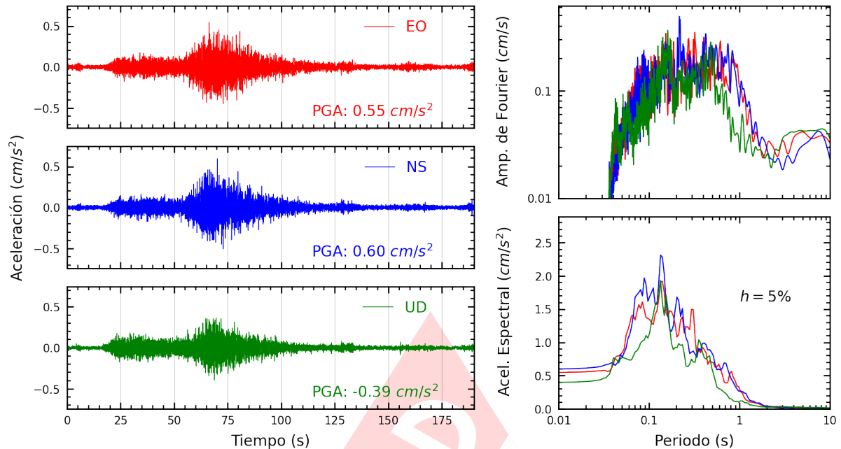
Figura A.29: Registros tiempo-historia, espectros de Fourier y de respuesta en las direcciones EO, NS y vertical de la estación UPCSM. Sismo de Palpa, Palpa - Ica del 2024-11-07, 01:24:37 (Hora local)
