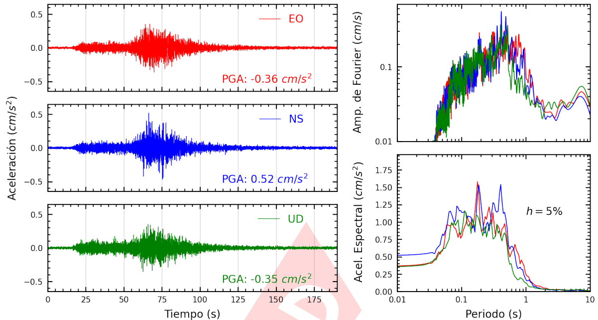
Figura A.35: Registros tiempo-historia, espectros de Fourier y de respuesta en las direcciones EO, NS y vertical de la estación UNFV. Sismo de Palpa, Palpa - Ica del 2024-11-07, 01:24:37 (Hora local)
