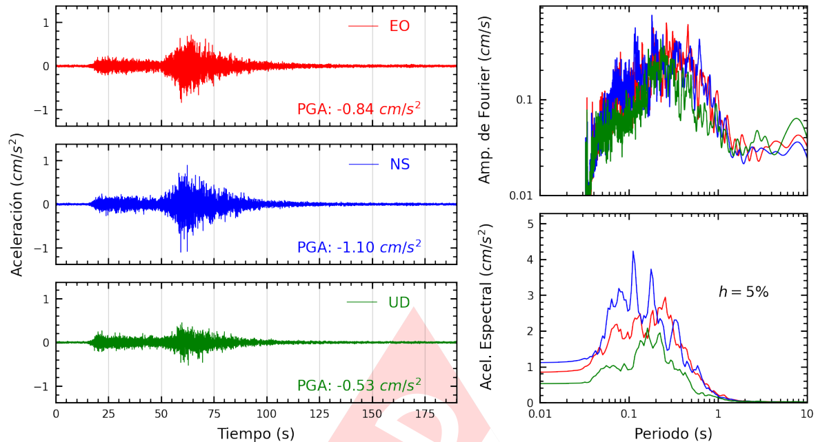
Figura A.15: Registros tiempo-historia, espectros de Fourier y de respuesta en las direcciones EO, NS y vertical de la estación UPCVI. Sismo de Palpa, Palpa - Ica del 2024-11-07, 01:24:37 (Hora local)
