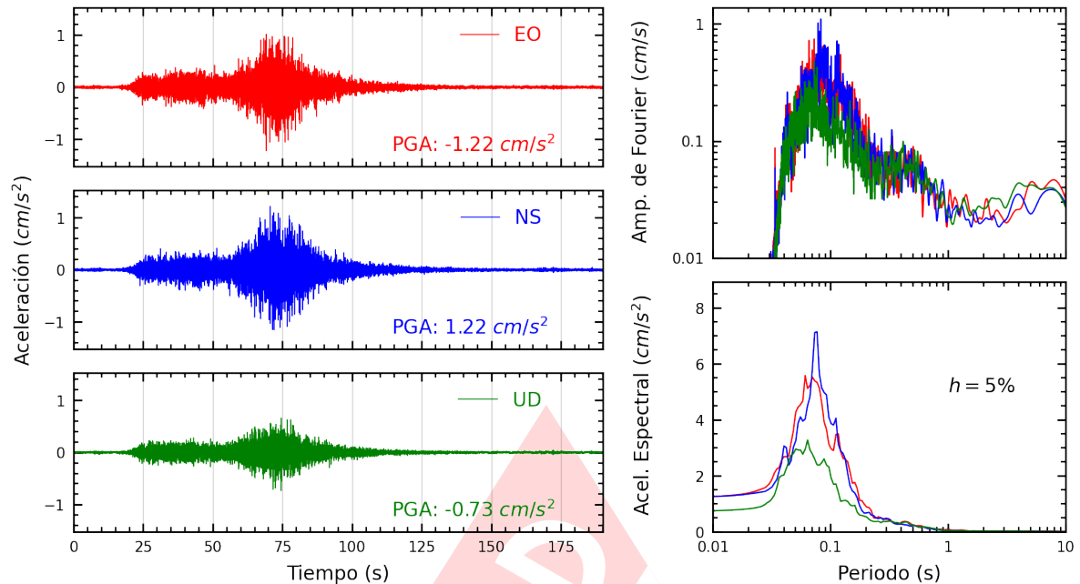
Figura A.13: Registros tiempo-historia, espectros de Fourier y de respuesta en las direcciones EO, NS y vertical de la estación JOSEO. Sismo de Palpa, Palpa - Ica del 2024-11-07, 01:24:37 (Hora local)
