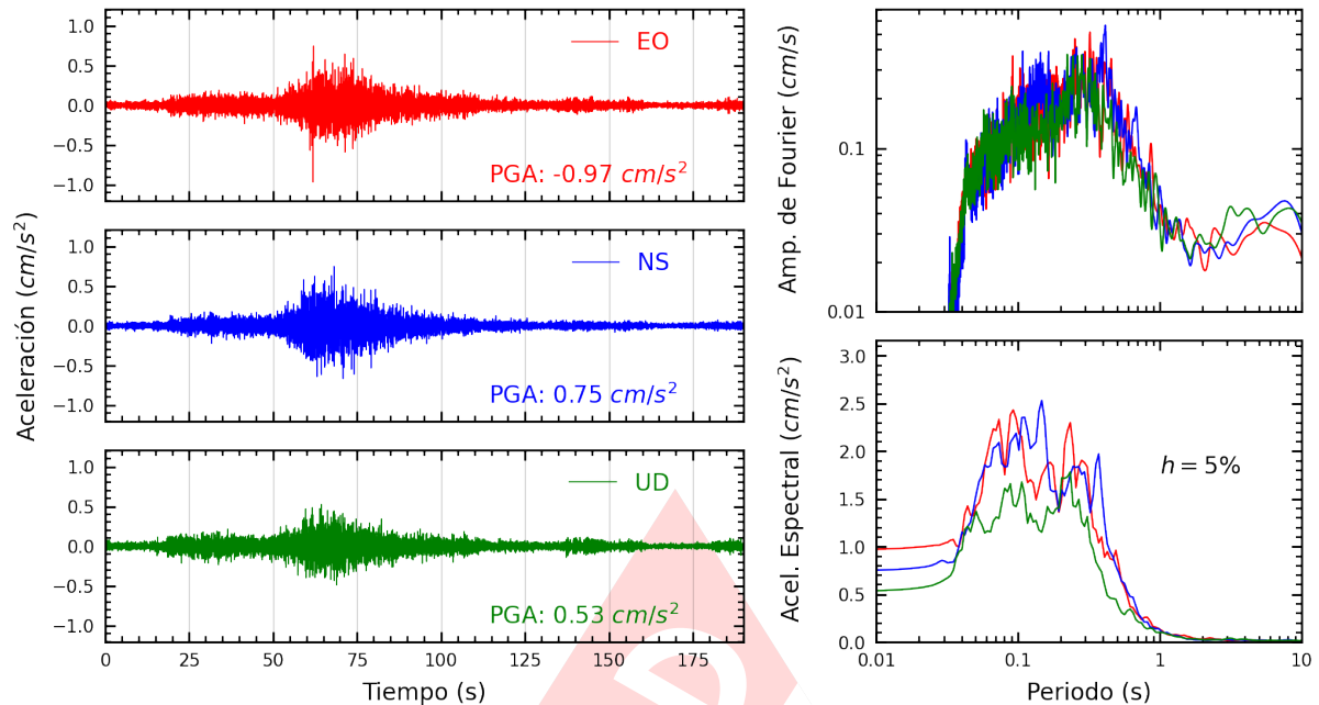
Figura A.17: Registros tiempo-historia, espectros de Fourier y de respuesta en las direcciones EO, NS y vertical de la estación URPE. Sismo de Palpa, Palpa - Ica del 2024-11-07, 01:24:37 (Hora local)
