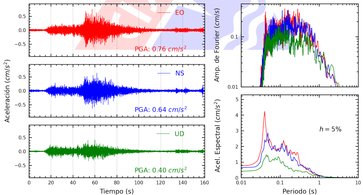
Figura A.20: Registros tiempo-historia, espectros de Fourier y de respuesta en las direcciones EO, NS y vertical de la estación PACHA. Sismo de Palpa, Palpa - Ica del 2024-11-07, 01:24:37 (Hora local)
