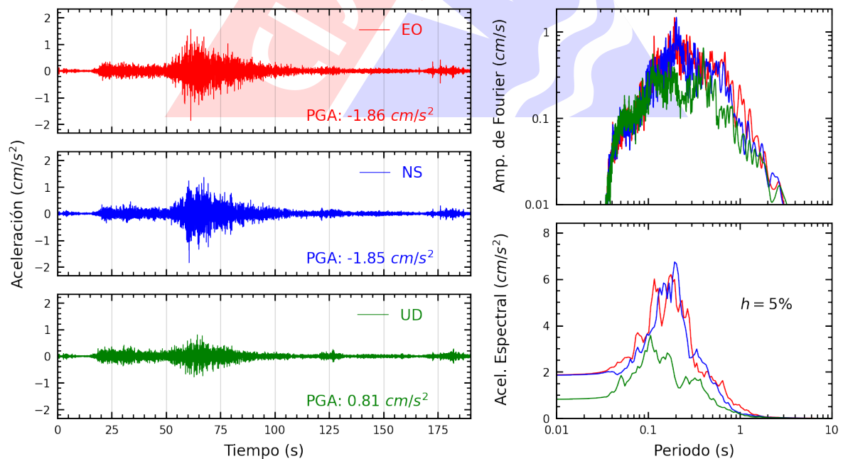
Figura A.8: Registros tiempo-historia, espectros de Fourier y de respuesta en las direcciones EO, NS y vertical de la estación SCCHO. Sismo de Palpa, Palpa - Ica del 2024-11-07, 01:24:37 (Hora local)
