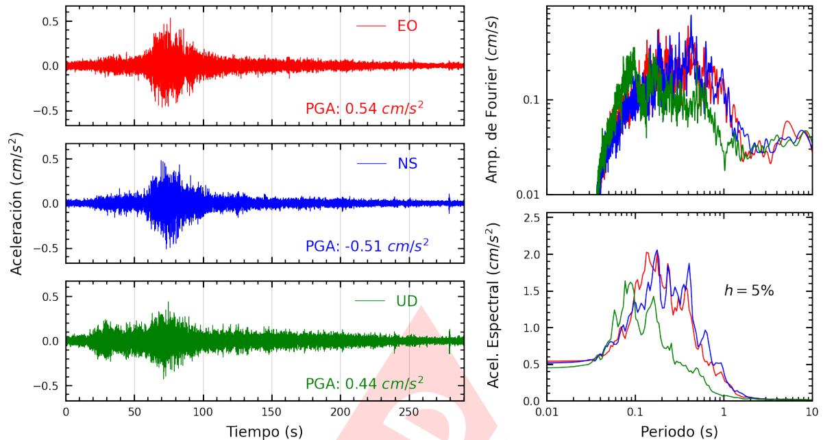
Figura A.33: Registros tiempo-historia, espectros de Fourier y de respuesta en las direcciones EO, NS y vertical de la estación RAMON. Sismo de Palpa, Palpa - Ica del 2024-11-07, 01:24:37 (Hora local)
