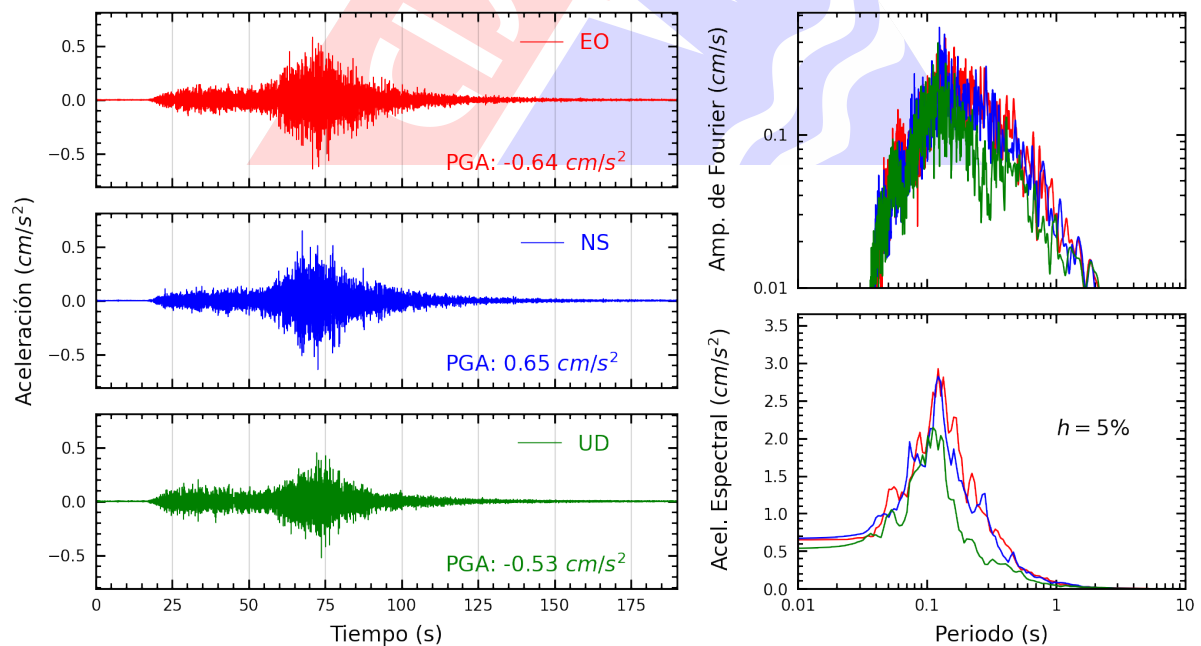
Figura A.28: Registros tiempo-historia, espectros de Fourier y de respuesta en las direcciones EO, NS y vertical de la estación JALV2. Sismo de Palpa, Palpa - Ica del 2024-11-07, 01:24:37 (Hora local)
