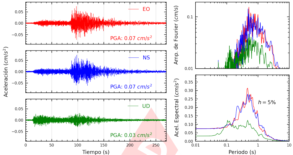
Figura A.47: Registros tiempo-historia, espectros de Fourier y de respuesta en las direcciones EO, NS y vertical de la estación UNIA. Sismo de Palpa, Palpa - Ica del 2024-11-07, 01:24:37 (Hora local)
