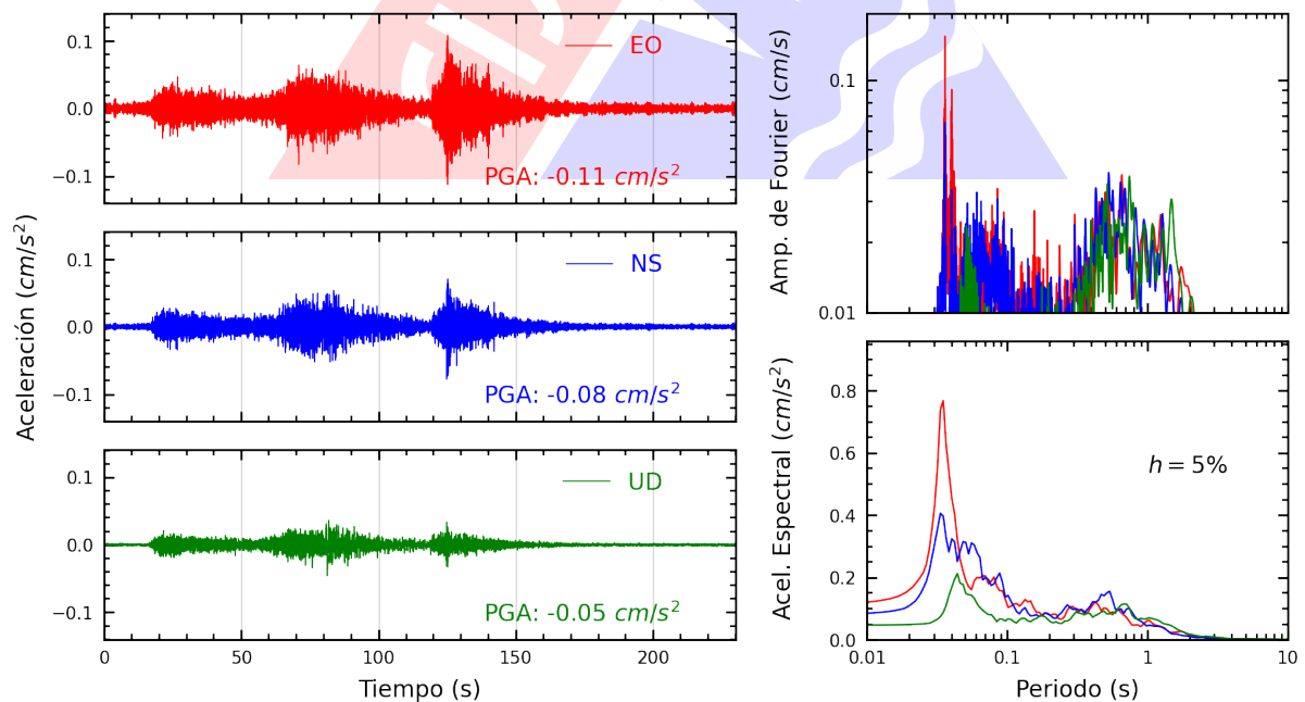
Figura A.46: Registros tiempo-historia, espectros de Fourier y de respuesta en las direcciones EO, NS y vertical de la estación UNAM. Sismo de Palpa, Palpa - Ica del 2024-11-07, 01:24:37 (Hora local)
