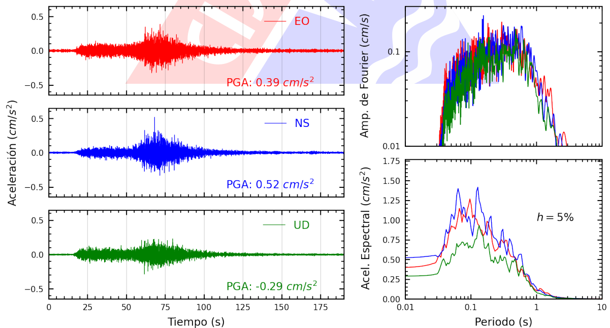
Figura A.36: Registros tiempo-historia, espectros de Fourier y de respuesta en las direcciones EO, NS y vertical de la estación BORJA. Sismo de Palpa, Palpa - Ica del 2024-11-07, 01:24:37 (Hora local)
