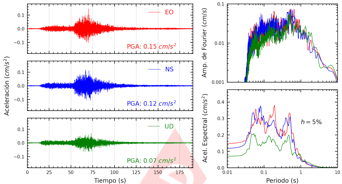
Figura A.45: Registros tiempo-historia, espectros de Fourier y de respuesta en las direcciones EO, NS y vertical de la estación UNSA2. Sismo de Palpa, Palpa - Ica del 2024-11-07, 01:24:37 (Hora local)
