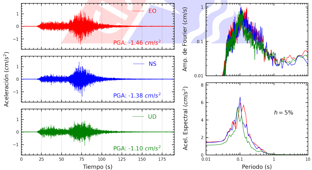
Figura A.10: Registros tiempo-historia, espectros de Fourier y de respuesta en las direcciones EO, NS y vertical de la estación AMORE. Sismo de Palpa, Palpa - Ica del 2024-11-07, 01:24:37 (Hora local)
