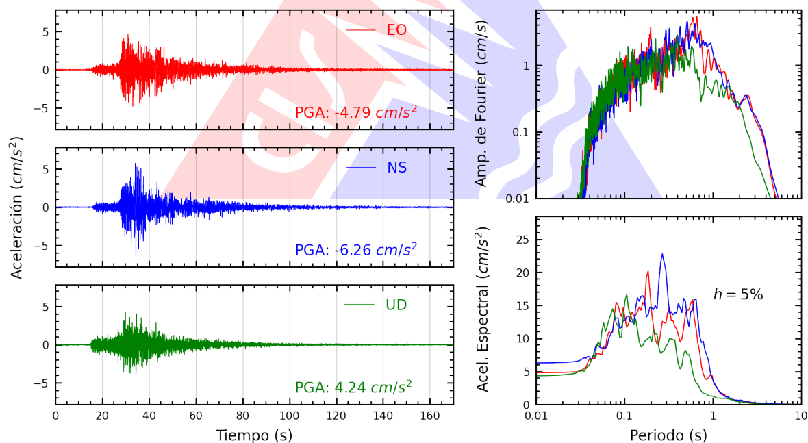
Figura A.2: Registros tiempo-historia, espectros de Fourier y de respuesta en las direcciones EO, NS y vertical de la estación SCICA. Sismo de Palpa, Palpa - Ica del 2024-11-07, 01:24:37 (Hora local)
