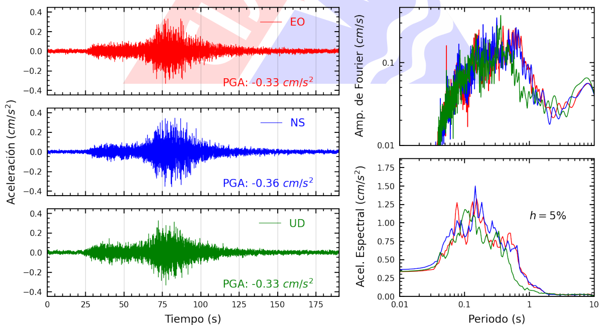
Figura A.40: Registros tiempo-historia, espectros de Fourier y de respuesta en las direcciones EO, NS y vertical de la estación UNMSM. Sismo de Palpa, Palpa - Ica del 2024-11-07, 01:24:37 (Hora local)
