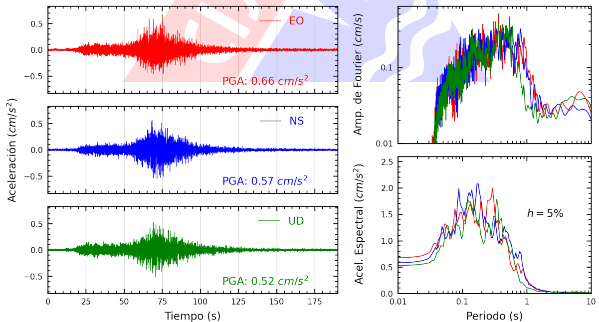
Figura A.26: Registros tiempo-historia, espectros de Fourier y de respuesta en las direcciones EO, NS y vertical de la estación IMCA. Sismo de Palpa, Palpa - Ica del 2024-11-07, 01:24:37 (Hora local)
