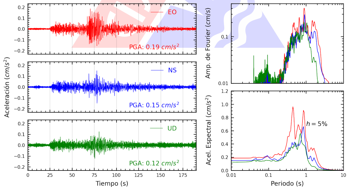
Figura A.44: Registros tiempo-historia, espectros de Fourier y de respuesta en las direcciones EO, NS y vertical de la estación SCCUS. Sismo de Palpa, Palpa - Ica del 2024-11-07, 01:24:37 (Hora local)
