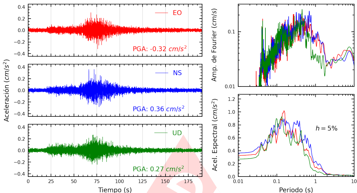
Figura A.39: Registros tiempo-historia, espectros de Fourier y de respuesta en las direcciones EO, NS y vertical de la estación BONDY. Sismo de Palpa, Palpa - Ica del 2024-11-07, 01:24:37 (Hora local)
