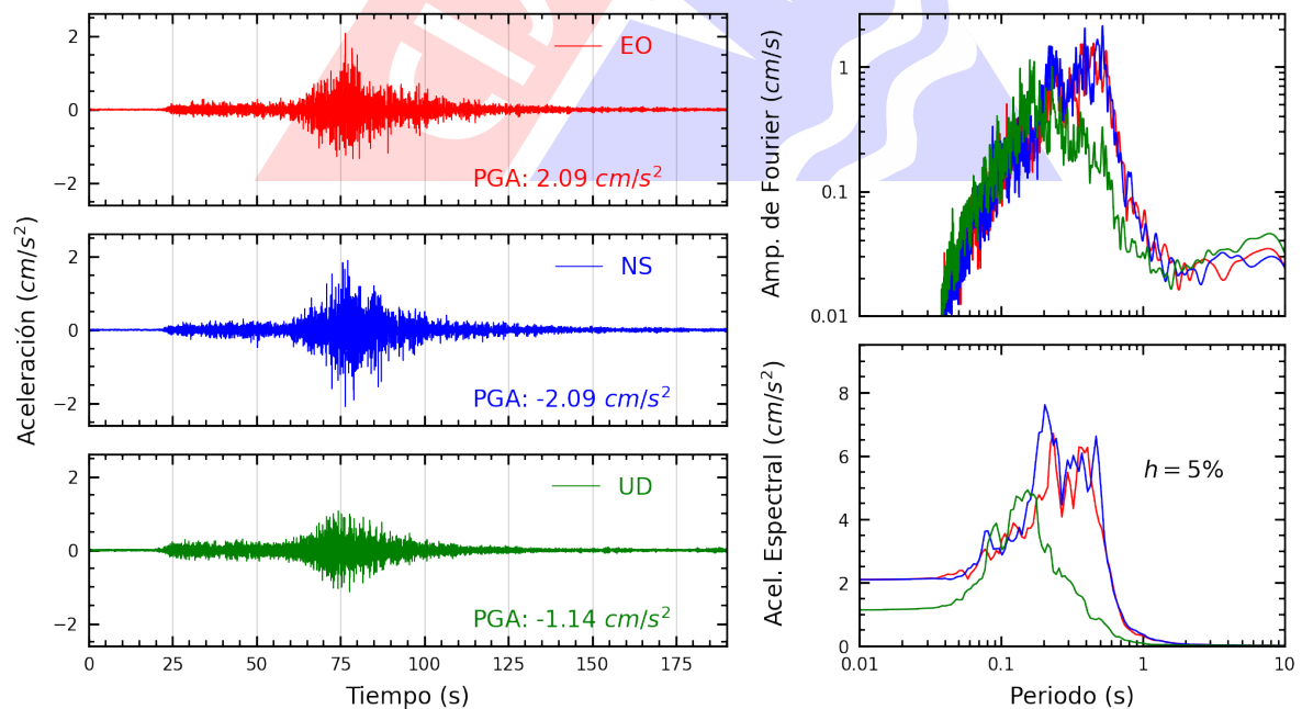
Figura A.4: Registros tiempo-historia, espectros de Fourier y de respuesta en las direcciones EO, NS y vertical de la estación MDPP. Sismo de Palpa, Palpa - Ica del 2024-11-07, 01:24:37 (Hora local)
