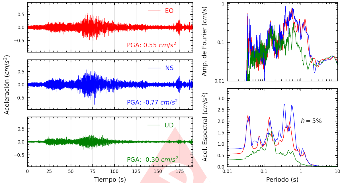
Figura A.19: Registros tiempo-historia, espectros de Fourier y de respuesta en las direcciones EO, NS y vertical de la estación DHNPE. Sismo de Palpa, Palpa - Ica del 2024-11-07, 01:24:37 (Hora local)
