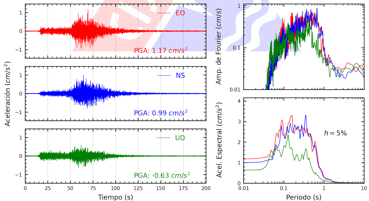
Figura A.14: Registros tiempo-historia, espectros de Fourier y de respuesta en las direcciones EO, NS y vertical de la estación USILP. Sismo de Palpa, Palpa - Ica del 2024-11-07, 01:24:37 (Hora local)
