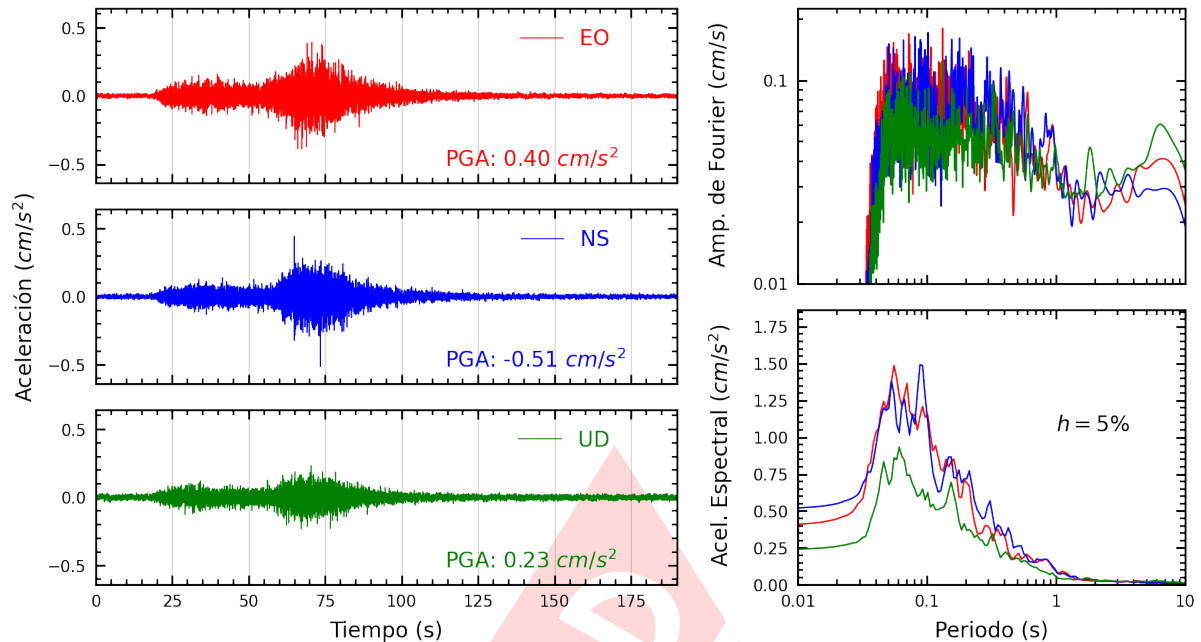
Figura A.37: Registros tiempo-historia, espectros de Fourier y de respuesta en las direcciones EO, NS y vertical de la estación UCSS. Sismo de Palpa, Palpa - Ica del 2024-11-07, 01:24:37 (Hora local)
