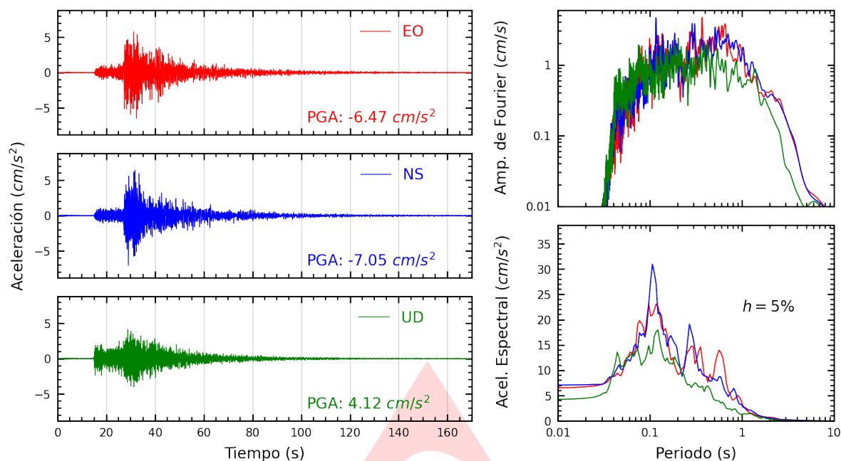
Figura A.1: Registros tiempo-historia, espectros de Fourier y de respuesta en las direcciones EO, NS y vertical de la estación UNICA. Sismo de Palpa, Palpa - Ica del 2024-11-07, 01:24:37 (Hora local)
