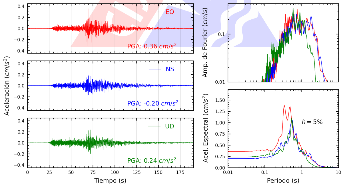
Figura A.38: Registros tiempo-historia, espectros de Fourier y de respuesta en las direcciones EO, NS y vertical de la estación UNCP. Sismo de Palpa, Palpa - Ica del 2024-11-07, 01:24:37 (Hora local)
