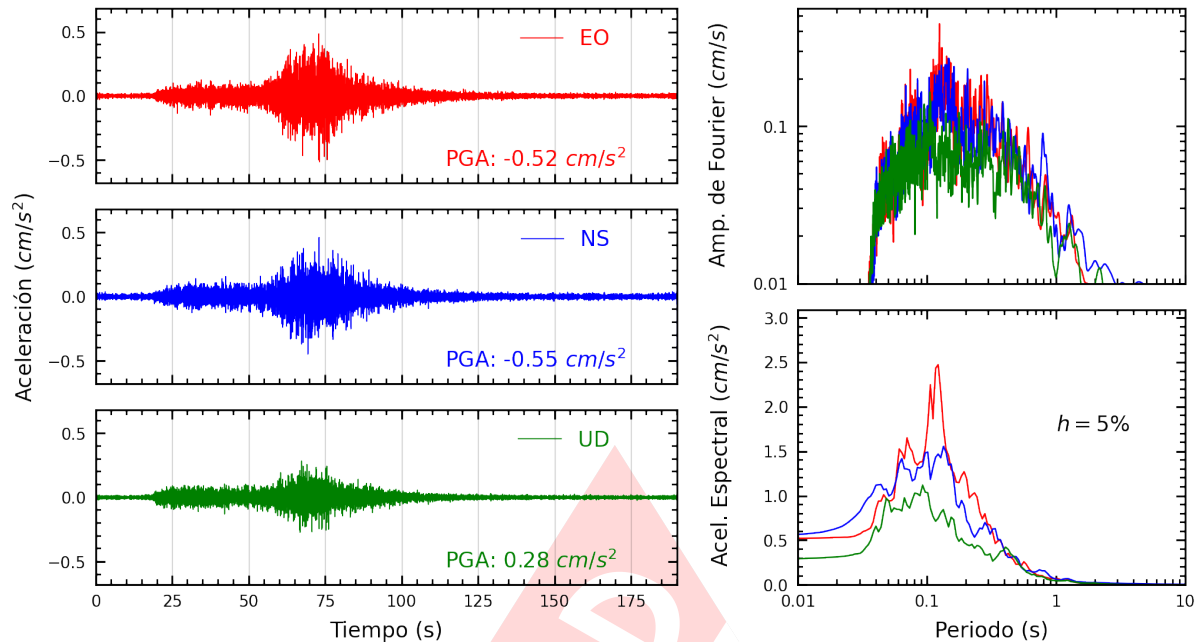
Figura A.31: Registros tiempo-historia, espectros de Fourier y de respuesta en las direcciones EO, NS y vertical de la estación ATARJ. Sismo de Palpa, Palpa - Ica del 2024-11-07, 01:24:37 (Hora local)
