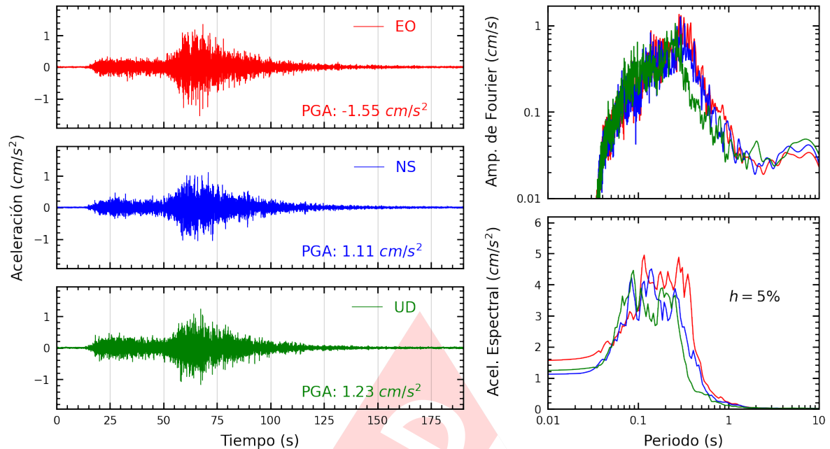
Figura A.9: Registros tiempo-historia, espectros de Fourier y de respuesta en las direcciones EO, NS y vertical de la estación SOVES. Sismo de Palpa, Palpa - Ica del 2024-11-07, 01:24:37 (Hora local)
