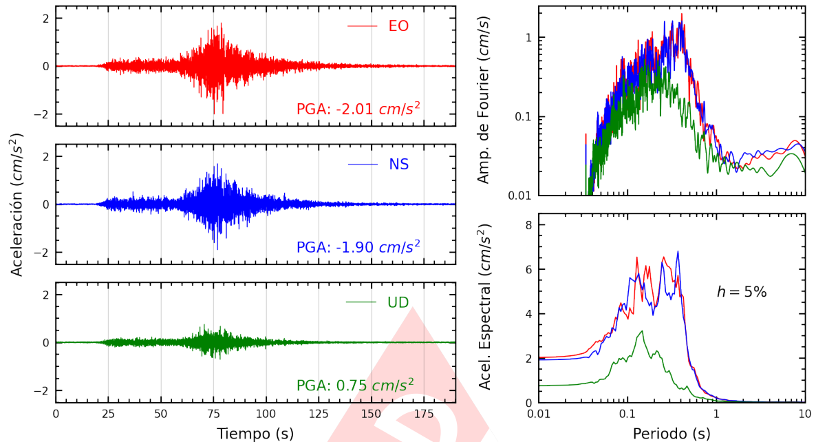
Figura A.5: Registros tiempo-historia, espectros de Fourier y de respuesta en las direcciones EO, NS y vertical de la estación DEFEN. Sismo de Palpa, Palpa - Ica del 2024-11-07, 01:24:37 (Hora local)
