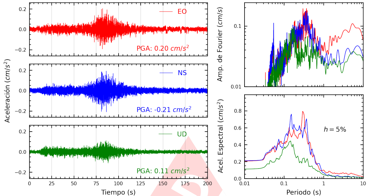
Figura A.43: Registros tiempo-historia, espectros de Fourier y de respuesta en las direcciones EO, NS y vertical de la estación UNAB. Sismo de Palpa, Palpa - Ica del 2024-11-07, 01:24:37 (Hora local)
