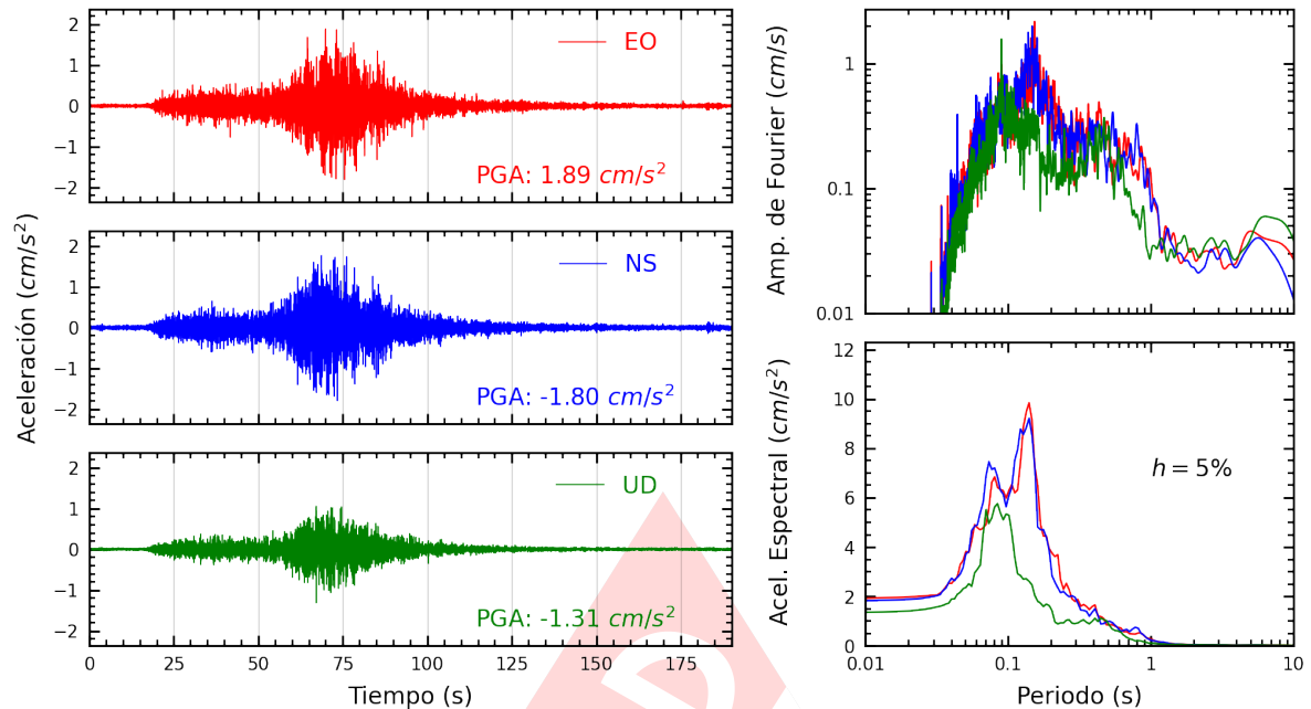
Figura A.7: Registros tiempo-historia, espectros de Fourier y de respuesta en las direcciones EO, NS y vertical de la estación USILM. Sismo de Palpa, Palpa - Ica del 2024-11-07, 01:24:37 (Hora local)
