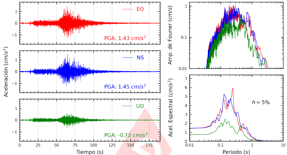
Figura A.11: Registros tiempo-historia, espectros de Fourier y de respuesta en las direcciones EO, NS y vertical de la estación BRISA. Sismo de Palpa, Palpa - Ica del 2024-11-07, 01:24:37 (Hora local)
