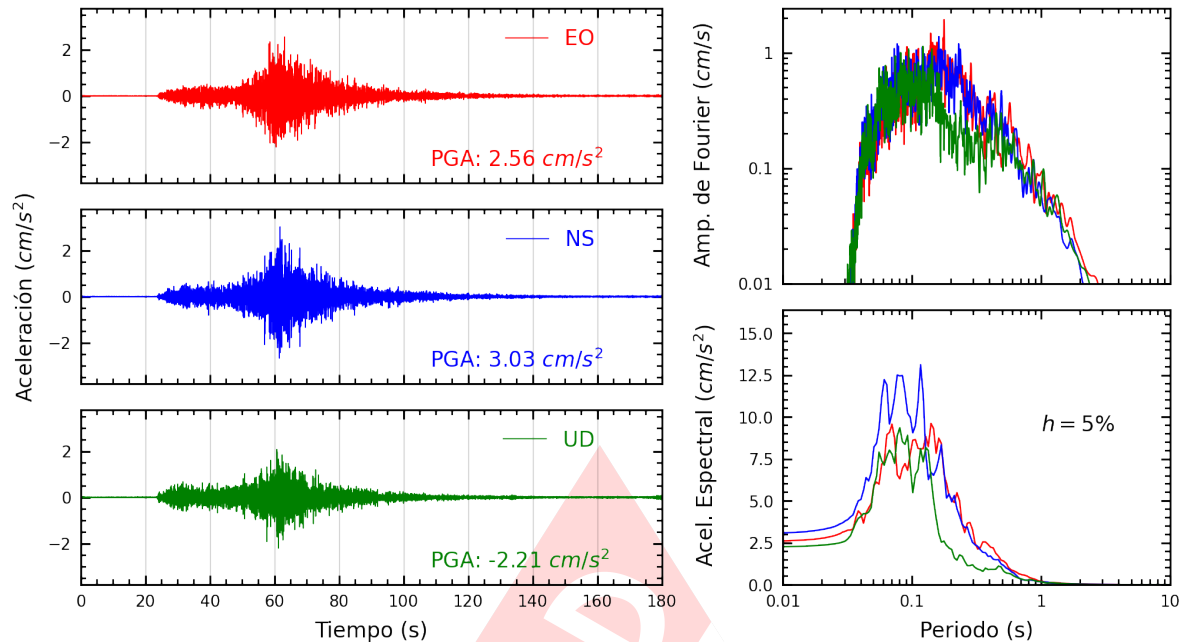
Figura A.3: Registros tiempo-historia, espectros de Fourier y de respuesta en las direcciones EO, NS y vertical de la estación ASIA. Sismo de Palpa, Palpa - Ica del 2024-11-07, 01:24:37 (Hora local)
