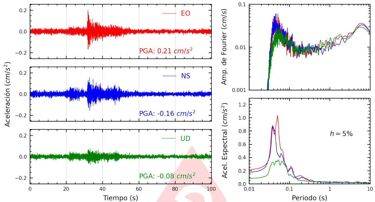
Figura A.13: Registros tiempo-historia, espectros de Fourier y de respuesta en las direcciones EO, NS y vertical de la estación COMAS. Sismo de Chilca, Cañete - Lima del 2024-11-07, 04:57:37 (Hora local)
