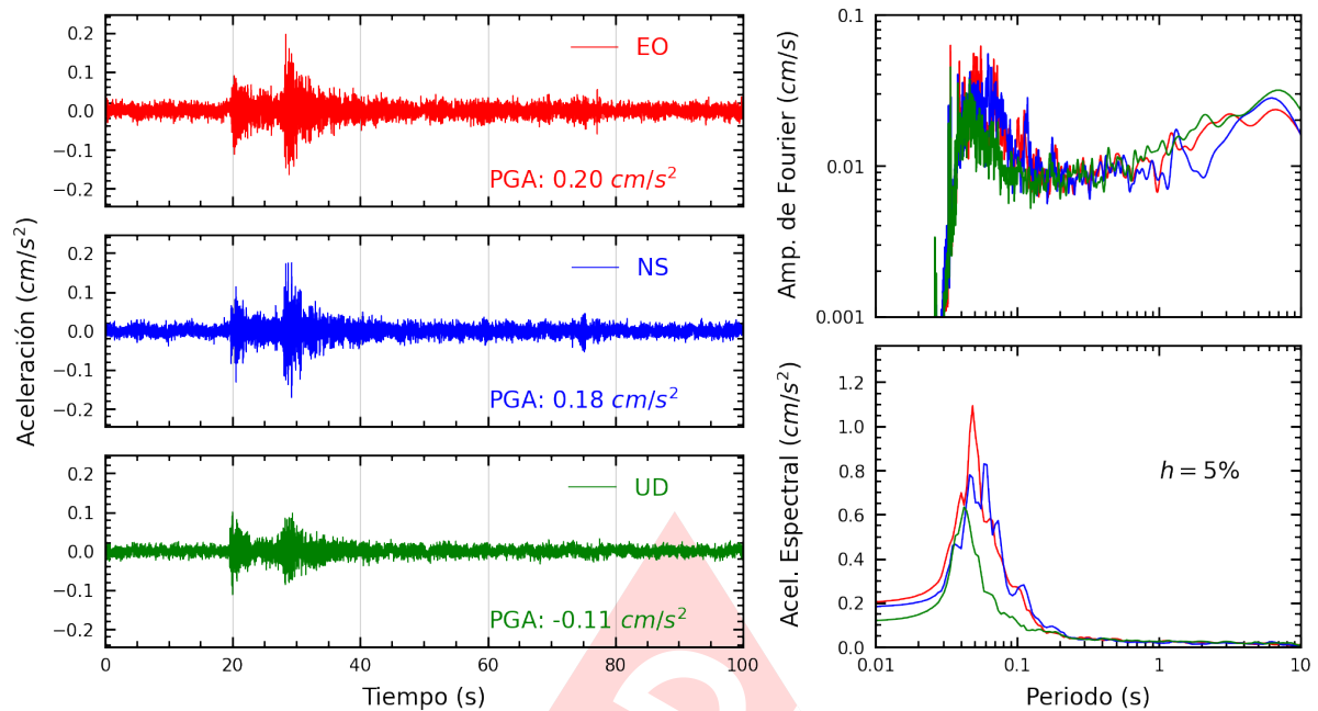
Figura A.15: Registros tiempo-historia, espectros de Fourier y de respuesta en las direcciones EO, NS y vertical de la estación UPCVI. Sismo de Chilca, Cañete - Lima del 2024-11-07, 04:57:37 (Hora local)
