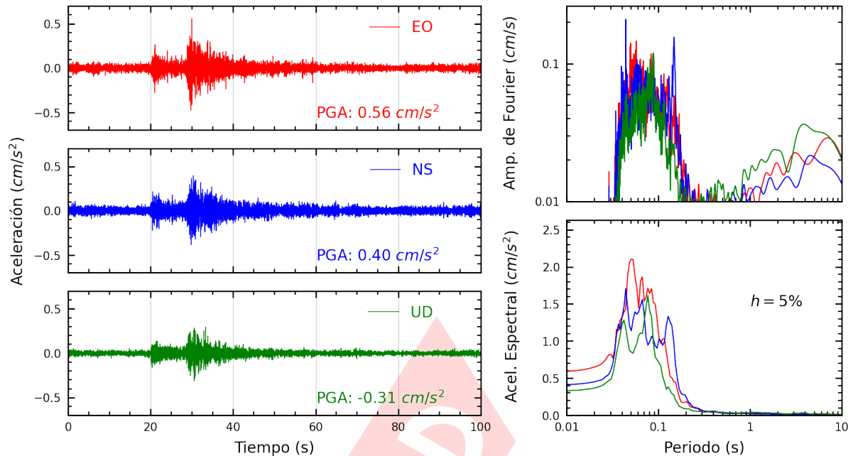
Figura A.3: Registros tiempo-historia, espectros de Fourier y de respuesta en las direcciones EO, NS y vertical de la estación USILM. Sismo de Chilca, Cañete - Lima del 2024-11-07, 04:57:37 (Hora local)
