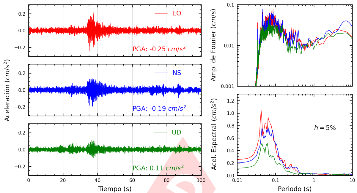
Figura A.9: Registros tiempo-historia, espectros de Fourier y de respuesta en las direcciones EO, NS y vertical de la estación DEFEN. Sismo de Chilca, Cañete - Lima del 2024-11-07, 04:57:37 (Hora local)
