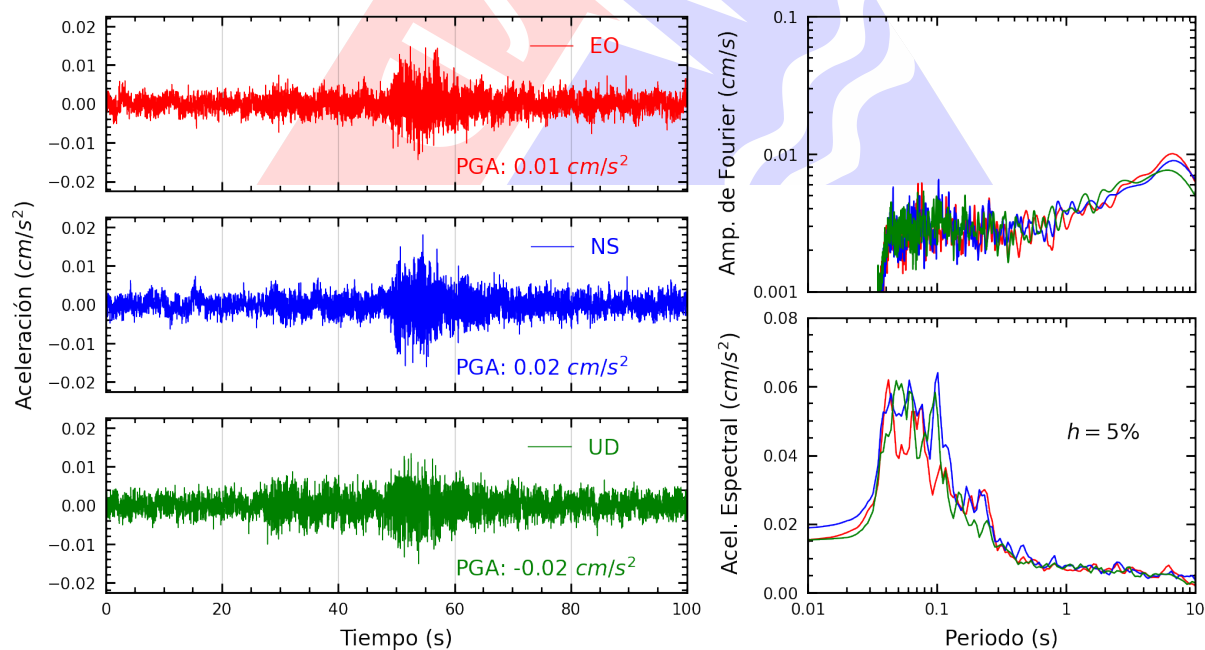
Figura A.22: Registros tiempo-historia, espectros de Fourier y de respuesta en las direcciones EO, NS y vertical de la estación CARAL. Sismo de Chilca, Cañete - Lima del 2024-11-07, 04:57:37 (Hora local)
