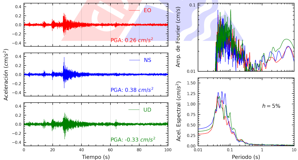
Figura A.6: Registros tiempo-historia, espectros de Fourier y de respuesta en las direcciones EO, NS y vertical de la estación SOVES. Sismo de Chilca, Cañete - Lima del 2024-11-07, 04:57:37 (Hora local)
