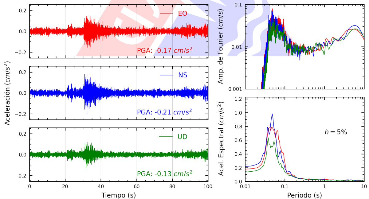
Figura A.12: Registros tiempo-historia, espectros de Fourier y de respuesta en las direcciones EO, NS y vertical de la estación FICPE. Sismo de Chilca, Cañete - Lima del 2024-11-07, 04:57:37 (Hora local)
