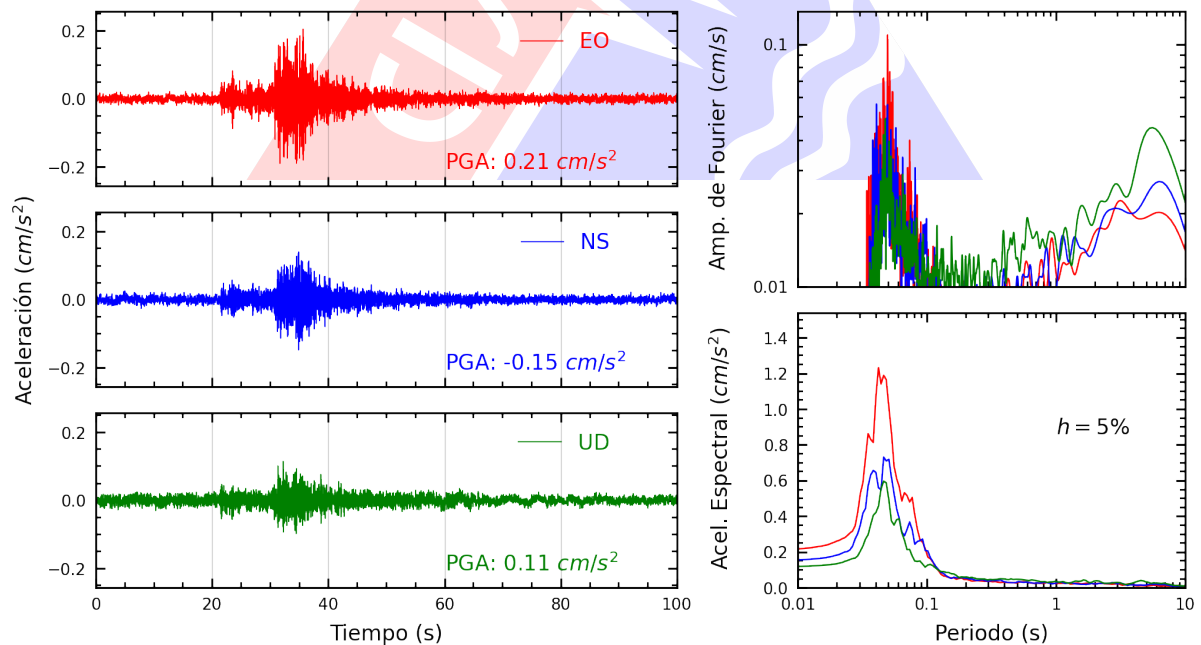
Figura A.14: Registros tiempo-historia, espectros de Fourier y de respuesta en las direcciones EO, NS y vertical de la estación UCSS. Sismo de Chilca, Cañete - Lima del 2024-11-07, 04:57:37 (Hora local)
