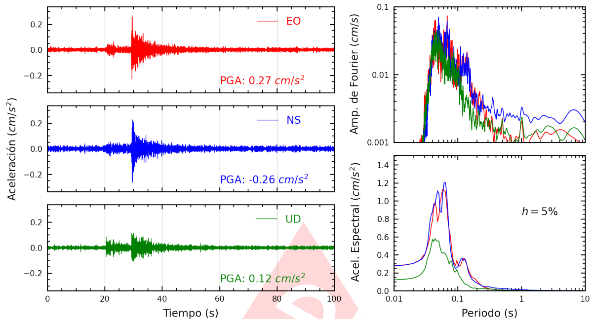
Figura A.7: Registros tiempo-historia, espectros de Fourier y de respuesta en las direcciones EO, NS y vertical de la estación ATARJ. Sismo de Chilca, Cañete - Lima del 2024-11-07, 04:57:37 (Hora local)
