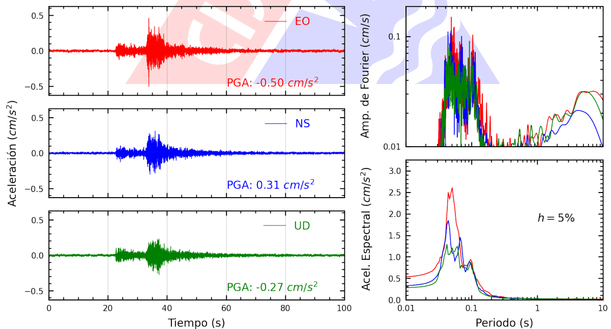
Figura A.4: Registros tiempo-historia, espectros de Fourier y de respuesta en las direcciones EO, NS y vertical de la estación AMORE. Sismo de Chilca, Cañete - Lima del 2024-11-07, 04:57:37 (Hora local)
