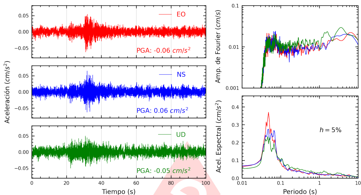
Figura A.21: Registros tiempo-historia, espectros de Fourier y de respuesta en las direcciones EO, NS y vertical de la estación UNFV. Sismo de Chilca, Cañete - Lima del 2024-11-07, 04:57:37 (Hora local)
