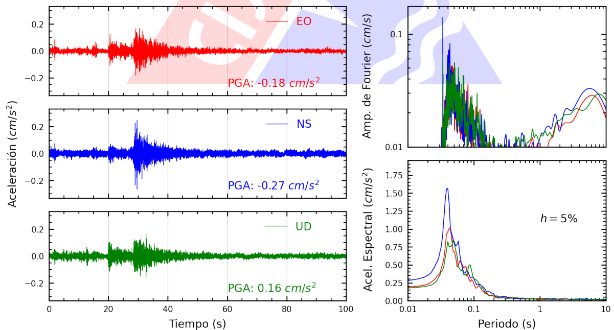
Figura A.8: Registros tiempo-historia, espectros de Fourier y de respuesta en las direcciones EO, NS y vertical de la estación USMP. Sismo de Chilca, Cañete - Lima del 2024-11-07, 04:57:37 (Hora local)
