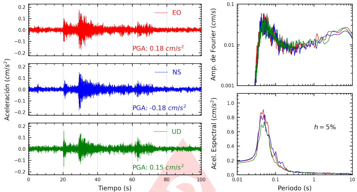
Figura A.17: Registros tiempo-historia, espectros de Fourier y de respuesta en las direcciones EO, NS y vertical de la estación IMCA. Sismo de Chilca, Cañete - Lima del 2024-11-07, 04:57:37 (Hora local)
