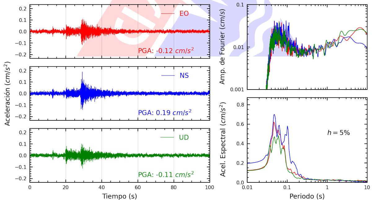
Figura A.16: Registros tiempo-historia, espectros de Fourier y de respuesta en las direcciones EO, NS y vertical de la estación SERVI. Sismo de Chilca, Cañete - Lima del 2024-11-07, 04:57:37 (Hora local)
