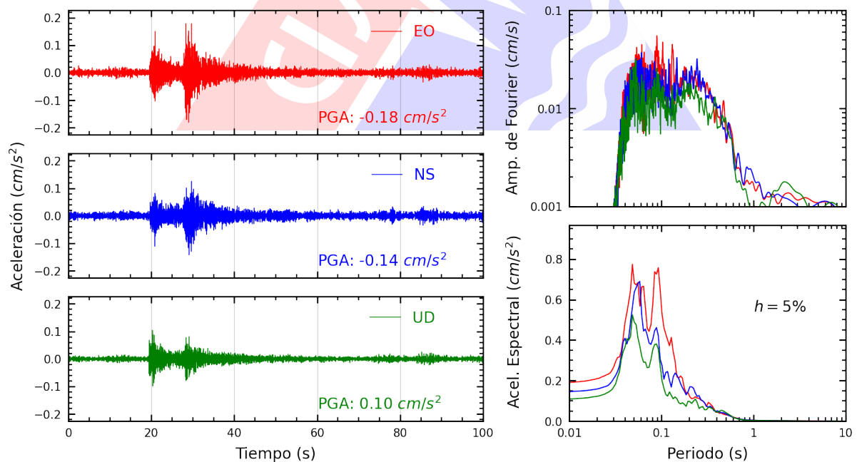
Figura A.18: Registros tiempo-historia, espectros de Fourier y de respuesta en las direcciones EO, NS y vertical de la estación BRISA. Sismo de Chilca, Cañete - Lima del 2024-11-07, 04:57:37 (Hora local)
