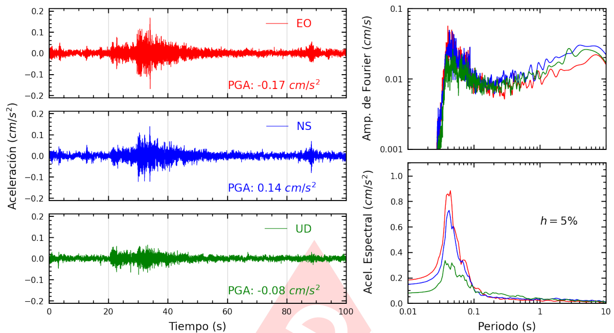
Figura A.19: Registros tiempo-historia, espectros de Fourier y de respuesta en las direcciones EO, NS y vertical de la estación CEPRE. Sismo de Chilca, Cañete - Lima del 2024-11-07, 04:57:37 (Hora local)
