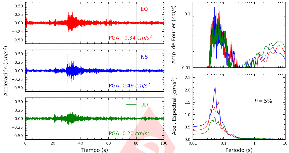
Figura A.5: Registros tiempo-historia, espectros de Fourier y de respuesta en las direcciones EO, NS y vertical de la estación INDEP. Sismo de Chilca, Cañete - Lima del 2024-11-07, 04:57:37 (Hora local)
