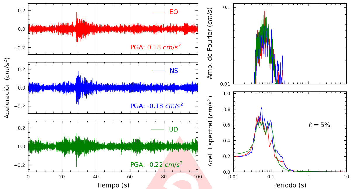
Figura A.11: Registros tiempo-historia, espectros de Fourier y de respuesta en las direcciones EO, NS y vertical de la estación ASIA. Sismo de Chilca, Cañete - Lima del 2024-11-07, 04:57:37 (Hora local)
