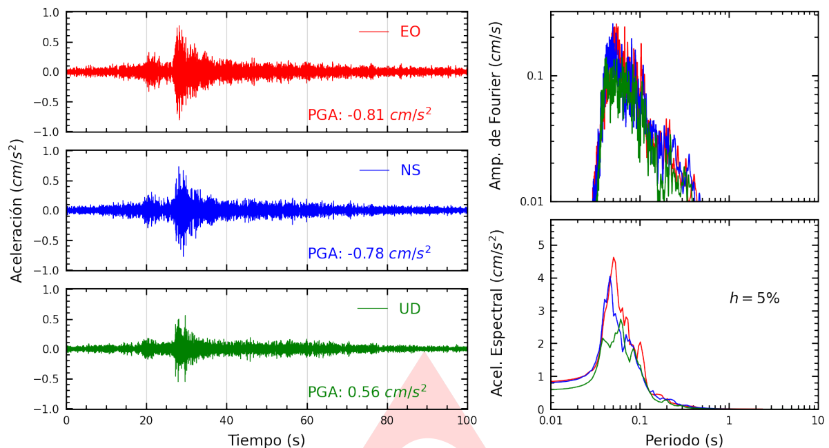
Figura A.1: Registros tiempo-historia, espectros de Fourier y de respuesta en las direcciones EO, NS y vertical de la estación UNTEL. Sismo de Chilca, Cañete - Lima del 2024-11-07, 04:57:37 (Hora local)
