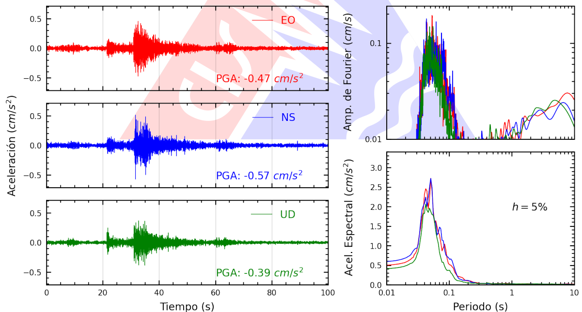
Figura A.2: Registros tiempo-historia, espectros de Fourier y de respuesta en las direcciones EO, NS y vertical de la estación JOSEO. Sismo de Chilca, Cañete - Lima del 2024-11-07, 04:57:37 (Hora local)
