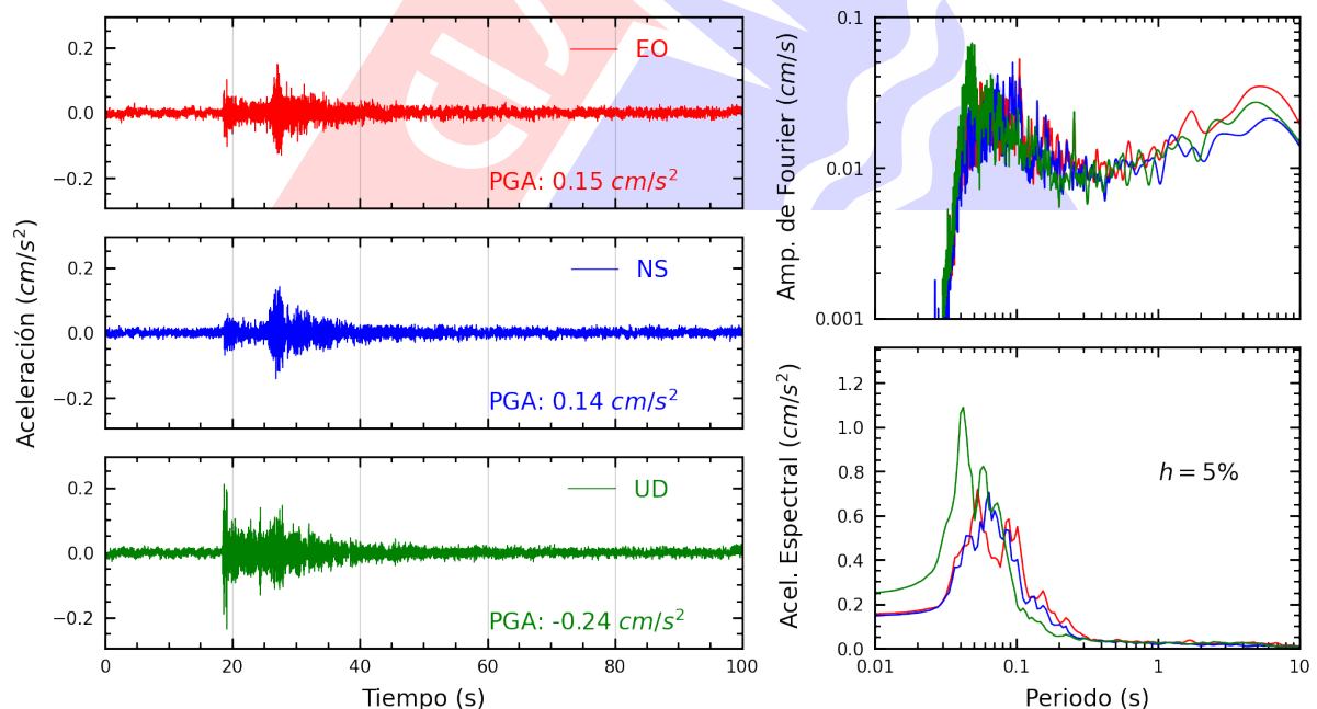
Figura A.10: Registros tiempo-historia, espectros de Fourier y de respuesta en las direcciones EO, NS y vertical de la estación USILP. Sismo de Chilca, Cañete - Lima del 2024-11-07, 04:57:37 (Hora local)
