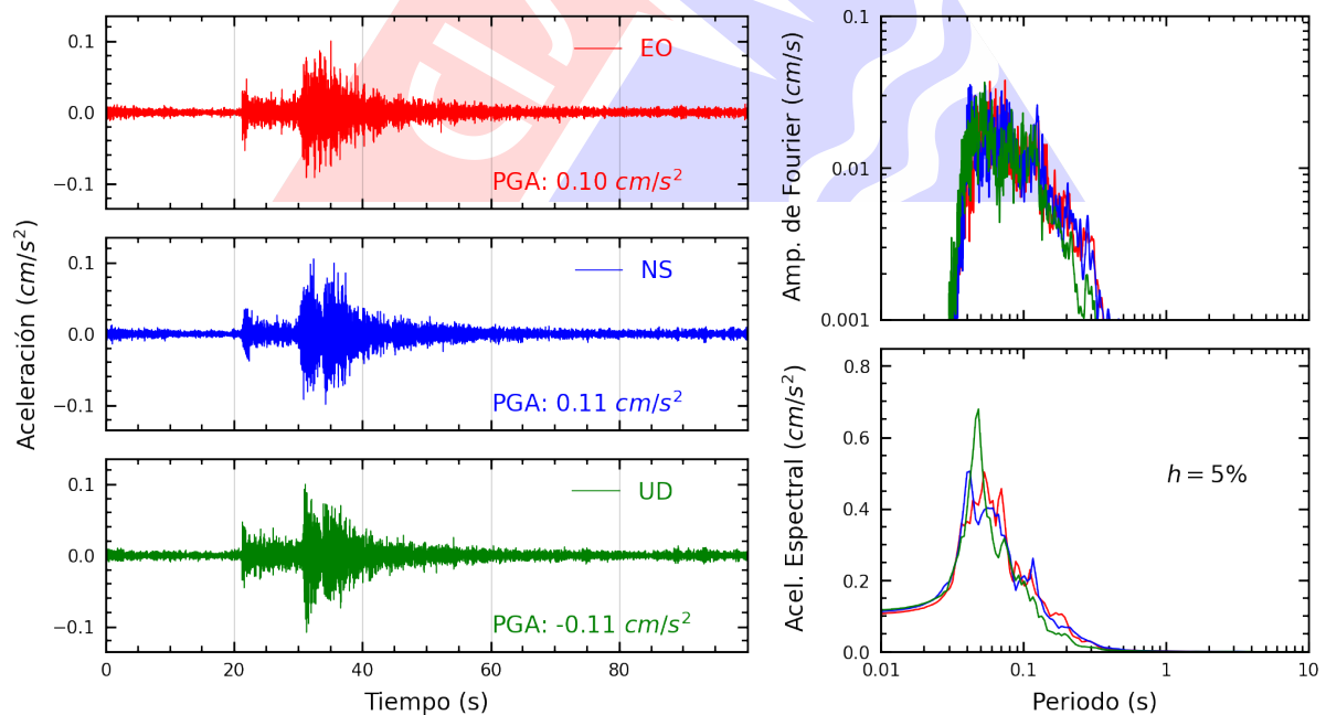
Figura A.20: Registros tiempo-historia, espectros de Fourier y de respuesta en las direcciones EO, NS y vertical de la estación JALV2. Sismo de Chilca, Cañete - Lima del 2024-11-07, 04:57:37 (Hora local)
