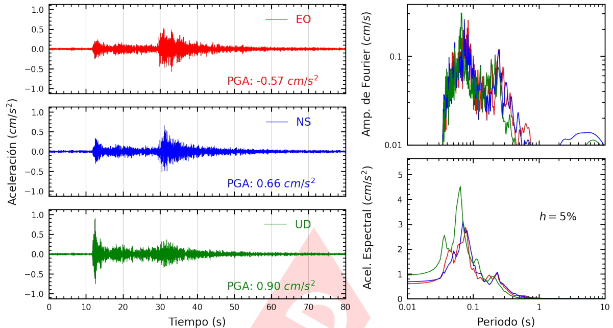
Figura A.3: Registros tiempo-historia, espectros de Fourier y de respuesta en las direcciones EO, NS y vertical de la estación CREY. Sismo de Tarata, Tarata - Tacna del 2024-11-07, 16:36:11 (Hora local)
