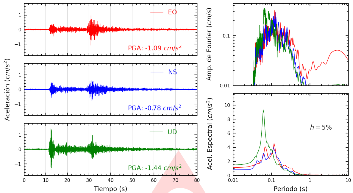
Figura A.1: Registros tiempo-historia, espectros de Fourier y de respuesta en las direcciones EO, NS y vertical de la estación UJBG3. Sismo de Tarata, Tarata - Tacna del 2024-11-07, 16:36:11 (Hora local)
