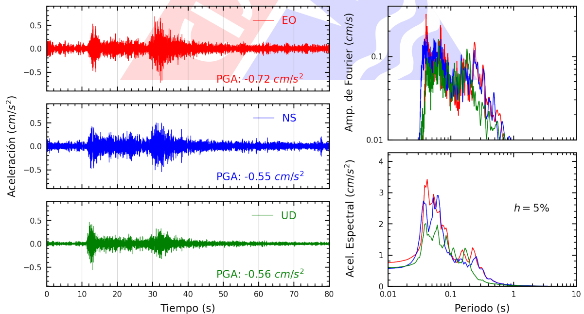
Figura A.4: Registros tiempo-historia, espectros de Fourier y de respuesta en las direcciones EO, NS y vertical de la estación UPTAC. Sismo de Tarata, Tarata - Tacna del 2024-11-07, 16:36:11 (Hora local)
