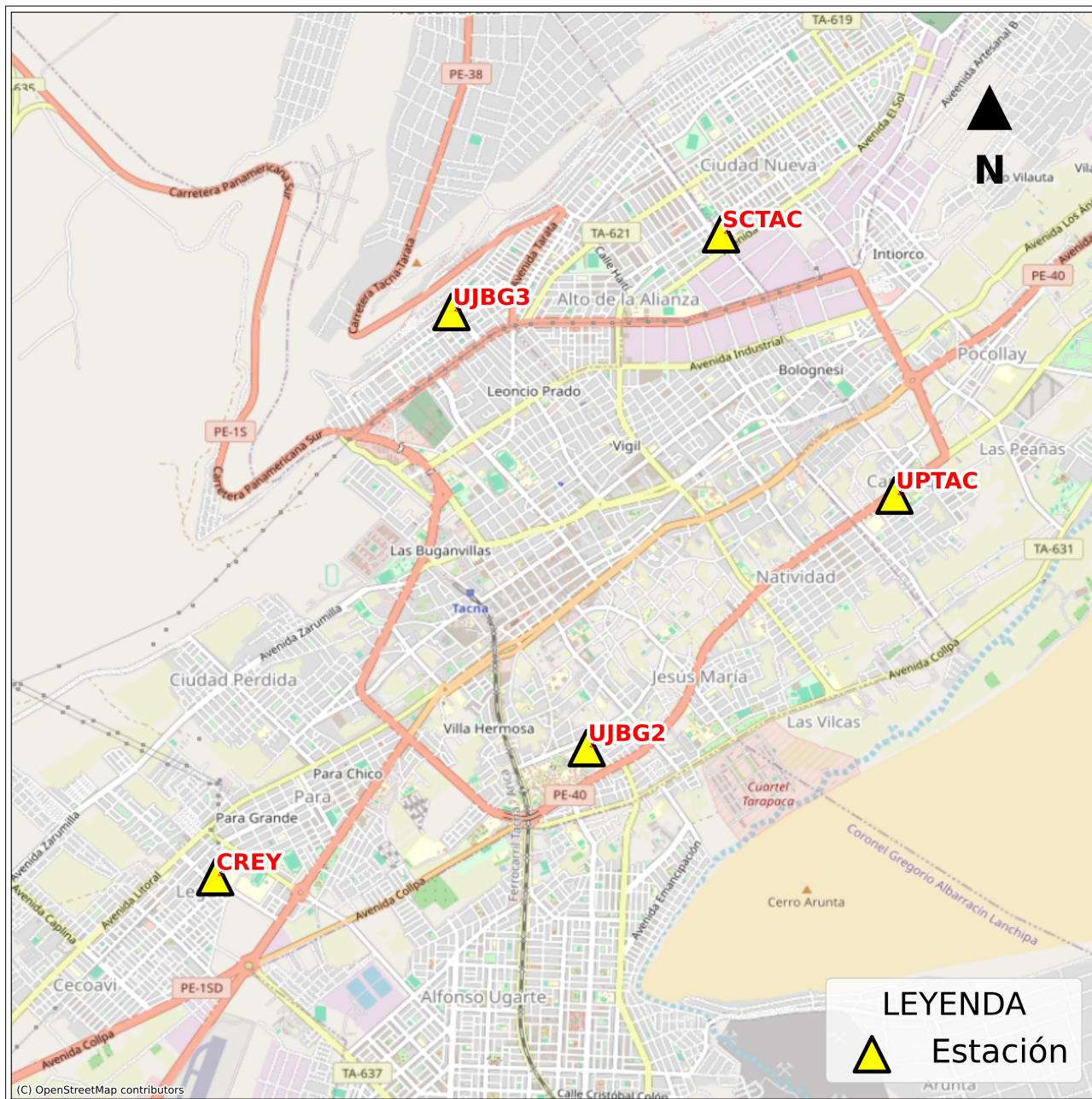
Figura 2: Mapa de ubicación de la(s) estación(es) acelerográfica(s) correspondiente(s) al Sismo de Tarata, Tarata - Tacna del 07 de noviembre de 2024 a las 16:36:11 (hora local)
