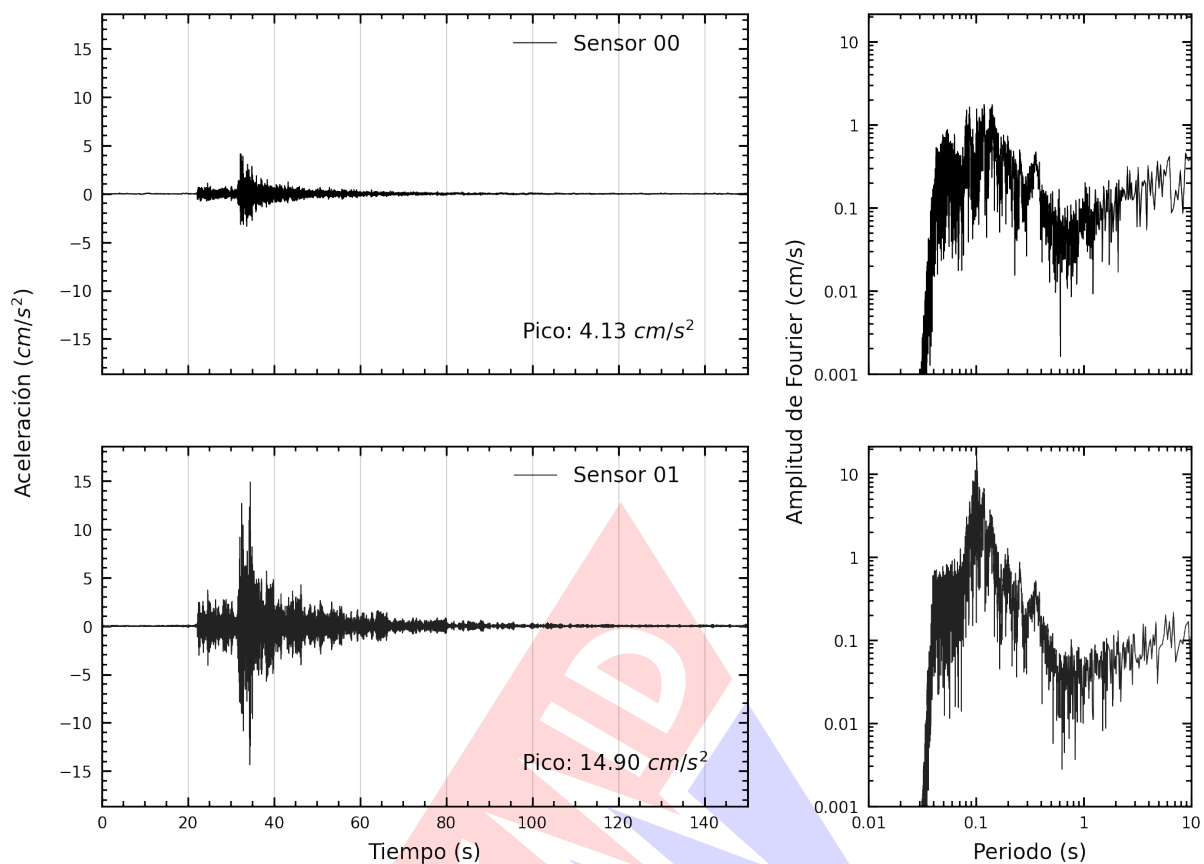
Figura A.1: Registros tiempo-historia y espectros de Fourier en la dirección EW de la edificación Laboratorio de Estructuras del CISMID-FIC-UNI. Sismo de Ancon, Lima - Lima del 2024-11-08, 20:17:18 (Hora local)
