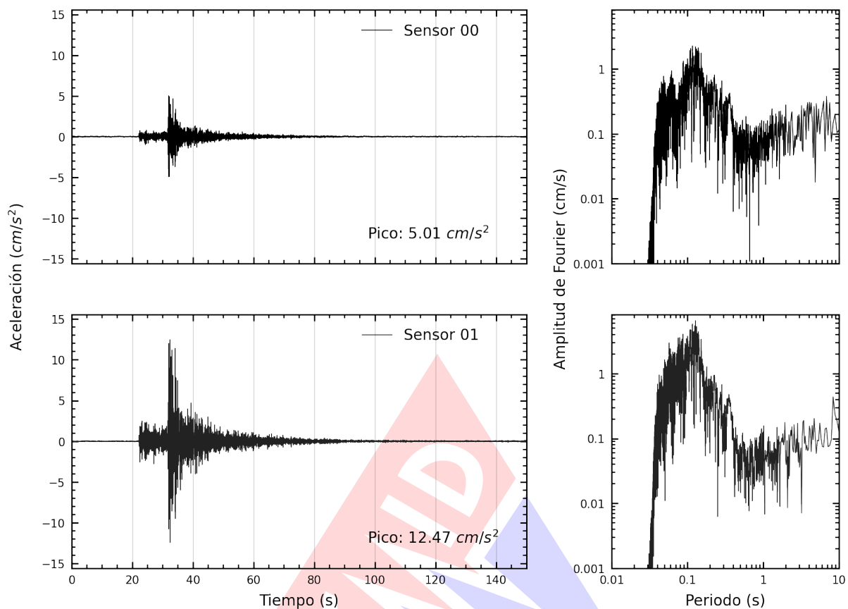
Figura A.2: Registros tiempo-historia y espectros de Fourier en la dirección NS de la edificación Laboratorio de Estructuras del CISMID-FIC-UNI. Sismo de Ancon, Lima - Lima del 2024-11-08, 20:17:18 (Hora local)
