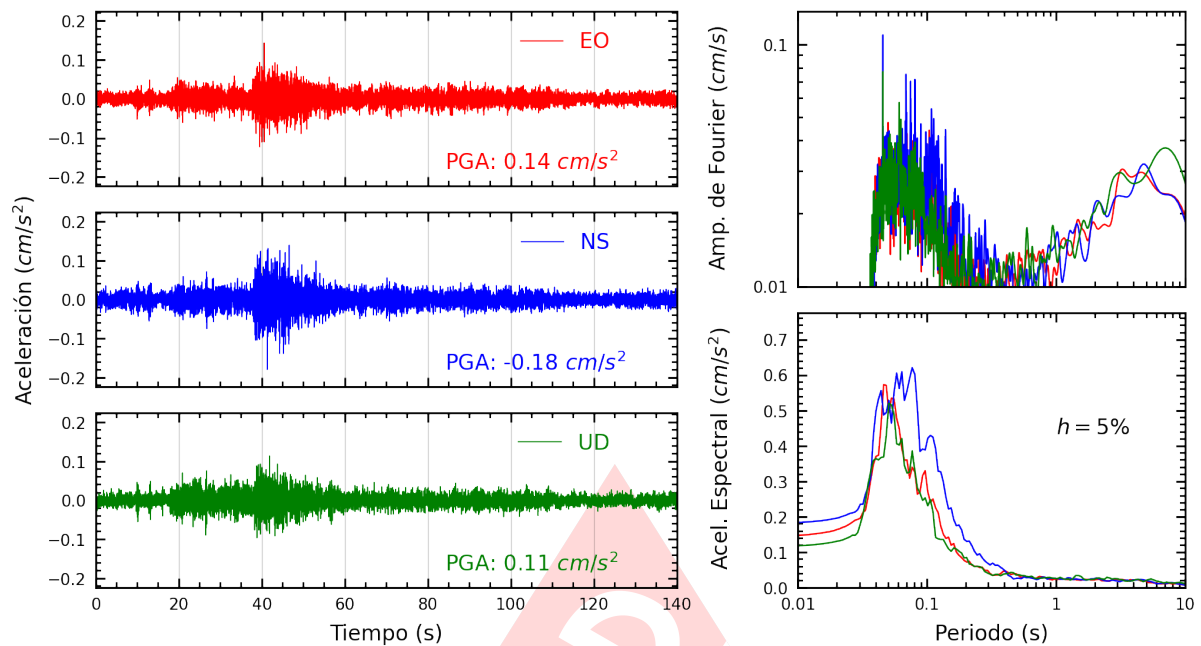
Figura A.17: Registros tiempo-historia, espectros de Fourier y de respuesta en las direcciones EO, NS y vertical de la estación SERVI. Sismo de Yauyos, Yauyos - Lima del 2024-11-10, 16:10:00 (Hora local)
