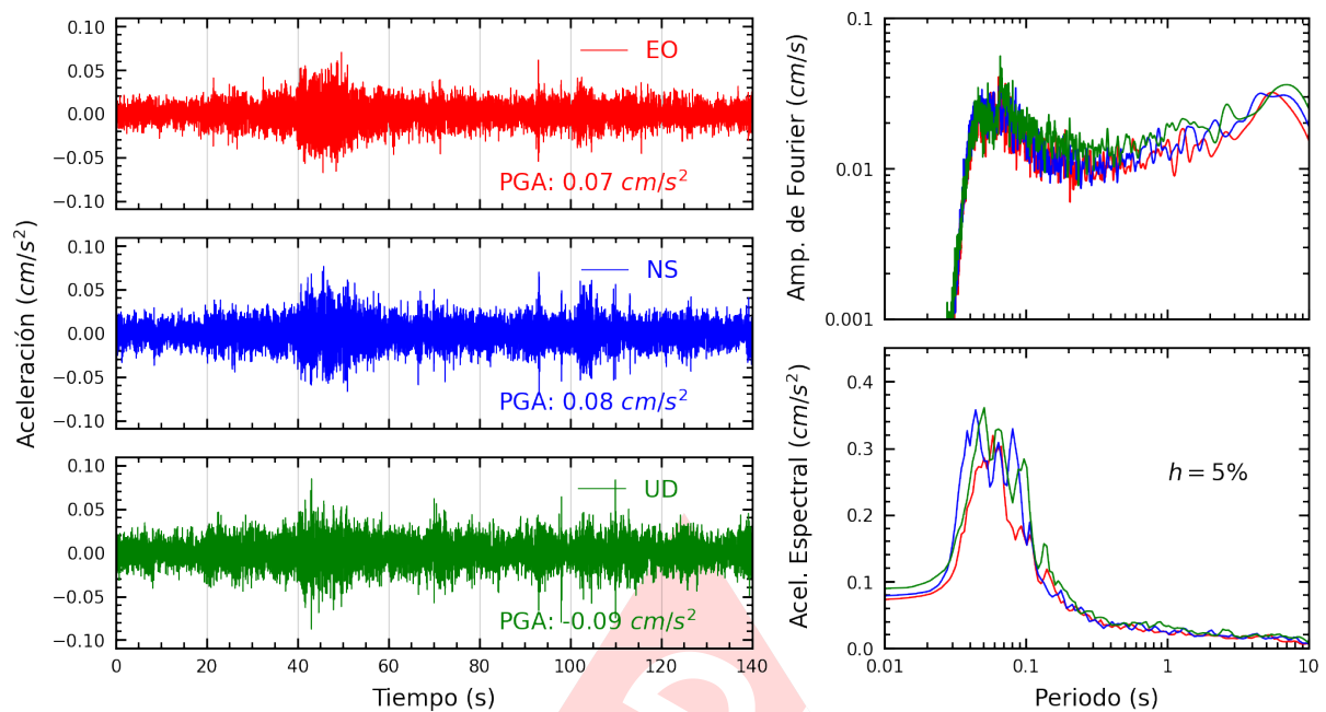
Figura A.25: Registros tiempo-historia, espectros de Fourier y de respuesta en las direcciones EO, NS y vertical de la estación UNFV. Sismo de Yauyos, Yauyos - Lima del 2024-11-10, 16:10:00 (Hora local)
