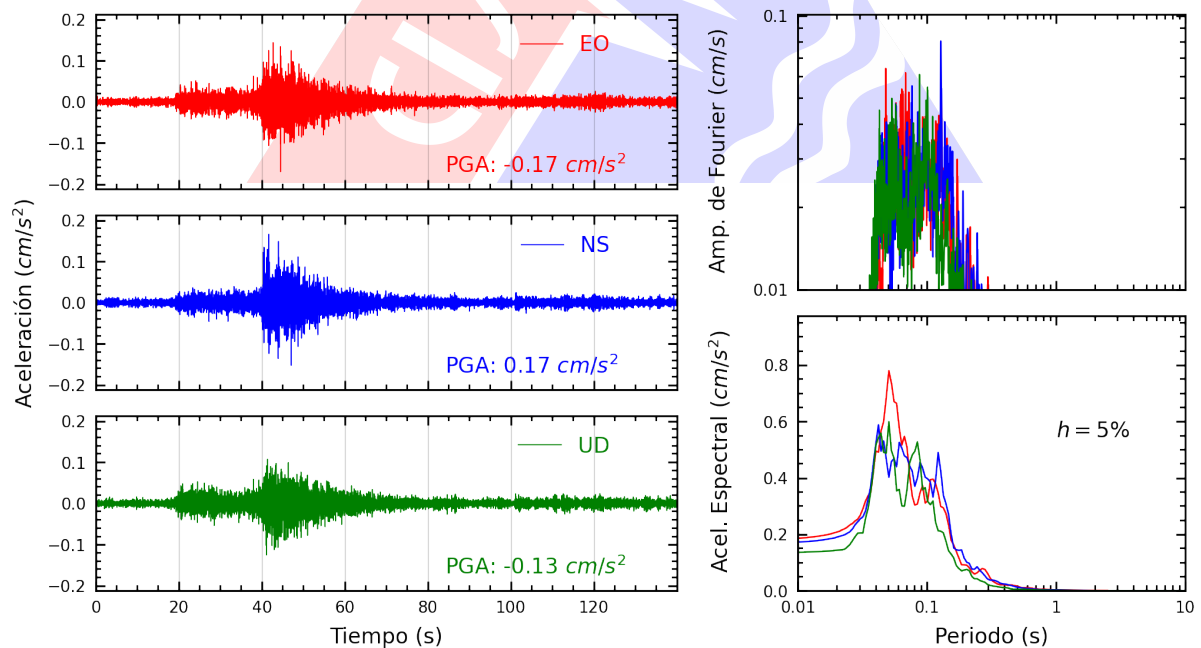
Figura A.20: Registros tiempo-historia, espectros de Fourier y de respuesta en las direcciones EO, NS y vertical de la estación JALV2. Sismo de Yauyos, Yauyos - Lima del 2024-11-10, 16:10:00 (Hora local)
