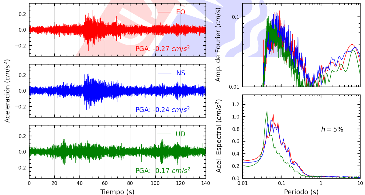
Figura A.10: Registros tiempo-historia, espectros de Fourier y de respuesta en las direcciones EO, NS y vertical de la estación DEFEN. Sismo de Yauyos, Yauyos - Lima del 2024-11-10, 16:10:00 (Hora local)
