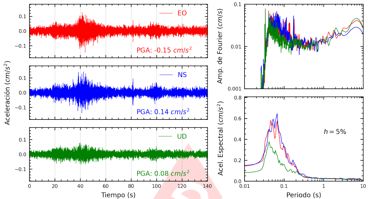
Figura A.23: Registros tiempo-historia, espectros de Fourier y de respuesta en las direcciones EO, NS y vertical de la estación UPCVI. Sismo de Yauyos, Yauyos - Lima del 2024-11-10, 16:10:00 (Hora local)
