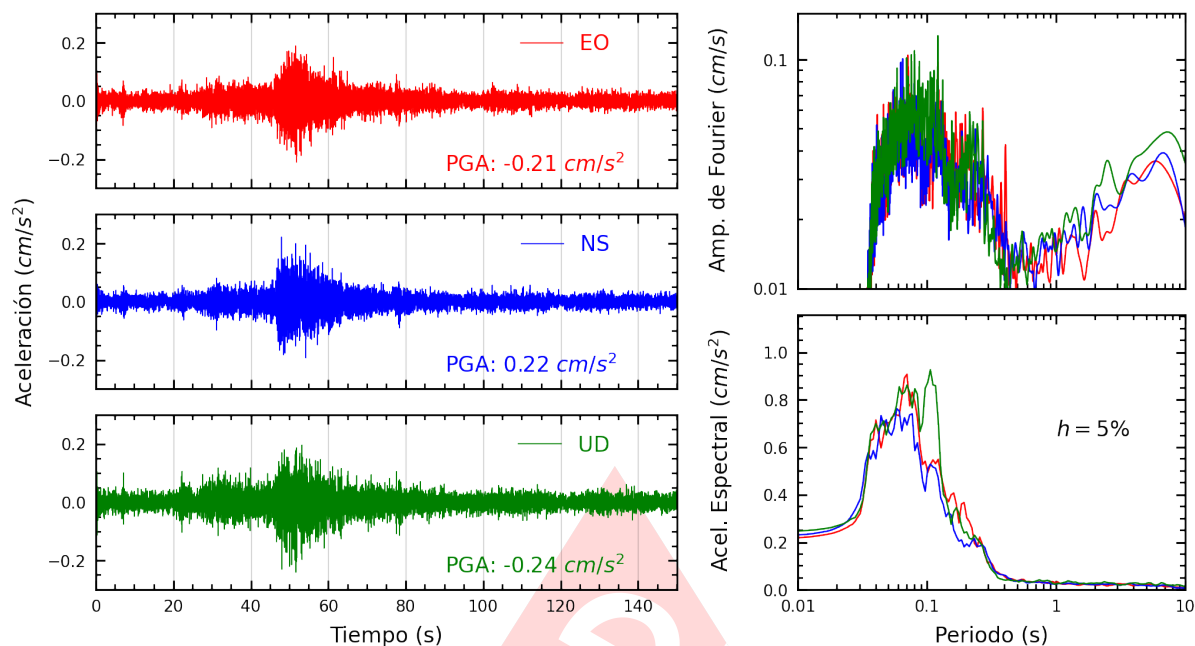
Figura A.11: Registros tiempo-historia, espectros de Fourier y de respuesta en las direcciones EO, NS y vertical de la estación SOVES. Sismo de Yauyos, Yauyos - Lima del 2024-11-10, 16:10:00 (Hora local)
