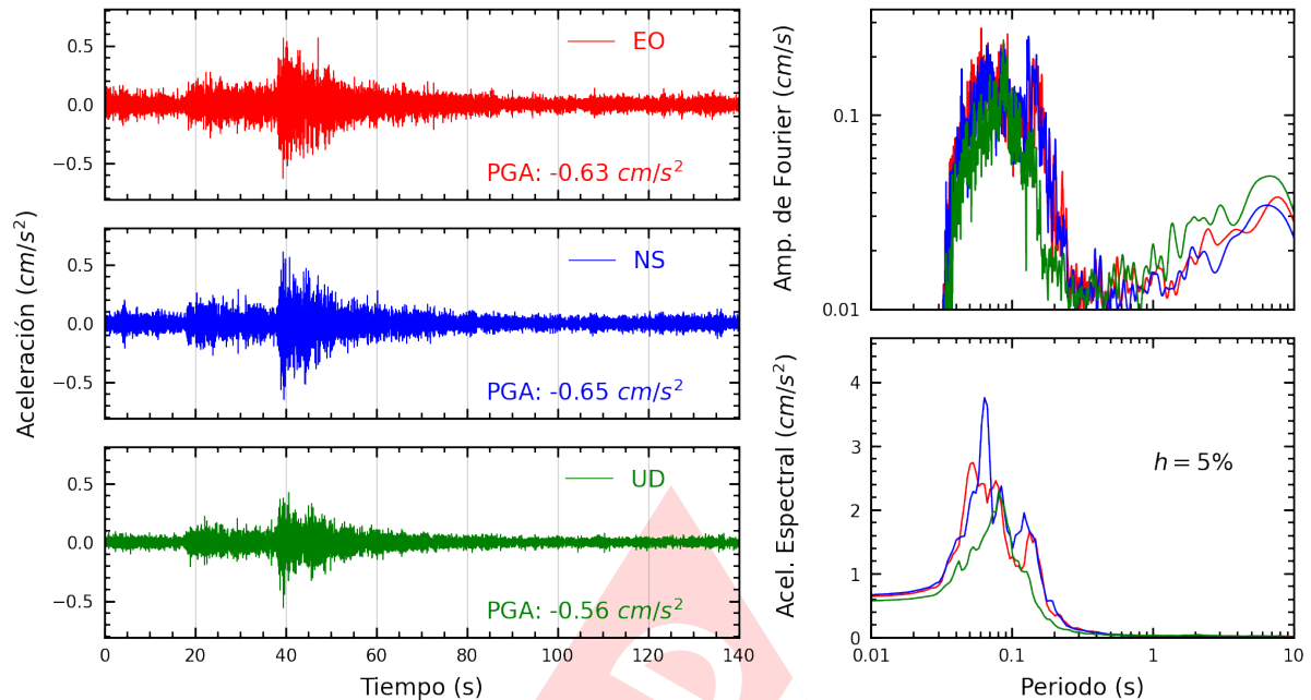
Figura A.3: Registros tiempo-historia, espectros de Fourier y de respuesta en las direcciones EO, NS y vertical de la estación USILM. Sismo de Yauyos, Yauyos - Lima del 2024-11-10, 16:10:00 (Hora local)
