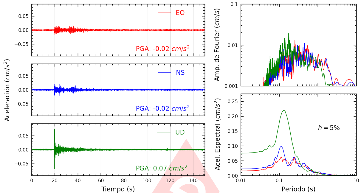
Figura A.27: Registros tiempo-historia, espectros de Fourier y de respuesta en las direcciones EO, NS y vertical de la estación UNCP. Sismo de Yauyos, Yauyos - Lima del 2024-11-10, 16:10:00 (Hora local)
