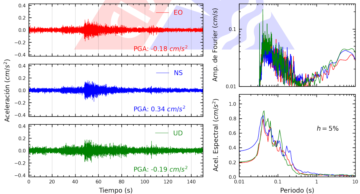
Figura A.8: Registros tiempo-historia, espectros de Fourier y de respuesta en las direcciones EO, NS y vertical de la estación USMP. Sismo de Yauyos, Yauyos - Lima del 2024-11-10, 16:10:00 (Hora local)
