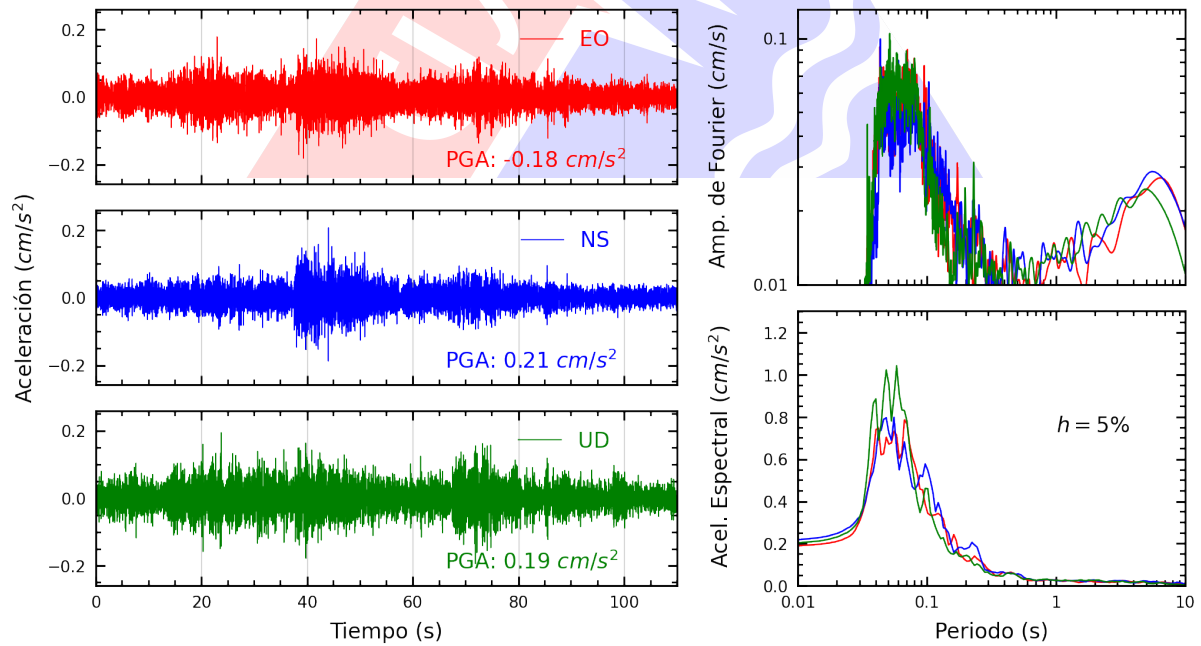
Figura A.14: Registros tiempo-historia, espectros de Fourier y de respuesta en las direcciones EO, NS y vertical de la estación URPE. Sismo de Yauyos, Yauyos - Lima del 2024-11-10, 16:10:00 (Hora local)
