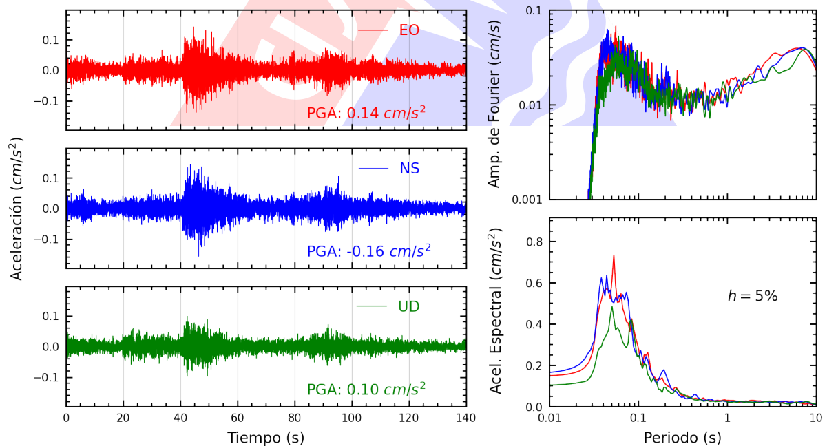
Figura A.22: Registros tiempo-historia, espectros de Fourier y de respuesta en las direcciones EO, NS y vertical de la estación COMAS. Sismo de Yauyos, Yauyos - Lima del 2024-11-10, 16:10:00 (Hora local)
