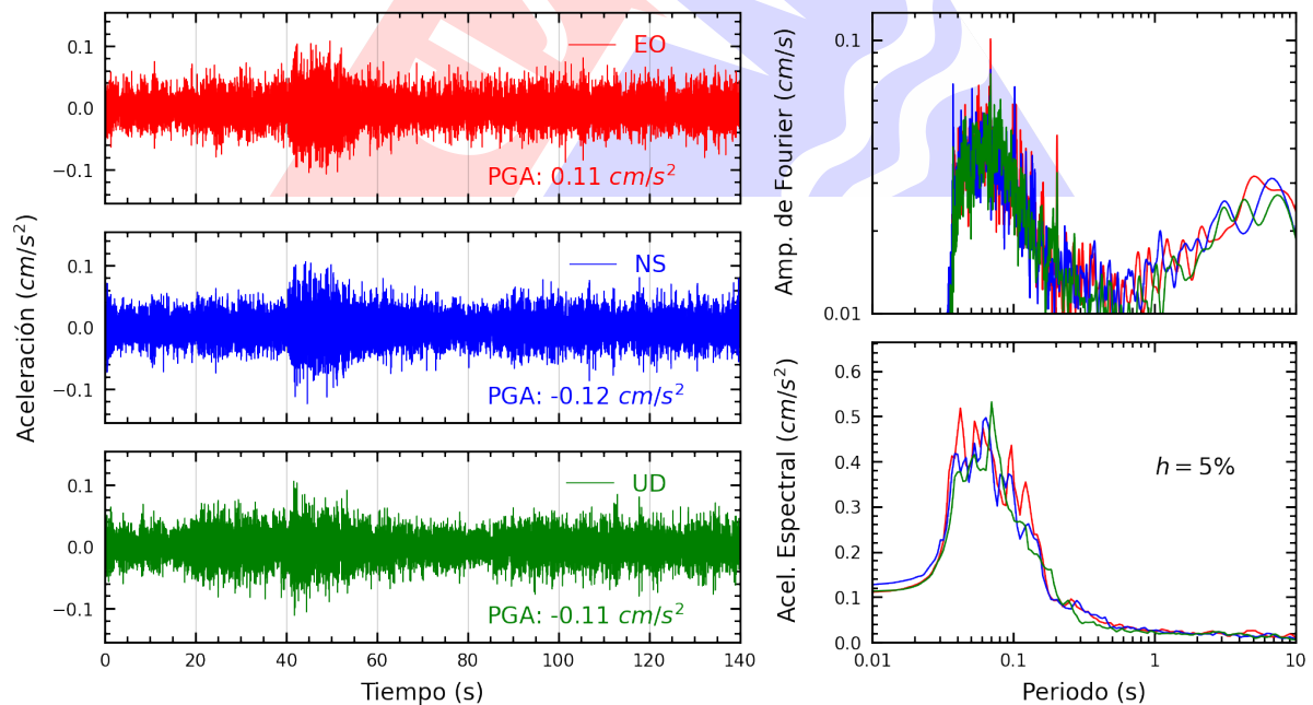
Figura A.24: Registros tiempo-historia, espectros de Fourier y de respuesta en las direcciones EO, NS y vertical de la estación MADRE. Sismo de Yauyos, Yauyos - Lima del 2024-11-10, 16:10:00 (Hora local)
