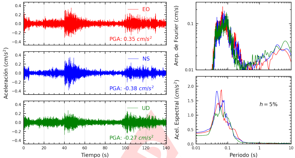
Figura A.7: Registros tiempo-historia, espectros de Fourier y de respuesta en las direcciones EO, NS y vertical de la estación INDEP. Sismo de Yauyos, Yauyos - Lima del 2024-11-10, 16:10:00 (Hora local)
