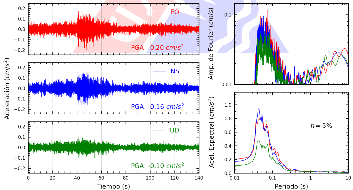
Figura A.16: Registros tiempo-historia, espectros de Fourier y de respuesta en las direcciones EO, NS y vertical de la estación FICPE. Sismo de Yauyos, Yauyos - Lima del 2024-11-10, 16:10:00 (Hora local)
