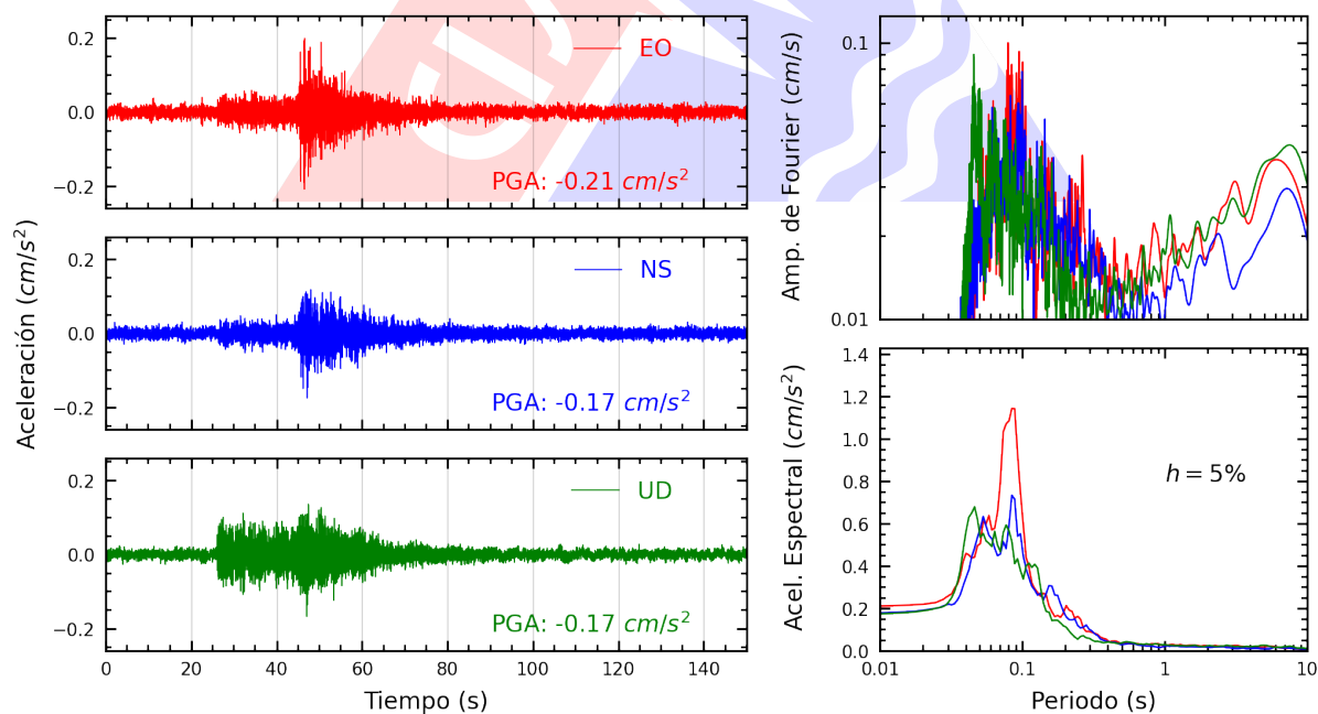
Figura A.12: Registros tiempo-historia, espectros de Fourier y de respuesta en las direcciones EO, NS y vertical de la estación USILP. Sismo de Yauyos, Yauyos - Lima del 2024-11-10, 16:10:00 (Hora local)
