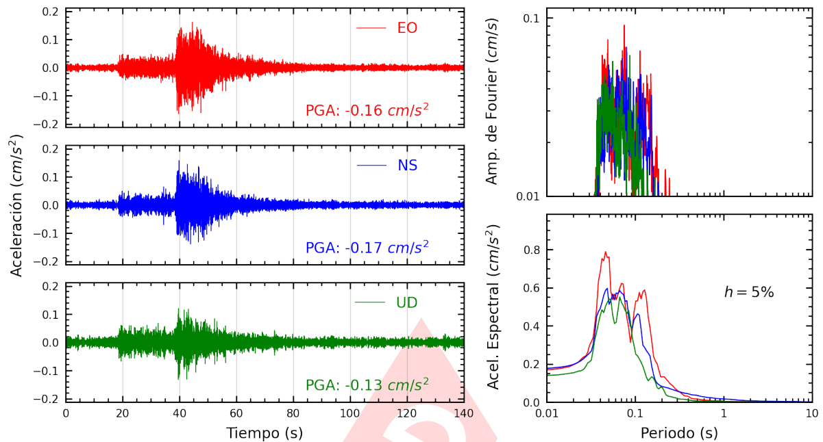
Figura A.19: Registros tiempo-historia, espectros de Fourier y de respuesta en las direcciones EO, NS y vertical de la estación ATARJ. Sismo de Yauyos, Yauyos - Lima del 2024-11-10, 16:10:00 (Hora local)
