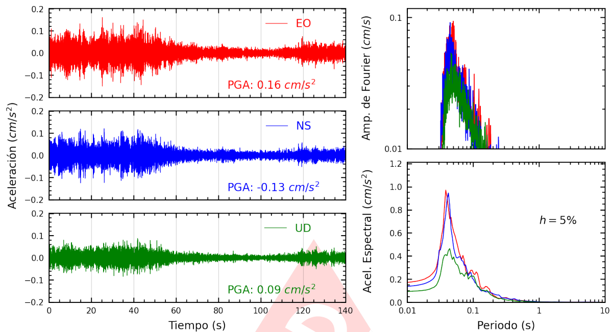
Figura A.21: Registros tiempo-historia, espectros de Fourier y de respuesta en las direcciones EO, NS y vertical de la estación BORJA. Sismo de Yauyos, Yauyos - Lima del 2024-11-10, 16:10:00 (Hora local)
