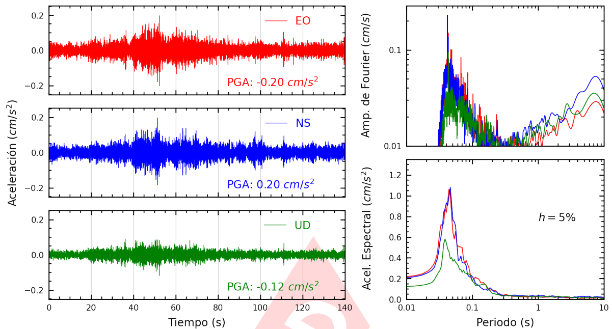
Figura A.15: Registros tiempo-historia, espectros de Fourier y de respuesta en las direcciones EO, NS y vertical de la estación CEPRE. Sismo de Yauyos, Yauyos - Lima del 2024-11-10, 16:10:00 (Hora local)
