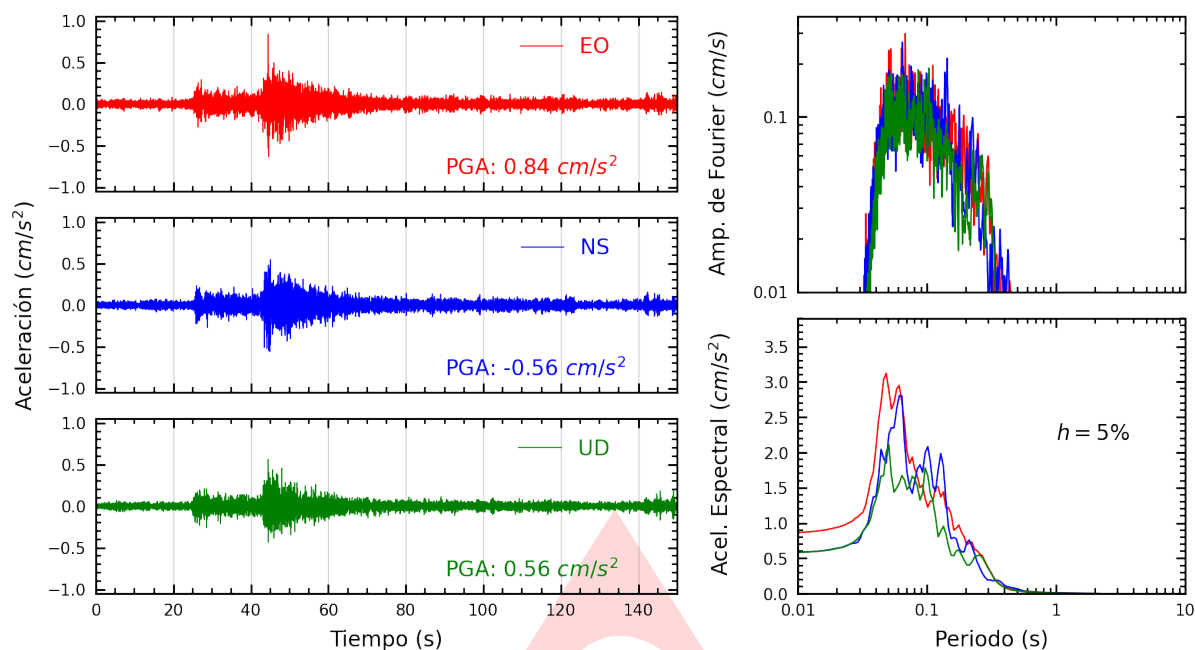
Figura A.1: Registros tiempo-historia, espectros de Fourier y de respuesta en las direcciones EO, NS y vertical de la estación PHER2. Sismo de Yauyos, Yauyos - Lima del 2024-11-10, 16:10:00 (Hora local)
