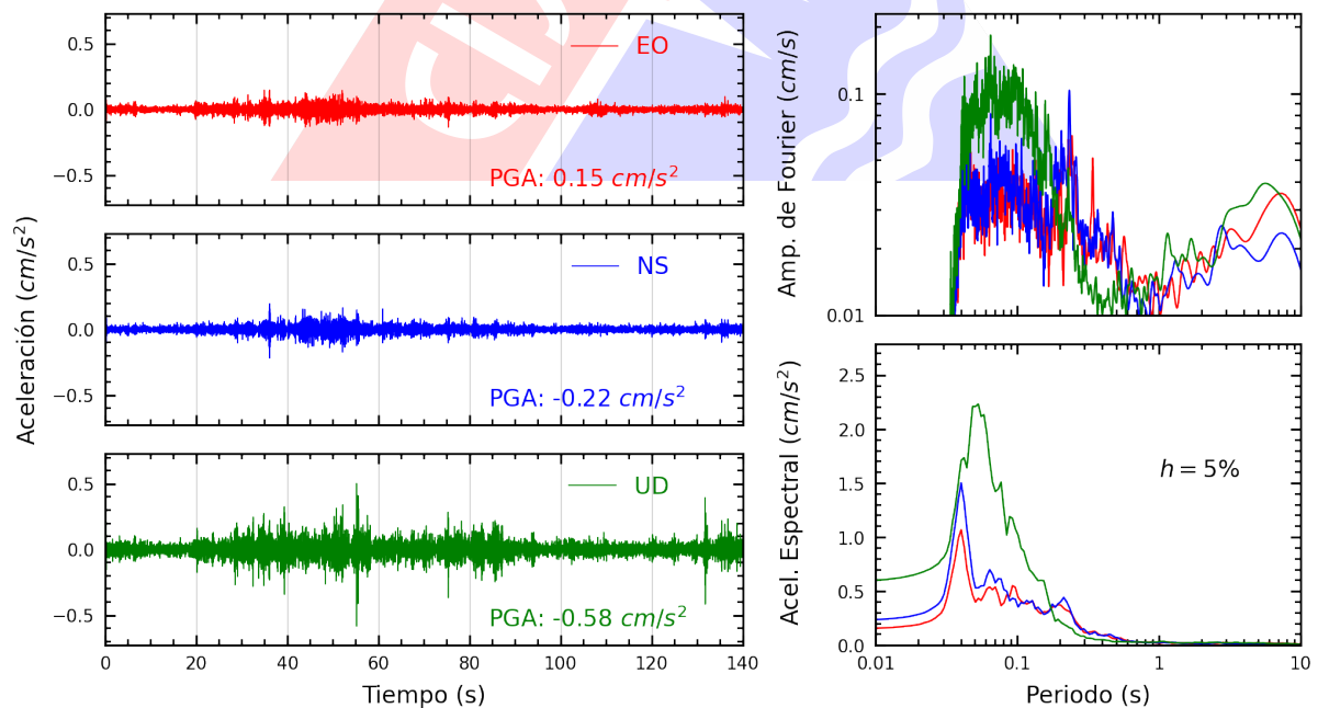
Figura A.4: Registros tiempo-historia, espectros de Fourier y de respuesta en las direcciones EO, NS y vertical de la estación MDPP. Sismo de Yauyos, Yauyos - Lima del 2024-11-10, 16:10:00 (Hora local)
