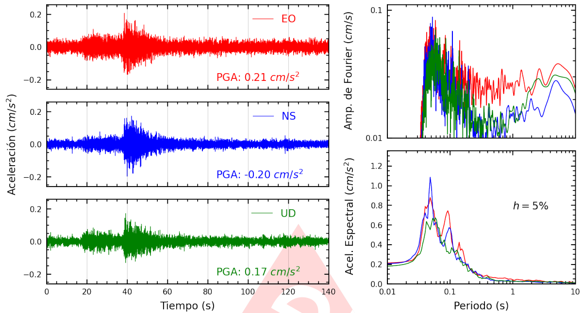
Figura A.13: Registros tiempo-historia, espectros de Fourier y de respuesta en las direcciones EO, NS y vertical de la estación IMCA. Sismo de Yauyos, Yauyos - Lima del 2024-11-10, 16:10:00 (Hora local)
