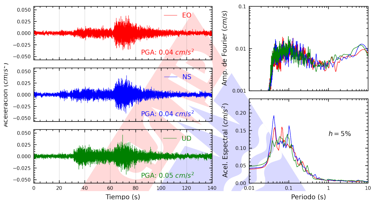
Figura A.29: Registros tiempo-historia, espectros de Fourier y de respuesta en las direcciones EO, NS y vertical de la estación CARAL. Sismo de Yauyos, Yauyos - Lima del 2024-11-10, 16:10:00 (Hora local)
