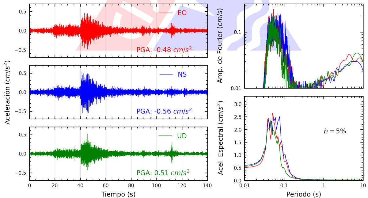
Figura A.6: Registros tiempo-historia, espectros de Fourier y de respuesta en las direcciones EO, NS y vertical de la estación JOSEO. Sismo de Yauyos, Yauyos - Lima del 2024-11-10, 16:10:00 (Hora local)
