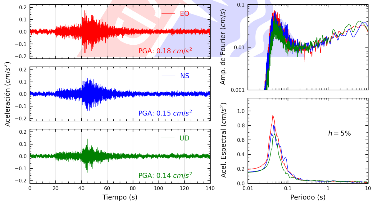
Figura A.18: Registros tiempo-historia, espectros de Fourier y de respuesta en las direcciones EO, NS y vertical de la estación UCSS. Sismo de Yauyos, Yauyos - Lima del 2024-11-10, 16:10:00 (Hora local)
