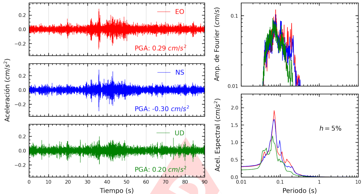
Figura A.9: Registros tiempo-historia, espectros de Fourier y de respuesta en las direcciones EO, NS y vertical de la estación SCCHO. Sismo de Yauyos, Yauyos - Lima del 2024-11-10, 16:10:00 (Hora local)
