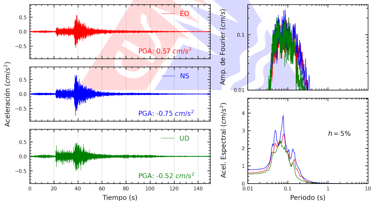
Figura A.2: Registros tiempo-historia, espectros de Fourier y de respuesta en las direcciones EO, NS y vertical de la estación ASIA. Sismo de Yauyos, Yauyos - Lima del 2024-11-10, 16:10:00 (Hora local)
