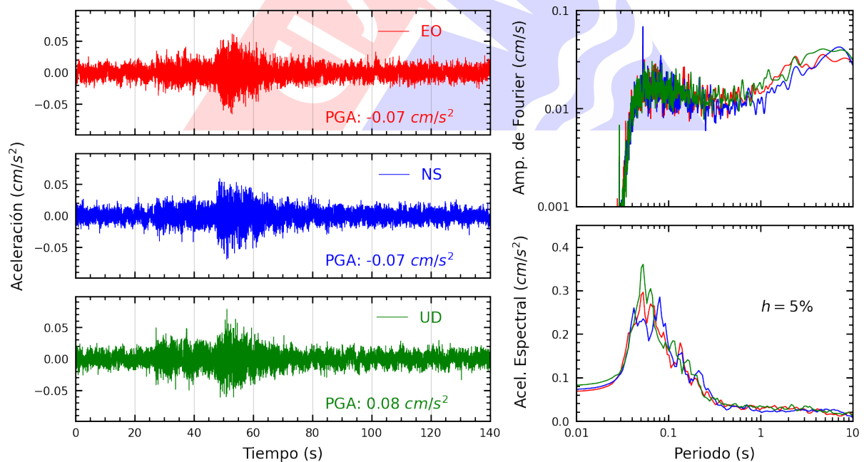
Figura A.26: Registros tiempo-historia, espectros de Fourier y de respuesta en las direcciones EO, NS y vertical de la estación UNMSM. Sismo de Yauyos, Yauyos - Lima del 2024-11-10, 16:10:00 (Hora local)
