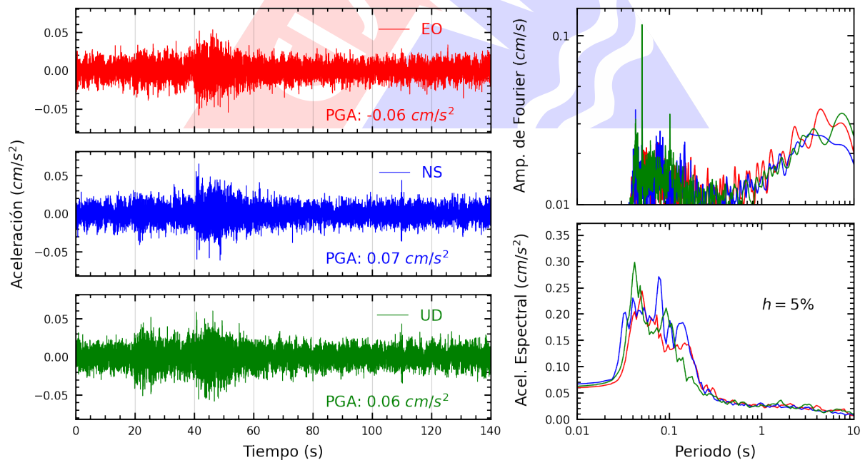
Figura A.28: Registros tiempo-historia, espectros de Fourier y de respuesta en las direcciones EO, NS y vertical de la estación BONDY. Sismo de Yauyos, Yauyos - Lima del 2024-11-10, 16:10:00 (Hora local)
