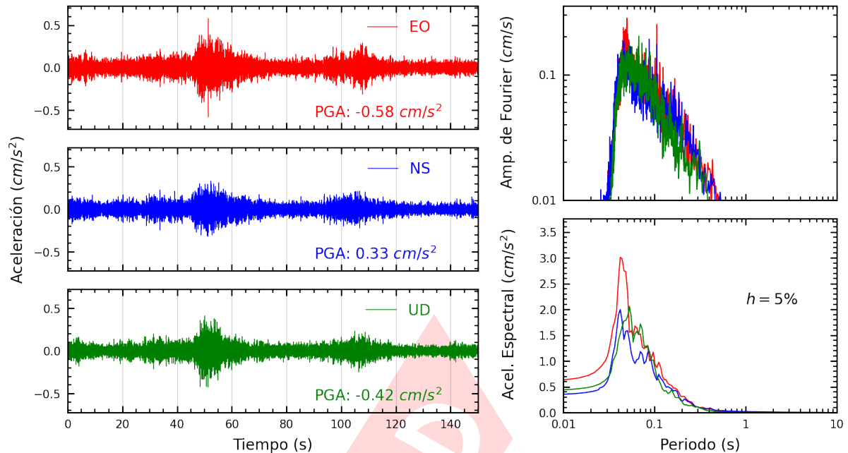
Figura A.5: Registros tiempo-historia, espectros de Fourier y de respuesta en las direcciones EO, NS y vertical de la estación UNTEL. Sismo de Yauyos, Yauyos - Lima del 2024-11-10, 16:10:00 (Hora local)
