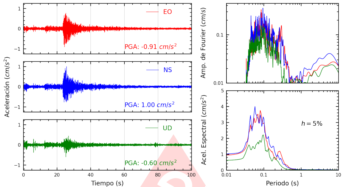
Figura A.11: Registros tiempo-historia, espectros de Fourier y de respuesta en las direcciones EO, NS y vertical de la estación DEFEN. Sismo de Chilca, Cañete - Lima del 2024-11-14, 19:27:48 (Hora local)
