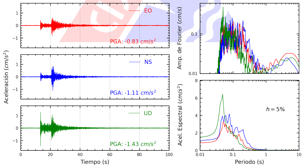
Figura A.6: Registros tiempo-historia, espectros de Fourier y de respuesta en las direcciones EO, NS y vertical de la estación USILP. Sismo de Chilca, Cañete - Lima del 2024-11-14, 19:27:48 (Hora local)
