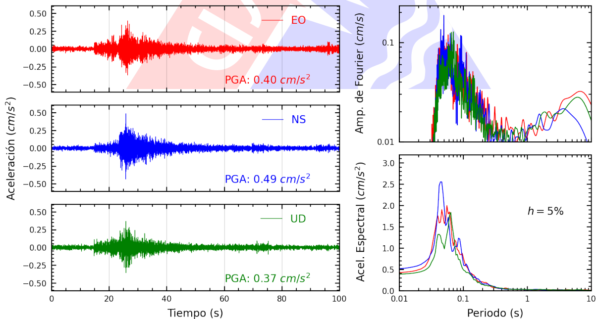
Figura A.22: Registros tiempo-historia, espectros de Fourier y de respuesta en las direcciones EO, NS y vertical de la estación IMCA. Sismo de Chilca, Cañete - Lima del 2024-11-14, 19:27:48 (Hora local)
