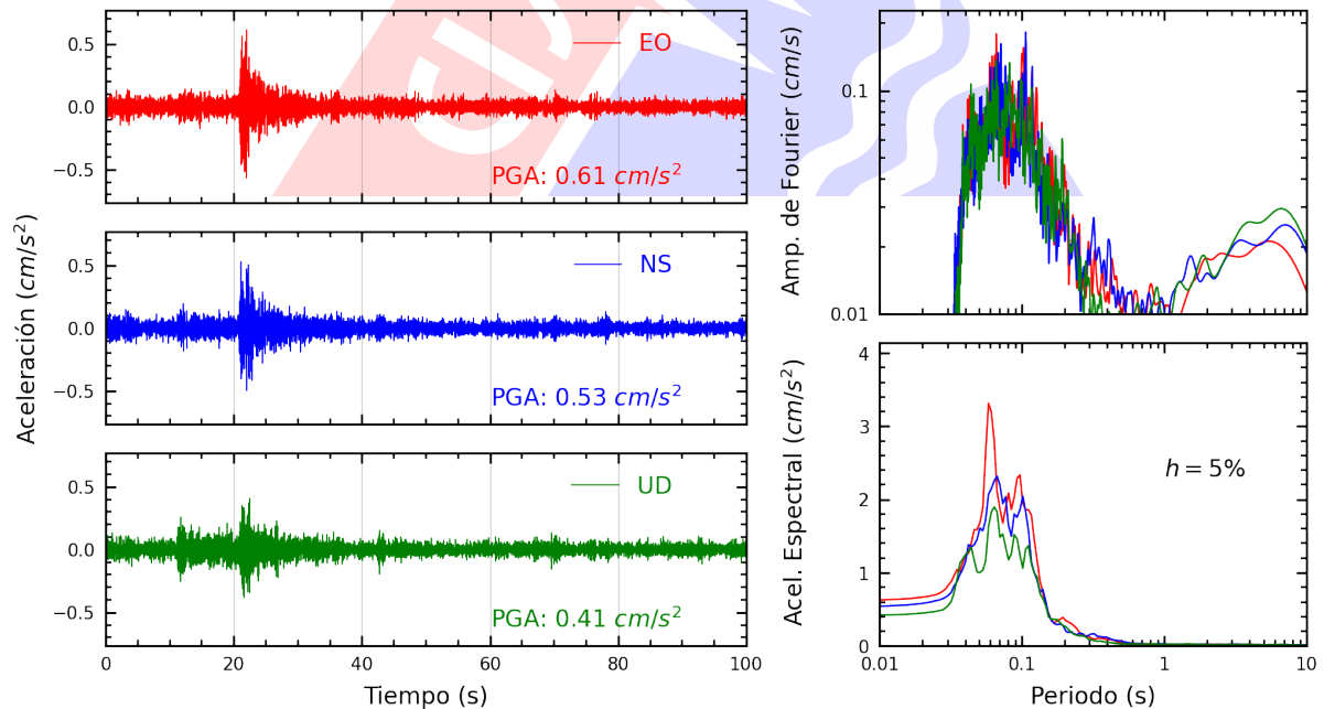
Figura A.18: Registros tiempo-historia, espectros de Fourier y de respuesta en las direcciones EO, NS y vertical de la estación MADRE. Sismo de Chilca, Cañete - Lima del 2024-11-14, 19:27:48 (Hora local)
