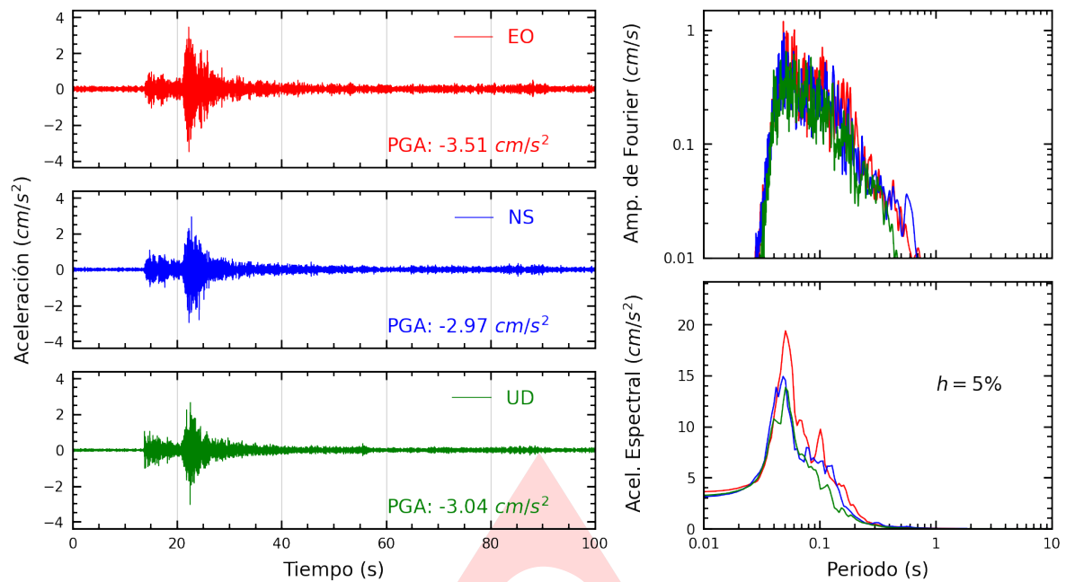
Figura A.1: Registros tiempo-historia, espectros de Fourier y de respuesta en las direcciones EO, NS y vertical de la estación UNTEL. Sismo de Chilca, Cañete - Lima del 2024-11-14, 19:27:48 (Hora local)
