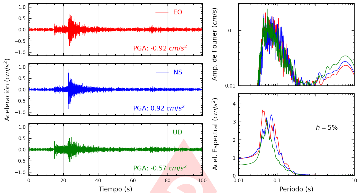
Figura A.13: Registros tiempo-historia, espectros de Fourier y de respuesta en las direcciones EO, NS y vertical de la estación URPPE. Sismo de Chilca, Cañete - Lima del 2024-11-14, 19:27:48 (Hora local)
