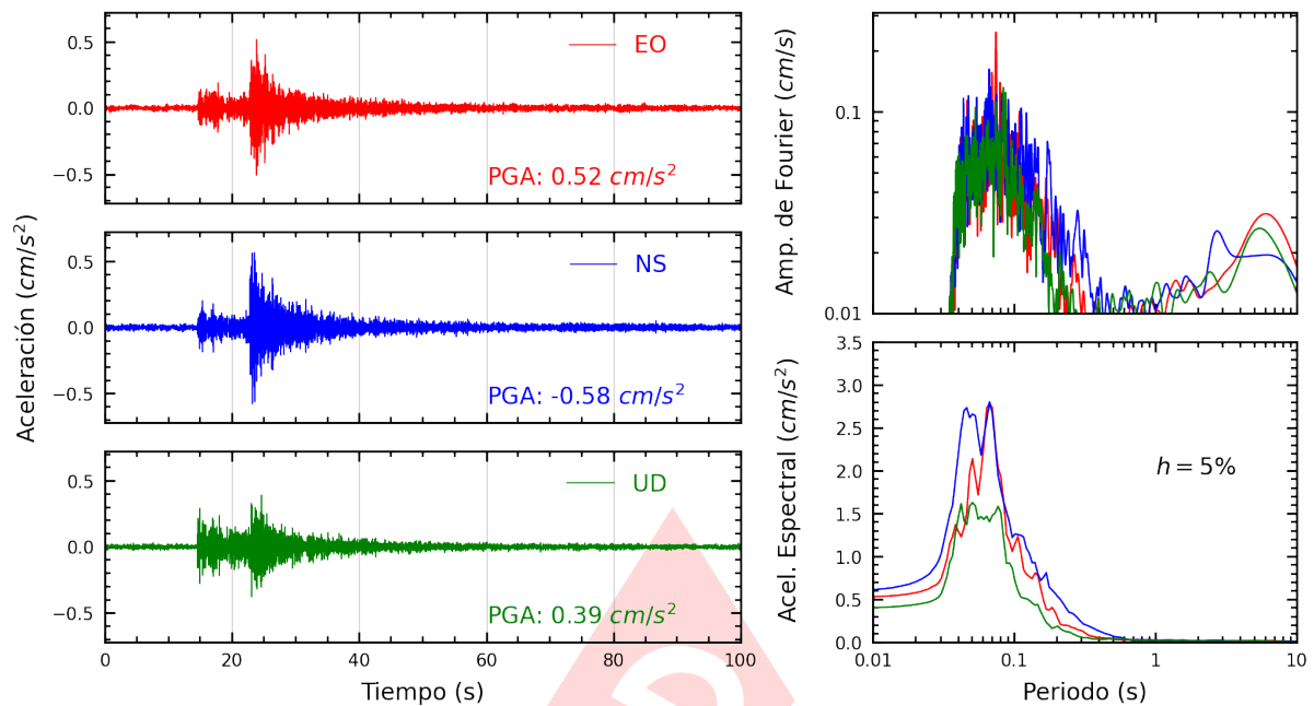
Figura A.19: Registros tiempo-historia, espectros de Fourier y de respuesta en las direcciones EO, NS y vertical de la estación SERVI. Sismo de Chilca, Cañete - Lima del 2024-11-14, 19:27:48 (Hora local)
