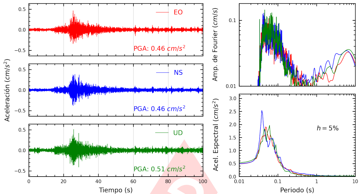
Figura A.21: Registros tiempo-historia, espectros de Fourier y de respuesta en las direcciones EO, NS y vertical de la estación USMP. Sismo de Chilca, Cañete - Lima del 2024-11-14, 19:27:48 (Hora local)
