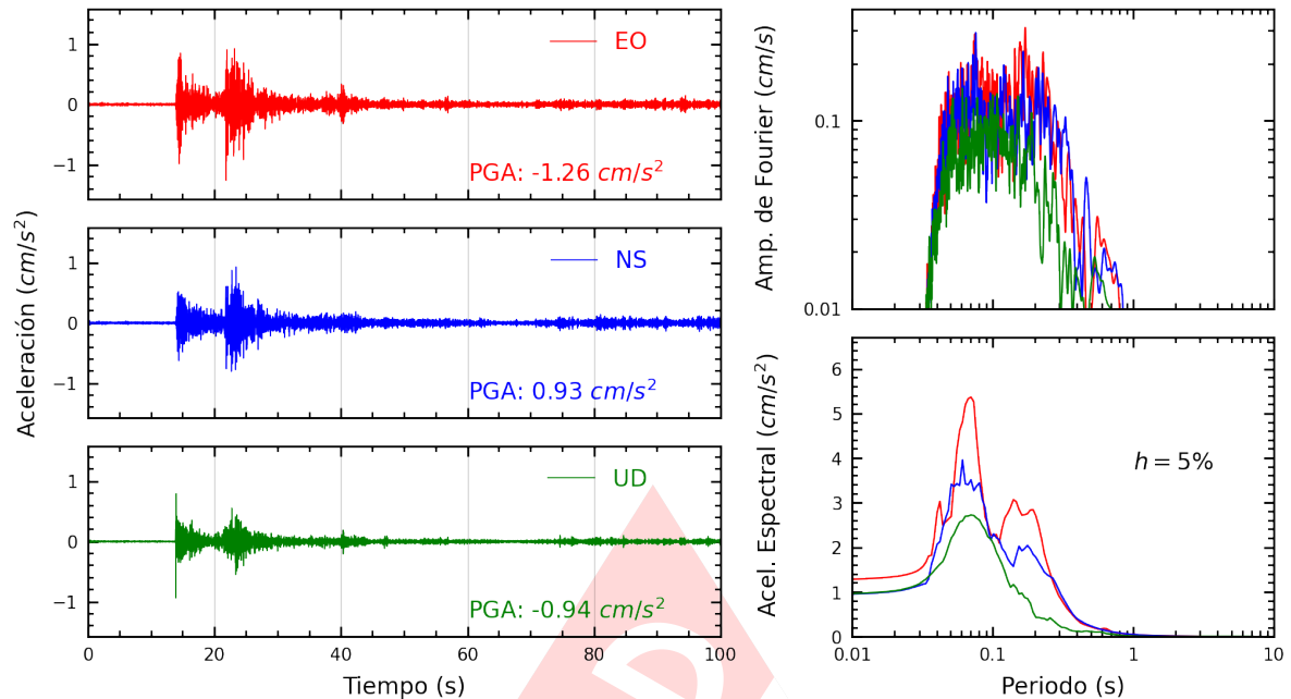
Figura A.7: Registros tiempo-historia, espectros de Fourier y de respuesta en las direcciones EO, NS y vertical de la estación BRISA. Sismo de Chilca, Cañete - Lima del 2024-11-14, 19:27:48 (Hora local)
