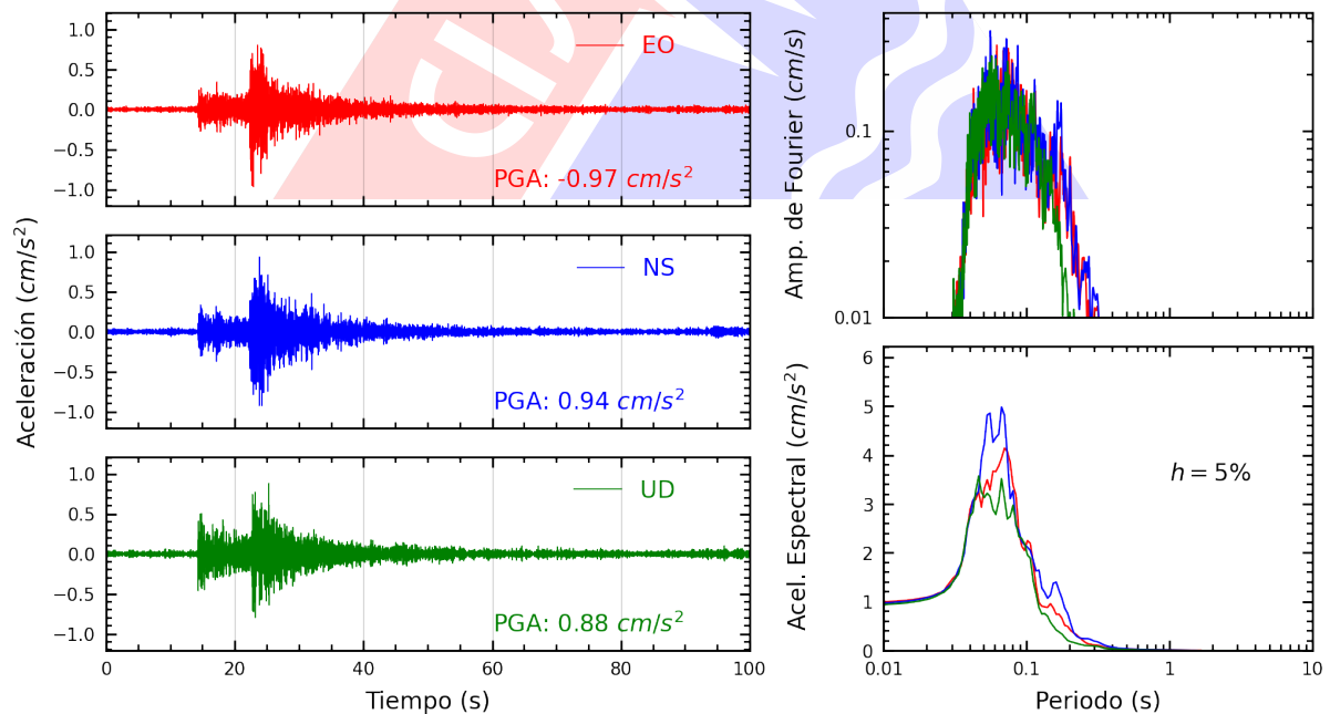
Figura A.12: Registros tiempo-historia, espectros de Fourier y de respuesta en las direcciones EO, NS y vertical de la estación ASIA. Sismo de Chilca, Cañete - Lima del 2024-11-14, 19:27:48 (Hora local)
