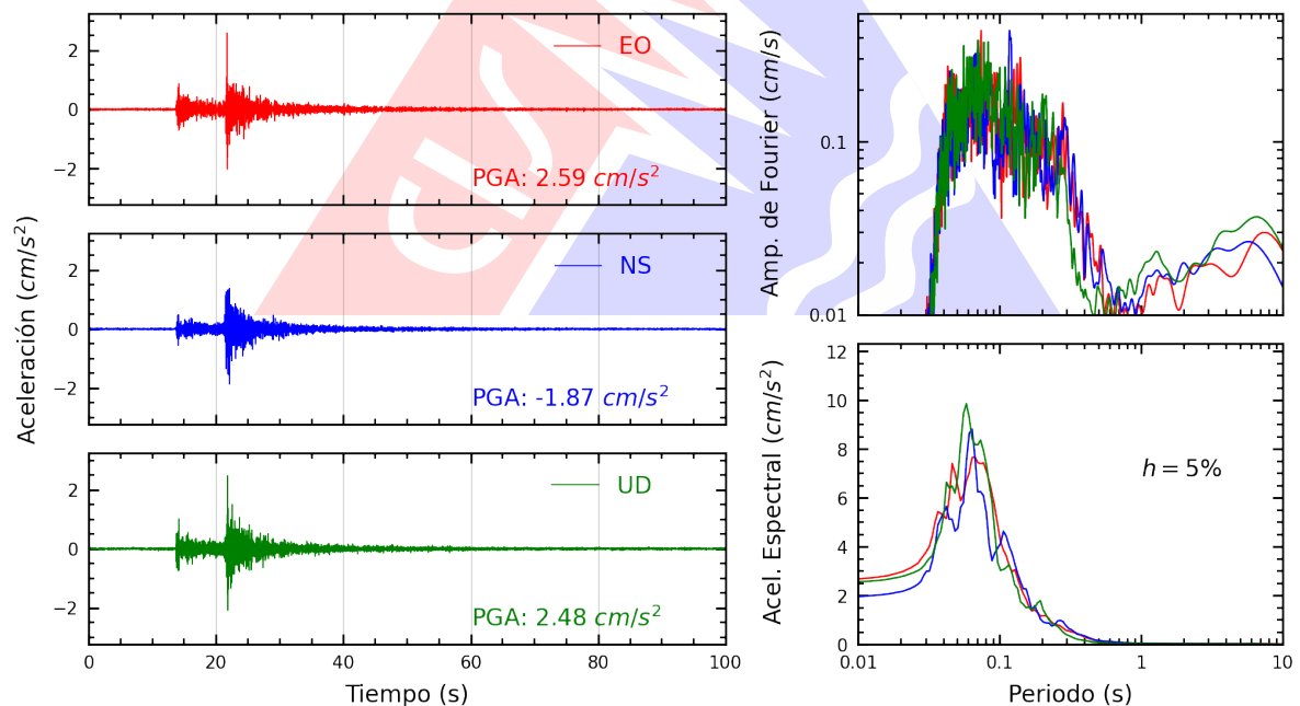
Figura A.2: Registros tiempo-historia, espectros de Fourier y de respuesta en las direcciones EO, NS y vertical de la estación SOVES. Sismo de Chilca, Cañete - Lima del 2024-11-14, 19:27:48 (Hora local)
