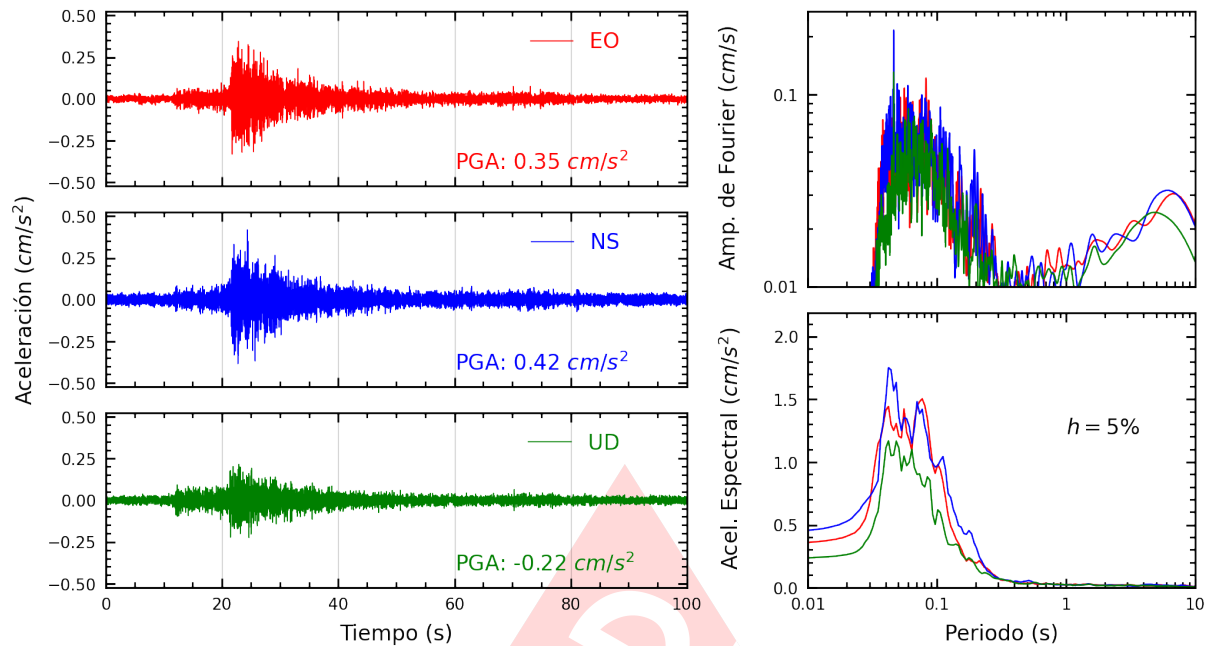
Figura A.23: Registros tiempo-historia, espectros de Fourier y de respuesta en las direcciones EO, NS y vertical de la estación COMAS. Sismo de Chilca, Cañete - Lima del 2024-11-14, 19:27:48 (Hora local)
