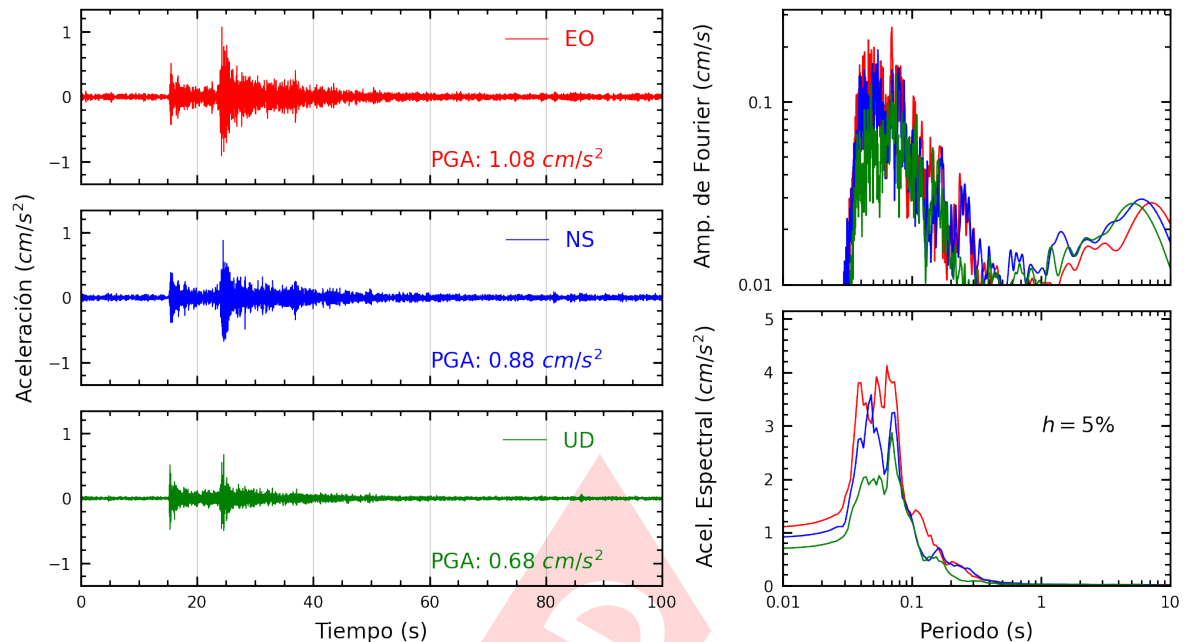
Figura A.9: Registros tiempo-historia, espectros de Fourier y de respuesta en las direcciones EO, NS y vertical de la estación CEPRE. Sismo de Chilca, Cañete - Lima del 2024-11-14, 19:27:48 (Hora local)
