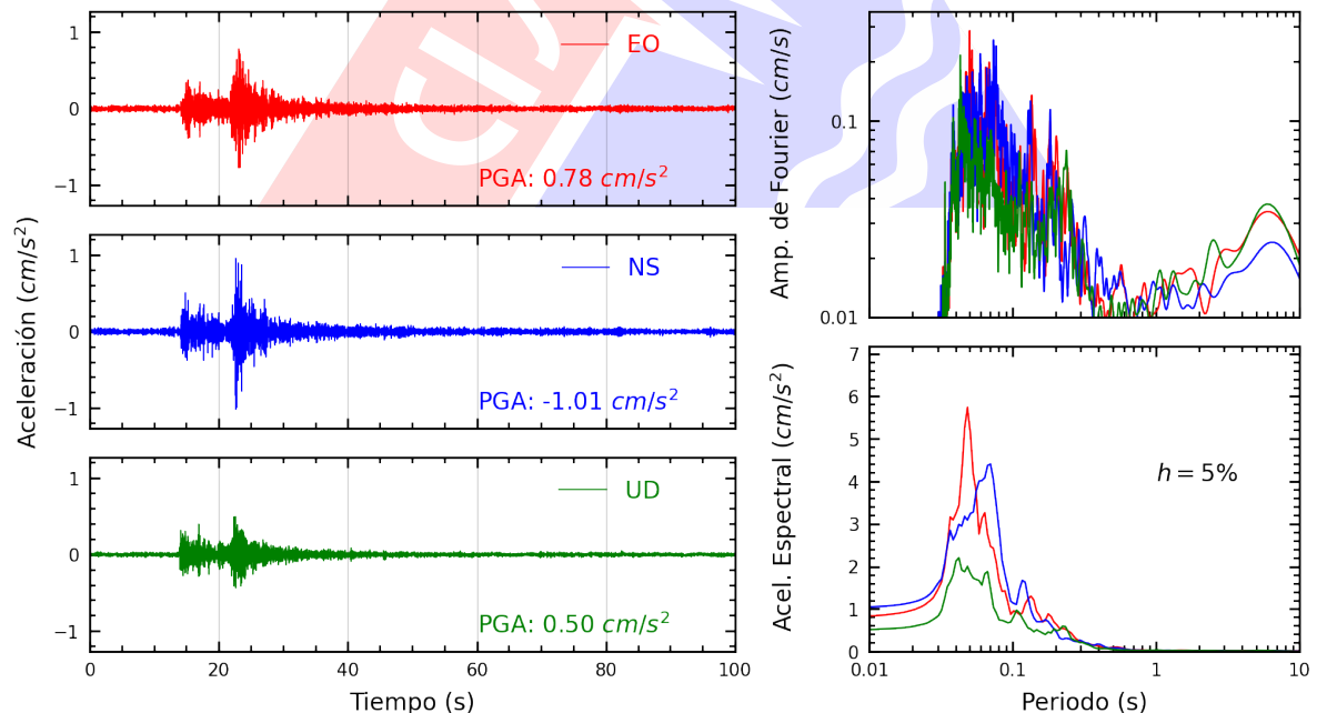
Figura A.10: Registros tiempo-historia, espectros de Fourier y de respuesta en las direcciones EO, NS y vertical de la estación UPCVI. Sismo de Chilca, Cañete - Lima del 2024-11-14, 19:27:48 (Hora local)
