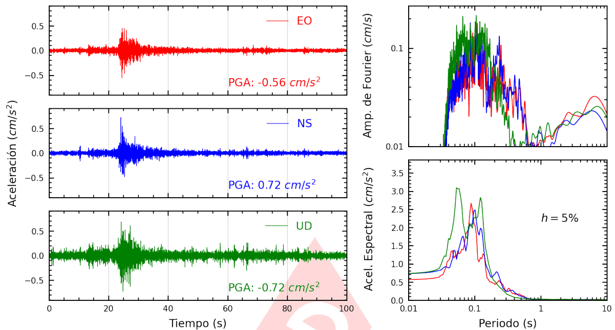
Figura A.15: Registros tiempo-historia, espectros de Fourier y de respuesta en las direcciones EO, NS y vertical de la estación MDPP. Sismo de Chilca, Cañete - Lima del 2024-11-14, 19:27:48 (Hora local)
