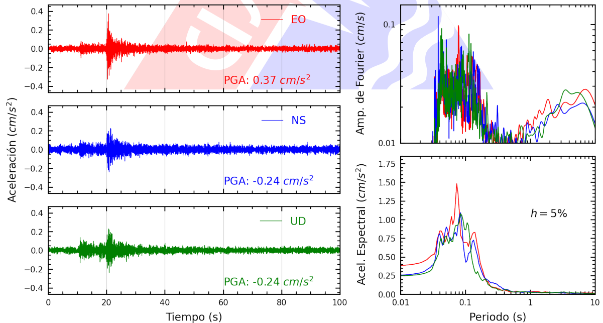
Figura A.24: Registros tiempo-historia, espectros de Fourier y de respuesta en las direcciones EO, NS y vertical de la estación BONDY. Sismo de Chilca, Cañete - Lima del 2024-11-14, 19:27:48 (Hora local)
