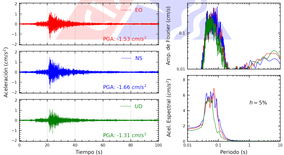
Figura A.4: Registros tiempo-historia, espectros de Fourier y de respuesta en las direcciones EO, NS y vertical de la estación JOSEO. Sismo de Chilca, Cañete - Lima del 2024-11-14, 19:27:48 (Hora local)
