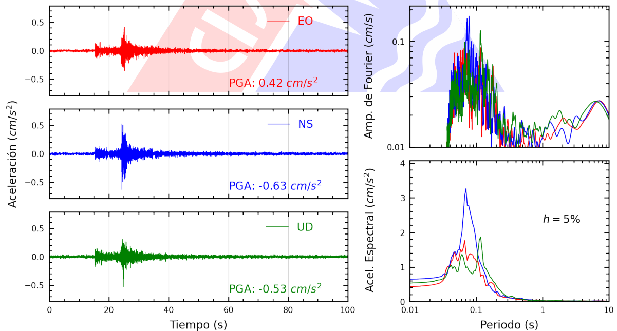
Figura A.16: Registros tiempo-historia, espectros de Fourier y de respuesta en las direcciones EO, NS y vertical de la estación UNFV. Sismo de Chilca, Cañete - Lima del 2024-11-14, 19:27:48 (Hora local)
