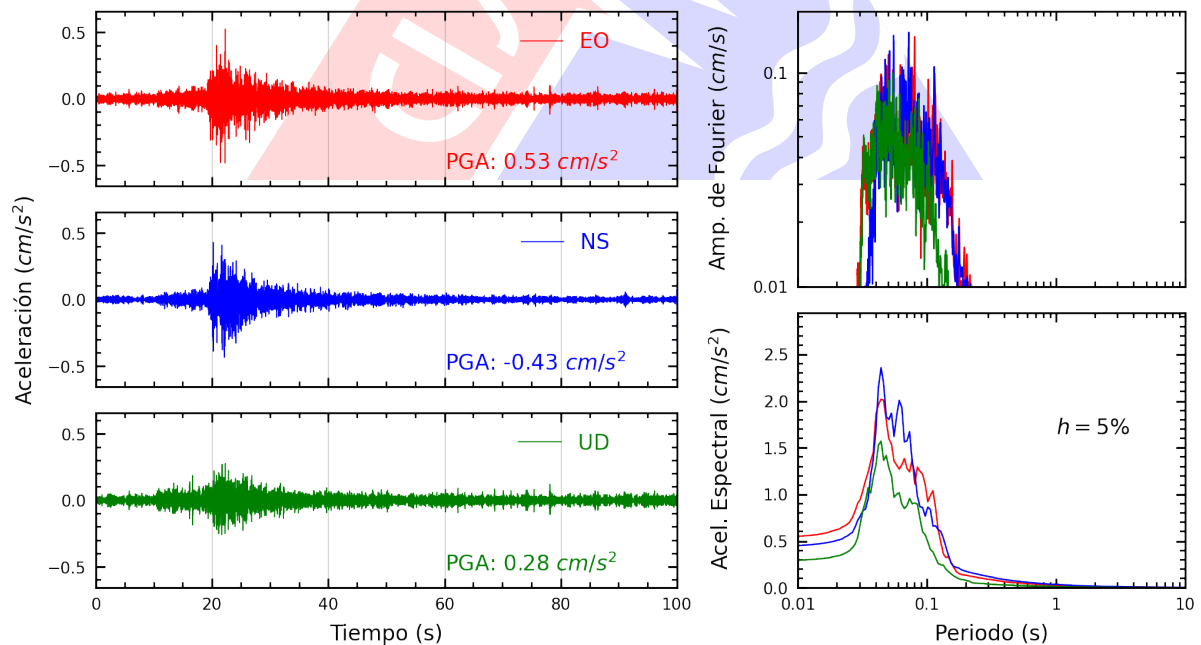
Figura A.20: Registros tiempo-historia, espectros de Fourier y de respuesta en las direcciones EO, NS y vertical de la estación ATARJ. Sismo de Chilca, Cañete - Lima del 2024-11-14, 19:27:48 (Hora local)
