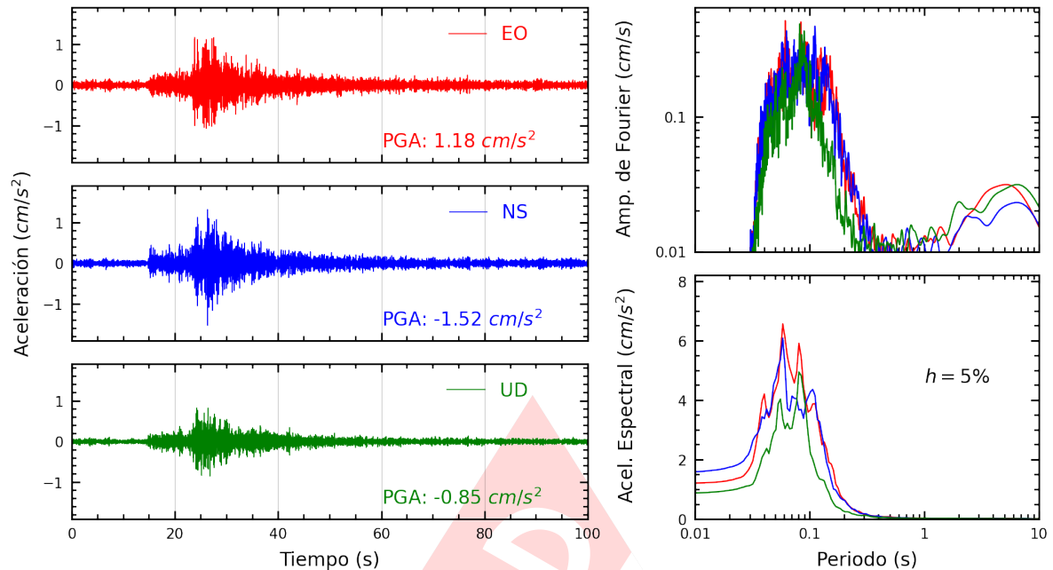
Figura A.5: Registros tiempo-historia, espectros de Fourier y de respuesta en las direcciones EO, NS y vertical de la estación USILM. Sismo de Chilca, Cañete - Lima del 2024-11-14, 19:27:48 (Hora local)
