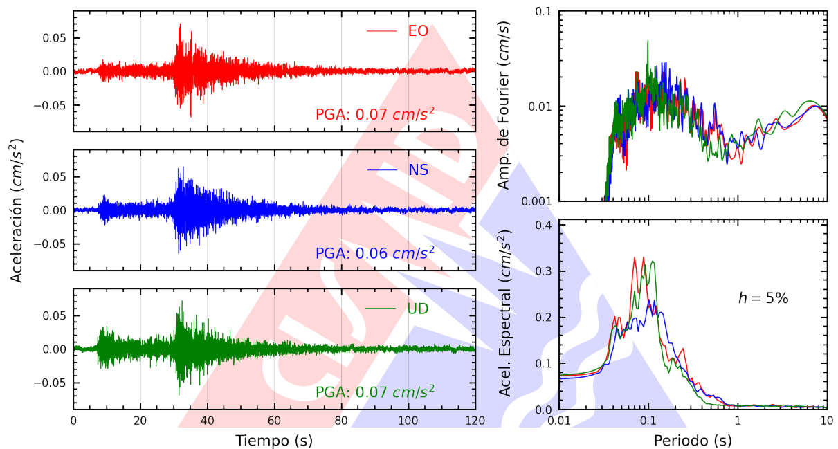
Figura A.25: Registros tiempo-historia, espectros de Fourier y de respuesta en las direcciones EO, NS y vertical de la estación CARAL. Sismo de Chilca, Cañete - Lima del 2024-11-14, 19:27:48 (Hora local)
