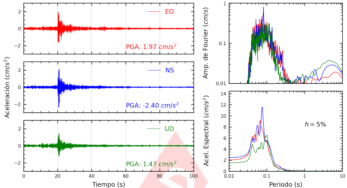
Figura A.3: Registros tiempo-historia, espectros de Fourier y de respuesta en las direcciones EO, NS y vertical de la estación INDEP. Sismo de Chilca, Cañete - Lima del 2024-11-14, 19:27:48 (Hora local)
