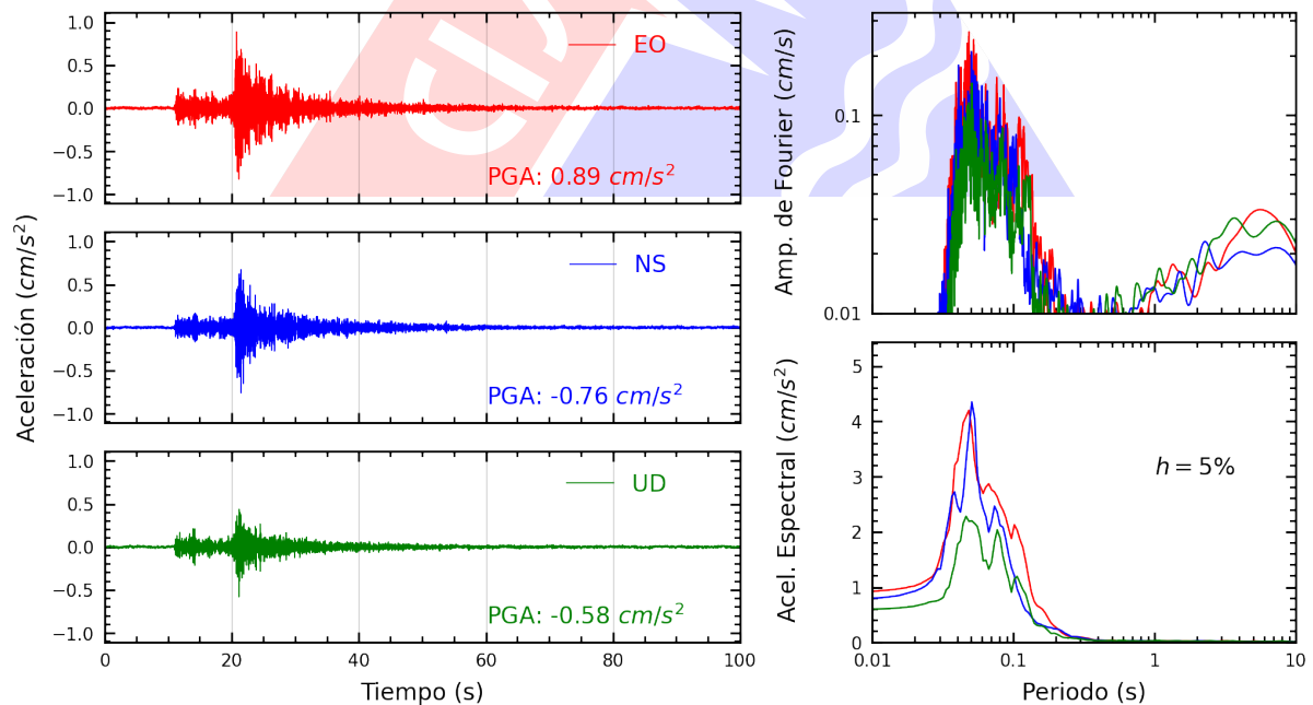
Figura A.14: Registros tiempo-historia, espectros de Fourier y de respuesta en las direcciones EO, NS y vertical de la estación UCSS. Sismo de Chilca, Cañete - Lima del 2024-11-14, 19:27:48 (Hora local)
