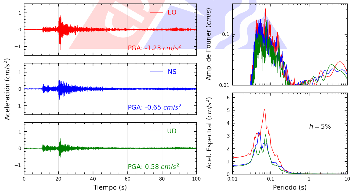
Figura A.8: Registros tiempo-historia, espectros de Fourier y de respuesta en las direcciones EO, NS y vertical de la estación FICPE. Sismo de Chilca, Cañete - Lima del 2024-11-14, 19:27:48 (Hora local)
