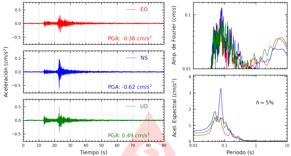
Figura A.17: Registros tiempo-historia, espectros de Fourier y de respuesta en las direcciones EO, NS y vertical de la estación UNMSM. Sismo de Chilca, Cañete - Lima del 2024-11-14, 19:27:48 (Hora local)
