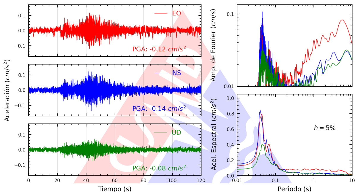
Figura A.33: Registros tiempo-historia, espectros de Fourier y de respuesta en las direcciones EO, NS y vertical de la estación UNAB. Sismo de Ancon, Lima - Lima del 2024-11-15, 22:26:20 (Hora local)
