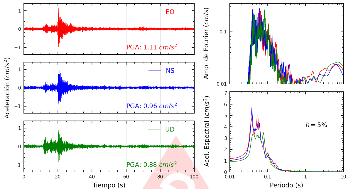
Figura A.15: Registros tiempo-historia, espectros de Fourier y de respuesta en las direcciones EO, NS y vertical de la estación MADRE. Sismo de Ancon, Lima - Lima del 2024-11-15, 22:26:20 (Hora local)
