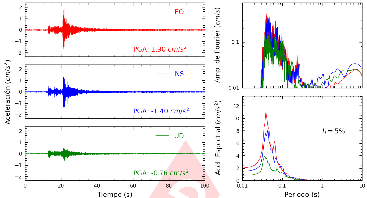
Figura A.9: Registros tiempo-historia, espectros de Fourier y de respuesta en las direcciones EO, NS y vertical de la estación CEPRE. Sismo de Ancon, Lima - Lima del 2024-11-15, 22:26:20 (Hora local)
