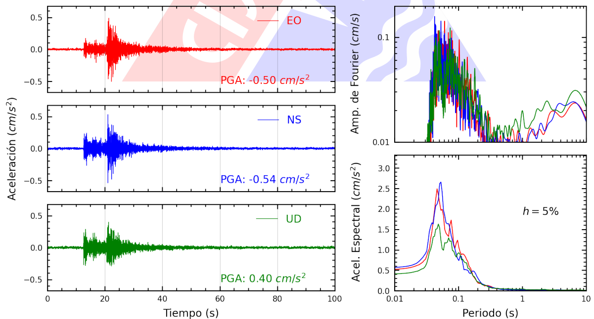
Figura A.24: Registros tiempo-historia, espectros de Fourier y de respuesta en las direcciones EO, NS y vertical de la estación UNFV. Sismo de Ancon, Lima - Lima del 2024-11-15, 22:26:20 (Hora local)
