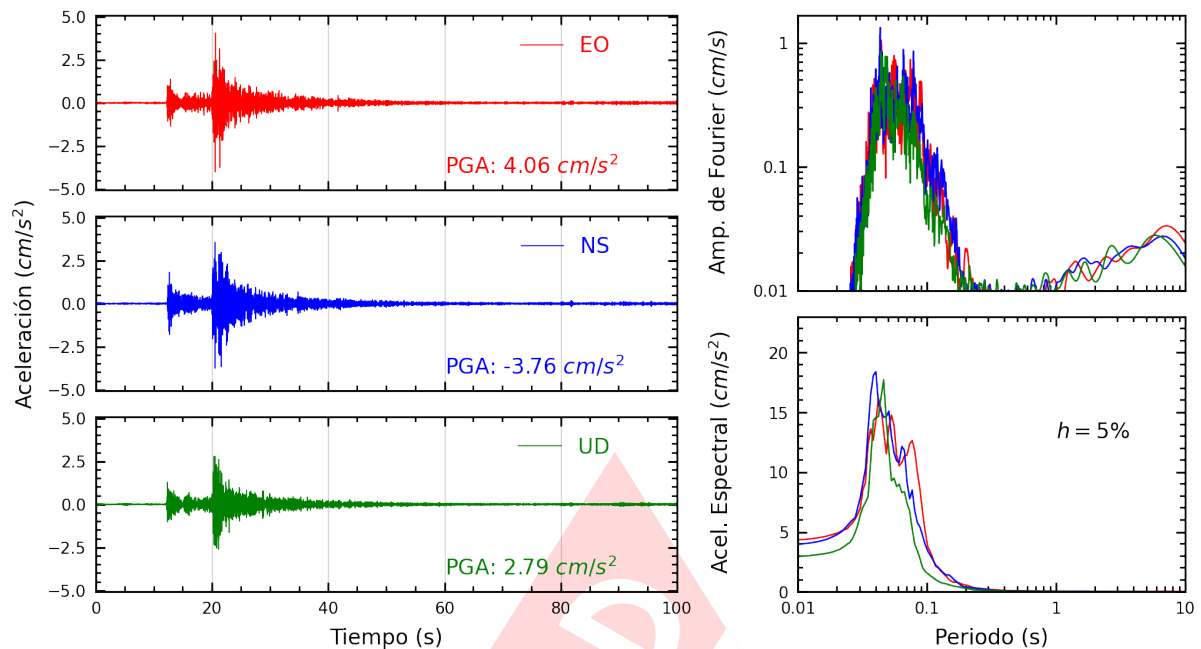
Figura A.5: Registros tiempo-historia, espectros de Fourier y de respuesta en las direcciones EO, NS y vertical de la estación JOSEO. Sismo de Ancon, Lima - Lima del 2024-11-15, 22:26:20 (Hora local)
