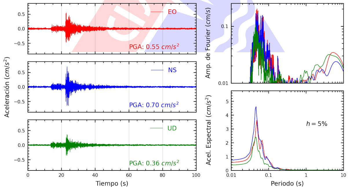
Figura A.22: Registros tiempo-historia, espectros de Fourier y de respuesta en las direcciones EO, NS y vertical de la estación UPCVI. Sismo de Ancon, Lima - Lima del 2024-11-15, 22:26:20 (Hora local)
