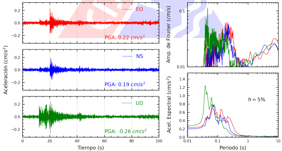
Figura A.30: Registros tiempo-historia, espectros de Fourier y de respuesta en las direcciones EO, NS y vertical de la estación DSMI. Sismo de Ancon, Lima - Lima del 2024-11-15, 22:26:20 (Hora local)
