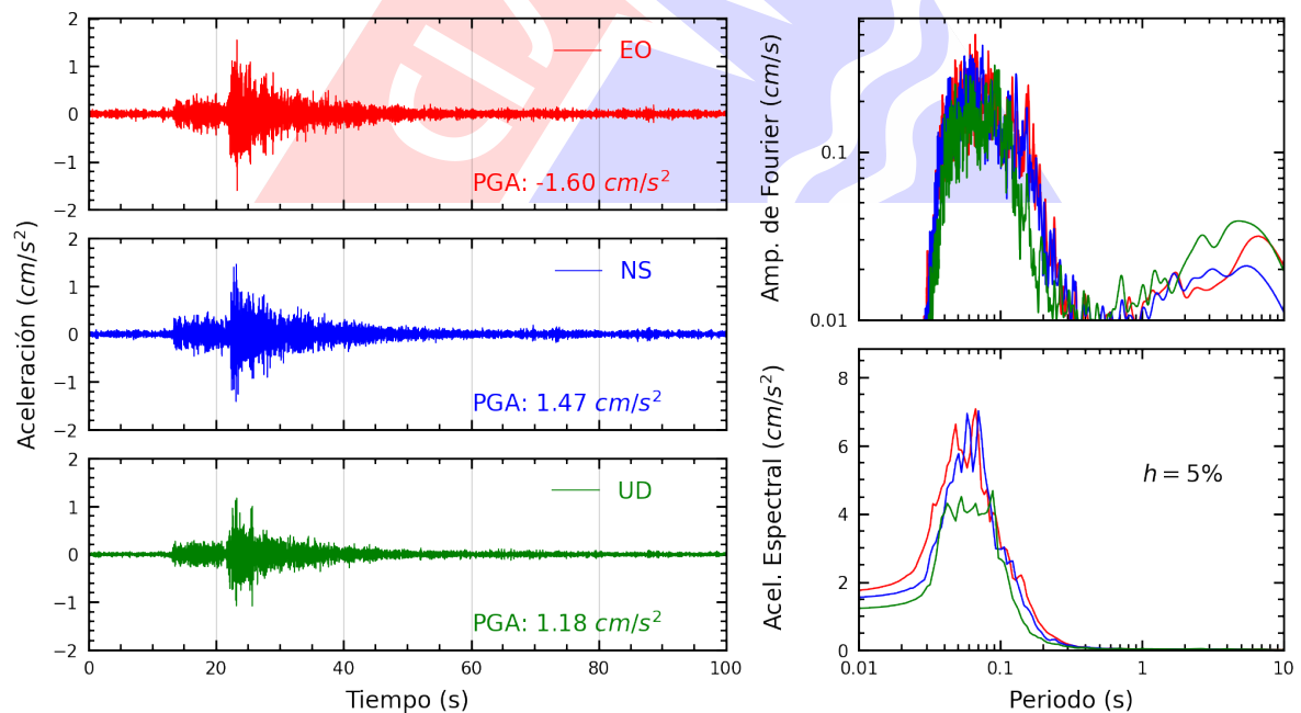
Figura A.12: Registros tiempo-historia, espectros de Fourier y de respuesta en las direcciones EO, NS y vertical de la estación USILM. Sismo de Ancon, Lima - Lima del 2024-11-15, 22:26:20 (Hora local)
