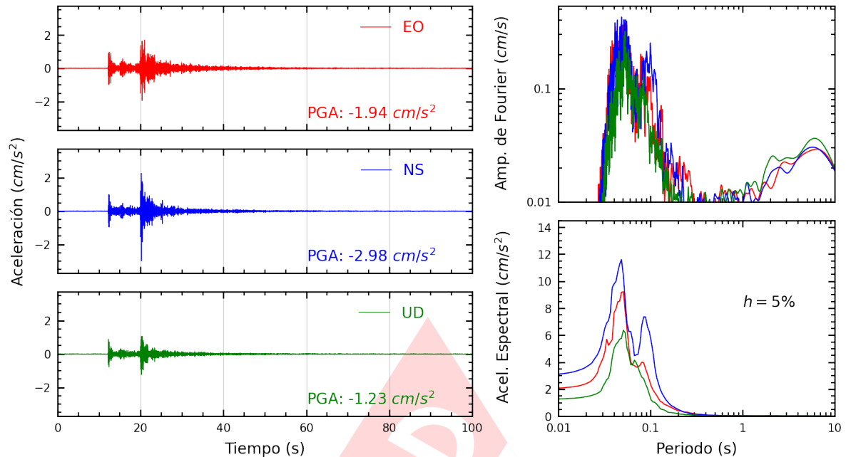
Figura A.7: Registros tiempo-historia, espectros de Fourier y de respuesta en las direcciones EO, NS y vertical de la estación UCSS. Sismo de Ancon, Lima - Lima del 2024-11-15, 22:26:20 (Hora local)
