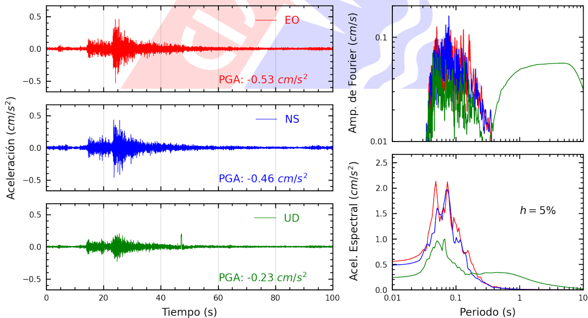
Figura A.26: Registros tiempo-historia, espectros de Fourier y de respuesta en las direcciones EO, NS y vertical de la estación BRISA. Sismo de Ancon, Lima - Lima del 2024-11-15, 22:26:20 (Hora local)
