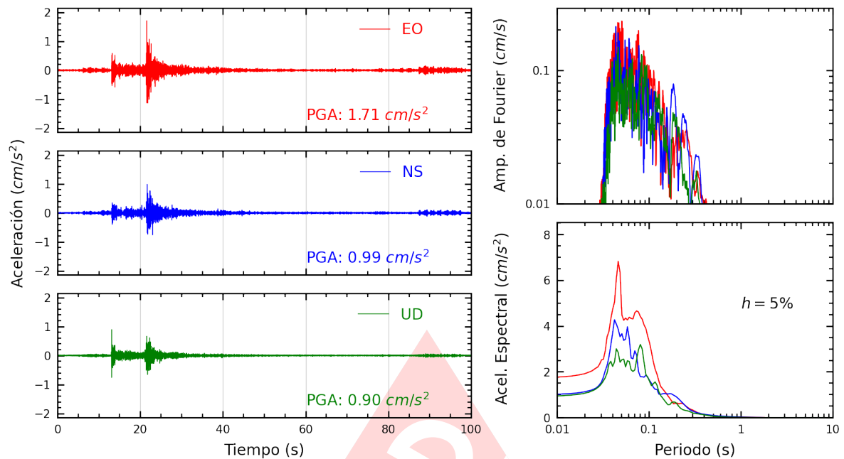
Figura A.11: Registros tiempo-historia, espectros de Fourier y de respuesta en las direcciones EO, NS y vertical de la estación BORJA. Sismo de Ancon, Lima - Lima del 2024-11-15, 22:26:20 (Hora local)
