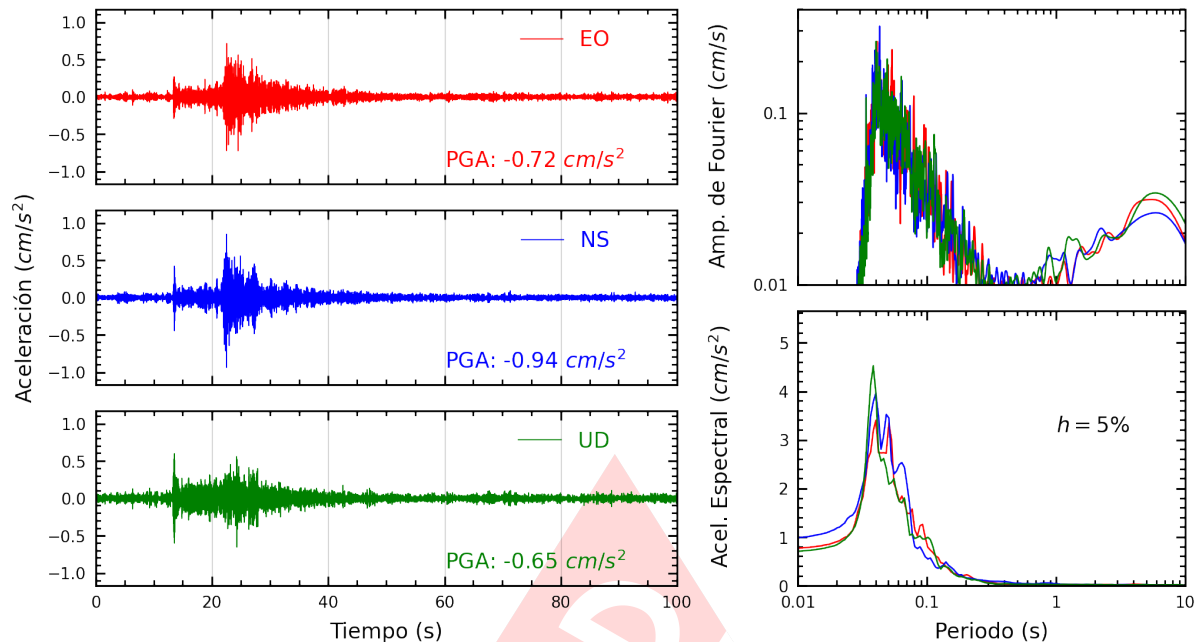
Figura A.19: Registros tiempo-historia, espectros de Fourier y de respuesta en las direcciones EO, NS y vertical de la estación USMP. Sismo de Ancon, Lima - Lima del 2024-11-15, 22:26:20 (Hora local)
