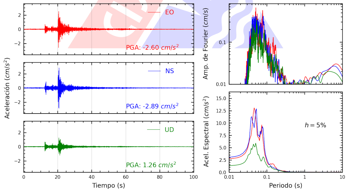
Figura A.8: Registros tiempo-historia, espectros de Fourier y de respuesta en las direcciones EO, NS y vertical de la estación FICPE. Sismo de Ancon, Lima - Lima del 2024-11-15, 22:26:20 (Hora local)
