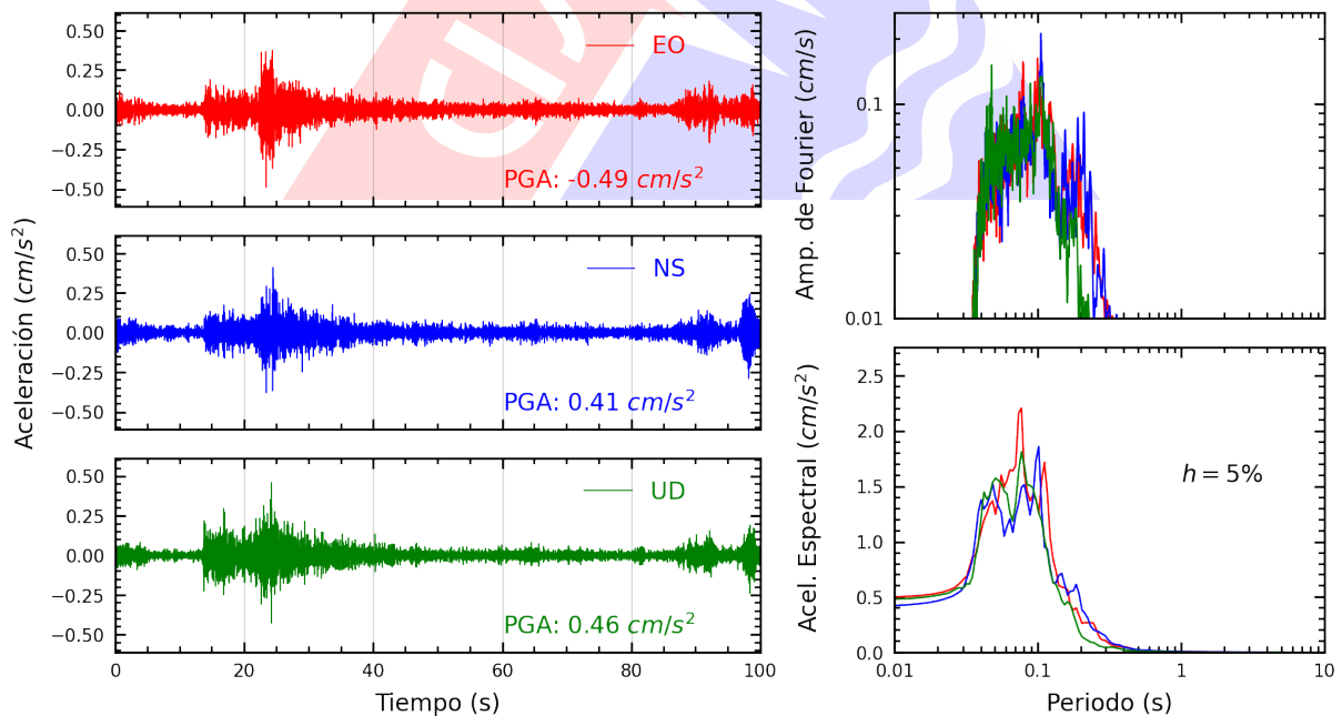
Figura A.28: Registros tiempo-historia, espectros de Fourier y de respuesta en las direcciones EO, NS y vertical de la estación SCCHO. Sismo de Ancon, Lima - Lima del 2024-11-15, 22:26:20 (Hora local)
