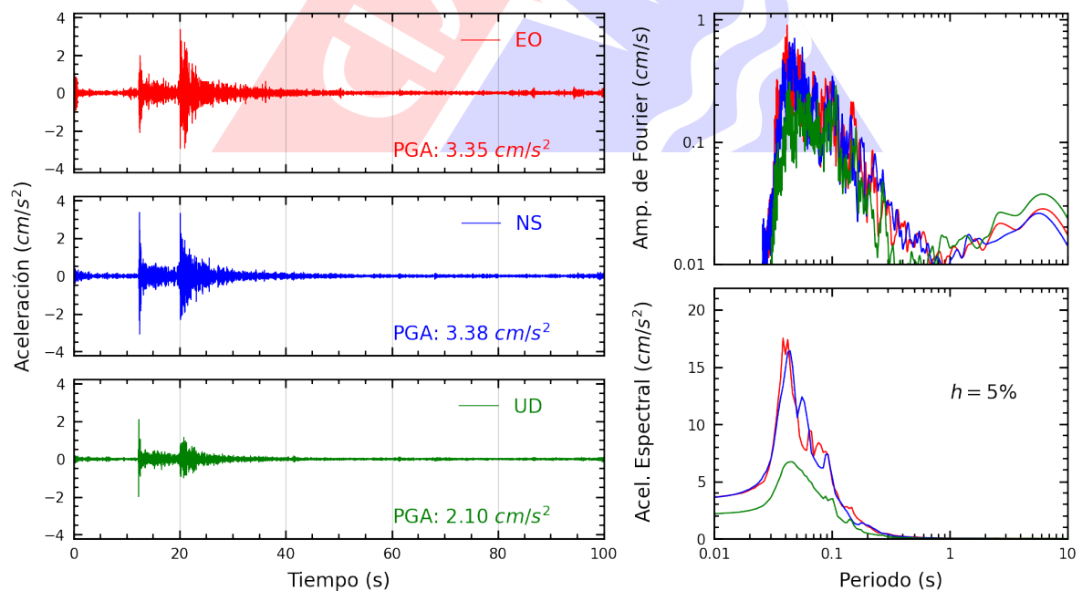
Figura A.6: Registros tiempo-historia, espectros de Fourier y de respuesta en las direcciones EO, NS y vertical de la estación OLIVO. Sismo de Ancon, Lima - Lima del 2024-11-15, 22:26:20 (Hora local)
