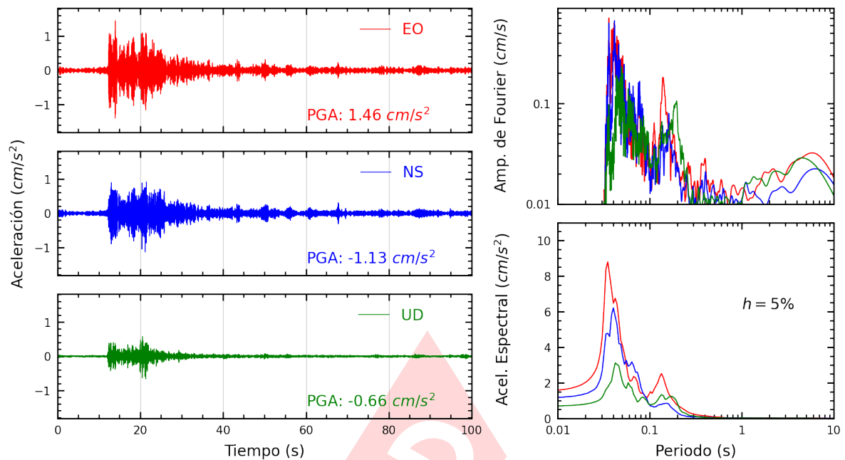
Figura A.13: Registros tiempo-historia, espectros de Fourier y de respuesta en las direcciones EO, NS y vertical de la estación DHNPE. Sismo de Ancon, Lima - Lima del 2024-11-15, 22:26:20 (Hora local)
