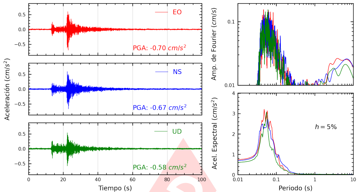
Figura A.21: Registros tiempo-historia, espectros de Fourier y de respuesta en las direcciones EO, NS y vertical de la estación SERVI. Sismo de Ancon, Lima - Lima del 2024-11-15, 22:26:20 (Hora local)
