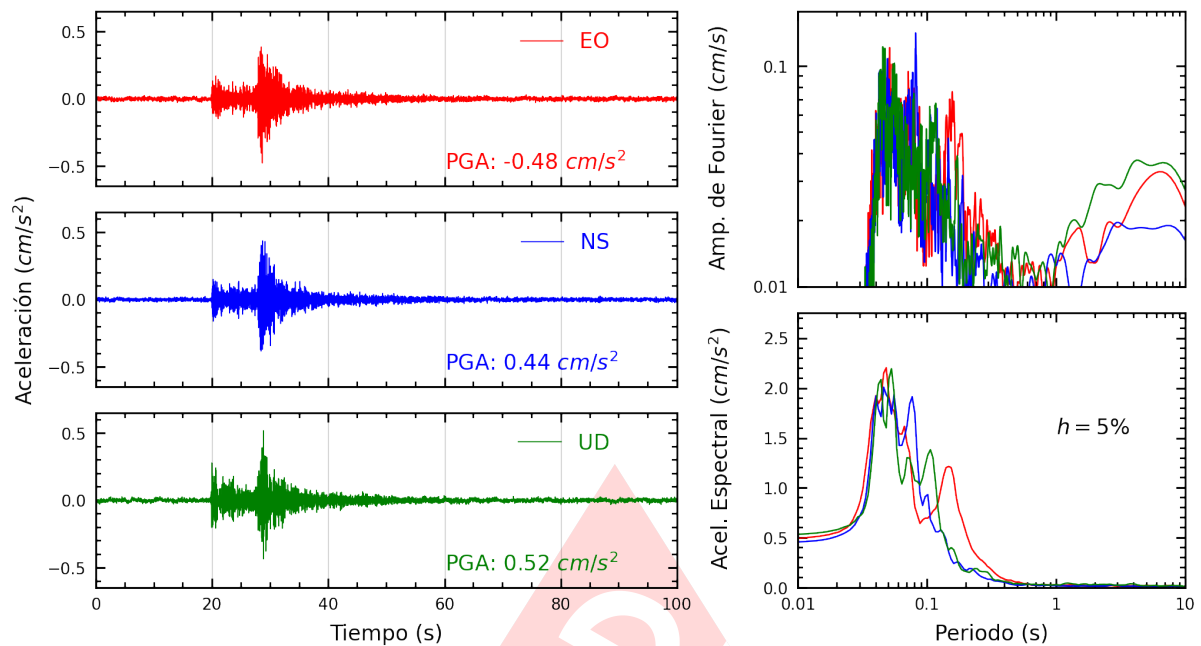
Figura A.27: Registros tiempo-historia, espectros de Fourier y de respuesta en las direcciones EO, NS y vertical de la estación UNMSM. Sismo de Ancon, Lima - Lima del 2024-11-15, 22:26:20 (Hora local)
