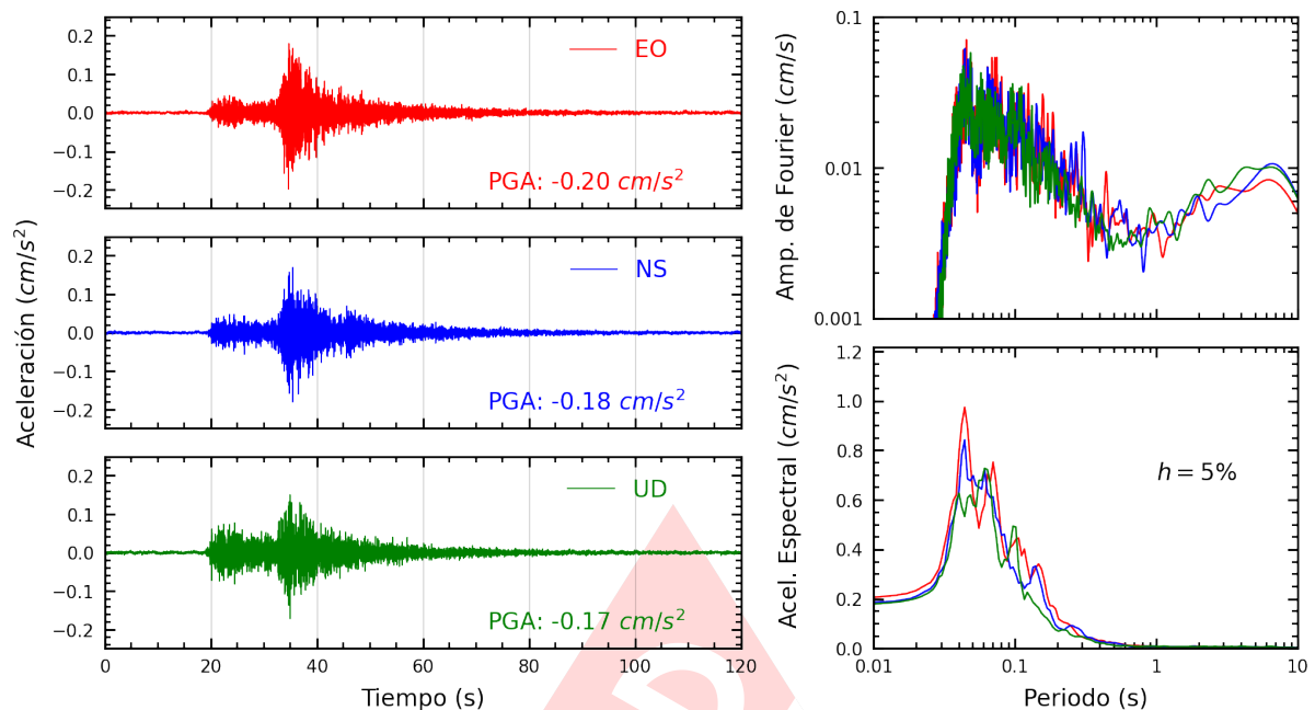
Figura A.31: Registros tiempo-historia, espectros de Fourier y de respuesta en las direcciones EO, NS y vertical de la estación CARAL. Sismo de Ancon, Lima - Lima del 2024-11-15, 22:26:20 (Hora local)
