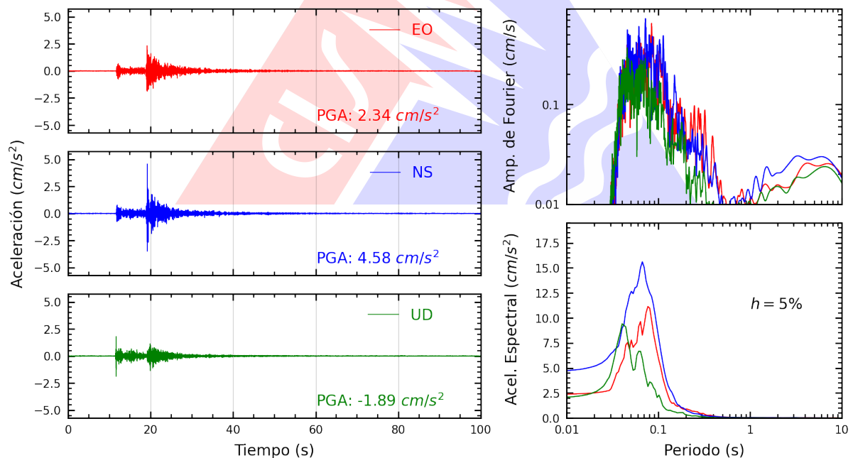
Figura A.2: Registros tiempo-historia, espectros de Fourier y de respuesta en las direcciones EO, NS y vertical de la estación DEFEN. Sismo de Ancon, Lima - Lima del 2024-11-15, 22:26:20 (Hora local)
