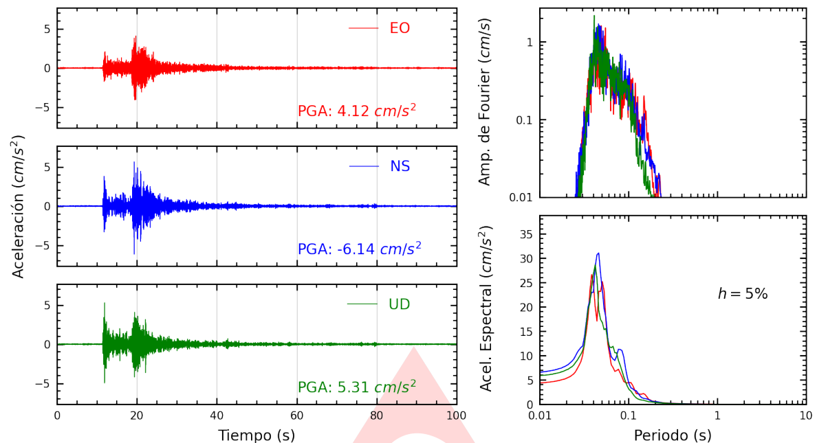
Figura A.1: Registros tiempo-historia, espectros de Fourier y de respuesta en las direcciones EO, NS y vertical de la estación SROS2. Sismo de Ancon, Lima - Lima del 2024-11-15, 22:26:20 (Hora local)
