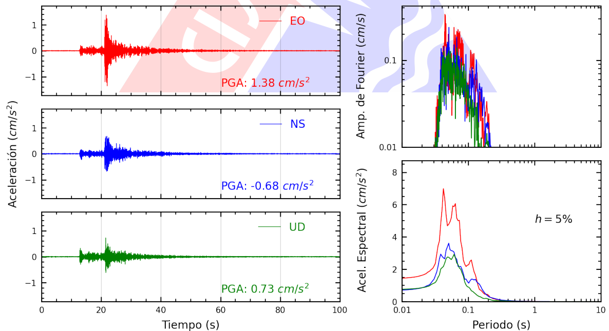
Figura A.14: Registros tiempo-historia, espectros de Fourier y de respuesta en las direcciones EO, NS y vertical de la estación ATARJ. Sismo de Ancon, Lima - Lima del 2024-11-15, 22:26:20 (Hora local)
