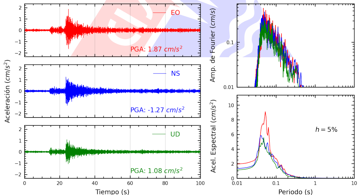
Figura A.10: Registros tiempo-historia, espectros de Fourier y de respuesta en las direcciones EO, NS y vertical de la estación UNTEL. Sismo de Ancon, Lima - Lima del 2024-11-15, 22:26:20 (Hora local)
