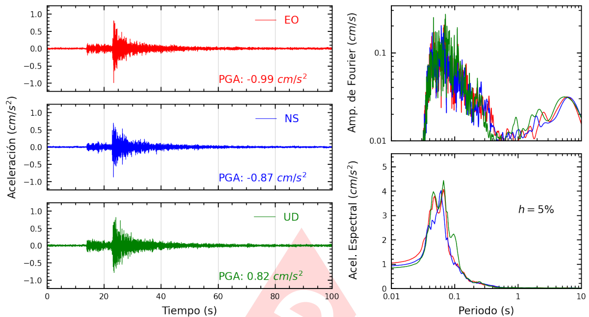
Figura A.17: Registros tiempo-historia, espectros de Fourier y de respuesta en las direcciones EO, NS y vertical de la estación SOVES. Sismo de Ancon, Lima - Lima del 2024-11-15, 22:26:20 (Hora local)
