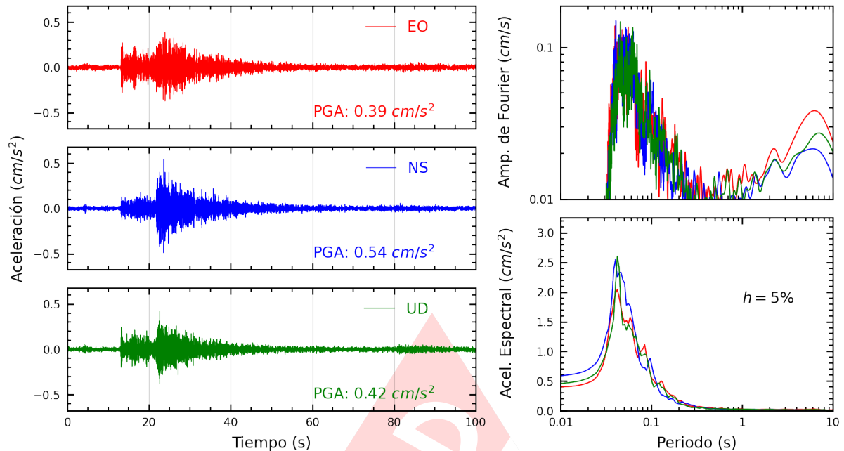
Figura A.23: Registros tiempo-historia, espectros de Fourier y de respuesta en las direcciones EO, NS y vertical de la estación IMCA. Sismo de Ancon, Lima - Lima del 2024-11-15, 22:26:20 (Hora local)
