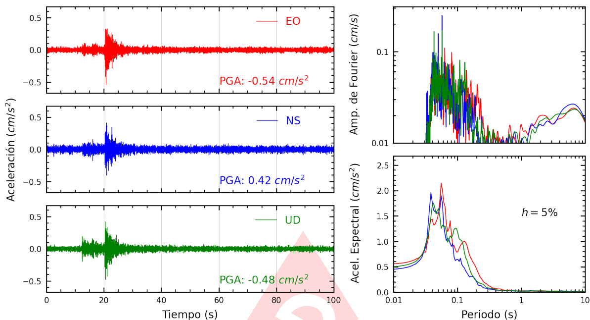
Figura A.25: Registros tiempo-historia, espectros de Fourier y de respuesta en las direcciones EO, NS y vertical de la estación BONDY. Sismo de Ancon, Lima - Lima del 2024-11-15, 22:26:20 (Hora local)
