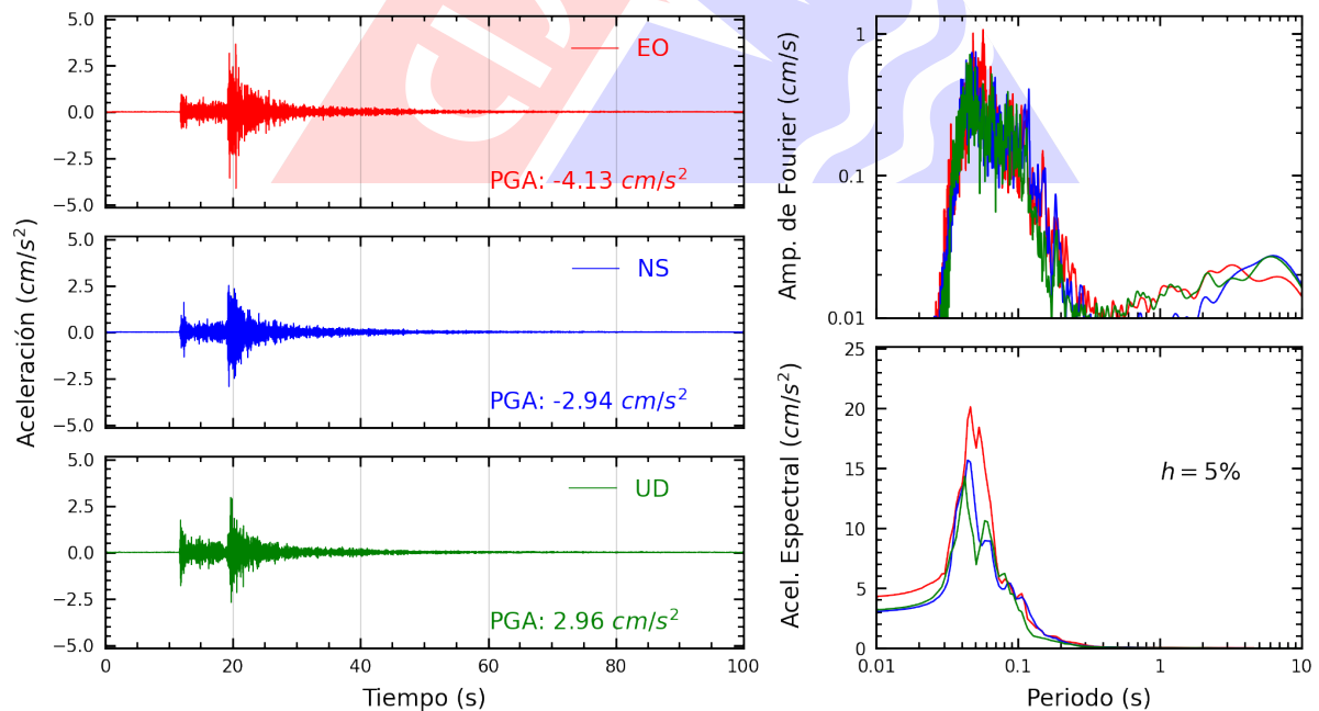
Figura A.4: Registros tiempo-historia, espectros de Fourier y de respuesta en las direcciones EO, NS y vertical de la estación AMORE. Sismo de Ancon, Lima - Lima del 2024-11-15, 22:26:20 (Hora local)
