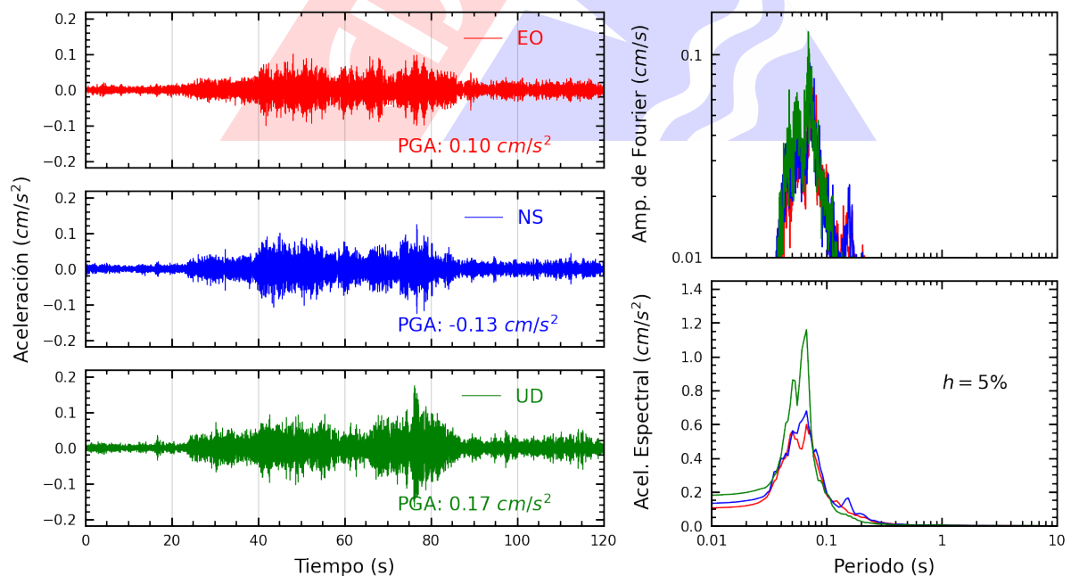
Figura A.32: Registros tiempo-historia, espectros de Fourier y de respuesta en las direcciones EO, NS y vertical de la estación ASIA. Sismo de Ancon, Lima - Lima del 2024-11-15, 22:26:20 (Hora local)
