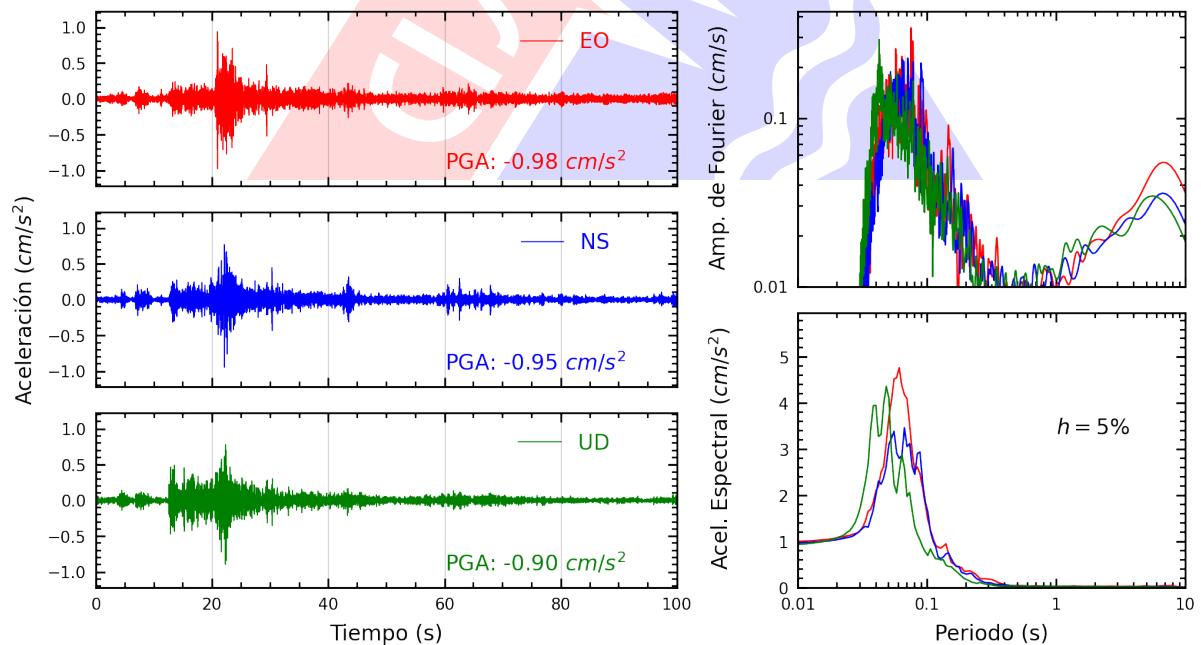
Figura A.18: Registros tiempo-historia, espectros de Fourier y de respuesta en las direcciones EO, NS y vertical de la estación UPCSM. Sismo de Ancon, Lima - Lima del 2024-11-15, 22:26:20 (Hora local)
