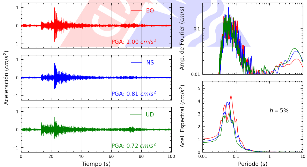
Figura A.16: Registros tiempo-historia, espectros de Fourier y de respuesta en las direcciones EO, NS y vertical de la estación URPE. Sismo de Ancon, Lima - Lima del 2024-11-15, 22:26:20 (Hora local)
