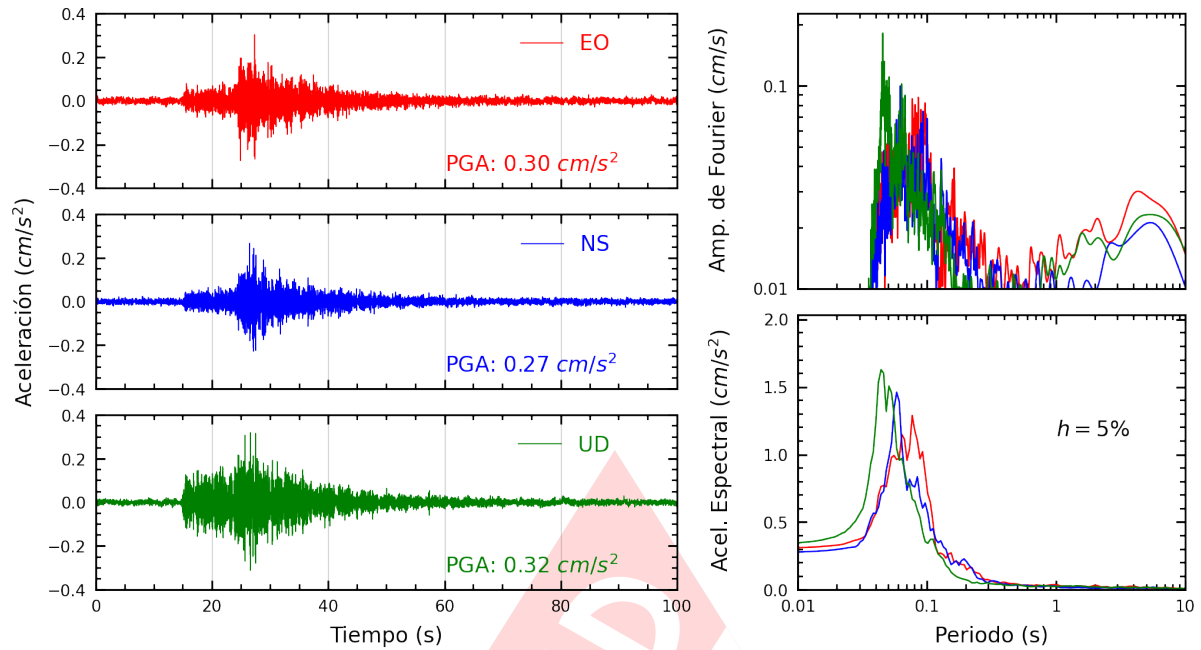
Figura A.29: Registros tiempo-historia, espectros de Fourier y de respuesta en las direcciones EO, NS y vertical de la estación USILP. Sismo de Ancon, Lima - Lima del 2024-11-15, 22:26:20 (Hora local)
