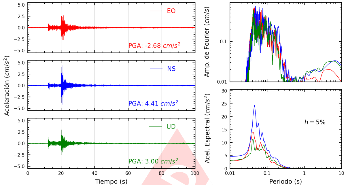
Figura A.3: Registros tiempo-historia, espectros de Fourier y de respuesta en las direcciones EO, NS y vertical de la estación INDEP. Sismo de Ancon, Lima - Lima del 2024-11-15, 22:26:20 (Hora local)
