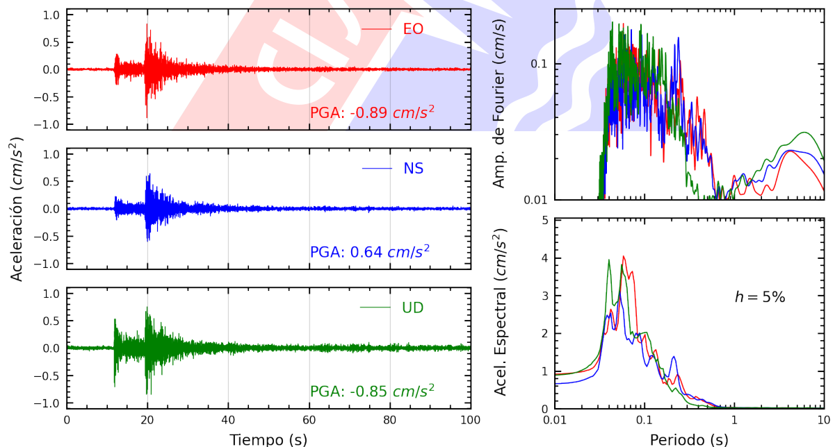
Figura A.20: Registros tiempo-historia, espectros de Fourier y de respuesta en las direcciones EO, NS y vertical de la estación MDPP. Sismo de Ancon, Lima - Lima del 2024-11-15, 22:26:20 (Hora local)
