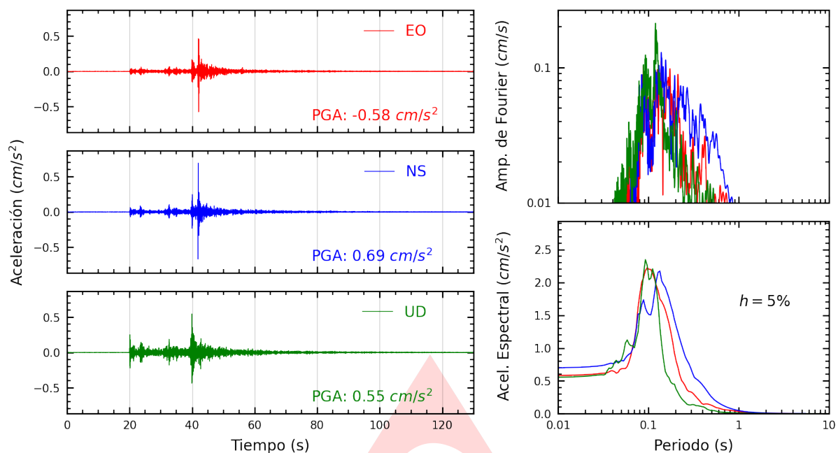
Figura A.1: Registros tiempo-historia, espectros de Fourier y de respuesta en las direcciones EO, NS y vertical de la estación UNIA. Sismo de Uchiza, Tocache - San Martin del 2024-11-20, 00:25:59 (Hora local)
