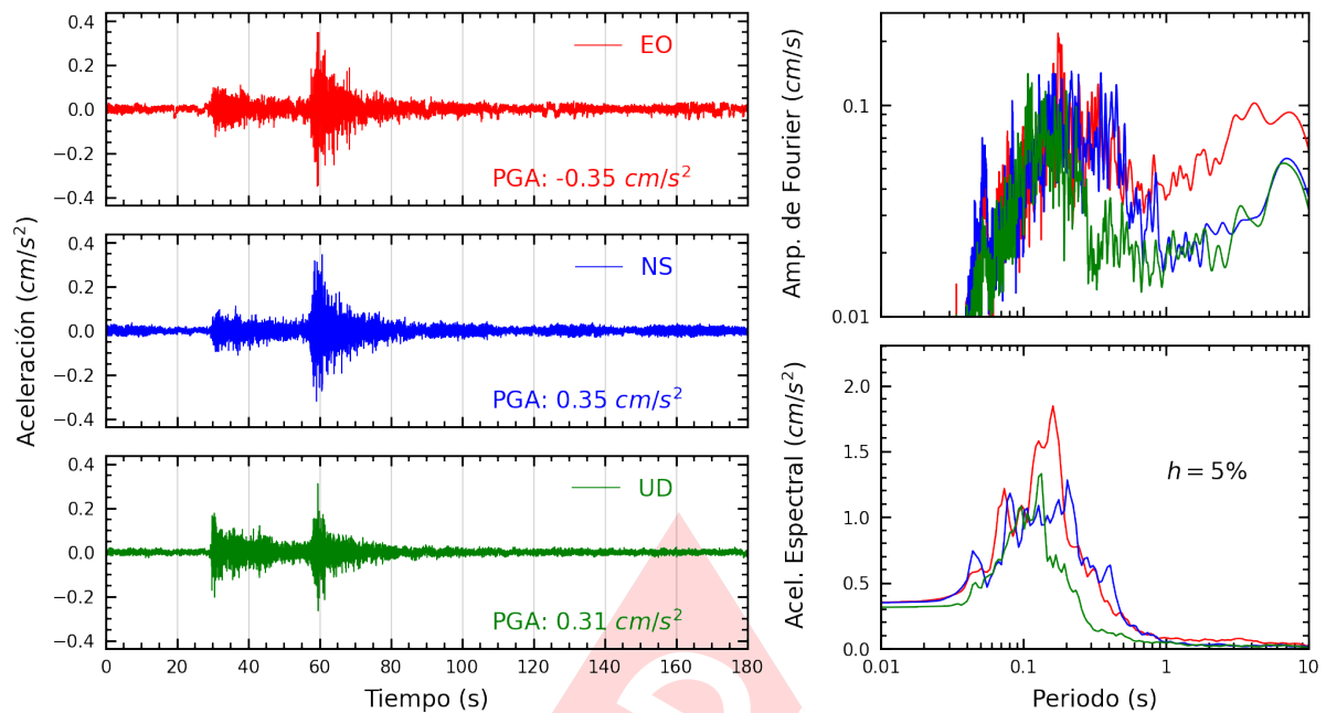
Figura A.7: Registros tiempo-historia, espectros de Fourier y de respuesta en las direcciones EO, NS y vertical de la estación UNAB. Sismo de Huancabamba, Oxapampa - Pasco del 2024-11-22, 04:24:07 (Hora local)
