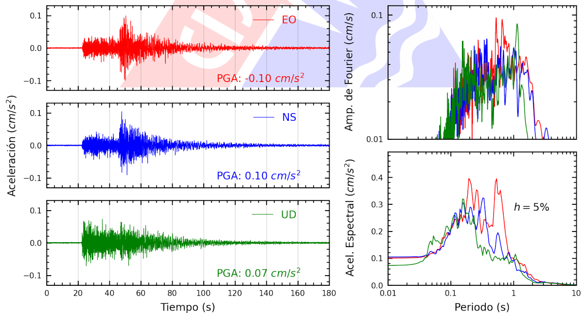
Figura A.30: Registros tiempo-historia, espectros de Fourier y de respuesta en las direcciones EO, NS y vertical de la estación UNCP. Sismo de Huancabamba, Oxapampa - Pasco del 2024-11-22, 04:24:07 (Hora local)
