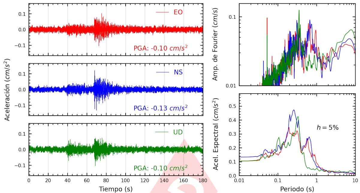
Figura A.25: Registros tiempo-historia, espectros de Fourier y de respuesta en las direcciones EO, NS y vertical de la estación UNMSM. Sismo de Huancabamba, Oxapampa - Pasco del 2024-11-22, 04:24:07 (Hora local)
