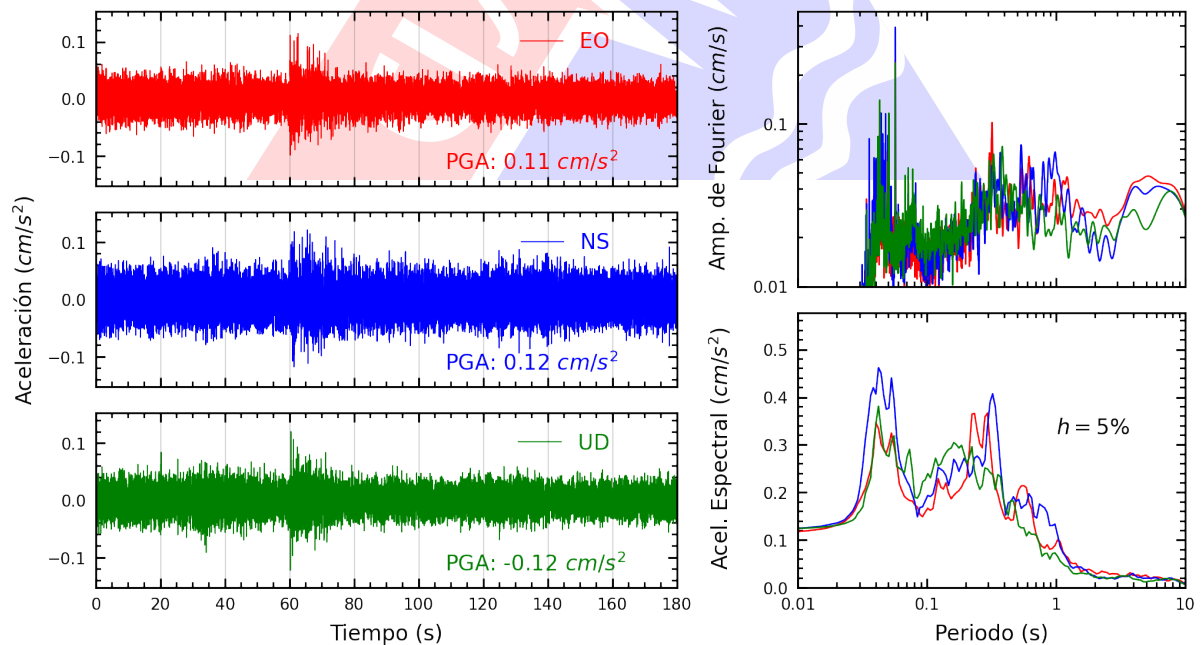
Figura A.28: Registros tiempo-historia, espectros de Fourier y de respuesta en las direcciones EO, NS y vertical de la estación BONDY. Sismo de Huancabamba, Oxapampa - Pasco del 2024-11-22, 04:24:07 (Hora local)
