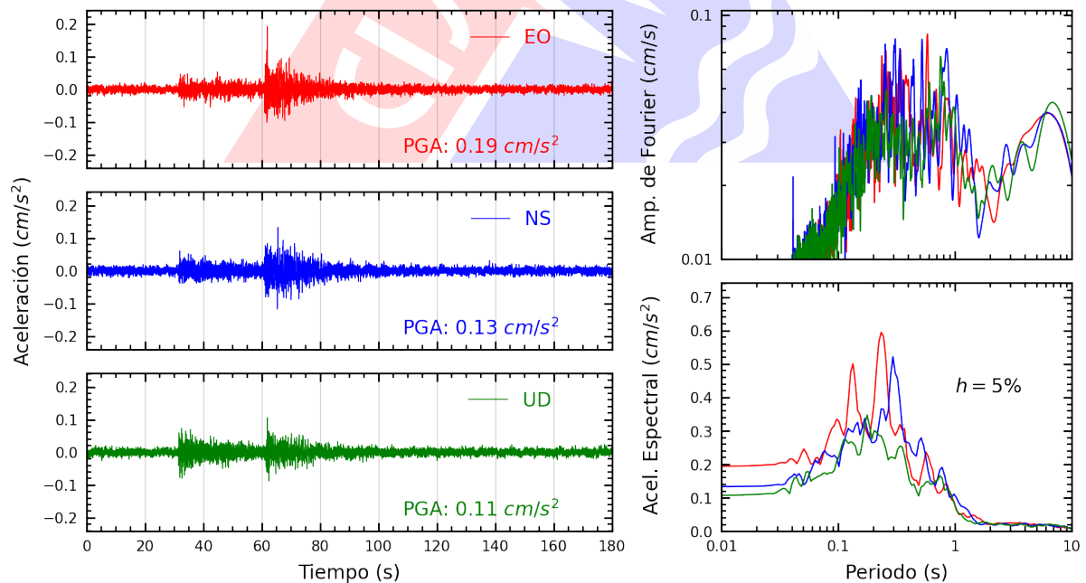
Figura A.18: Registros tiempo-historia, espectros de Fourier y de respuesta en las direcciones EO, NS y vertical de la estación SERVI. Sismo de Huancabamba, Oxapampa - Pasco del 2024-11-22, 04:24:07 (Hora local)
