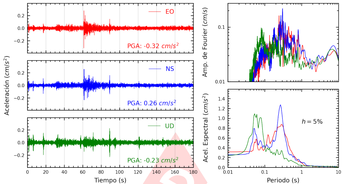
Figura A.9: Registros tiempo-historia, espectros de Fourier y de respuesta en las direcciones EO, NS y vertical de la estación RAMON. Sismo de Huancabamba, Oxapampa - Pasco del 2024-11-22, 04:24:07 (Hora local)
