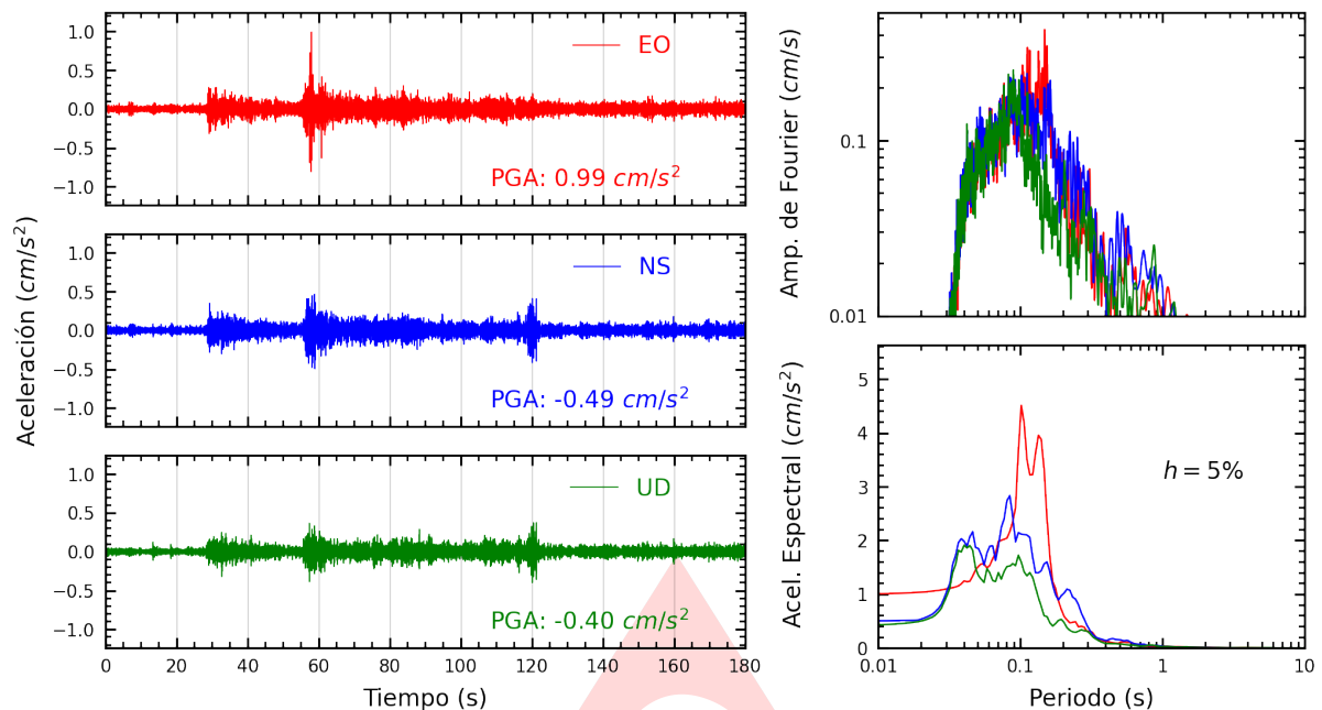
Figura A.1: Registros tiempo-historia, espectros de Fourier y de respuesta en las direcciones EO, NS y vertical de la estación SROS2. Sismo de Huancabamba, Oxapampa - Pasco del 2024-11-22, 04:24:07 (Hora local)
