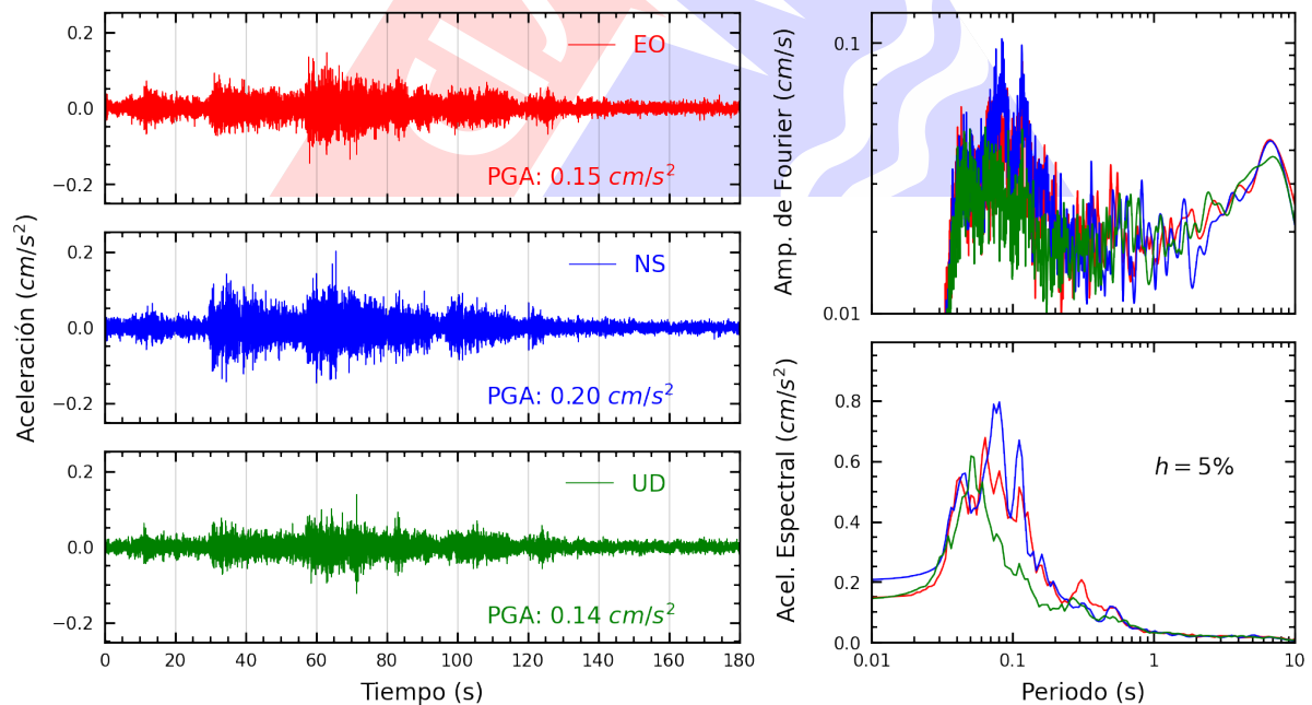
Figura A.16: Registros tiempo-historia, espectros de Fourier y de respuesta en las direcciones EO, NS y vertical de la estación JOSEO. Sismo de Huancabamba, Oxapampa - Pasco del 2024-11-22, 04:24:07 (Hora local)
