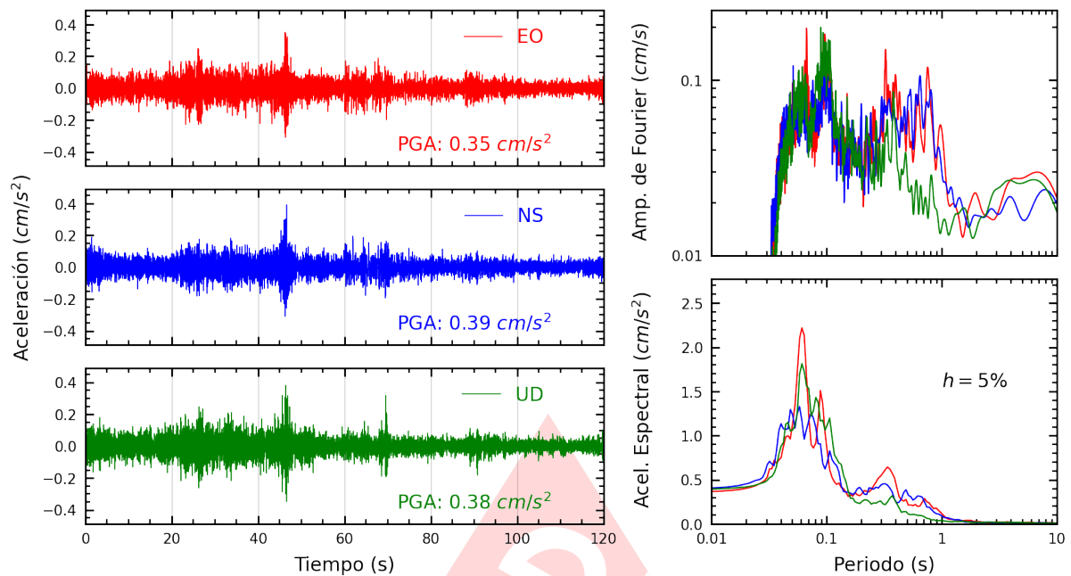
Figura A.5: Registros tiempo-historia, espectros de Fourier y de respuesta en las direcciones EO, NS y vertical de la estación MADRE. Sismo de Huancabamba, Oxapampa - Pasco del 2024-11-22, 04:24:07 (Hora local)
