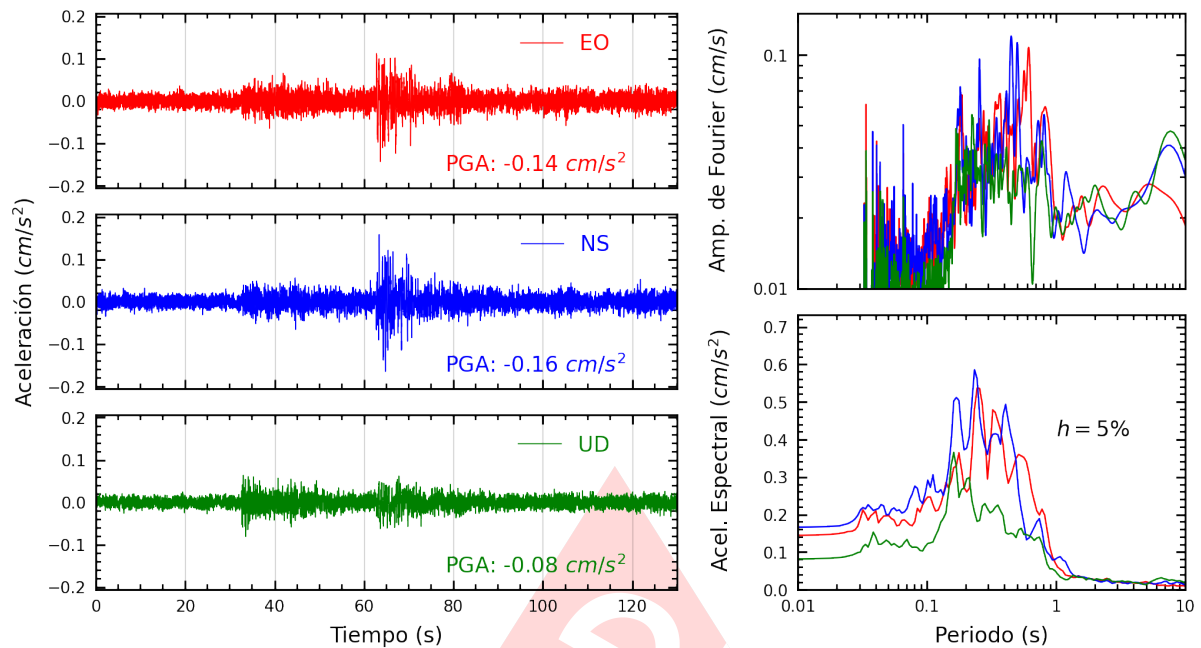
Figura A.21: Registros tiempo-historia, espectros de Fourier y de respuesta en las direcciones EO, NS y vertical de la estación UPCVI. Sismo de Huancabamba, Oxapampa - Pasco del 2024-11-22, 04:24:07 (Hora local)
