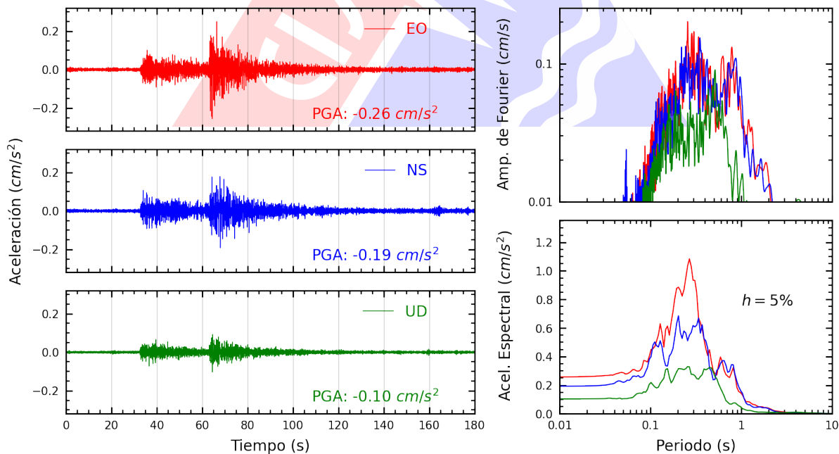
Figura A.14: Registros tiempo-historia, espectros de Fourier y de respuesta en las direcciones EO, NS y vertical de la estación BRISA. Sismo de Huancabamba, Oxapampa - Pasco del 2024-11-22, 04:24:07 (Hora local)
