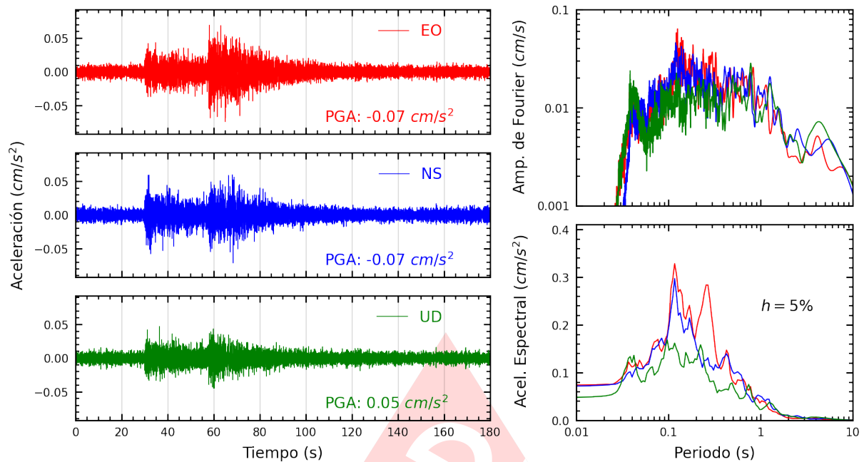
Figura A.33: Registros tiempo-historia, espectros de Fourier y de respuesta en las direcciones EO, NS y vertical de la estación ATARJ. Sismo de Huancabamba, Oxapampa - Pasco del 2024-11-22, 04:24:07 (Hora local)
