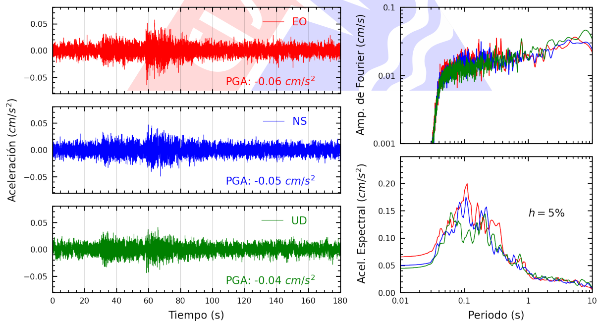
Figura A.34: Registros tiempo-historia, espectros de Fourier y de respuesta en las direcciones EO, NS y vertical de la estación UCSS. Sismo de Huancabamba, Oxapampa - Pasco del 2024-11-22, 04:24:07 (Hora local)
