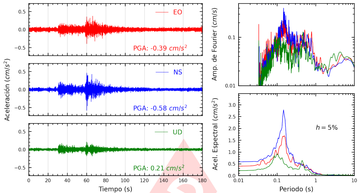
Figura A.3: Registros tiempo-historia, espectros de Fourier y de respuesta en las direcciones EO, NS y vertical de la estación USILM. Sismo de Huancabamba, Oxapampa - Pasco del 2024-11-22, 04:24:07 (Hora local)
