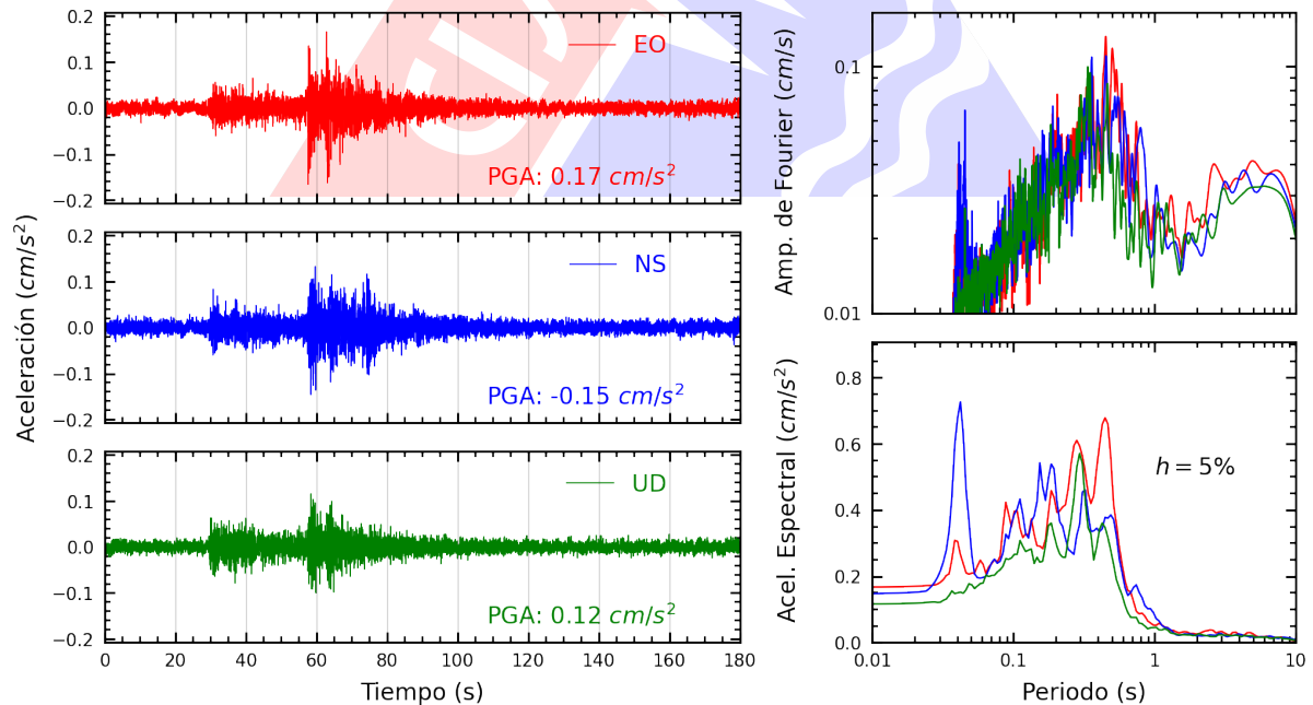
Figura A.20: Registros tiempo-historia, espectros de Fourier y de respuesta en las direcciones EO, NS y vertical de la estación COMAS. Sismo de Huancabamba, Oxapampa - Pasco del 2024-11-22, 04:24:07 (Hora local)
