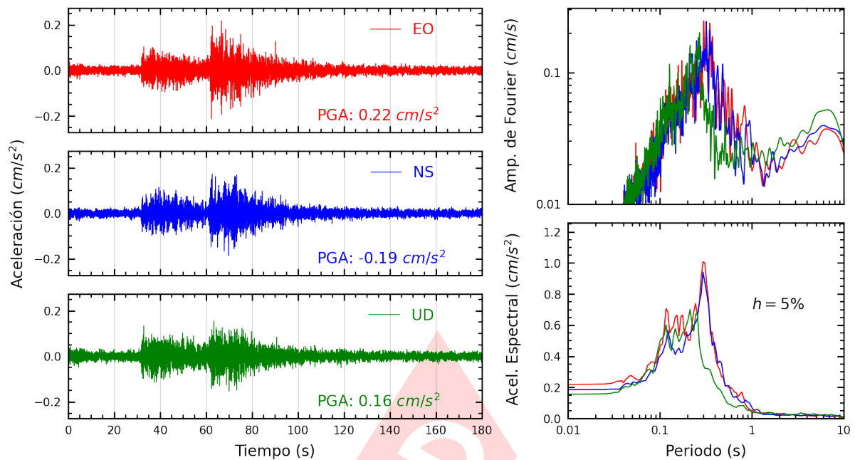
Figura A.15: Registros tiempo-historia, espectros de Fourier y de respuesta en las direcciones EO, NS y vertical de la estación SOVES. Sismo de Huancabamba, Oxapampa - Pasco del 2024-11-22, 04:24:07 (Hora local)
