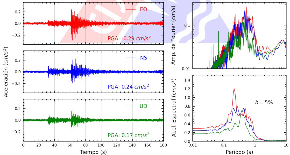
Figura A.12: Registros tiempo-historia, espectros de Fourier y de respuesta en las direcciones EO, NS y vertical de la estación USILP. Sismo de Huancabamba, Oxapampa - Pasco del 2024-11-22, 04:24:07 (Hora local)
