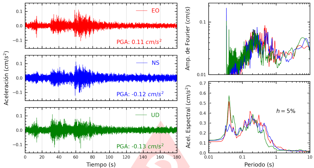
Figura A.27: Registros tiempo-historia, espectros de Fourier y de respuesta en las direcciones EO, NS y vertical de la estación USMP. Sismo de Huancabamba, Oxapampa - Pasco del 2024-11-22, 04:24:07 (Hora local)
