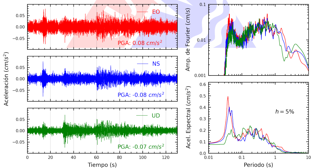
Figura A.32: Registros tiempo-historia, espectros de Fourier y de respuesta en las direcciones EO, NS y vertical de la estación BORJA. Sismo de Huancabamba, Oxapampa - Pasco del 2024-11-22, 04:24:07 (Hora local)
