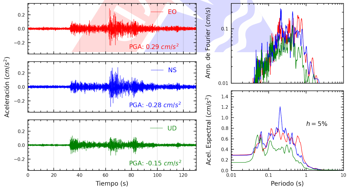
Figura A.10: Registros tiempo-historia, espectros de Fourier y de respuesta en las direcciones EO, NS y vertical de la estación SCCHO. Sismo de Huancabamba, Oxapampa - Pasco del 2024-11-22, 04:24:07 (Hora local)
