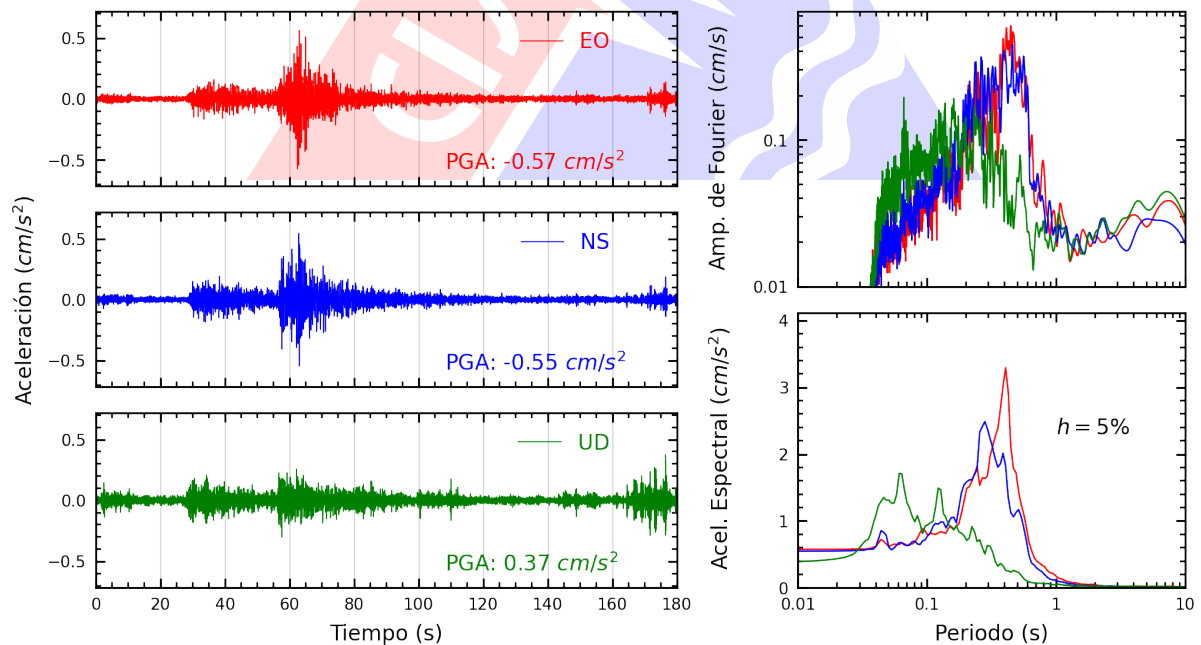
Figura A.4: Registros tiempo-historia, espectros de Fourier y de respuesta en las direcciones EO, NS y vertical de la estación MDPP. Sismo de Huancabamba, Oxapampa - Pasco del 2024-11-22, 04:24:07 (Hora local)
