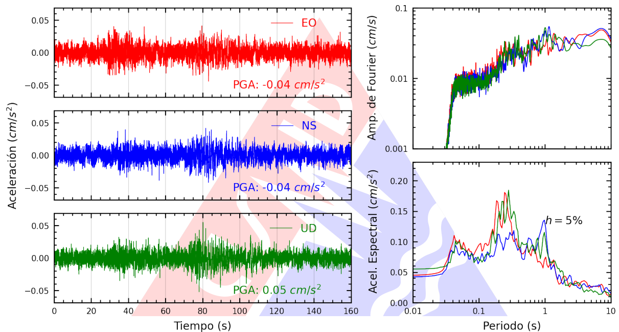
Figura A.35: Registros tiempo-historia, espectros de Fourier y de respuesta en las direcciones EO, NS y vertical de la estación UNSCH. Sismo de Huancabamba, Oxapampa - Pasco del 2024-11-22, 04:24:07 (Hora local)
