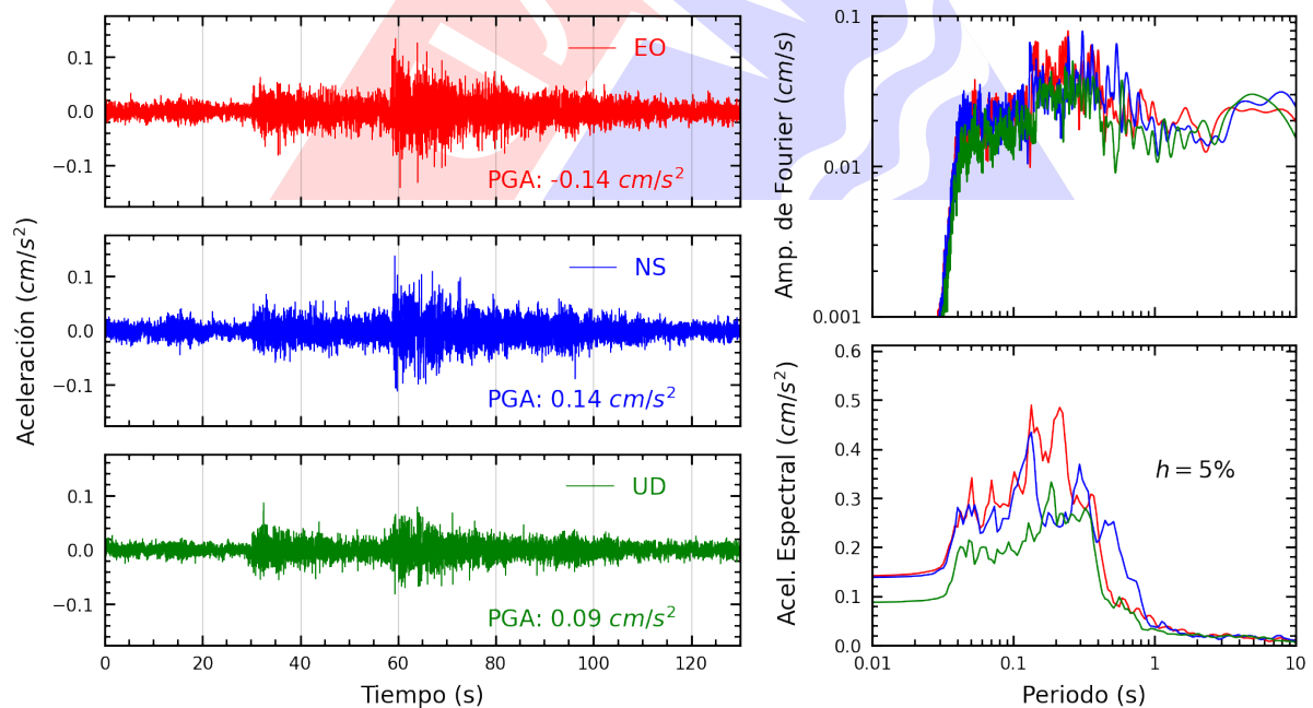
Figura A.24: Registros tiempo-historia, espectros de Fourier y de respuesta en las direcciones EO, NS y vertical de la estación FICPE. Sismo de Huancabamba, Oxapampa - Pasco del 2024-11-22, 04:24:07 (Hora local)
