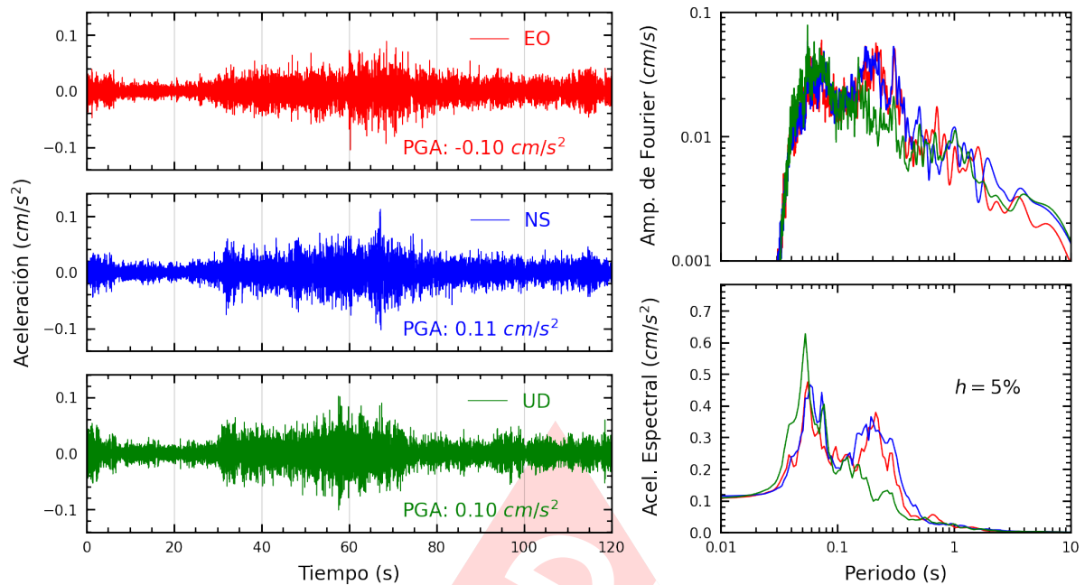
Figura A.29: Registros tiempo-historia, espectros de Fourier y de respuesta en las direcciones EO, NS y vertical de la estación ASIA. Sismo de Huancabamba, Oxapampa - Pasco del 2024-11-22, 04:24:07 (Hora local)
