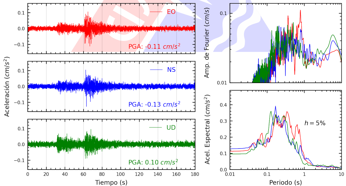
Figura A.26: Registros tiempo-historia, espectros de Fourier y de respuesta en las direcciones EO, NS y vertical de la estación UNFV. Sismo de Huancabamba, Oxapampa - Pasco del 2024-11-22, 04:24:07 (Hora local)
