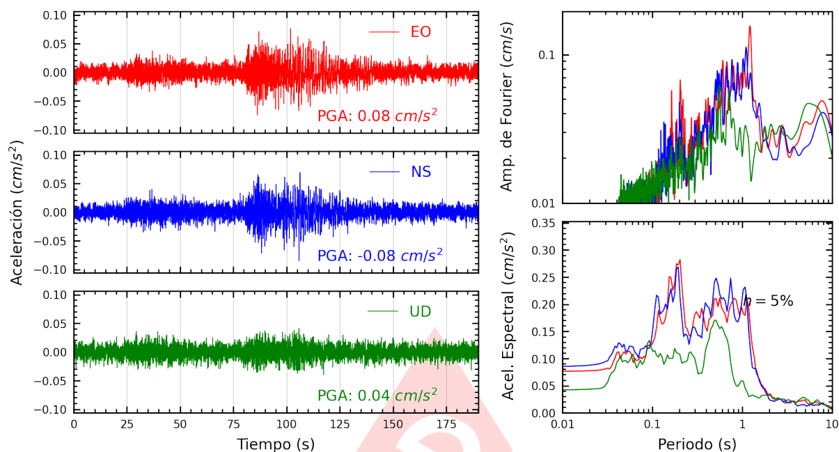
Figura A.31: Registros tiempo-historia, espectros de Fourier y de respuesta en las direcciones EO, NS y vertical de la estación UNTRM. Sismo de Huancabamba, Oxapampa - Pasco del 2024-11-22, 04:24:07 (Hora local)
