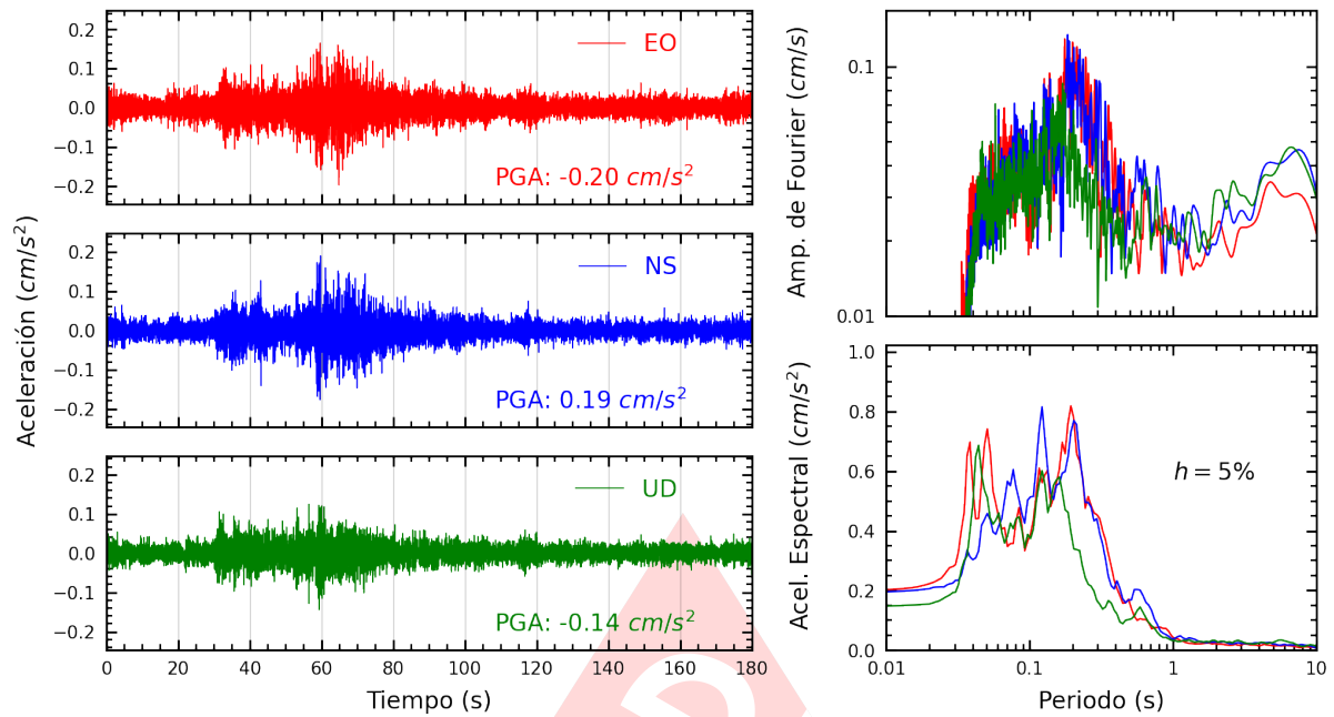
Figura A.17: Registros tiempo-historia, espectros de Fourier y de respuesta en las direcciones EO, NS y vertical de la estación INDEP. Sismo de Huancabamba, Oxapampa - Pasco del 2024-11-22, 04:24:07 (Hora local)
