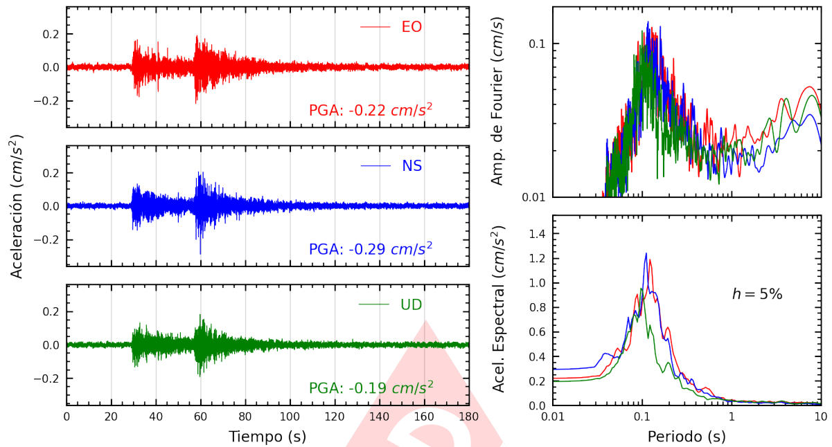
Figura A.11: Registros tiempo-historia, espectros de Fourier y de respuesta en las direcciones EO, NS y vertical de la estación AMORE. Sismo de Huancabamba, Oxapampa - Pasco del 2024-11-22, 04:24:07 (Hora local)
