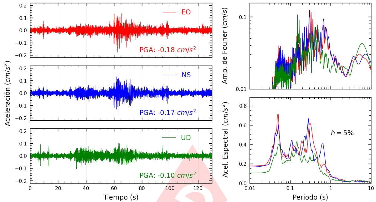
Figura A.19: Registros tiempo-historia, espectros de Fourier y de respuesta en las direcciones EO, NS y vertical de la estación UPCSM. Sismo de Huancabamba, Oxapampa - Pasco del 2024-11-22, 04:24:07 (Hora local)
