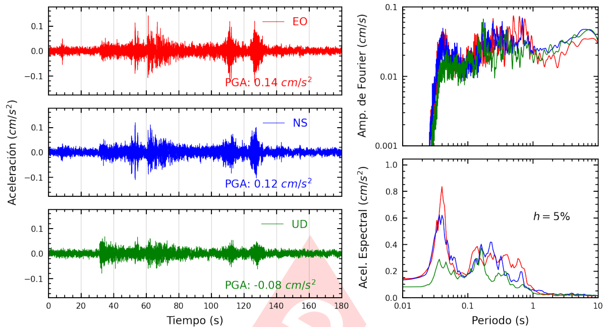
Figura A.23: Registros tiempo-historia, espectros de Fourier y de respuesta en las direcciones EO, NS y vertical de la estación CEPRE. Sismo de Huancabamba, Oxapampa - Pasco del 2024-11-22, 04:24:07 (Hora local)
