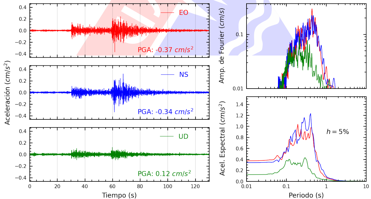
Figura A.6: Registros tiempo-historia, espectros de Fourier y de respuesta en las direcciones EO, NS y vertical de la estación VHAY2. Sismo de Huancabamba, Oxapampa - Pasco del 2024-11-22, 04:24:07 (Hora local)
