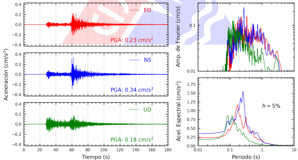
Figura A.8: Registros tiempo-historia, espectros de Fourier y de respuesta en las direcciones EO, NS y vertical de la estación UNIA. Sismo de Huancabamba, Oxapampa - Pasco del 2024-11-22, 04:24:07 (Hora local)
