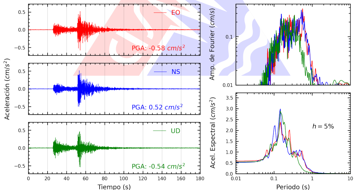
Figura A.2: Registros tiempo-historia, espectros de Fourier y de respuesta en las direcciones EO, NS y vertical de la estación CARAL. Sismo de Huancabamba, Oxapampa - Pasco del 2024-11-22, 04:24:07 (Hora local)
