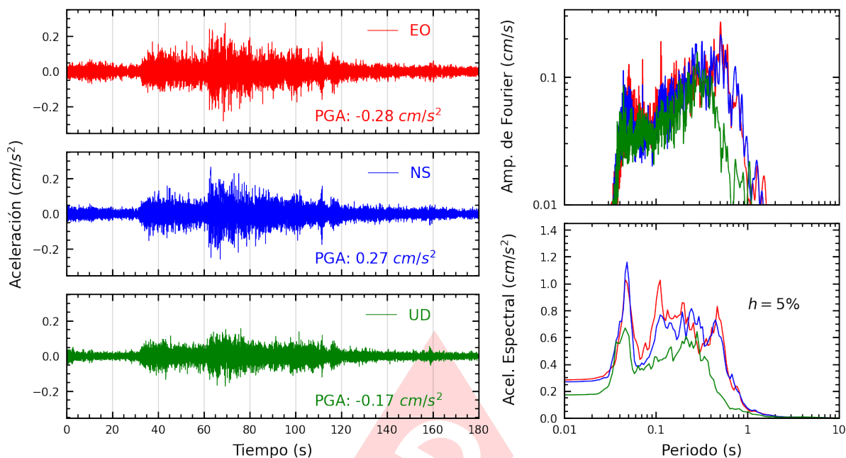
Figura A.13: Registros tiempo-historia, espectros de Fourier y de respuesta en las direcciones EO, NS y vertical de la estación UNTEL. Sismo de Huancabamba, Oxapampa - Pasco del 2024-11-22, 04:24:07 (Hora local)
