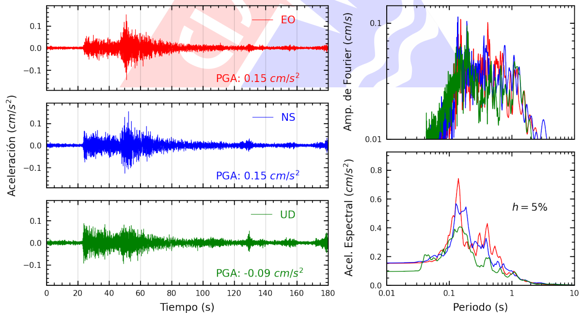
Figura A.22: Registros tiempo-historia, espectros de Fourier y de respuesta en las direcciones EO, NS y vertical de la estación SCHYO. Sismo de Huancabamba, Oxapampa - Pasco del 2024-11-22, 04:24:07 (Hora local)
