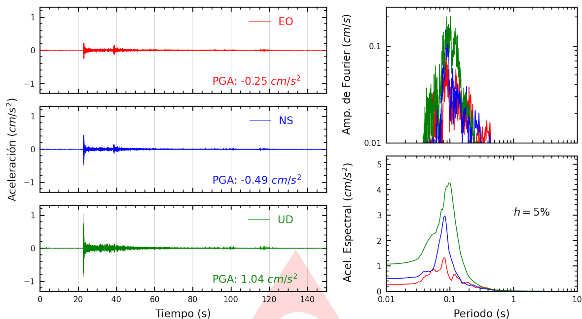
Figura A.1: Registros tiempo-historia, espectros de Fourier y de respuesta en las direcciones EO, NS y vertical de la estación UNIA. Sismo de Puerto Inca, Puerto Inca - Huanuco del 2024-11-23, 05:23:50 (Hora local)
