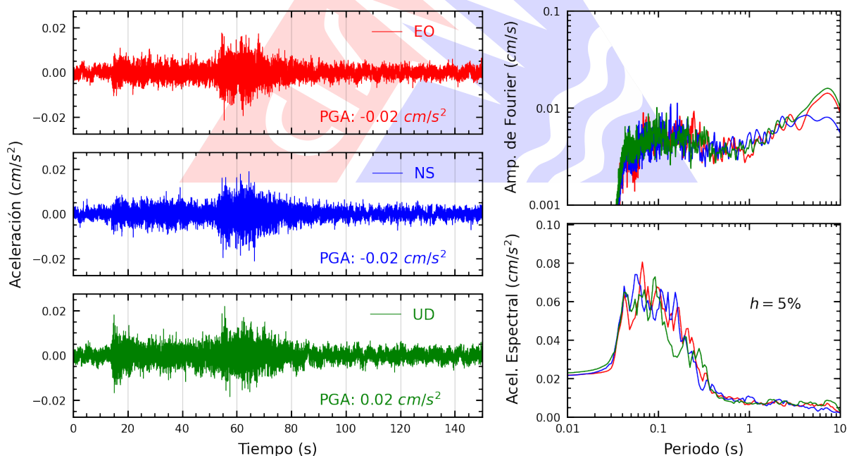
Figura A.2: Registros tiempo-historia, espectros de Fourier y de respuesta en las direcciones EO, NS y vertical de la estación CARAL. Sismo de Puerto Inca, Puerto Inca - Huanuco del 2024-11-23, 05:23:50 (Hora local)
