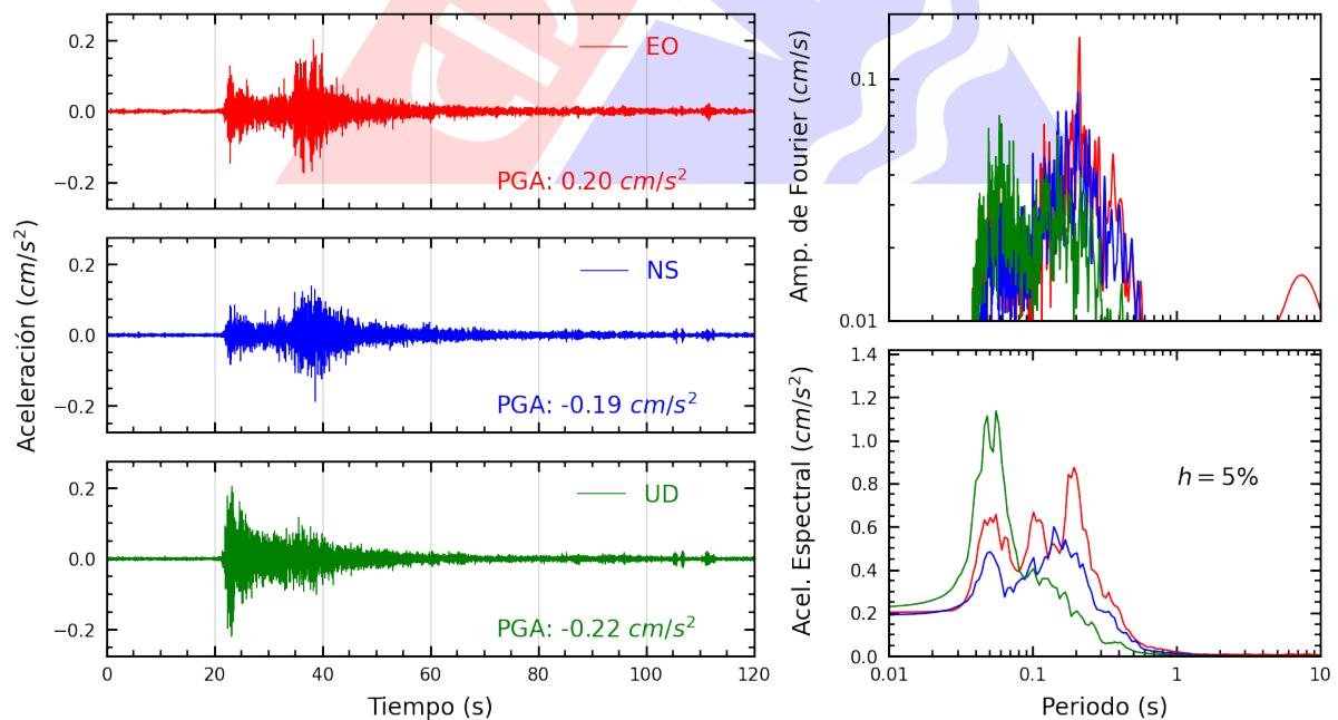
Figura A.4: Registros tiempo-historia, espectros de Fourier y de respuesta en las direcciones EO, NS y vertical de la estación SCCHL. Sismo de Sechura, Sechura - Piura del 2024-11-23, 14:25:42 (Hora local)
