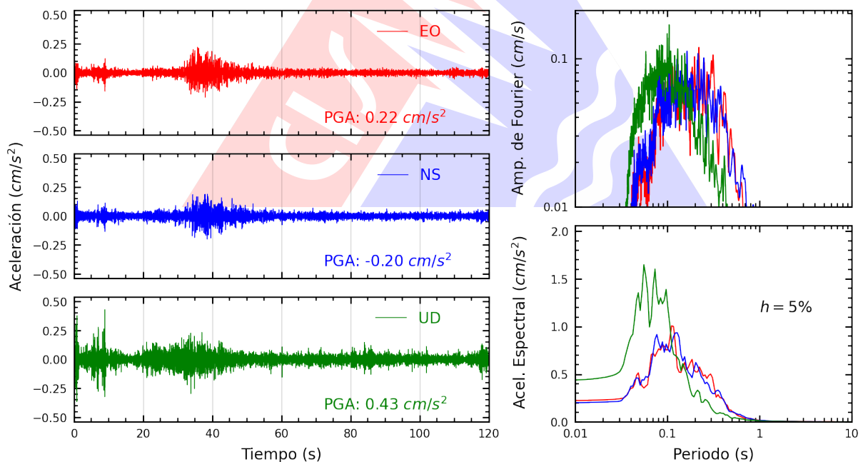
Figura A.2: Registros tiempo-historia, espectros de Fourier y de respuesta en las direcciones EO, NS y vertical de la estación UNP. Sismo de Sechura, Sechura - Piura del 2024-11-23, 14:25:42 (Hora local)
