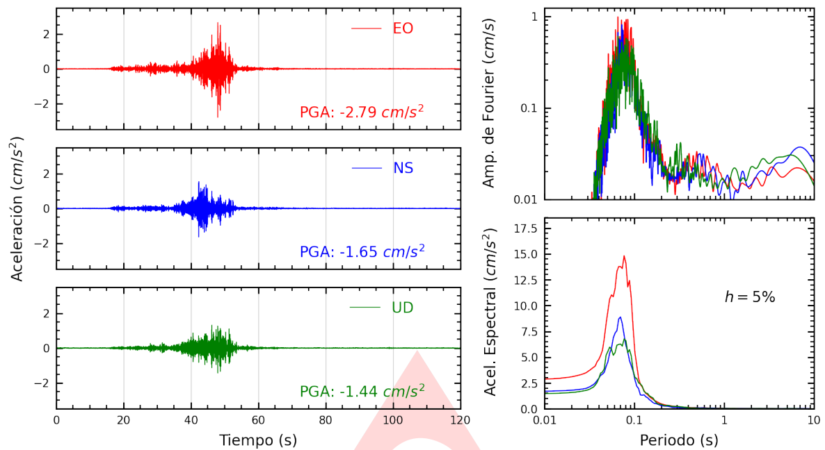
Figura A.1: Registros tiempo-historia, espectros de Fourier y de respuesta en las direcciones EO, NS y vertical de la estación UNTRM. Sismo de Sechura, Sechura - Piura del 2024-11-23, 14:25:42 (Hora local)
