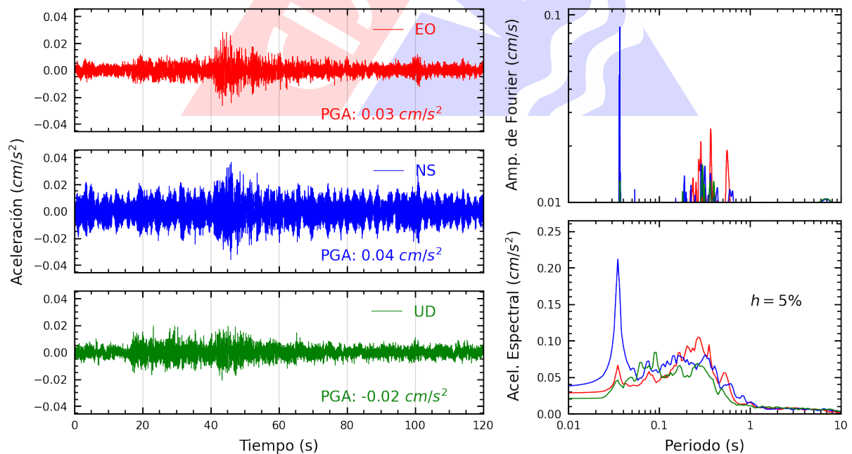
Figura A.8: Registros tiempo-historia, espectros de Fourier y de respuesta en las direcciones EO, NS y vertical de la estación UNJ. Sismo de Sechura, Sechura - Piura del 2024-11-23, 14:25:42 (Hora local)
