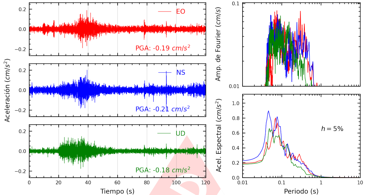
Figura A.5: Registros tiempo-historia, espectros de Fourier y de respuesta en las direcciones EO, NS y vertical de la estación UPAOP. Sismo de Sechura, Sechura - Piura del 2024-11-23, 14:25:42 (Hora local)
