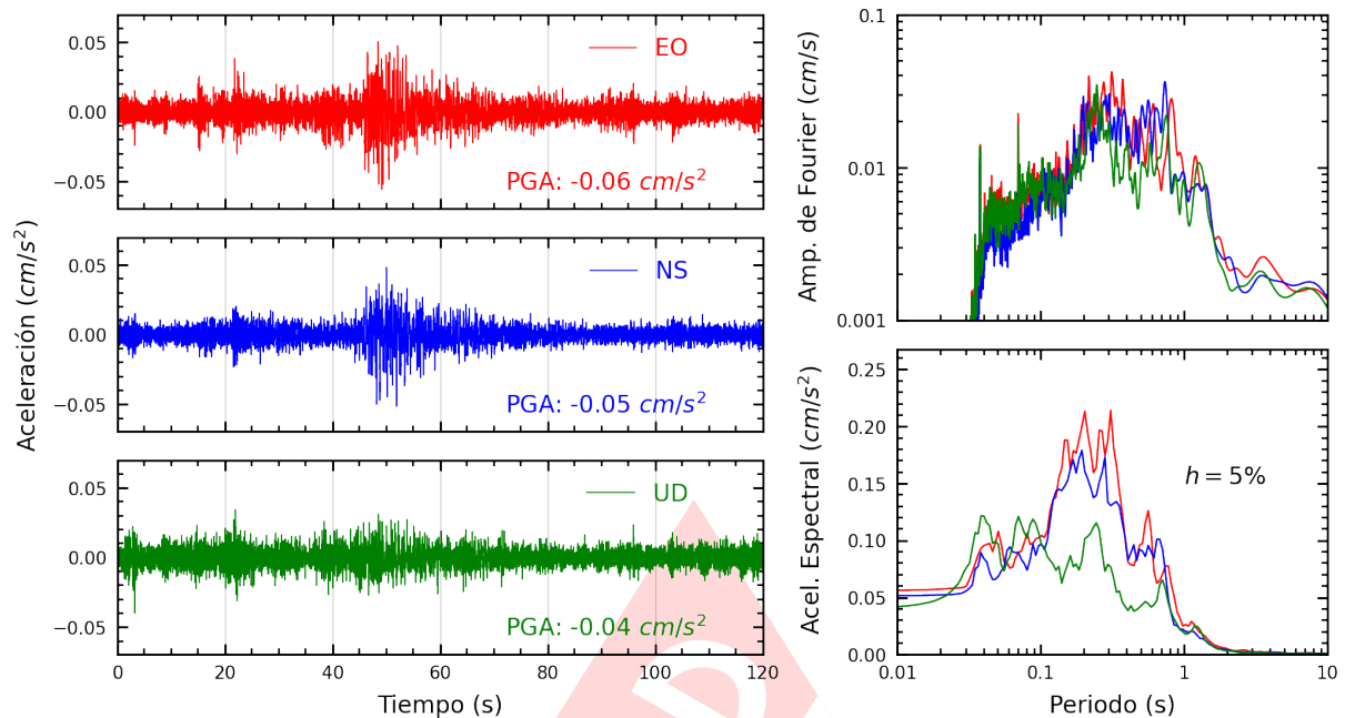
Figura A.7: Registros tiempo-historia, espectros de Fourier y de respuesta en las direcciones EO, NS y vertical de la estación UNC. Sismo de Sechura, Sechura - Piura del 2024-11-23, 14:25:42 (Hora local)
