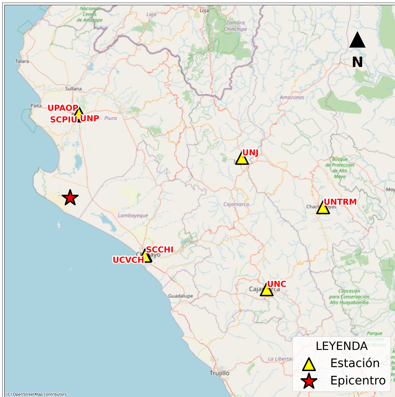
Figura 2: Mapa de ubicación de la(s) estación(es) acelerográfica(s) correspondiente(s) al Sismo de Sechura, Sechura - Piura del 23 de noviembre de 2024 a las 14:25:42 (hora local)
