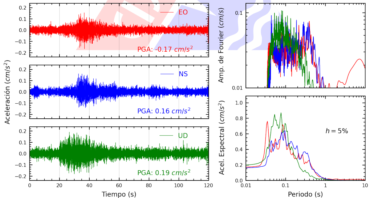
Figura A.6: Registros tiempo-historia, espectros de Fourier y de respuesta en las direcciones EO, NS y vertical de la estación SCPIU. Sismo de Sechura, Sechura - Piura del 2024-11-23, 14:25:42 (Hora local)
