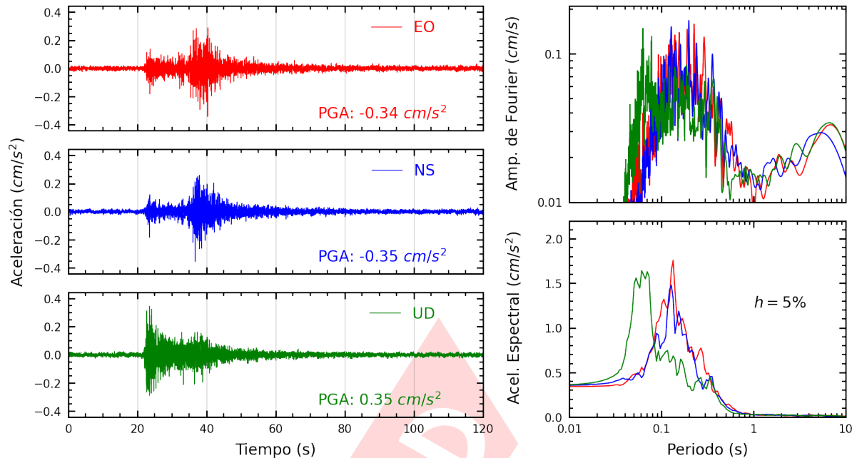
Figura A.3: Registros tiempo-historia, espectros de Fourier y de respuesta en las direcciones EO, NS y vertical de la estación UCVCH. Sismo de Sechura, Sechura - Piura del 2024-11-23, 14:25:42 (Hora local)
