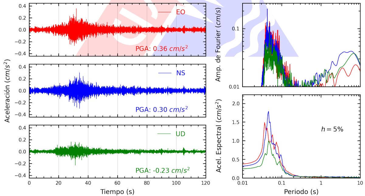
Figura A.18: Registros tiempo-historia, espectros de Fourier y de respuesta en las direcciones EO, NS y vertical de la estación CEPRE. Sismo de Mala, Cañete - Lima del 2024-11-24, 21:51:22 (Hora local)
