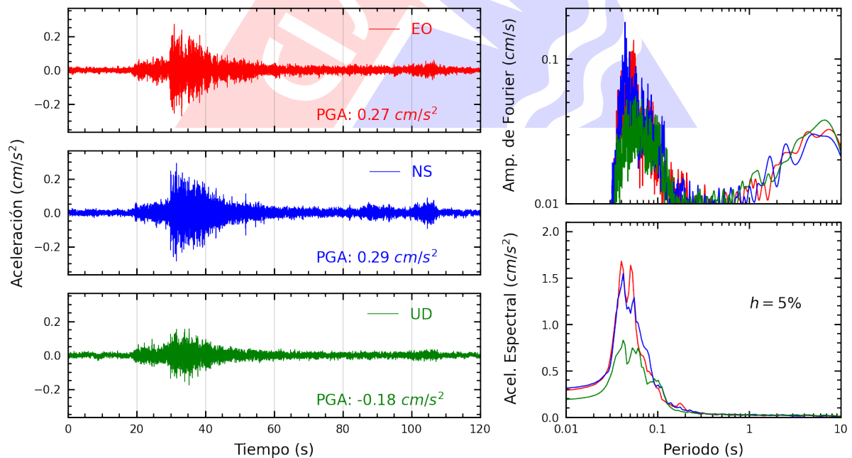
Figura A.24: Registros tiempo-historia, espectros de Fourier y de respuesta en las direcciones EO, NS y vertical de la estación COMAS. Sismo de Mala, Cañete - Lima del 2024-11-24, 21:51:22 (Hora local)
