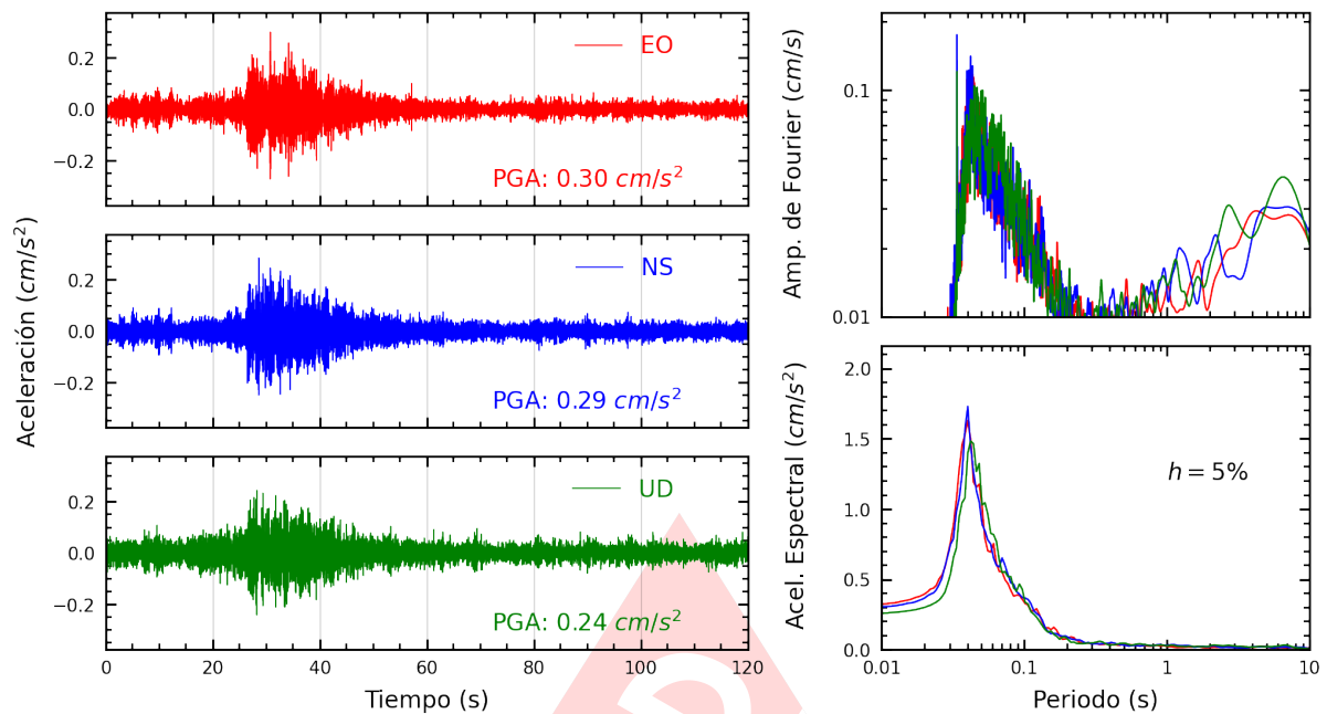
Figura A.23: Registros tiempo-historia, espectros de Fourier y de respuesta en las direcciones EO, NS y vertical de la estación USMP. Sismo de Mala, Cañete - Lima del 2024-11-24, 21:51:22 (Hora local)
