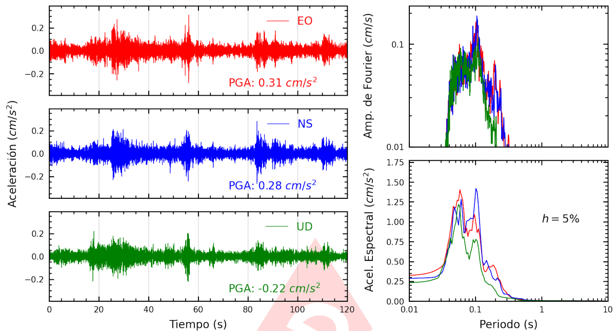
Figura A.21: Registros tiempo-historia, espectros de Fourier y de respuesta en las direcciones EO, NS y vertical de la estación SCCHO. Sismo de Mala, Cañete - Lima del 2024-11-24, 21:51:22 (Hora local)
