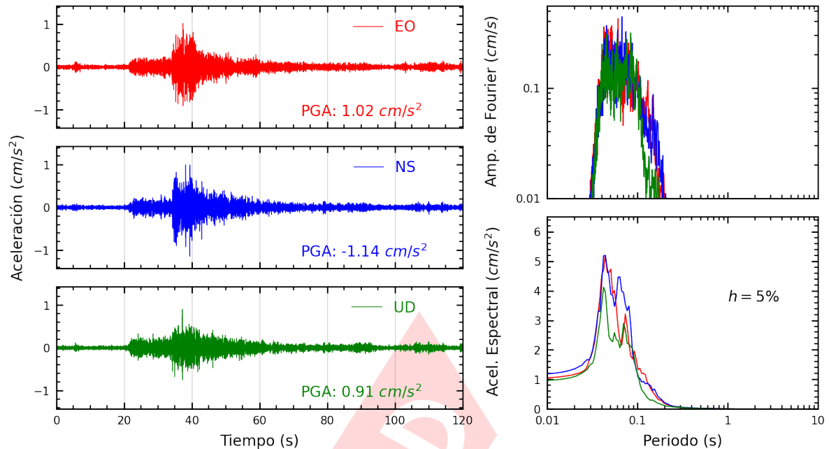
Figura A.3: Registros tiempo-historia, espectros de Fourier y de respuesta en las direcciones EO, NS y vertical de la estación SROS2. Sismo de Mala, Cañete - Lima del 2024-11-24, 21:51:22 (Hora local)
