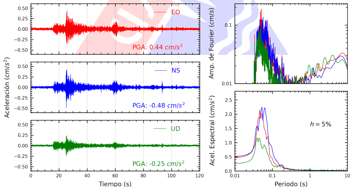
Figura A.10: Registros tiempo-historia, espectros de Fourier y de respuesta en las direcciones EO, NS y vertical de la estación UPCVI. Sismo de Mala, Cañete - Lima del 2024-11-24, 21:51:22 (Hora local)
