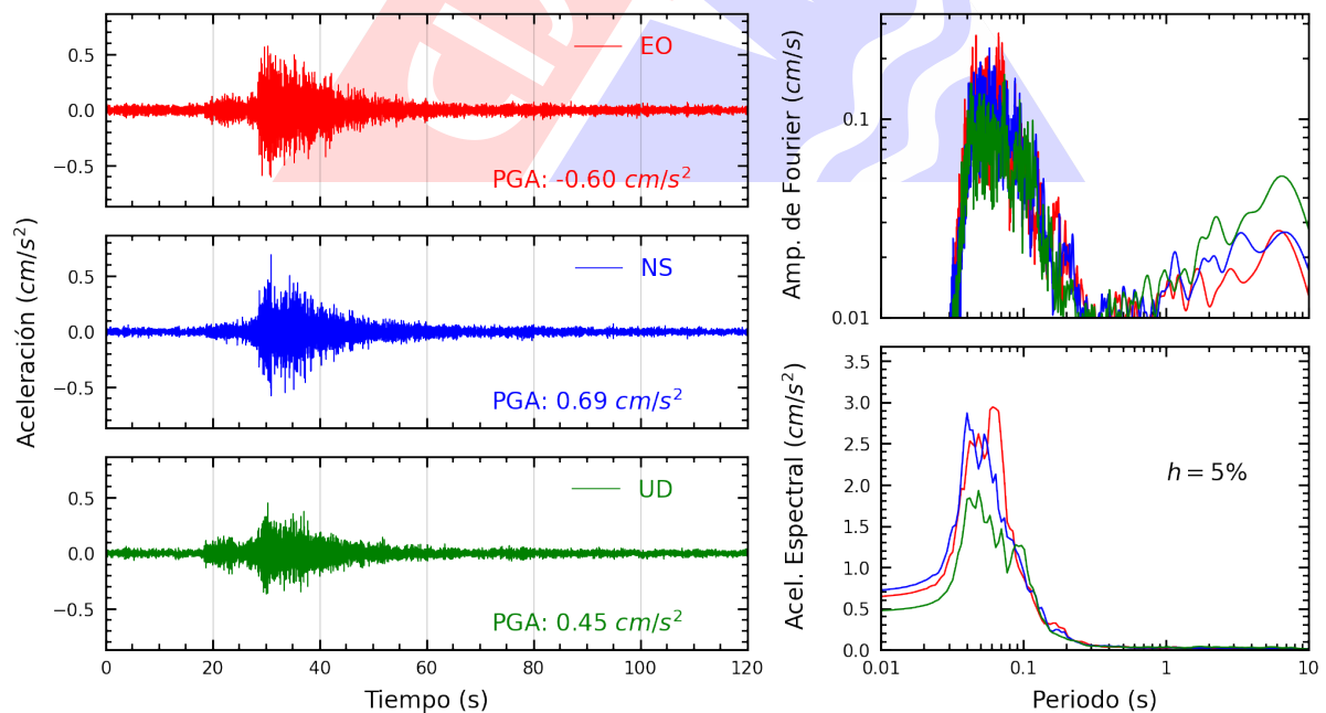
Figura A.8: Registros tiempo-historia, espectros de Fourier y de respuesta en las direcciones EO, NS y vertical de la estación INDEP. Sismo de Mala, Cañete - Lima del 2024-11-24, 21:51:22 (Hora local)
