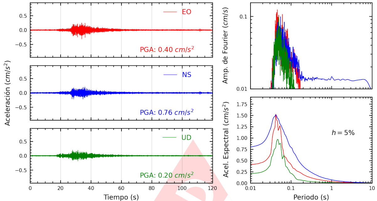
Figura A.5: Registros tiempo-historia, espectros de Fourier y de respuesta en las direcciones EO, NS y vertical de la estación ATARJ. Sismo de Mala, Cañete - Lima del 2024-11-24, 21:51:22 (Hora local)
