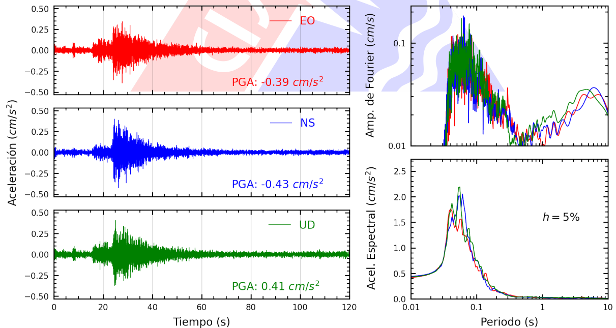
Figura A.12: Registros tiempo-historia, espectros de Fourier y de respuesta en las direcciones EO, NS y vertical de la estación SOVES. Sismo de Mala, Cañete - Lima del 2024-11-24, 21:51:22 (Hora local)
