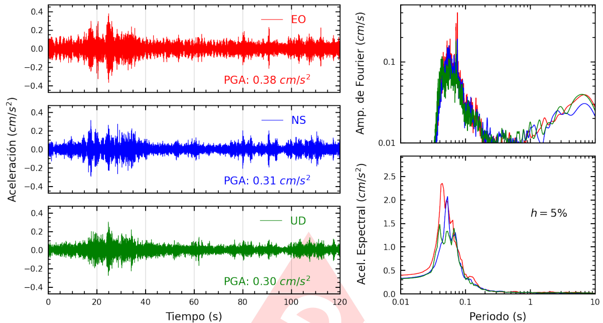
Figura A.13: Registros tiempo-historia, espectros de Fourier y de respuesta en las direcciones EO, NS y vertical de la estación UPCSM. Sismo de Mala, Cañete - Lima del 2024-11-24, 21:51:22 (Hora local)
