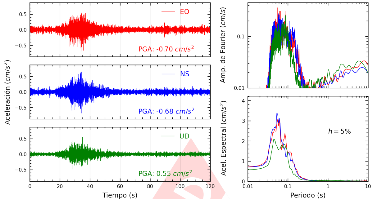
Figura A.7: Registros tiempo-historia, espectros de Fourier y de respuesta en las direcciones EO, NS y vertical de la estación USILM. Sismo de Mala, Cañete - Lima del 2024-11-24, 21:51:22 (Hora local)
