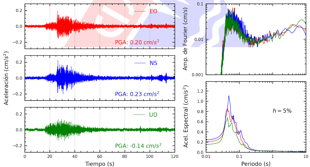
Figura A.26: Registros tiempo-historia, espectros de Fourier y de respuesta en las direcciones EO, NS y vertical de la estación SERVI. Sismo de Mala, Cañete - Lima del 2024-11-24, 21:51:22 (Hora local)
