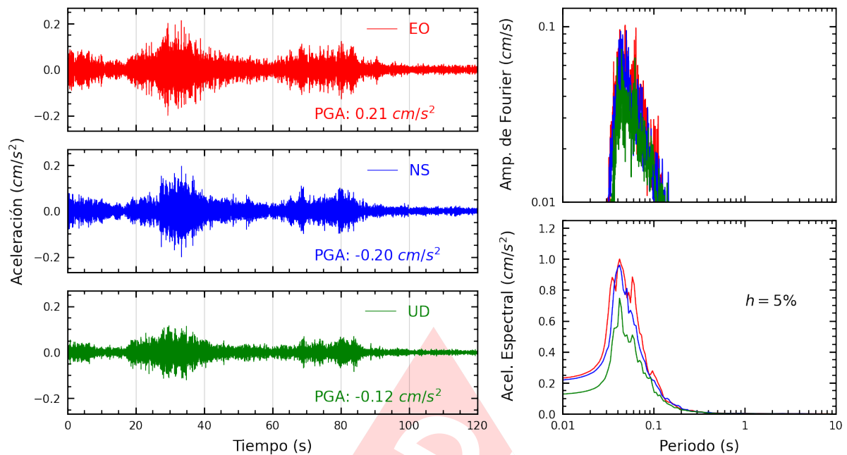
Figura A.27: Registros tiempo-historia, espectros de Fourier y de respuesta en las direcciones EO, NS y vertical de la estación BORJA. Sismo de Mala, Cañete - Lima del 2024-11-24, 21:51:22 (Hora local)
