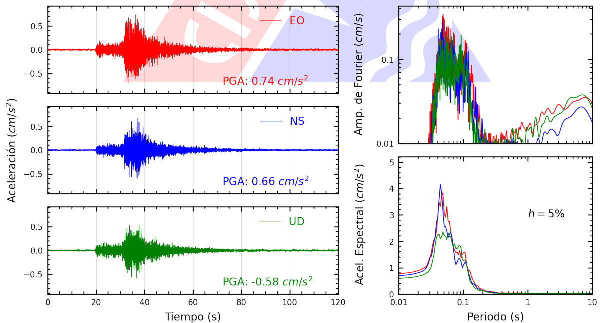
Figura A.6: Registros tiempo-historia, espectros de Fourier y de respuesta en las direcciones EO, NS y vertical de la estación AMORE. Sismo de Mala, Cañete - Lima del 2024-11-24, 21:51:22 (Hora local)
