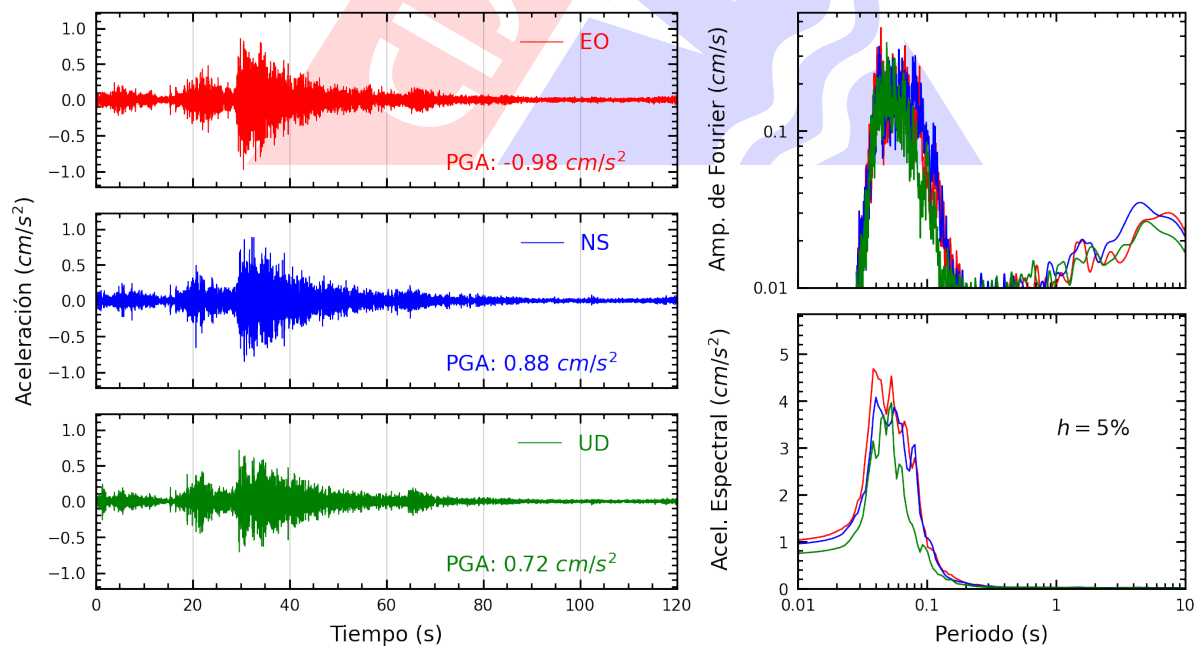
Figura A.4: Registros tiempo-historia, espectros de Fourier y de respuesta en las direcciones EO, NS y vertical de la estación JOSEO. Sismo de Mala, Cañete - Lima del 2024-11-24, 21:51:22 (Hora local)
