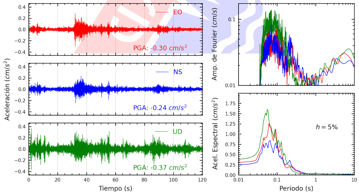
Figura A.16: Registros tiempo-historia, espectros de Fourier y de respuesta en las direcciones EO, NS y vertical de la estación MDPP. Sismo de Mala, Cañete - Lima del 2024-11-24, 21:51:22 (Hora local)
