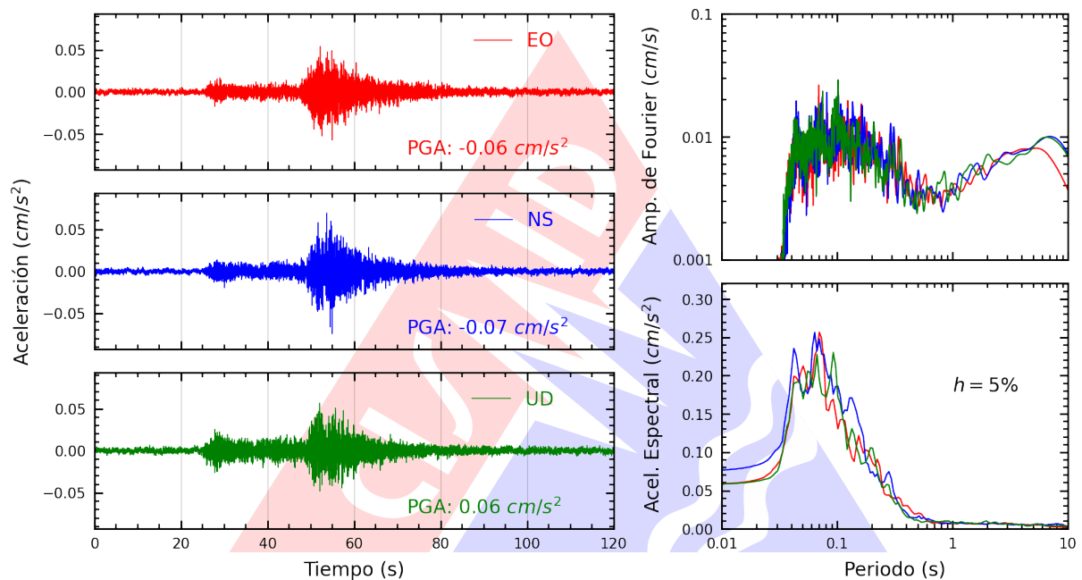
Figura A.31: Registros tiempo-historia, espectros de Fourier y de respuesta en las direcciones EO, NS y vertical de la estación CARAL. Sismo de Mala, Cañete - Lima del 2024-11-24, 21:51:22 (Hora local)
