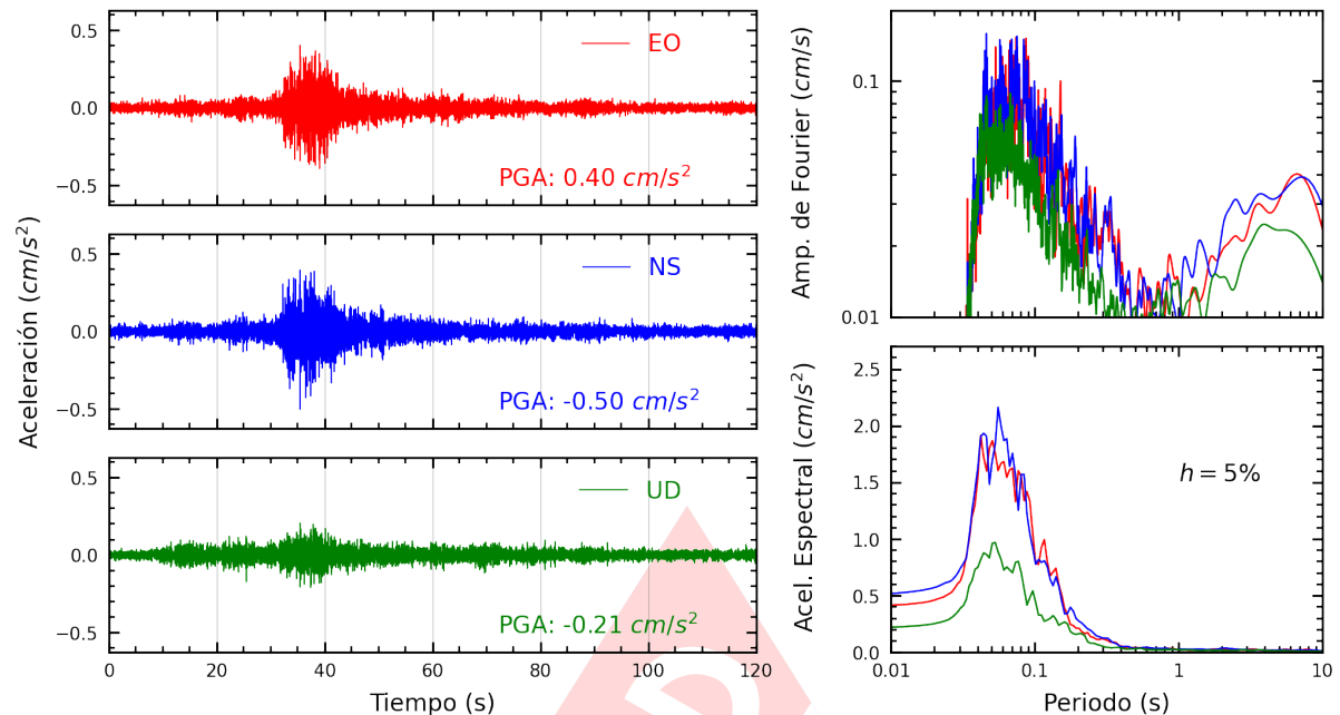
Figura A.9: Registros tiempo-historia, espectros de Fourier y de respuesta en las direcciones EO, NS y vertical de la estación DEFEN. Sismo de Mala, Cañete - Lima del 2024-11-24, 21:51:22 (Hora local)
