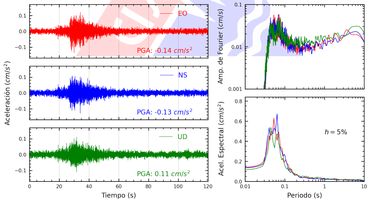
Figura A.28: Registros tiempo-historia, espectros de Fourier y de respuesta en las direcciones EO, NS y vertical de la estación UNFV. Sismo de Mala, Cañete - Lima del 2024-11-24, 21:51:22 (Hora local)
