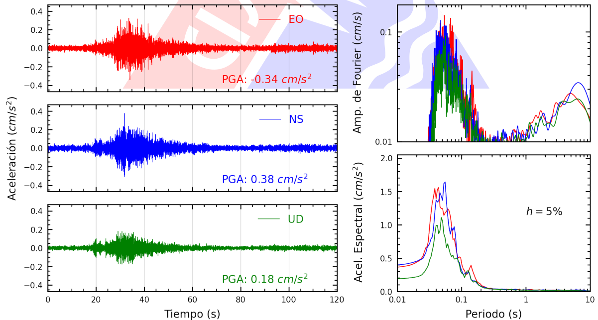
Figura A.14: Registros tiempo-historia, espectros de Fourier y de respuesta en las direcciones EO, NS y vertical de la estación FICPE. Sismo de Mala, Cañete - Lima del 2024-11-24, 21:51:22 (Hora local)
