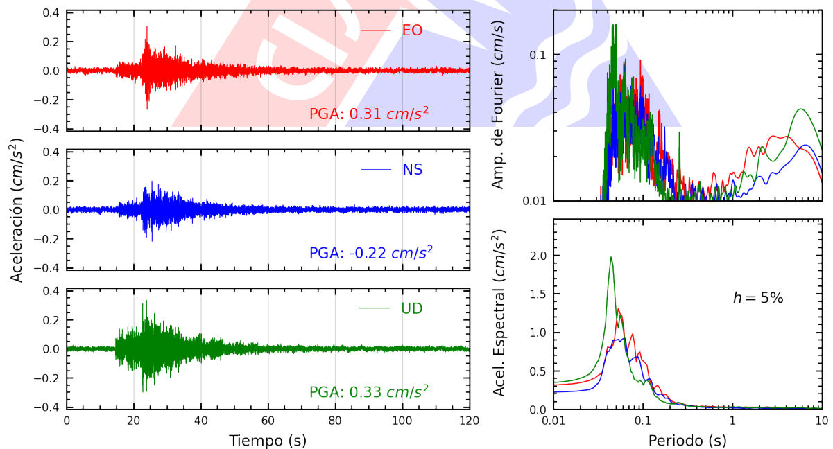
Figura A.20: Registros tiempo-historia, espectros de Fourier y de respuesta en las direcciones EO, NS y vertical de la estación USILP. Sismo de Mala, Cañete - Lima del 2024-11-24, 21:51:22 (Hora local)
