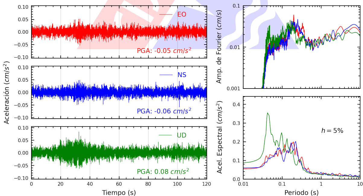
Figura A.30: Registros tiempo-historia, espectros de Fourier y de respuesta en las direcciones EO, NS y vertical de la estación DSMI. Sismo de Mala, Cañete - Lima del 2024-11-24, 21:51:22 (Hora local)
