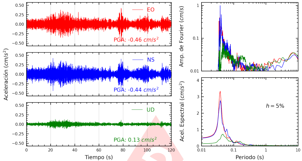
Figura A.11: Registros tiempo-historia, espectros de Fourier y de respuesta en las direcciones EO, NS y vertical de la estación DHNPE. Sismo de Mala, Cañete - Lima del 2024-11-24, 21:51:22 (Hora local)
