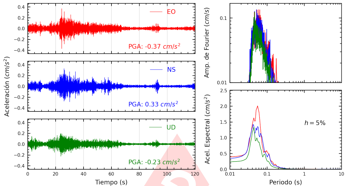
Figura A.15: Registros tiempo-historia, espectros de Fourier y de respuesta en las direcciones EO, NS y vertical de la estación PACHA. Sismo de Mala, Cañete - Lima del 2024-11-24, 21:51:22 (Hora local)
