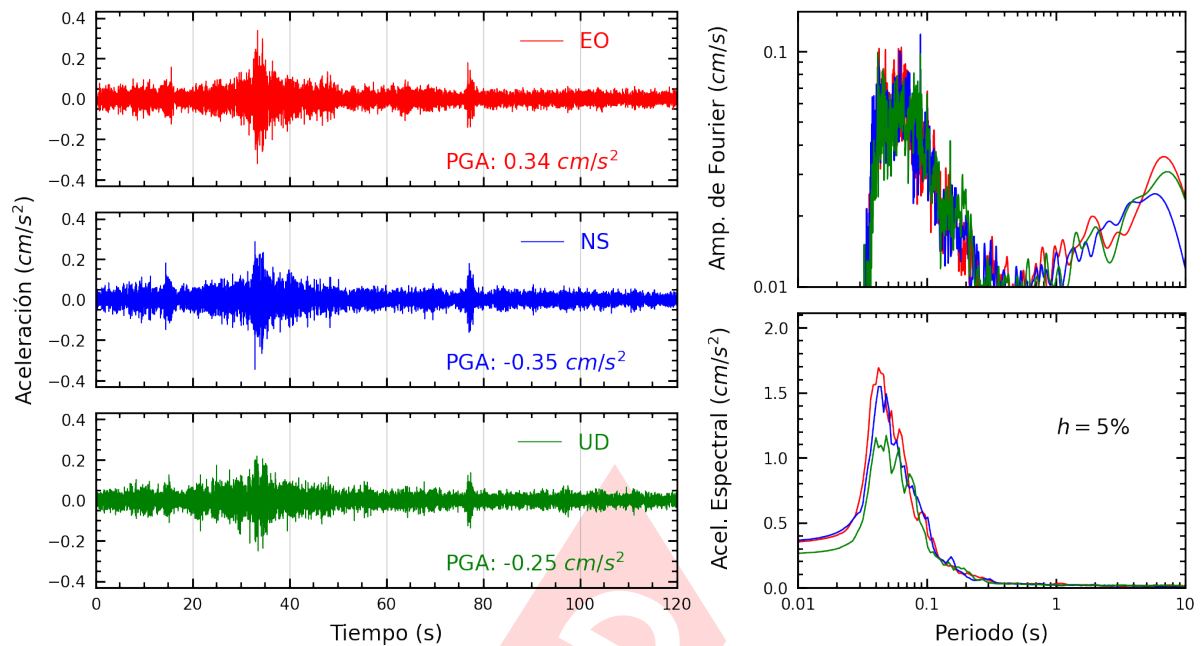
Figura A.19: Registros tiempo-historia, espectros de Fourier y de respuesta en las direcciones EO, NS y vertical de la estación MADRE. Sismo de Mala, Cañete - Lima del 2024-11-24, 21:51:22 (Hora local)
