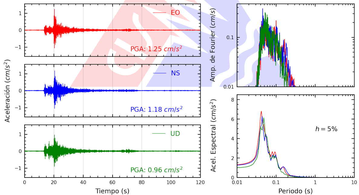
Figura A.2: Registros tiempo-historia, espectros de Fourier y de respuesta en las direcciones EO, NS y vertical de la estación ASIA. Sismo de Mala, Cañete - Lima del 2024-11-24, 21:51:22 (Hora local)
