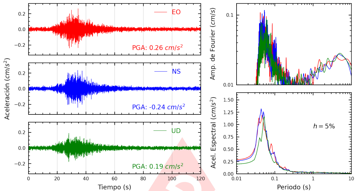
Figura A.25: Registros tiempo-historia, espectros de Fourier y de respuesta en las direcciones EO, NS y vertical de la estación IMCA. Sismo de Mala, Cañete - Lima del 2024-11-24, 21:51:22 (Hora local)
