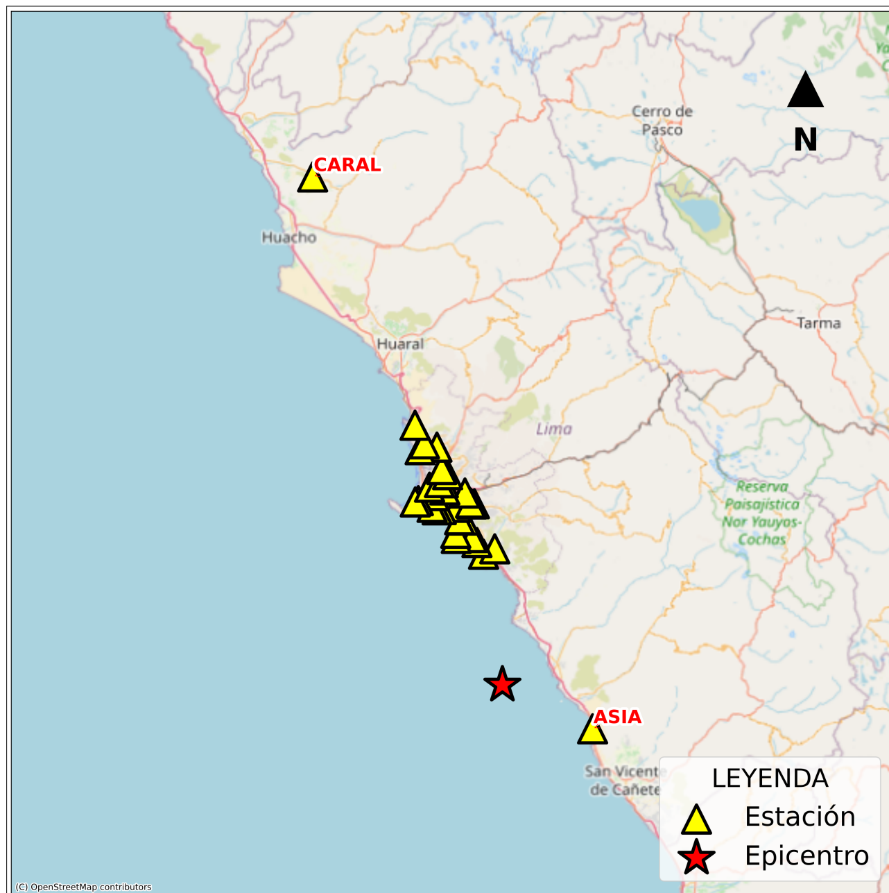
Figura 2: Mapa de ubicación de la(s) estación(es) acelerográfica(s) a nivel nacional correspondiente(s) al Sismo de Mala, Cañete - Lima del 24 de noviembre de 2024 a las 21:51:22 (hora local)
