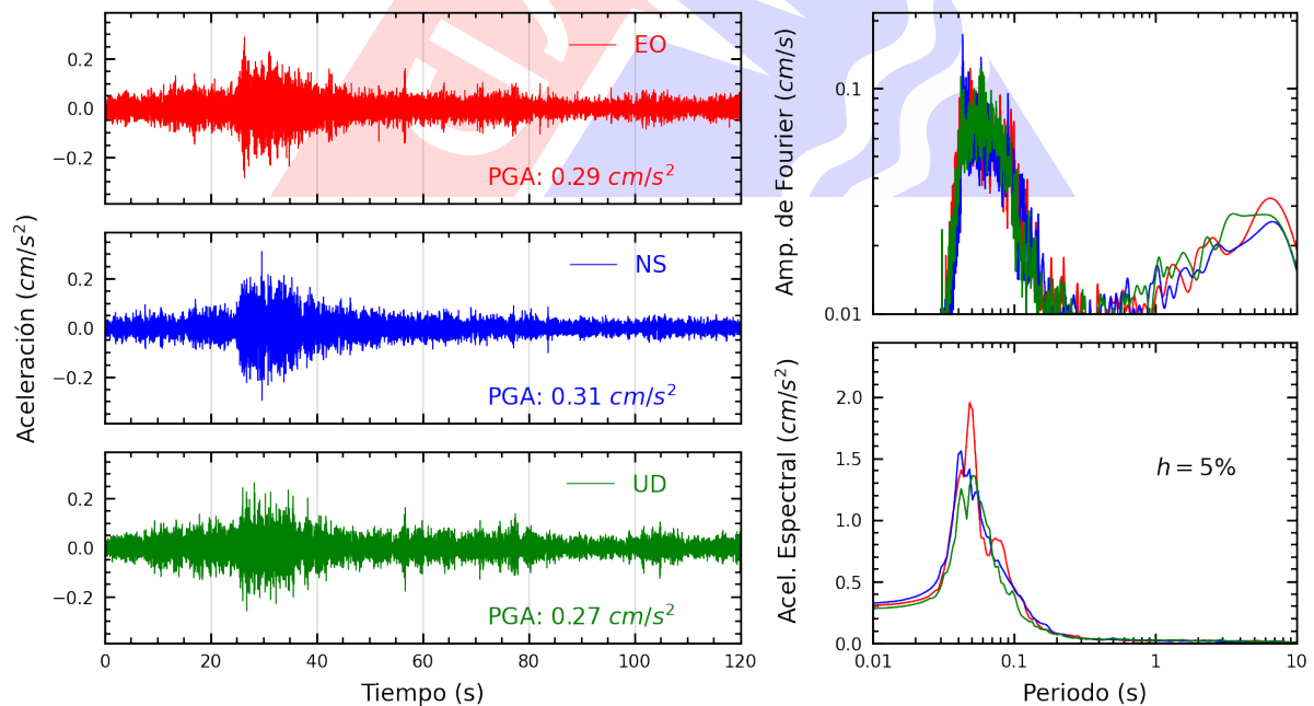
Figura A.22: Registros tiempo-historia, espectros de Fourier y de respuesta en las direcciones EO, NS y vertical de la estación URPE. Sismo de Mala, Cañete - Lima del 2024-11-24, 21:51:22 (Hora local)
