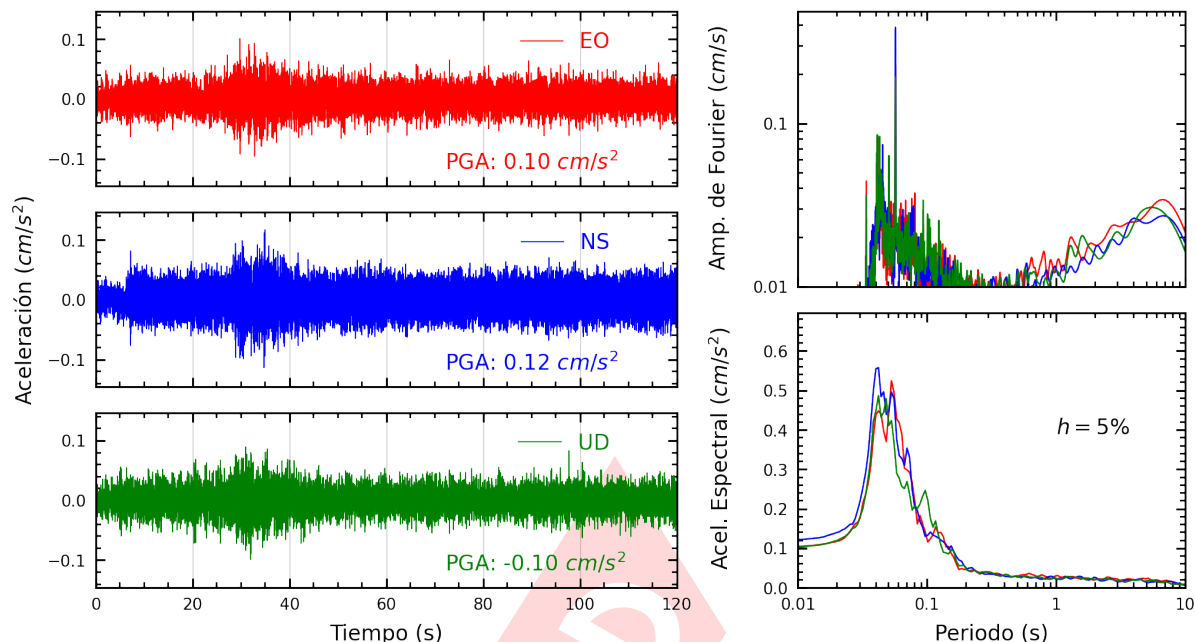
Figura A.29: Registros tiempo-historia, espectros de Fourier y de respuesta en las direcciones EO, NS y vertical de la estación BONDY. Sismo de Mala, Cañete - Lima del 2024-11-24, 21:51:22 (Hora local)
