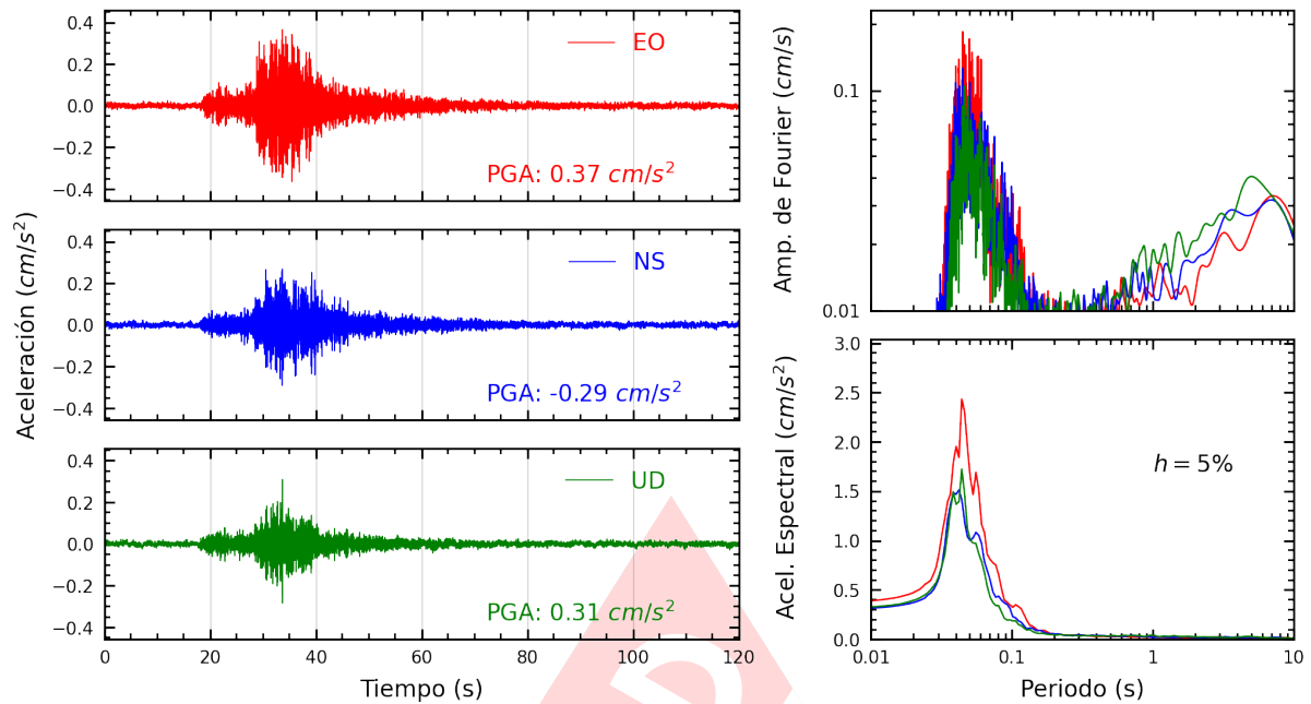
Figura A.17: Registros tiempo-historia, espectros de Fourier y de respuesta en las direcciones EO, NS y vertical de la estación UCSS. Sismo de Mala, Cañete - Lima del 2024-11-24, 21:51:22 (Hora local)
