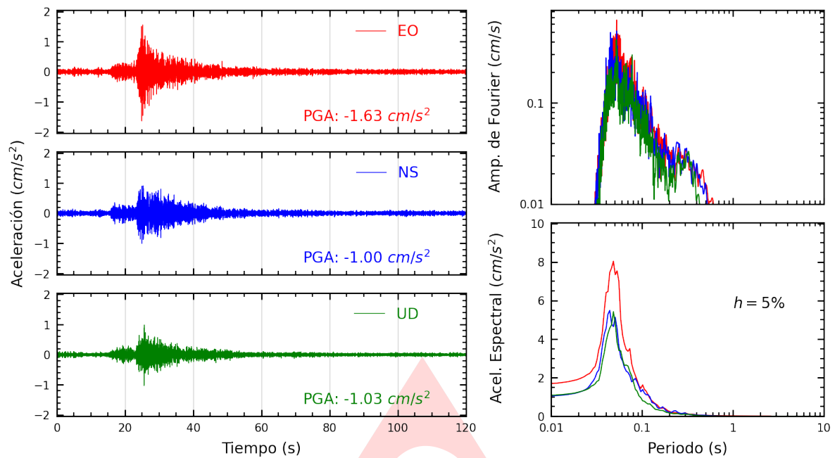
Figura A.1: Registros tiempo-historia, espectros de Fourier y de respuesta en las direcciones EO, NS y vertical de la estación UNTEL. Sismo de Mala, Cañete - Lima del 2024-11-24, 21:51:22 (Hora local)
