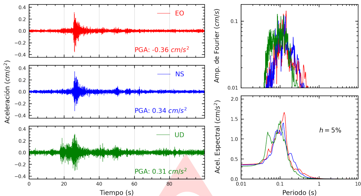
Figura A.1: Registros tiempo-historia, espectros de Fourier y de respuesta en las direcciones EO, NS y vertical de la estación UNP. Sismo de Sechura, Sechura - Piura del 2024-11-25, 14:30:08 (Hora local)
