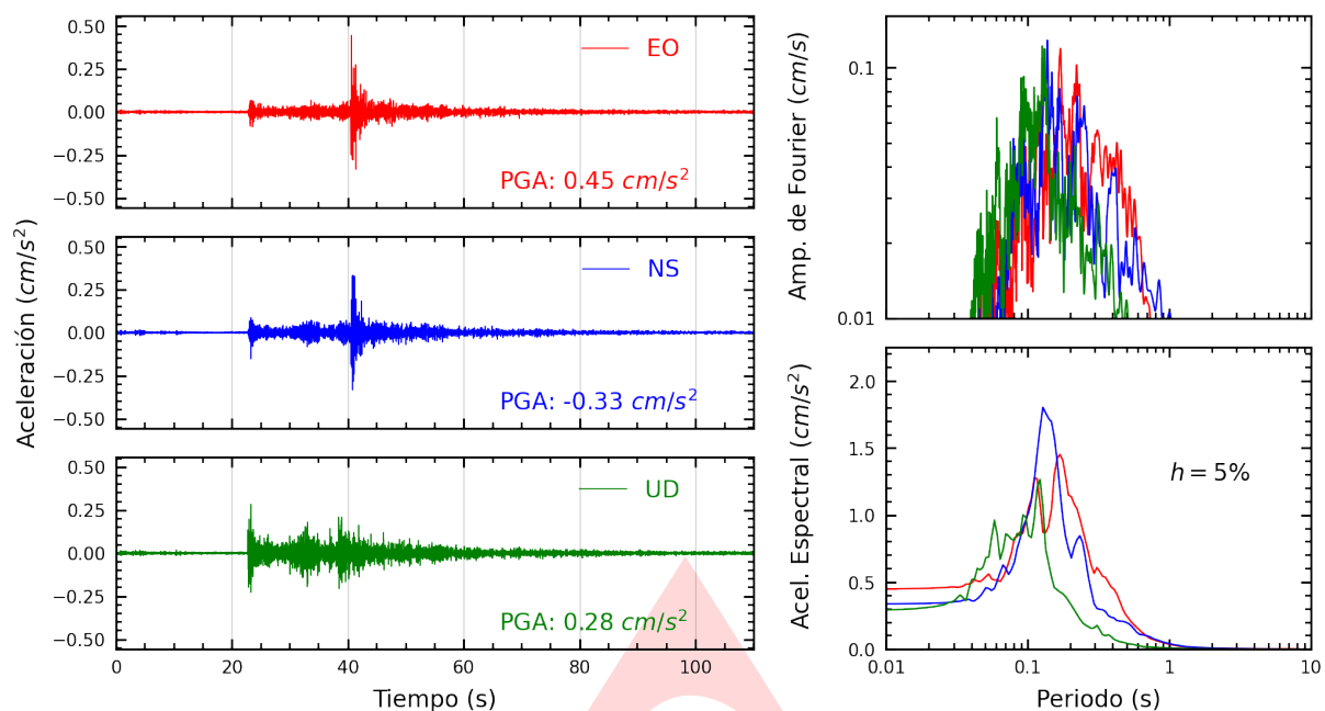
Figura A.1: Registros tiempo-historia, espectros de Fourier y de respuesta en las direcciones EO, NS y vertical de la estación UNIA. Sismo de Aguaytia, Padre Abad - Ucayali del 2024-11-25, 19:21:49 (Hora local)
