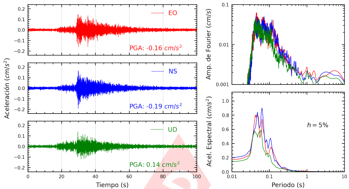
Figura A.9: Registros tiempo-historia, espectros de Fourier y de respuesta en las direcciones EO, NS y vertical de la estación ATARJ. Sismo de Mala, Cañete - Lima del 2024-08-19, 07:07:00 (Hora local)
