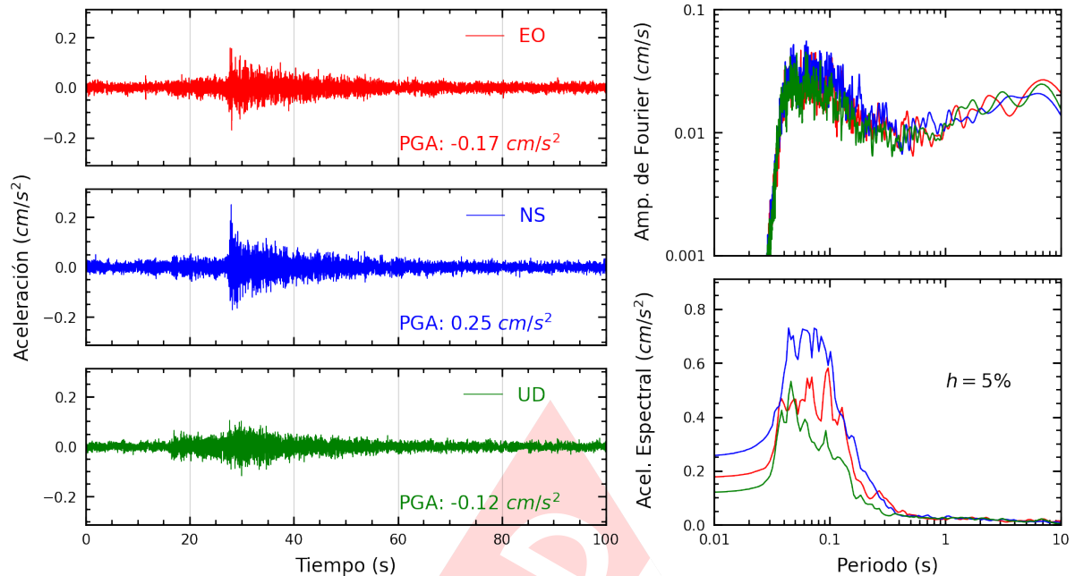
Figura A.7: Registros tiempo-historia, espectros de Fourier y de respuesta en las direcciones EO, NS y vertical de la estación SERVI. Sismo de Mala, Cañete - Lima del 2024-08-19, 07:07:00 (Hora local)
