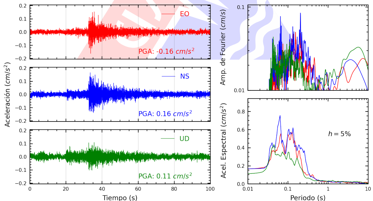
Figura A.10: Registros tiempo-historia, espectros de Fourier y de respuesta en las direcciones EO, NS y vertical de la estación VHAYA. Sismo de Mala, Cañete - Lima del 2024-08-19, 07:07:00 (Hora local)
