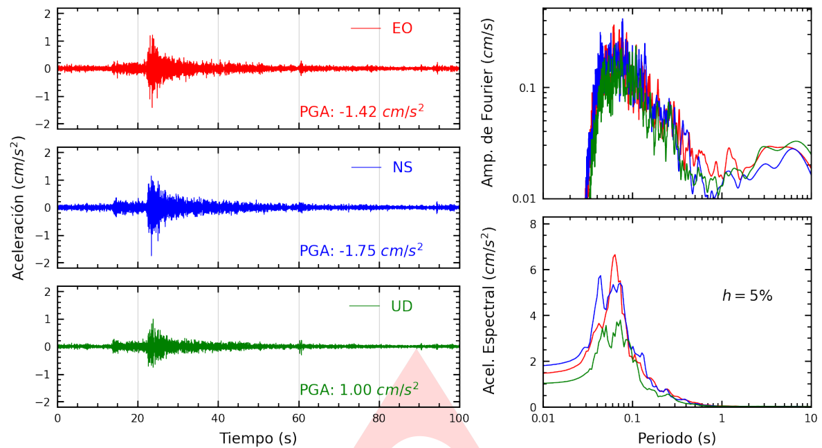
Figura A.1: Registros tiempo-historia, espectros de Fourier y de respuesta en las direcciones EO, NS y vertical de la estación PHERM. Sismo de Mala, Cañete - Lima del 2024-08-19, 07:07:00 (Hora local)
