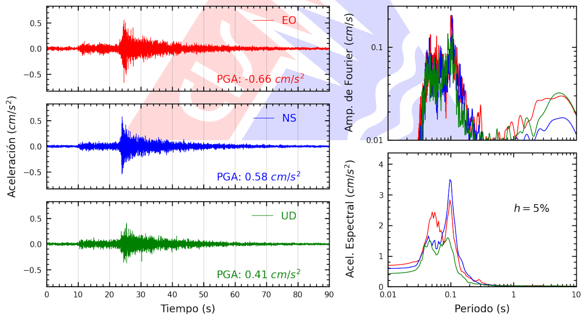
Figura A.2: Registros tiempo-historia, espectros de Fourier y de respuesta en las direcciones EO, NS y vertical de la estación AMORE. Sismo de Mala, Cañete - Lima del 2024-08-19, 07:07:00 (Hora local)
