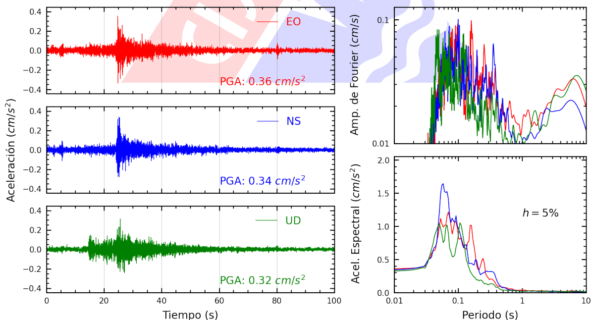
Figura A.4: Registros tiempo-historia, espectros de Fourier y de respuesta en las direcciones EO, NS y vertical de la estación USILP. Sismo de Mala, Cañete - Lima del 2024-08-19, 07:07:00 (Hora local)
