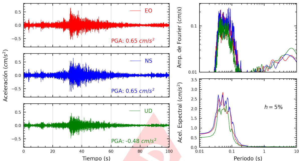
Figura A.3: Registros tiempo-historia, espectros de Fourier y de respuesta en las direcciones EO, NS y vertical de la estación JOSEO. Sismo de Mala, Cañete - Lima del 2024-08-19, 07:07:00 (Hora local)
