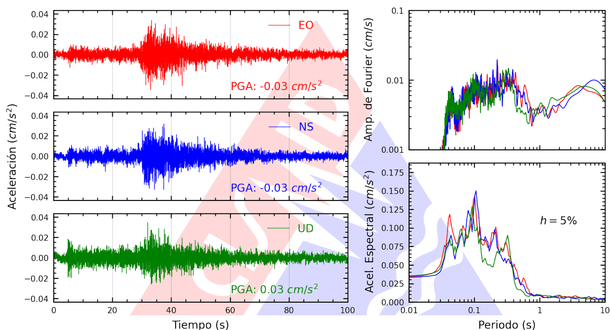
Figura A.11: Registros tiempo-historia, espectros de Fourier y de respuesta en las direcciones EO, NS y vertical de la estación CARAL. Sismo de Mala, Cañete - Lima del 2024-08-19, 07:07:00 (Hora local)
