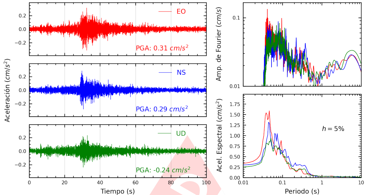
Figura A.5: Registros tiempo-historia, espectros de Fourier y de respuesta en las direcciones EO, NS y vertical de la estación UCVAT. Sismo de Mala, Cañete - Lima del 2024-08-19, 07:07:00 (Hora local)
