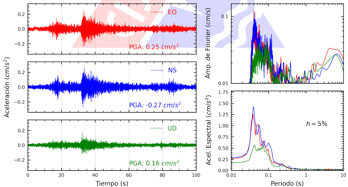
Figura A.6: Registros tiempo-historia, espectros de Fourier y de respuesta en las direcciones EO, NS y vertical de la estación COMAS. Sismo de Mala, Cañete - Lima del 2024-08-19, 07:07:00 (Hora local)
