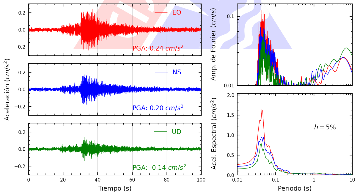
Figura A.8: Registros tiempo-historia, espectros de Fourier y de respuesta en las direcciones EO, NS y vertical de la estación UCSS. Sismo de Mala, Cañete - Lima del 2024-08-19, 07:07:00 (Hora local)
