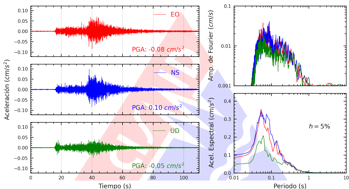
Figura A.3: Registros tiempo-historia, espectros de Fourier y de respuesta en las direcciones EO, NS y vertical de la estación UNSA2. Sismo de Chivay, Caylloma - Arequipa del 2024-12-05, 03:35:32 (Hora local)
