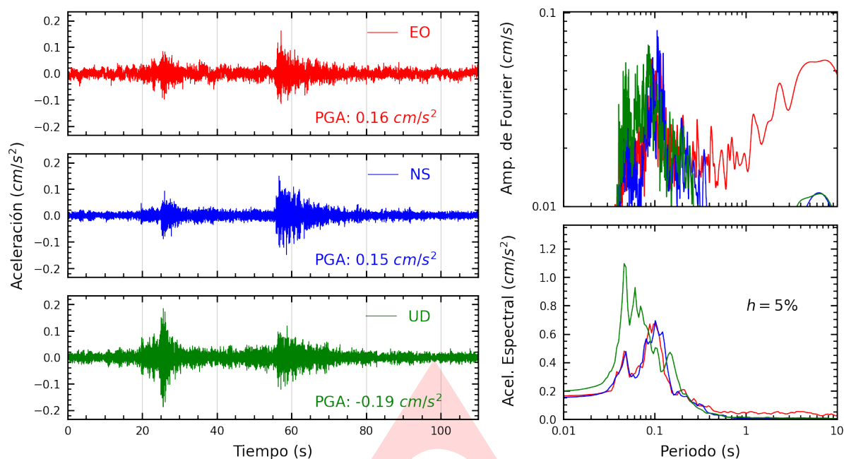
Figura A.1: Registros tiempo-historia, espectros de Fourier y de respuesta en las direcciones EO, NS y vertical de la estación UJBG3. Sismo de Chivay, Caylloma - Arequipa del 2024-12-05, 03:35:32 (Hora local)
