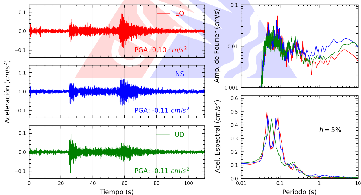
Figura A.2: Registros tiempo-historia, espectros de Fourier y de respuesta en las direcciones EO, NS y vertical de la estación CREY. Sismo de Chivay, Caylloma - Arequipa del 2024-12-05, 03:35:32 (Hora local)
