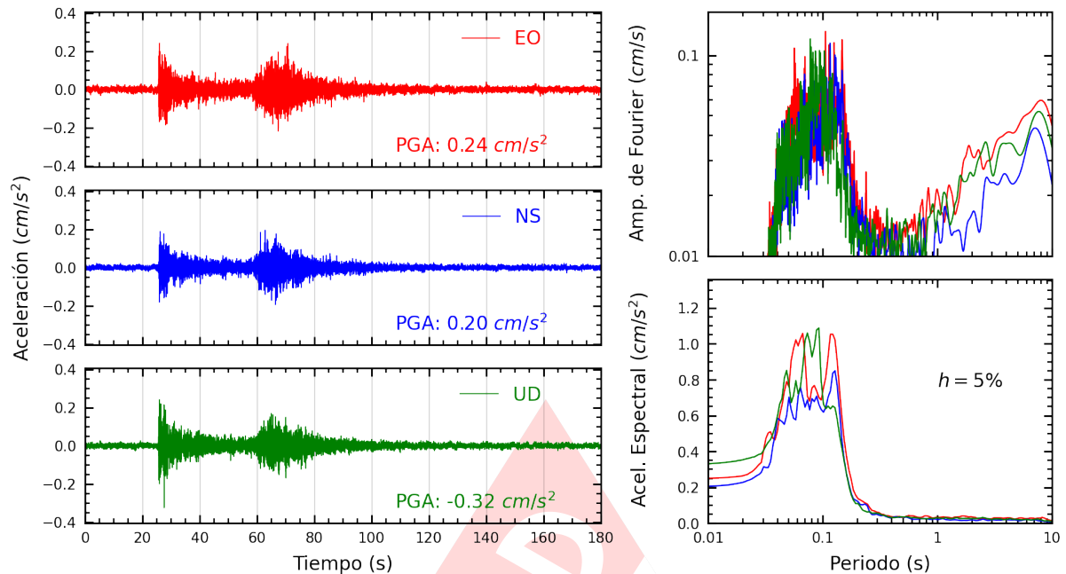
Figura A.3: Registros tiempo-historia, espectros de Fourier y de respuesta en las direcciones EO, NS y vertical de la estación AMORE. Sismo de Chimbote, Santa - Ancash del 2024-12-07, 12:53:45 (Hora local)
