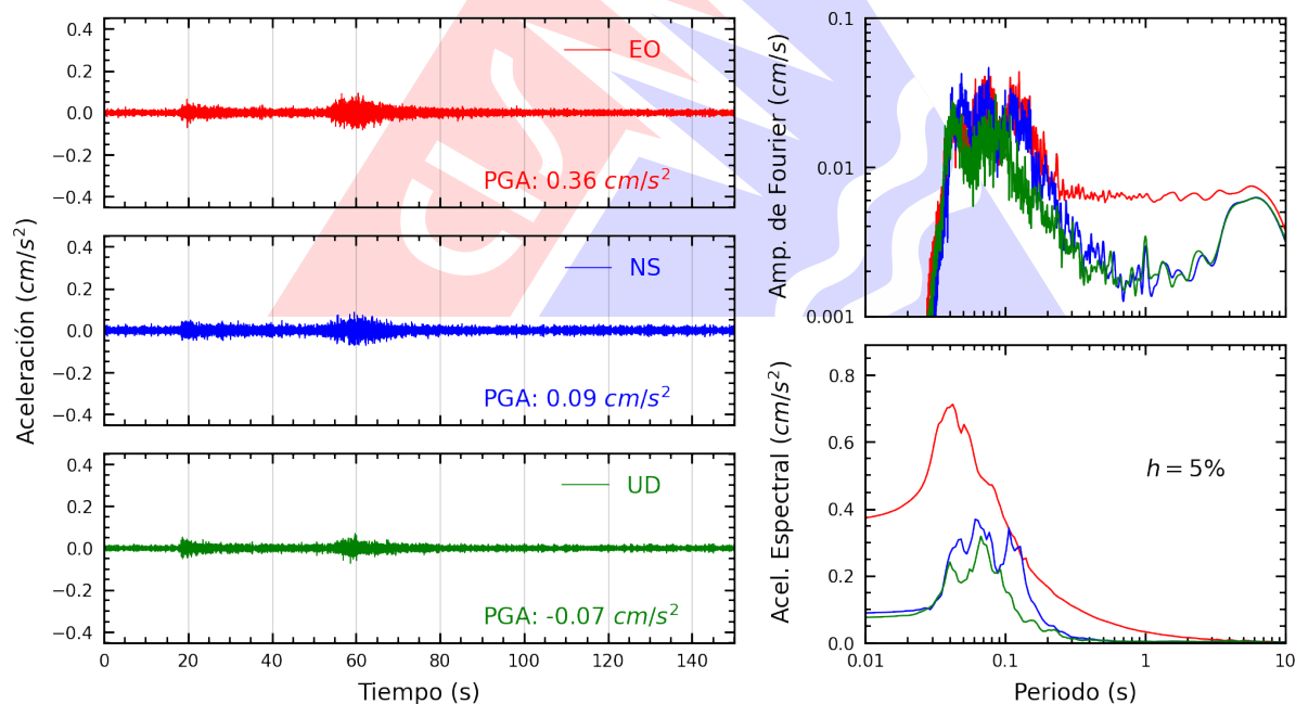
Figura A.2: Registros tiempo-historia, espectros de Fourier y de respuesta en las direcciones EO, NS y vertical de la estación ATARJ. Sismo de Chimbote, Santa - Ancash del 2024-12-07, 12:53:45 (Hora local)
