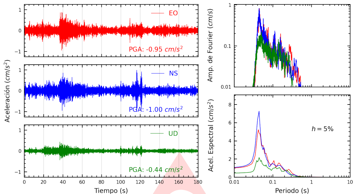
Figura A.1: Registros tiempo-historia, espectros de Fourier y de respuesta en las direcciones EO, NS y vertical de la estación SCTRU. Sismo de Chimbote, Santa - Ancash del 2024-12-07, 12:53:45 (Hora local)
