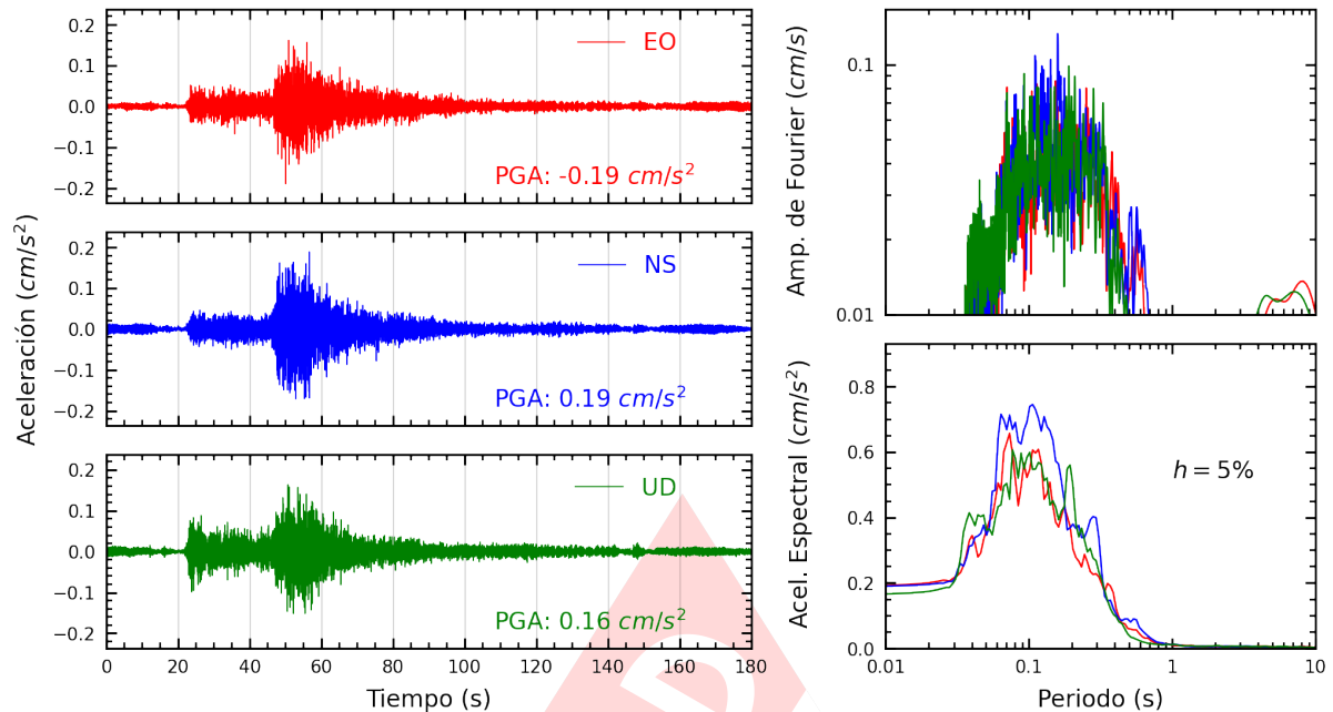
Figura A.5: Registros tiempo-historia, espectros de Fourier y de respuesta en las direcciones EO, NS y vertical de la estación CARAL. Sismo de Chimbote, Santa - Ancash del 2024-12-07, 12:53:45 (Hora local)
