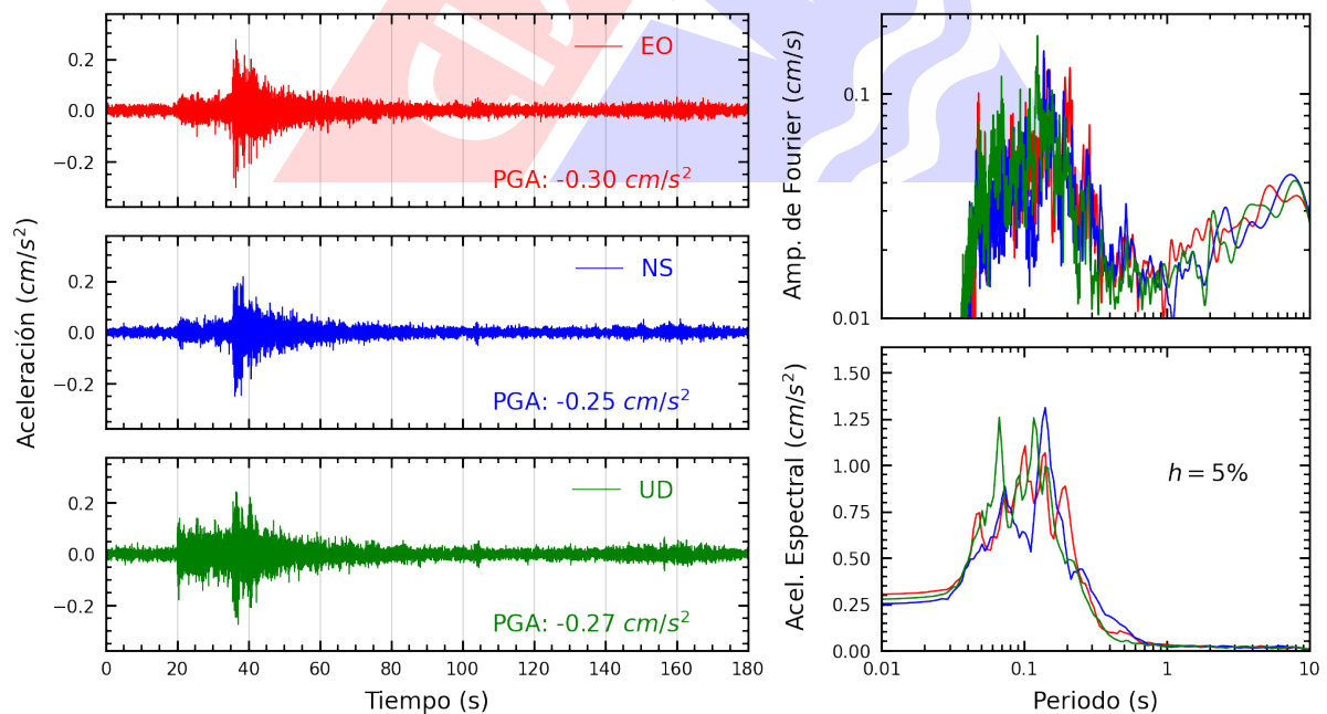
Figura A.4: Registros tiempo-historia, espectros de Fourier y de respuesta en las direcciones EO, NS y vertical de la estación UPAOT. Sismo de Chimbote, Santa - Ancash del 2024-12-07, 12:53:45 (Hora local)
