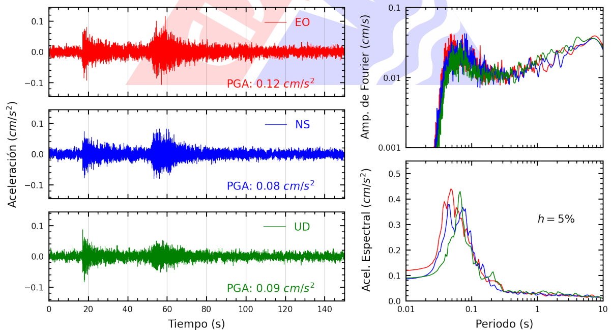
Figura A.6: Registros tiempo-historia, espectros de Fourier y de respuesta en las direcciones EO, NS y vertical de la estación UCSS. Sismo de Chimbote, Santa - Ancash del 2024-12-07, 12:53:45 (Hora local)
