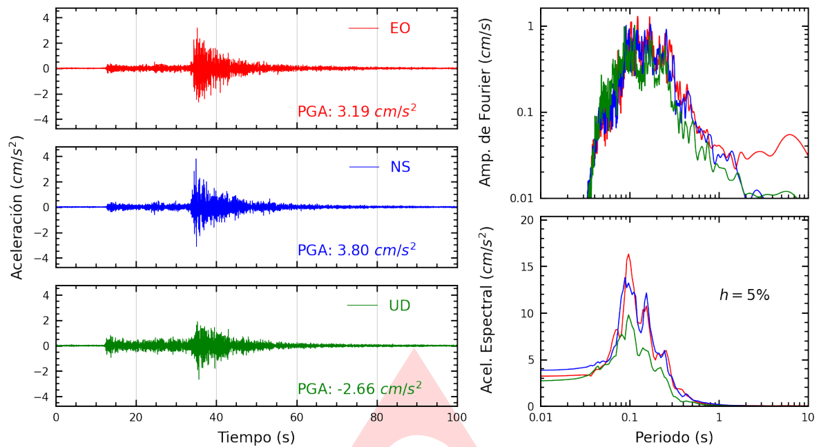
Figura A.1: Registros tiempo-historia, espectros de Fourier y de respuesta en las direcciones EO, NS y vertical de la estación UJBG3. Sismo de La Capilla, General Sanchez Cerro - Moquegua del 2024-12-10, 09:19:23 (Hora local)
