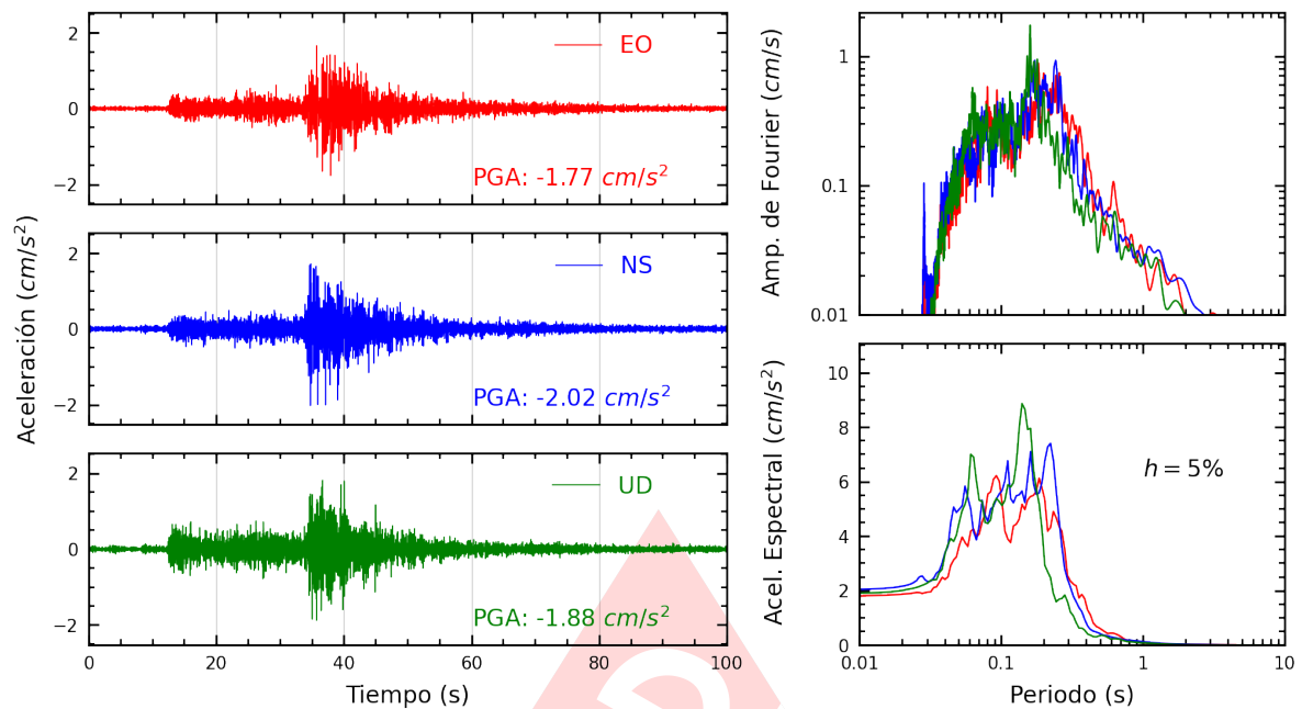
Figura A.3: Registros tiempo-historia, espectros de Fourier y de respuesta en las direcciones EO, NS y vertical de la estación UJB4. Sismo de La Capilla, General Sanchez Cerro - Moquegua del 2024-12-10, 09:19:23 (Hora local)
