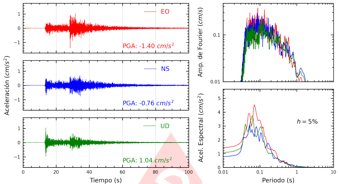
Figura A.5: Registros tiempo-historia, espectros de Fourier y de respuesta en las direcciones EO, NS y vertical de la estación UNSA2. Sismo de La Capilla, General Sanchez Cerro - Moquegua del 2024-12-10, 09:19:23 (Hora local)
