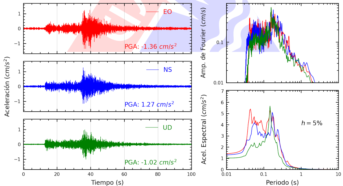
Figura A.6: Registros tiempo-historia, espectros de Fourier y de respuesta en las direcciones EO, NS y vertical de la estación UPTAC. Sismo de La Capilla, General Sanchez Cerro - Moquegua del 2024-12-10, 09:19:23 (Hora local)
