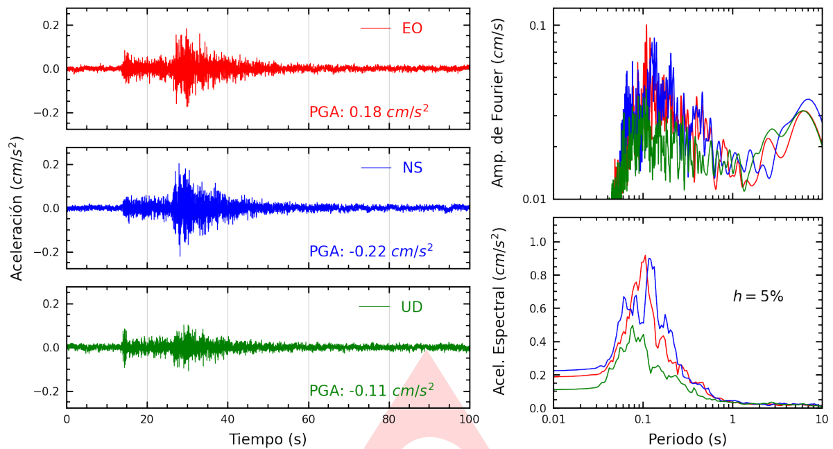
Figura A.1: Registros tiempo-historia, espectros de Fourier y de respuesta en las direcciones EO, NS y vertical de la estación UNTRM. Sismo de Jaen, Jaen - Cajamarca del 2024-12-11, 02:35:55 (Hora local)
