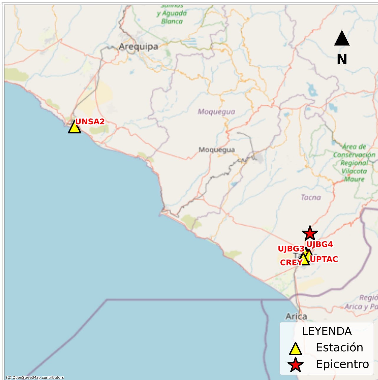
Figura 2: Mapa de ubicación de la(s) estación(es) acelerográfica(s) correspondiente(s) al Sismo de Calana, Tacna - Tacna del 12 de diciembre de 2024 a las 08:21:26 (hora local)
