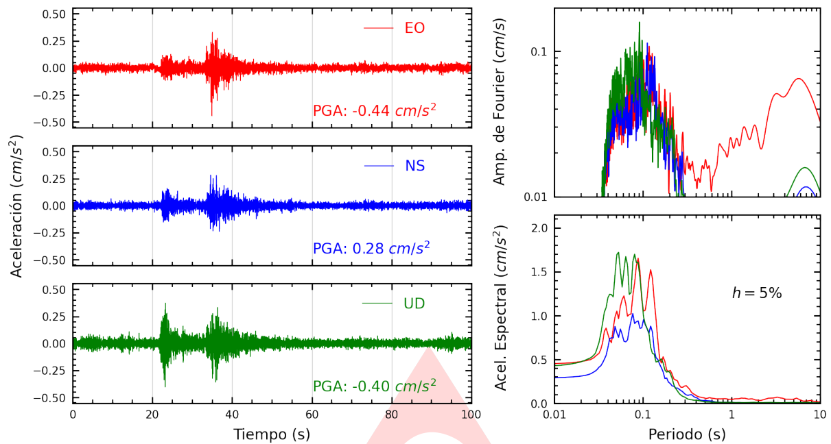
Figura A.1: Registros tiempo-historia, espectros de Fourier y de respuesta en las direcciones EO, NS y vertical de la estación UJBG3. Sismo de Calana, Tacna - Tacna del 2024-12-12, 08:21:26 (Hora local)
