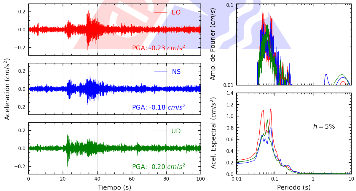
Figura A.4: Registros tiempo-historia, espectros de Fourier y de respuesta en las direcciones EO, NS y vertical de la estación CREY. Sismo de Calana, Tacna - Tacna del 2024-12-12, 08:21:26 (Hora local)
