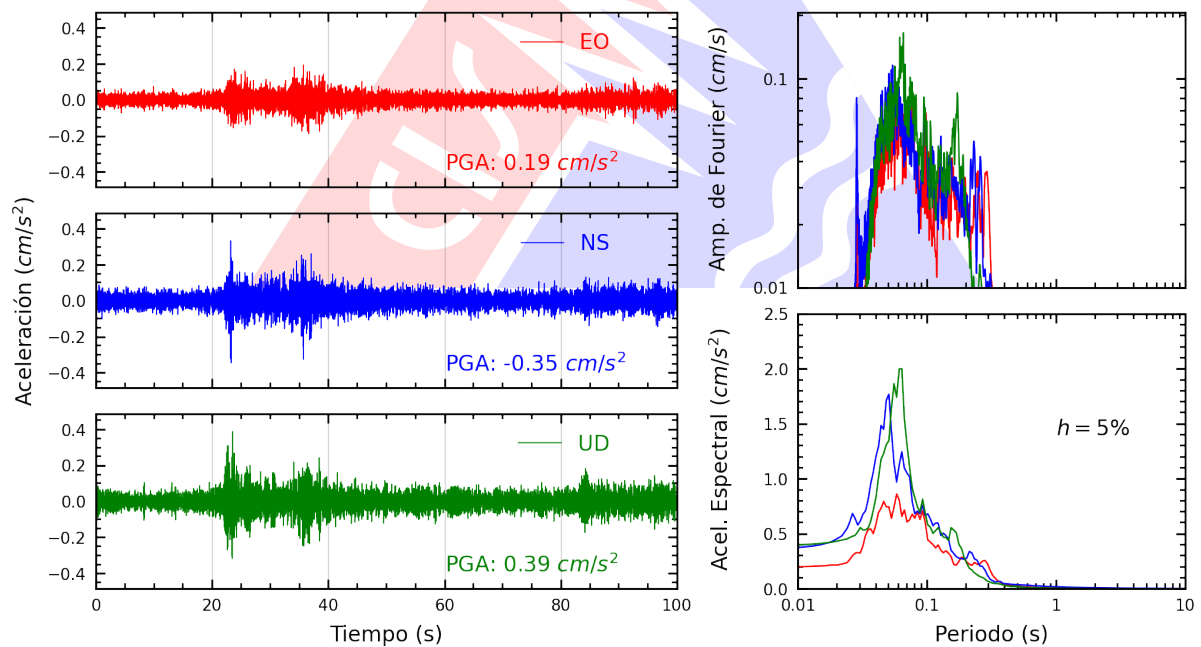
Figura A.2: Registros tiempo-historia, espectros de Fourier y de respuesta en las direcciones EO, NS y vertical de la estación UJBG4. Sismo de Calana, Tacna - Tacna del 2024-12-12, 08:21:26 (Hora local)
