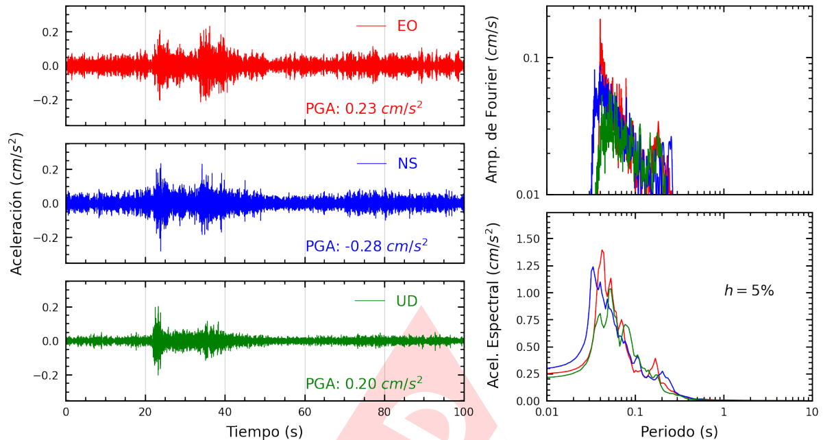
Figura A.3: Registros tiempo-historia, espectros de Fourier y de respuesta en las direcciones EO, NS y vertical de la estación UPTAC. Sismo de Calana, Tacna - Tacna del 2024-12-12, 08:21:26 (Hora local)
