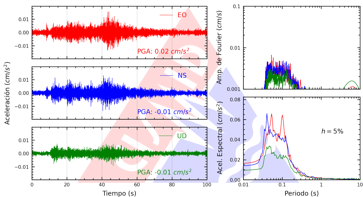
Figura A.5: Registros tiempo-historia, espectros de Fourier y de respuesta en las direcciones EO, NS y vertical de la estación UNSA2. Sismo de Calana, Tacna - Tacna del 2024-12-12, 08:21:26 (Hora local)
