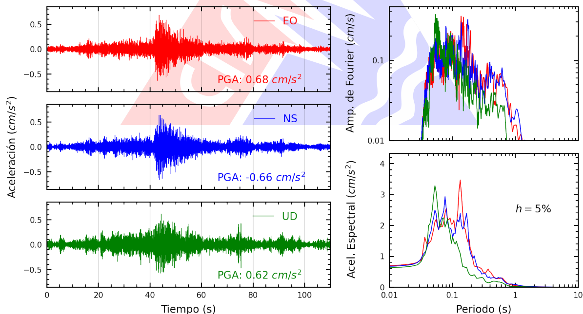
Figura A.2: Registros tiempo-historia, espectros de Fourier y de respuesta en las direcciones EO, NS y vertical de la estación SCAR2. Sismo de Camana, Camana - Arequipa del 2024-12-17, 04:02:19 (Hora local)
