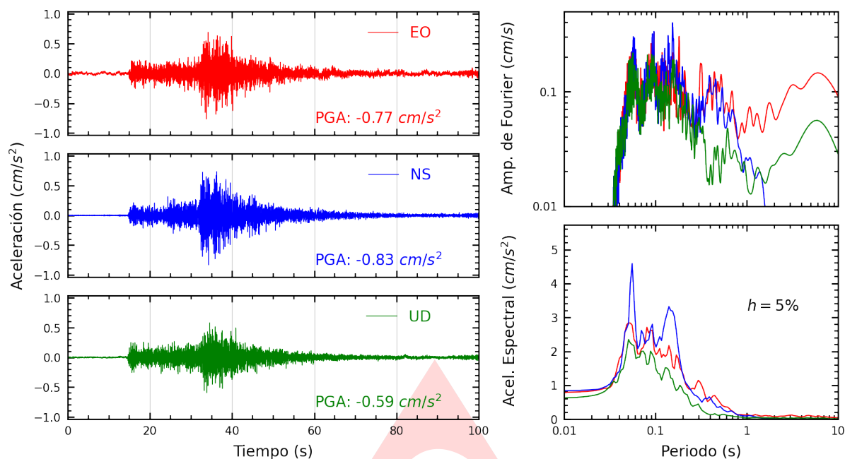
Figura A.1: Registros tiempo-historia, espectros de Fourier y de respuesta en las direcciones EO, NS y vertical de la estación SCARQ. Sismo de Camana, Camana - Arequipa del 2024-12-17, 04:02:19 (Hora local)
