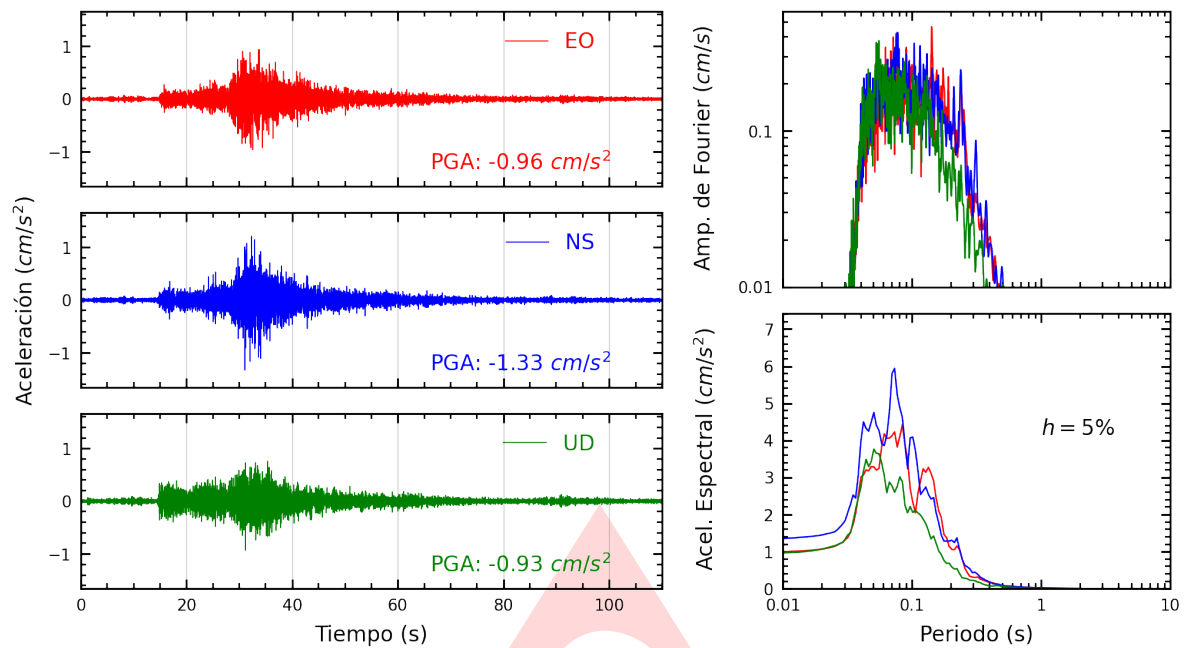
Figura A.1: Registros tiempo-historia, espectros de Fourier y de respuesta en las direcciones EO, NS y vertical de la estación ASIA. Sismo de Chinchá Alta, Chinchá - Ica del 2024-12-17, 17:02:05 (Hora local)
