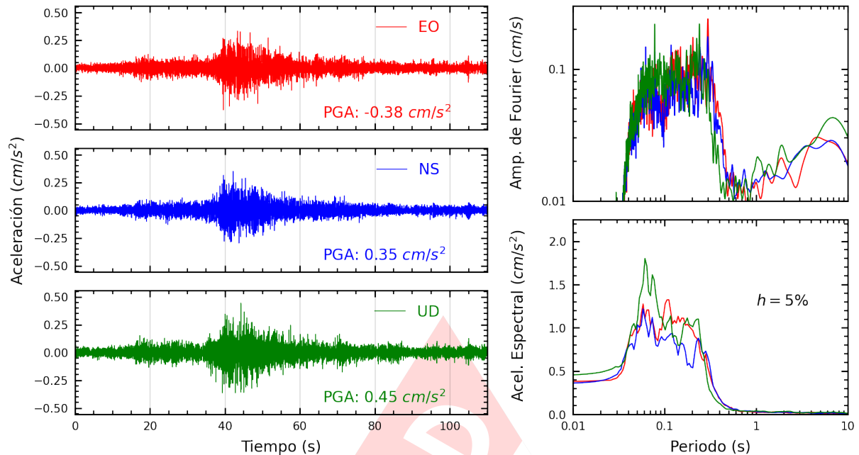
Figura A.5: Registros tiempo-historia, espectros de Fourier y de respuesta en las direcciones EO, NS y vertical de la estación SOVES. Sismo de Chincha Alta, Chincha - Ica del 2024-12-17, 17:02:05 (Hora local)
