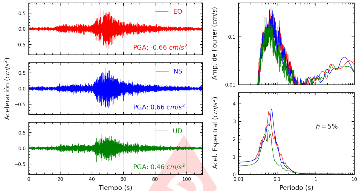
Figura A.3: Registros tiempo-historia, espectros de Fourier y de respuesta en las direcciones EO, NS y vertical de la estación JOSEO. Sismo de Chinchá Alta, Chinchá - Ica del 2024-12-17, 17:02:05 (Hora local)
