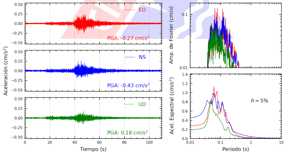
Figura A.6: Registros tiempo-historia, espectros de Fourier y de respuesta en las direcciones EO, NS y vertical de la estación ATARJ. Sismo de Chincha Alta, Chincha - Ica del 2024-12-17, 17:02:05 (Hora local)
