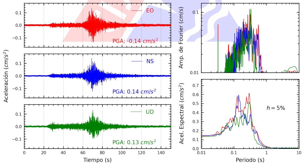
Figura A.8: Registros tiempo-historia, espectros de Fourier y de respuesta en las direcciones EO, NS y vertical de la estación CARAL. Sismo de Chinchá Alta, Chinchá - Ica del 2024-12-17, 17:02:05 (Hora local)
