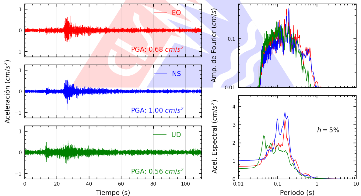
Figura A.2: Registros tiempo-historia, espectros de Fourier y de respuesta en las direcciones EO, NS y vertical de la estación SCICA. Sismo de Chinchá Alta, Chinchá - Ica del 2024-12-17, 17:02:05 (Hora local)
