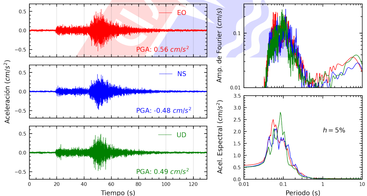
Figura A.4: Registros tiempo-historia, espectros de Fourier y de respuesta en las direcciones EO, NS y vertical de la estación AMORE. Sismo de Chinchá Alta, Chinchá - Ica del 2024-12-17, 17:02:05 (Hora local)
