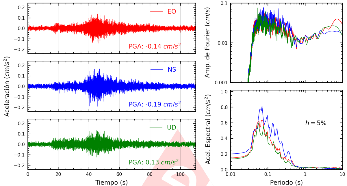
Figura A.7: Registros tiempo-historia, espectros de Fourier y de respuesta en las direcciones EO, NS y vertical de la estación SERVI. Sismo de Chinchá Alta, Chinchá - Ica del 2024-12-17, 17:02:05 (Hora local)
