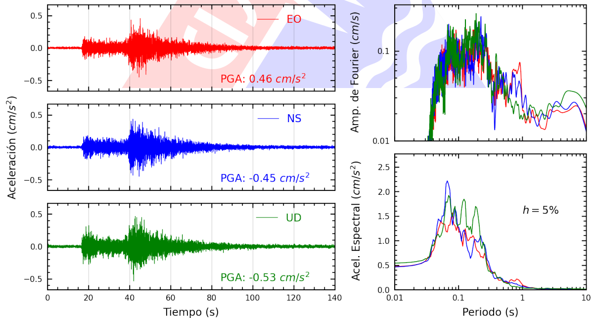
Figura A.30: Registros tiempo-historia, espectros de Fourier y de respuesta en las direcciones EO, NS y vertical de la estación UNFV. Sismo de Barranca, Barranca - Lima del 2024-12-22, 16:38:35 (Hora local)
