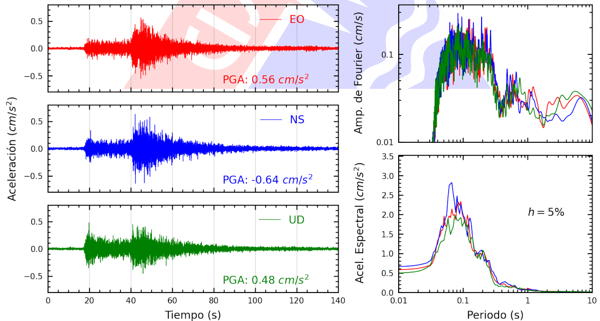
Figura A.28: Registros tiempo-historia, espectros de Fourier y de respuesta en las direcciones EO, NS y vertical de la estación SERVI. Sismo de Barranca, Barranca - Lima del 2024-12-22, 16:38:35 (Hora local)
