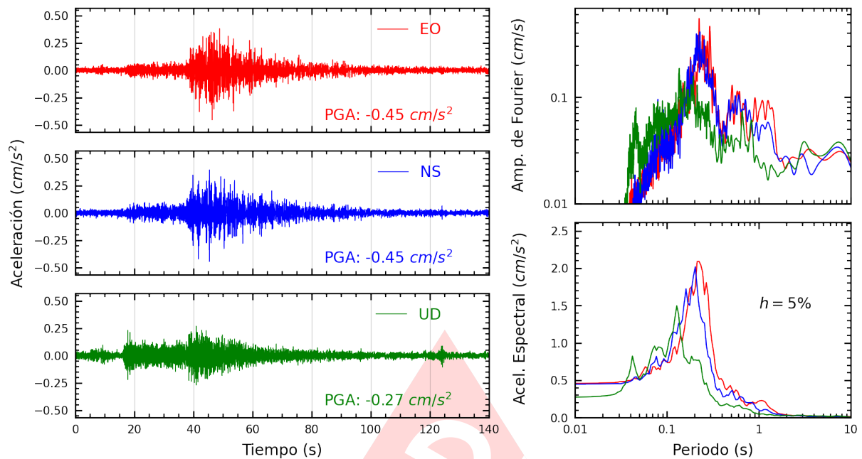
Figura A.31: Registros tiempo-historia, espectros de Fourier y de respuesta en las direcciones EO, NS y vertical de la estación DDMI. Sismo de Barranca, Barranca - Lima del 2024-12-22, 16:38:35 (Hora local)
