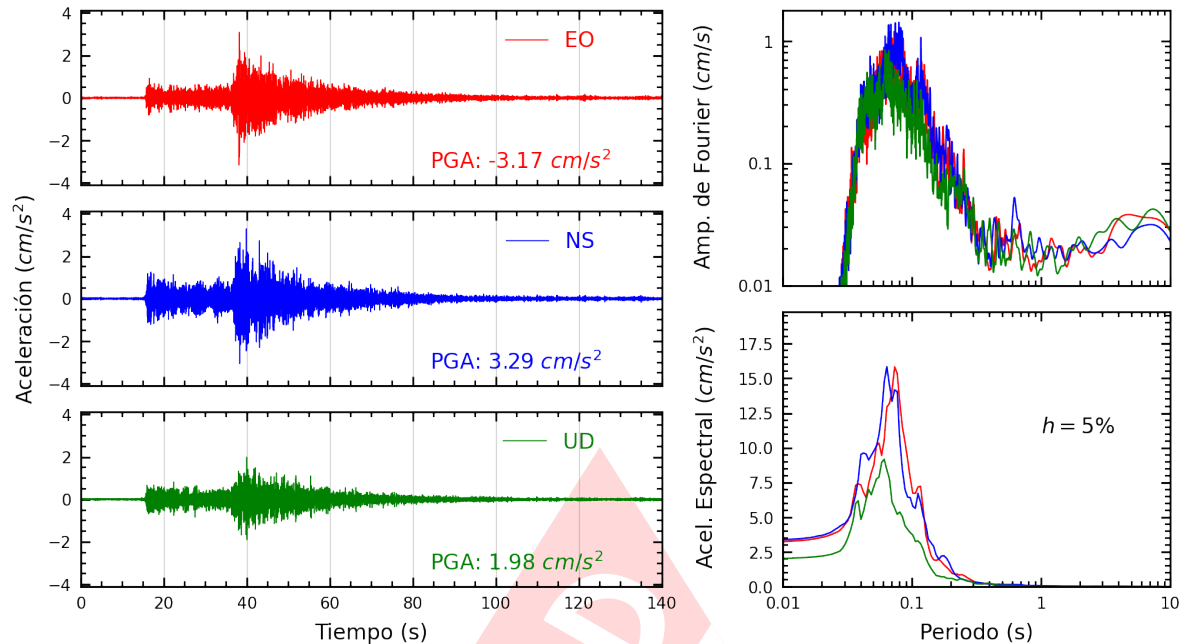
Figura A.3: Registros tiempo-historia, espectros de Fourier y de respuesta en las direcciones EO, NS y vertical de la estación JOSEO. Sismo de Barranca, Barranca - Lima del 2024-12-22, 16:38:35 (Hora local)
