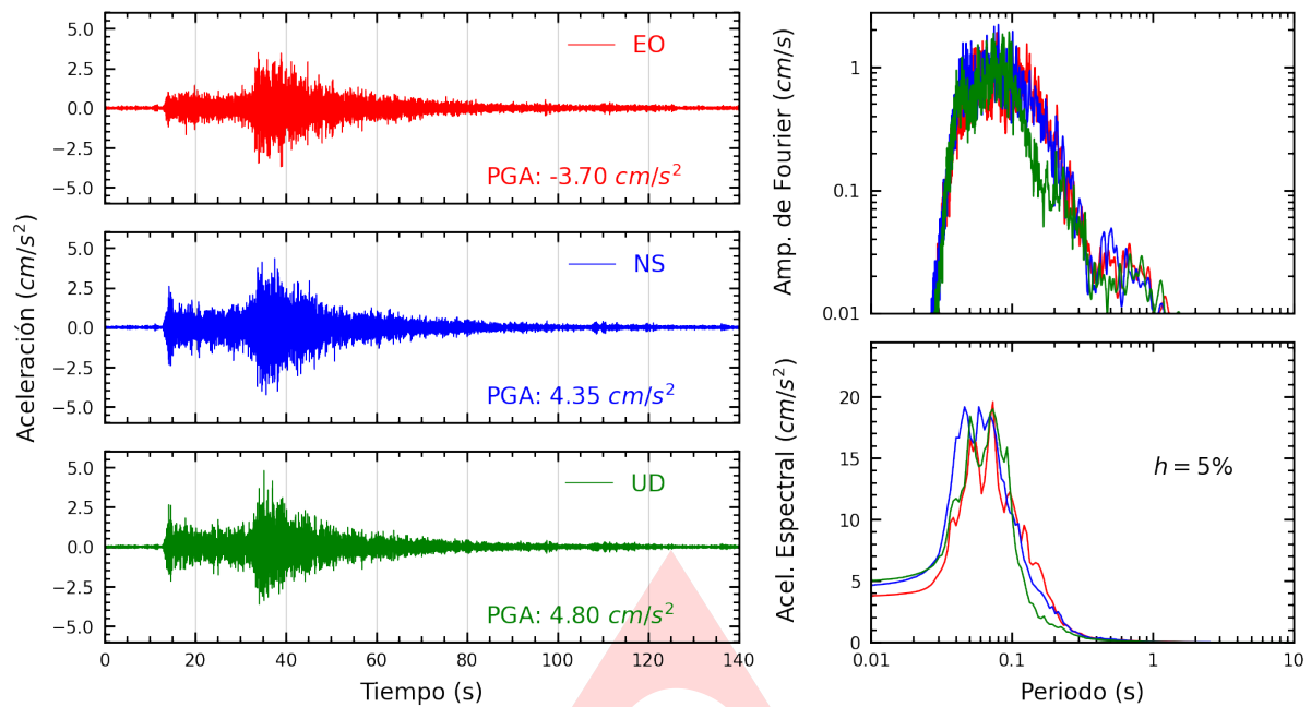
Figura A.1: Registros tiempo-historia, espectros de Fourier y de respuesta en las direcciones EO, NS y vertical de la estación SROS2. Sismo de Barranca, Barranca - Lima del 2024-12-22, 16:38:35 (Hora local)
