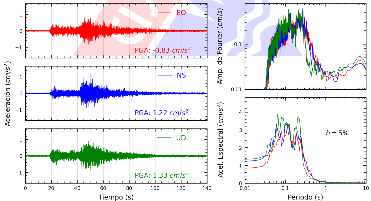
Figura A.14: Registros tiempo-historia, espectros de Fourier y de respuesta en las direcciones EO, NS y vertical de la estación SOVES. Sismo de Barranca, Barranca - Lima del 2024-12-22, 16:38:35 (Hora local)
