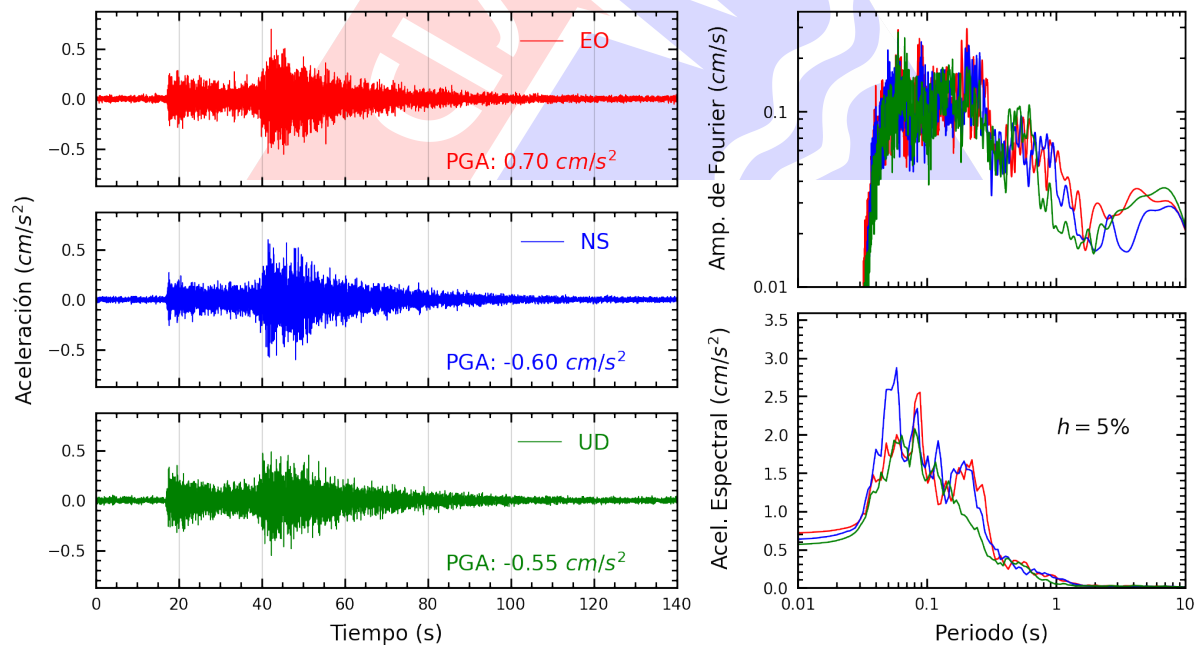
Figura A.26: Registros tiempo-historia, espectros de Fourier y de respuesta en las direcciones EO, NS y vertical de la estación IMCA. Sismo de Barranca, Barranca - Lima del 2024-12-22, 16:38:35 (Hora local)
