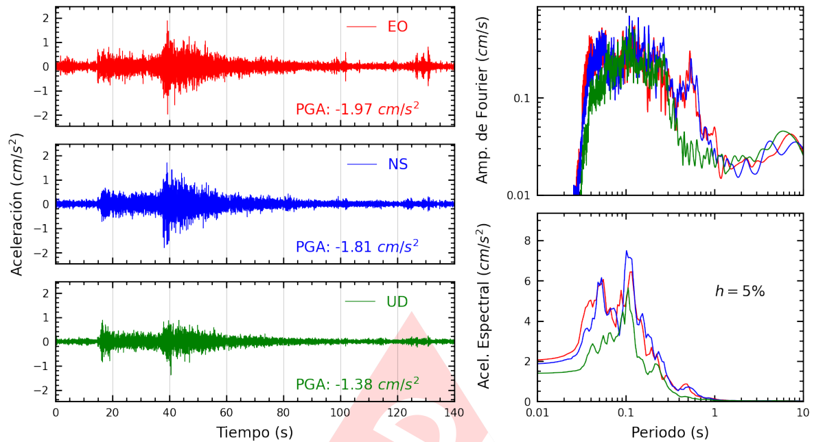
Figura A.9: Registros tiempo-historia, espectros de Fourier y de respuesta en las direcciones EO, NS y vertical de la estación OLIVO. Sismo de Barranca, Barranca - Lima del 2024-12-22, 16:38:35 (Hora local)
