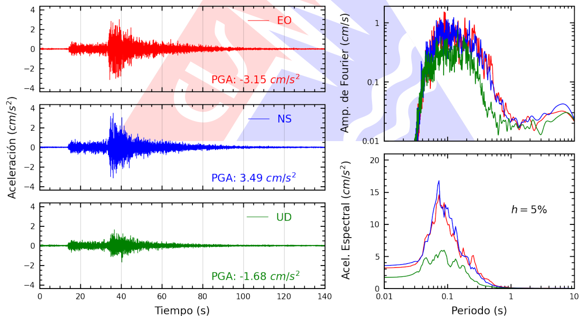
Figura A.2: Registros tiempo-historia, espectros de Fourier y de respuesta en las direcciones EO, NS y vertical de la estación DEFEN. Sismo de Barranca, Barranca - Lima del 2024-12-22, 16:38:35 (Hora local)
