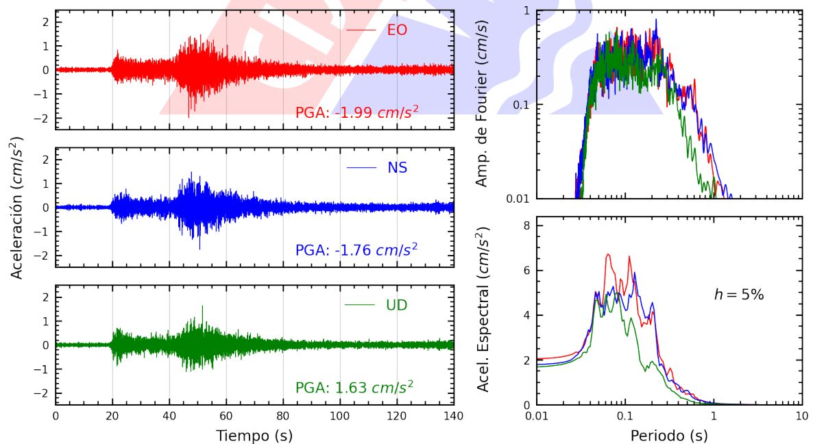
Figura A.8: Registros tiempo-historia, espectros de Fourier y de respuesta en las direcciones EO, NS y vertical de la estación UNTEL. Sismo de Barranca, Barranca - Lima del 2024-12-22, 16:38:35 (Hora local)
