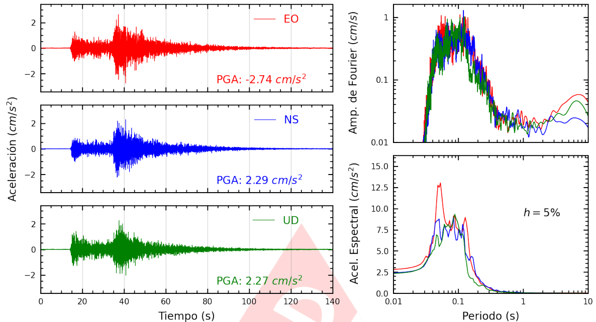
Figura A.5: Registros tiempo-historia, espectros de Fourier y de respuesta en las direcciones EO, NS y vertical de la estación AMORE. Sismo de Barranca, Barranca - Lima del 2024-12-22, 16:38:35 (Hora local)
