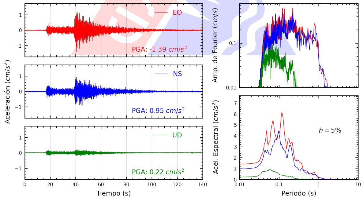
Figura A.12: Registros tiempo-historia, espectros de Fourier y de respuesta en las direcciones EO, NS y vertical de la estación UCVA2. Sismo de Barranca, Barranca - Lima del 2024-12-22, 16:38:35 (Hora local)
