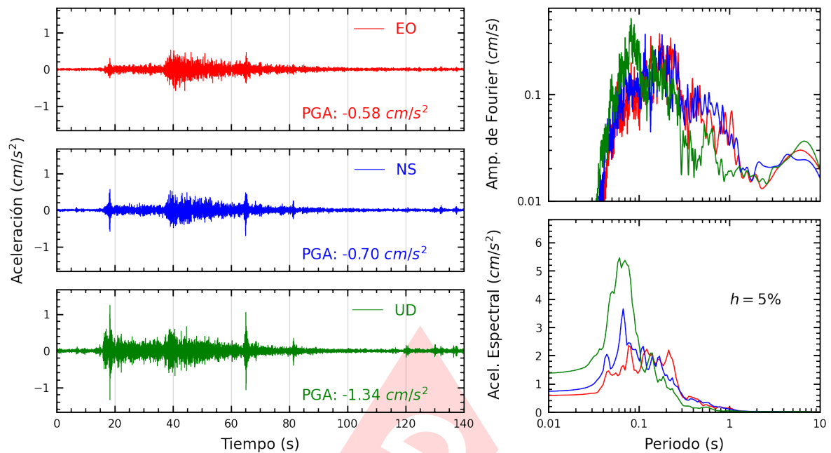
Figura A.13: Registros tiempo-historia, espectros de Fourier y de respuesta en las direcciones EO, NS y vertical de la estación RAMON. Sismo de Barranca, Barranca - Lima del 2024-12-22, 16:38:35 (Hora local)
