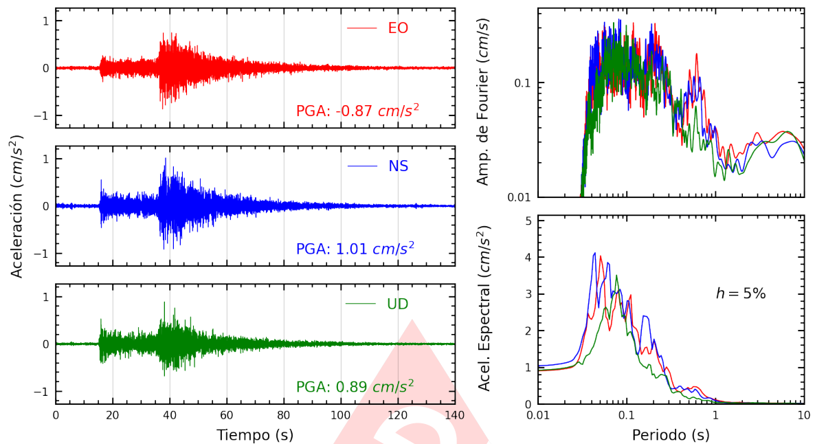
Figura A.17: Registros tiempo-historia, espectros de Fourier y de respuesta en las direcciones EO, NS y vertical de la estación COMAS. Sismo de Barranca, Barranca - Lima del 2024-12-22, 16:38:35 (Hora local)
