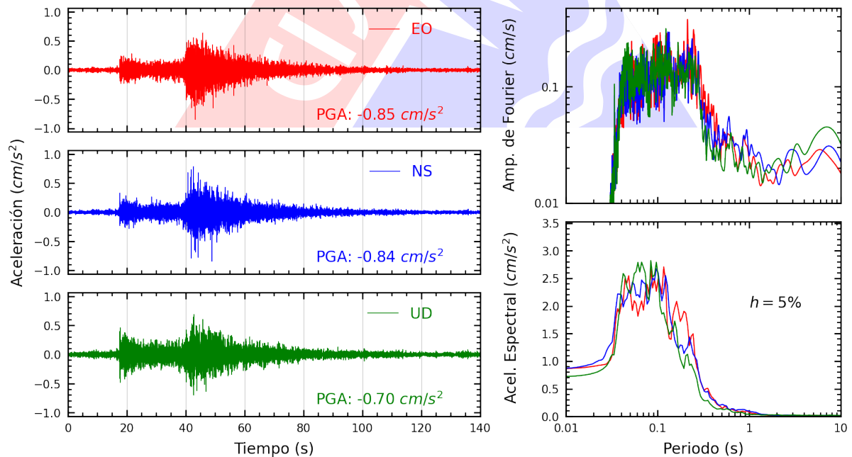
Figura A.24: Registros tiempo-historia, espectros de Fourier y de respuesta en las direcciones EO, NS y vertical de la estación USMP. Sismo de Barranca, Barranca - Lima del 2024-12-22, 16:38:35 (Hora local)
