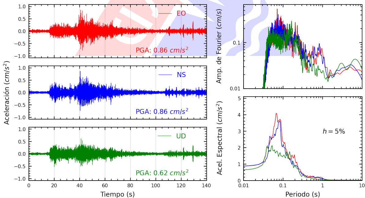
Figura A.22: Registros tiempo-historia, espectros de Fourier y de respuesta en las direcciones EO, NS y vertical de la estación UPCSM. Sismo de Barranca, Barranca - Lima del 2024-12-22, 16:38:35 (Hora local)
