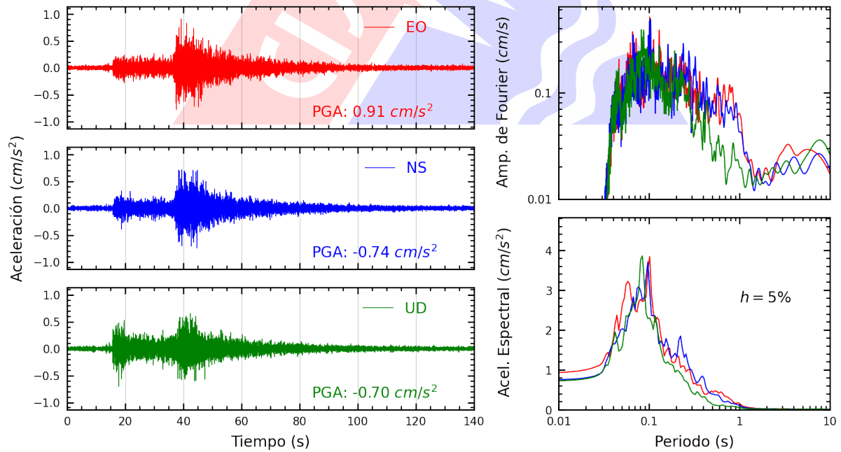
Figura A.20: Registros tiempo-historia, espectros de Fourier y de respuesta en las direcciones EO, NS y vertical de la estación MADRE. Sismo de Barranca, Barranca - Lima del 2024-12-22, 16:38:35 (Hora local)
