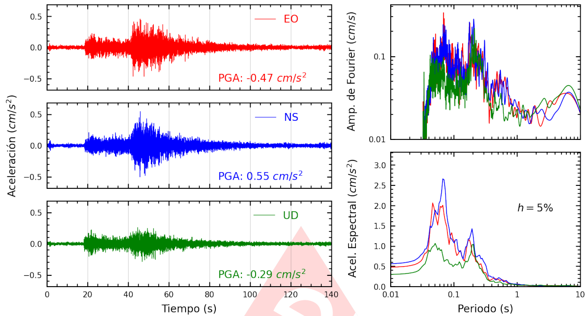
Figura A.29: Registros tiempo-historia, espectros de Fourier y de respuesta en las direcciones EO, NS y vertical de la estación UPCVI. Sismo de Barranca, Barranca - Lima del 2024-12-22, 16:38:35 (Hora local)
