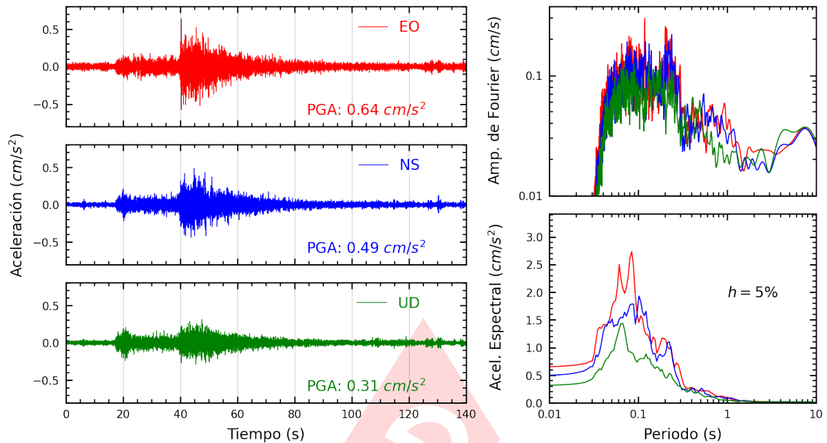
Figura A.27: Registros tiempo-historia, espectros de Fourier y de respuesta en las direcciones EO, NS y vertical de la estación INICT. Sismo de Barranca, Barranca - Lima del 2024-12-22, 16:38:35 (Hora local)
