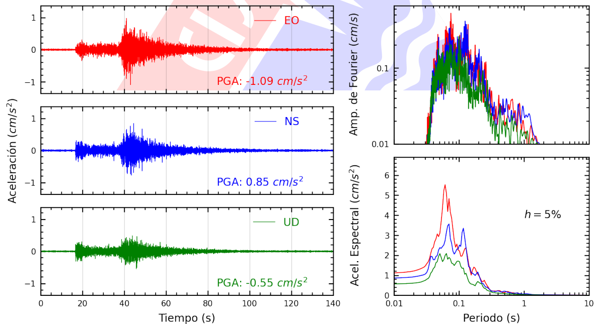
Figura A.16: Registros tiempo-historia, espectros de Fourier y de respuesta en las direcciones EO, NS y vertical de la estación ATARJ. Sismo de Barranca, Barranca - Lima del 2024-12-22, 16:38:35 (Hora local)
