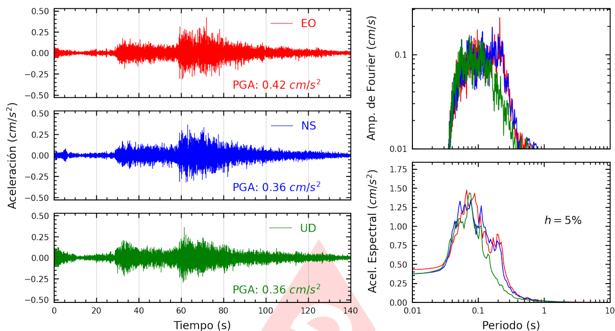
Figura A.33: Registros tiempo-historia, espectros de Fourier y de respuesta en las direcciones EO, NS y vertical de la estación ASIA. Sismo de Barranca, Barranca - Lima del 2024-12-22, 16:38:35 (Hora local)
