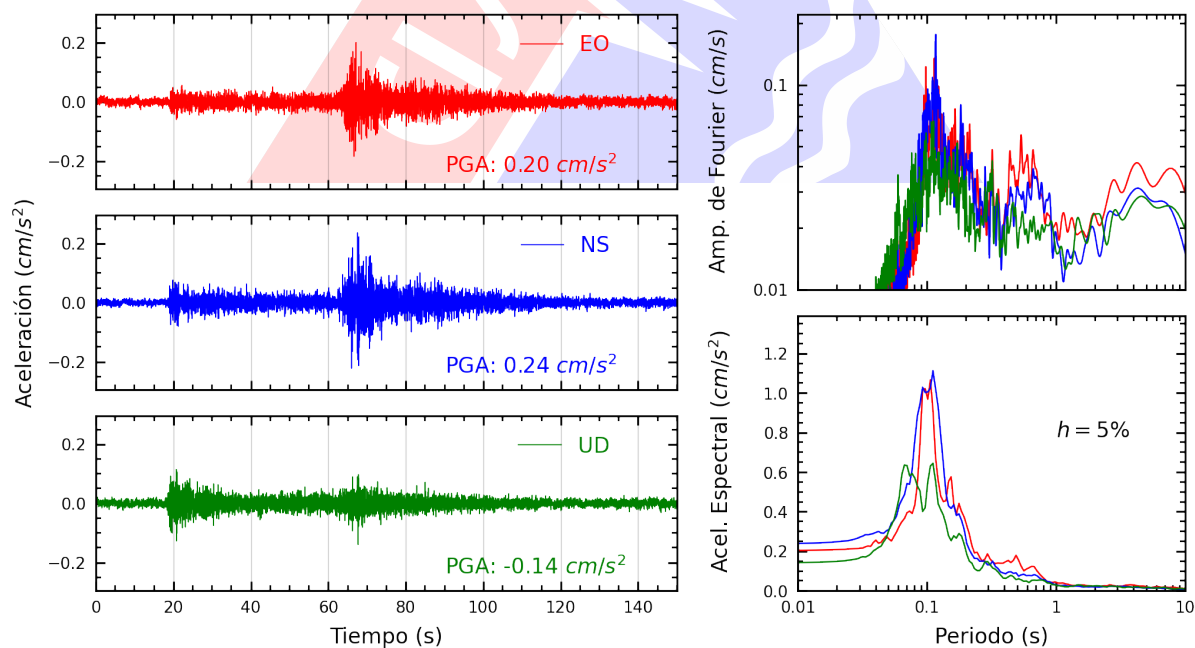
Figura A.34: Registros tiempo-historia, espectros de Fourier y de respuesta en las direcciones EO, NS y vertical de la estación UCVCH. Sismo de Barranca, Barranca - Lima del 2024-12-22, 16:38:35 (Hora local)
