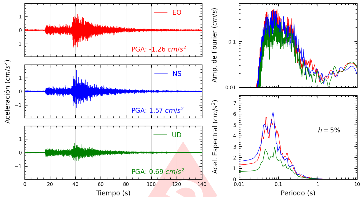
Figura A.11: Registros tiempo-historia, espectros de Fourier y de respuesta en las direcciones EO, NS y vertical de la estación FICPE. Sismo de Barranca, Barranca - Lima del 2024-12-22, 16:38:35 (Hora local)
