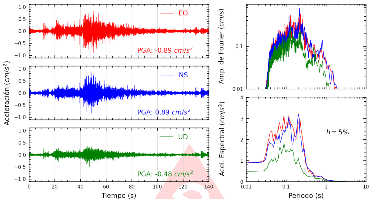
Figura A.21: Registros tiempo-historia, espectros de Fourier y de respuesta en las direcciones EO, NS y vertical de la estación BRISA. Sismo de Barranca, Barranca - Lima del 2024-12-22, 16:38:35 (Hora local)
