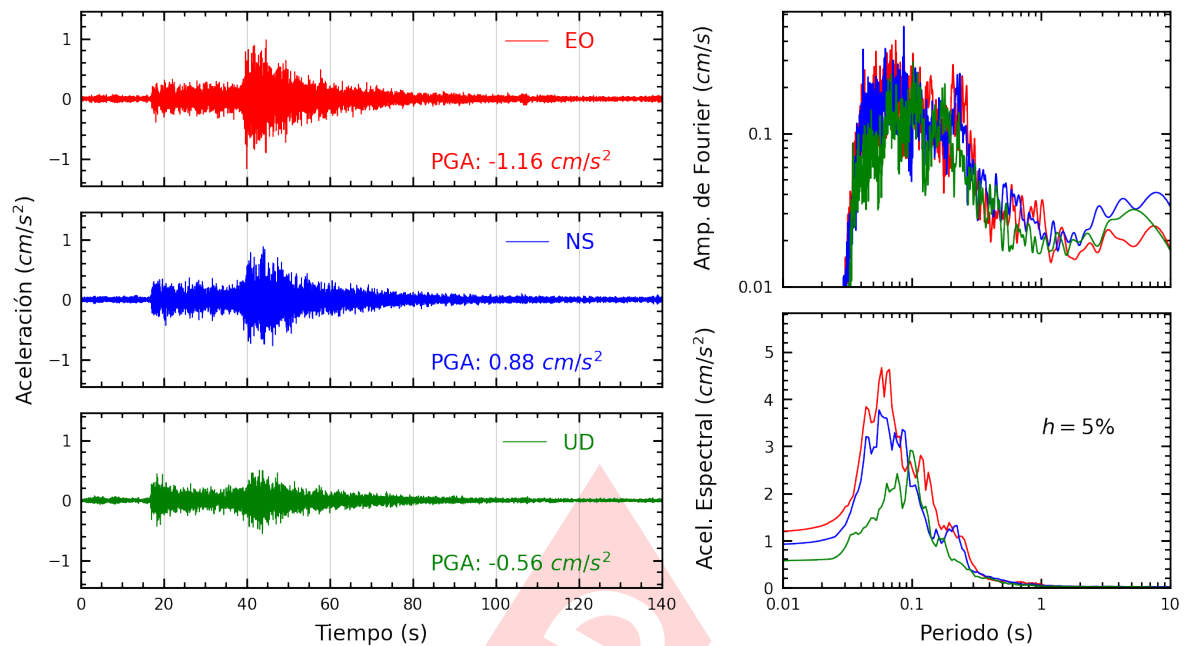
Figura A.15: Registros tiempo-historia, espectros de Fourier y de respuesta en las direcciones EO, NS y vertical de la estación CEPRE. Sismo de Barranca, Barranca - Lima del 2024-12-22, 16:38:35 (Hora local)
