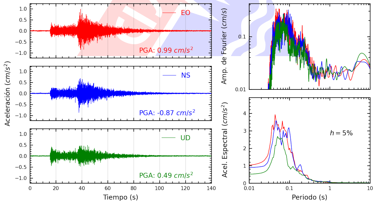
Figura A.18: Registros tiempo-historia, espectros de Fourier y de respuesta en las direcciones EO, NS y vertical de la estación UCSS. Sismo de Barranca, Barranca - Lima del 2024-12-22, 16:38:35 (Hora local)
