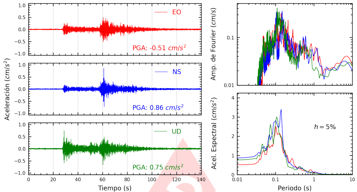
Figura A.23: Registros tiempo-historia, espectros de Fourier y de respuesta en las direcciones EO, NS y vertical de la estación UPAOT. Sismo de Barranca, Barranca - Lima del 2024-12-22, 16:38:35 (Hora local)
