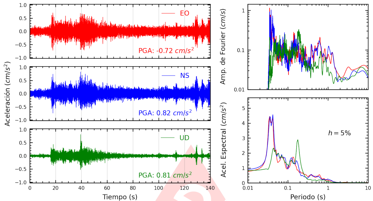
Figura A.25: Registros tiempo-historia, espectros de Fourier y de respuesta en las direcciones EO, NS y vertical de la estación DHNPE. Sismo de Barranca, Barranca - Lima del 2024-12-22, 16:38:35 (Hora local)
