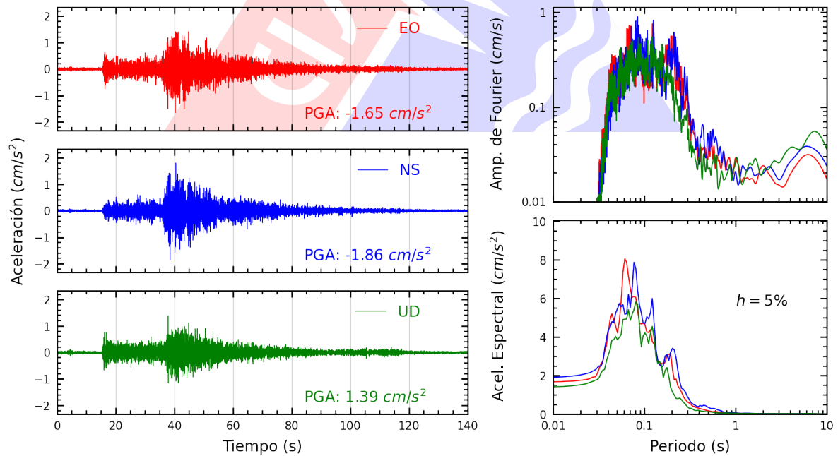
Figura A.10: Registros tiempo-historia, espectros de Fourier y de respuesta en las direcciones EO, NS y vertical de la estación INDEP. Sismo de Barranca, Barranca - Lima del 2024-12-22, 16:38:35 (Hora local)
