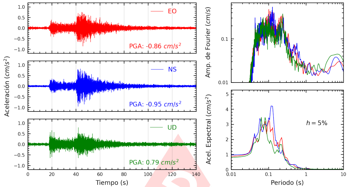
Figura A.19: Registros tiempo-historia, espectros de Fourier y de respuesta en las direcciones EO, NS y vertical de la estación URPPE. Sismo de Barranca, Barranca - Lima del 2024-12-22, 16:38:35 (Hora local)
