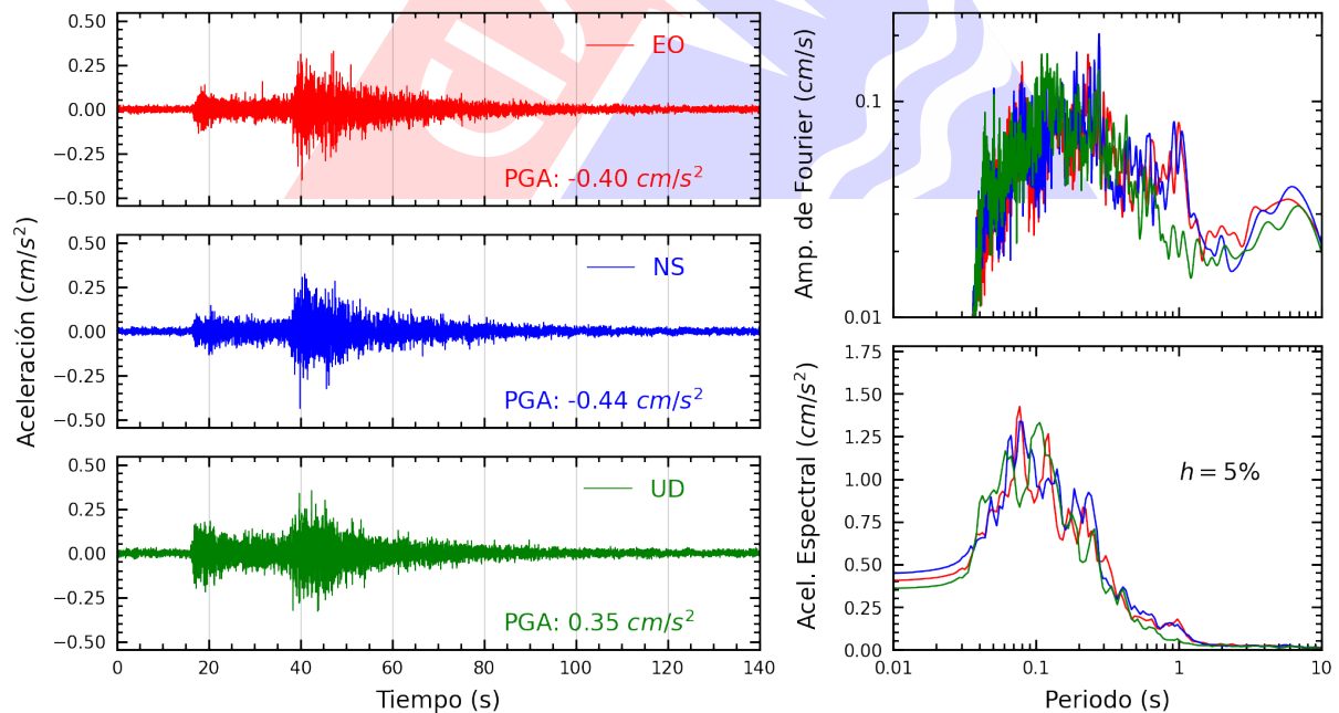
Figura A.32: Registros tiempo-historia, espectros de Fourier y de respuesta en las direcciones EO, NS y vertical de la estación BONDY. Sismo de Barranca, Barranca - Lima del 2024-12-22, 16:38:35 (Hora local)
