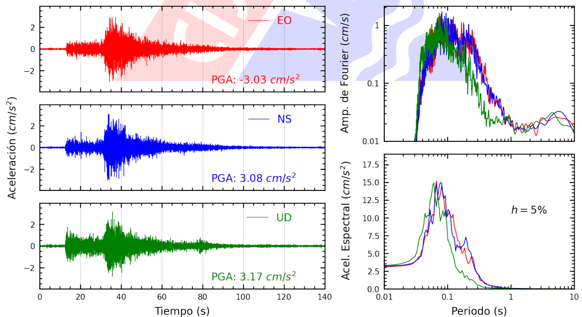
Figura A.4: Registros tiempo-historia, espectros de Fourier y de respuesta en las direcciones EO, NS y vertical de la estación ANCON. Sismo de Barranca, Barranca - Lima del 2024-12-22, 16:38:35 (Hora local)
