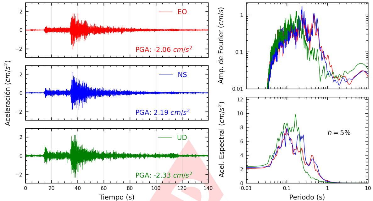
Figura A.7: Registros tiempo-historia, espectros de Fourier y de respuesta en las direcciones EO, NS y vertical de la estación MDPP. Sismo de Barranca, Barranca - Lima del 2024-12-22, 16:38:35 (Hora local)
