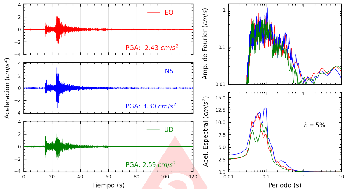
Figura A.25: Registros tiempo-historia, espectros de Fourier y de respuesta en las direcciones EO, NS y vertical de la estación MADRE. Sismo de Chilca, Cañete - Lima del 2024-12-23, 21:05:42 (Hora local)
