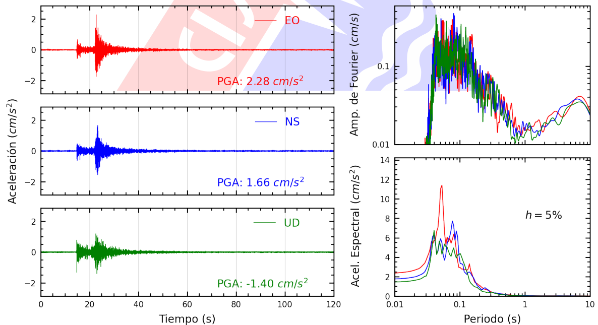
Figura A.28: Registros tiempo-historia, espectros de Fourier y de respuesta en las direcciones EO, NS y vertical de la estación BONDY. Sismo de Chilca, Cañete - Lima del 2024-12-23, 21:05:42 (Hora local)
