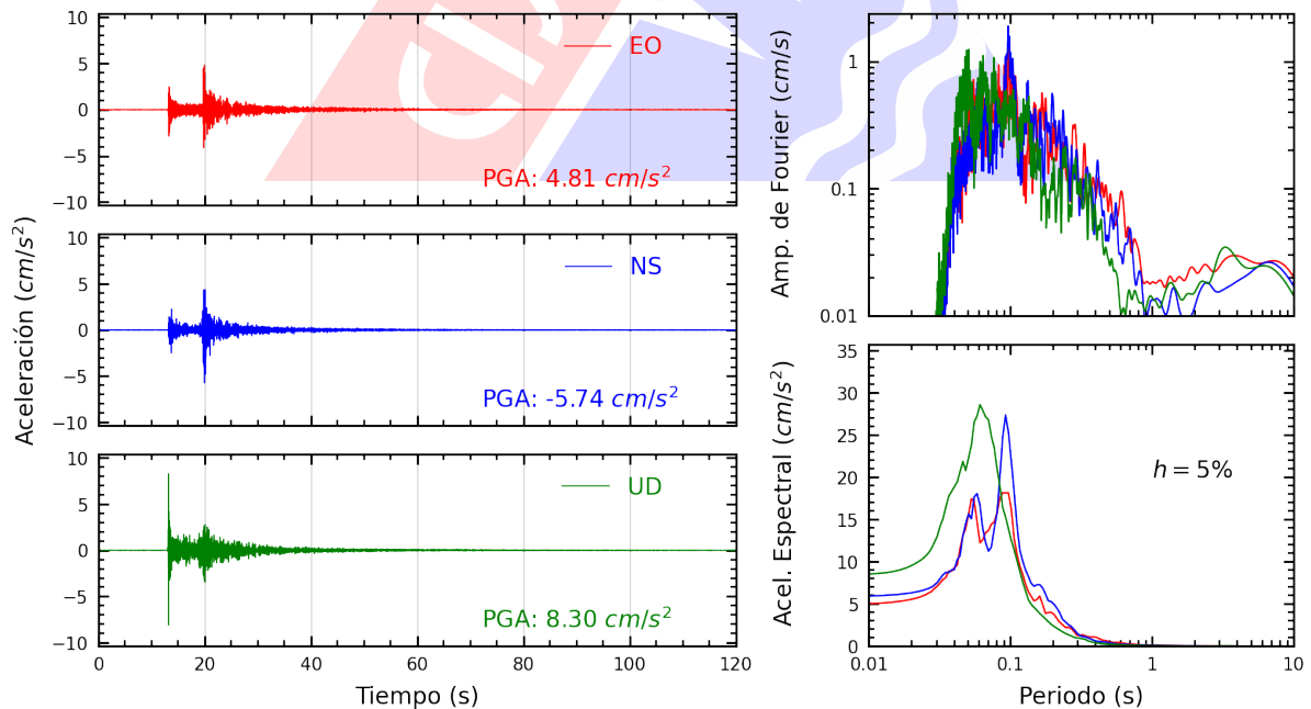
Figura A.8: Registros tiempo-historia, espectros de Fourier y de respuesta en las direcciones EO, NS y vertical de la estación USILP. Sismo de Chilca, Cañete - Lima del 2024-12-23, 21:05:42 (Hora local)
