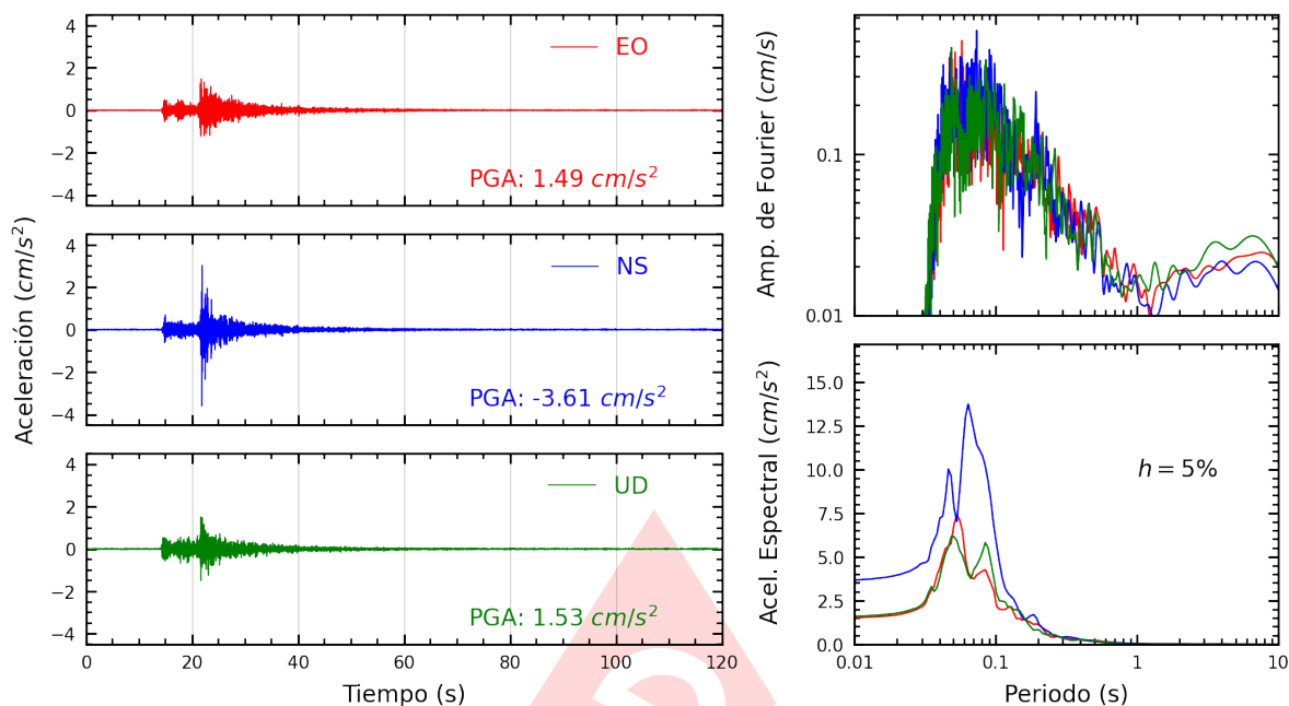
Figura A.23: Registros tiempo-historia, espectros de Fourier y de respuesta en las direcciones EO, NS y vertical de la estación UNFV. Sismo de Chilca, Cañete - Lima del 2024-12-23, 21:05:42 (Hora local)
