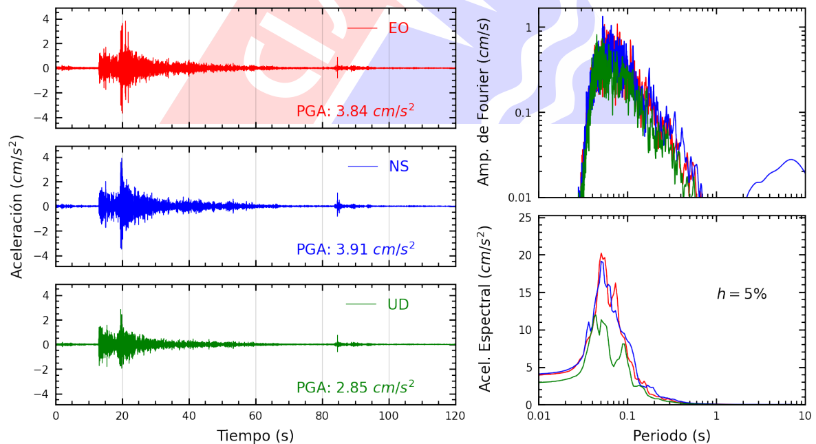
Figura A.22: Registros tiempo-historia, espectros de Fourier y de respuesta en las direcciones EO, NS y vertical de la estación PACHA. Sismo de Chilca, Cañete - Lima del 2024-12-23, 21:05:42 (Hora local)
