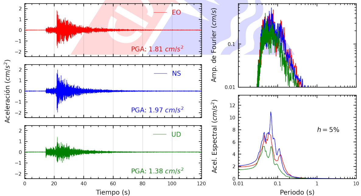
Figura A.30: Registros tiempo-historia, espectros de Fourier y de respuesta en las direcciones EO, NS y vertical de la estación ATARJ. Sismo de Chilca, Cañete - Lima del 2024-12-23, 21:05:42 (Hora local)
