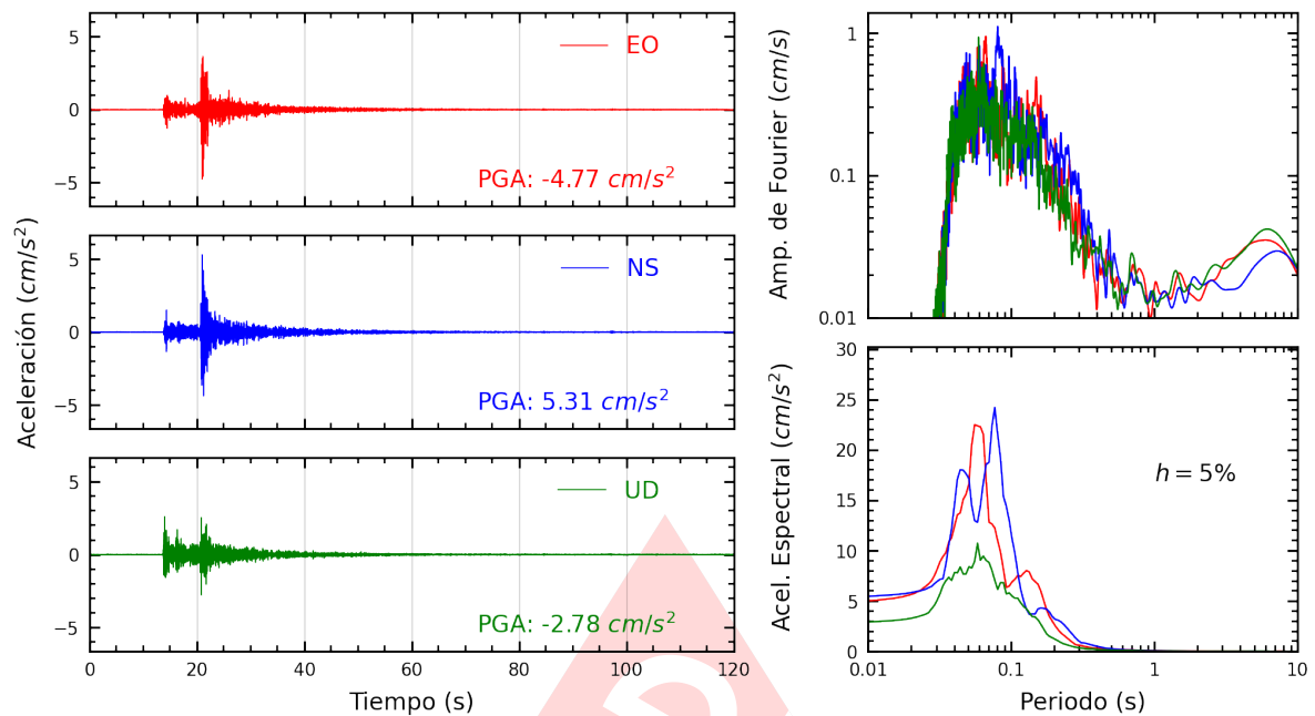
Figura A.13: Registros tiempo-historia, espectros de Fourier y de respuesta en las direcciones EO, NS y vertical de la estación SERVI. Sismo de Chilca, Cañete - Lima del 2024-12-23, 21:05:42 (Hora local)
