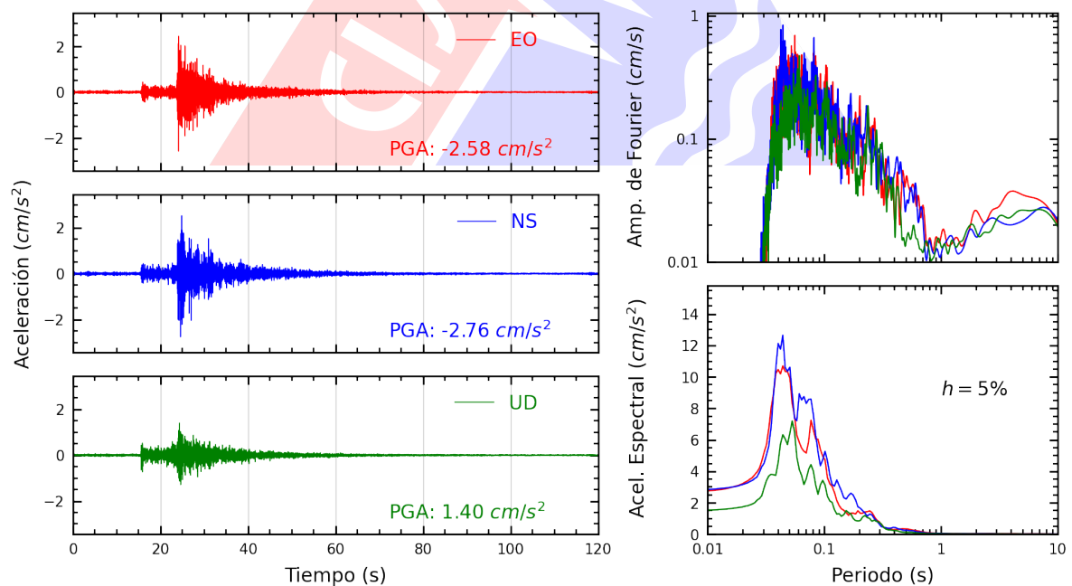
Figura A.26: Registros tiempo-historia, espectros de Fourier y de respuesta en las direcciones EO, NS y vertical de la estación COMAS. Sismo de Chilca, Cañete - Lima del 2024-12-23, 21:05:42 (Hora local)
