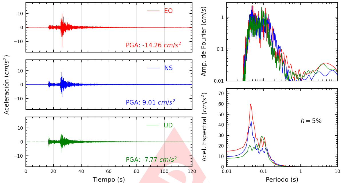
Figura A.3: Registros tiempo-historia, espectros de Fourier y de respuesta en las direcciones EO, NS y vertical de la estación AMORE. Sismo de Chilca, Cañete - Lima del 2024-12-23, 21:05:42 (Hora local)
