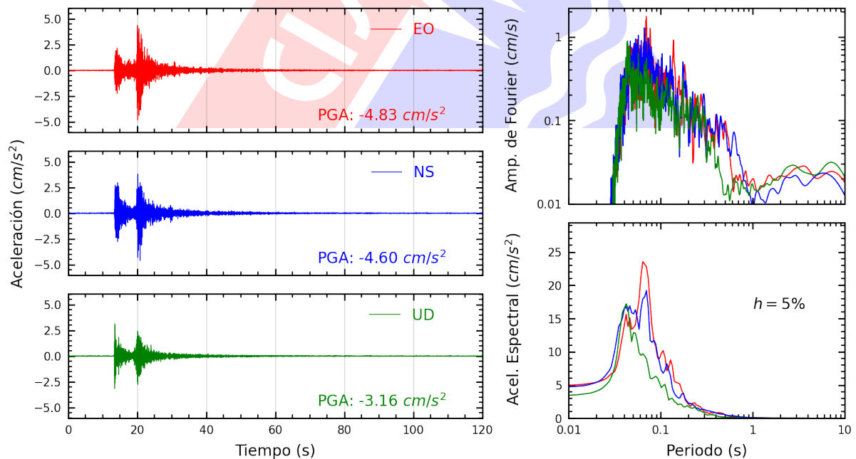
Figura A.14: Registros tiempo-historia, espectros de Fourier y de respuesta en las direcciones EO, NS y vertical de la estación UPCVI. Sismo de Chilca, Cañete - Lima del 2024-12-23, 21:05:42 (Hora local)
