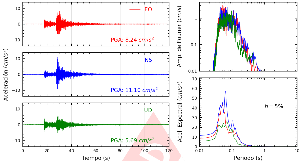
Figura A.5: Registros tiempo-historia, espectros de Fourier y de respuesta en las direcciones EO, NS y vertical de la estación SROS2. Sismo de Chilca, Cañete - Lima del 2024-12-23, 21:05:42 (Hora local)
