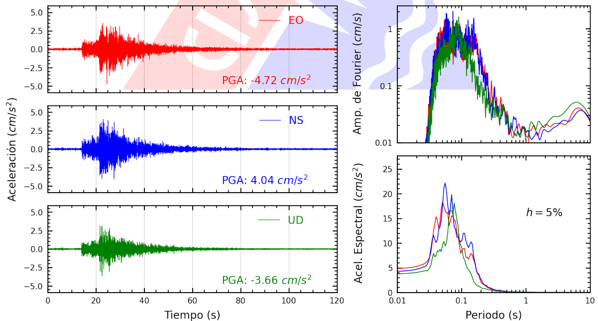
Figura A.16: Registros tiempo-historia, espectros de Fourier y de respuesta en las direcciones EO, NS y vertical de la estación USILM. Sismo de Chilca, Cañete - Lima del 2024-12-23, 21:05:42 (Hora local)
