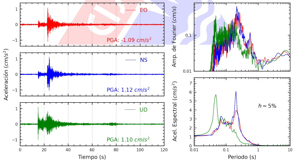
Figura A.34: Registros tiempo-historia, espectros de Fourier y de respuesta en las direcciones EO, NS y vertical de la estación DSMI. Sismo de Chilca, Cañete - Lima del 2024-12-23, 21:05:42 (Hora local)
