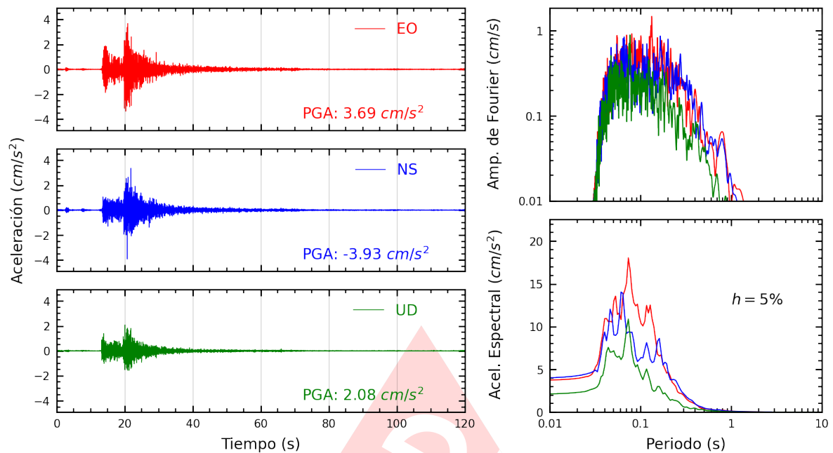
Figura A.21: Registros tiempo-historia, espectros de Fourier y de respuesta en las direcciones EO, NS y vertical de la estación BRISA. Sismo de Chilca, Cañete - Lima del 2024-12-23, 21:05:42 (Hora local)
