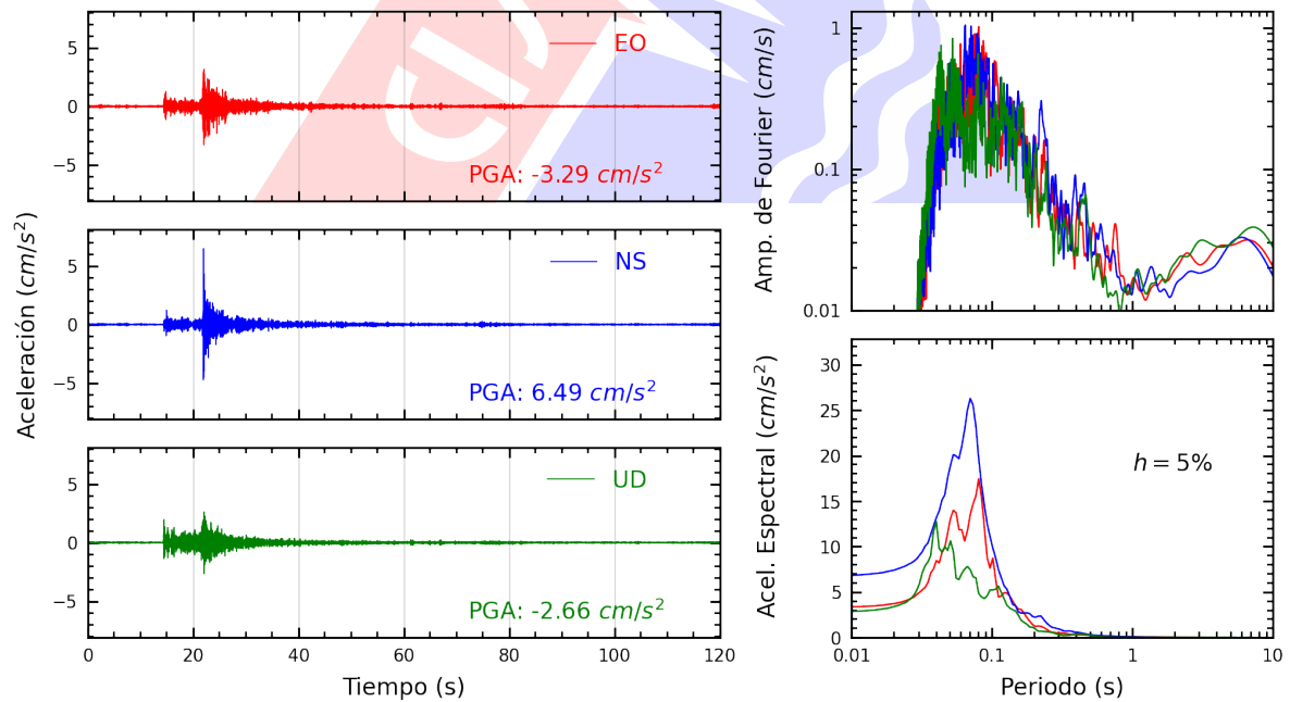
Figura A.10: Registros tiempo-historia, espectros de Fourier y de respuesta en las direcciones EO, NS y vertical de la estación UPCSM. Sismo de Chilca, Cañete - Lima del 2024-12-23, 21:05:42 (Hora local)
