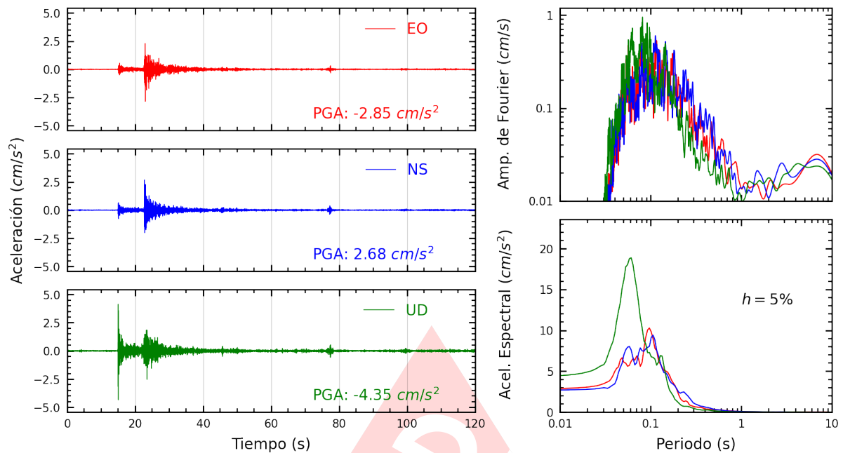
Figura A.19: Registros tiempo-historia, espectros de Fourier y de respuesta en las direcciones EO, NS y vertical de la estación RAMON. Sismo de Chilca, Cañete - Lima del 2024-12-23, 21:05:42 (Hora local)
