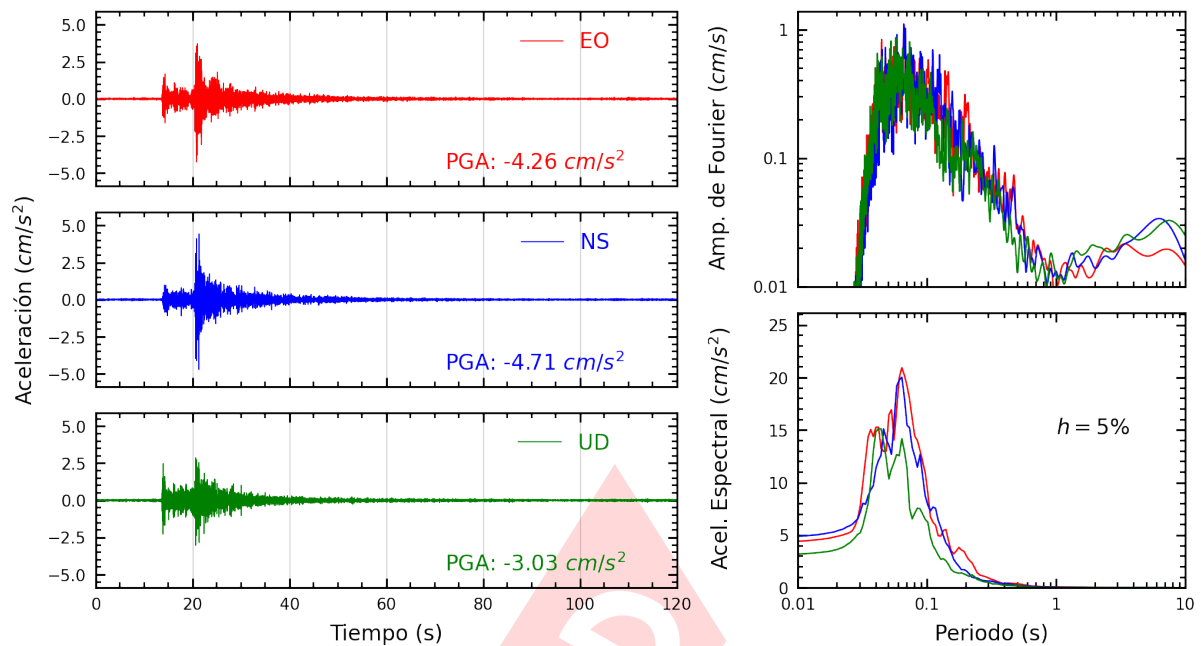
Figura A.17: Registros tiempo-historia, espectros de Fourier y de respuesta en las direcciones EO, NS y vertical de la estación URPPE. Sismo de Chilca, Cañete - Lima del 2024-12-23, 21:05:42 (Hora local)
