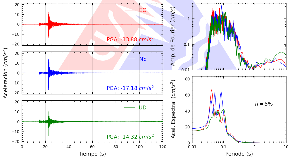
Figura A.2: Registros tiempo-historia, espectros de Fourier y de respuesta en las direcciones EO, NS y vertical de la estación INDEP. Sismo de Chilca, Cañete - Lima del 2024-12-23, 21:05:42 (Hora local)
