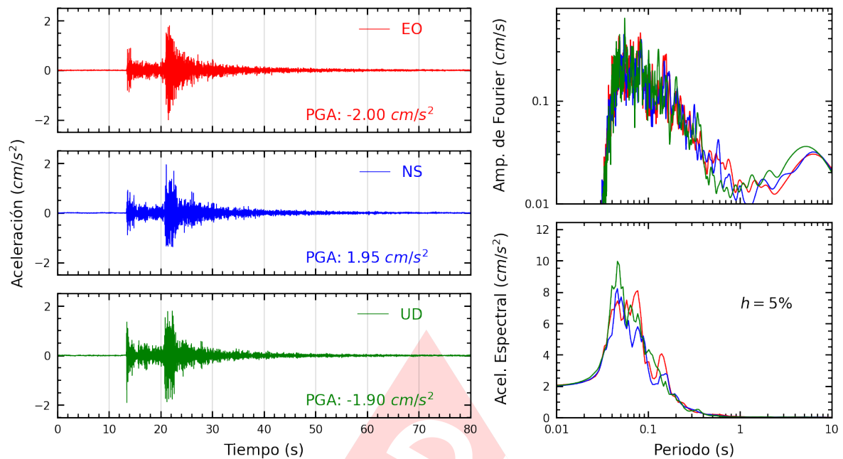
Figura A.29: Registros tiempo-historia, espectros de Fourier y de respuesta en las direcciones EO, NS y vertical de la estación UNMSM. Sismo de Chilca, Cañete - Lima del 2024-12-23, 21:05:42 (Hora local)
