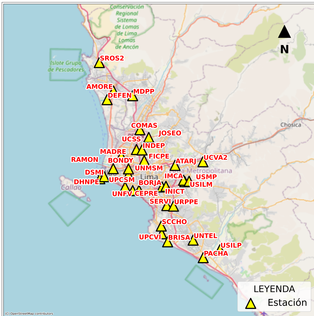
Figura 3: Mapa de ubicación de la(s) estación(es) acelerográfica(s) en Lima Metropolitana correspondiente(s) al Sismo de Chilca, Cañete - Lima del 23 de diciembre de 2024 a las 21:05:42 (hora local)
