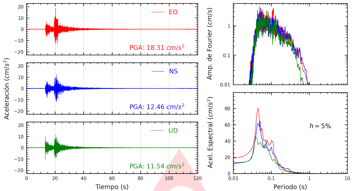
Figura A.1: Registros tiempo-historia, espectros de Fourier y de respuesta en las direcciones EO, NS y vertical de la estación UNTEL. Sismo de Chilca, Cañete - Lima del 2024-12-23, 21:05:42 (Hora local)
