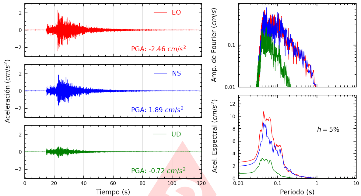
Figura A.27: Registros tiempo-historia, espectros de Fourier y de respuesta en las direcciones EO, NS y vertical de la estación UCVA2. Sismo de Chilca, Cañete - Lima del 2024-12-23, 21:05:42 (Hora local)
