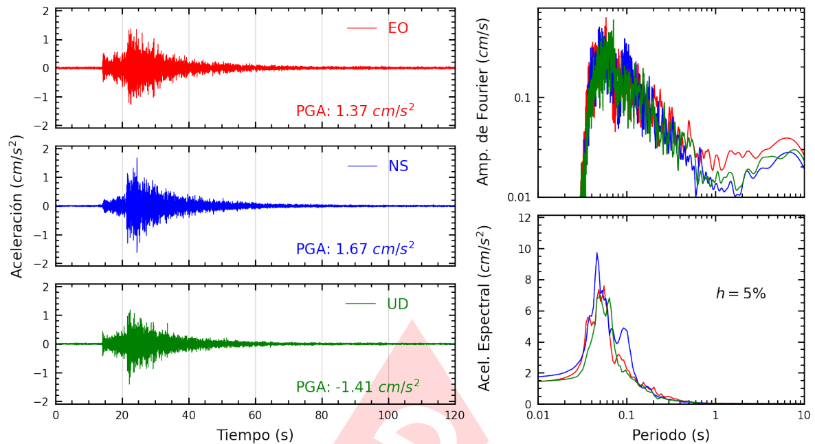
Figura A.31: Registros tiempo-historia, espectros de Fourier y de respuesta en las direcciones EO, NS y vertical de la estación IMCA. Sismo de Chilca, Cañete - Lima del 2024-12-23, 21:05:42 (Hora local)
