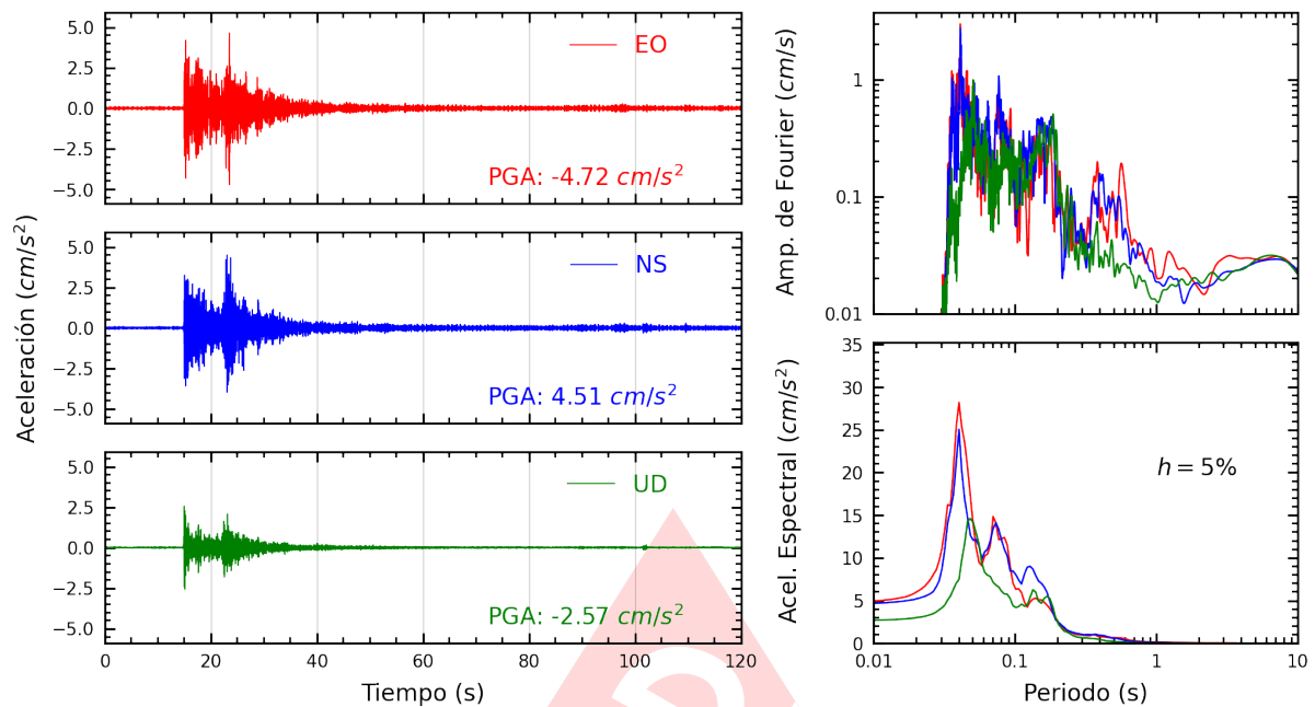
Figura A.15: Registros tiempo-historia, espectros de Fourier y de respuesta en las direcciones EO, NS y vertical de la estación DHNPE. Sismo de Chilca, Cañete - Lima del 2024-12-23, 21:05:42 (Hora local)
