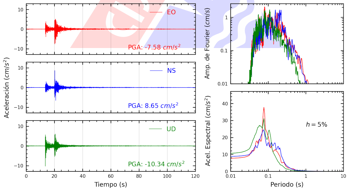
Figura A.6: Registros tiempo-historia, espectros de Fourier y de respuesta en las direcciones EO, NS y vertical de la estación SCCHO. Sismo de Chilca, Cañete - Lima del 2024-12-23, 21:05:42 (Hora local)
