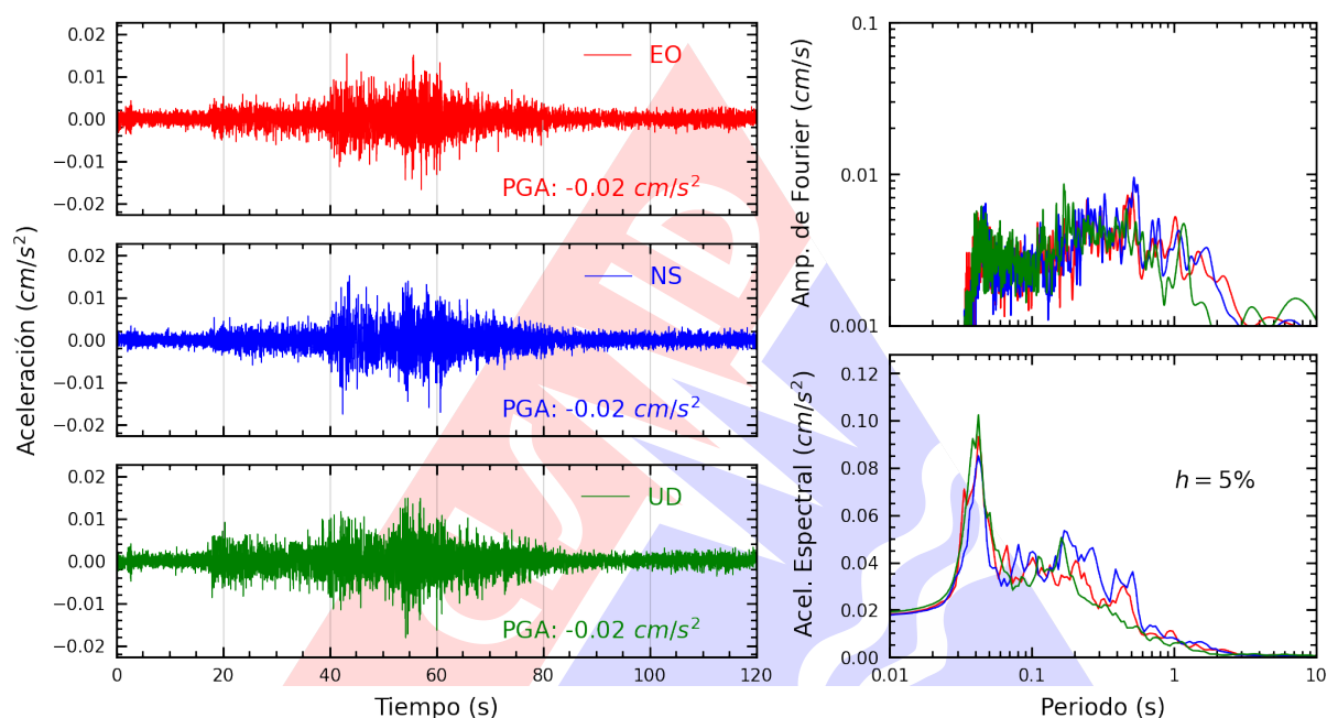
Figura A.35: Registros tiempo-historia, espectros de Fourier y de respuesta en las direcciones EO, NS y vertical de la estación UNCP. Sismo de Chilca, Cañete - Lima del 2024-12-23, 21:05:42 (Hora local)
