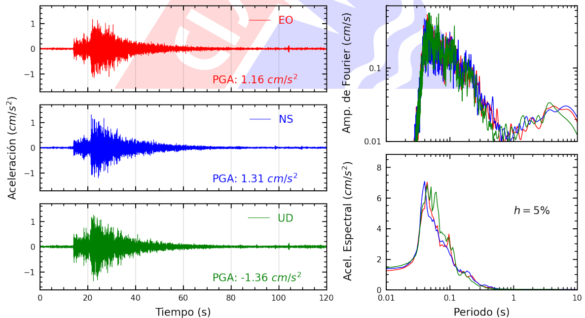
Figura A.32: Registros tiempo-historia, espectros de Fourier y de respuesta en las direcciones EO, NS y vertical de la estación USMP. Sismo de Chilca, Cañete - Lima del 2024-12-23, 21:05:42 (Hora local)
