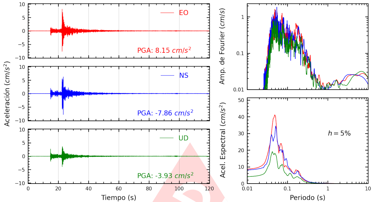
Figura A.9: Registros tiempo-historia, espectros de Fourier y de respuesta en las direcciones EO, NS y vertical de la estación FICPE. Sismo de Chilca, Cañete - Lima del 2024-12-23, 21:05:42 (Hora local)
