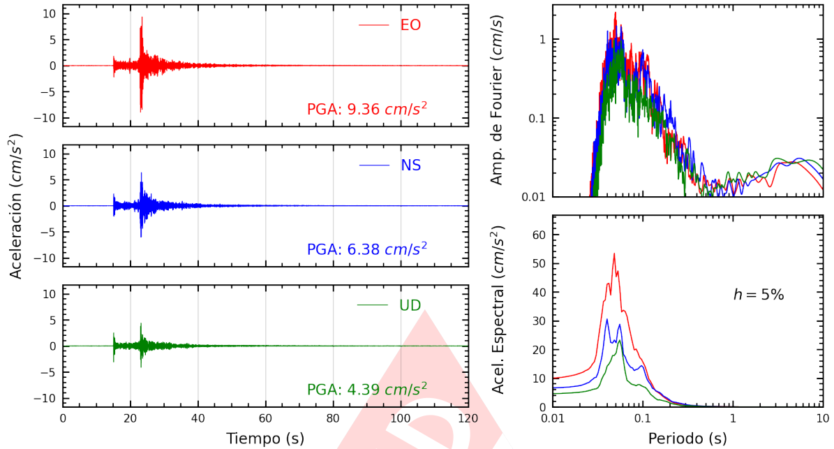
Figura A.7: Registros tiempo-historia, espectros de Fourier y de respuesta en las direcciones EO, NS y vertical de la estación UCSS. Sismo de Chilca, Cañete - Lima del 2024-12-23, 21:05:42 (Hora local)
