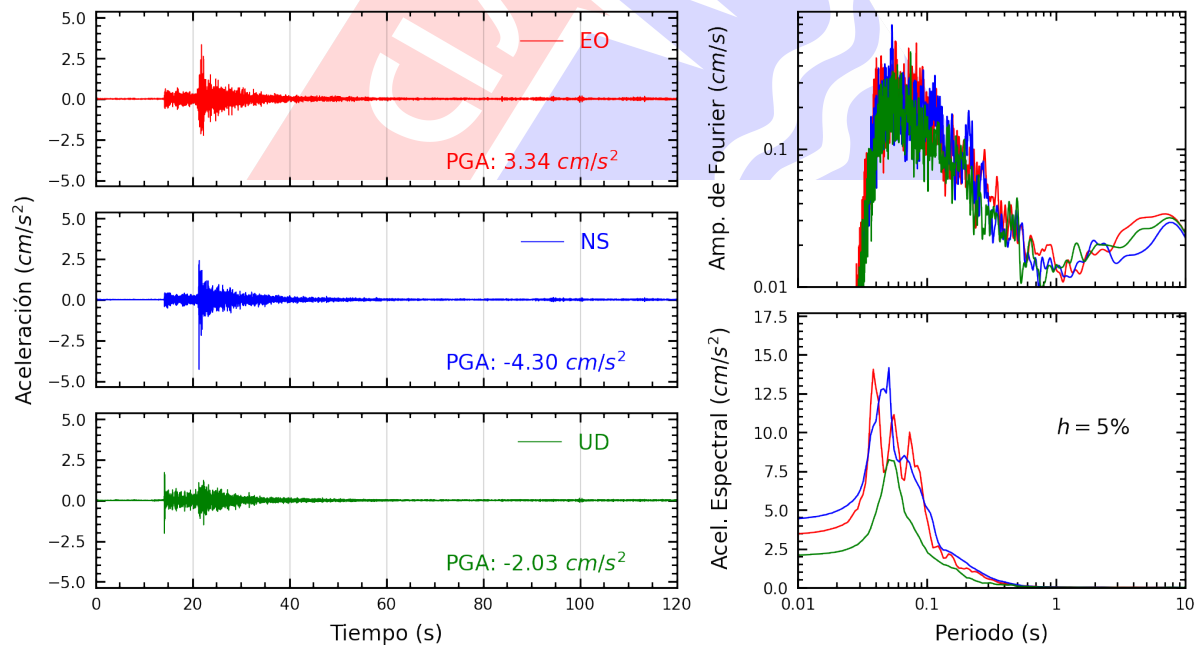
Figura A.20: Registros tiempo-historia, espectros de Fourier y de respuesta en las direcciones EO, NS y vertical de la estación INICT. Sismo de Chilca, Cañete - Lima del 2024-12-23, 21:05:42 (Hora local)
