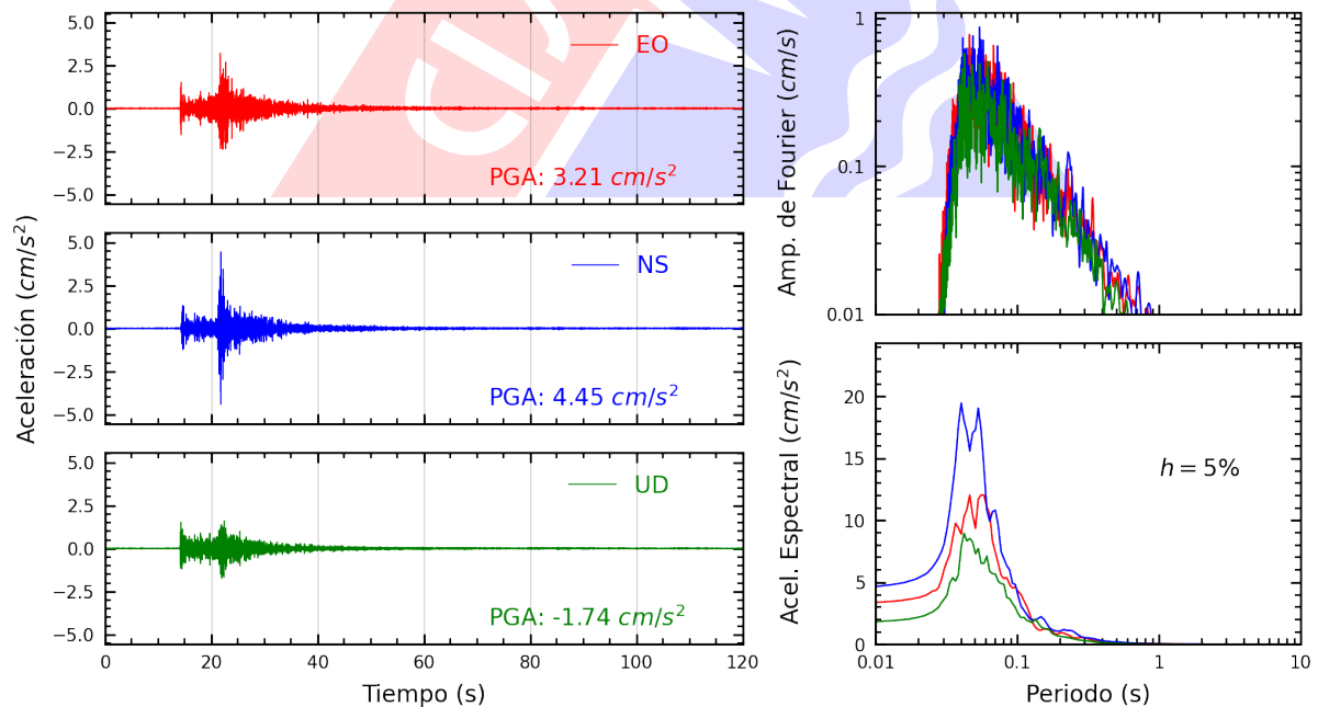
Figura A.18: Registros tiempo-historia, espectros de Fourier y de respuesta en las direcciones EO, NS y vertical de la estación BORJA. Sismo de Chilca, Cañete - Lima del 2024-12-23, 21:05:42 (Hora local)
