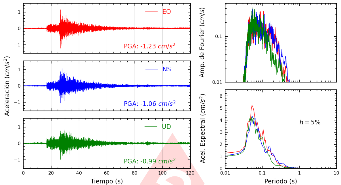
Figura A.33: Registros tiempo-historia, espectros de Fourier y de respuesta en las direcciones EO, NS y vertical de la estación ASIA. Sismo de Chilca, Cañete - Lima del 2024-12-23, 21:05:42 (Hora local)
