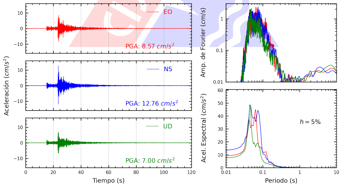
Figura A.4: Registros tiempo-historia, espectros de Fourier y de respuesta en las direcciones EO, NS y vertical de la estación JOSEO. Sismo de Chilca, Cañete - Lima del 2024-12-23, 21:05:42 (Hora local)
