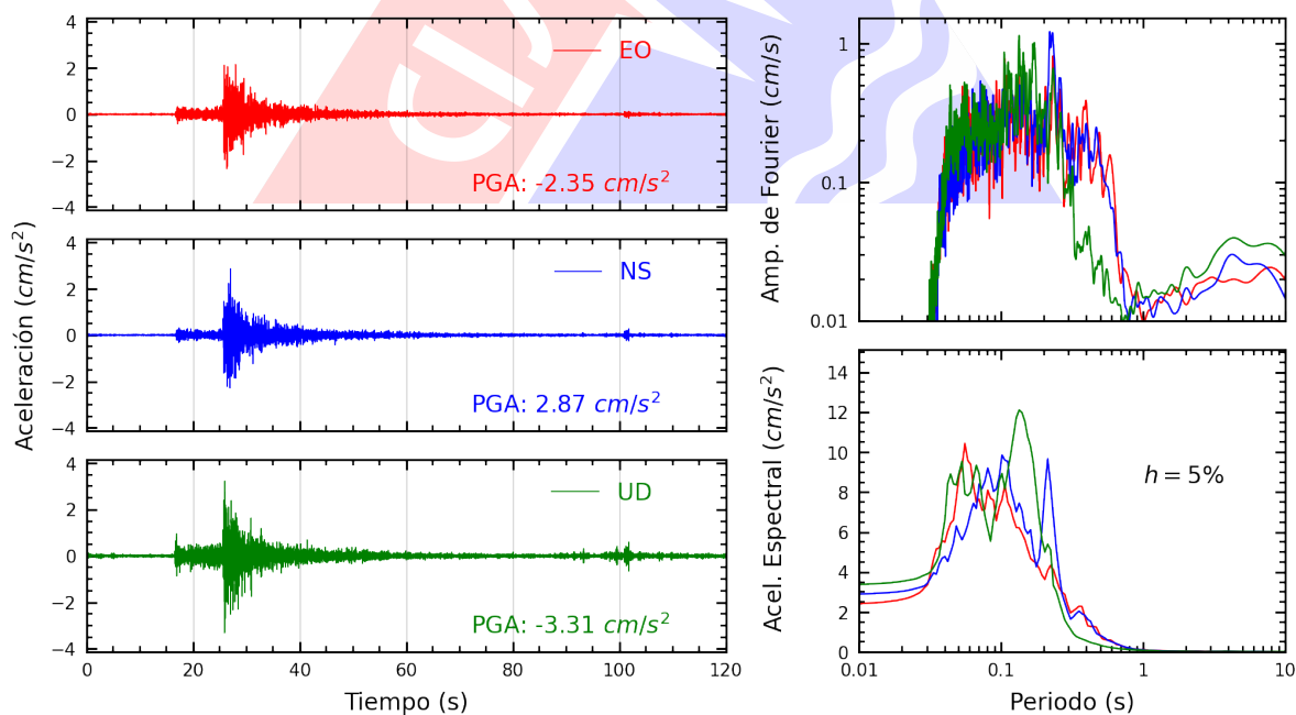
Figura A.24: Registros tiempo-historia, espectros de Fourier y de respuesta en las direcciones EO, NS y vertical de la estación MDPP. Sismo de Chilca, Cañete - Lima del 2024-12-23, 21:05:42 (Hora local)
