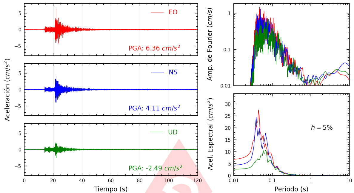
Figura A.11: Registros tiempo-historia, espectros de Fourier y de respuesta en las direcciones EO, NS y vertical de la estación CEPRE. Sismo de Chilca, Cañete - Lima del 2024-12-23, 21:05:42 (Hora local)
