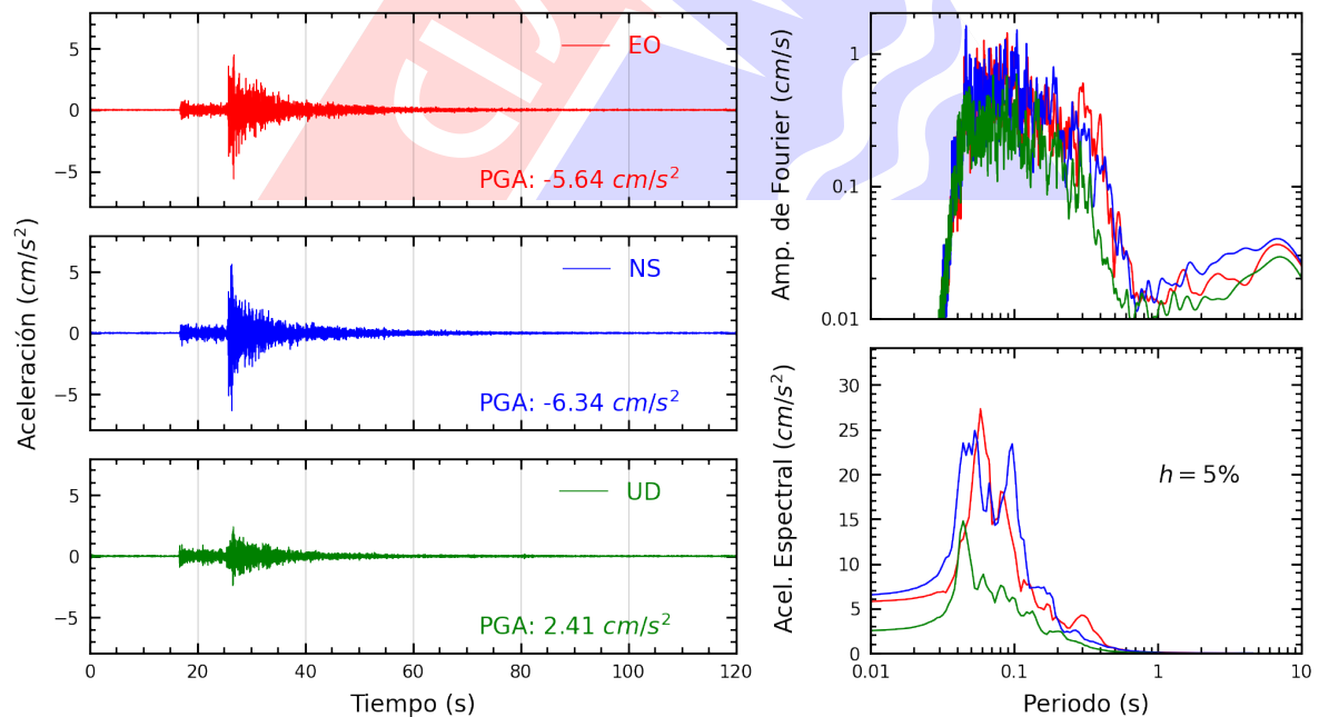
Figura A.12: Registros tiempo-historia, espectros de Fourier y de respuesta en las direcciones EO, NS y vertical de la estación DEFEN. Sismo de Chilca, Cañete - Lima del 2024-12-23, 21:05:42 (Hora local)
