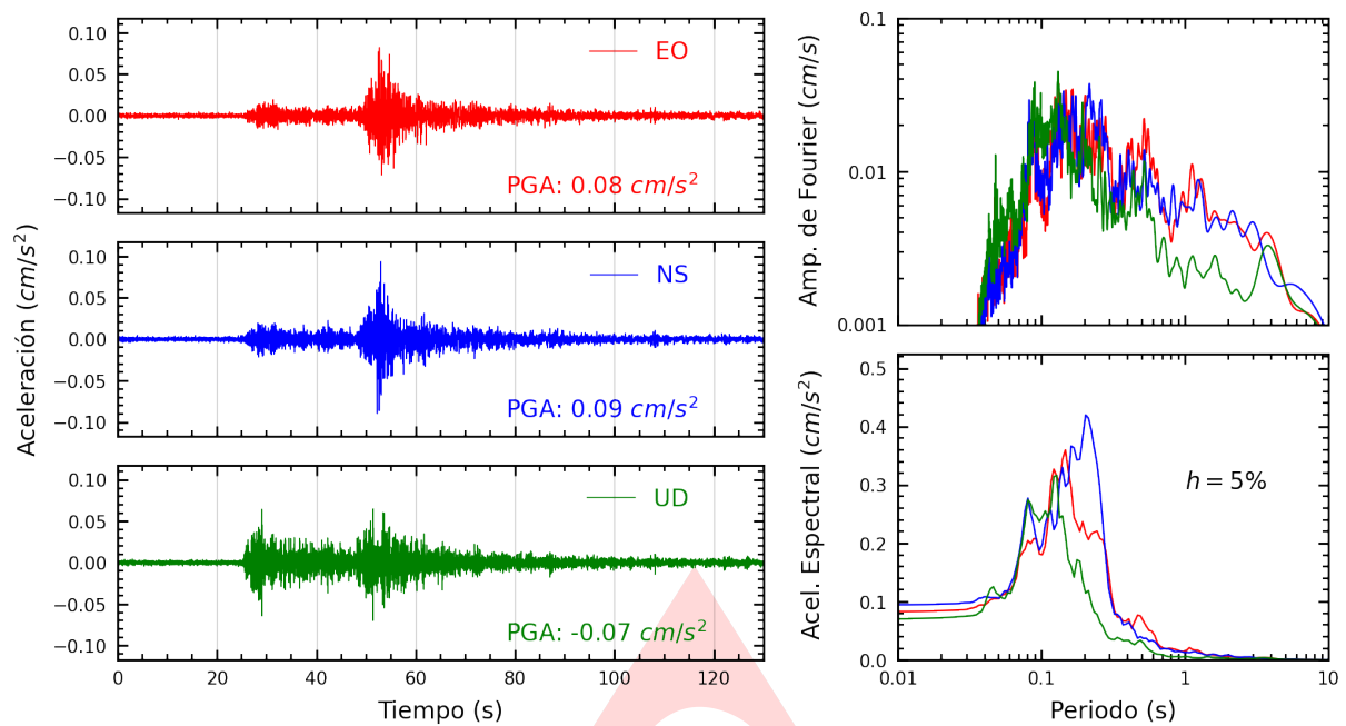
Figura A.1: Registros tiempo-historia, espectros de Fourier y de respuesta en las direcciones EO, NS y vertical de la estación UNIA. Sismo de Tingo Maria, Leoncio Prado - Huanuco del 2024-12-25, 09:47:23 (Hora local)
