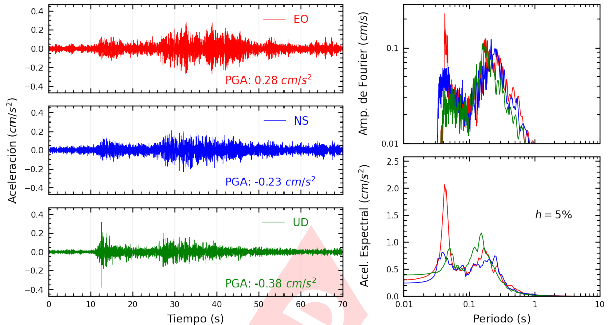
Figura A.3: Registros tiempo-historia, espectros de Fourier y de respuesta en las direcciones EO, NS y vertical de la estación UPTAC. Sismo de Ilo, Ilo - Moquegua del 2024-12-26, 12:12:18 (Hora local)
