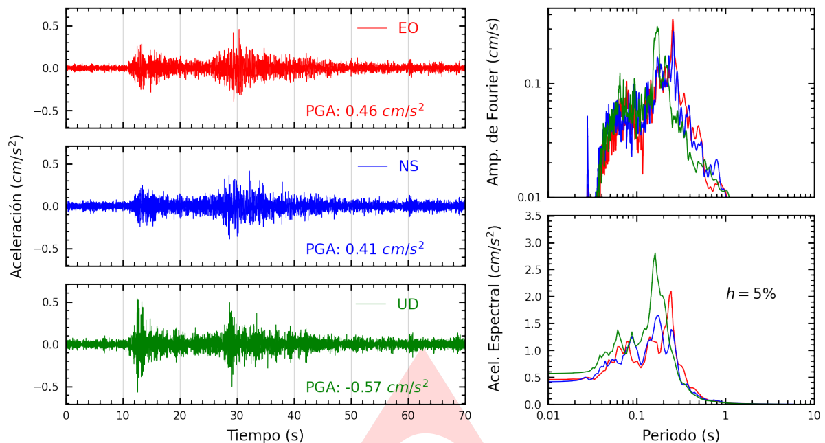
Figura A.1: Registros tiempo-historia, espectros de Fourier y de respuesta en las direcciones EO, NS y vertical de la estación UJBG4. Sismo de Ilo, Ilo - Moquegua del 2024-12-26, 12:12:18 (Hora local)
