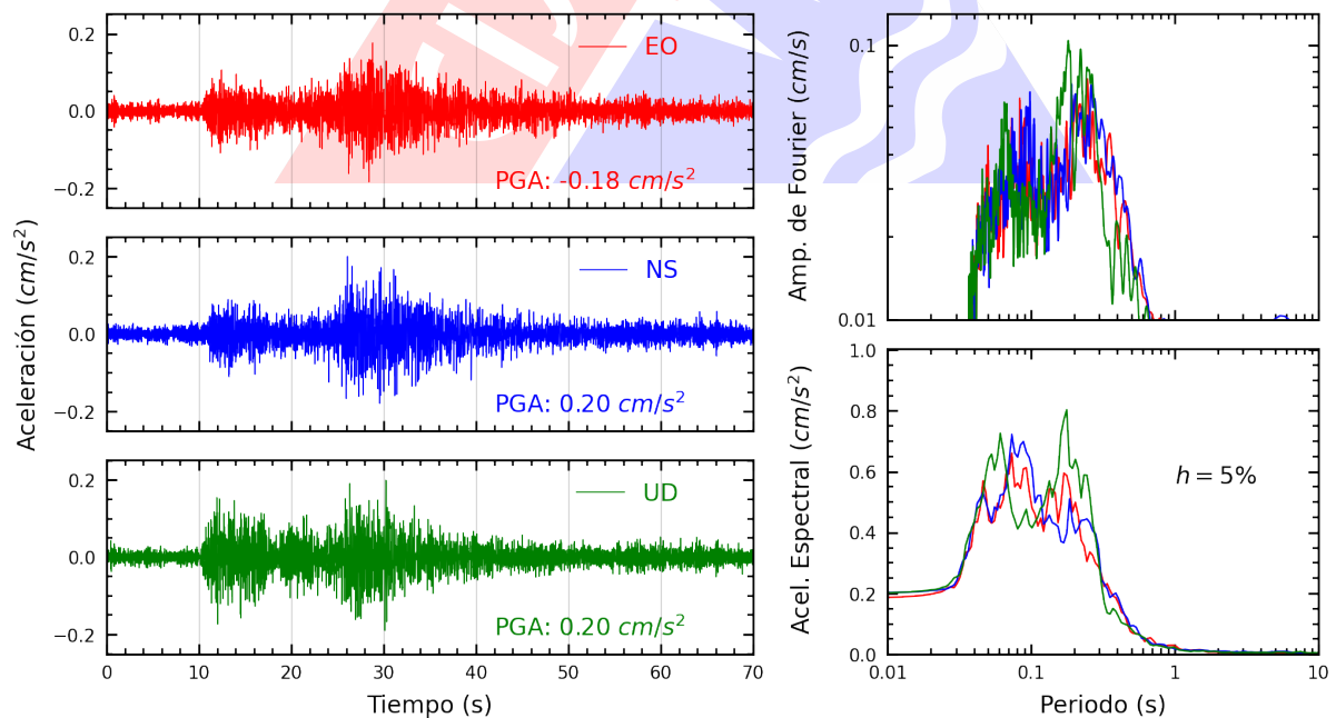
Figura A.4: Registros tiempo-historia, espectros de Fourier y de respuesta en las direcciones EO, NS y vertical de la estación CREY. Sismo de Ilo, Ilo - Moquegua del 2024-12-26, 12:12:18 (Hora local)
