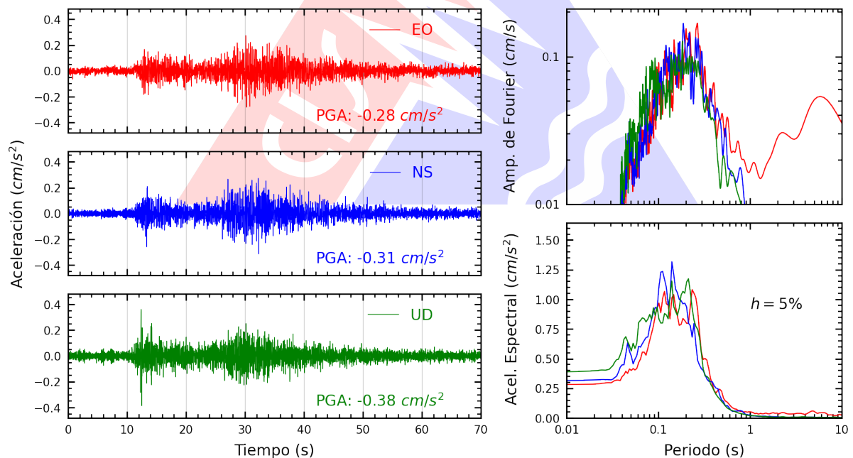
Figura A.2: Registros tiempo-historia, espectros de Fourier y de respuesta en las direcciones EO, NS y vertical de la estación UJBG3. Sismo de Ilo, Ilo - Moquegua del 2024-12-26, 12:12:18 (Hora local)
