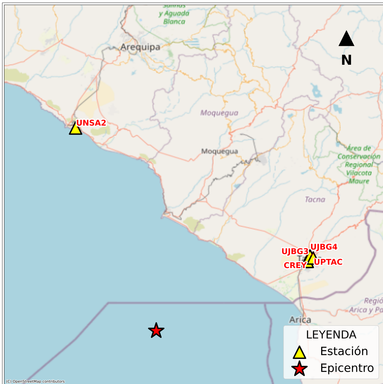
Figura 2: Mapa de ubicación de la(s) estación(es) acelerográfica(s) correspondiente(s) al Sismo de Ilo, Ilo - Moquegua del 26 de diciembre de 2024 a las 12:12:18 (hora local)
