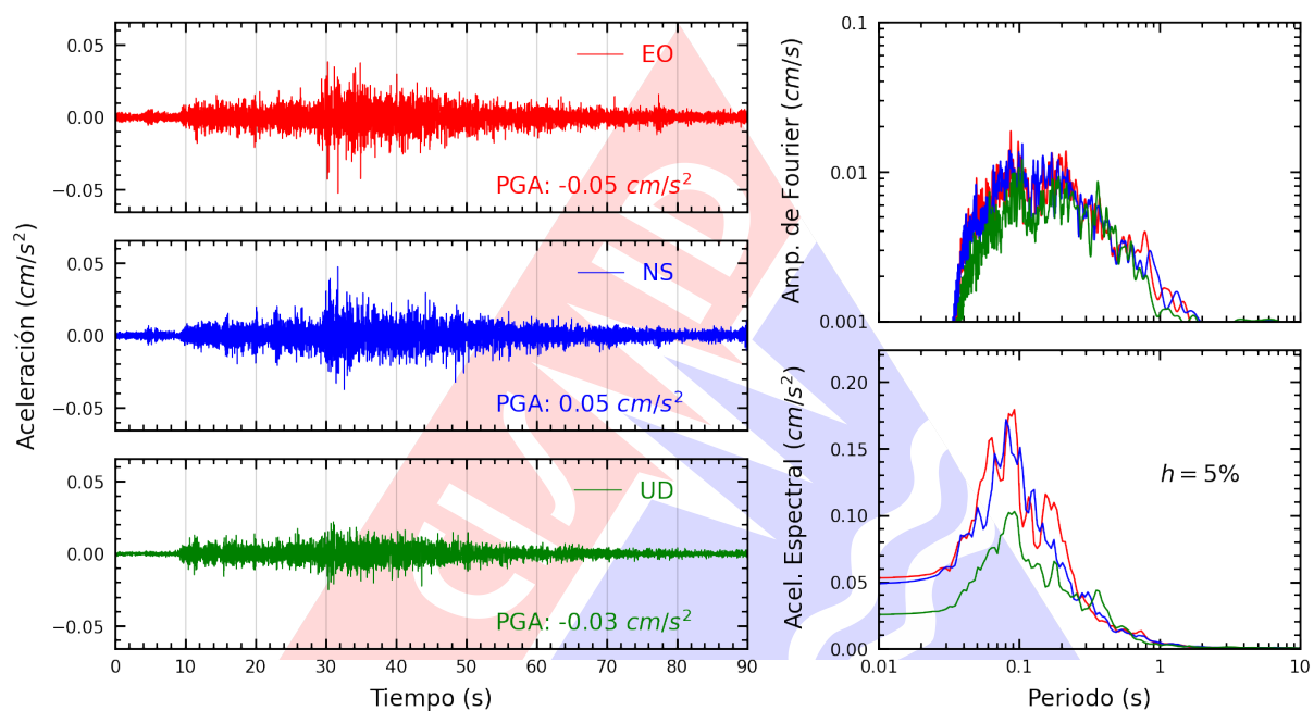
Figura A.5: Registros tiempo-historia, espectros de Fourier y de respuesta en las direcciones EO, NS y vertical de la estación UNSA2. Sismo de Ilo, Ilo - Moquegua del 2024-12-26, 12:12:18 (Hora local)
