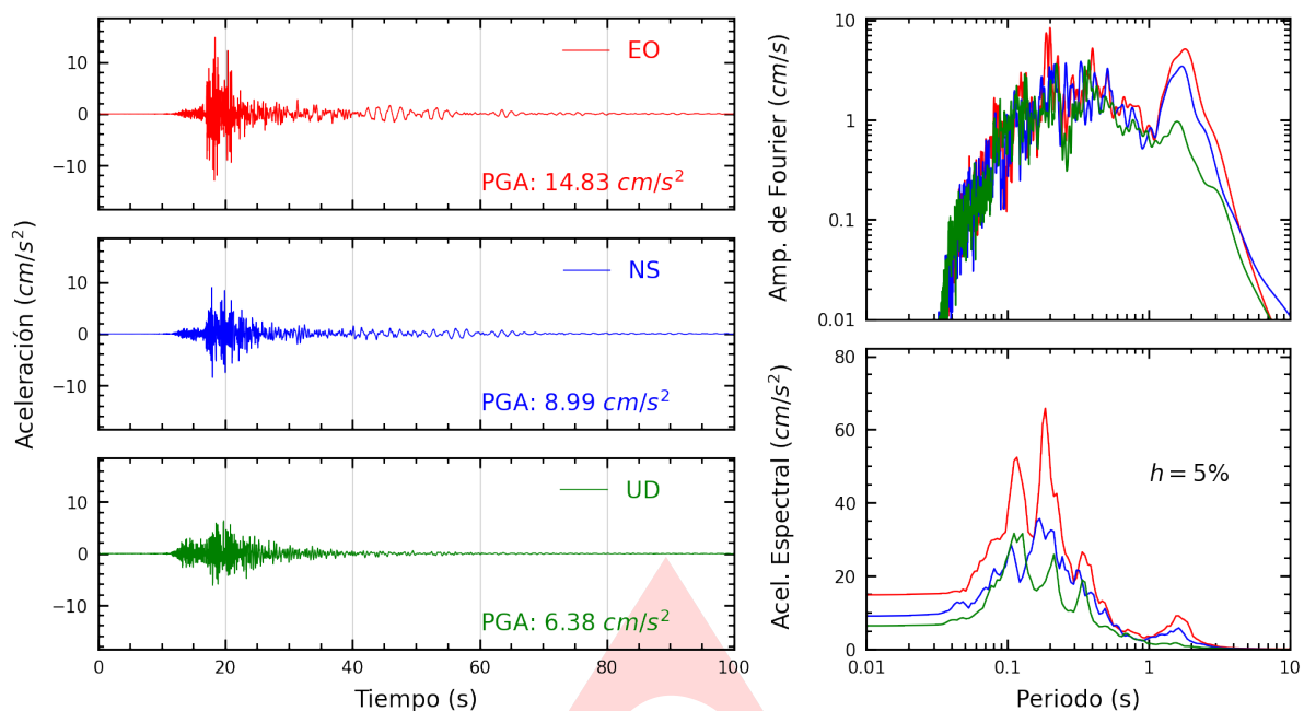
Figura A.1: Registros tiempo-historia, espectros de Fourier y de respuesta en las direcciones EO, NS y vertical de la estación SCCUS. Sismo de Lucre, Quispicanchi - Cusco del 2024-05-04, 23:38:15 (Hora local)
