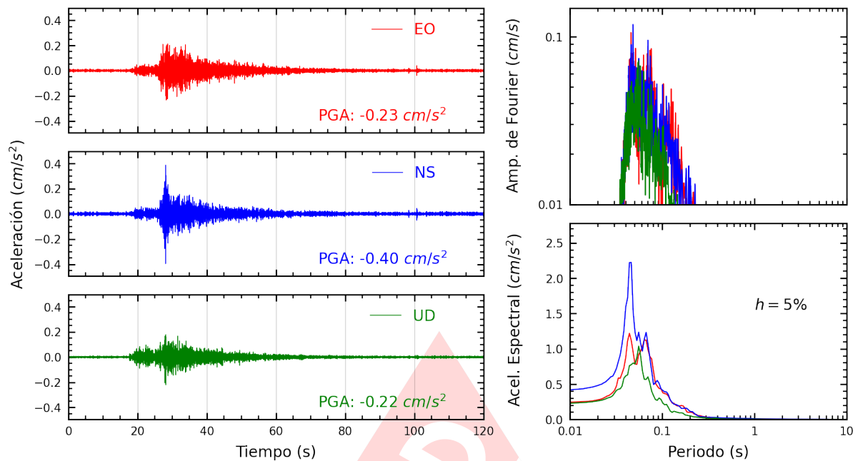
Figura A.21: Registros tiempo-historia, espectros de Fourier y de respuesta en las direcciones EO, NS y vertical de la estación ATARJ. Sismo de Chilca, Cañete - Lima del 2024-10-26, 23:10:06 (Hora local)
