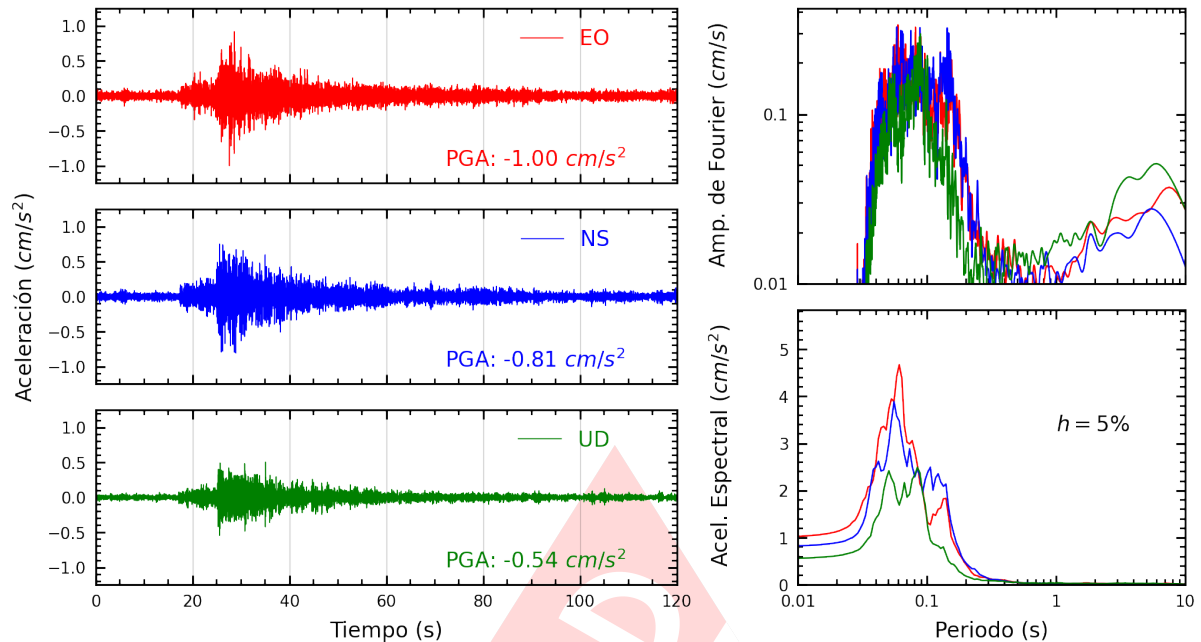
Figura A.5: Registros tiempo-historia, espectros de Fourier y de respuesta en las direcciones EO, NS y vertical de la estación USILM. Sismo de Chilca, Cañete - Lima del 2024-10-26, 23:10:06 (Hora local)
