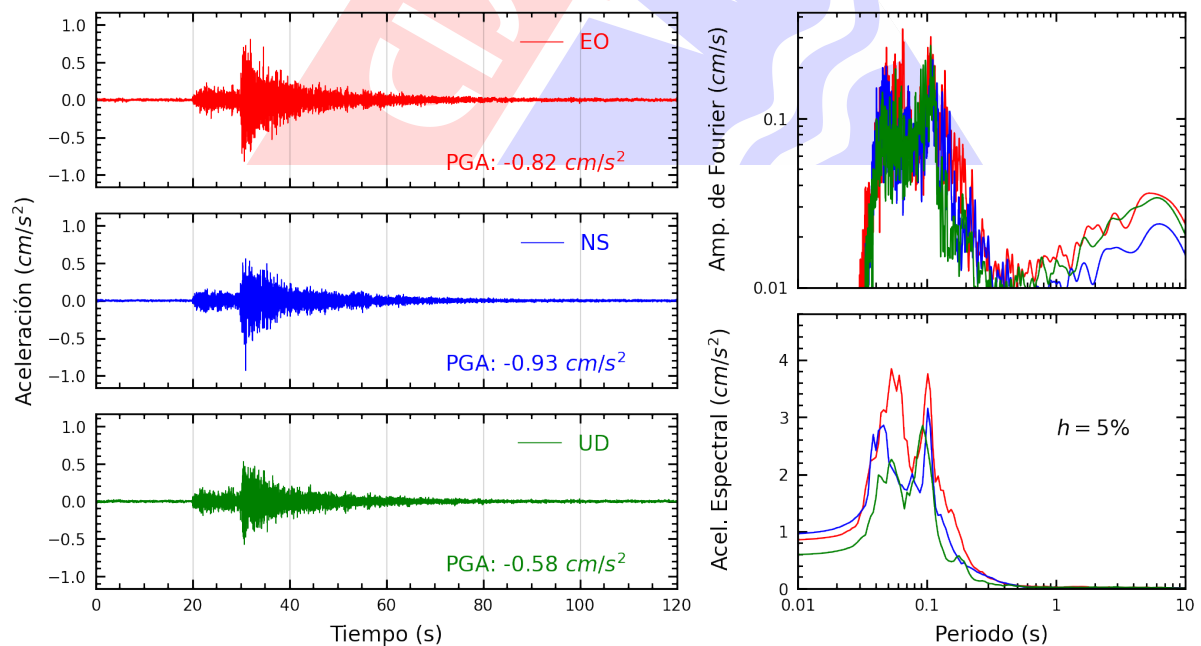
Figura A.6: Registros tiempo-historia, espectros de Fourier y de respuesta en las direcciones EO, NS y vertical de la estación AMORE. Sismo de Chilca, Cañete - Lima del 2024-10-26, 23:10:06 (Hora local)
