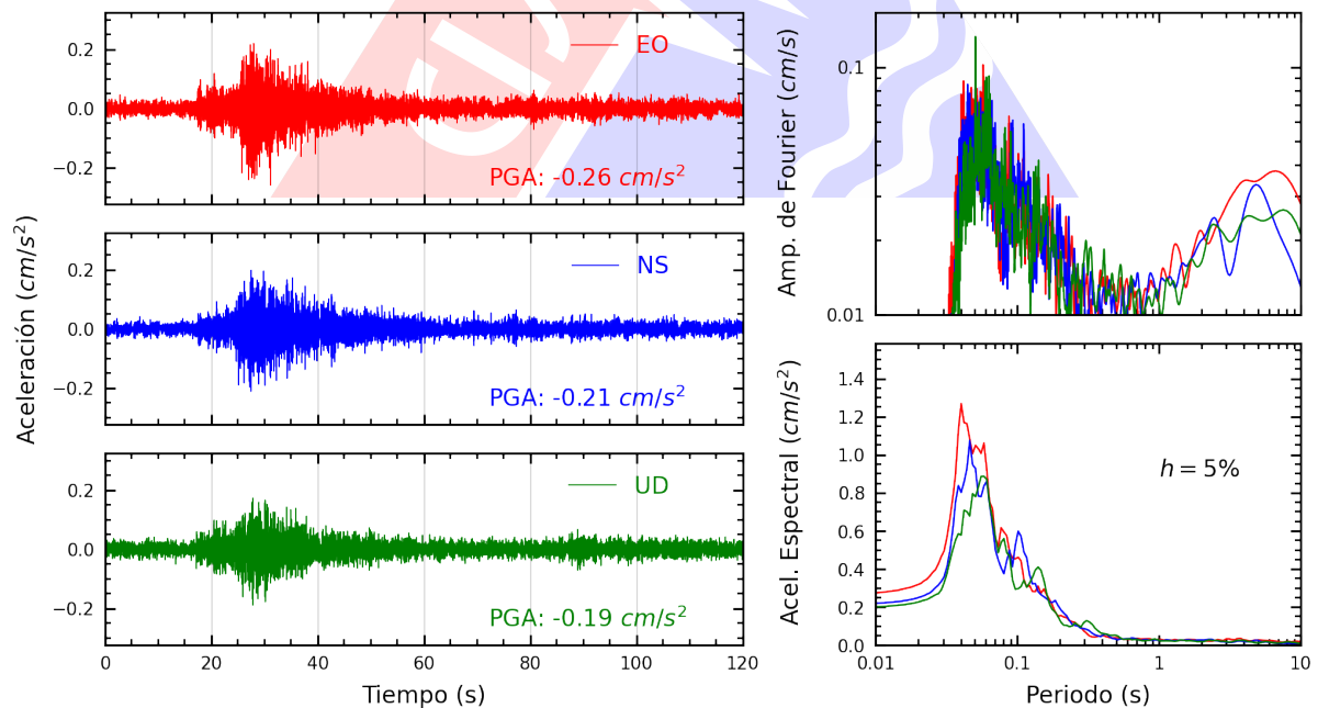
Figura A.26: Registros tiempo-historia, espectros de Fourier y de respuesta en las direcciones EO, NS y vertical de la estación IMCA. Sismo de Chilca, Cañete - Lima del 2024-10-26, 23:10:06 (Hora local)
