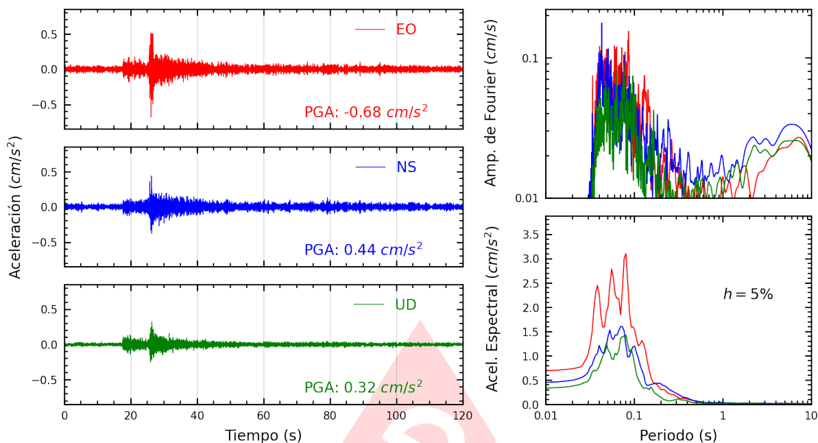
Figura A.11: Registros tiempo-historia, espectros de Fourier y de respuesta en las direcciones EO, NS y vertical de la estación CEPRE. Sismo de Chilca, Cañete - Lima del 2024-10-26, 23:10:06 (Hora local)
