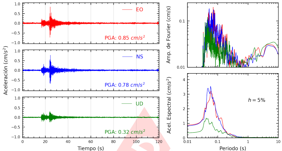
Figura A.9: Registros tiempo-historia, espectros de Fourier y de respuesta en las direcciones EO, NS y vertical de la estación UPCVI. Sismo de Chilca, Cañete - Lima del 2024-10-26, 23:10:06 (Hora local)
