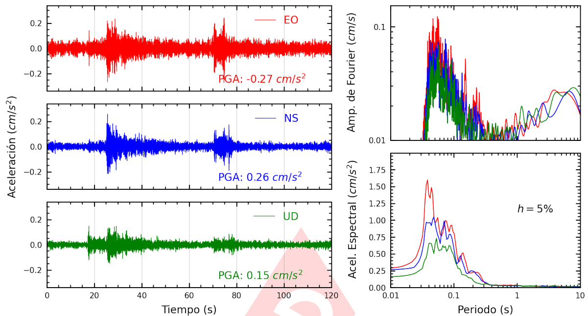
Figura A.25: Registros tiempo-historia, espectros de Fourier y de respuesta en las direcciones EO, NS y vertical de la estación INICT. Sismo de Chilca, Cañete - Lima del 2024-10-26, 23:10:06 (Hora local)
