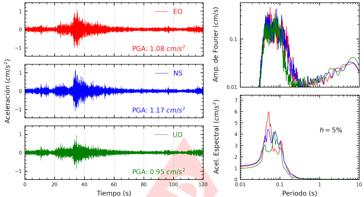
Figura A.3: Registros tiempo-historia, espectros de Fourier y de respuesta en las direcciones EO, NS y vertical de la estación SROSA. Sismo de Chilca, Cañete - Lima del 2024-10-26, 23:10:06 (Hora local)
