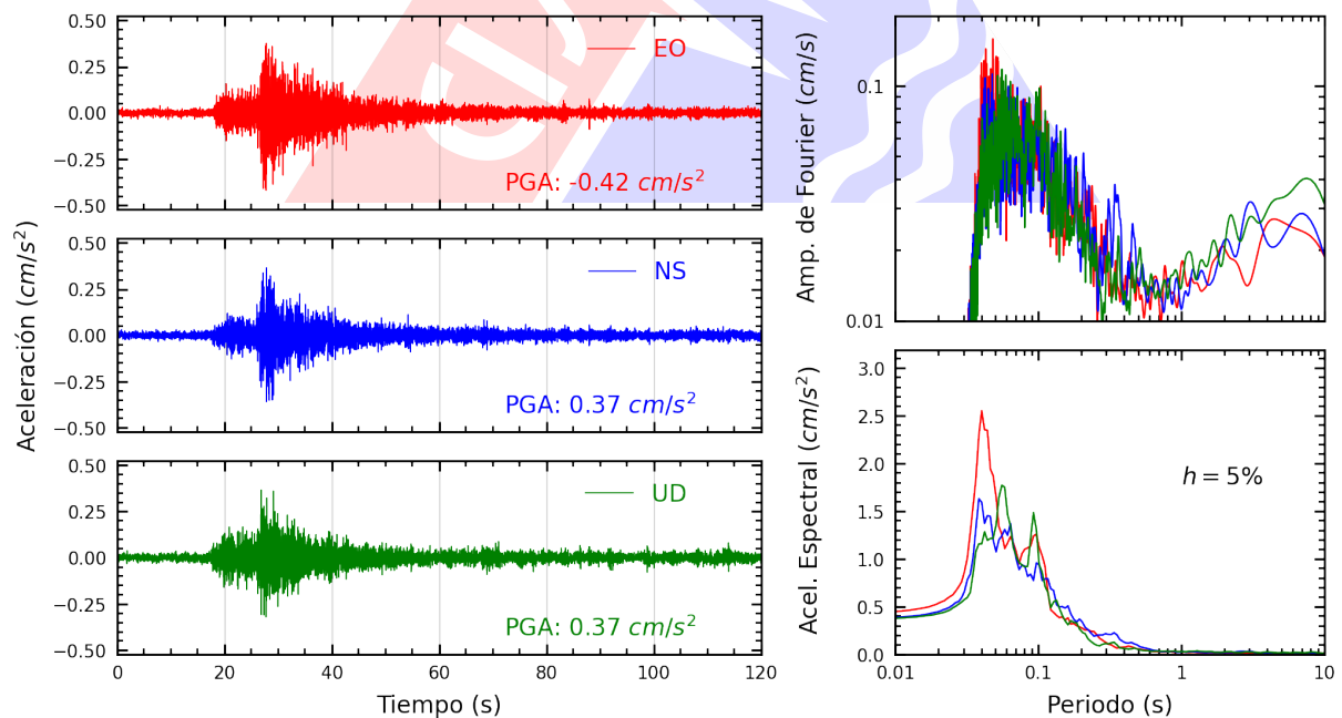
Figura A.18: Registros tiempo-historia, espectros de Fourier y de respuesta en las direcciones EO, NS y vertical de la estación UCVAT. Sismo de Chilca, Cañete - Lima del 2024-10-26, 23:10:06 (Hora local)
