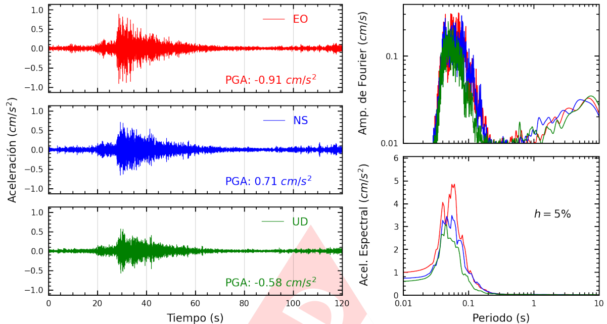
Figura A.7: Registros tiempo-historia, espectros de Fourier y de respuesta en las direcciones EO, NS y vertical de la estación JOSEO. Sismo de Chilca, Cañete - Lima del 2024-10-26, 23:10:06 (Hora local)
