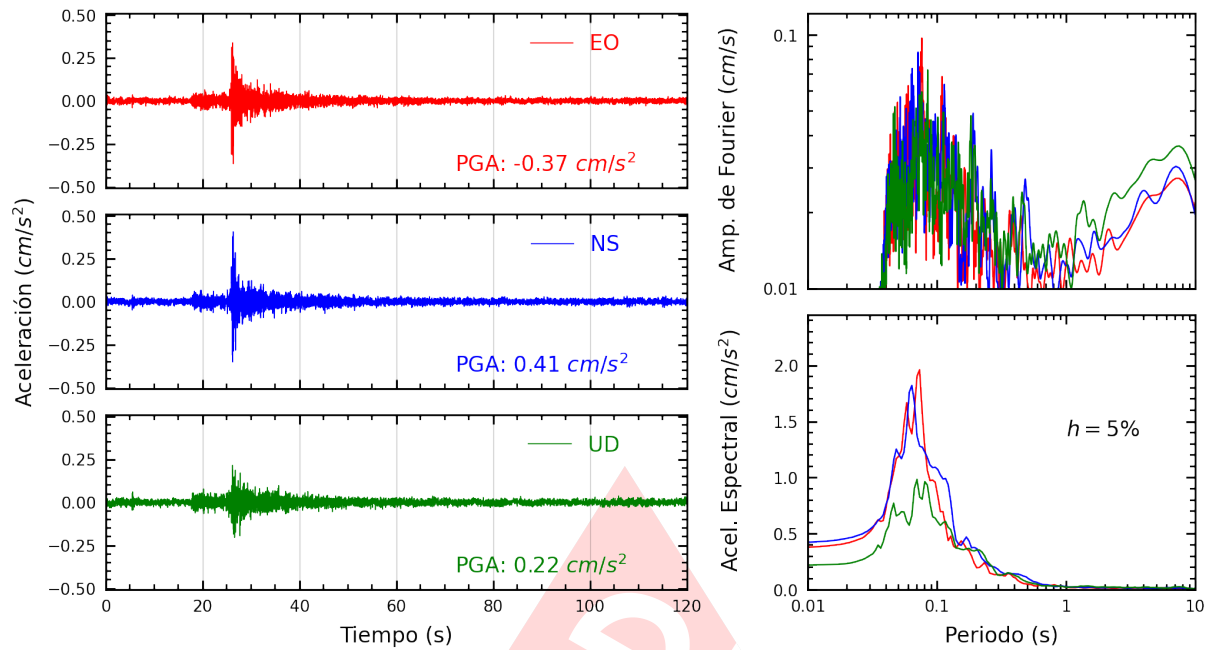
Figura A.19: Registros tiempo-historia, espectros de Fourier y de respuesta en las direcciones EO, NS y vertical de la estación UNFV. Sismo de Chilca, Cañete - Lima del 2024-10-26, 23:10:06 (Hora local)
