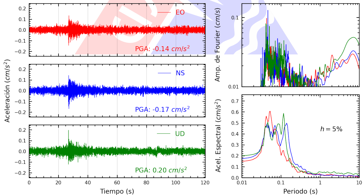
Figura A.28: Registros tiempo-historia, espectros de Fourier y de respuesta en las direcciones EO, NS y vertical de la estación BONDY. Sismo de Chilca, Cañete - Lima del 2024-10-26, 23:10:06 (Hora local)
