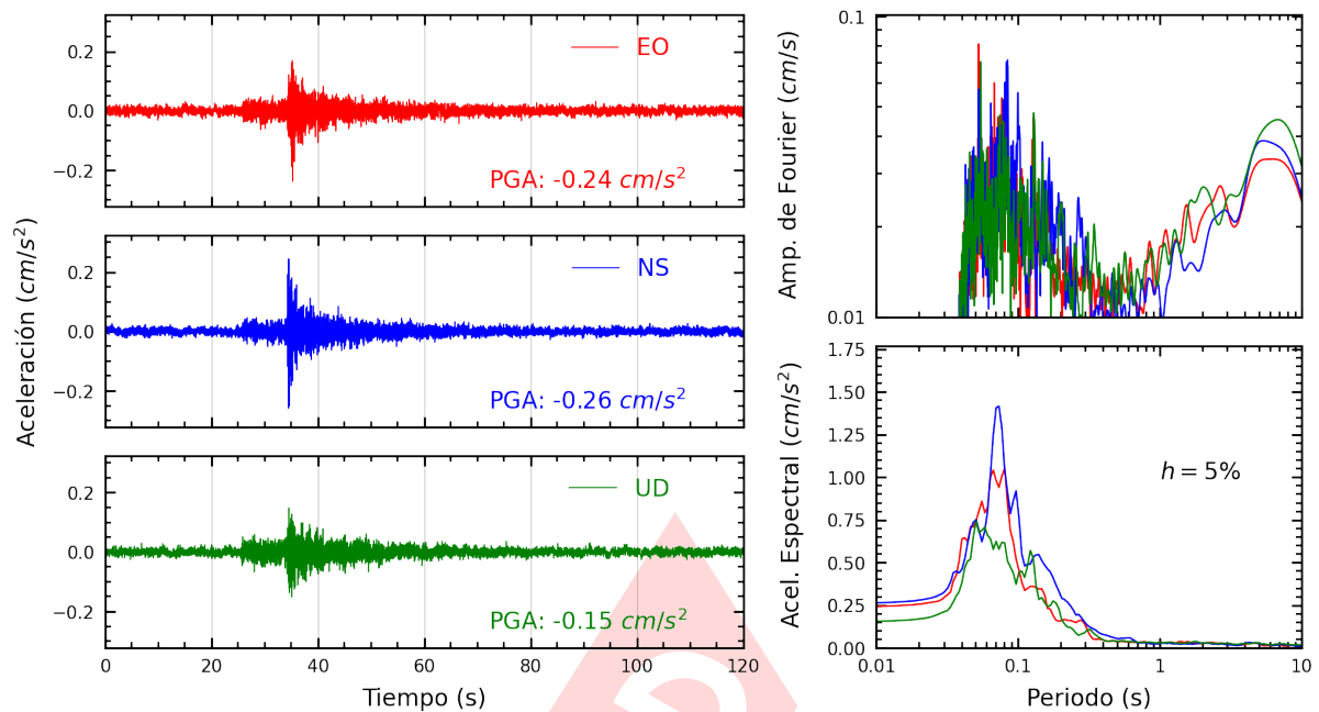
Figura A.27: Registros tiempo-historia, espectros de Fourier y de respuesta en las direcciones EO, NS y vertical de la estación UNMSM. Sismo de Chilca, Cañete - Lima del 2024-10-26, 23:10:06 (Hora local)
