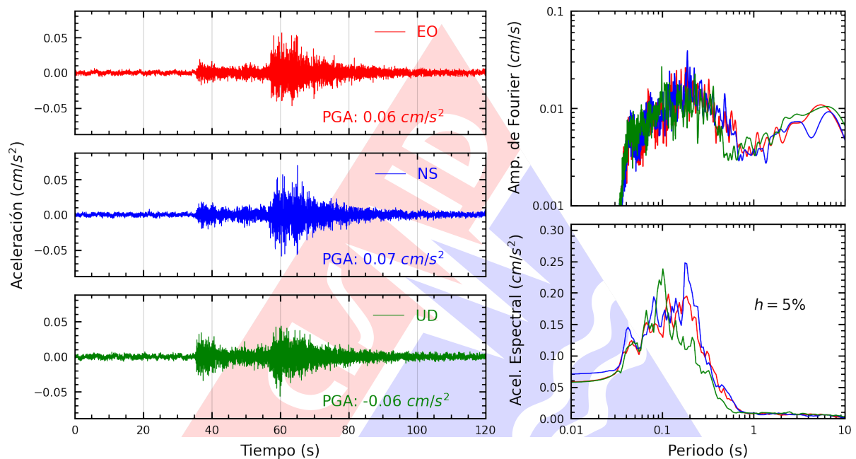
Figura A.29: Registros tiempo-historia, espectros de Fourier y de respuesta en las direcciones EO, NS y vertical de la estación CARAL. Sismo de Chilca, Cañete - Lima del 2024-10-26, 23:10:06 (Hora local)
