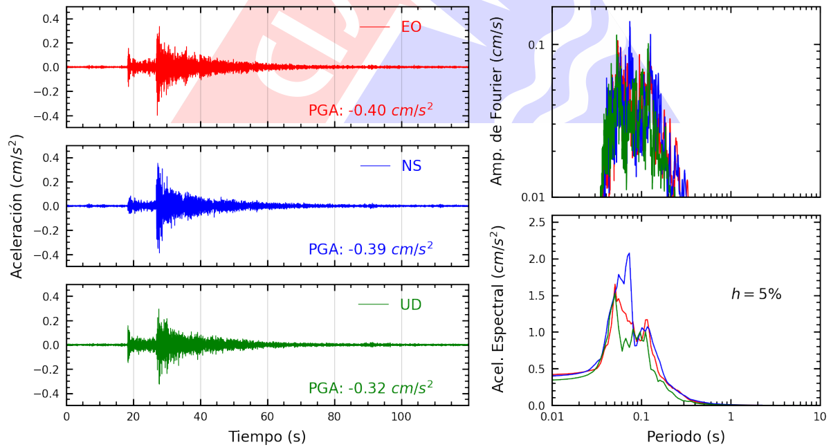
Figura A.20: Registros tiempo-historia, espectros de Fourier y de respuesta en las direcciones EO, NS y vertical de la estación JALV2. Sismo de Chilca, Cañete - Lima del 2024-10-26, 23:10:06 (Hora local)
