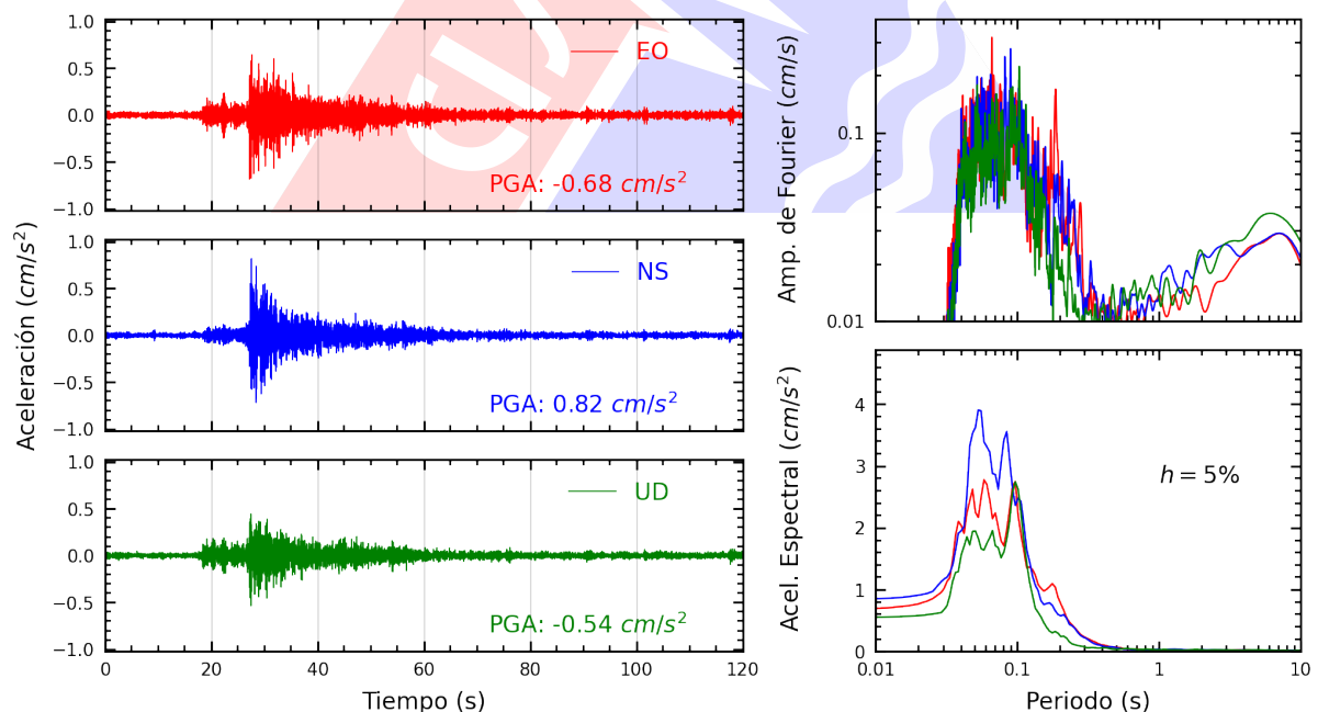
Figura A.10: Registros tiempo-historia, espectros de Fourier y de respuesta en las direcciones EO, NS y vertical de la estación INDEP. Sismo de Chilca, Cañete - Lima del 2024-10-26, 23:10:06 (Hora local)
