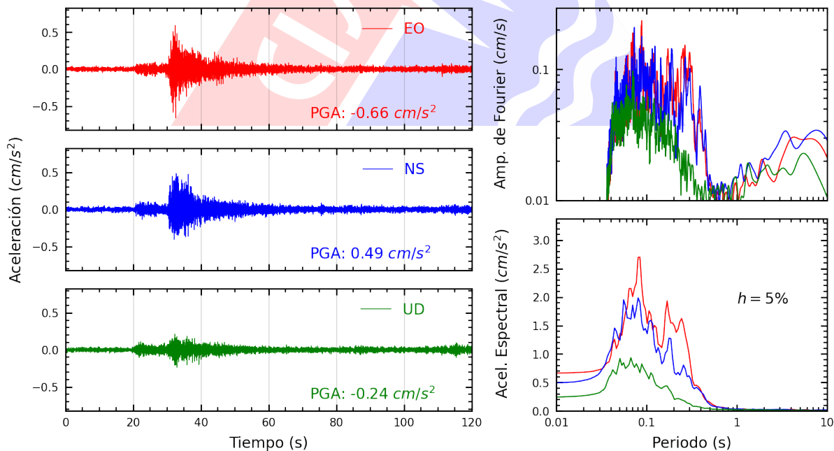
Figura A.12: Registros tiempo-historia, espectros de Fourier y de respuesta en las direcciones EO, NS y vertical de la estación DEFEN. Sismo de Chilca, Cañete - Lima del 2024-10-26, 23:10:06 (Hora local)
