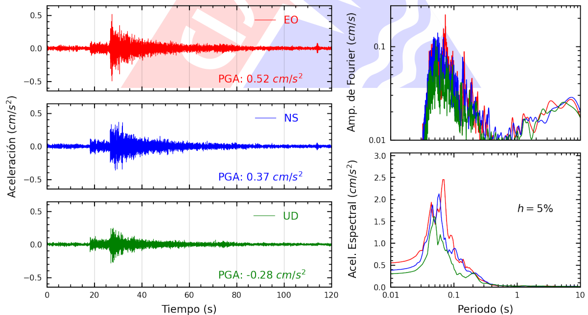
Figura A.16: Registros tiempo-historia, espectros de Fourier y de respuesta en las direcciones EO, NS y vertical de la estación FICPE. Sismo de Chilca, Cañete - Lima del 2024-10-26, 23:10:06 (Hora local)
