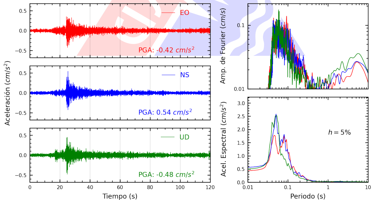
Figura A.14: Registros tiempo-historia, espectros de Fourier y de respuesta en las direcciones EO, NS y vertical de la estación URPPE. Sismo de Chilca, Cañete - Lima del 2024-10-26, 23:10:06 (Hora local)
