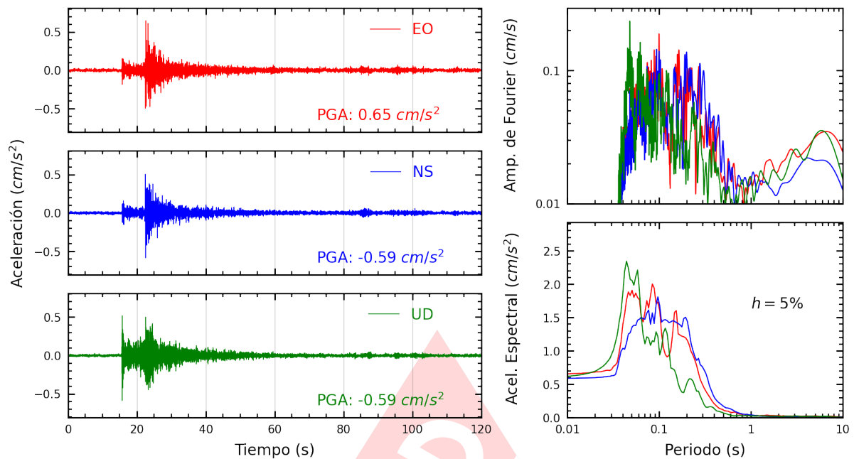
Figura A.13: Registros tiempo-historia, espectros de Fourier y de respuesta en las direcciones EO, NS y vertical de la estación USILP. Sismo de Chilca, Cañete - Lima del 2024-10-26, 23:10:06 (Hora local)
