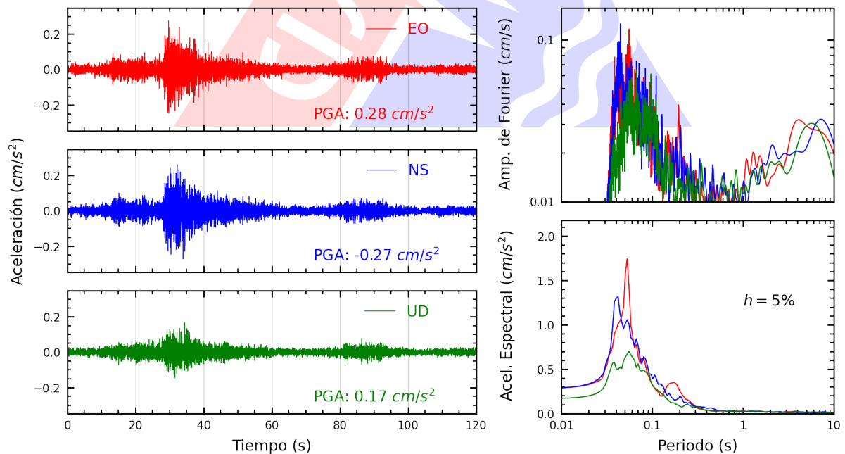
Figura A.24: Registros tiempo-historia, espectros de Fourier y de respuesta en las direcciones EO, NS y vertical de la estación COMAS. Sismo de Chilca, Cañete - Lima del 2024-10-26, 23:10:06 (Hora local)
