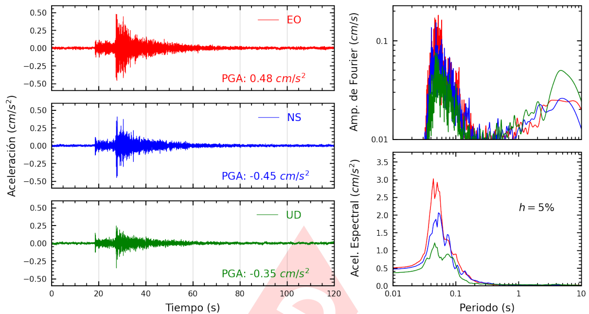
Figura A.17: Registros tiempo-historia, espectros de Fourier y de respuesta en las direcciones EO, NS y vertical de la estación UCSS. Sismo de Chilca, Cañete - Lima del 2024-10-26, 23:10:06 (Hora local)
