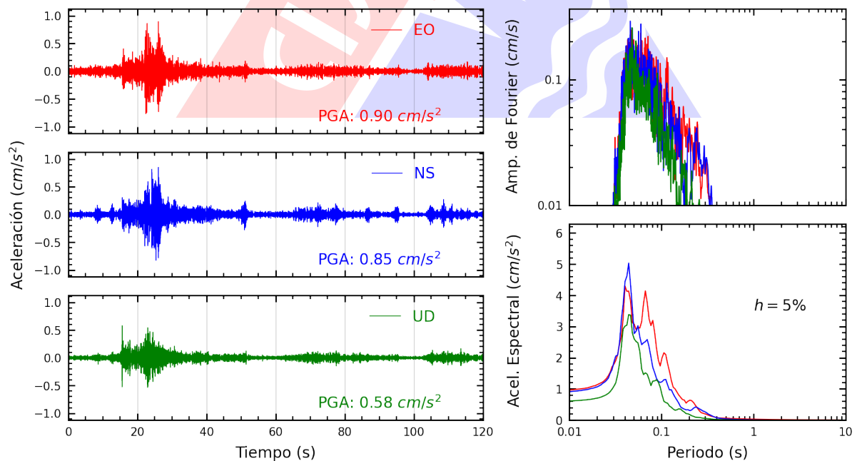
Figura A.8: Registros tiempo-historia, espectros de Fourier y de respuesta en las direcciones EO, NS y vertical de la estación PACHA. Sismo de Chilca, Cañete - Lima del 2024-10-26, 23:10:06 (Hora local)
