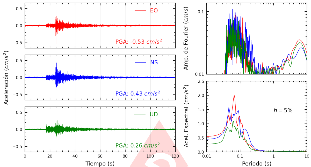
Figura A.15: Registros tiempo-historia, espectros de Fourier y de respuesta en las direcciones EO, NS y vertical de la estación SERVI. Sismo de Chilca, Cañete - Lima del 2024-10-26, 23:10:06 (Hora local)
