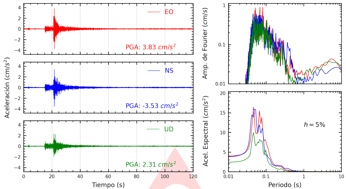
Figura A.1: Registros tiempo-historia, espectros de Fourier y de respuesta en las direcciones EO, NS y vertical de la estación PHERM. Sismo de Chilca, Cañete - Lima del 2024-10-26, 23:10:06 (Hora local)
