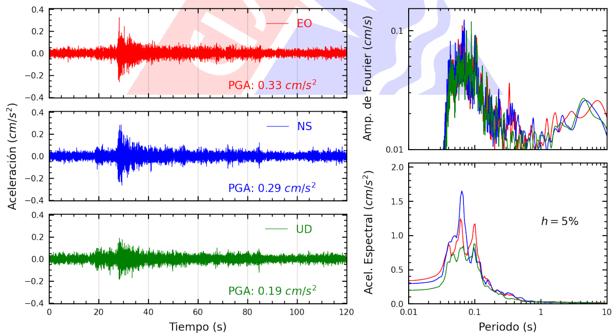
Figura A.22: Registros tiempo-historia, espectros de Fourier y de respuesta en las direcciones EO, NS y vertical de la estación MADRE. Sismo de Chilca, Cañete - Lima del 2024-10-26, 23:10:06 (Hora local)
