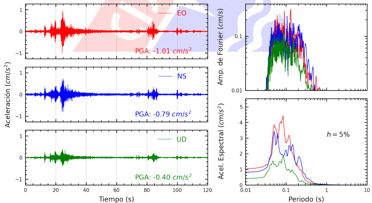
Figura A.4: Registros tiempo-historia, espectros de Fourier y de respuesta en las direcciones EO, NS y vertical de la estación BRISA. Sismo de Chilca, Cañete - Lima del 2024-10-26, 23:10:06 (Hora local)
