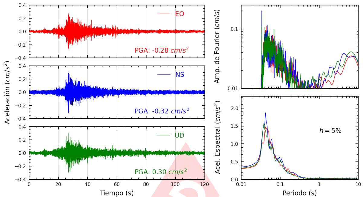
Figura A.23: Registros tiempo-historia, espectros de Fourier y de respuesta en las direcciones EO, NS y vertical de la estación USMP. Sismo de Chilca, Cañete - Lima del 2024-10-26, 23:10:06 (Hora local)
