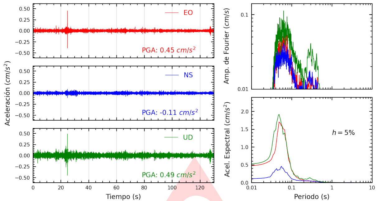
Figura A.1: Registros tiempo-historia, espectros de Fourier y de respuesta en las direcciones EO, NS y vertical de la estación SCCUS. Sismo de Atico, Caraveli - Arequipa del 2024-11-15, 16:43:23 (Hora local)
