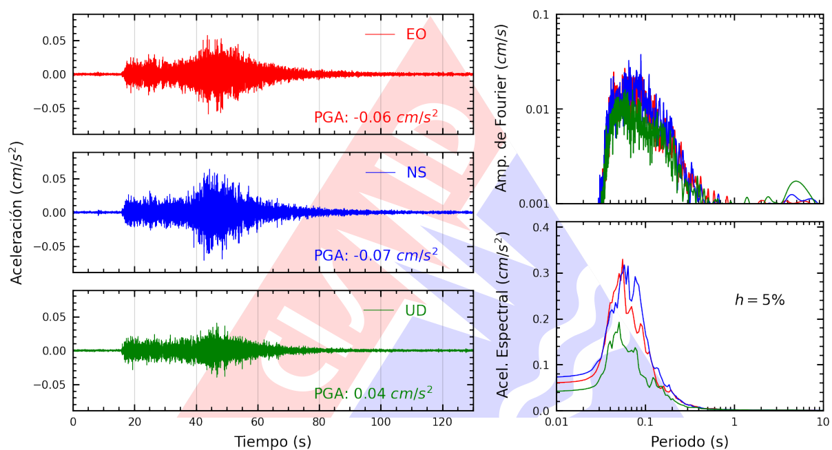
Figura A.3: Registros tiempo-historia, espectros de Fourier y de respuesta en las direcciones EO, NS y vertical de la estación UNSA2. Sismo de Atico, Caraveli - Arequipa del 2024-11-15, 16:43:23 (Hora local)
