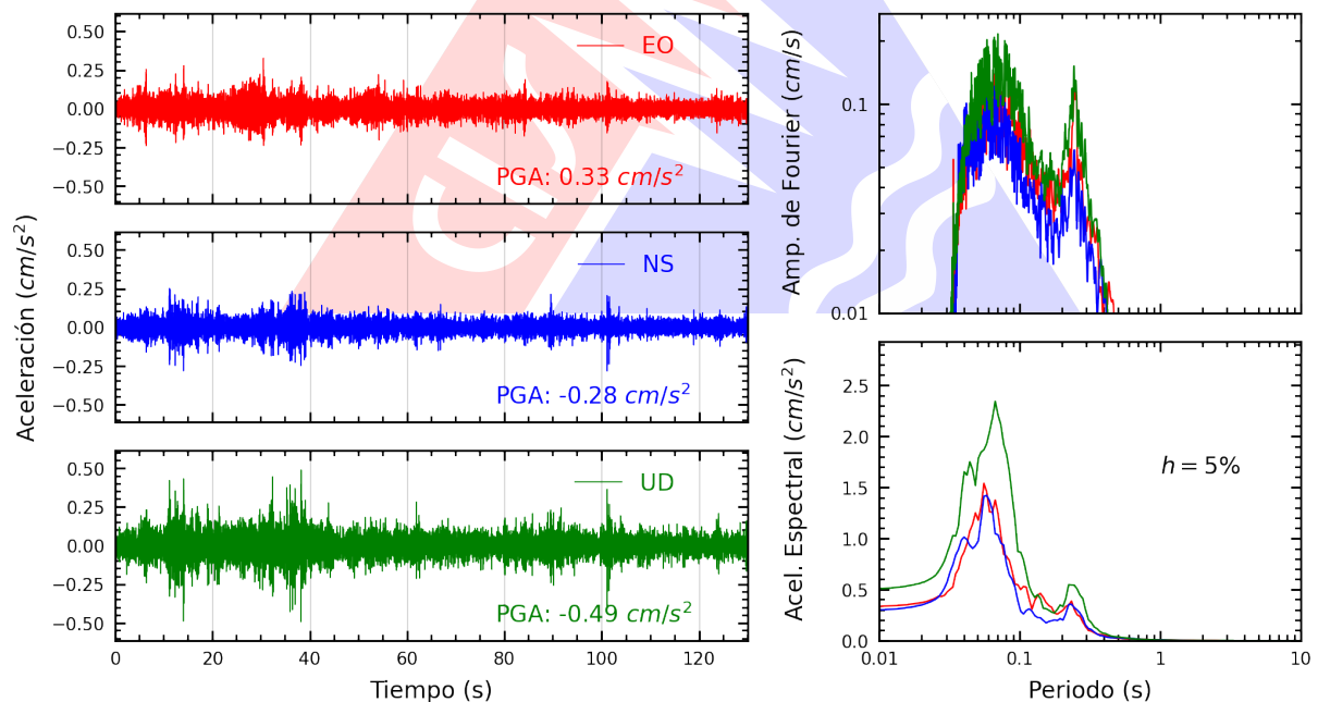
Figura A.2: Registros tiempo-historia, espectros de Fourier y de respuesta en las direcciones EO, NS y vertical de la estación SCICA. Sismo de Atico, Caraveli - Arequipa del 2024-11-15, 16:43:23 (Hora local)
