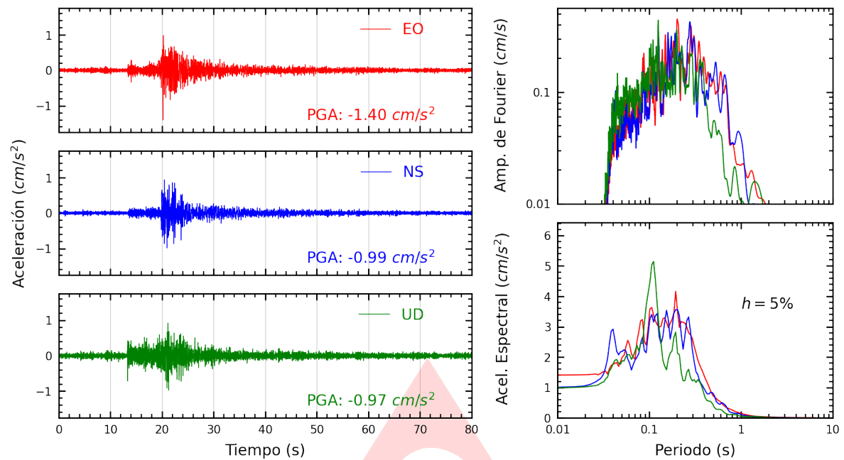
Figura A.1: Registros tiempo-historia, espectros de Fourier y de respuesta en las direcciones EO, NS y vertical de la estación SCICA. Sismo de Ica, Ica - Ica del 2024-12-05, 20:29:23 (Hora local)
