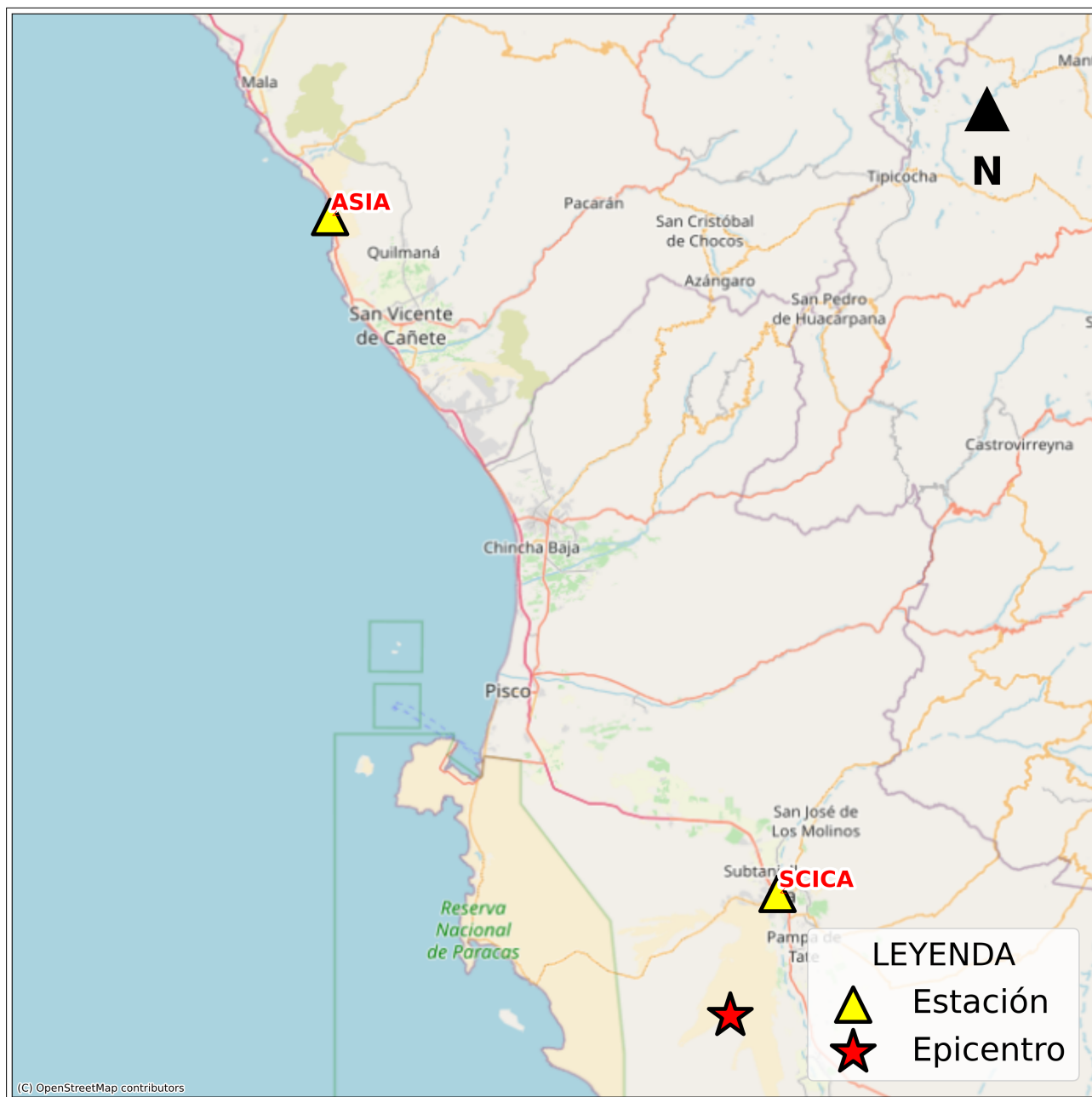
Figura 2: Mapa de ubicación de la(s) estación(es) acelerográfica(s) correspondiente(s) al Sismo de Ica, Ica - Ica del 05 de diciembre de 2024 a las 20:29:23 (hora local)
