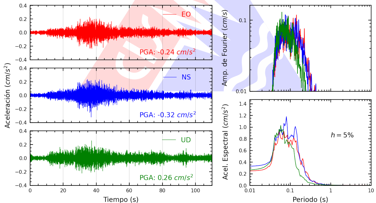
Figura A.2: Registros tiempo-historia, espectros de Fourier y de respuesta en las direcciones EO, NS y vertical de la estación ASIA. Sismo de Ica, Ica - Ica del 2024-12-05, 20:29:23 (Hora local)
