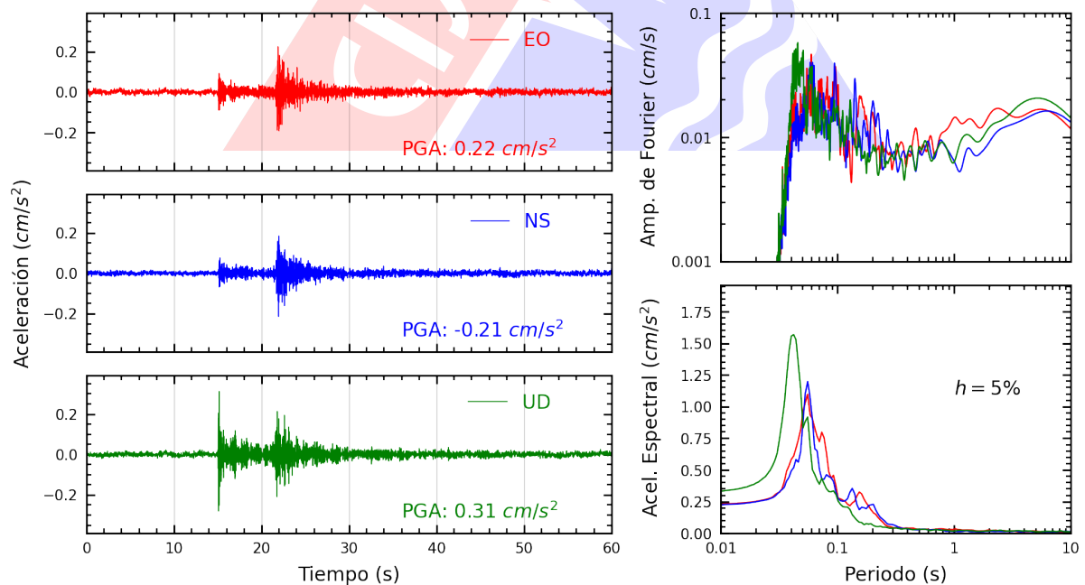
Figura A.6: Registros tiempo-historia, espectros de Fourier y de respuesta en las direcciones EO, NS y vertical de la estación USILP. Sismo de Chilca, Cañete - Lima del 2025-01-10, 01:18:15 (Hora local)
