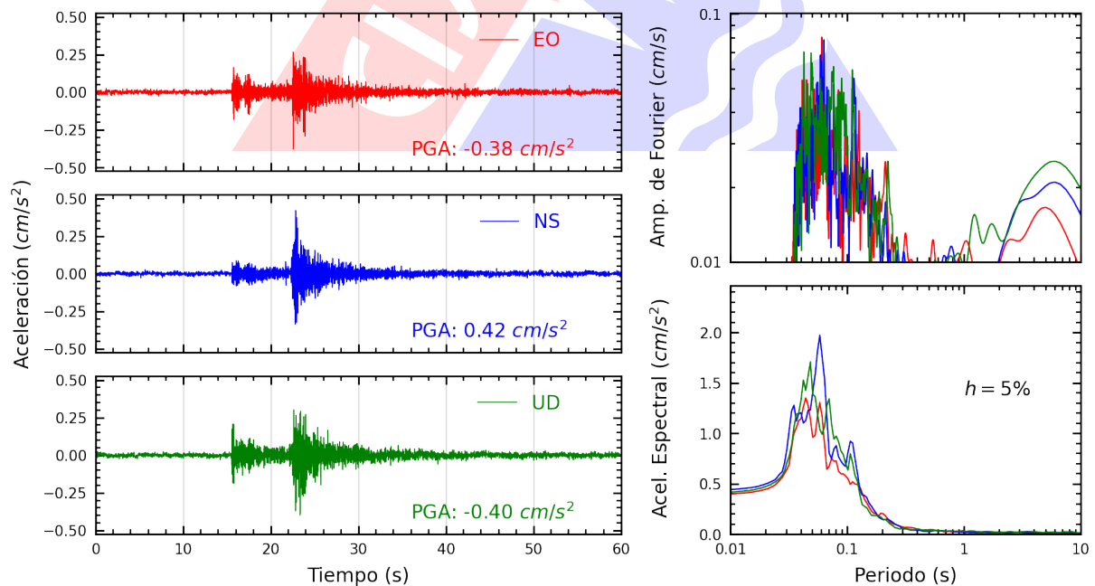
Figura A.4: Registros tiempo-historia, espectros de Fourier y de respuesta en las direcciones EO, NS y vertical de la estación SOVES. Sismo de Chilca, Cañete - Lima del 2025-01-10, 01:18:15 (Hora local)
