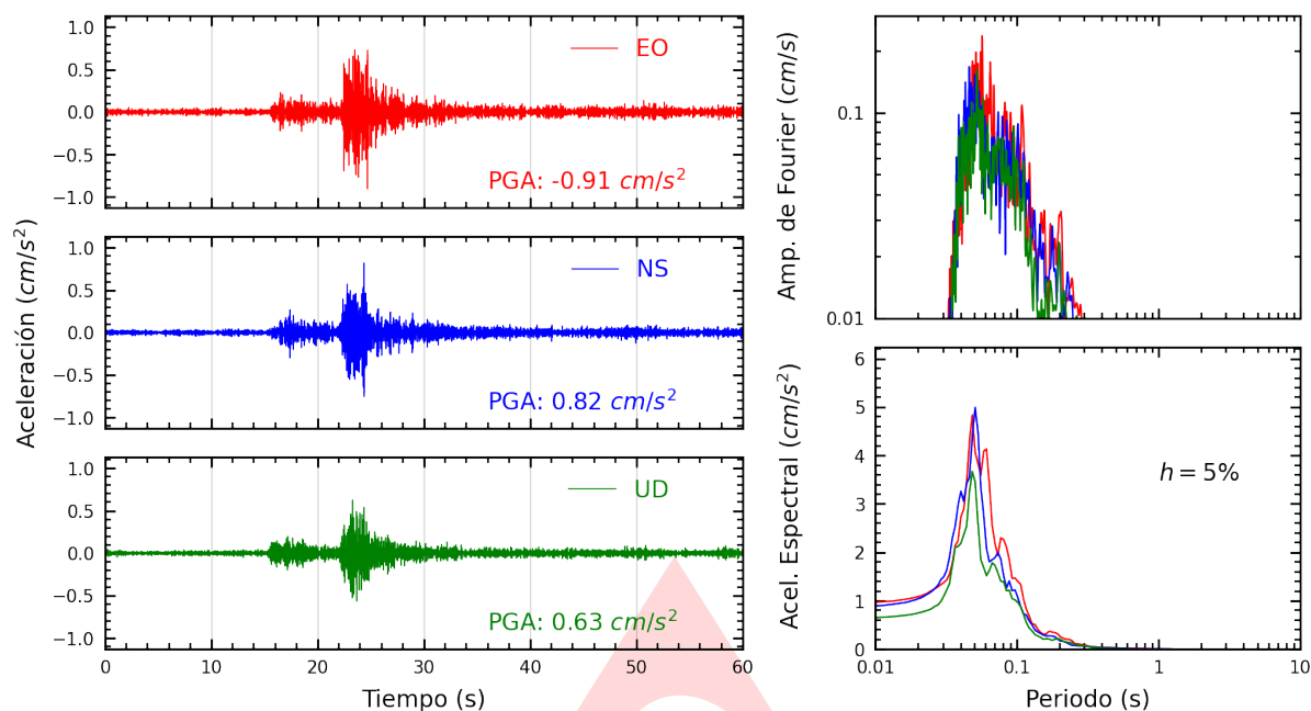
Figura A.1: Registros tiempo-historia, espectros de Fourier y de respuesta en las direcciones EO, NS y vertical de la estación UNTEL. Sismo de Chilca, Cañete - Lima del 2025-01-10, 01:18:15 (Hora local)
