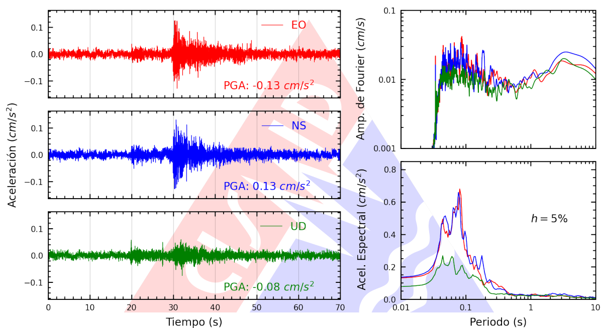
Figura A.15: Registros tiempo-historia, espectros de Fourier y de respuesta en las direcciones EO, NS y vertical de la estación DEFEN. Sismo de Chilca, Cañete - Lima del 2025-01-10, 01:18:15 (Hora local)
