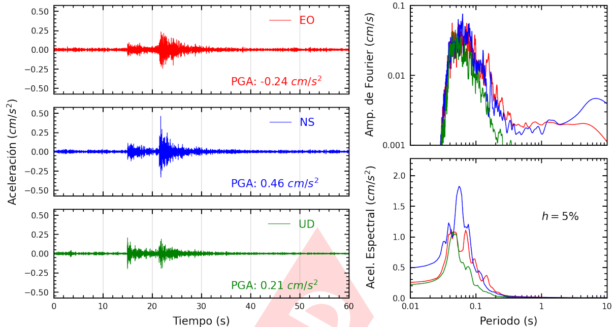
Figura A.3: Registros tiempo-historia, espectros de Fourier y de respuesta en las direcciones EO, NS y vertical de la estación PACHA. Sismo de Chilca, Cañete - Lima del 2025-01-10, 01:18:15 (Hora local)
