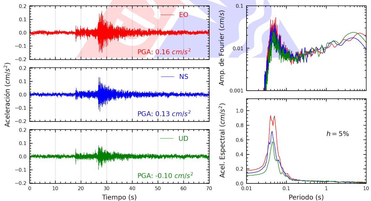
Figura A.12: Registros tiempo-historia, espectros de Fourier y de respuesta en las direcciones EO, NS y vertical de la estación UCSS. Sismo de Chilca, Cañete - Lima del 2025-01-10, 01:18:15 (Hora local)
