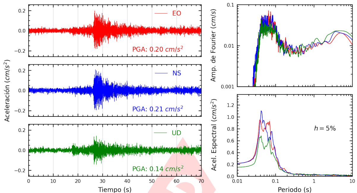
Figura A.9: Registros tiempo-historia, espectros de Fourier y de respuesta en las direcciones EO, NS y vertical de la estación INDEP. Sismo de Chilca, Cañete - Lima del 2025-01-10, 01:18:15 (Hora local)
