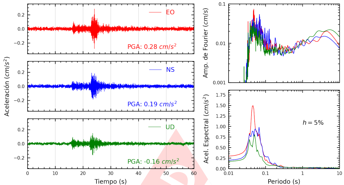
Figura A.7: Registros tiempo-historia, espectros de Fourier y de respuesta en las direcciones EO, NS y vertical de la estación UPCVI. Sismo de Chilca, Cañete - Lima del 2025-01-10, 01:18:15 (Hora local)
