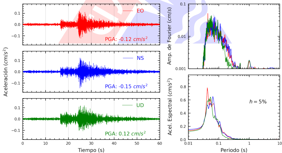
Figura A.14: Registros tiempo-historia, espectros de Fourier y de respuesta en las direcciones EO, NS y vertical de la estación ASIA. Sismo de Chilca, Cañete - Lima del 2025-01-10, 01:18:15 (Hora local)
