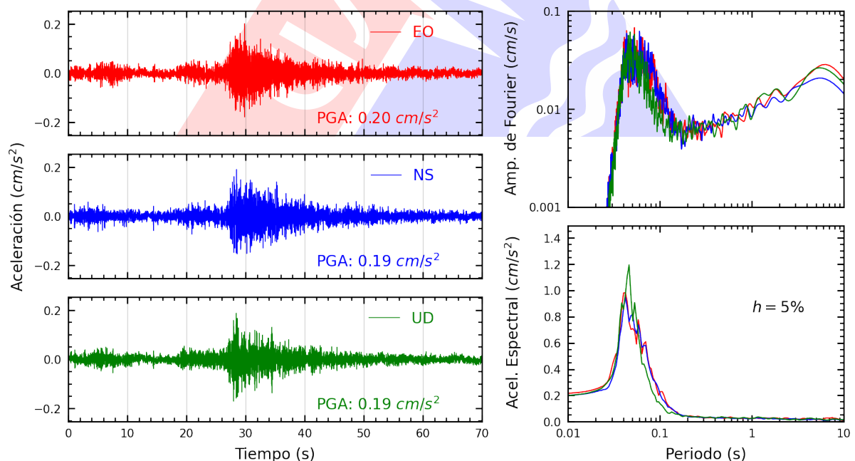
Figura A.10: Registros tiempo-historia, espectros de Fourier y de respuesta en las direcciones EO, NS y vertical de la estación JOSEO. Sismo de Chilca, Cañete - Lima del 2025-01-10, 01:18:15 (Hora local)
