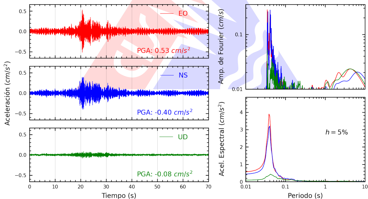
Figura A.2: Registros tiempo-historia, espectros de Fourier y de respuesta en las direcciones EO, NS y vertical de la estación DHNPE. Sismo de Chilca, Cañete - Lima del 2025-01-10, 01:18:15 (Hora local)
