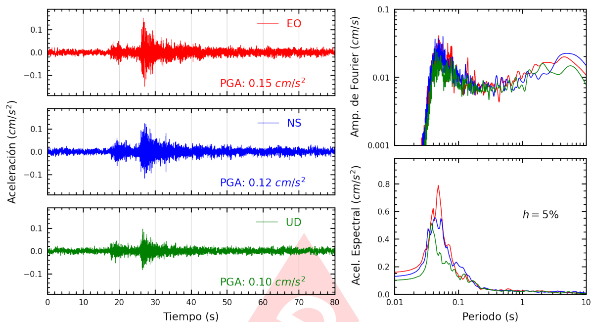
Figura A.13: Registros tiempo-historia, espectros de Fourier y de respuesta en las direcciones EO, NS y vertical de la estación FICPE. Sismo de Chilca, Cañete - Lima del 2025-01-10, 01:18:15 (Hora local)
