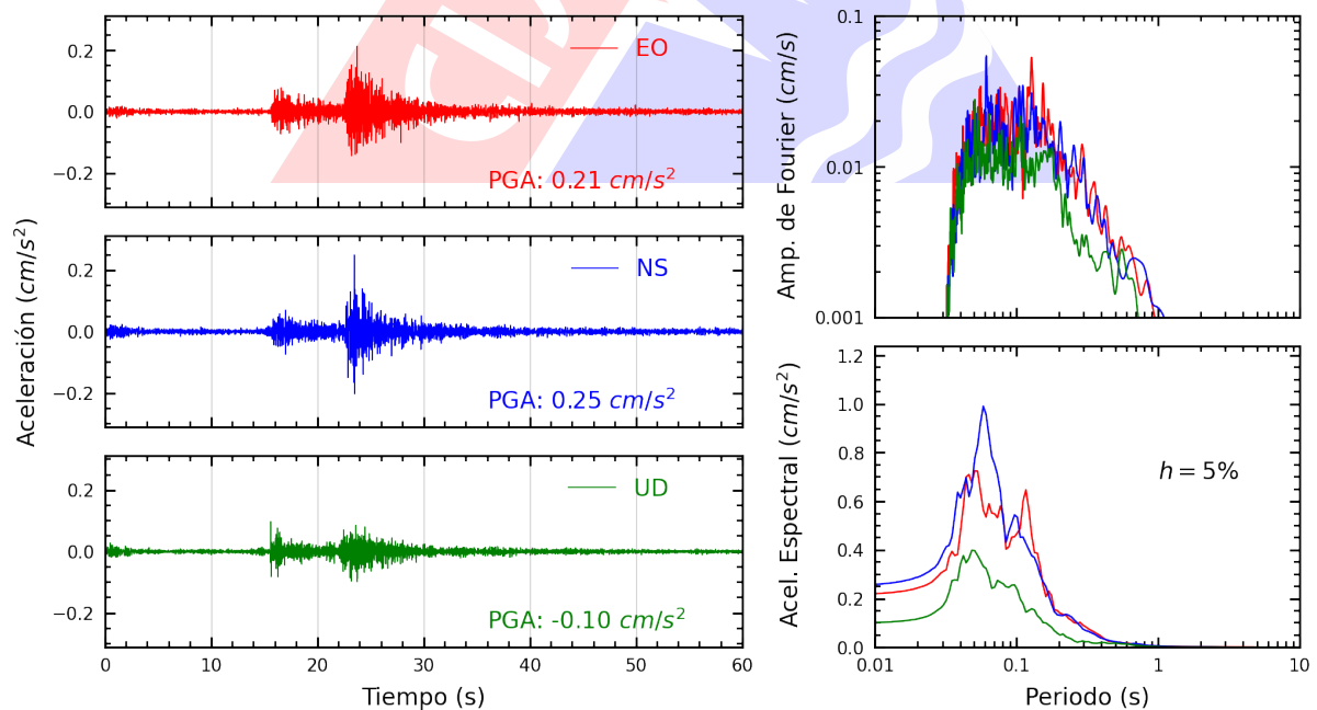
Figura A.8: Registros tiempo-historia, espectros de Fourier y de respuesta en las direcciones EO, NS y vertical de la estación BRISA. Sismo de Chilca, Cañete - Lima del 2025-01-10, 01:18:15 (Hora local)
