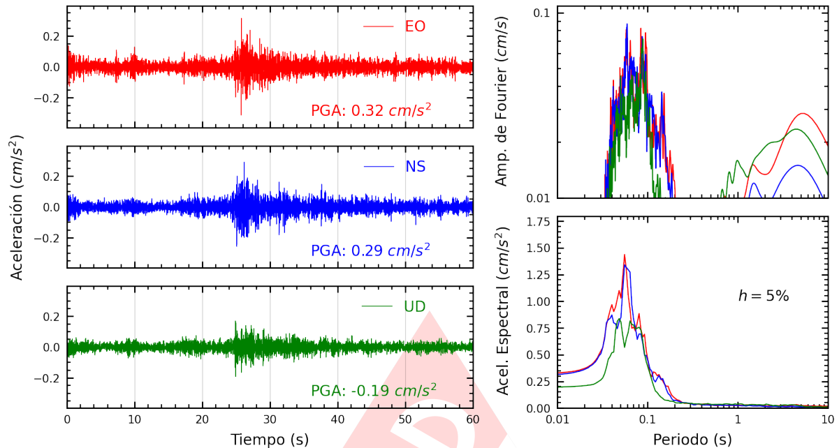
Figura A.5: Registros tiempo-historia, espectros de Fourier y de respuesta en las direcciones EO, NS y vertical de la estación USILM. Sismo de Chilca, Cañete - Lima del 2025-01-10, 01:18:15 (Hora local)
