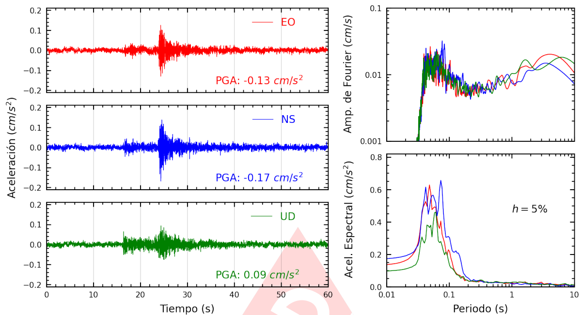
Figura A.11: Registros tiempo-historia, espectros de Fourier y de respuesta en las direcciones EO, NS y vertical de la estación SERVI. Sismo de Chilca, Cañete - Lima del 2025-01-10, 01:18:15 (Hora local)
