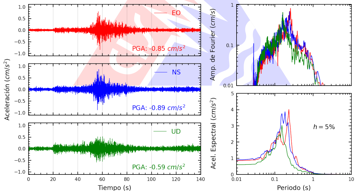
Figura A.2: Registros tiempo-historia, espectros de Fourier y de respuesta en las direcciones EO, NS y vertical de la estación UJBG4. Sismo de Tacna, Tacna - Tacna del 2025-01-13, 19:23:28 (Hora local)
