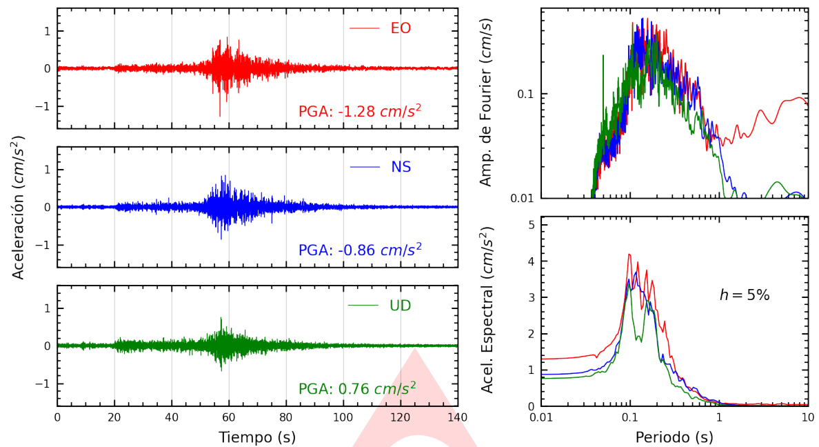
Figura A.1: Registros tiempo-historia, espectros de Fourier y de respuesta en las direcciones EO, NS y vertical de la estación UJBG3. Sismo de Tacna, Tacna - Tacna del 2025-01-13, 19:23:28 (Hora local)
