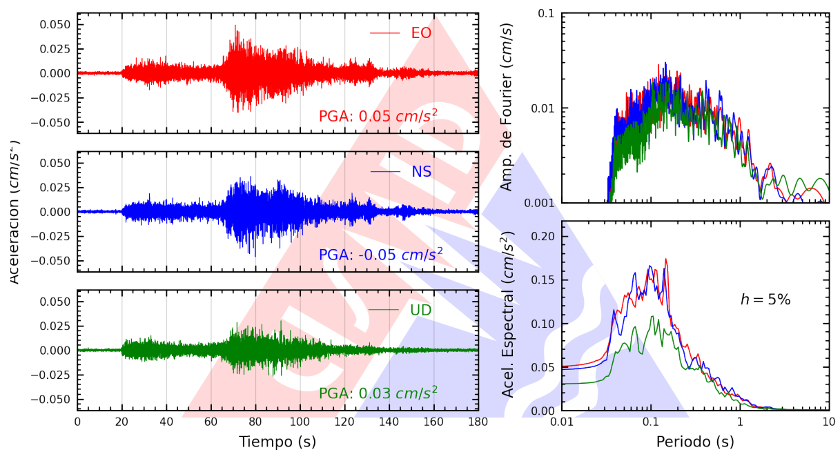
Figura A.5: Registros tiempo-historia, espectros de Fourier y de respuesta en las direcciones EO, NS y vertical de la estación UNSA2. Sismo de Tacna, Tacna - Tacna del 2025-01-13, 19:23:28 (Hora local)
