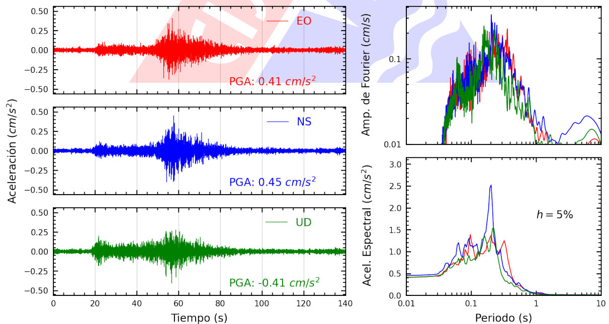
Figura A.4: Registros tiempo-historia, espectros de Fourier y de respuesta en las direcciones EO, NS y vertical de la estación CREY. Sismo de Tacna, Tacna - Tacna del 2025-01-13, 19:23:28 (Hora local)
