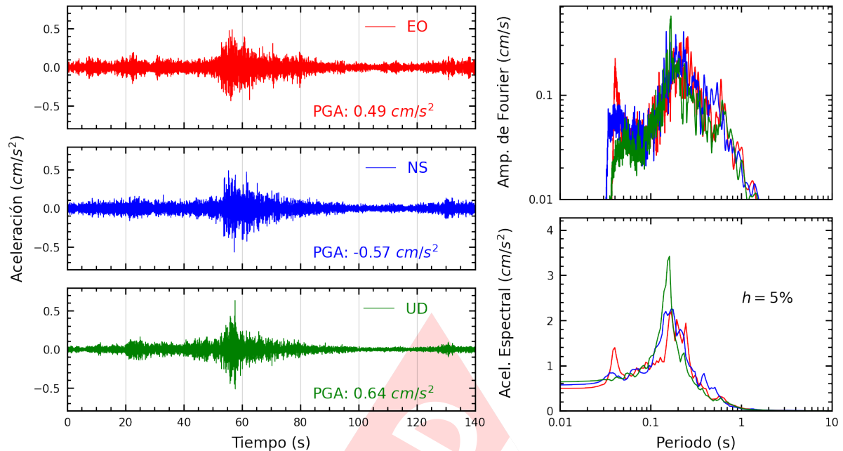
Figura A.3: Registros tiempo-historia, espectros de Fourier y de respuesta en las direcciones EO, NS y vertical de la estación UPTAC. Sismo de Tacna, Tacna - Tacna del 2025-01-13, 19:23:28 (Hora local)
