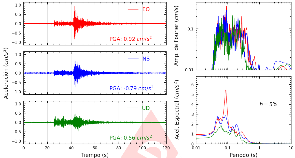
Figura A.3: Registros tiempo-historia, espectros de Fourier y de respuesta en las direcciones EO, NS y vertical de la estación CREY. Sismo de Tarata, Tarata - Tacna del 2025-01-17, 15:39:40 (Hora local)
