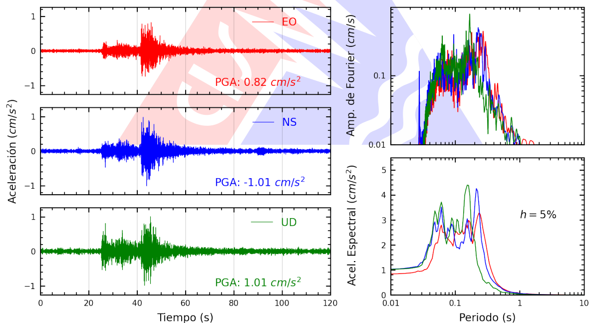
Figura A.2: Registros tiempo-historia, espectros de Fourier y de respuesta en las direcciones EO, NS y vertical de la estación UJBG4. Sismo de Tarata, Tarata - Tacna del 2025-01-17, 15:39:40 (Hora local)
