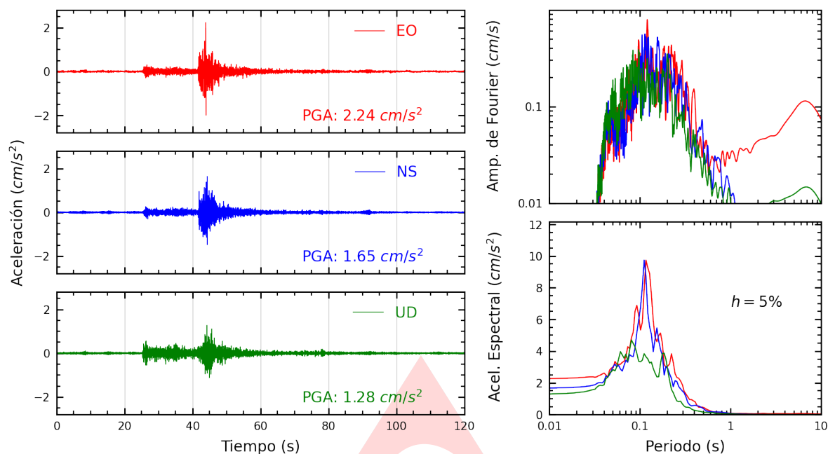
Figura A.1: Registros tiempo-historia, espectros de Fourier y de respuesta en las direcciones EO, NS y vertical de la estación UJBG3. Sismo de Tarata, Tarata - Tacna del 2025-01-17, 15:39:40 (Hora local)
