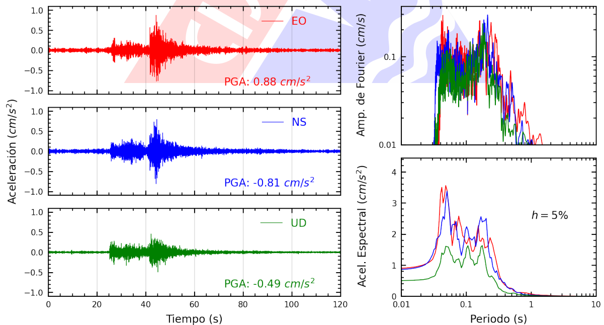
Figura A.4: Registros tiempo-historia, espectros de Fourier y de respuesta en las direcciones EO, NS y vertical de la estación UPTAC. Sismo de Tarata, Tarata - Tacna del 2025-01-17, 15:39:40 (Hora local)
