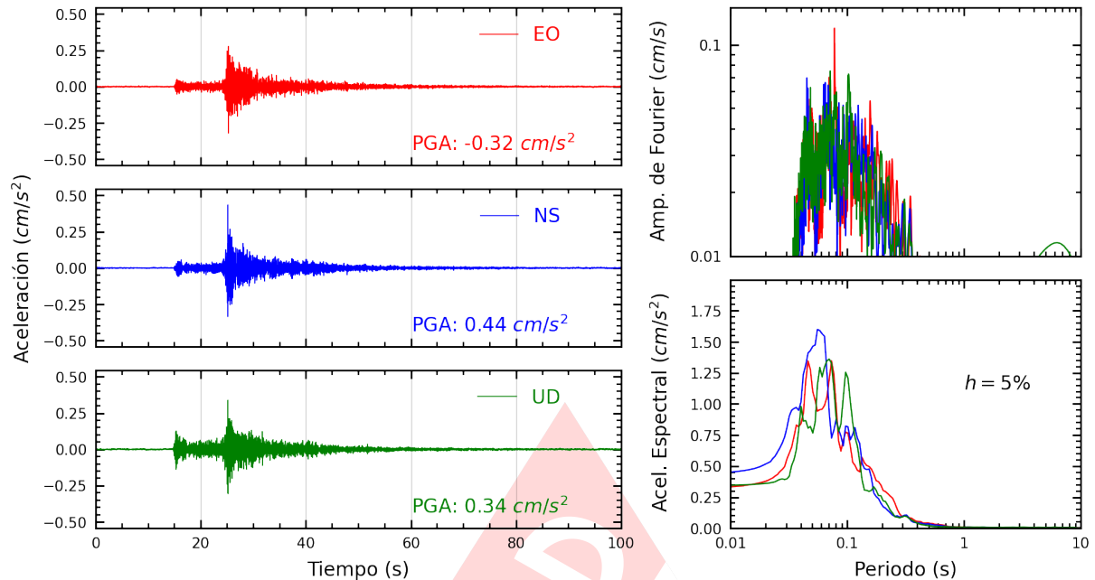
Figura A.5: Registros tiempo-historia, espectros de Fourier y de respuesta en las direcciones EO, NS y vertical de la estación CARAL. Sismo de Huacho, Huaura - Lima del 2025-01-19, 03:41:30 (Hora local)
