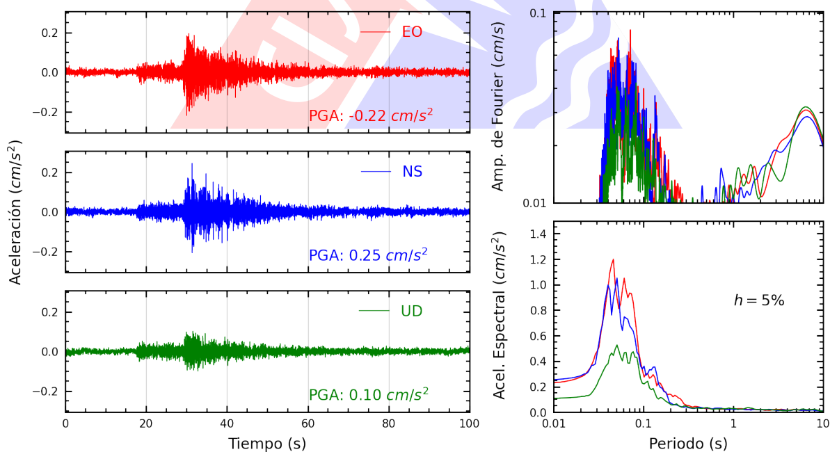
Figura A.12: Registros tiempo-historia, espectros de Fourier y de respuesta en las direcciones EO, NS y vertical de la estación FICPE. Sismo de Huacho, Huaura - Lima del 2025-01-19, 03:41:30 (Hora local)
