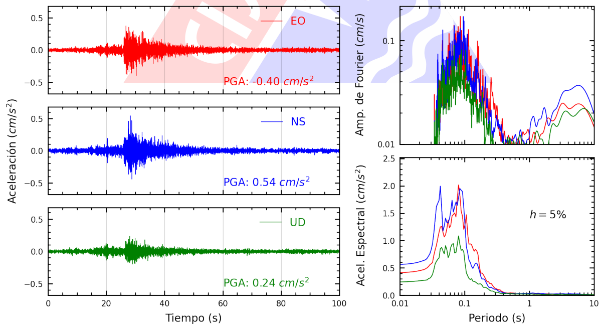
Figura A.4: Registros tiempo-historia, espectros de Fourier y de respuesta en las direcciones EO, NS y vertical de la estación DEFEN. Sismo de Huacho, Huaura - Lima del 2025-01-19, 03:41:30 (Hora local)
