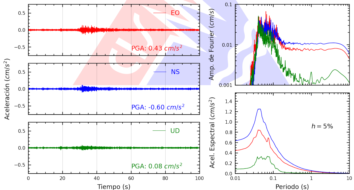
Figura A.2: Registros tiempo-historia, espectros de Fourier y de respuesta en las direcciones EO, NS y vertical de la estación ATARJ. Sismo de Huacho, Huaura - Lima del 2025-01-19, 03:41:30 (Hora local)
