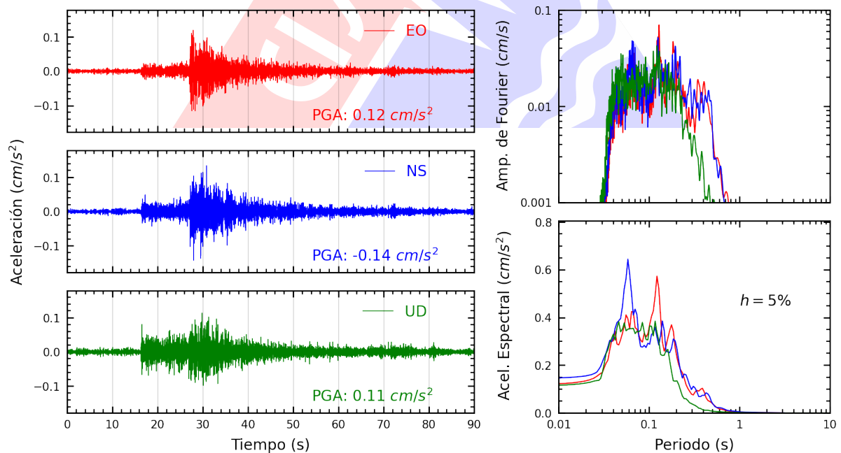
Figura A.18: Registros tiempo-historia, espectros de Fourier y de respuesta en las direcciones EO, NS y vertical de la estación VHAY2. Sismo de Huacho, Huaura - Lima del 2025-01-19, 03:41:30 (Hora local)
