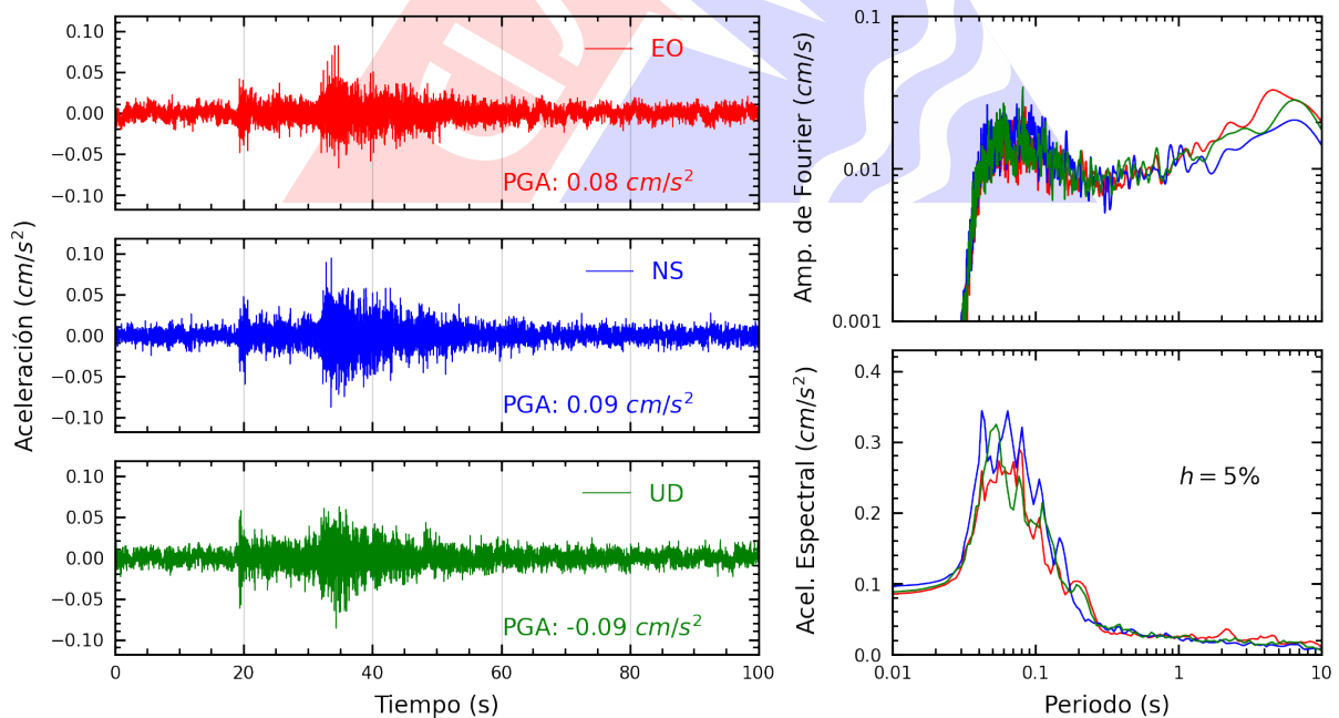
Figura A.20: Registros tiempo-historia, espectros de Fourier y de respuesta en las direcciones EO, NS y vertical de la estación SERVI. Sismo de Huacho, Huaura - Lima del 2025-01-19, 03:41:30 (Hora local)
