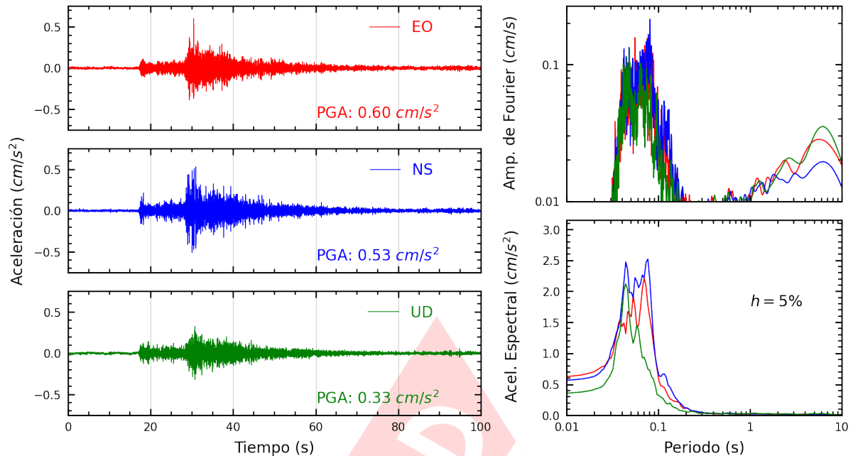
Figura A.3: Registros tiempo-historia, espectros de Fourier y de respuesta en las direcciones EO, NS y vertical de la estación JOSEO. Sismo de Huacho, Huaura - Lima del 2025-01-19, 03:41:30 (Hora local)
