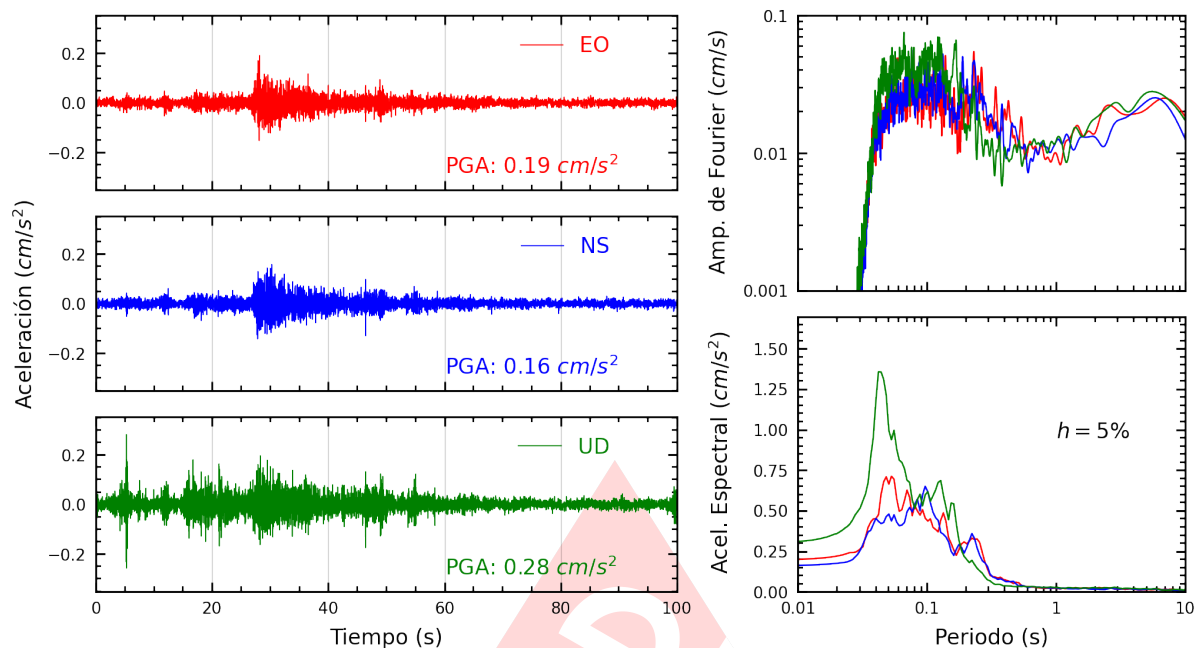
Figura A.9: Registros tiempo-historia, espectros de Fourier y de respuesta en las direcciones EO, NS y vertical de la estación MDPP. Sismo de Huacho, Huaura - Lima del 2025-01-19, 03:41:30 (Hora local)
