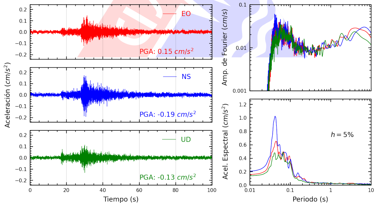
Figura A.14: Registros tiempo-historia, espectros de Fourier y de respuesta en las direcciones EO, NS y vertical de la estación COMAS. Sismo de Huacho, Huaura - Lima del 2025-01-19, 03:41:30 (Hora local)
