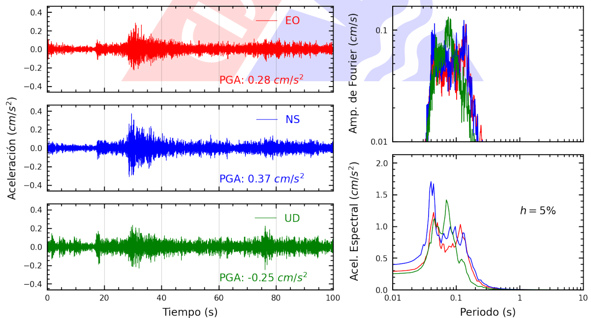
Figura A.6: Registros tiempo-historia, espectros de Fourier y de respuesta en las direcciones EO, NS y vertical de la estación CARA2. Sismo de Huacho, Huaura - Lima del 2025-01-19, 03:41:30 (Hora local)
