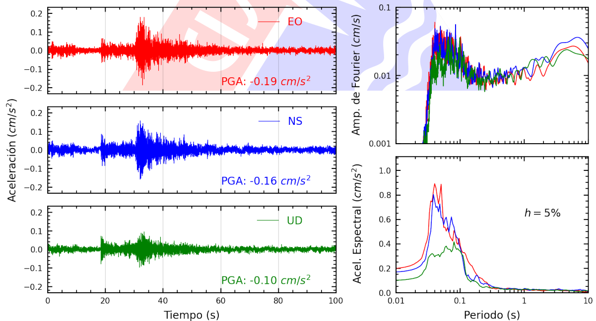
Figura A.16: Registros tiempo-historia, espectros de Fourier y de respuesta en las direcciones EO, NS y vertical de la estación CEPRE. Sismo de Huacho, Huaura - Lima del 2025-01-19, 03:41:30 (Hora local)
