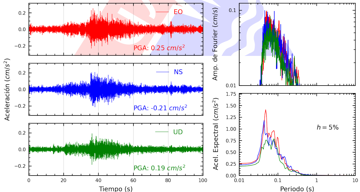
Figura A.10: Registros tiempo-historia, espectros de Fourier y de respuesta en las direcciones EO, NS y vertical de la estación UNTEL. Sismo de Huacho, Huaura - Lima del 2025-01-19, 03:41:30 (Hora local)
