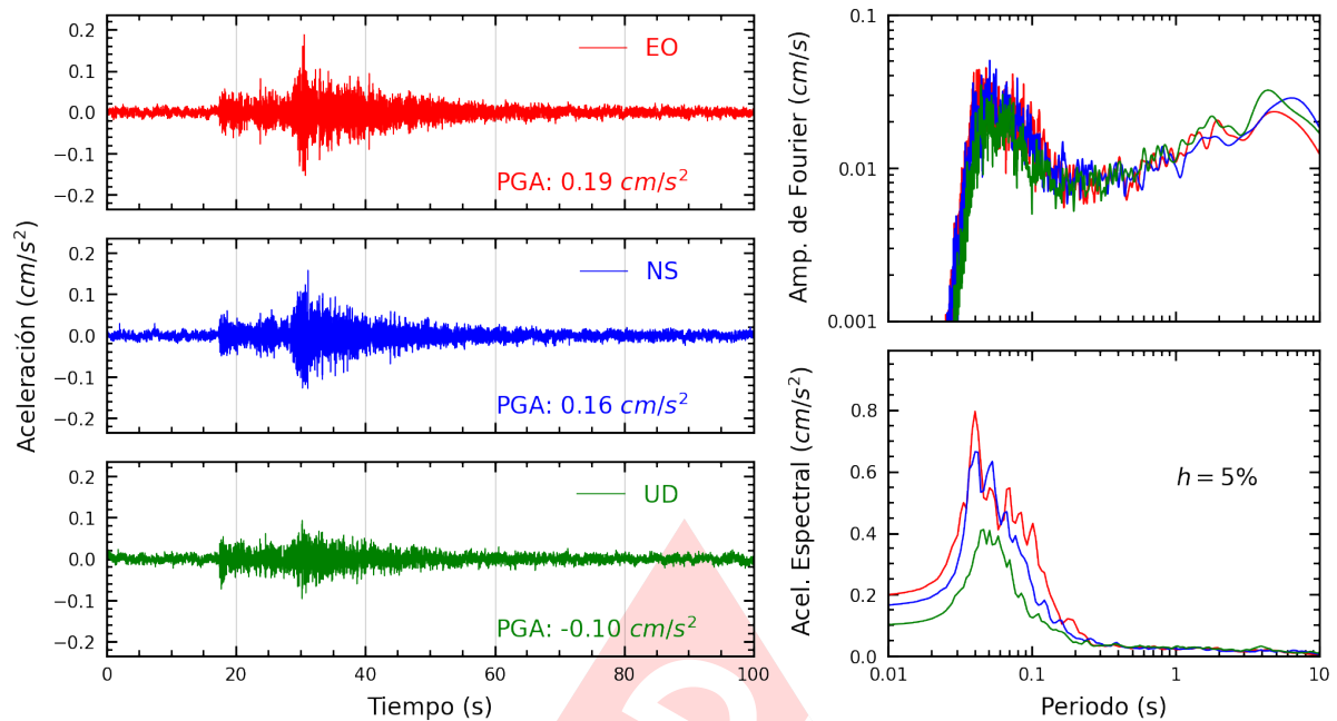
Figura A.15: Registros tiempo-historia, espectros de Fourier y de respuesta en las direcciones EO, NS y vertical de la estación UCSS. Sismo de Huacho, Huaura - Lima del 2025-01-19, 03:41:30 (Hora local)
