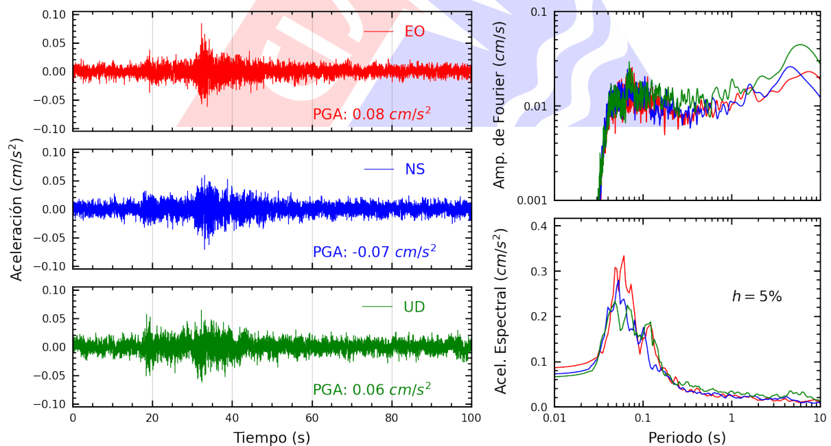
Figura A.22: Registros tiempo-historia, espectros de Fourier y de respuesta en las direcciones EO, NS y vertical de la estación UNFV. Sismo de Huacho, Huaura - Lima del 2025-01-19, 03:41:30 (Hora local)
