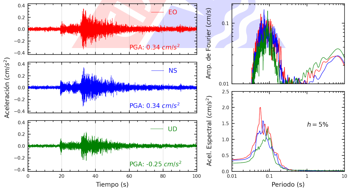
Figura A.8: Registros tiempo-historia, espectros de Fourier y de respuesta en las direcciones EO, NS y vertical de la estación USILM. Sismo de Huacho, Huaura - Lima del 2025-01-19, 03:41:30 (Hora local)
