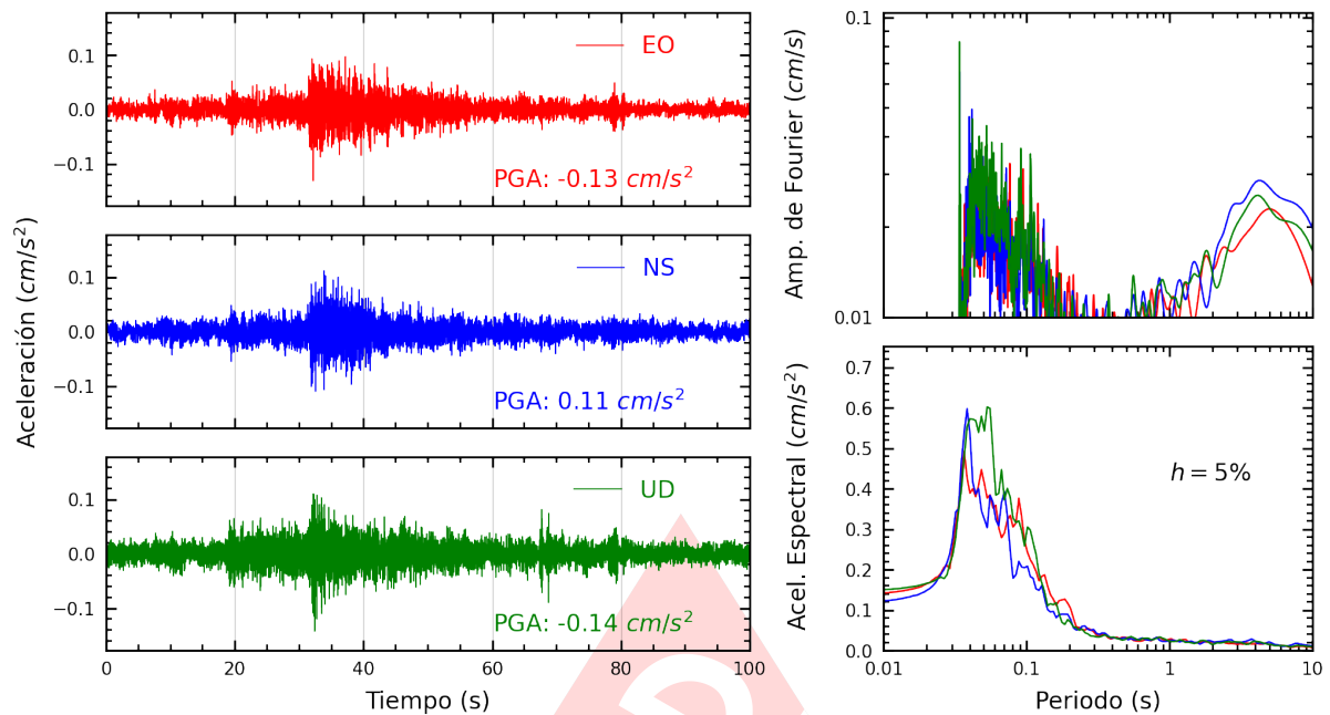
Figura A.19: Registros tiempo-historia, espectros de Fourier y de respuesta en las direcciones EO, NS y vertical de la estación USMP. Sismo de Huacho, Huaura - Lima del 2025-01-19, 03:41:30 (Hora local)
