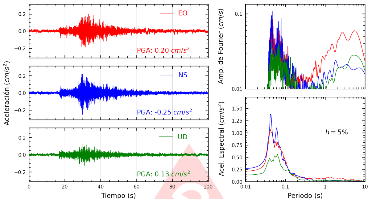
Figura A.11: Registros tiempo-historia, espectros de Fourier y de respuesta en las direcciones EO, NS y vertical de la estación UNAB. Sismo de Huacho, Huaura - Lima del 2025-01-19, 03:41:30 (Hora local)
