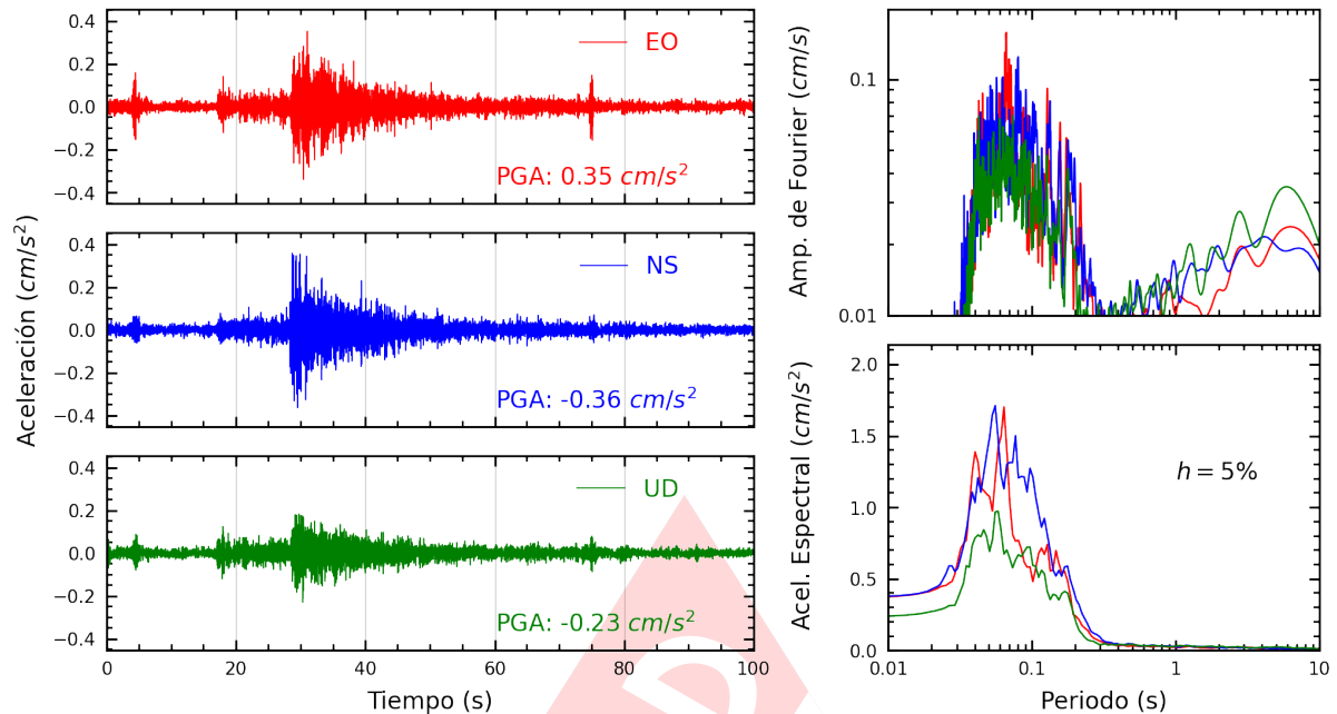
Figura A.7: Registros tiempo-historia, espectros de Fourier y de respuesta en las direcciones EO, NS y vertical de la estación INDEP. Sismo de Huacho, Huaura - Lima del 2025-01-19, 03:41:30 (Hora local)
