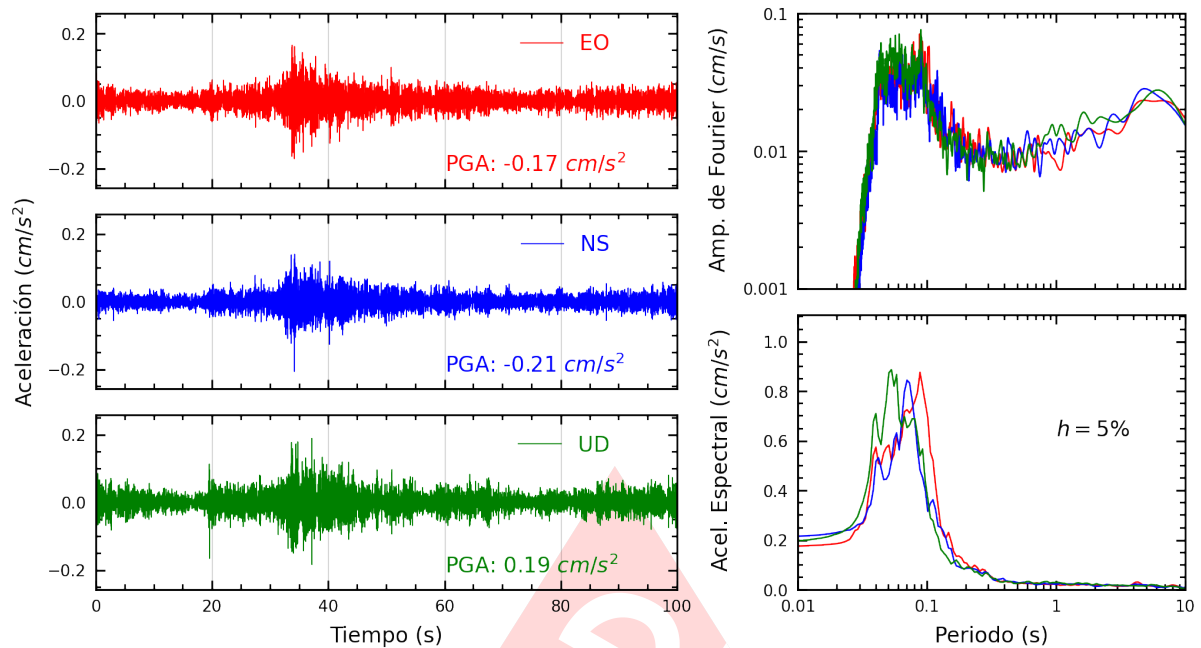
Figura A.13: Registros tiempo-historia, espectros de Fourier y de respuesta en las direcciones EO, NS y vertical de la estación URPE. Sismo de Huacho, Huaura - Lima del 2025-01-19, 03:41:30 (Hora local)
