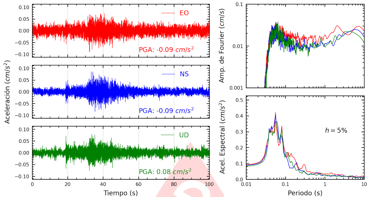
Figura A.21: Registros tiempo-historia, espectros de Fourier y de respuesta en las direcciones EO, NS y vertical de la estación IMCA. Sismo de Huacho, Huaura - Lima del 2025-01-19, 03:41:30 (Hora local)
