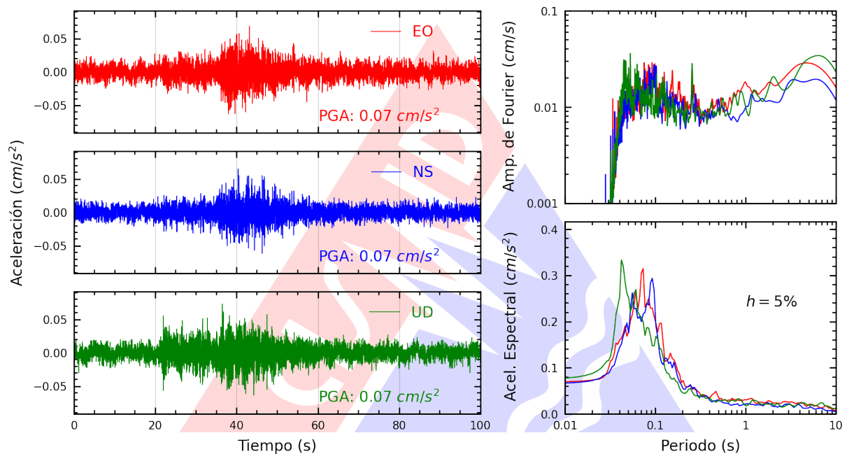
Figura A.23: Registros tiempo-historia, espectros de Fourier y de respuesta en las direcciones EO, NS y vertical de la estación USILP. Sismo de Huacho, Huaura - Lima del 2025-01-19, 03:41:30 (Hora local)
