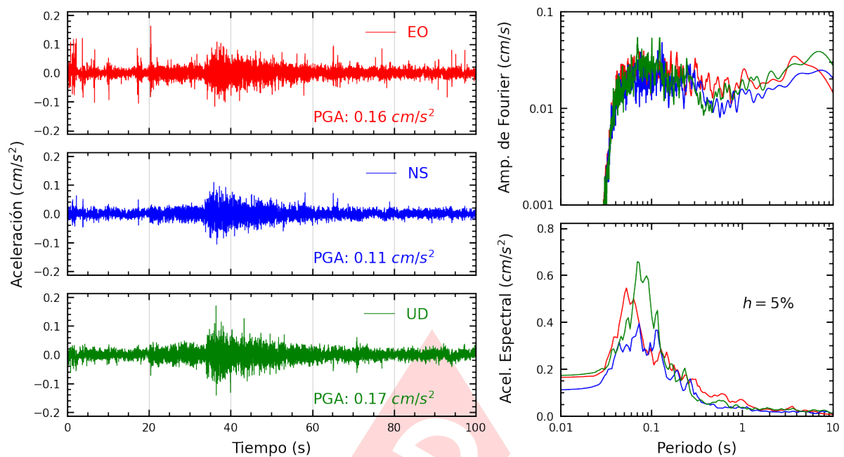
Figura A.17: Registros tiempo-historia, espectros de Fourier y de respuesta en las direcciones EO, NS y vertical de la estación SOVES. Sismo de Huacho, Huaura - Lima del 2025-01-19, 03:41:30 (Hora local)
