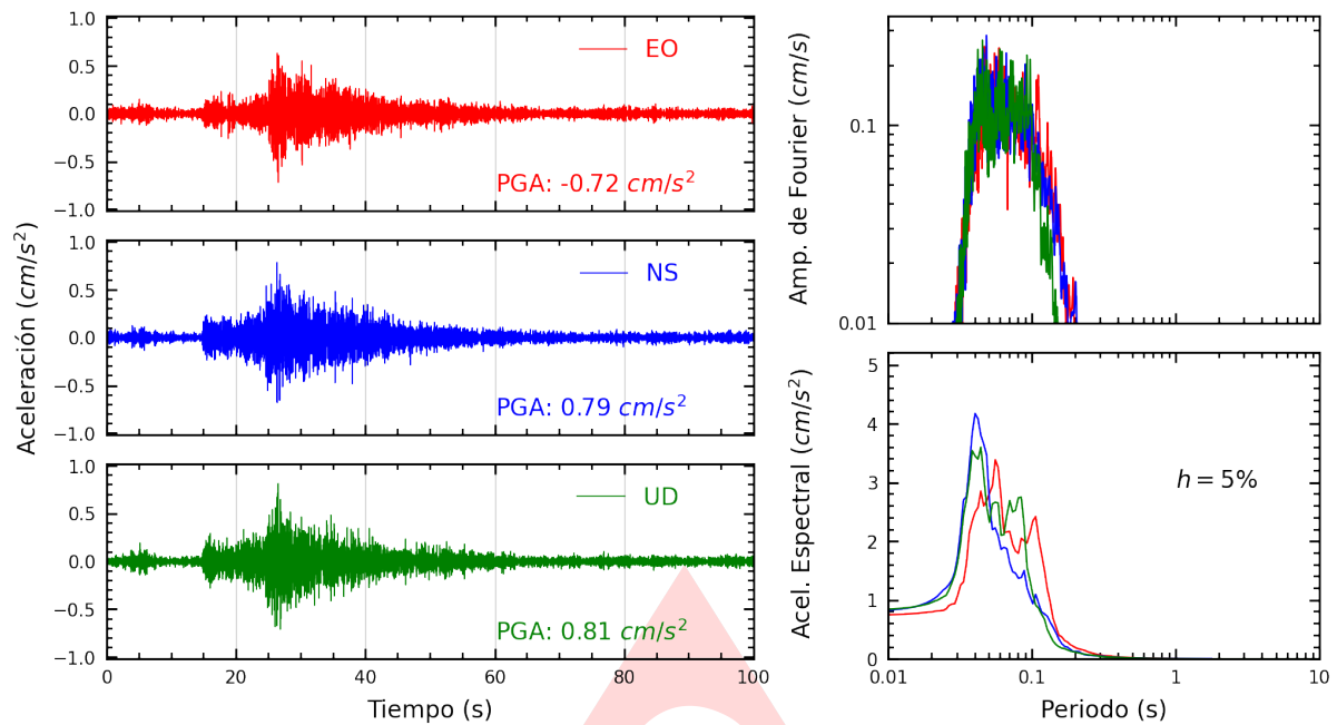
Figura A.1: Registros tiempo-historia, espectros de Fourier y de respuesta en las direcciones EO, NS y vertical de la estación SROS2. Sismo de Huacho, Huaura - Lima del 2025-01-19, 03:41:30 (Hora local)
