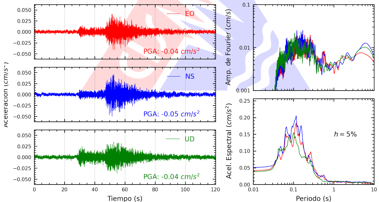
Figura A.2: Registros tiempo-historia, espectros de Fourier y de respuesta en las direcciones EO, NS y vertical de la estación CARAL. Sismo de Casma, Casma - Ancash del 2025-01-21, 05:45:11 (Hora local)
