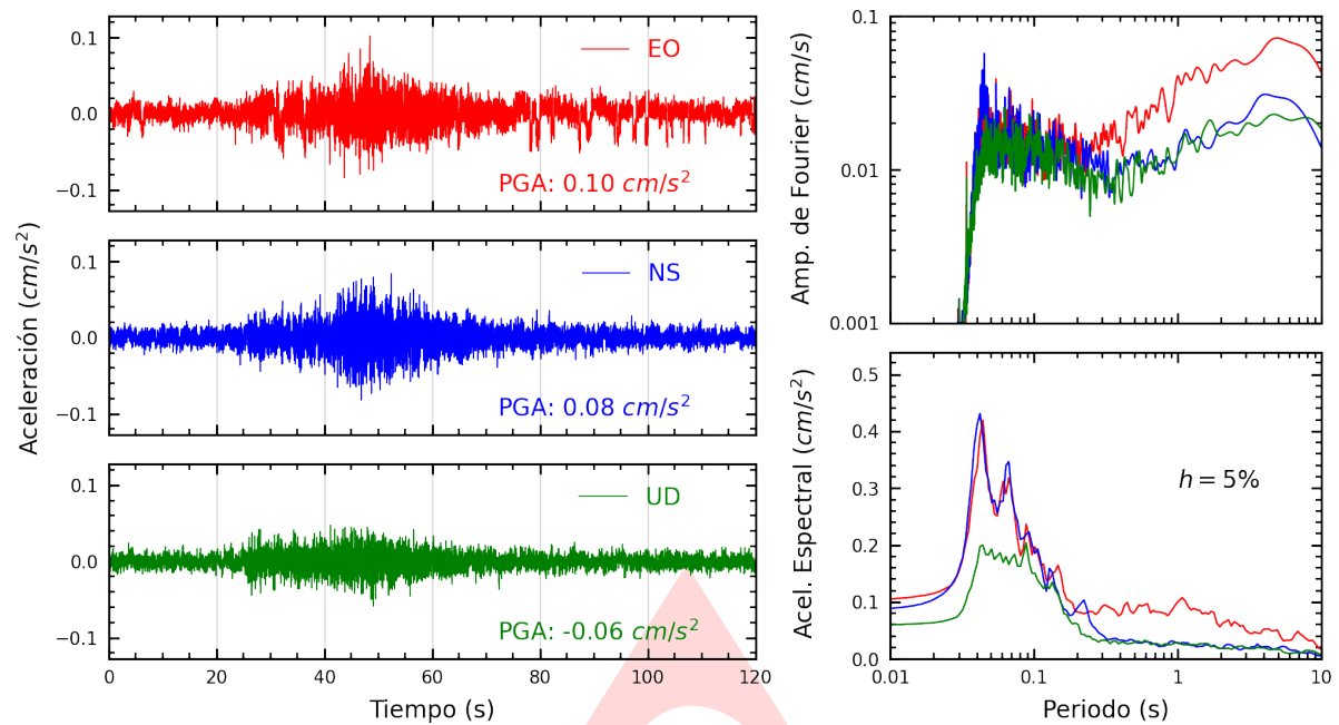
Figura A.1: Registros tiempo-historia, espectros de Fourier y de respuesta en las direcciones EO, NS y vertical de la estación UNAB. Sismo de Casma, Casma - Ancash del 2025-01-21, 05:45:11 (Hora local)
