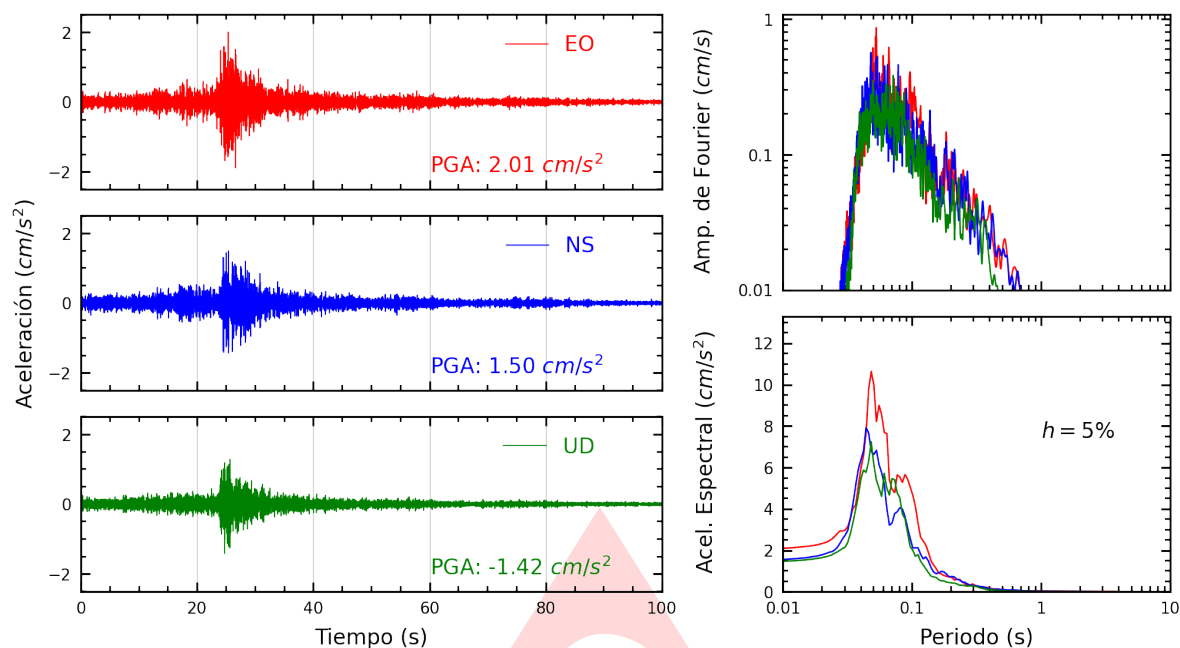
Figura A.1: Registros tiempo-historia, espectros de Fourier y de respuesta en las direcciones EO, NS y vertical de la estación UNTEL. Sismo de Chilca, Cañete - Lima del 2025-01-24, 05:39:04 (Hora local)
