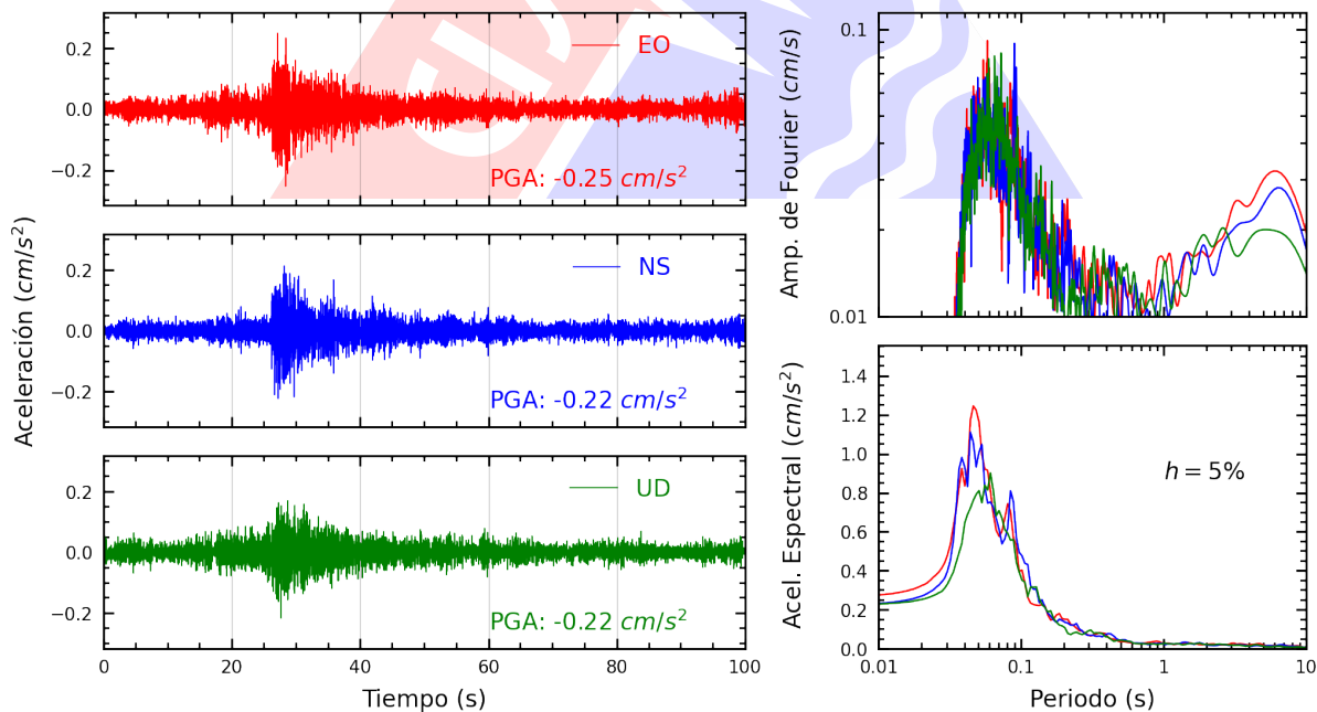
Figura A.24: Registros tiempo-historia, espectros de Fourier y de respuesta en las direcciones EO, NS y vertical de la estación IMCA. Sismo de Chilca, Cañete - Lima del 2025-01-24, 05:39:04 (Hora local)
