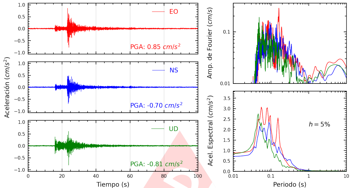
Figura A.7: Registros tiempo-historia, espectros de Fourier y de respuesta en las direcciones EO, NS y vertical de la estación USILP. Sismo de Chilca, Cañete - Lima del 2025-01-24, 05:39:04 (Hora local)
