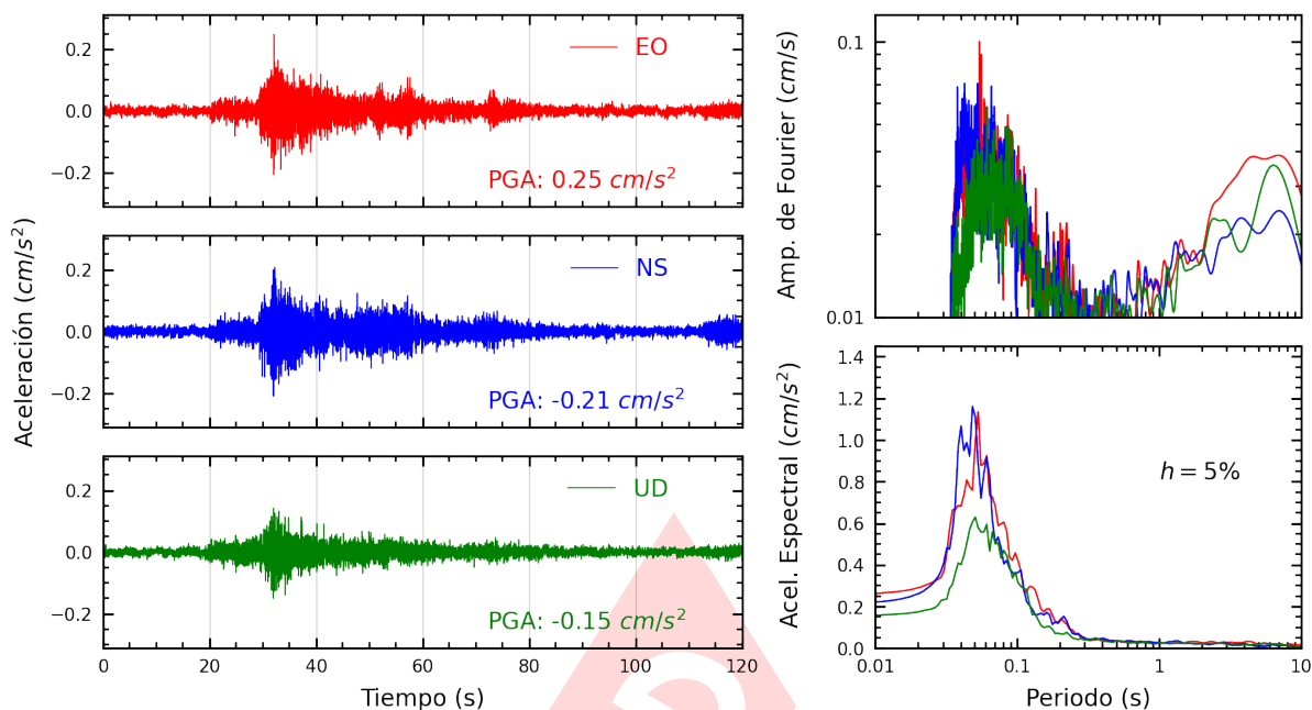
Figura A.25: Registros tiempo-historia, espectros de Fourier y de respuesta en las direcciones EO, NS y vertical de la estación COMAS. Sismo de Chilca, Cañete - Lima del 2025-01-24, 05:39:04 (Hora local)
