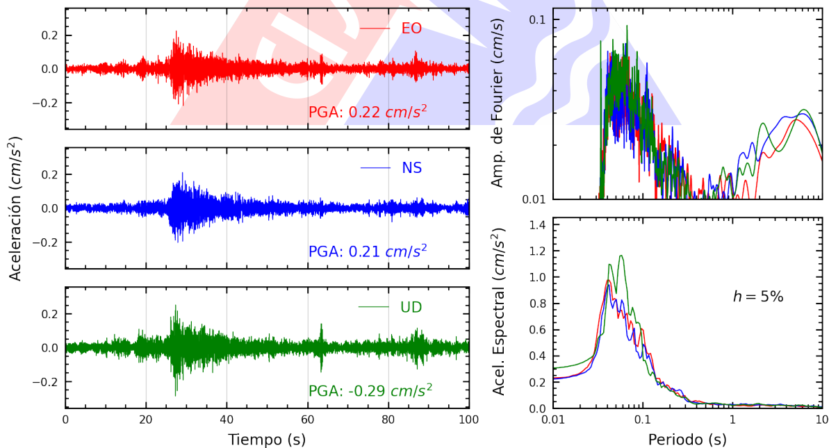
Figura A.22: Registros tiempo-historia, espectros de Fourier y de respuesta en las direcciones EO, NS y vertical de la estación USMP. Sismo de Chilca, Cañete - Lima del 2025-01-24, 05:39:04 (Hora local)
