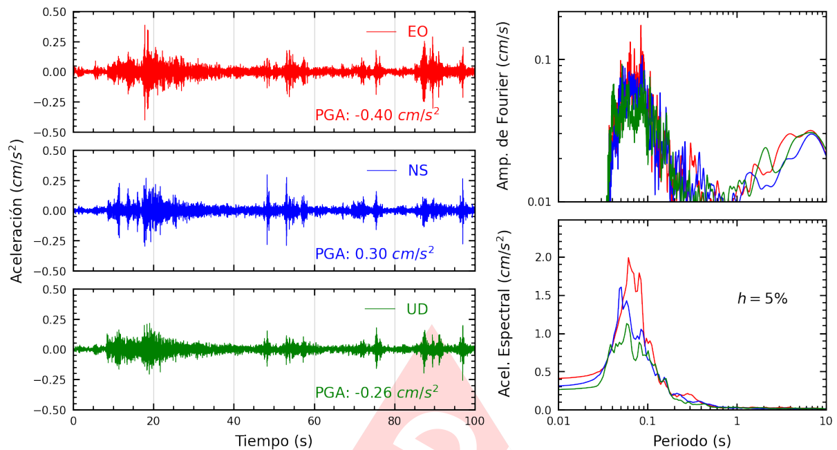
Figura A.17: Registros tiempo-historia, espectros de Fourier y de respuesta en las direcciones EO, NS y vertical de la estación UPCSM. Sismo de Chilca, Cañete - Lima del 2025-01-24, 05:39:04 (Hora local)
