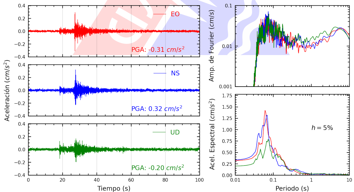
Figura A.20: Registros tiempo-historia, espectros de Fourier y de respuesta en las direcciones EO, NS y vertical de la estación UNFV. Sismo de Chilca, Cañete - Lima del 2025-01-24, 05:39:04 (Hora local)
