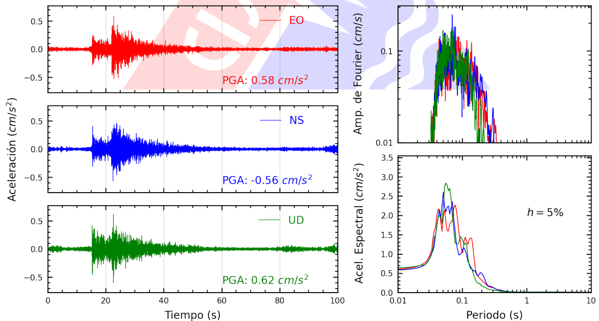
Figura A.12: Registros tiempo-historia, espectros de Fourier y de respuesta en las direcciones EO, NS y vertical de la estación ASIA. Sismo de Chilca, Cañete - Lima del 2025-01-24, 05:39:04 (Hora local)
