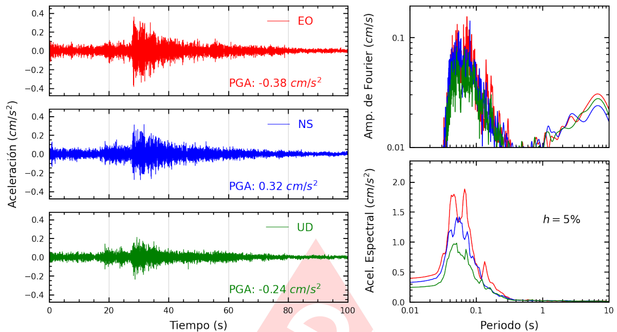
Figura A.19: Registros tiempo-historia, espectros de Fourier y de respuesta en las direcciones EO, NS y vertical de la estación FICPE. Sismo de Chilca, Cañete - Lima del 2025-01-24, 05:39:04 (Hora local)
