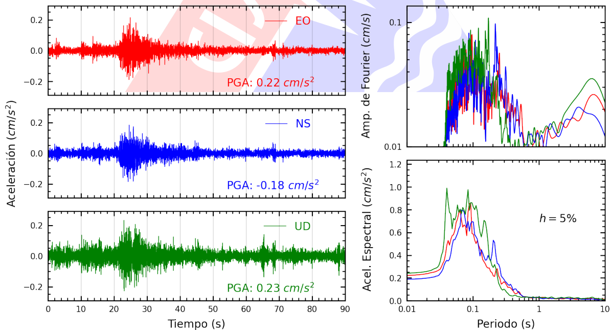
Figura A.26: Registros tiempo-historia, espectros de Fourier y de respuesta en las direcciones EO, NS y vertical de la estación MDPP. Sismo de Chilca, Cañete - Lima del 2025-01-24, 05:39:04 (Hora local)
