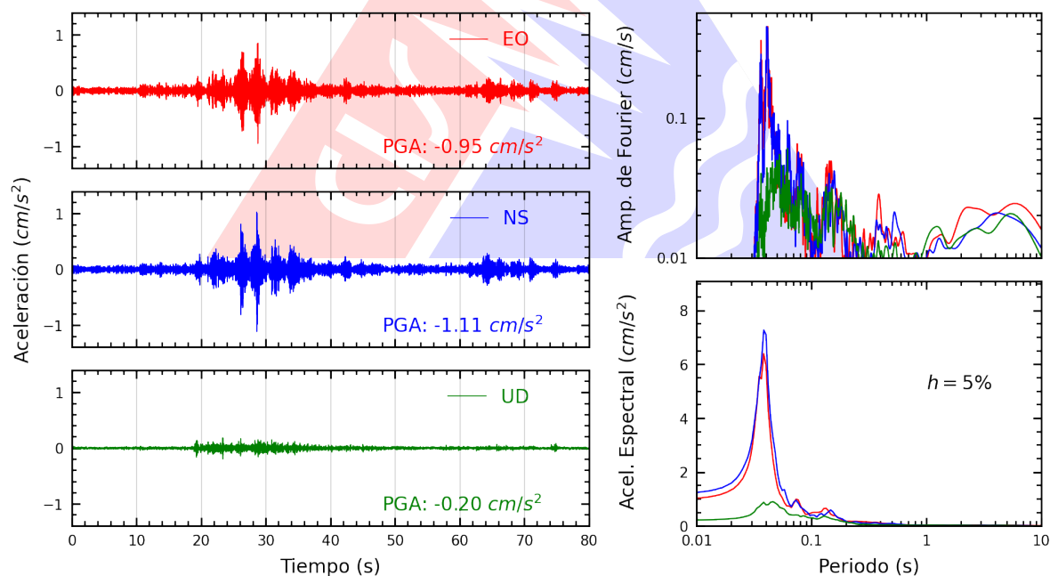
Figura A.2: Registros tiempo-historia, espectros de Fourier y de respuesta en las direcciones EO, NS y vertical de la estación DHNPE. Sismo de Chilca, Cañete - Lima del 2025-01-24, 05:39:04 (Hora local)
