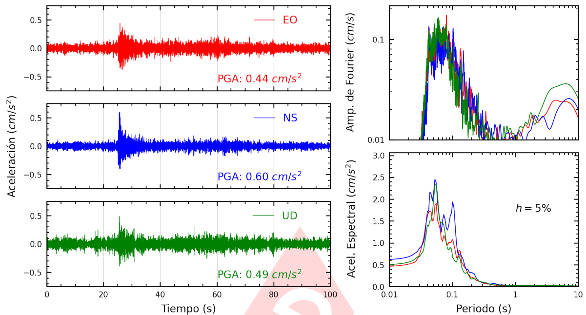
Figura A.13: Registros tiempo-historia, espectros de Fourier y de respuesta en las direcciones EO, NS y vertical de la estación URPPE. Sismo de Chilca, Cañete - Lima del 2025-01-24, 05:39:04 (Hora local)
