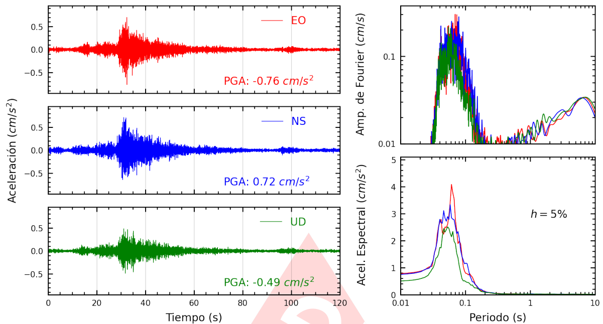
Figura A.11: Registros tiempo-historia, espectros de Fourier y de respuesta en las direcciones EO, NS y vertical de la estación JOSEO. Sismo de Chilca, Cañete - Lima del 2025-01-24, 05:39:04 (Hora local)
