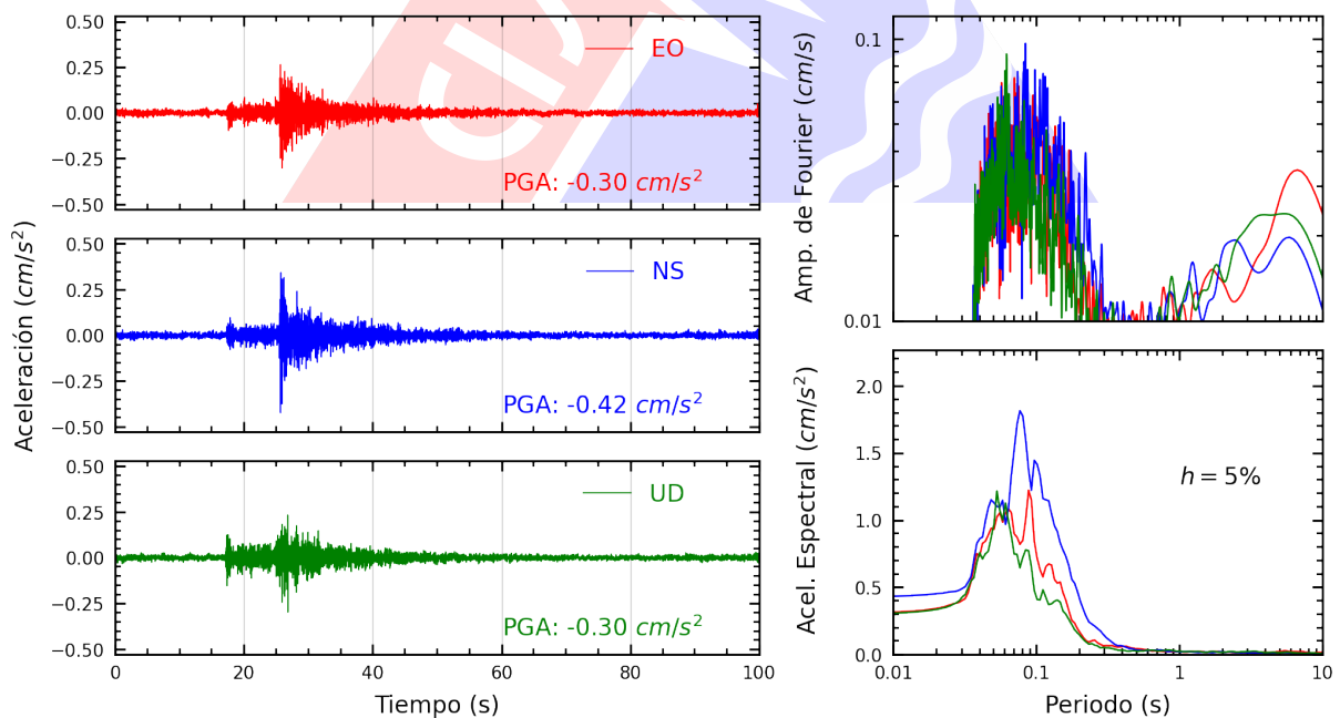
Figura A.16: Registros tiempo-historia, espectros de Fourier y de respuesta en las direcciones EO, NS y vertical de la estación SERVI. Sismo de Chilca, Cañete - Lima del 2025-01-24, 05:39:04 (Hora local)
