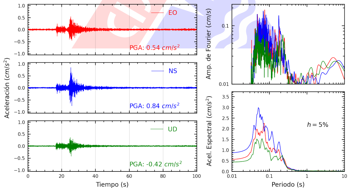
Figura A.8: Registros tiempo-historia, espectros de Fourier y de respuesta en las direcciones EO, NS y vertical de la estación UPCVI. Sismo de Chilca, Cañete - Lima del 2025-01-24, 05:39:04 (Hora local)
