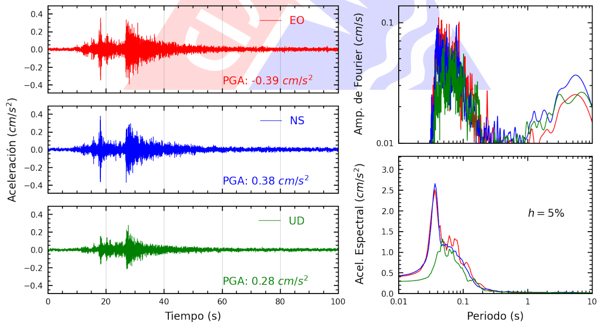
Figura A.18: Registros tiempo-historia, espectros de Fourier y de respuesta en las direcciones EO, NS y vertical de la estación CEPRE. Sismo de Chilca, Cañete - Lima del 2025-01-24, 05:39:04 (Hora local)
