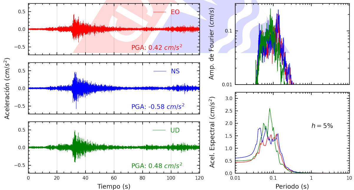
Figura A.14: Registros tiempo-historia, espectros de Fourier y de respuesta en las direcciones EO, NS y vertical de la estación CARA2. Sismo de Chilca, Cañete - Lima del 2025-01-24, 05:39:04 (Hora local)
