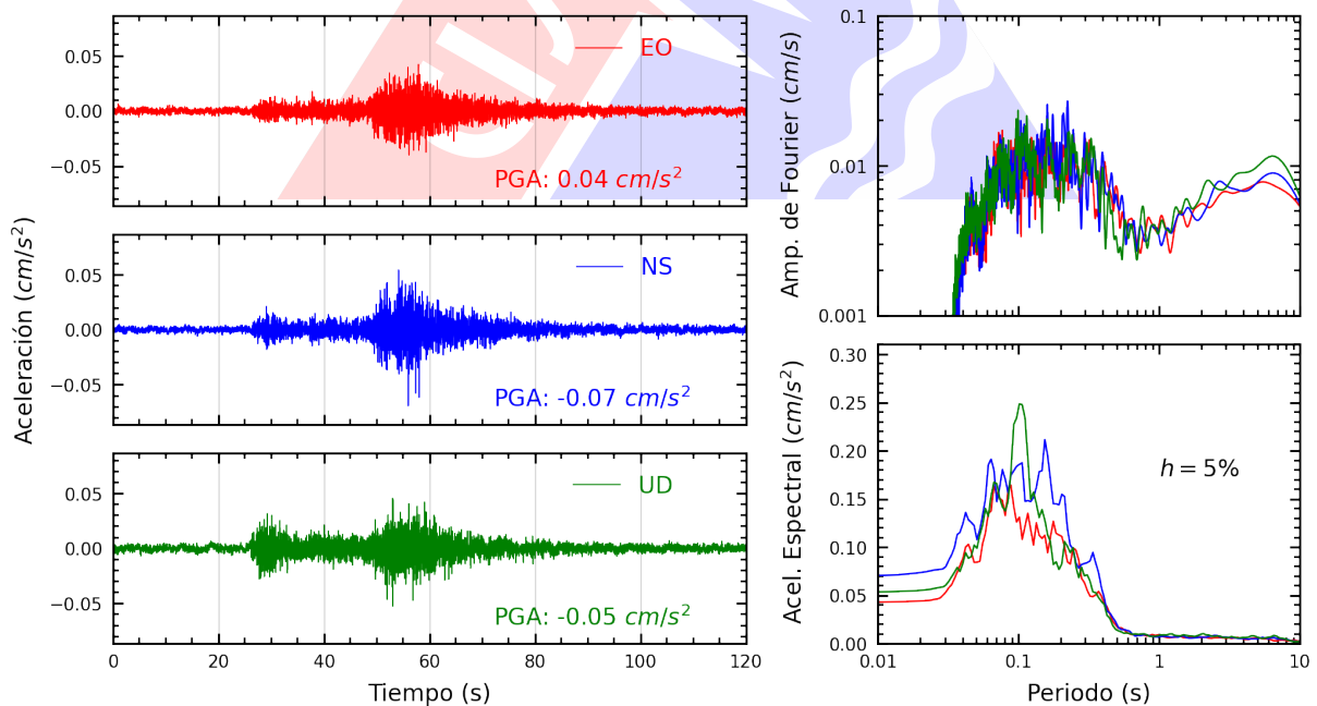
Figura A.28: Registros tiempo-historia, espectros de Fourier y de respuesta en las direcciones EO, NS y vertical de la estación CARAL. Sismo de Chilca, Cañete - Lima del 2025-01-24, 05:39:04 (Hora local)
