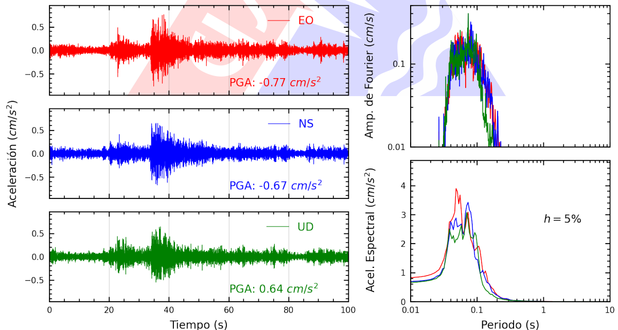
Figura A.10: Registros tiempo-historia, espectros de Fourier y de respuesta en las direcciones EO, NS y vertical de la estación SROS2. Sismo de Chilca, Cañete - Lima del 2025-01-24, 05:39:04 (Hora local)
