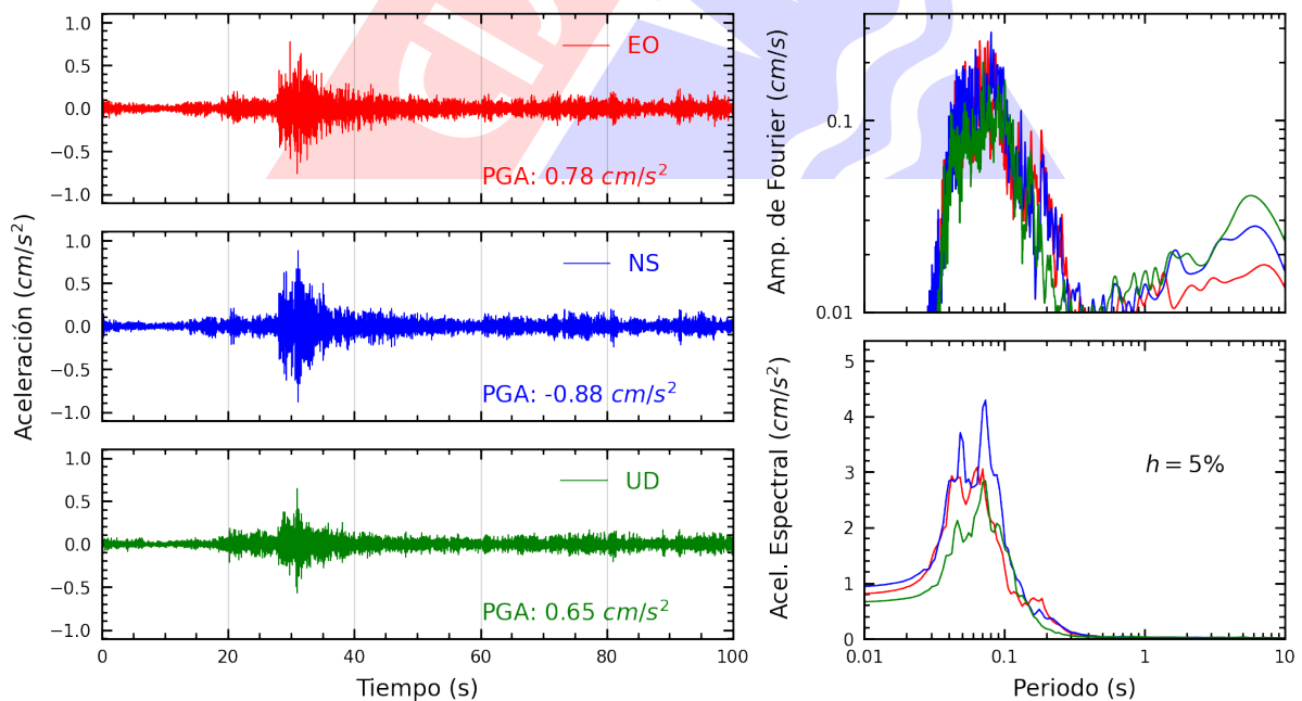
Figura A.6: Registros tiempo-historia, espectros de Fourier y de respuesta en las direcciones EO, NS y vertical de la estación INDEP. Sismo de Chilca, Cañete - Lima del 2025-01-24, 05:39:04 (Hora local)
