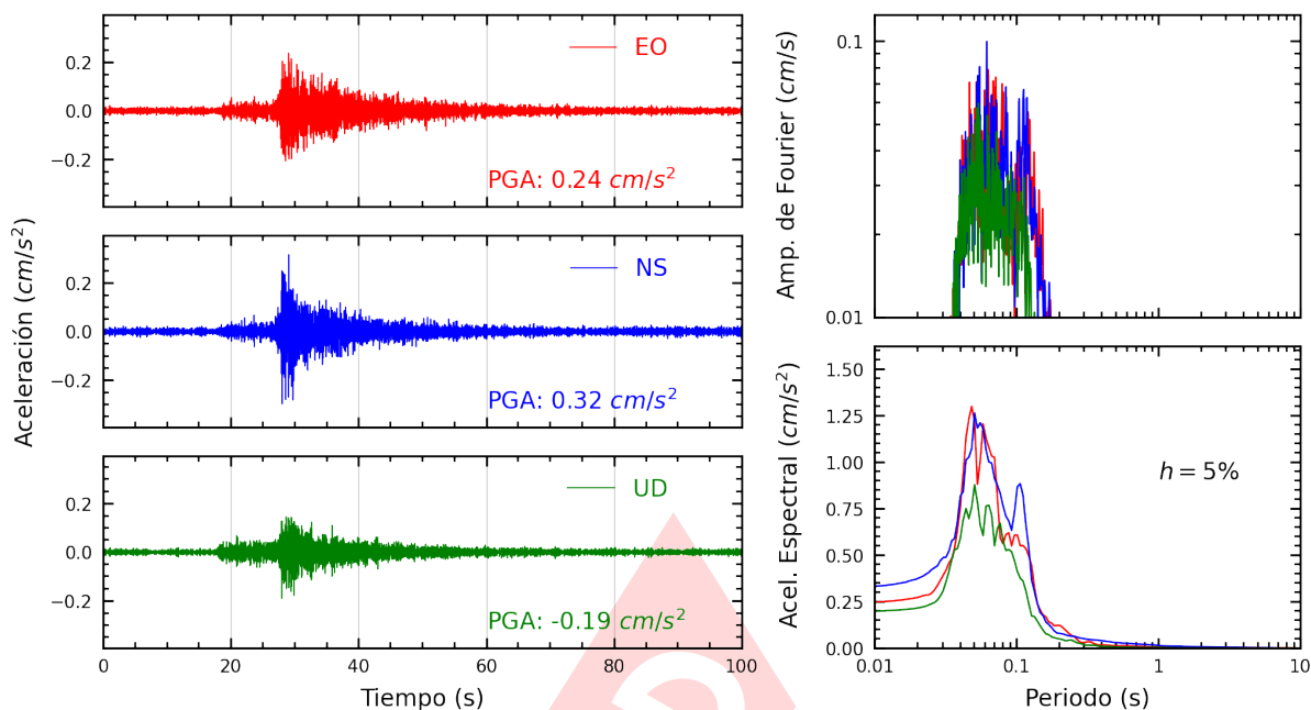
Figura A.21: Registros tiempo-historia, espectros de Fourier y de respuesta en las direcciones EO, NS y vertical de la estación ATARJ. Sismo de Chilca, Cañete - Lima del 2025-01-24, 05:39:04 (Hora local)
