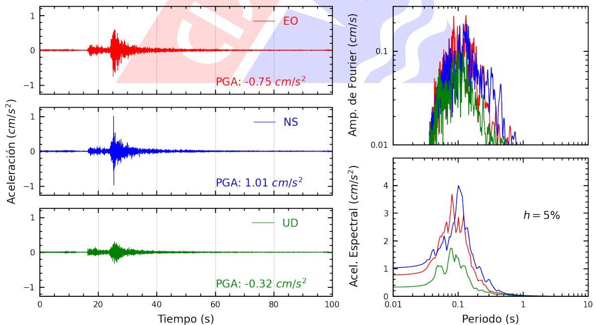
Figura A.4: Registros tiempo-historia, espectros de Fourier y de respuesta en las direcciones EO, NS y vertical de la estación BRISA. Sismo de Chilca, Cañete - Lima del 2025-01-24, 05:39:04 (Hora local)
