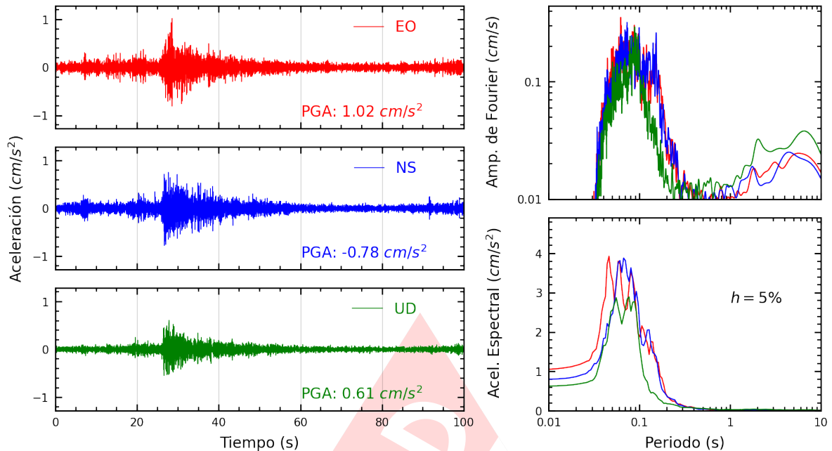
Figura A.3: Registros tiempo-historia, espectros de Fourier y de respuesta en las direcciones EO, NS y vertical de la estación USILM. Sismo de Chilca, Cañete - Lima del 2025-01-24, 05:39:04 (Hora local)
