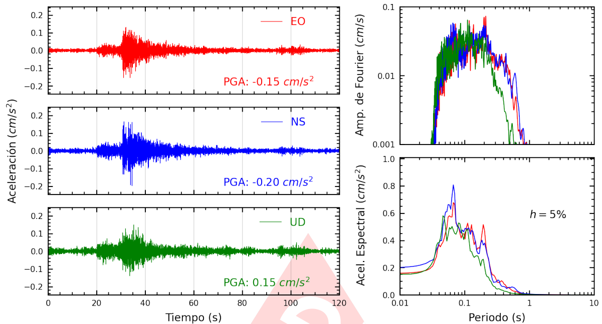
Figura A.27: Registros tiempo-historia, espectros de Fourier y de respuesta en las direcciones EO, NS y vertical de la estación VHAY2. Sismo de Chilca, Cañete - Lima del 2025-01-24, 05:39:04 (Hora local)
