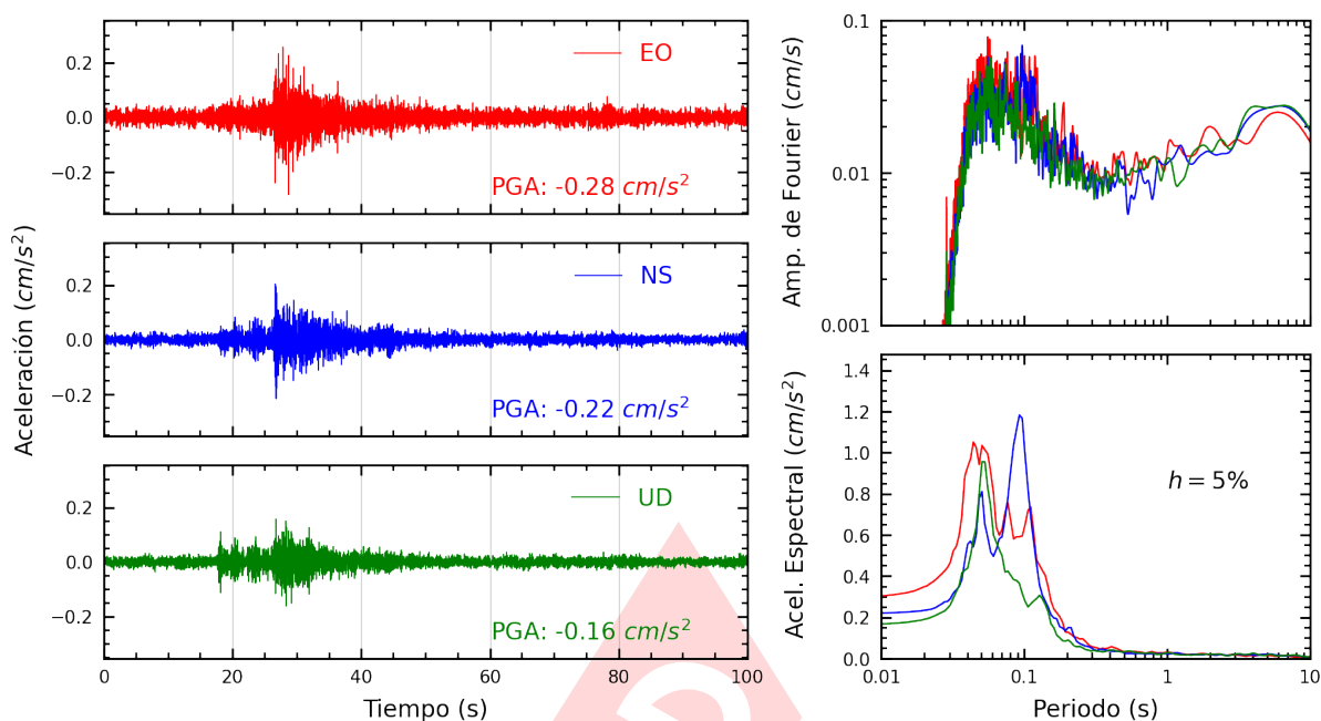
Figura A.23: Registros tiempo-historia, espectros de Fourier y de respuesta en las direcciones EO, NS y vertical de la estación INICT. Sismo de Chilca, Cañete - Lima del 2025-01-24, 05:39:04 (Hora local)
