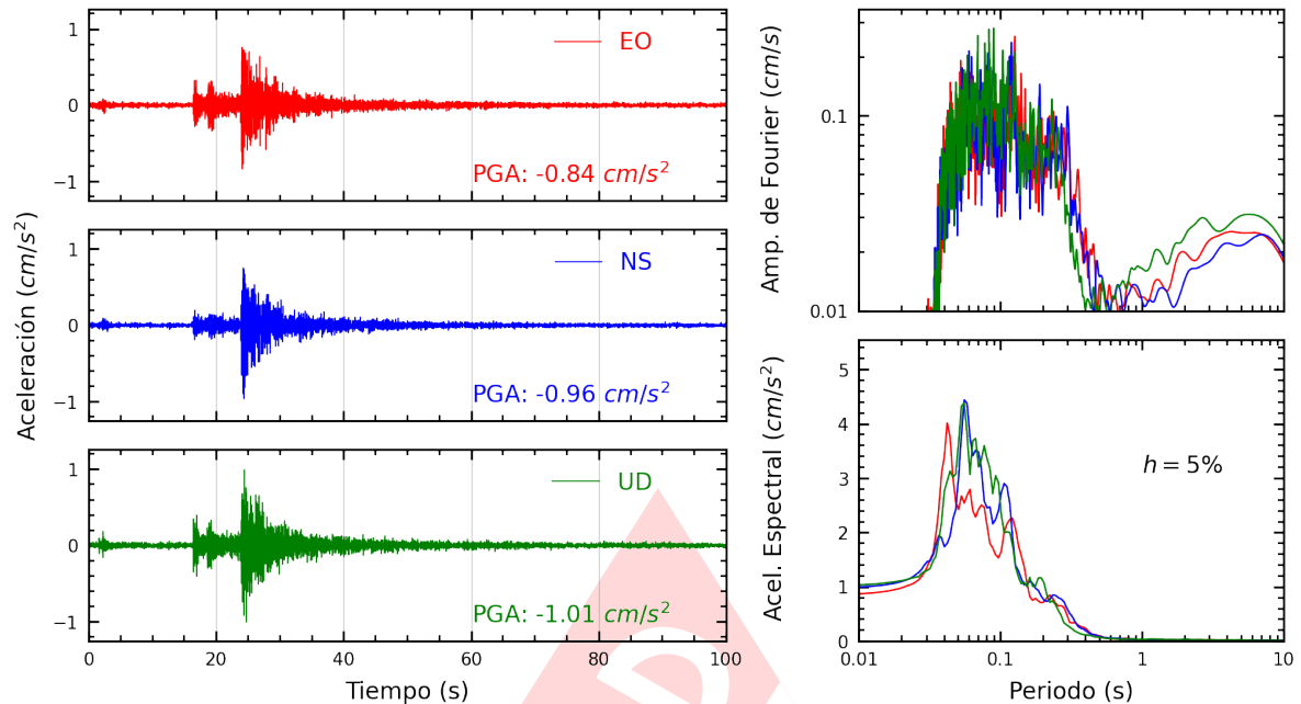
Figura A.5: Registros tiempo-historia, espectros de Fourier y de respuesta en las direcciones EO, NS y vertical de la estación SOVES. Sismo de Chilca, Cañete - Lima del 2025-01-24, 05:39:04 (Hora local)
