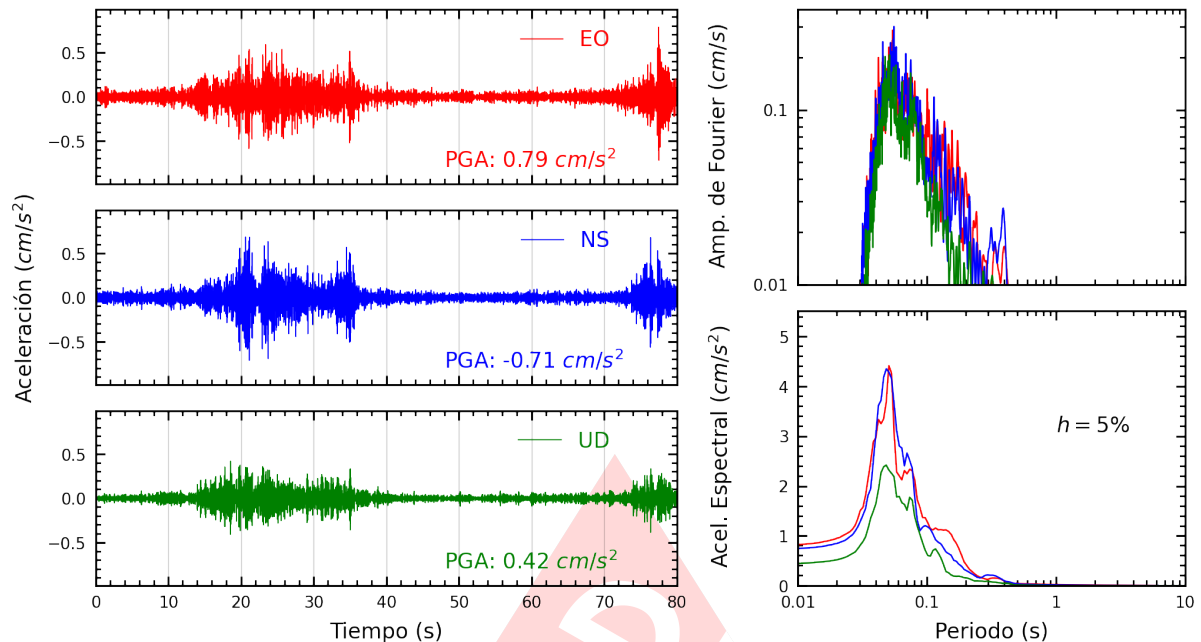
Figura A.9: Registros tiempo-historia, espectros de Fourier y de respuesta en las direcciones EO, NS y vertical de la estación PACHA. Sismo de Chilca, Cañete - Lima del 2025-01-24, 05:39:04 (Hora local)
