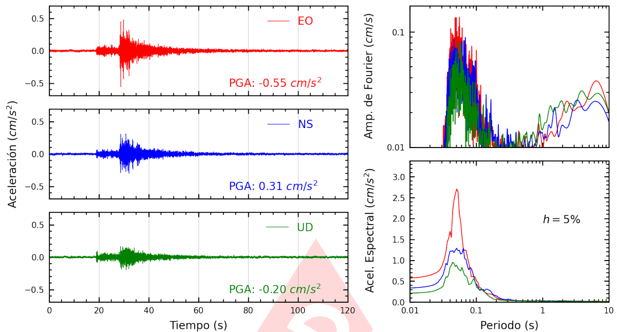
Figura A.15: Registros tiempo-historia, espectros de Fourier y de respuesta en las direcciones EO, NS y vertical de la estación UCSS. Sismo de Chilca, Cañete - Lima del 2025-01-24, 05:39:04 (Hora local)
