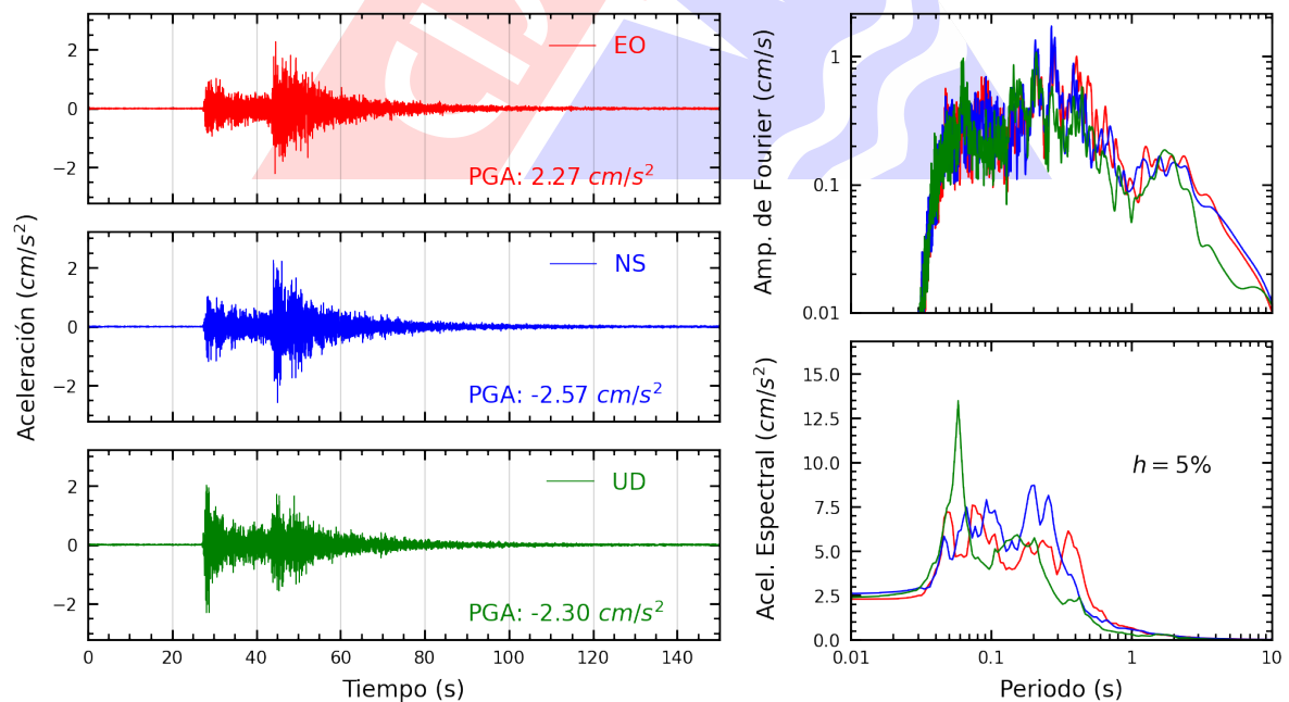
Figura A.4: Registros tiempo-historia, espectros de Fourier y de respuesta en las direcciones EO, NS y vertical de la estación CREY. Sismo de Calana, Tacna - Tacna del 2025-01-24, 11:19:05 (Hora local)
