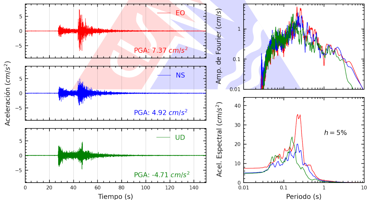
Figura A.2: Registros tiempo-historia, espectros de Fourier y de respuesta en las direcciones EO, NS y vertical de la estación UJBG4. Sismo de Calana, Tacna - Tacna del 2025-01-24, 11:19:05 (Hora local)
