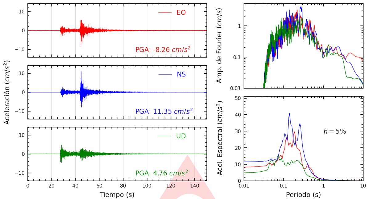
Figura A.1: Registros tiempo-historia, espectros de Fourier y de respuesta en las direcciones EO, NS y vertical de la estación UJBG3. Sismo de Calana, Tacna - Tacna del 2025-01-24, 11:19:05 (Hora local)
