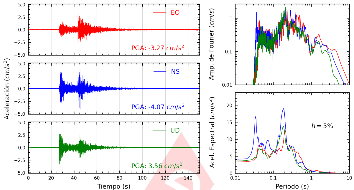
Figura A.3: Registros tiempo-historia, espectros de Fourier y de respuesta en las direcciones EO, NS y vertical de la estación UPTAC. Sismo de Calana, Tacna - Tacna del 2025-01-24, 11:19:05 (Hora local)
