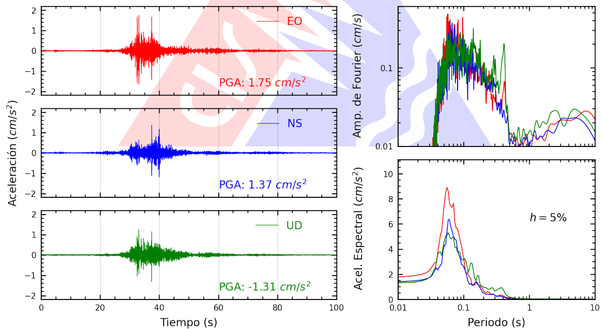
Figura A.2: Registros tiempo-historia, espectros de Fourier y de respuesta en las direcciones EO, NS y vertical de la estación UNTRM. Sismo de Jaen, Jaen - Cajamarca del 2025-01-24, 17:52:16 (Hora local)
