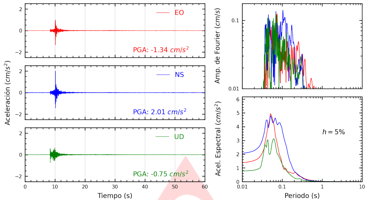
Figura A.1: Registros tiempo-historia, espectros de Fourier y de respuesta en las direcciones EO, NS y vertical de la estación UNJ. Sismo de Jaen, Jaen - Cajamarca del 2025-01-24, 17:52:16 (Hora local)
