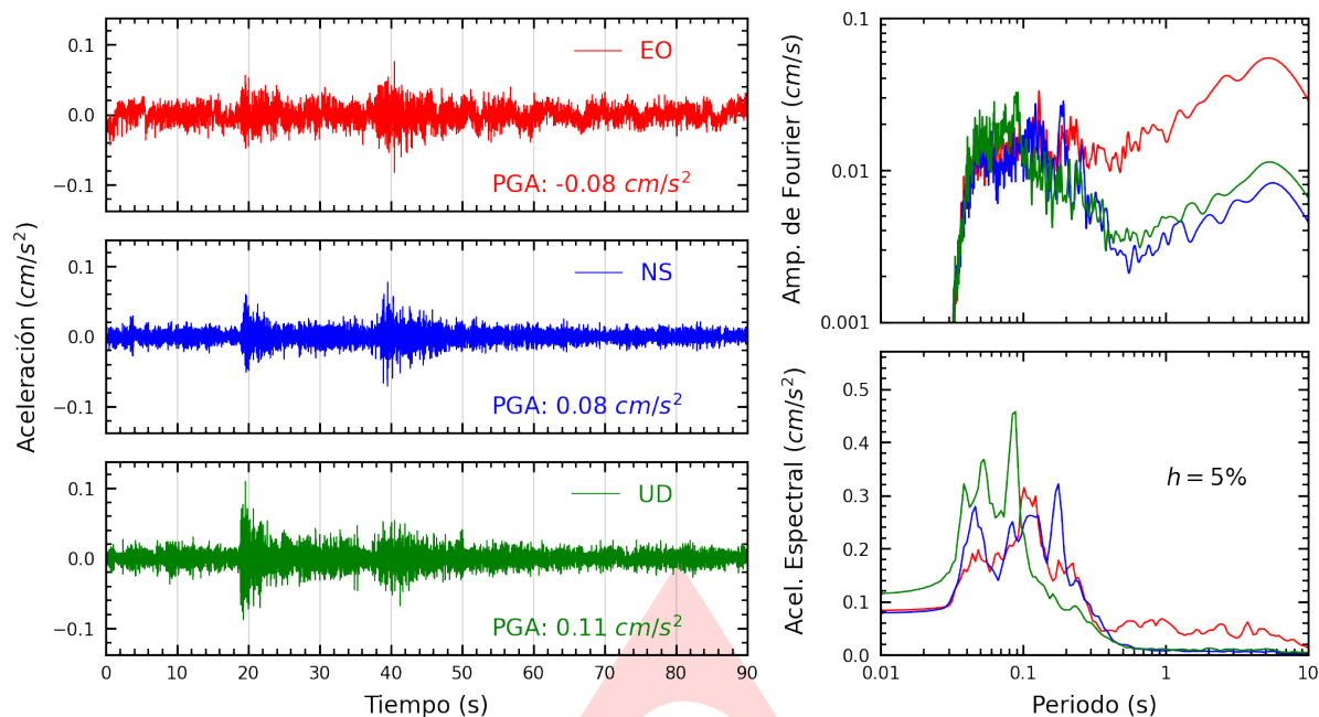
Figura A.1: Registros tiempo-historia, espectros de Fourier y de respuesta en las direcciones EO, NS y vertical de la estación UJBG3. Sismo de Calana, Tacna - Tacna del 2025-01-25, 04:14:52 (Hora local)
