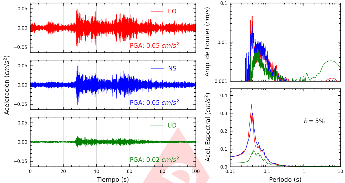
Figura A.3: Registros tiempo-historia, espectros de Fourier y de respuesta en las direcciones EO, NS y vertical de la estación UNAM. Sismo de Calana, Tacna - Tacna del 2025-01-25, 04:14:52 (Hora local)
