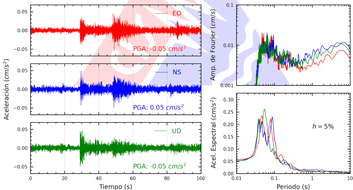
Figura A.2: Registros tiempo-historia, espectros de Fourier y de respuesta en las direcciones EO, NS y vertical de la estación CREY. Sismo de Calana, Tacna - Tacna del 2025-01-25, 04:14:52 (Hora local)
