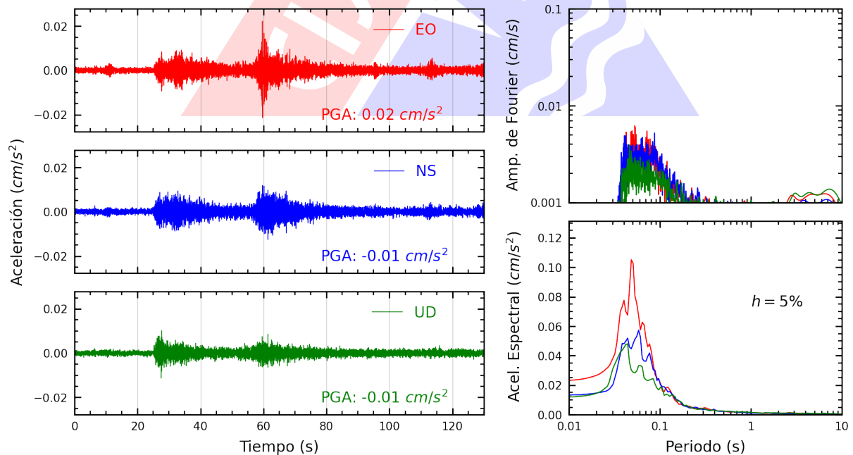
Figura A.4: Registros tiempo-historia, espectros de Fourier y de respuesta en las direcciones EO, NS y vertical de la estación UNSA2. Sismo de Calana, Tacna - Tacna del 2025-01-25, 04:14:52 (Hora local)
