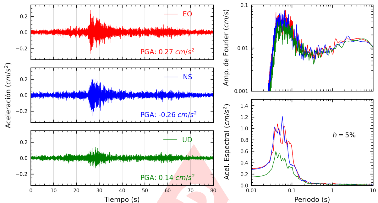
Figura A.9: Registros tiempo-historia, espectros de Fourier y de respuesta en las direcciones EO, NS y vertical de la estación FICPE. Sismo de Chilca, Cañete - Lima del 2025-01-25, 20:54:31 (Hora local)
