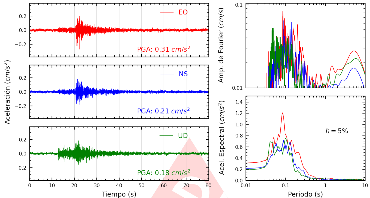
Figura A.7: Registros tiempo-historia, espectros de Fourier y de respuesta en las direcciones EO, NS y vertical de la estación USILP. Sismo de Chilca, Cañete - Lima del 2025-01-25, 20:54:31 (Hora local)
