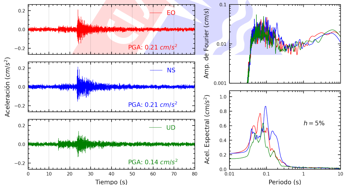
Figura A.10: Registros tiempo-historia, espectros de Fourier y de respuesta en las direcciones EO, NS y vertical de la estación SERVI. Sismo de Chilca, Cañete - Lima del 2025-01-25, 20:54:31 (Hora local)
