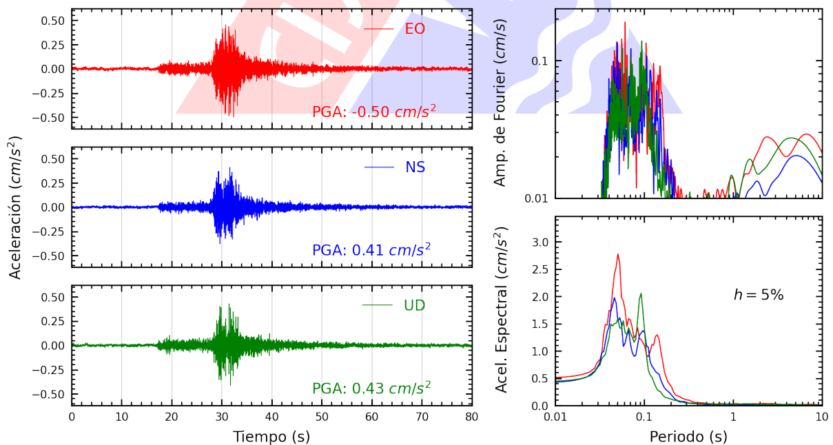
Figura A.4: Registros tiempo-historia, espectros de Fourier y de respuesta en las direcciones EO, NS y vertical de la estación AMORE. Sismo de Chilca, Cañete - Lima del 2025-01-25, 20:54:31 (Hora local)
