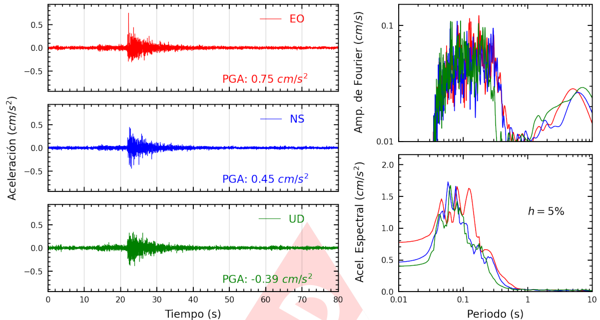
Figura A.3: Registros tiempo-historia, espectros de Fourier y de respuesta en las direcciones EO, NS y vertical de la estación SOVES. Sismo de Chilca, Cañete - Lima del 2025-01-25, 20:54:31 (Hora local)
