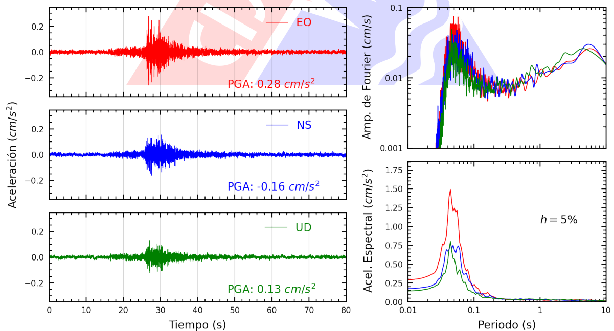
Figura A.8: Registros tiempo-historia, espectros de Fourier y de respuesta en las direcciones EO, NS y vertical de la estación UCSS. Sismo de Chilca, Cañete - Lima del 2025-01-25, 20:54:31 (Hora local)
