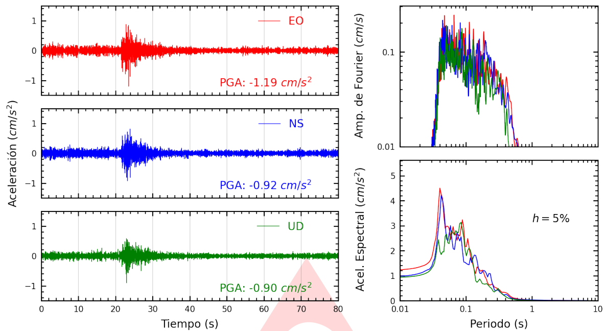
Figura A.1: Registros tiempo-historia, espectros de Fourier y de respuesta en las direcciones EO, NS y vertical de la estación UNTEL. Sismo de Chilca, Cañete - Lima del 2025-01-25, 20:54:31 (Hora local)
