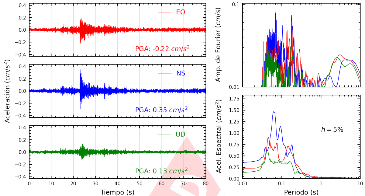
Figura A.5: Registros tiempo-historia, espectros de Fourier y de respuesta en las direcciones EO, NS y vertical de la estación UPCVI. Sismo de Chilca, Cañete - Lima del 2025-01-25, 20:54:31 (Hora local)
