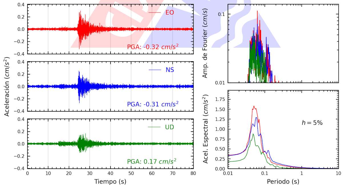
Figura A.6: Registros tiempo-historia, espectros de Fourier y de respuesta en las direcciones EO, NS y vertical de la estación ATARJ. Sismo de Chilca, Cañete - Lima del 2025-01-25, 20:54:31 (Hora local)
