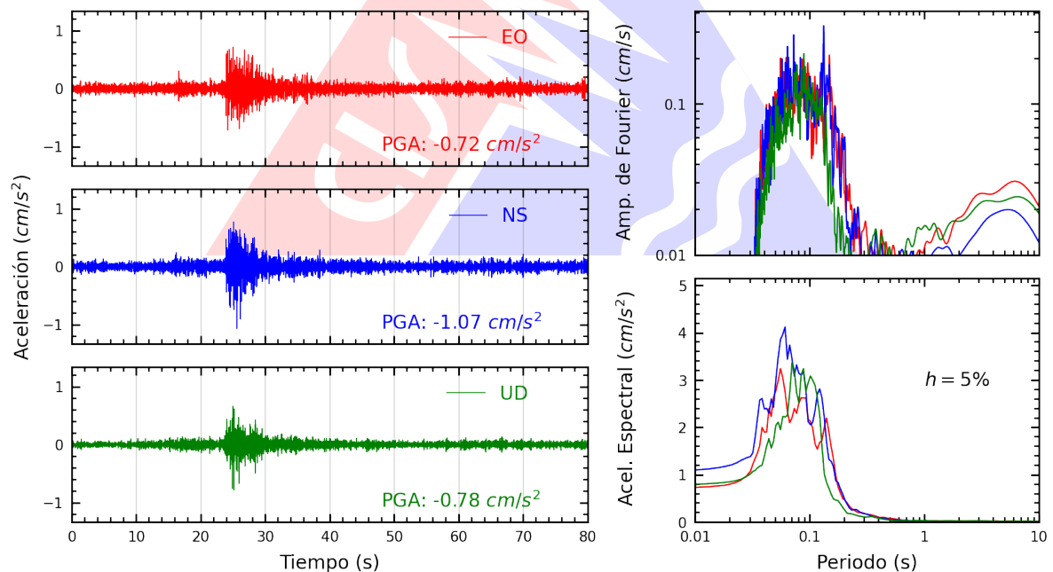
Figura A.2: Registros tiempo-historia, espectros de Fourier y de respuesta en las direcciones EO, NS y vertical de la estación USILM. Sismo de Chilca, Cañete - Lima del 2025-01-25, 20:54:31 (Hora local)
