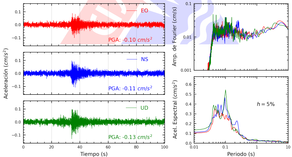
Figura A.30: Registros tiempo-historia, espectros de Fourier y de respuesta en las direcciones EO, NS y vertical de la estación BONDY. Sismo de Chilca, Cañete - Lima del 2025-01-26, 20:20:48 (Hora local)
