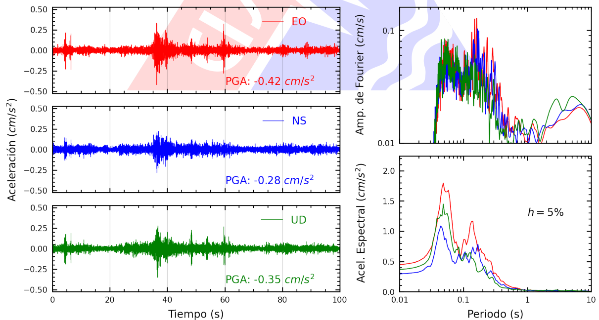
Figura A.16: Registros tiempo-historia, espectros de Fourier y de respuesta en las direcciones EO, NS y vertical de la estación PRADO. Sismo de Chilca, Cañete - Lima del 2025-01-26, 20:20:48 (Hora local)
