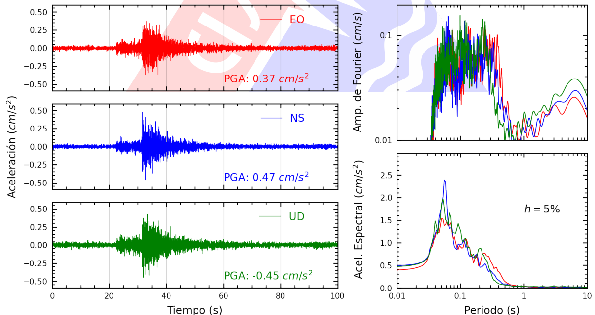
Figura A.10: Registros tiempo-historia, espectros de Fourier y de respuesta en las direcciones EO, NS y vertical de la estación SOVES. Sismo de Chilca, Cañete - Lima del 2025-01-26, 20:20:48 (Hora local)
