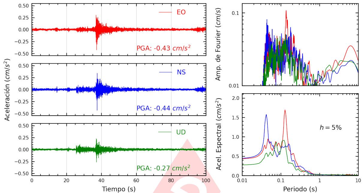
Figura A.13: Registros tiempo-historia, espectros de Fourier y de respuesta en las direcciones EO, NS y vertical de la estación COMAS. Sismo de Chilca, Cañete - Lima del 2025-01-26, 20:20:48 (Hora local)
