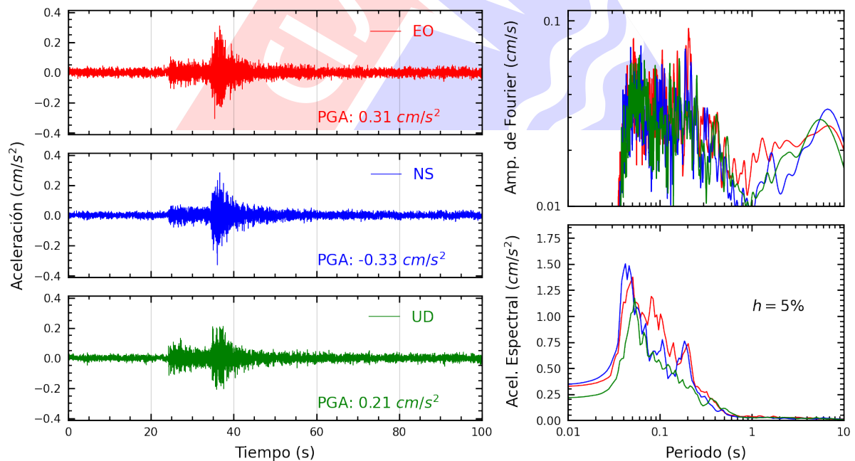
Figura A.20: Registros tiempo-historia, espectros de Fourier y de respuesta en las direcciones EO, NS y vertical de la estación IMCA. Sismo de Chilca, Cañete - Lima del 2025-01-26, 20:20:48 (Hora local)
