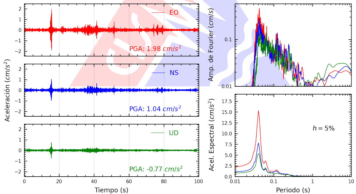
Figura A.2: Registros tiempo-historia, espectros de Fourier y de respuesta en las direcciones EO, NS y vertical de la estación OLIVO. Sismo de Chilca, Cañete - Lima del 2025-01-26, 20:20:48 (Hora local)
