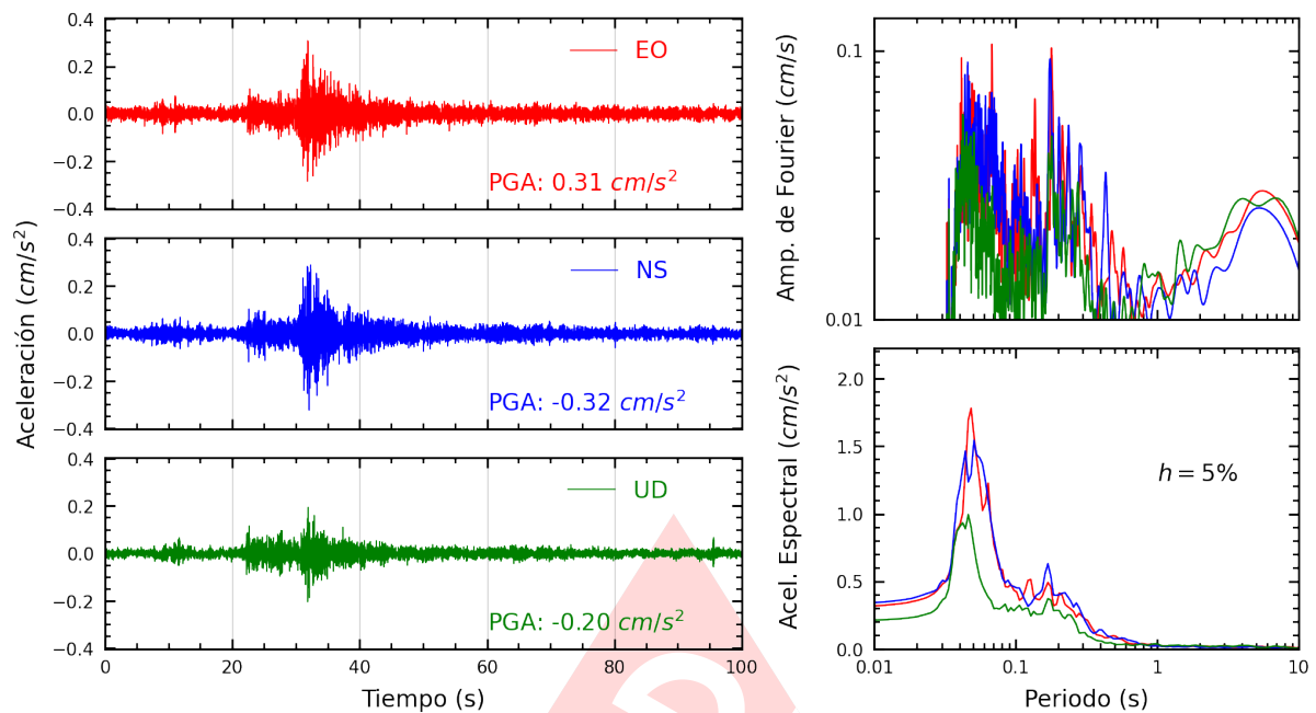
Figura A.23: Registros tiempo-historia, espectros de Fourier y de respuesta en las direcciones EO, NS y vertical de la estación UPCVI. Sismo de Chilca, Cañete - Lima del 2025-01-26, 20:20:48 (Hora local)
