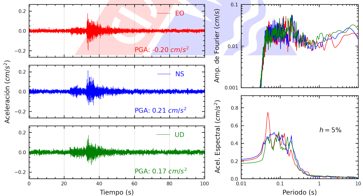
Figura A.28: Registros tiempo-historia, espectros de Fourier y de respuesta en las direcciones EO, NS y vertical de la estación UNFV. Sismo de Chilca, Cañete - Lima del 2025-01-26, 20:20:48 (Hora local)
