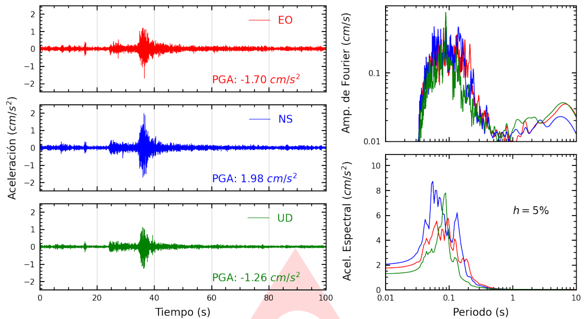
Figura A.1: Registros tiempo-historia, espectros de Fourier y de respuesta en las direcciones EO, NS y vertical de la estación USILM. Sismo de Chilca, Cañete - Lima del 2025-01-26, 20:20:48 (Hora local)
