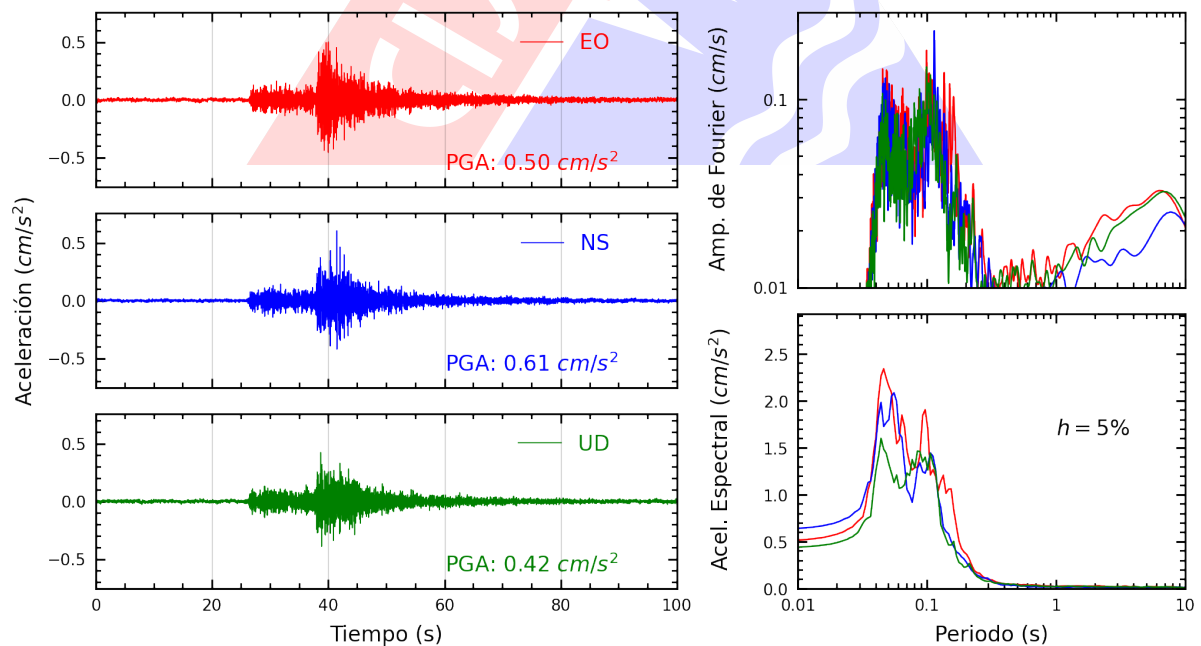
Figura A.8: Registros tiempo-historia, espectros de Fourier y de respuesta en las direcciones EO, NS y vertical de la estación AMORE. Sismo de Chilca, Cañete - Lima del 2025-01-26, 20:20:48 (Hora local)
