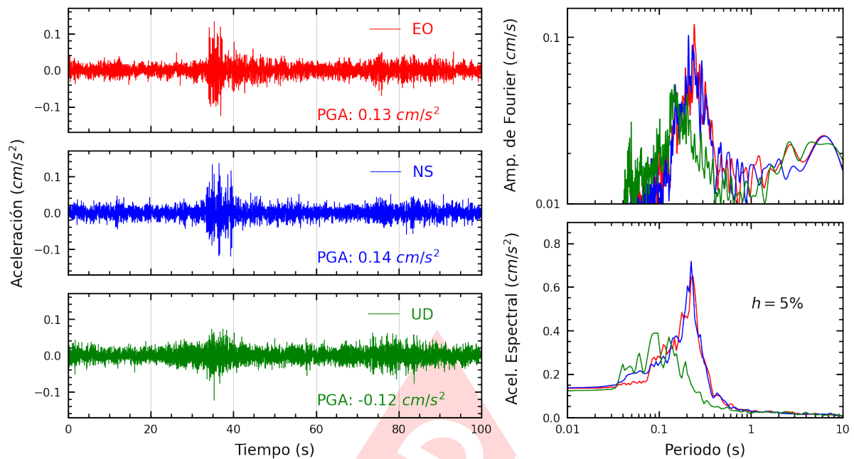
Figura A.29: Registros tiempo-historia, espectros de Fourier y de respuesta en las direcciones EO, NS y vertical de la estación DSMI. Sismo de Chilca, Cañete - Lima del 2025-01-26, 20:20:48 (Hora local)
