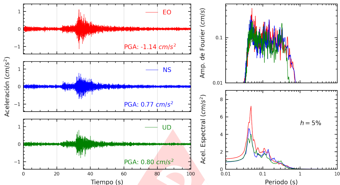
Figura A.3: Registros tiempo-historia, espectros de Fourier y de respuesta en las direcciones EO, NS y vertical de la estación UNTEL. Sismo de Chilca, Cañete - Lima del 2025-01-26, 20:20:48 (Hora local)
