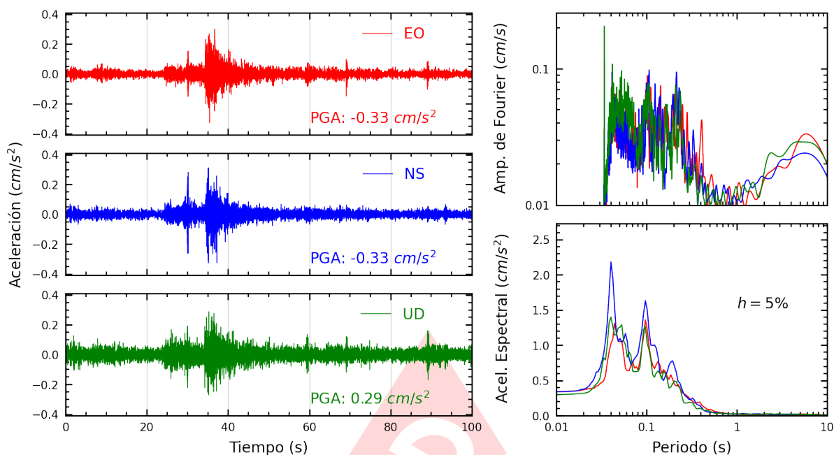
Figura A.21: Registros tiempo-historia, espectros de Fourier y de respuesta en las direcciones EO, NS y vertical de la estación USMP. Sismo de Chilca, Cañete - Lima del 2025-01-26, 20:20:48 (Hora local)
