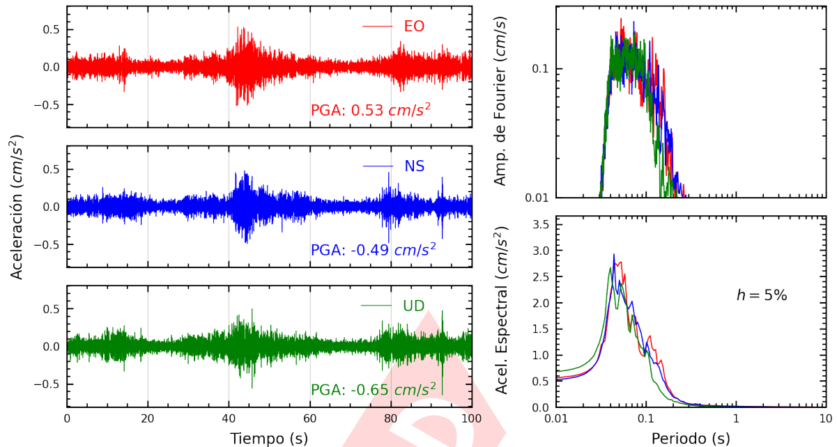
Figura A.7: Registros tiempo-historia, espectros de Fourier y de respuesta en las direcciones EO, NS y vertical de la estación SROS2. Sismo de Chilca, Cañete - Lima del 2025-01-26, 20:20:48 (Hora local)
