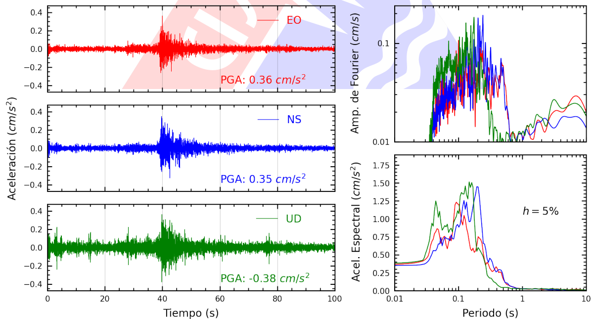
Figura A.18: Registros tiempo-historia, espectros de Fourier y de respuesta en las direcciones EO, NS y vertical de la estación MDPP. Sismo de Chilca, Cañete - Lima del 2025-01-26, 20:20:48 (Hora local)
