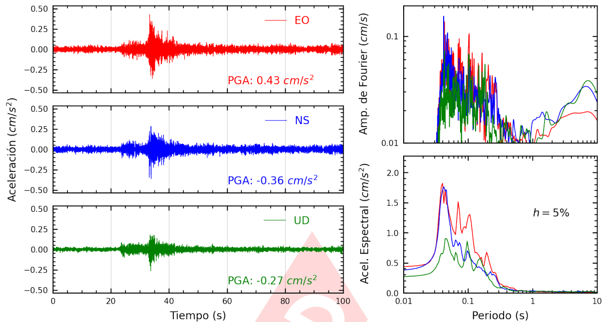
Figura A.15: Registros tiempo-historia, espectros de Fourier y de respuesta en las direcciones EO, NS y vertical de la estación CEPRE. Sismo de Chilca, Cañete - Lima del 2025-01-26, 20:20:48 (Hora local)
