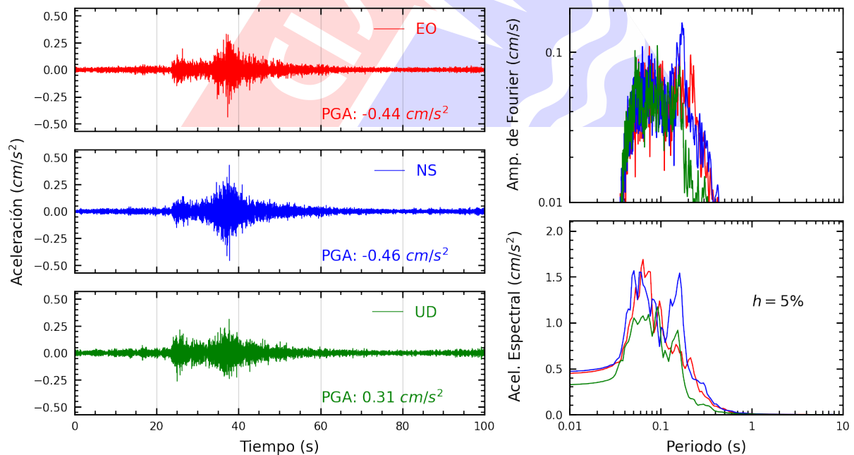
Figura A.12: Registros tiempo-historia, espectros de Fourier y de respuesta en las direcciones EO, NS y vertical de la estación ASIA. Sismo de Chilca, Cañete - Lima del 2025-01-26, 20:20:48 (Hora local)
