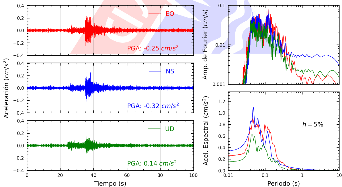
Figura A.22: Registros tiempo-historia, espectros de Fourier y de respuesta en las direcciones EO, NS y vertical de la estación ATARJ. Sismo de Chilca, Cañete - Lima del 2025-01-26, 20:20:48 (Hora local)
