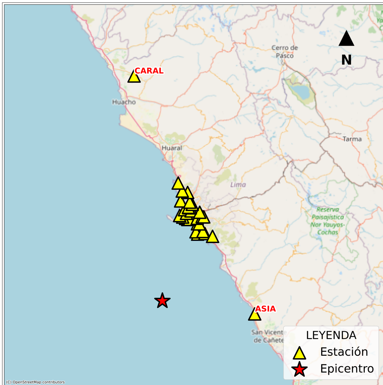
Figura 2: Mapa de ubicación de la(s) estación(es) acelerográfica(s) a nivel nacional correspondiente(s) al Sismo de Chilca, Cañete - Lima del 26 de enero de 2025 a las 20:20:48 (hora local)
