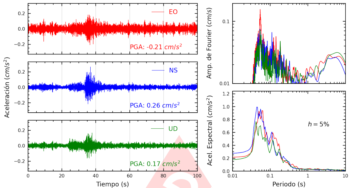
Figura A.25: Registros tiempo-historia, espectros de Fourier y de respuesta en las direcciones EO, NS y vertical de la estación INICT. Sismo de Chilca, Cañete - Lima del 2025-01-26, 20:20:48 (Hora local)
