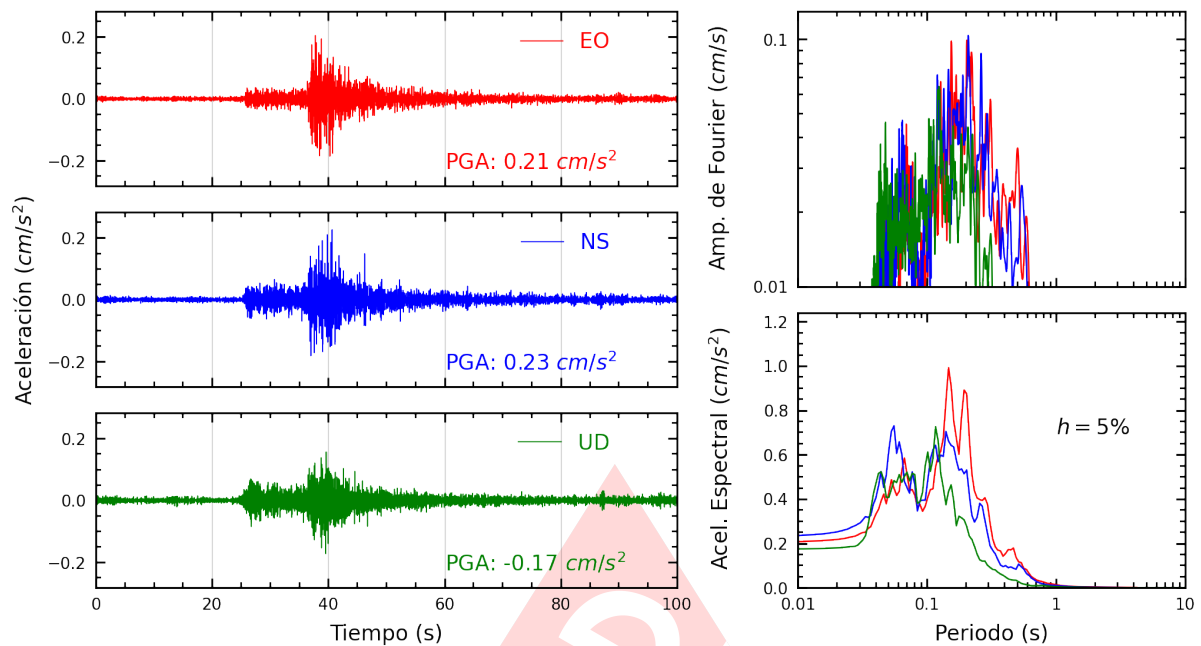
Figura A.27: Registros tiempo-historia, espectros de Fourier y de respuesta en las direcciones EO, NS y vertical de la estación VHAY2. Sismo de Chilca, Cañete - Lima del 2025-01-26, 20:20:48 (Hora local)
