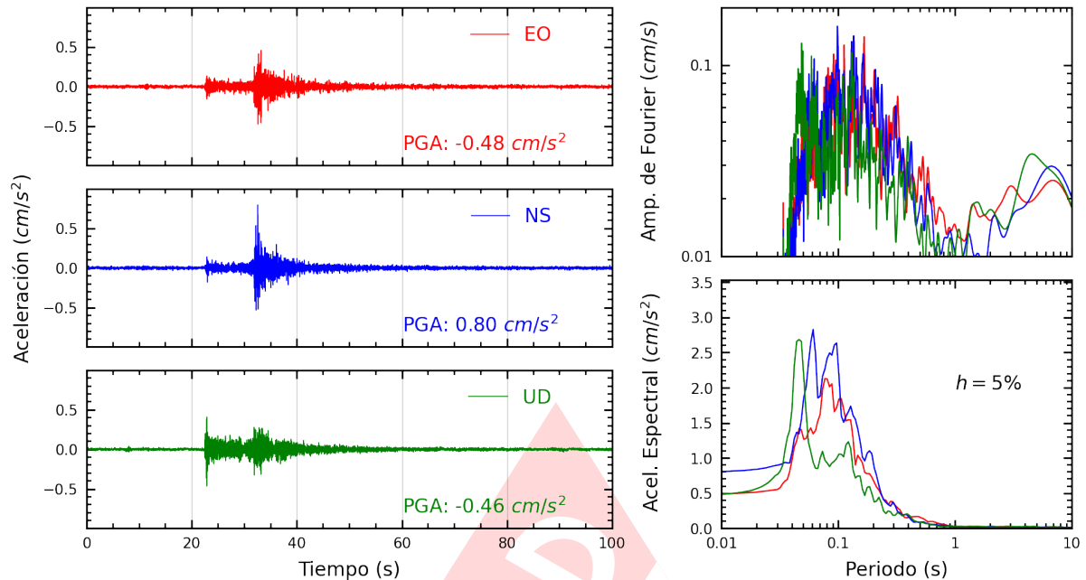
Figura A.5: Registros tiempo-historia, espectros de Fourier y de respuesta en las direcciones EO, NS y vertical de la estación USILP. Sismo de Chilca, Cañete - Lima del 2025-01-26, 20:20:48 (Hora local)
