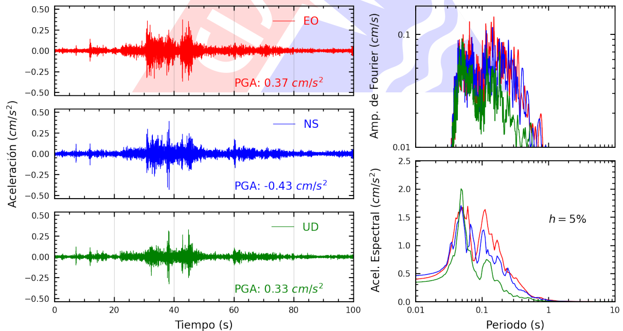
Figura A.14: Registros tiempo-historia, espectros de Fourier y de respuesta en las direcciones EO, NS y vertical de la estación BRISA. Sismo de Chilca, Cañete - Lima del 2025-01-26, 20:20:48 (Hora local)
