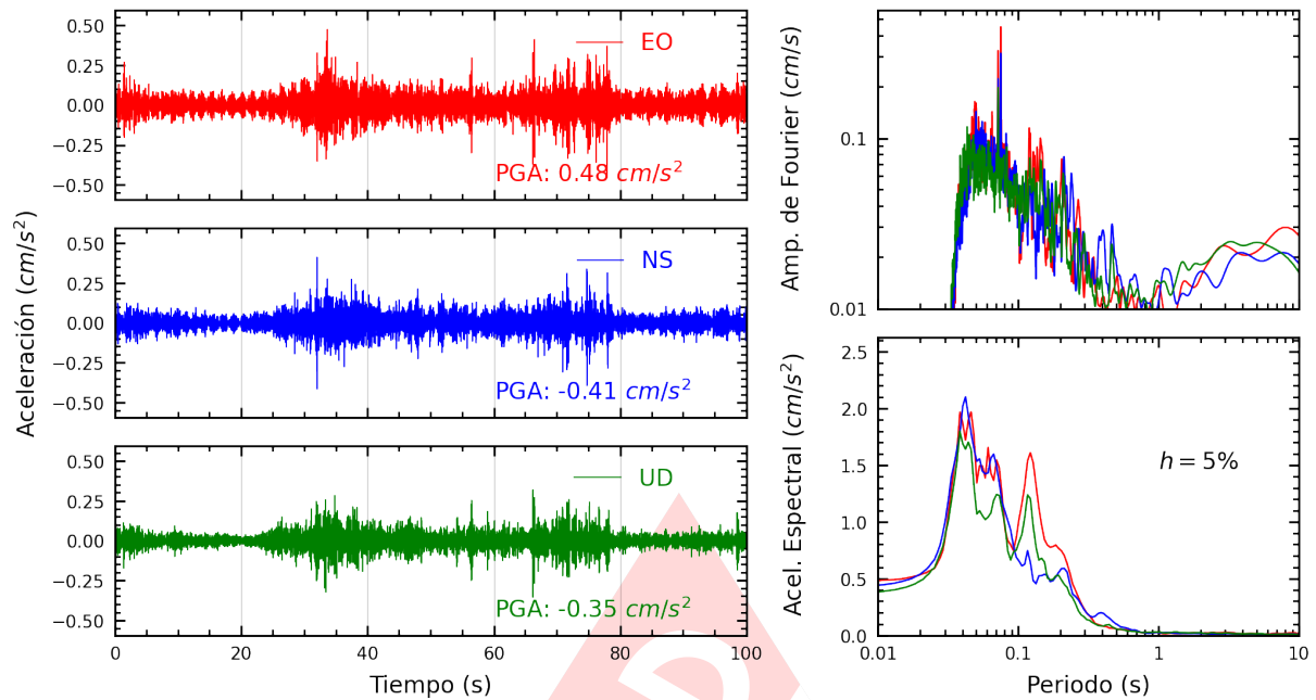
Figura A.9: Registros tiempo-historia, espectros de Fourier y de respuesta en las direcciones EO, NS y vertical de la estación UPCSM. Sismo de Chilca, Cañete - Lima del 2025-01-26, 20:20:48 (Hora local)
