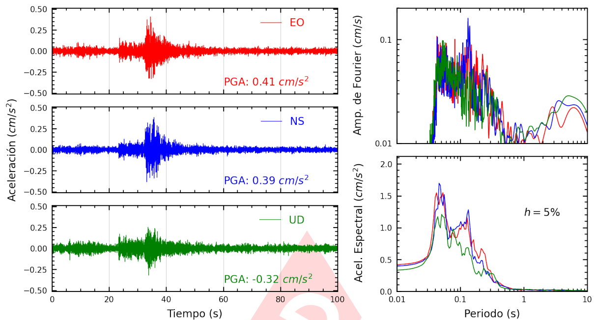
Figura A.17: Registros tiempo-historia, espectros de Fourier y de respuesta en las direcciones EO, NS y vertical de la estación URPPE. Sismo de Chilca, Cañete - Lima del 2025-01-26, 20:20:48 (Hora local)
