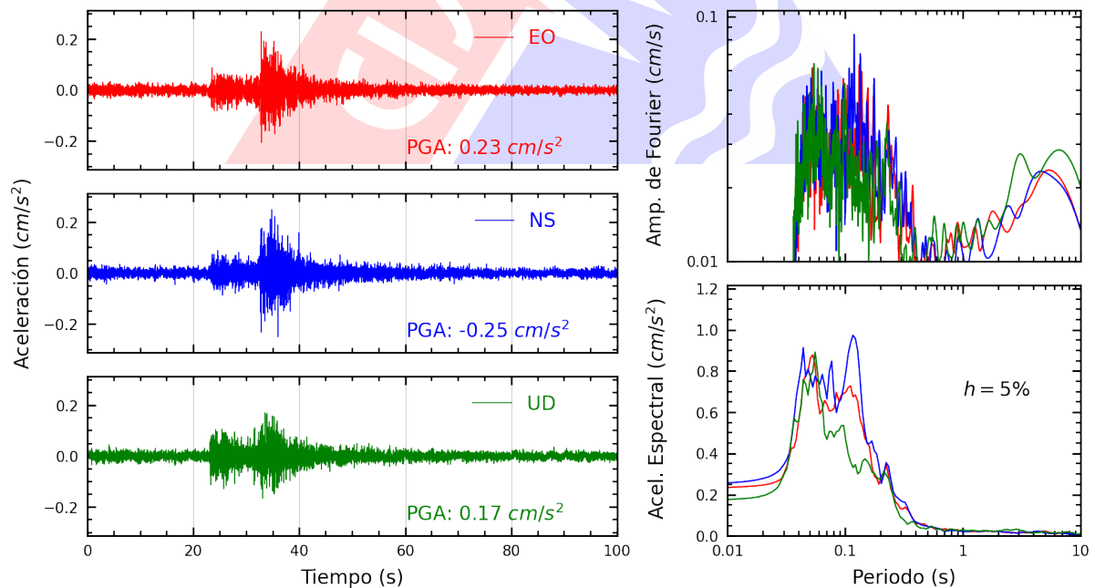
Figura A.26: Registros tiempo-historia, espectros de Fourier y de respuesta en las direcciones EO, NS y vertical de la estación SERVI. Sismo de Chilca, Cañete - Lima del 2025-01-26, 20:20:48 (Hora local)
