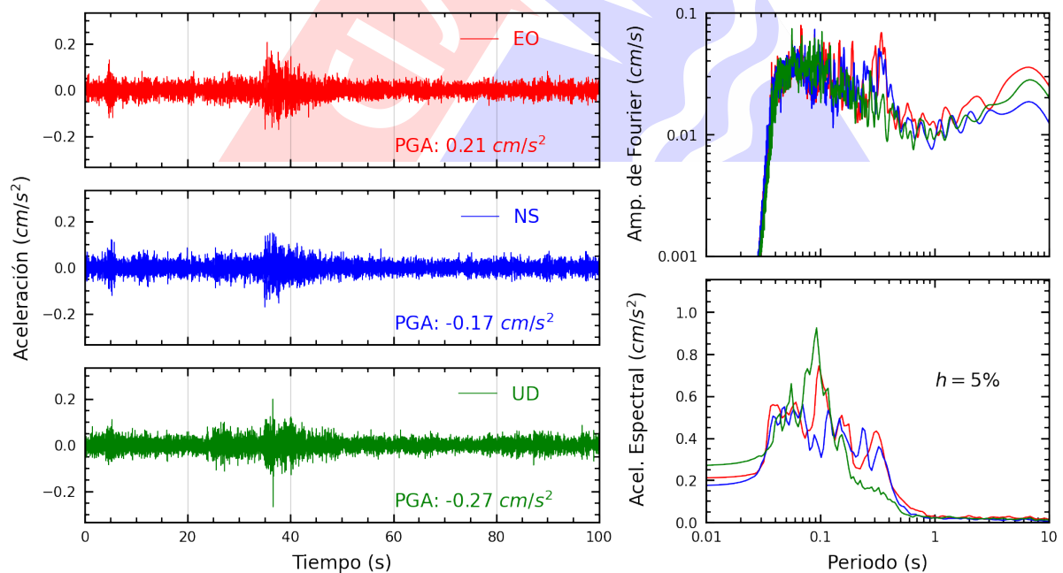
Figura A.24: Registros tiempo-historia, espectros de Fourier y de respuesta en las direcciones EO, NS y vertical de la estación MADRE. Sismo de Chilca, Cañete - Lima del 2025-01-26, 20:20:48 (Hora local)
