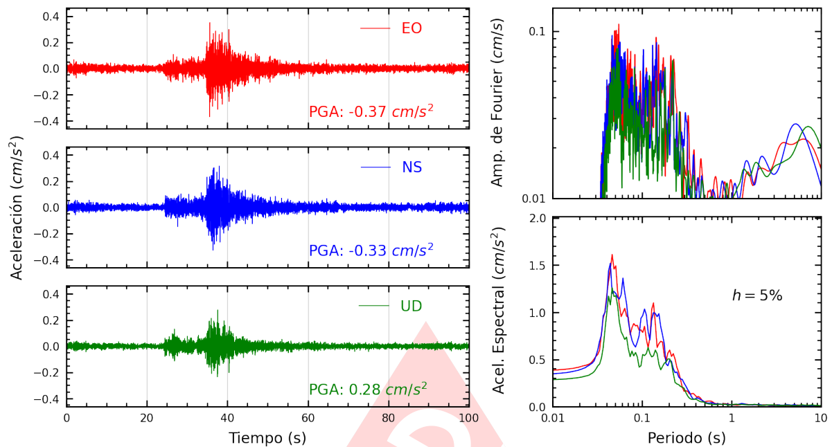
Figura A.19: Registros tiempo-historia, espectros de Fourier y de respuesta en las direcciones EO, NS y vertical de la estación FICPE. Sismo de Chilca, Cañete - Lima del 2025-01-26, 20:20:48 (Hora local)
