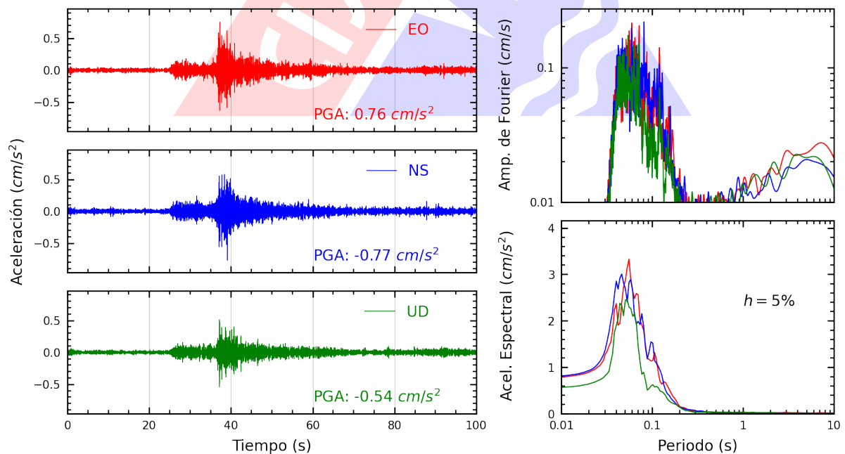
Figura A.6: Registros tiempo-historia, espectros de Fourier y de respuesta en las direcciones EO, NS y vertical de la estación JOSEO. Sismo de Chilca, Cañete - Lima del 2025-01-26, 20:20:48 (Hora local)
