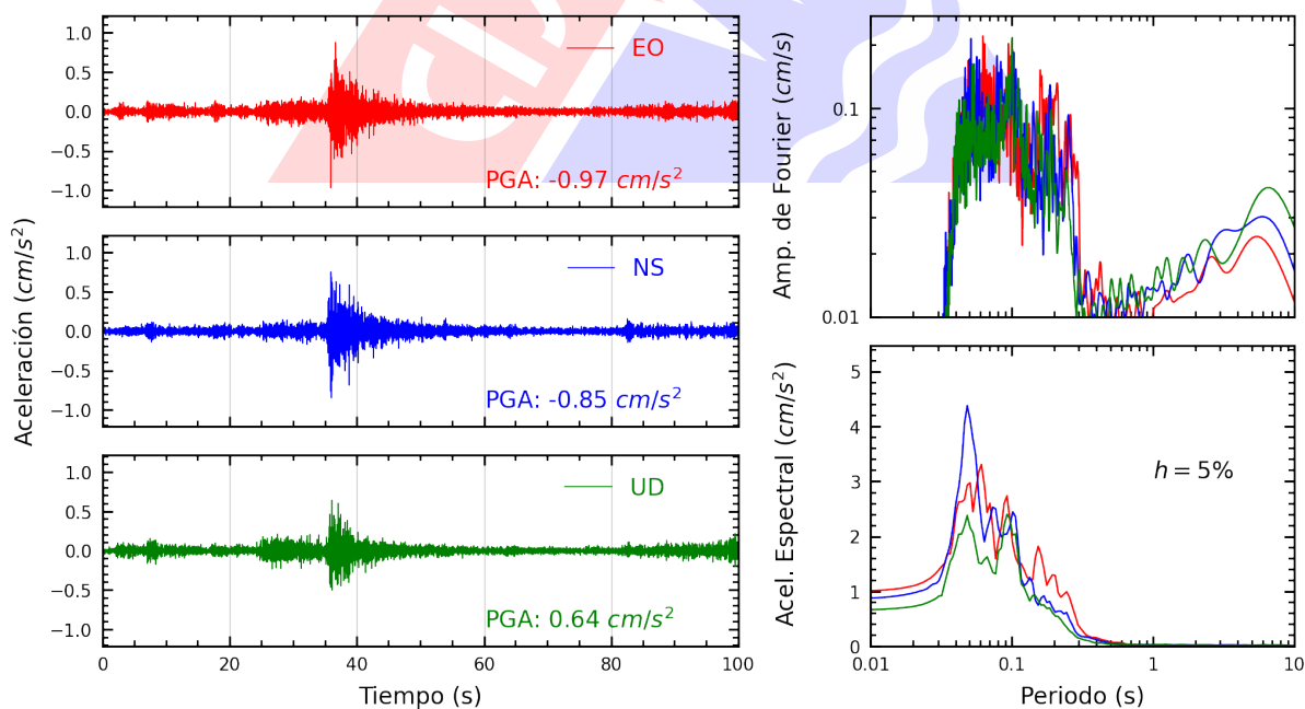
Figura A.4: Registros tiempo-historia, espectros de Fourier y de respuesta en las direcciones EO, NS y vertical de la estación INDEP. Sismo de Chilca, Cañete - Lima del 2025-01-26, 20:20:48 (Hora local)
