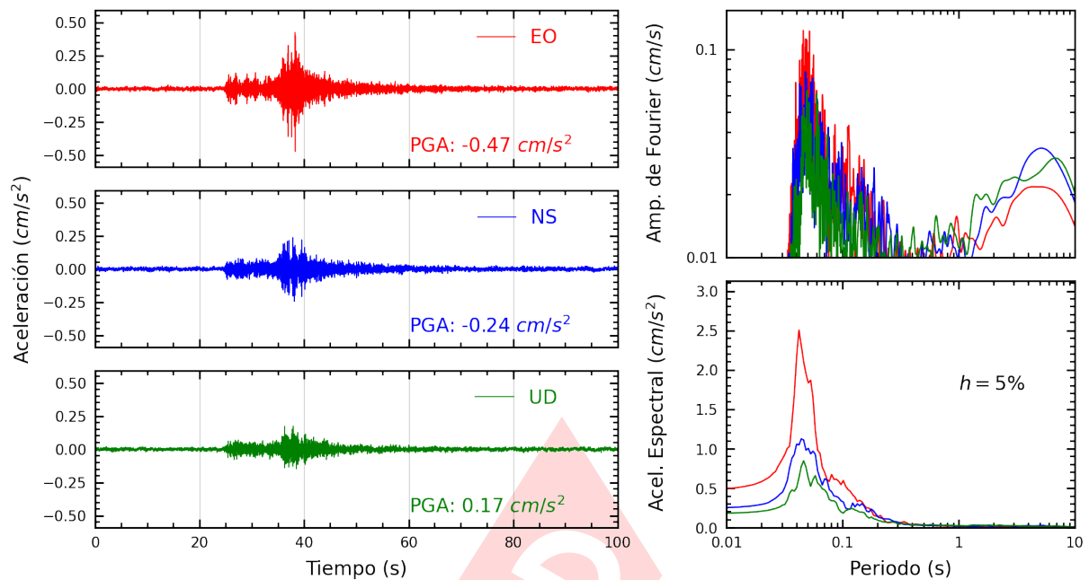
Figura A.11: Registros tiempo-historia, espectros de Fourier y de respuesta en las direcciones EO, NS y vertical de la estación UCSS. Sismo de Chilca, Cañete - Lima del 2025-01-26, 20:20:48 (Hora local)
