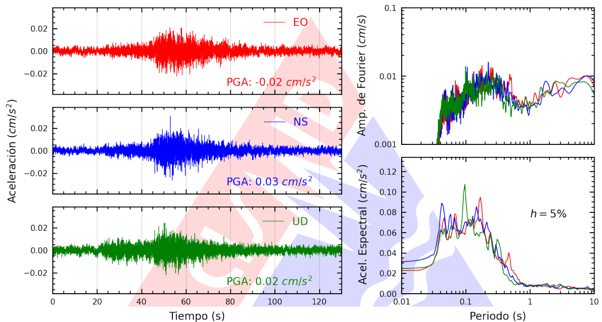
Figura A.31: Registros tiempo-historia, espectros de Fourier y de respuesta en las direcciones EO, NS y vertical de la estación CARAL. Sismo de Chilca, Cañete - Lima del 2025-01-26, 20:20:48 (Hora local)
