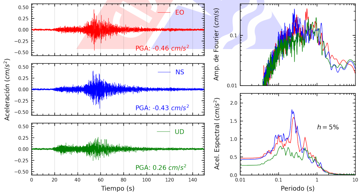
Figura A.20: Registros tiempo-historia, espectros de Fourier y de respuesta en las direcciones EO, NS y vertical de la estación SERVI. Sismo de Pisco, Pisco - Ica del 2025-01-28, 00:09:28 (Hora local)
