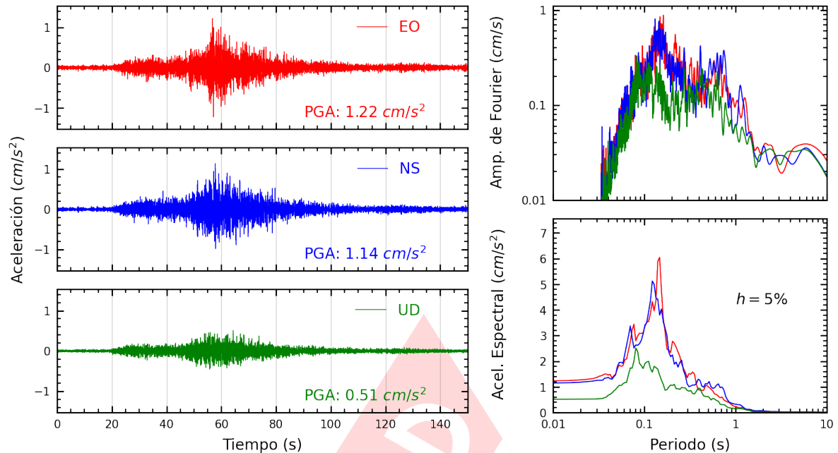
Figura A.5: Registros tiempo-historia, espectros de Fourier y de respuesta en las direcciones EO, NS y vertical de la estación USILM. Sismo de Pisco, Pisco - Ica del 2025-01-28, 00:09:28 (Hora local)
