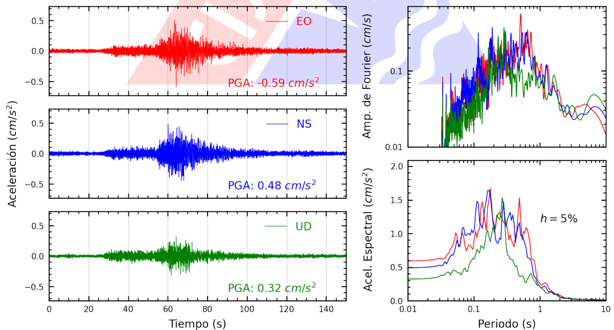
Figura A.14: Registros tiempo-historia, espectros de Fourier y de respuesta en las direcciones EO, NS y vertical de la estación UPCVI. Sismo de Pisco, Pisco - Ica del 2025-01-28, 00:09:28 (Hora local)
