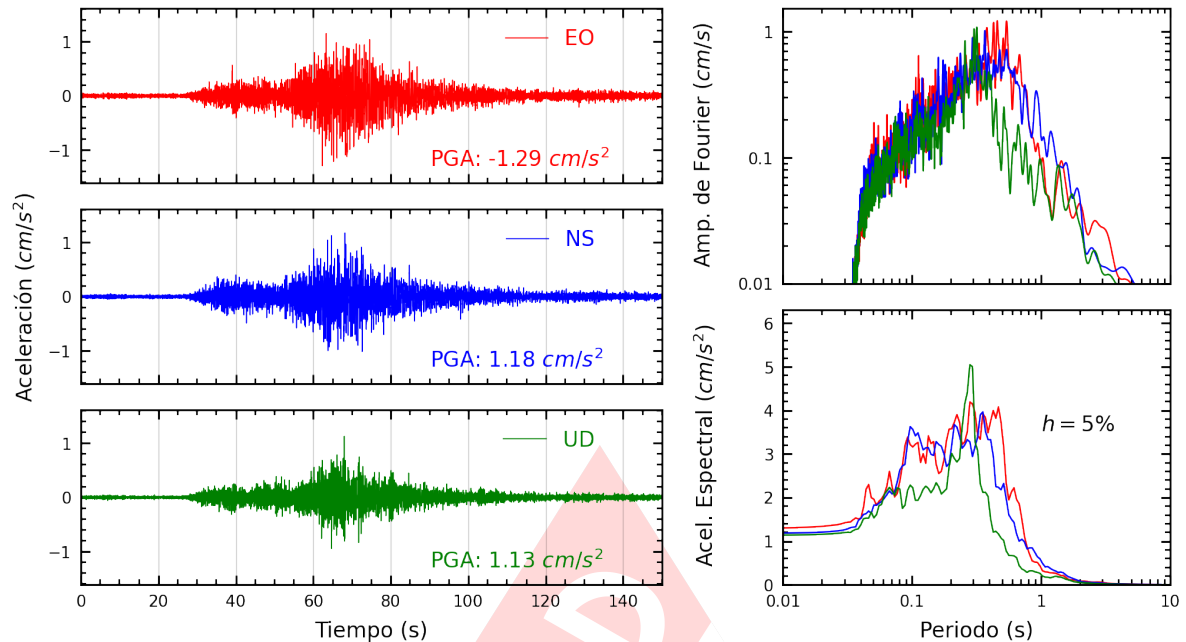
Figura A.3: Registros tiempo-historia, espectros de Fourier y de respuesta en las direcciones EO, NS y vertical de la estación UNTEL. Sismo de Pisco, Pisco - Ica del 2025-01-28, 00:09:28 (Hora local)
