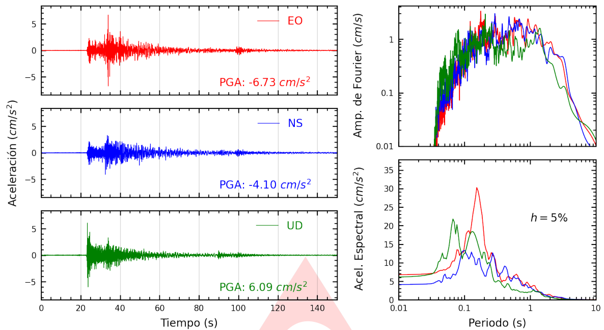
Figura A.1: Registros tiempo-historia, espectros de Fourier y de respuesta en las direcciones EO, NS y vertical de la estación UNICA. Sismo de Pisco, Pisco - Ica del 2025-01-28, 00:09:28 (Hora local)
