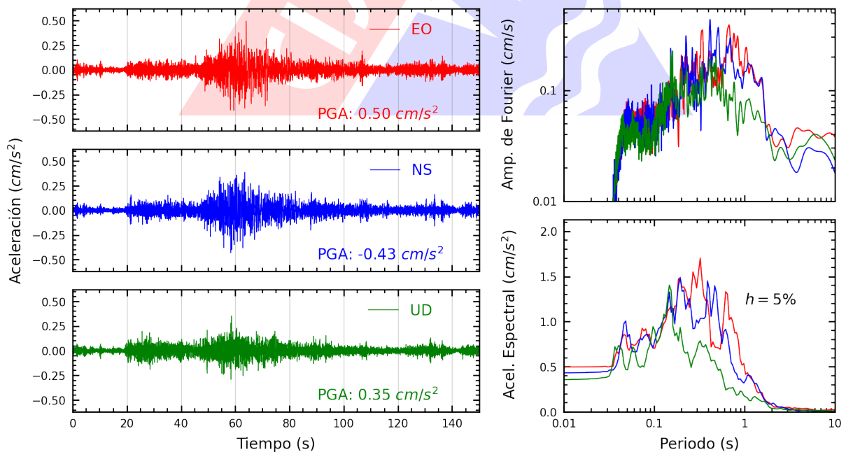
Figura A.18: Registros tiempo-historia, espectros de Fourier y de respuesta en las direcciones EO, NS y vertical de la estación UPCSM. Sismo de Pisco, Pisco - Ica del 2025-01-28, 00:09:28 (Hora local)
