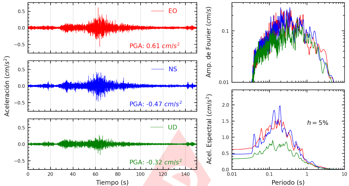
Figura A.13: Registros tiempo-historia, espectros de Fourier y de respuesta en las direcciones EO, NS y vertical de la estación PACHA. Sismo de Pisco, Pisco - Ica del 2025-01-28, 00:09:28 (Hora local)
