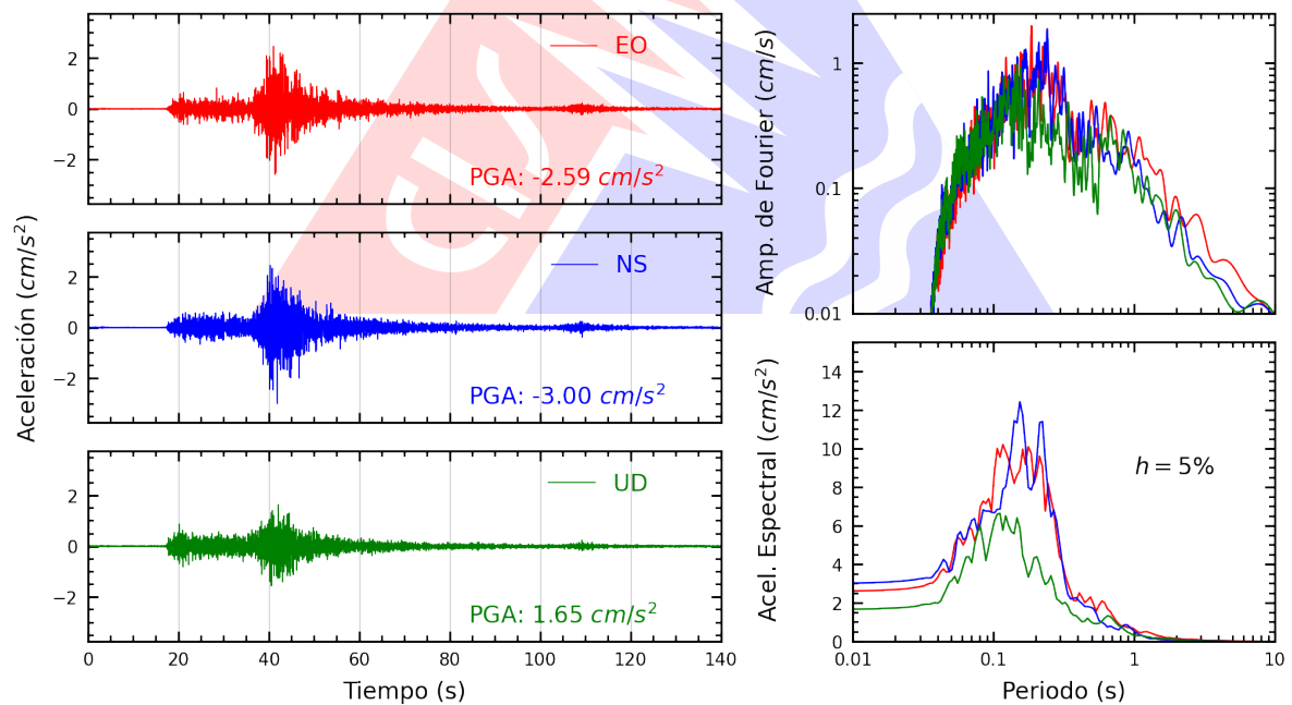
Figura A.2: Registros tiempo-historia, espectros de Fourier y de respuesta en las direcciones EO, NS y vertical de la estación ASIA. Sismo de Pisco, Pisco - Ica del 2025-01-28, 00:09:28 (Hora local)
