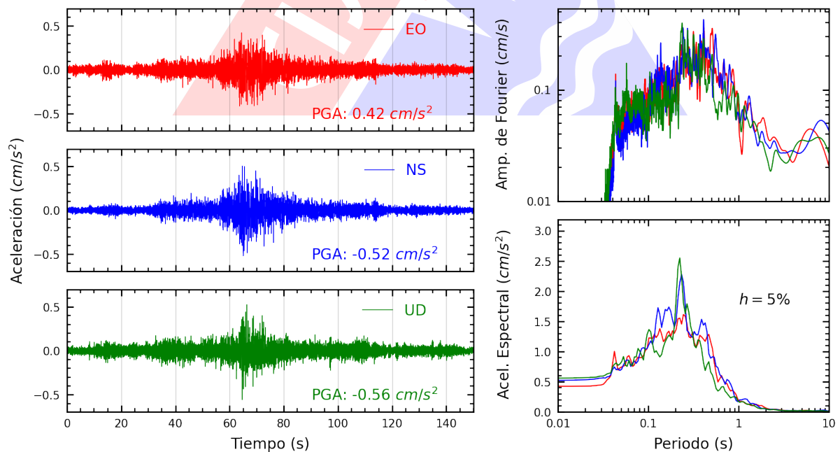
Figura A.16: Registros tiempo-historia, espectros de Fourier y de respuesta en las direcciones EO, NS y vertical de la estación URPPE. Sismo de Pisco, Pisco - Ica del 2025-01-28, 00:09:28 (Hora local)
