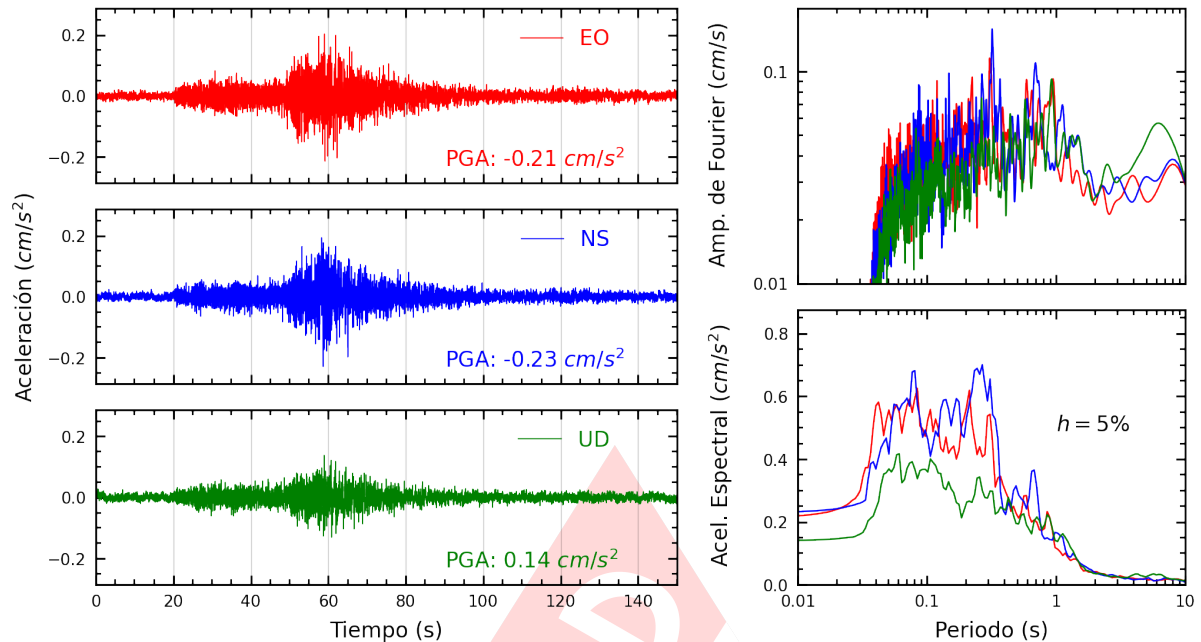
Figura A.31: Registros tiempo-historia, espectros de Fourier y de respuesta en las direcciones EO, NS y vertical de la estación UCSS. Sismo de Pisco, Pisco - Ica del 2025-01-28, 00:09:28 (Hora local)
