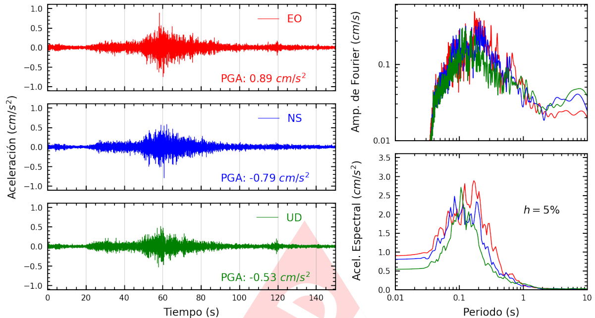
Figura A.9: Registros tiempo-historia, espectros de Fourier y de respuesta en las direcciones EO, NS y vertical de la estación INDEP. Sismo de Pisco, Pisco - Ica del 2025-01-28, 00:09:28 (Hora local)
