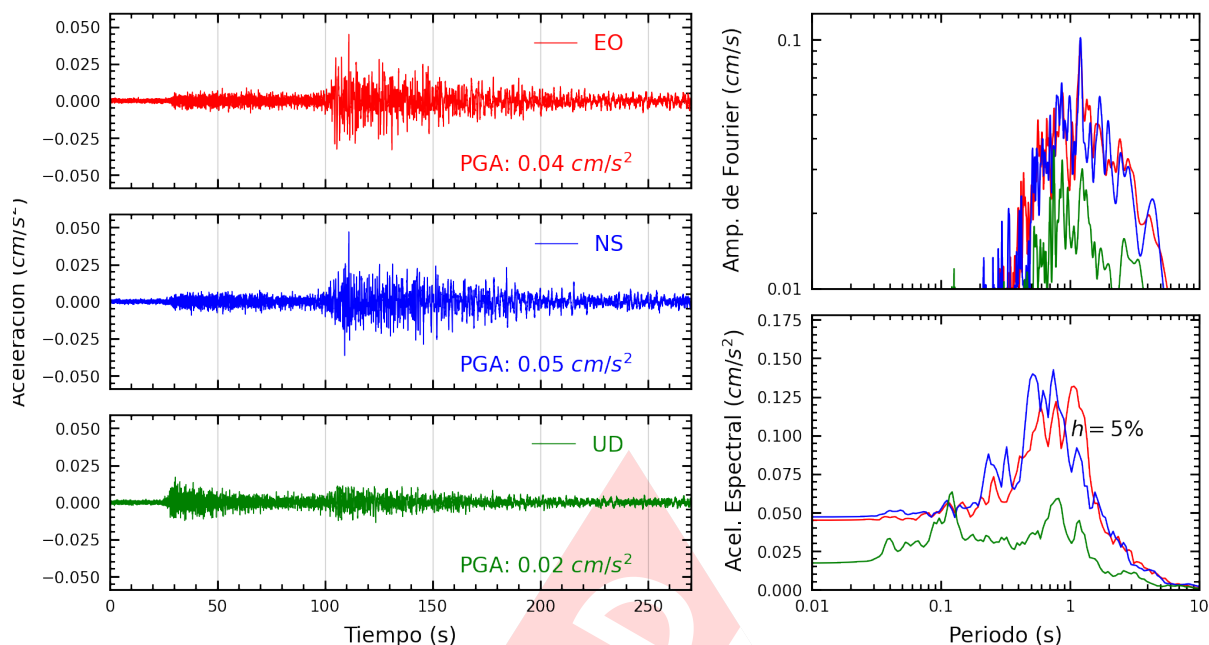
Figura A.33: Registros tiempo-historia, espectros de Fourier y de respuesta en las direcciones EO, NS y vertical de la estación UNIA. Sismo de Pisco, Pisco - Ica del 2025-01-28, 00:09:28 (Hora local)
