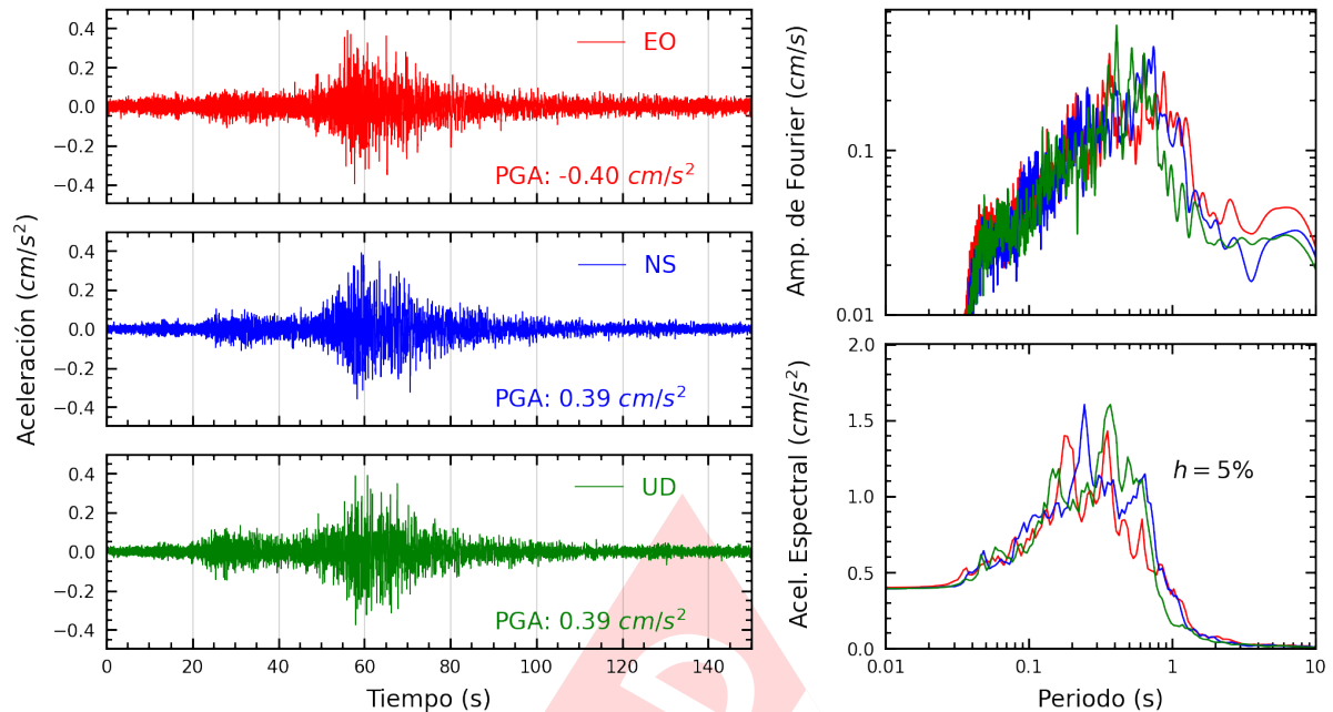
Figura A.23: Registros tiempo-historia, espectros de Fourier y de respuesta en las direcciones EO, NS y vertical de la estación IMCA. Sismo de Pisco, Pisco - Ica del 2025-01-28, 00:09:28 (Hora local)
