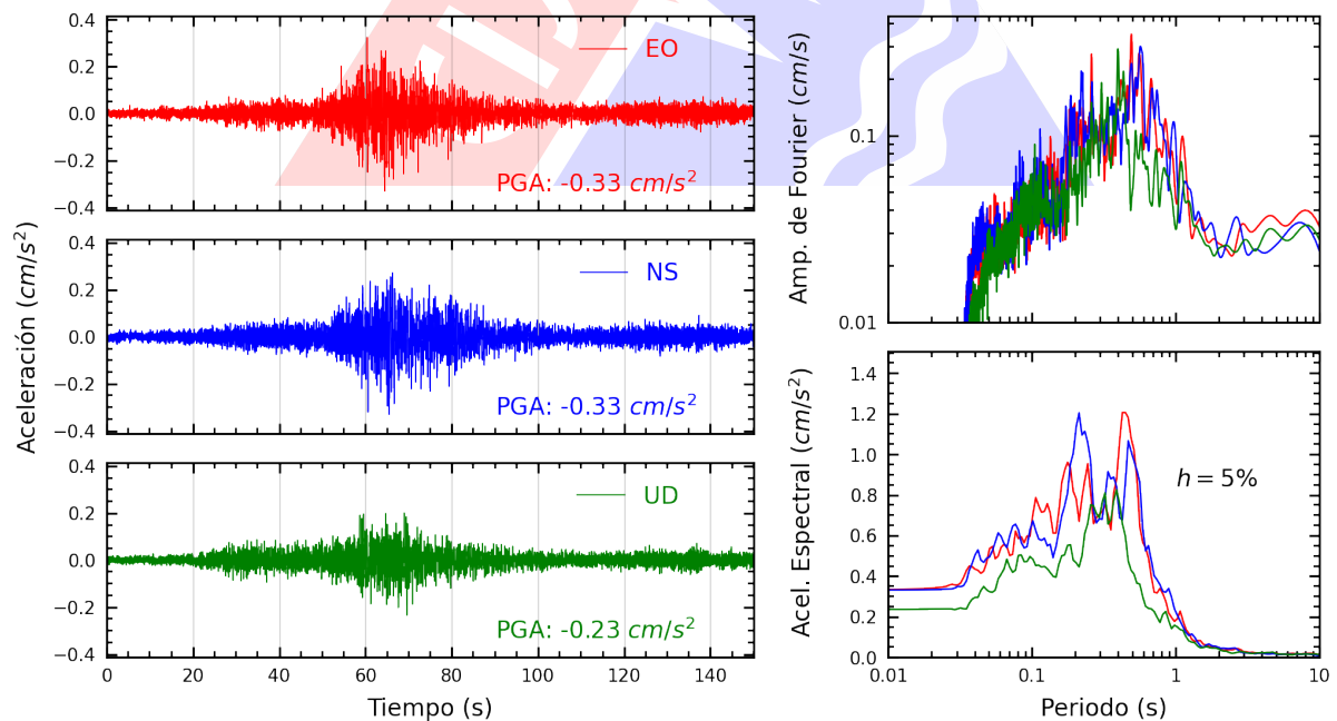
Figura A.28: Registros tiempo-historia, espectros de Fourier y de respuesta en las direcciones EO, NS y vertical de la estación COMAS. Sismo de Pisco, Pisco - Ica del 2025-01-28, 00:09:28 (Hora local)
