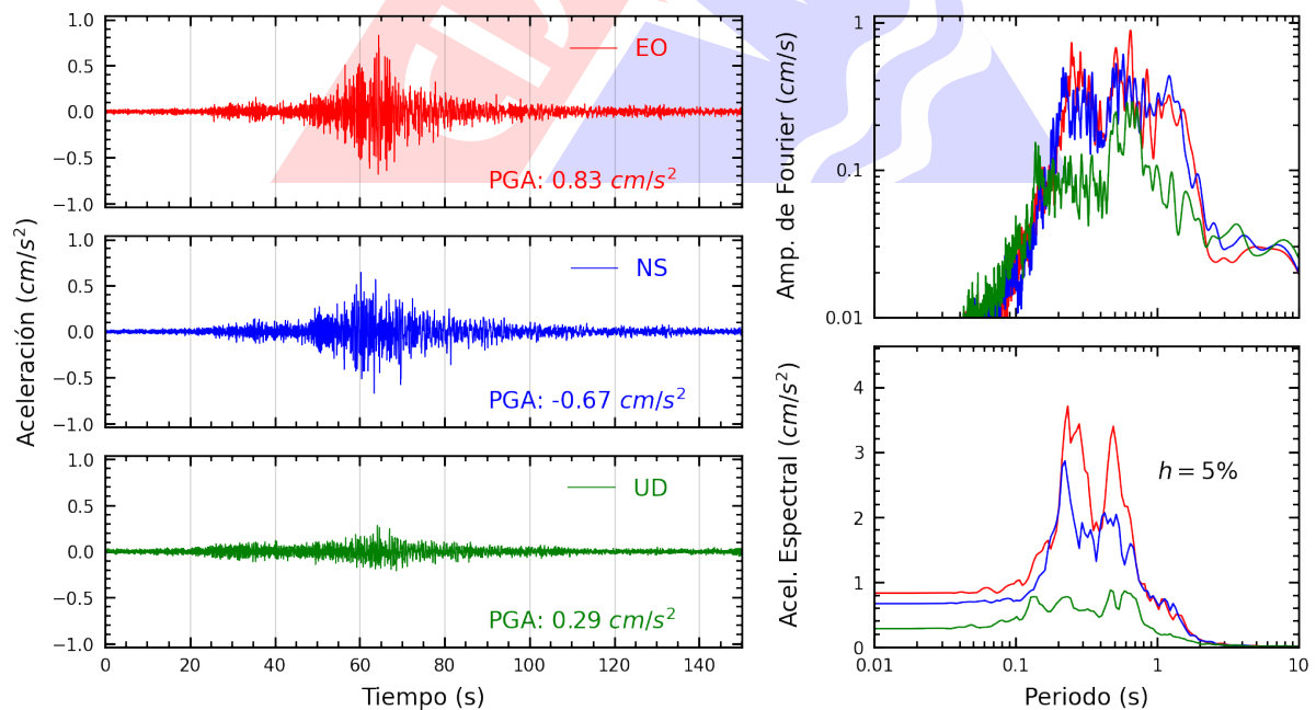
Figura A.10: Registros tiempo-historia, espectros de Fourier y de respuesta en las direcciones EO, NS y vertical de la estación DSMI. Sismo de Pisco, Pisco - Ica del 2025-01-28, 00:09:28 (Hora local)
