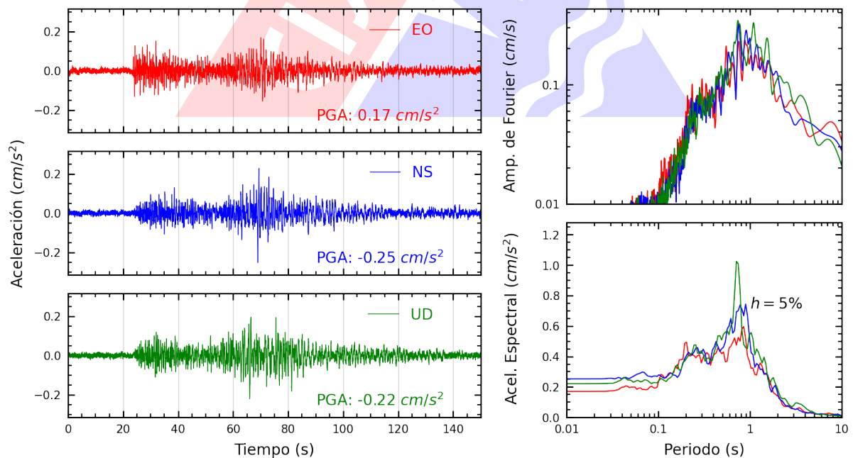
Figura A.30: Registros tiempo-historia, espectros de Fourier y de respuesta en las direcciones EO, NS y vertical de la estación UNSCH. Sismo de Pisco, Pisco - Ica del 2025-01-28, 00:09:28 (Hora local)
