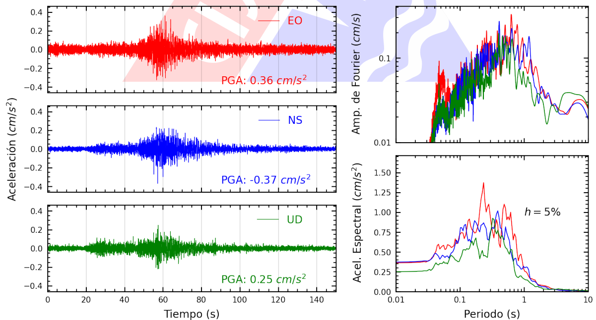
Figura A.26: Registros tiempo-historia, espectros de Fourier y de respuesta en las direcciones EO, NS y vertical de la estación INICT. Sismo de Pisco, Pisco - Ica del 2025-01-28, 00:09:28 (Hora local)
