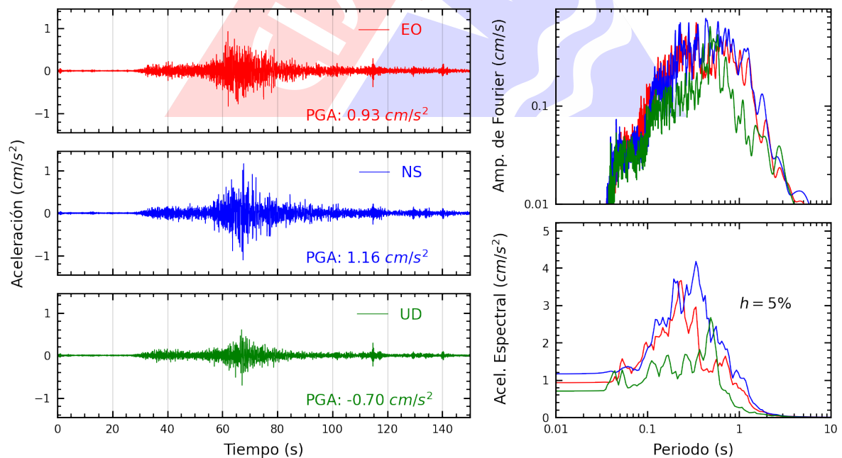
Figura A.6: Registros tiempo-historia, espectros de Fourier y de respuesta en las direcciones EO, NS y vertical de la estación BRISA. Sismo de Pisco, Pisco - Ica del 2025-01-28, 00:09:28 (Hora local)
