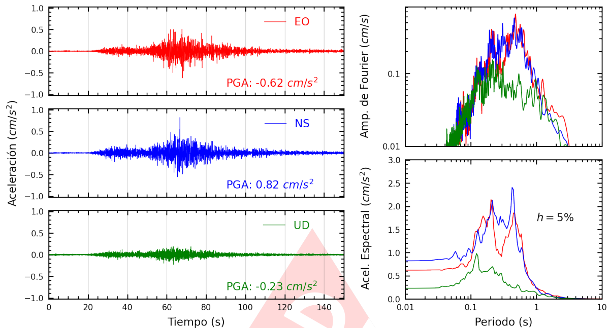
Figura A.11: Registros tiempo-historia, espectros de Fourier y de respuesta en las direcciones EO, NS y vertical de la estación VHAY2. Sismo de Pisco, Pisco - Ica del 2025-01-28, 00:09:28 (Hora local)
