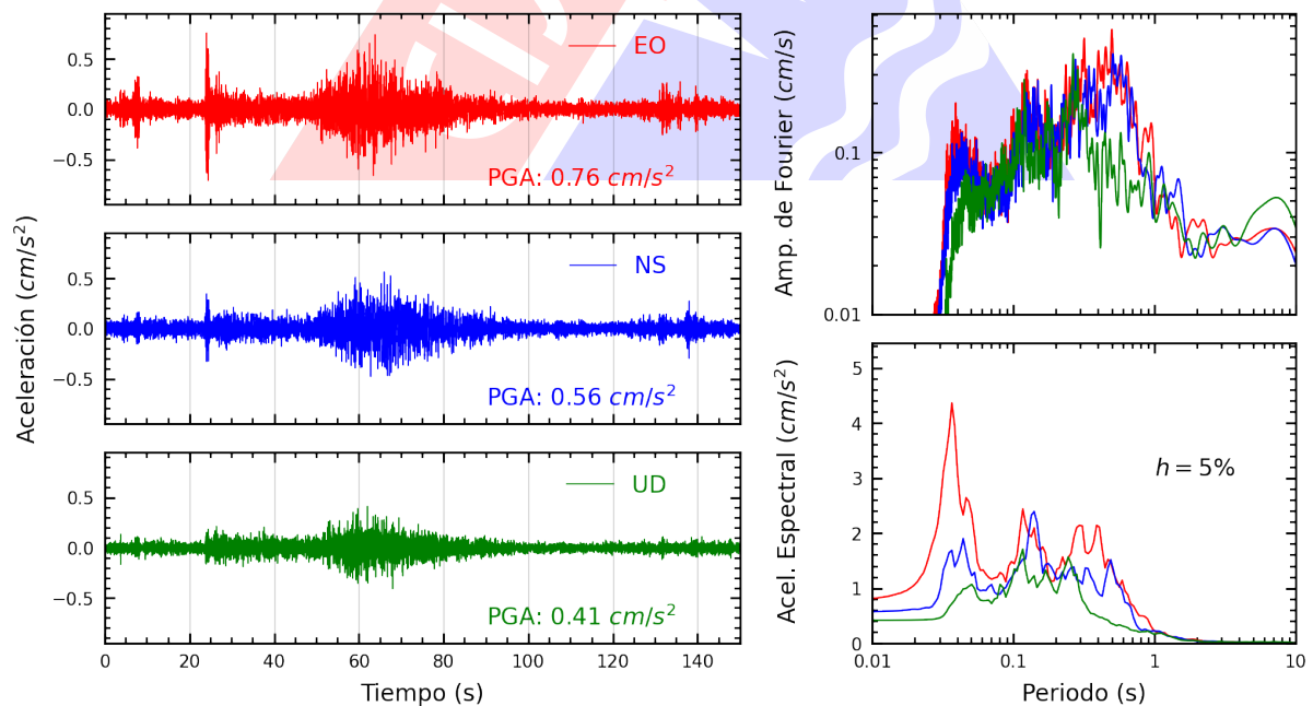
Figura A.12: Registros tiempo-historia, espectros de Fourier y de respuesta en las direcciones EO, NS y vertical de la estación OLIVO. Sismo de Pisco, Pisco - Ica del 2025-01-28, 00:09:28 (Hora local)
