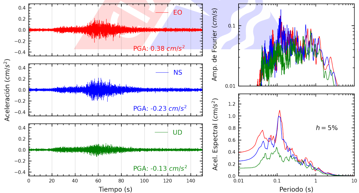
Figura A.24: Registros tiempo-historia, espectros de Fourier y de respuesta en las direcciones EO, NS y vertical de la estación ATARJ. Sismo de Pisco, Pisco - Ica del 2025-01-28, 00:09:28 (Hora local)
