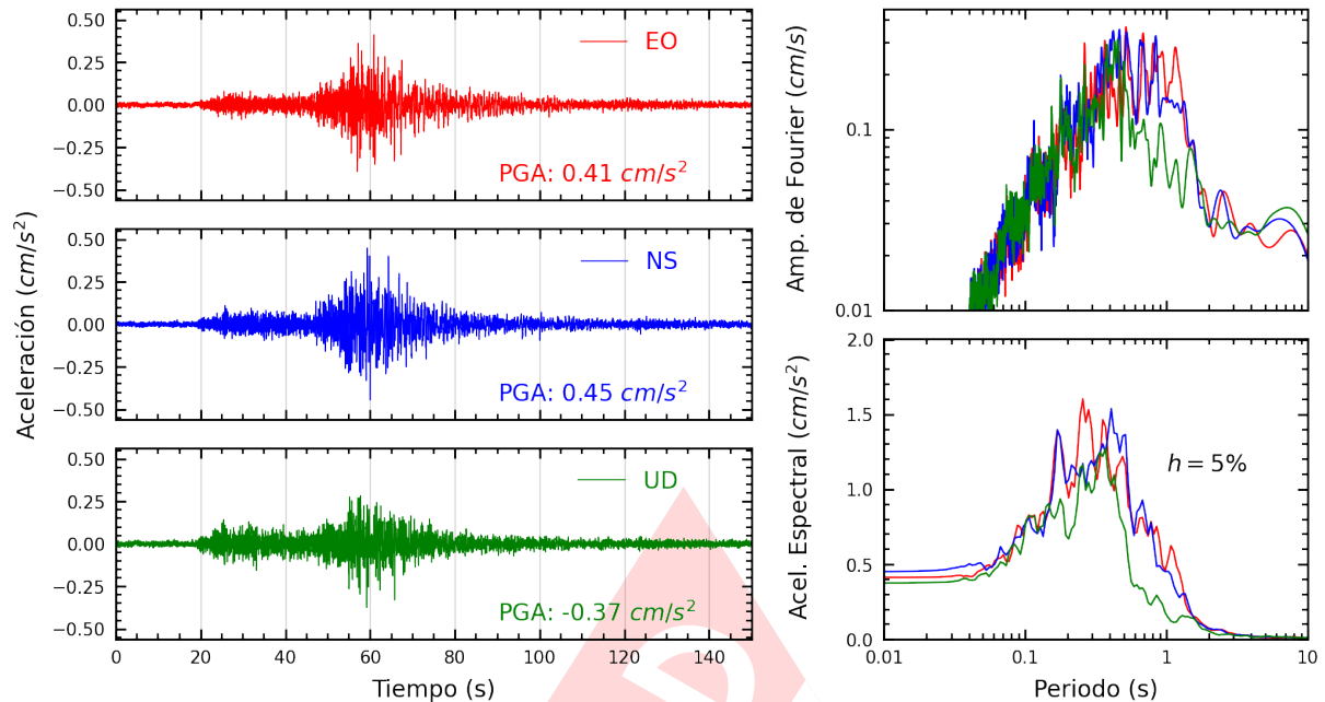
Figura A.21: Registros tiempo-historia, espectros de Fourier y de respuesta en las direcciones EO, NS y vertical de la estación UNFV. Sismo de Pisco, Pisco - Ica del 2025-01-28, 00:09:28 (Hora local)
