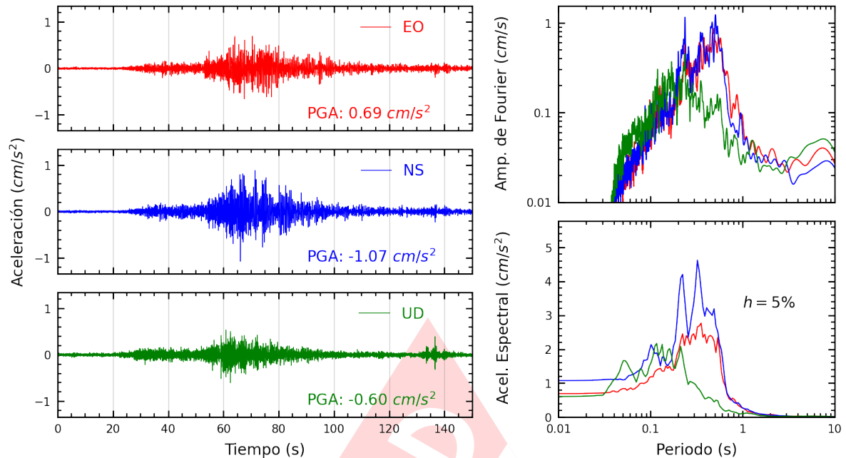
Figura A.7: Registros tiempo-historia, espectros de Fourier y de respuesta en las direcciones EO, NS y vertical de la estación MDPP. Sismo de Pisco, Pisco - Ica del 2025-01-28, 00:09:28 (Hora local)
