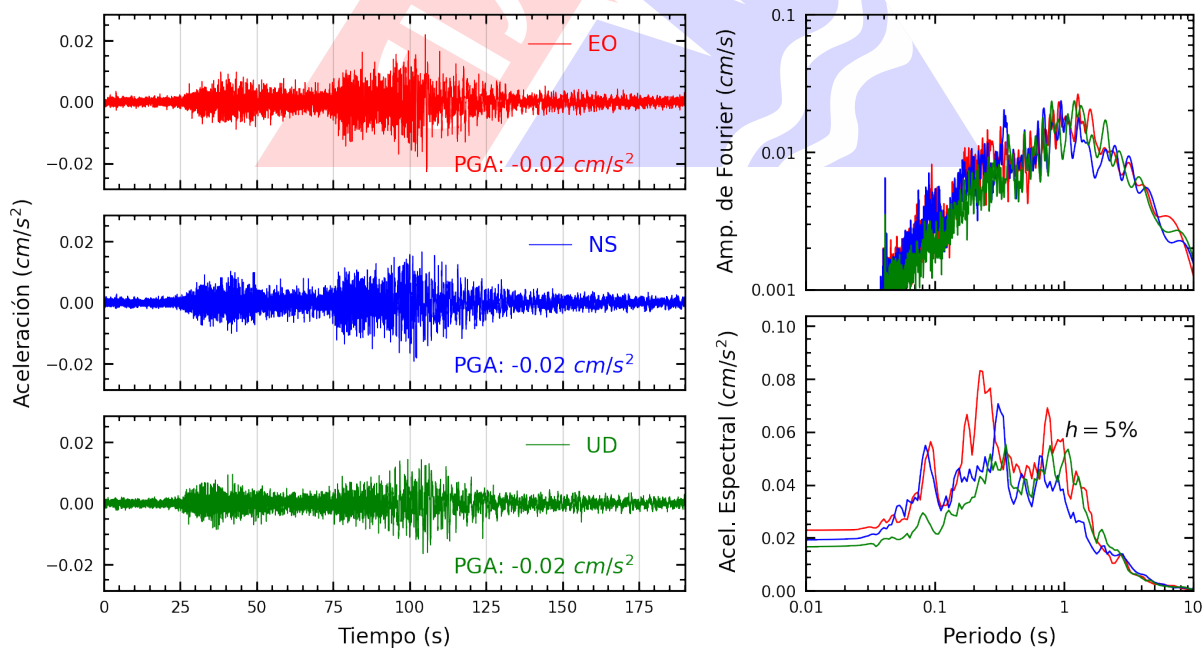
Figura A.34: Registros tiempo-historia, espectros de Fourier y de respuesta en las direcciones EO, NS y vertical de la estación UNSA2. Sismo de Pisco, Pisco - Ica del 2025-01-28, 00:09:28 (Hora local)
