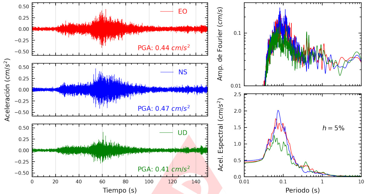
Figura A.19: Registros tiempo-historia, espectros de Fourier y de respuesta en las direcciones EO, NS y vertical de la estación JOSEO. Sismo de Pisco, Pisco - Ica del 2025-01-28, 00:09:28 (Hora local)
