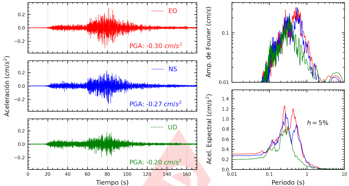
Figura A.29: Registros tiempo-historia, espectros de Fourier y de respuesta en las direcciones EO, NS y vertical de la estación CARAL. Sismo de Pisco, Pisco - Ica del 2025-01-28, 00:09:28 (Hora local)
