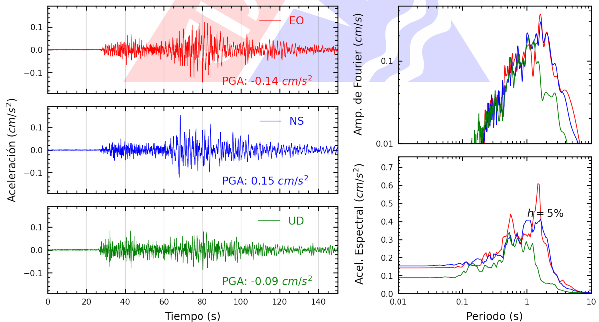
Figura A.32: Registros tiempo-historia, espectros de Fourier y de respuesta en las direcciones EO, NS y vertical de la estación UNCP. Sismo de Pisco, Pisco - Ica del 2025-01-28, 00:09:28 (Hora local)
