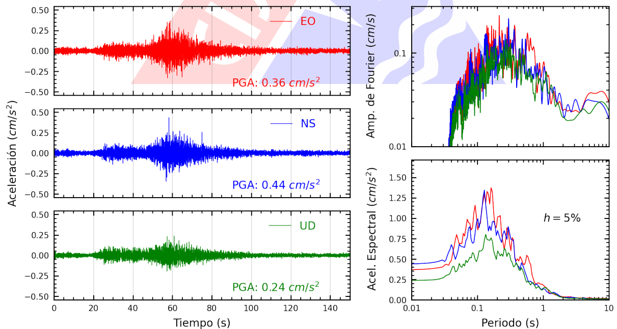
Figura A.22: Registros tiempo-historia, espectros de Fourier y de respuesta en las direcciones EO, NS y vertical de la estación FICPE. Sismo de Pisco, Pisco - Ica del 2025-01-28, 00:09:28 (Hora local)
