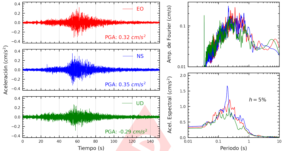
Figura A.27: Registros tiempo-historia, espectros de Fourier y de respuesta en las direcciones EO, NS y vertical de la estación USMP. Sismo de Pisco, Pisco - Ica del 2025-01-28, 00:09:28 (Hora local)
