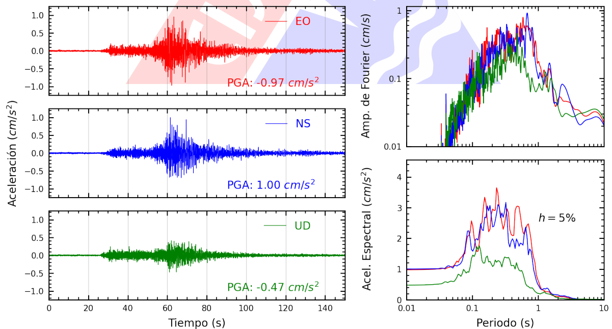
Figura A.8: Registros tiempo-historia, espectros de Fourier y de respuesta en las direcciones EO, NS y vertical de la estación USILP. Sismo de Pisco, Pisco - Ica del 2025-01-28, 00:09:28 (Hora local)
