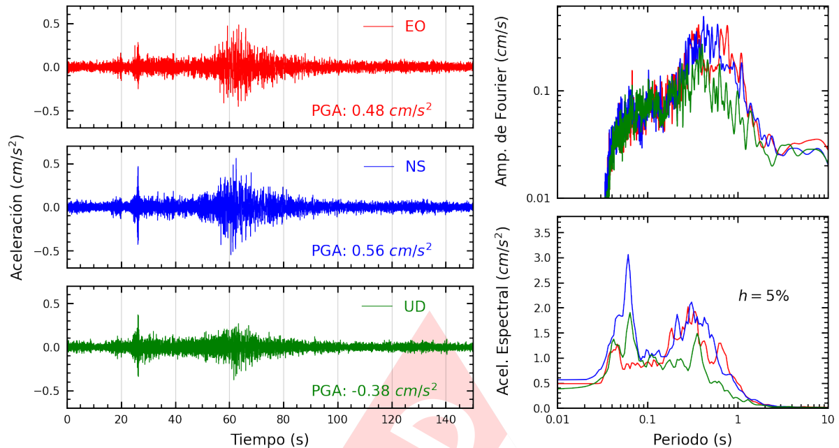
Figura A.15: Registros tiempo-historia, espectros de Fourier y de respuesta en las direcciones EO, NS y vertical de la estación MADRE. Sismo de Pisco, Pisco - Ica del 2025-01-28, 00:09:28 (Hora local)
