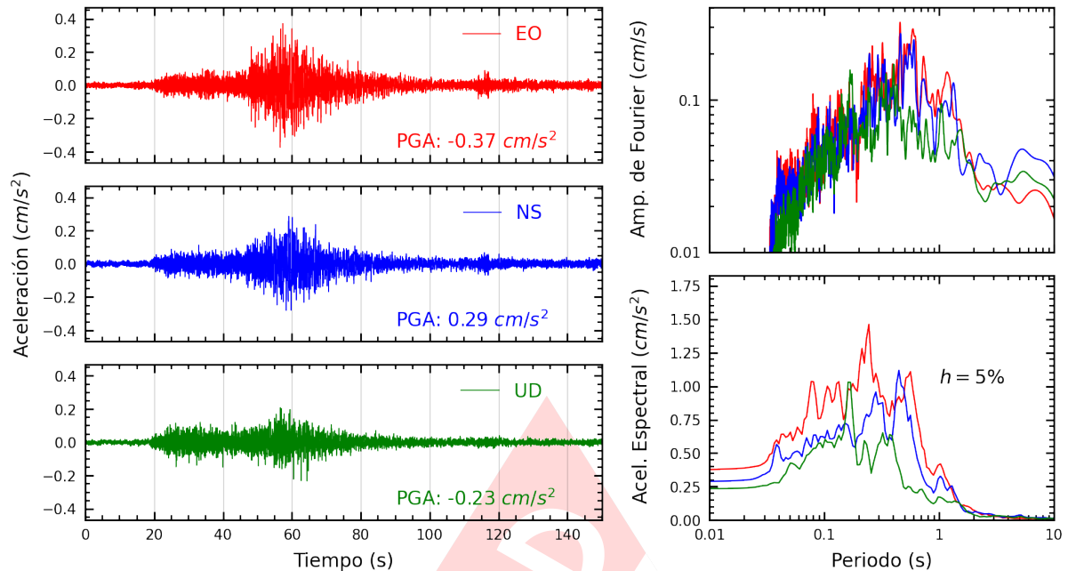
Figura A.25: Registros tiempo-historia, espectros de Fourier y de respuesta en las direcciones EO, NS y vertical de la estación CEPRE. Sismo de Pisco, Pisco - Ica del 2025-01-28, 00:09:28 (Hora local)
