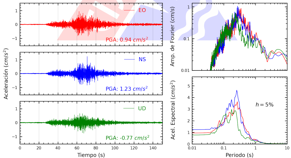
Figura A.4: Registros tiempo-historia, espectros de Fourier y de respuesta en las direcciones EO, NS y vertical de la estación SOVES. Sismo de Pisco, Pisco - Ica del 2025-01-28, 00:09:28 (Hora local)
