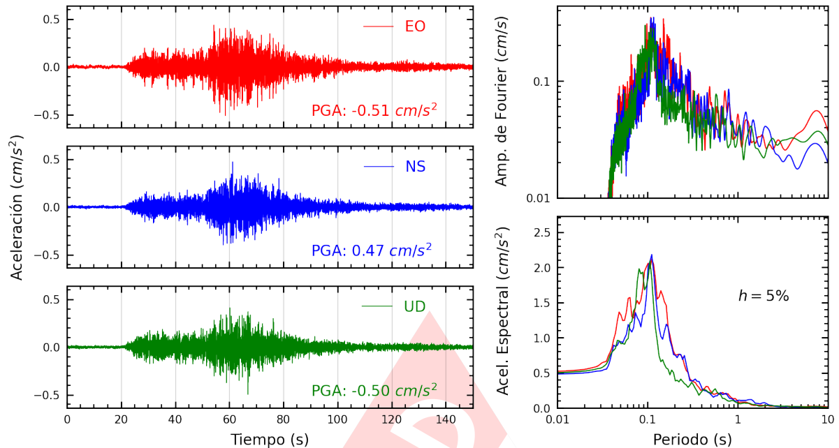
Figura A.17: Registros tiempo-historia, espectros de Fourier y de respuesta en las direcciones EO, NS y vertical de la estación AMORE. Sismo de Pisco, Pisco - Ica del 2025-01-28, 00:09:28 (Hora local)
