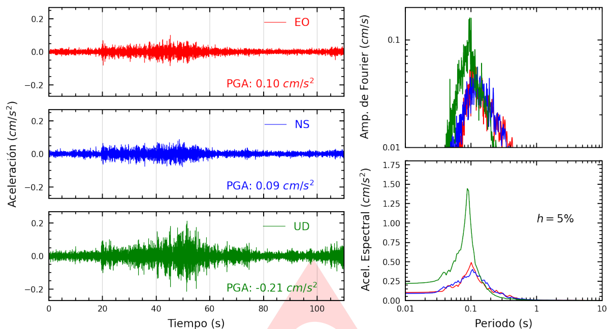
Figura A.1: Registros tiempo-historia, espectros de Fourier y de respuesta en las direcciones EO, NS y vertical de la estación UNP. Sismo de Zorritos, Contralmirante Villar - Tumbes del 2025-01-29, 05:48:52 (Hora local)
