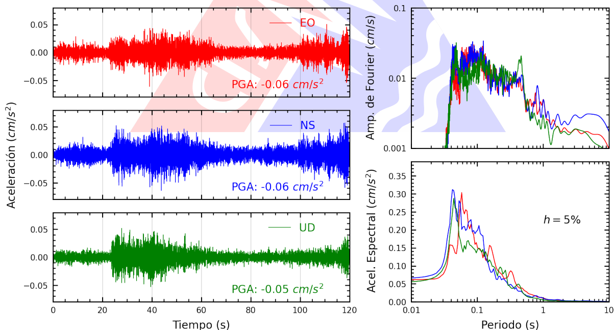
Figura A.2: Registros tiempo-historia, espectros de Fourier y de respuesta en las direcciones EO, NS y vertical de la estación UNF. Sismo de Zorritos, Contralmirante Villar - Tumbes del 2025-01-29, 05:48:52 (Hora local)
