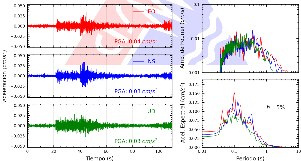
Figura A.2: Registros tiempo-historia, espectros de Fourier y de respuesta en las direcciones EO, NS y vertical de la estación UNCP. Sismo de Oxapampa, Oxapampa - Pasco del 2025-01-31, 14:09:44 (Hora local)
