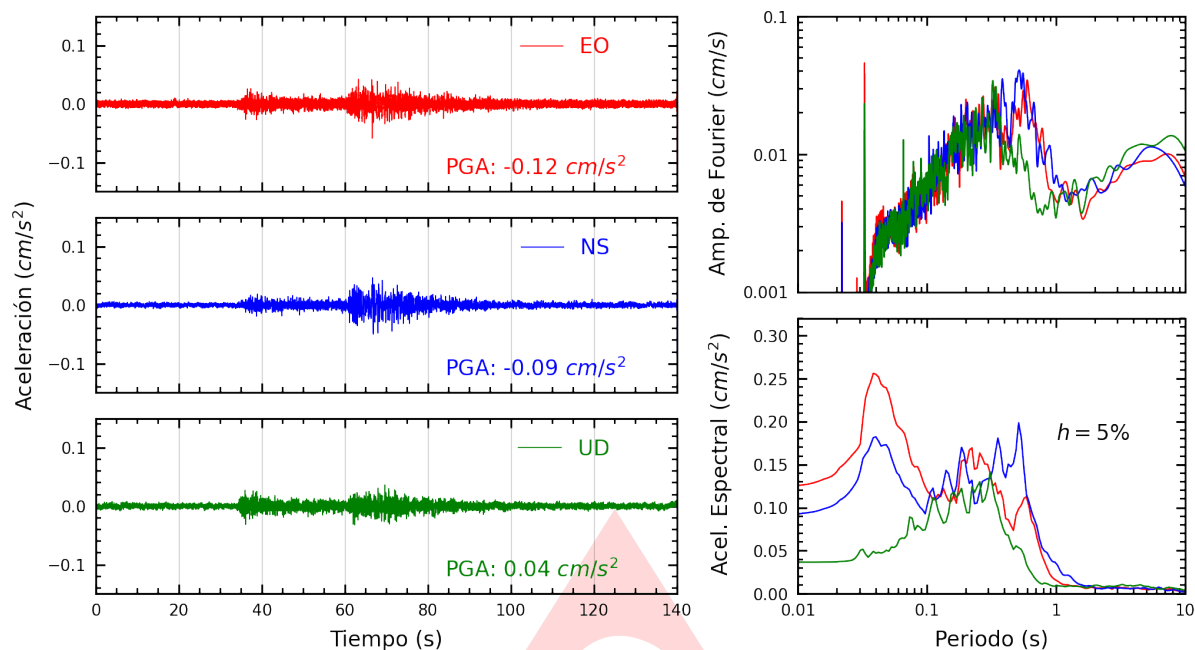
Figura A.1: Registros tiempo-historia, espectros de Fourier y de respuesta en las direcciones EO, NS y vertical de la estación CARAL. Sismo de Oxapampa, Oxapampa - Pasco del 2025-01-31, 14:09:44 (Hora local)
